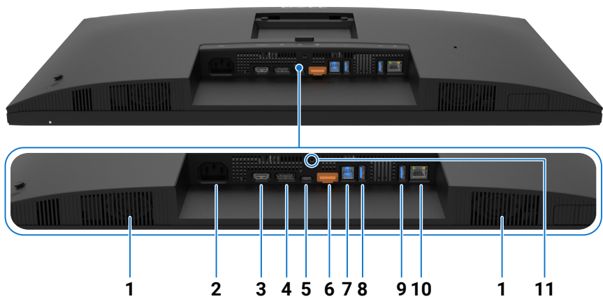
Figure 3. Vue de dessous du moniteur
