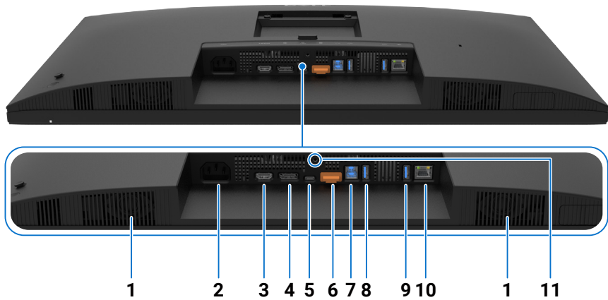
Figure 3. Vue de dessous du moniteur
