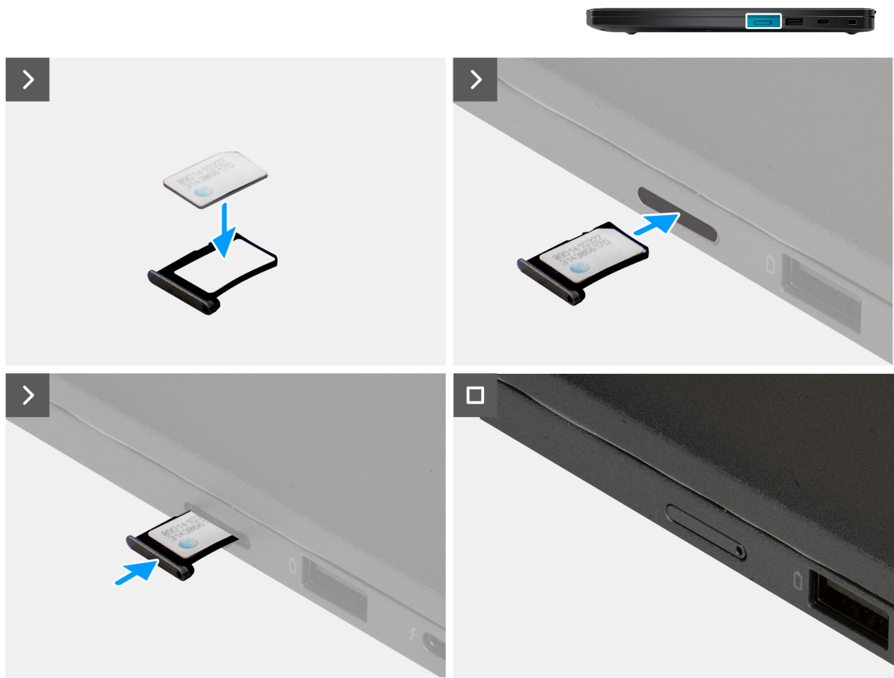
Abbildung 15. Installieren des Nano-SIM-Kartenfachs
