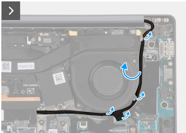
Abbildung 30. Entfernen des linken Lüfters
