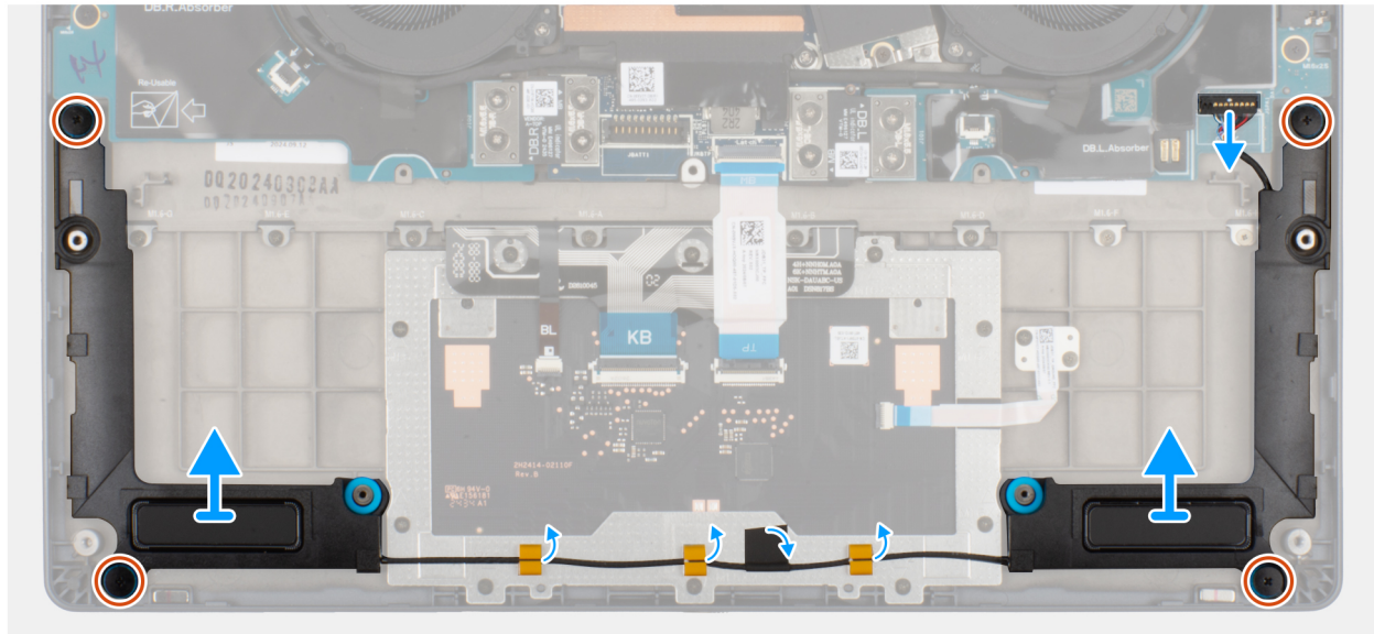
Abbildung 34. Entfernen der Lautsprecher ohne Antenne (WLAN-Konfiguration)
