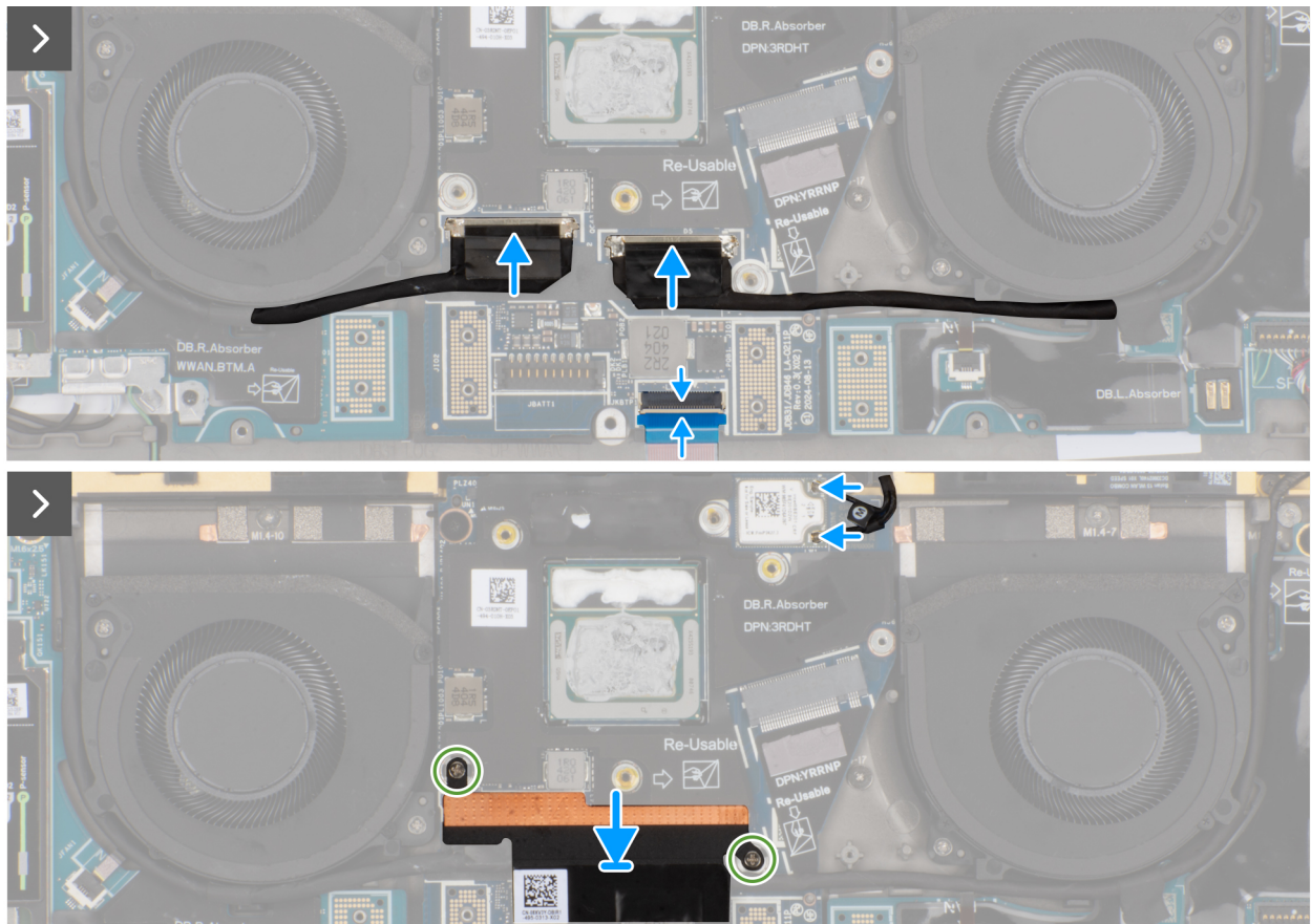
Abbildung 70. Einbauen der Systemplatine
