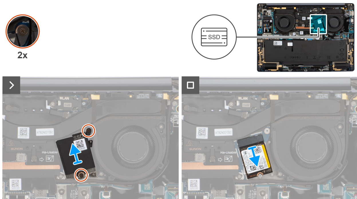
Abbildung 26. Entfernen des SSD
