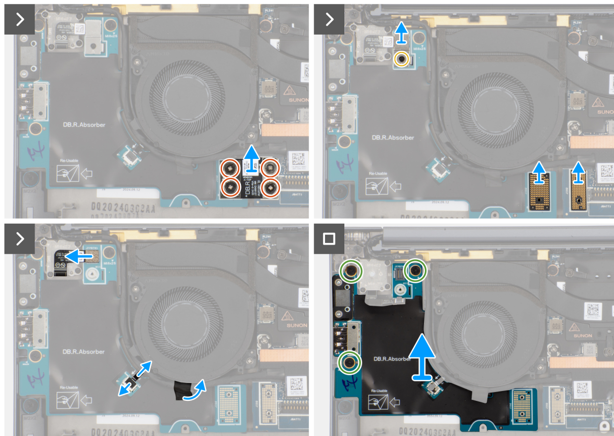
Abbildung 44. Entfernen der rechten I/O-Platine (ohne WWAN-Antennen)
