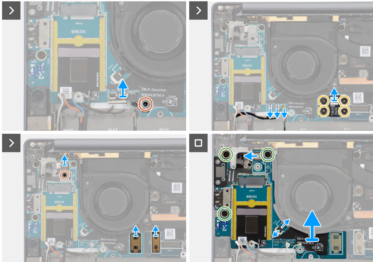
Abbildung 48. Entfernen der rechten I/O-Platine (mit WWAN)
