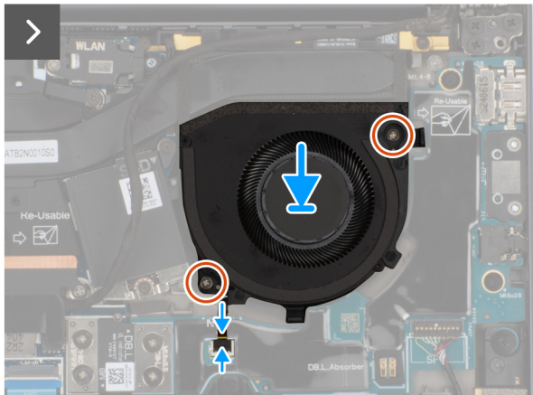
Abbildung 31. Installieren des linken Lüfters
