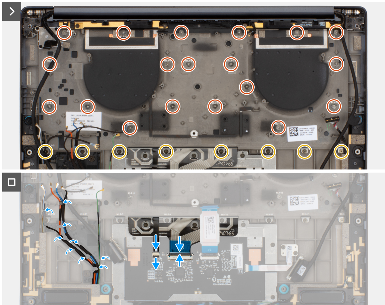
Abbildung 76. Installieren der Tastaturbaugruppe
