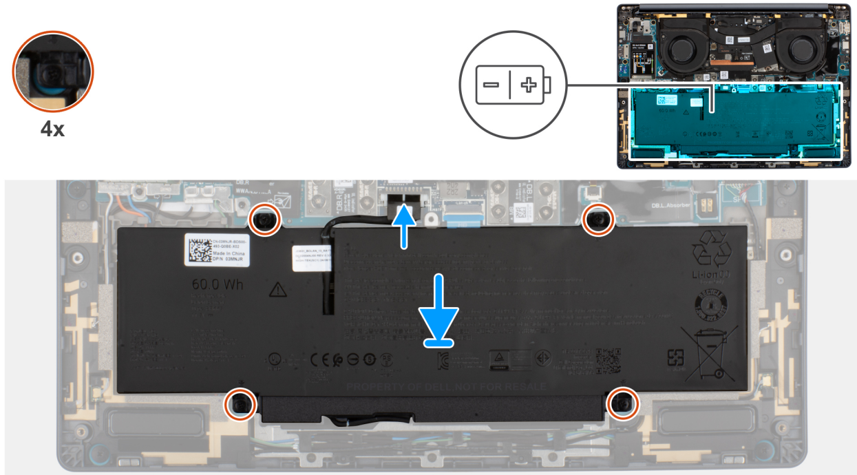
Abbildung 23. Einsetzen des Akkus
