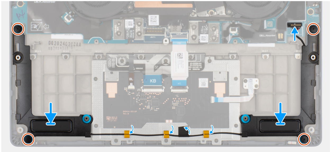
Abbildung 35. Installieren der Lautsprecher (ohne WWAN)
