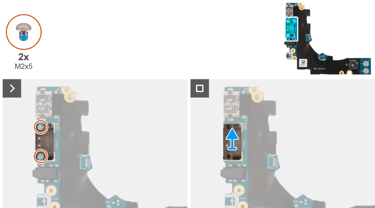
Abbildung 54. Entfernen des rechten USB-Typ-C-Moduls
