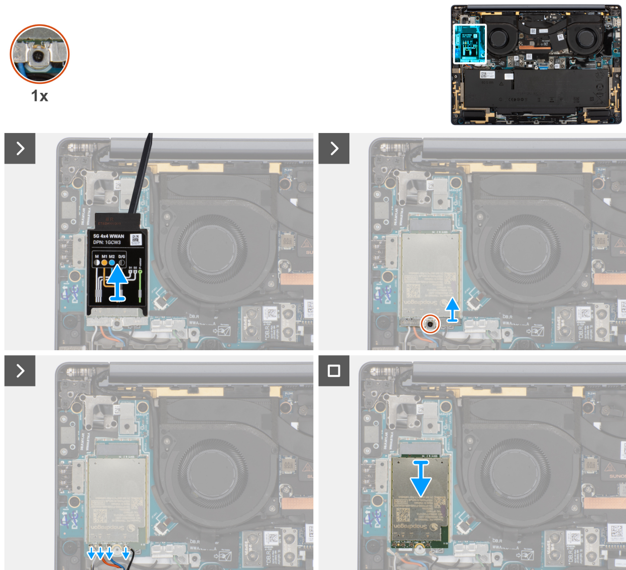
Abbildung 28. Entfernen der WWAN-Karte
