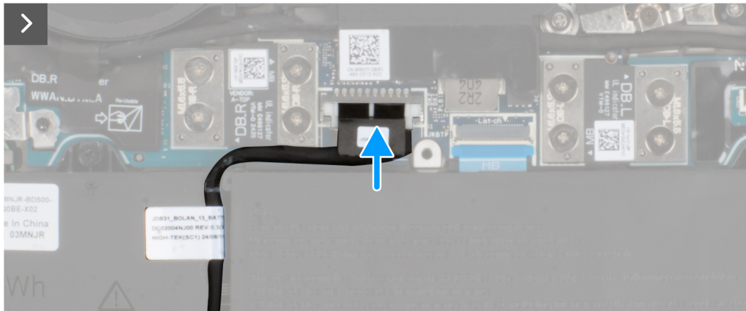
Abbildung 19. Verbinden des Batteriekabels mit der Hauptplatine
