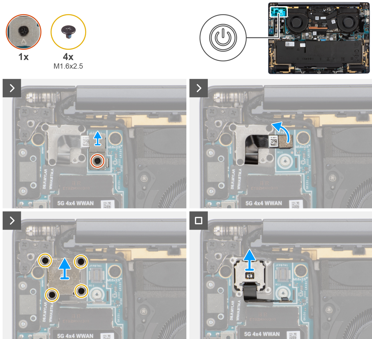
Abbildung 56. Entfernen des Netzschalters
