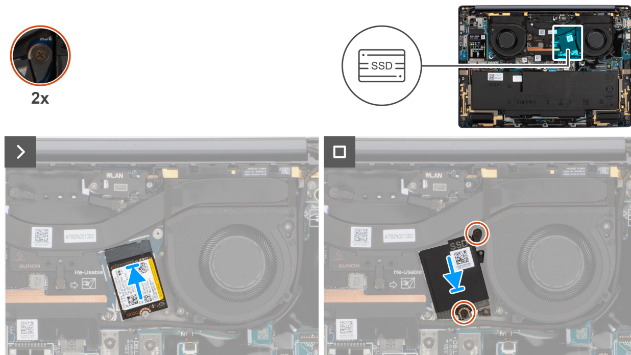
Abbildung 27. Einbauen der SSD-Karte
