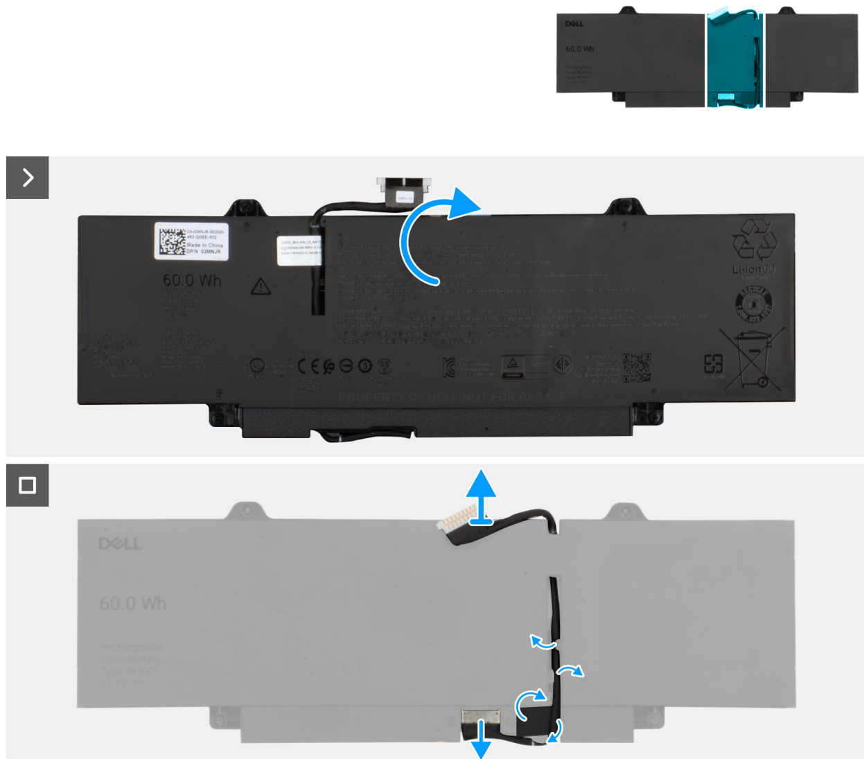
Abbildung 24. Entfernen und Trennen des Akkukabels
