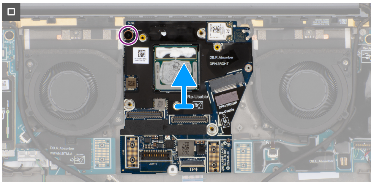
Abbildung 66. Entfernen der Systemplatine
