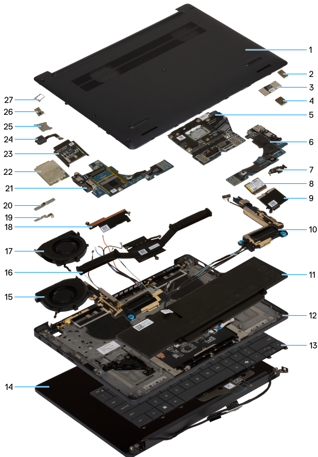
Abbildung 11. Hauptkomponenten Ihres Systems/Explosionsansicht
