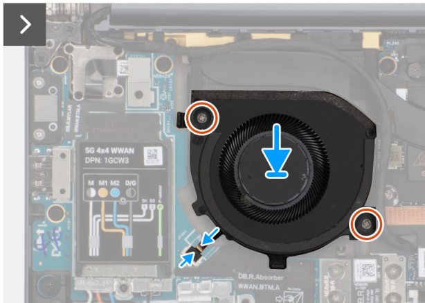
Abbildung 33. Installieren des rechten Lüfters
