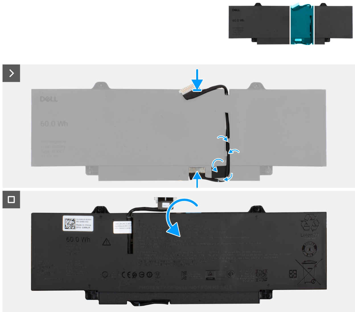
Abbildung 25. Anschließen und Installieren des Akkukabels
