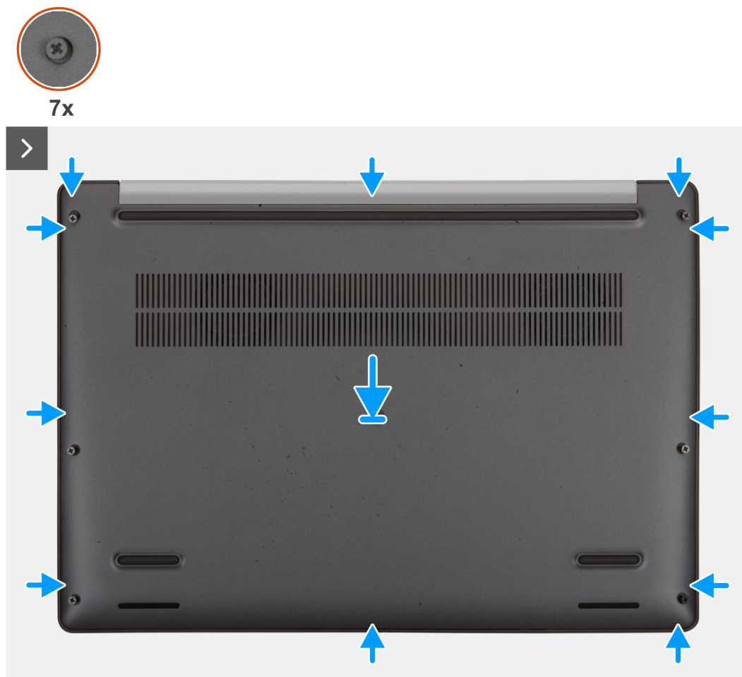
Abbildung 20. der Bodenabdeckung
