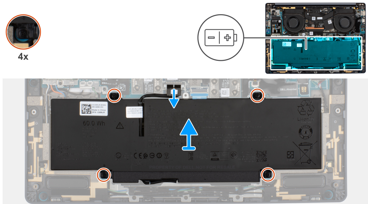
Abbildung 22. Lösen der unverlierbaren Schrauben
