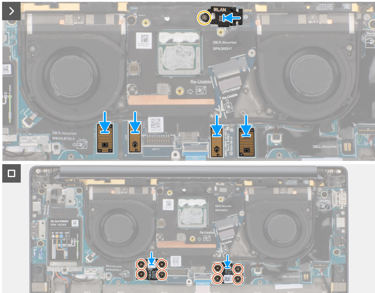
Abbildung 71. Einbauen der Systemplatine
