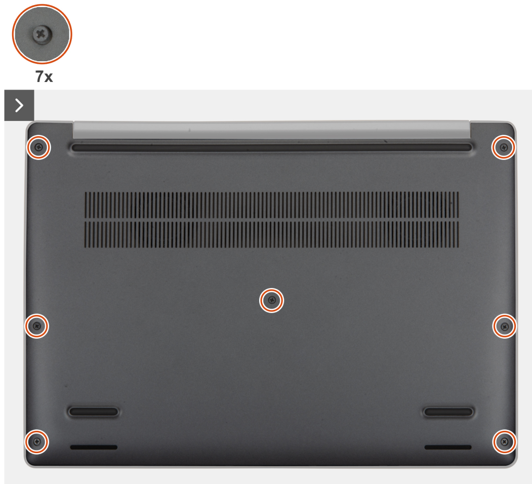
Abbildung 16. Lösen der unverlierbaren Schrauben
