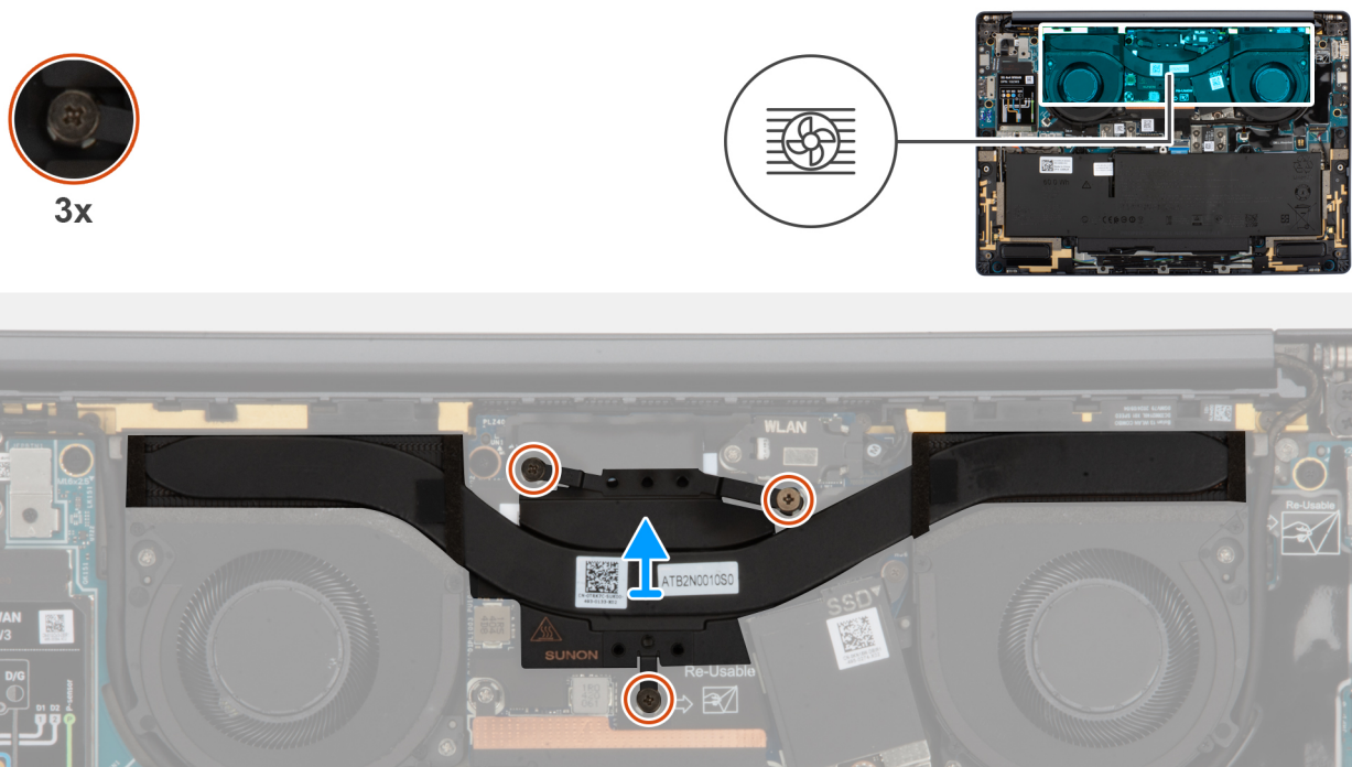
Abbildung 38. Kühlkörper entfernen
