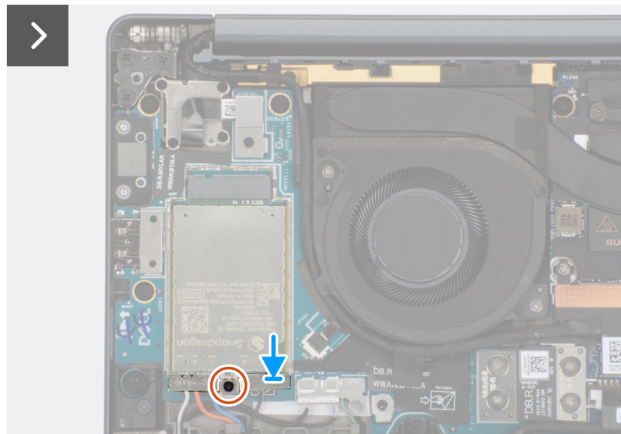
Abbildung 29. Einbauen der WWAN-Karte
