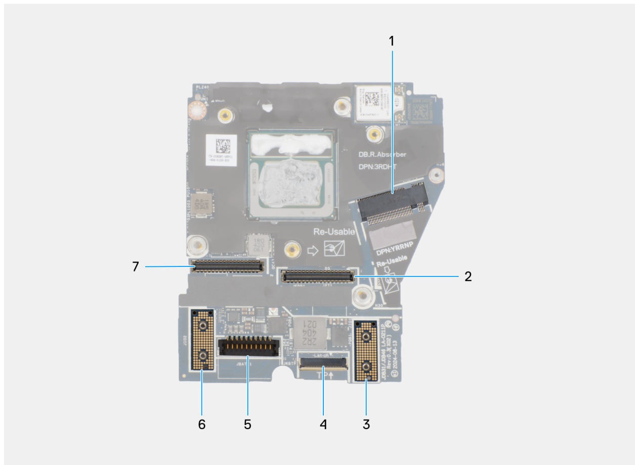
Abbildung 63. Komponenten auf der Hauptplatine
