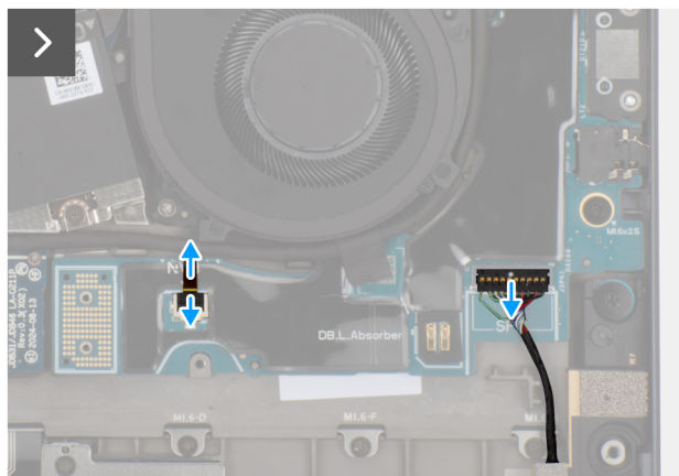
Abbildung 40. Entfernen der linken E/A-Platine
