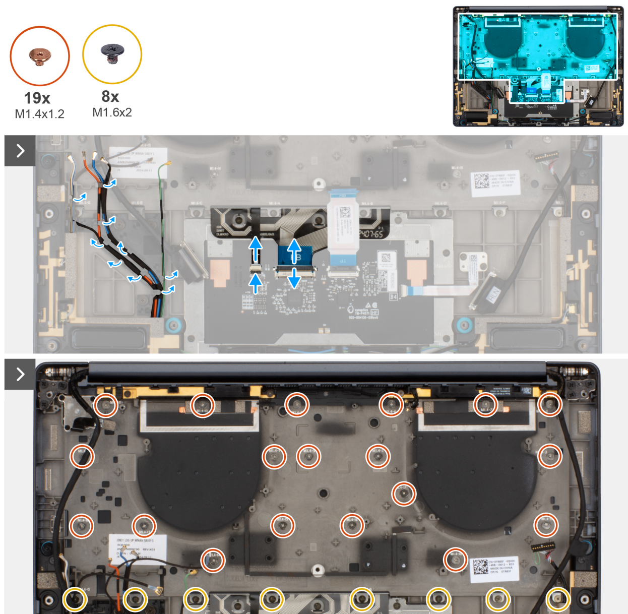
Abbildung 73. Entfernen der Tastaturbaugruppe
