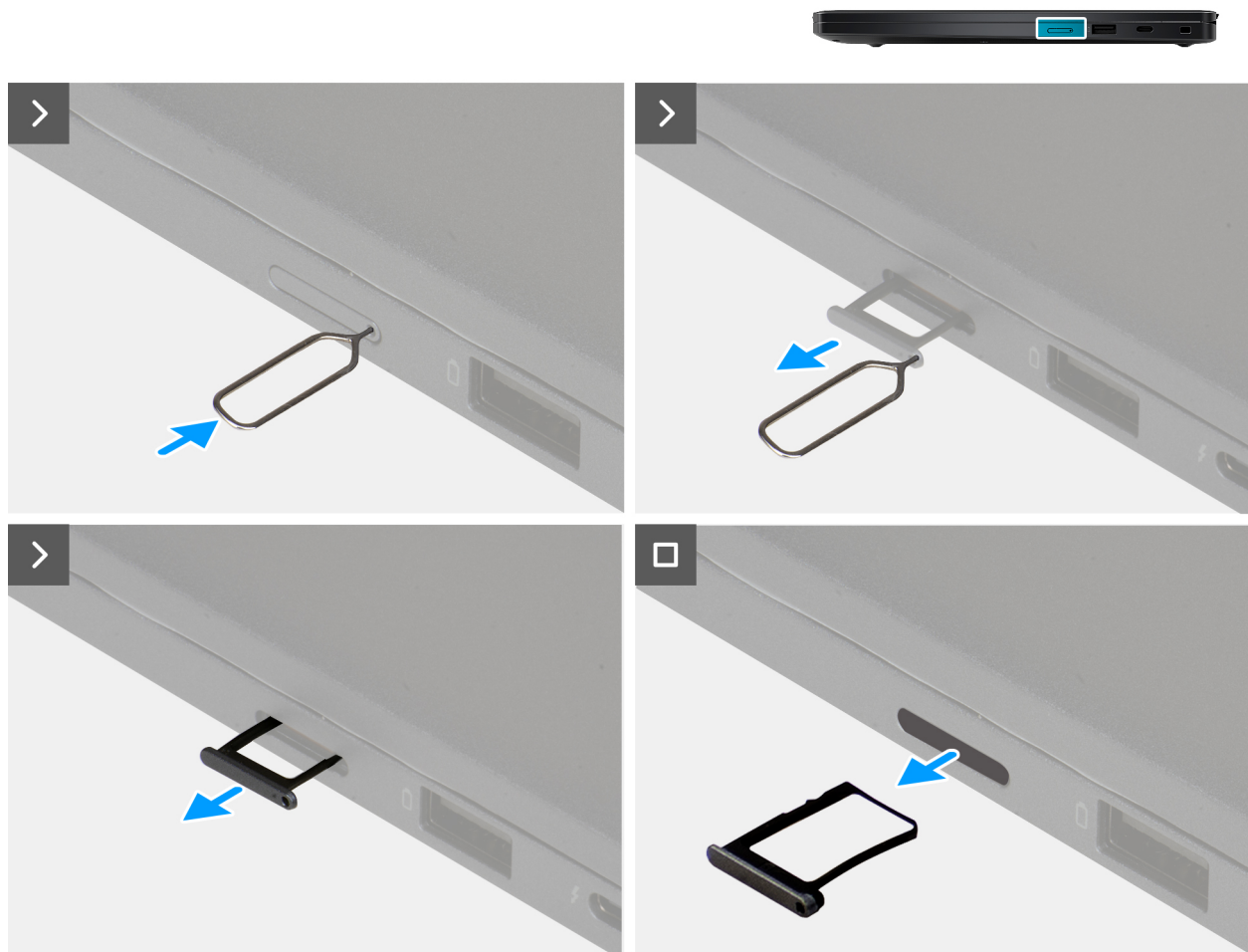
Abbildung 12. Entfernen des Nano-SIM-Kartenfachs
