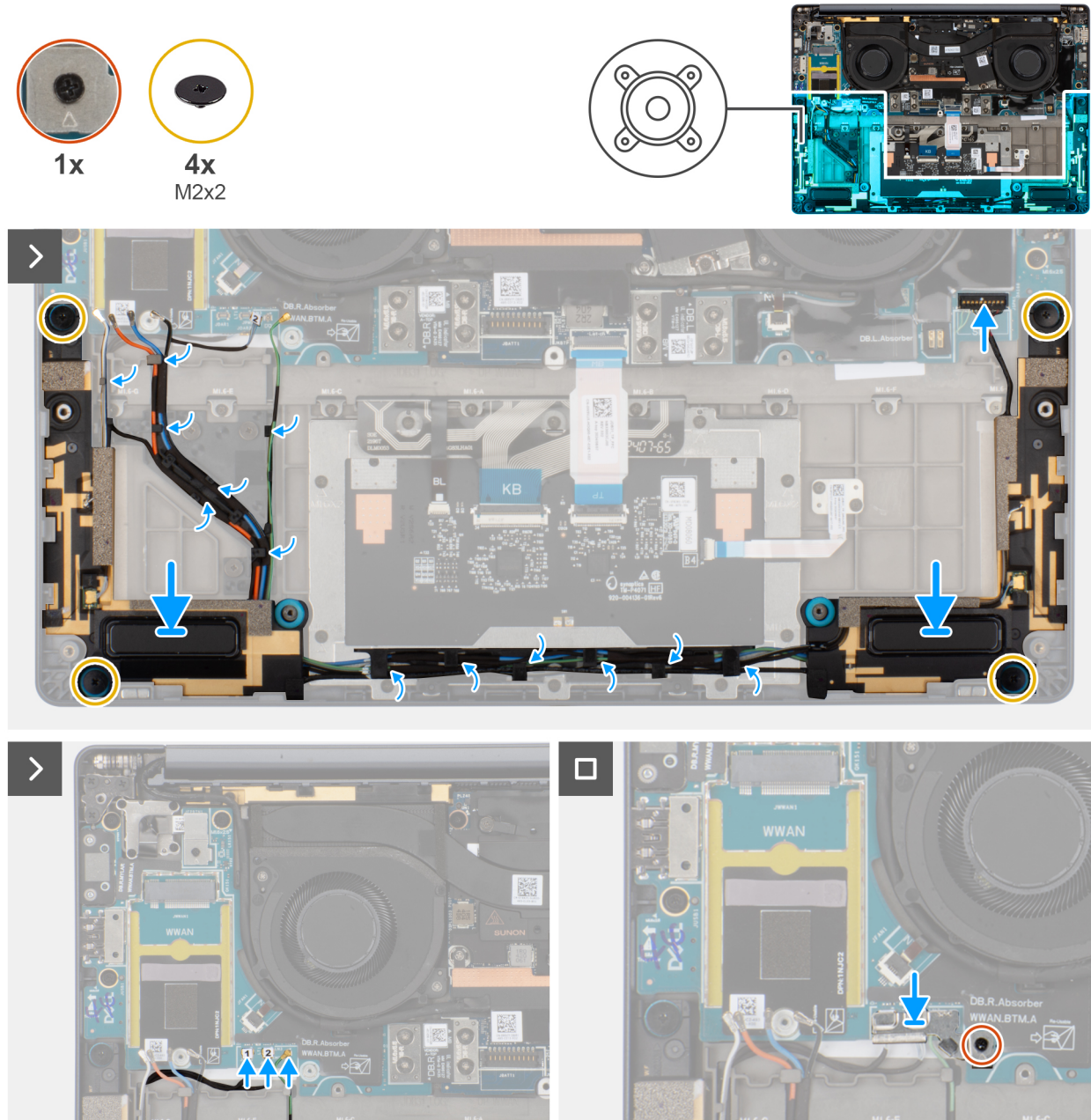
Abbildung 37. Installieren der Lautsprecher mit Antennen (WWAN-Konfiguration)
