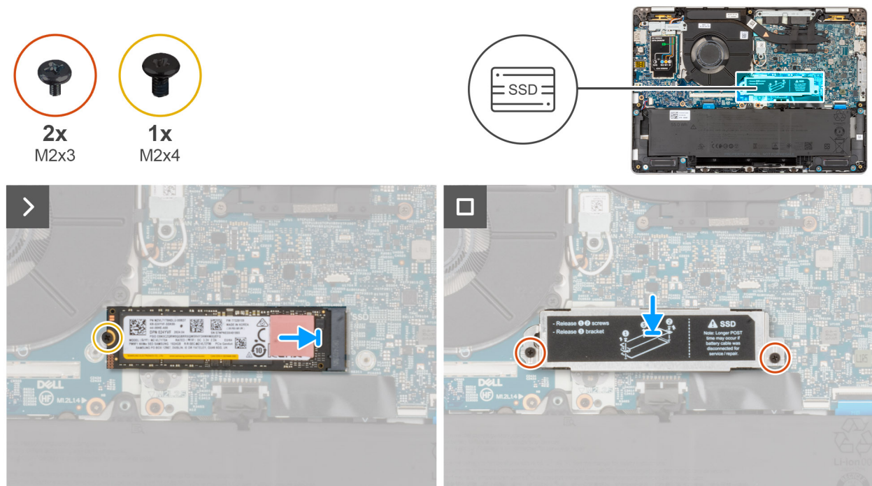
Abbildung 28. Installieren der M.2-2280-SSD
