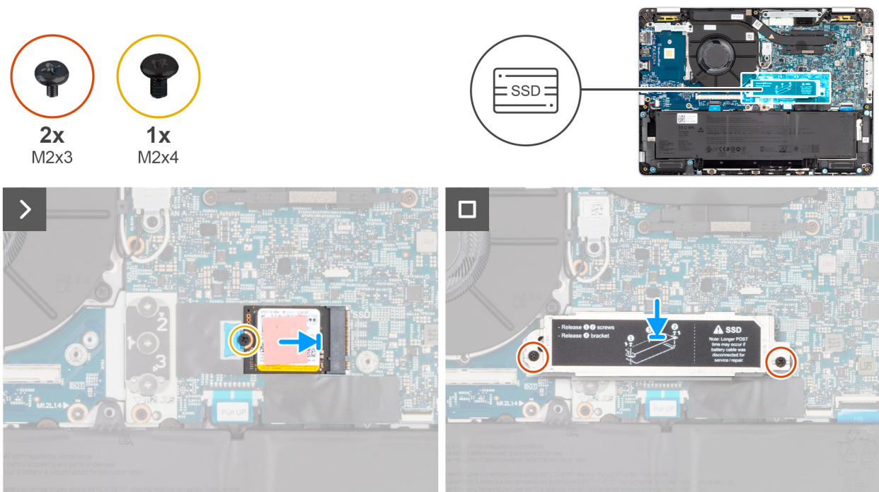
Abbildung 26. Einbauen des M.2-2280-SSD
