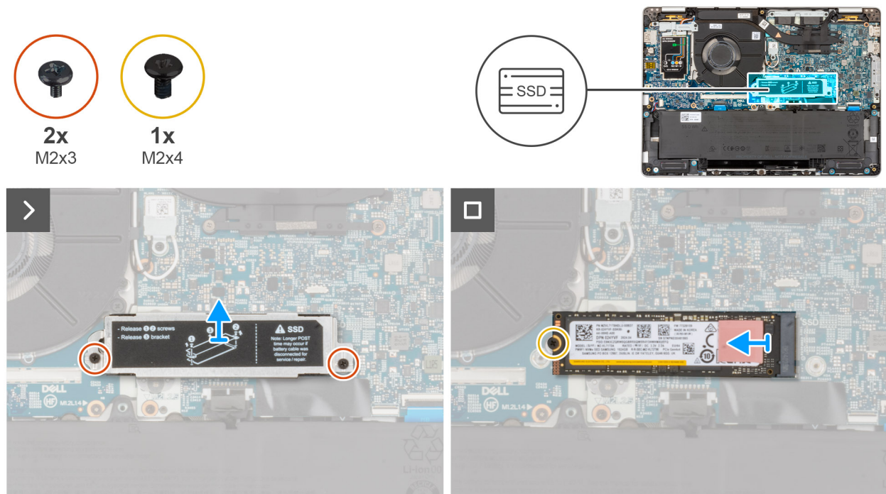
Abbildung 27. Entfernen der M.2-2280-SSD
