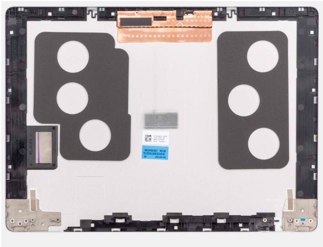
Abbildung 74. Einbauen der hinteren Bildschirmabdeckung
