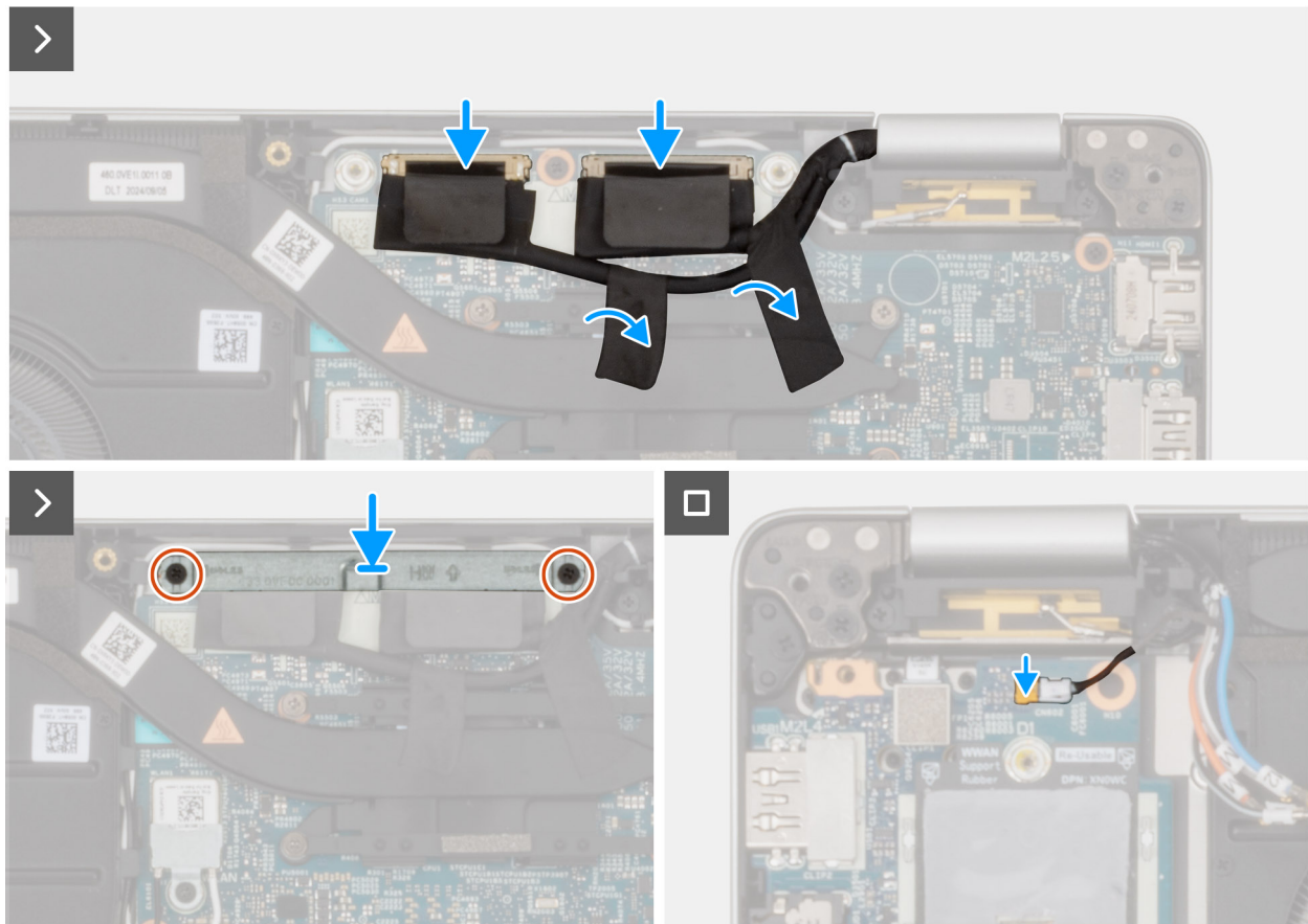
Abbildung 42. Einbauen der Bildschirmbaugruppe
