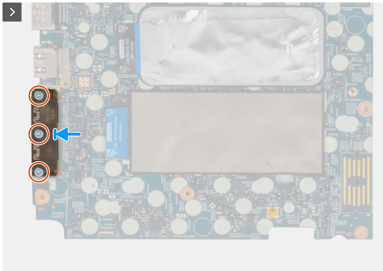
Abbildung 49. Installieren des USB-Typ-C-Anschlussmoduls
