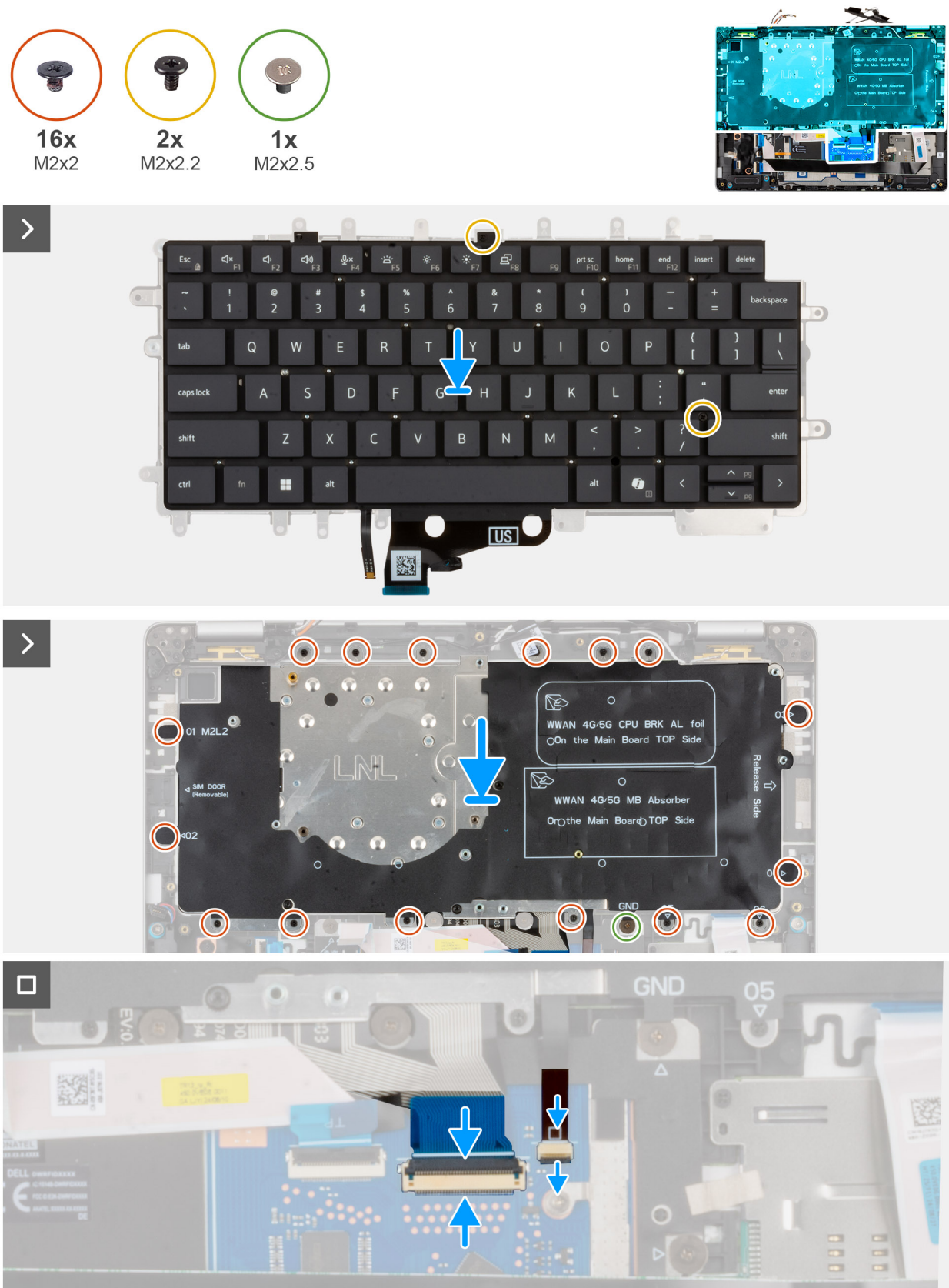
Abbildung 60. Einbauen der Tastatur
