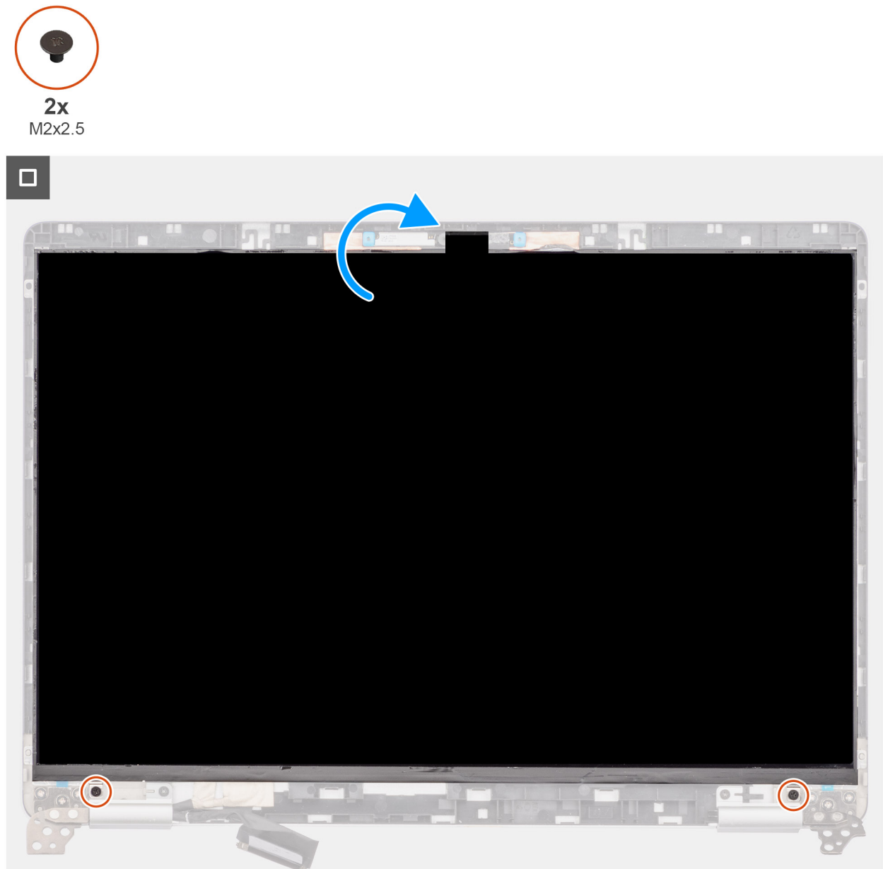
Abbildung 67. Einbauen des Bildschirms
