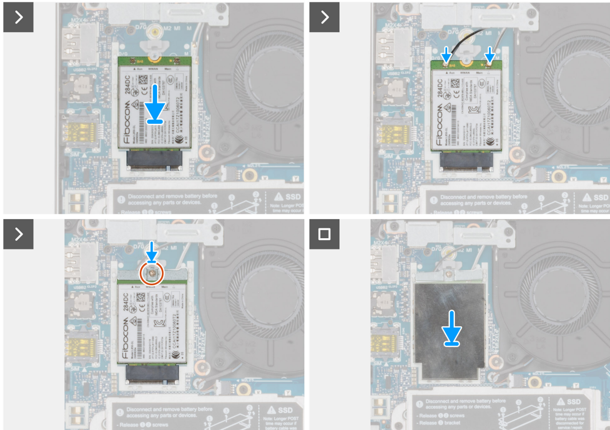
Abbildung 32. Installieren der 5G-WWAN-Karte
