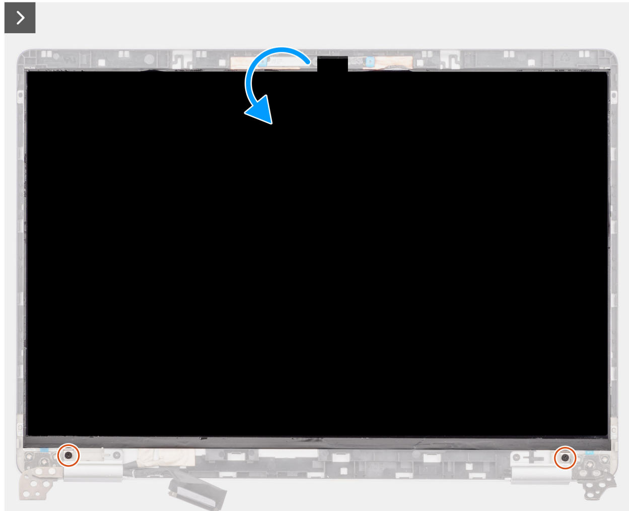
Abbildung 77. Entfernen des Bildschirms
