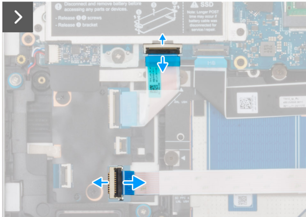
Abbildung 45. Entfernen der USH-Platine
