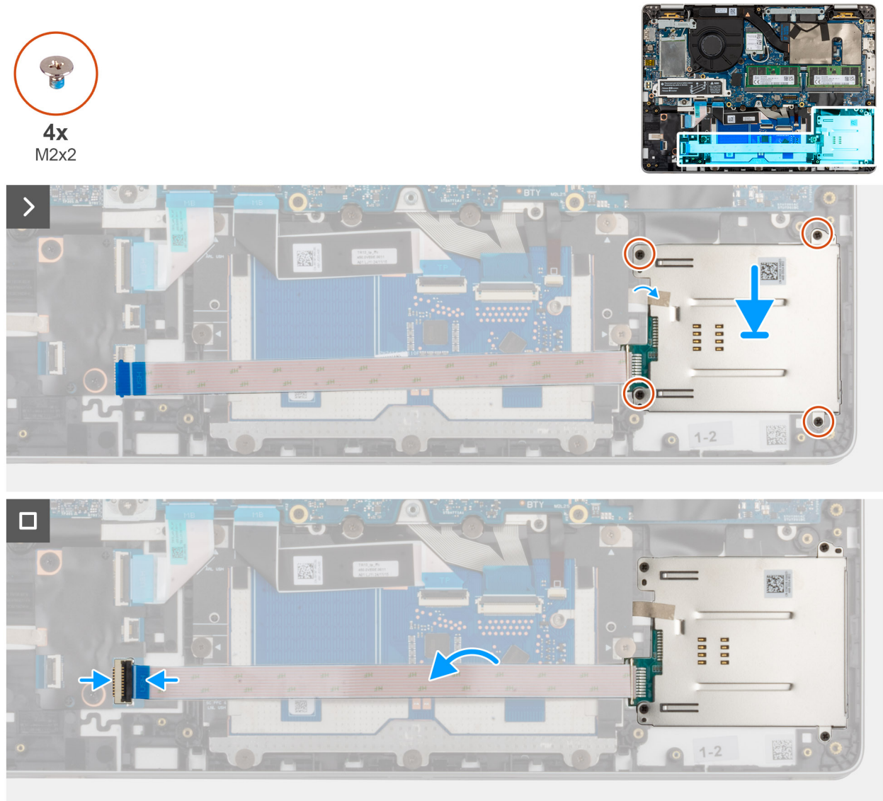
Abbildung 49. Einbauen des Smartcardlesegeräts
