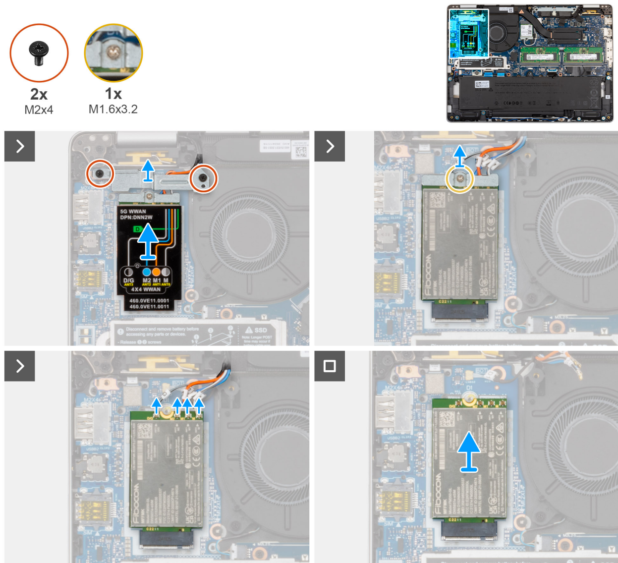
Abbildung 29. Entfernen der 5G-WWAN-Karte
