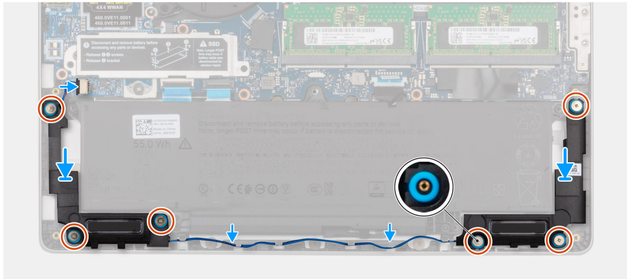
Abbildung 42. Installieren der Lautsprecher
