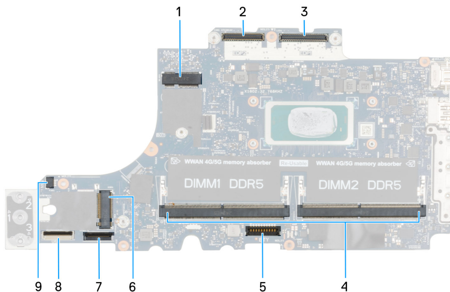
Abbildung 56. Anschlüsse auf der Hauptplatine
