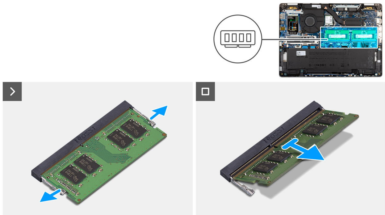
Abbildung 27. Entfernen des Arbeitsspeichersmoduls
