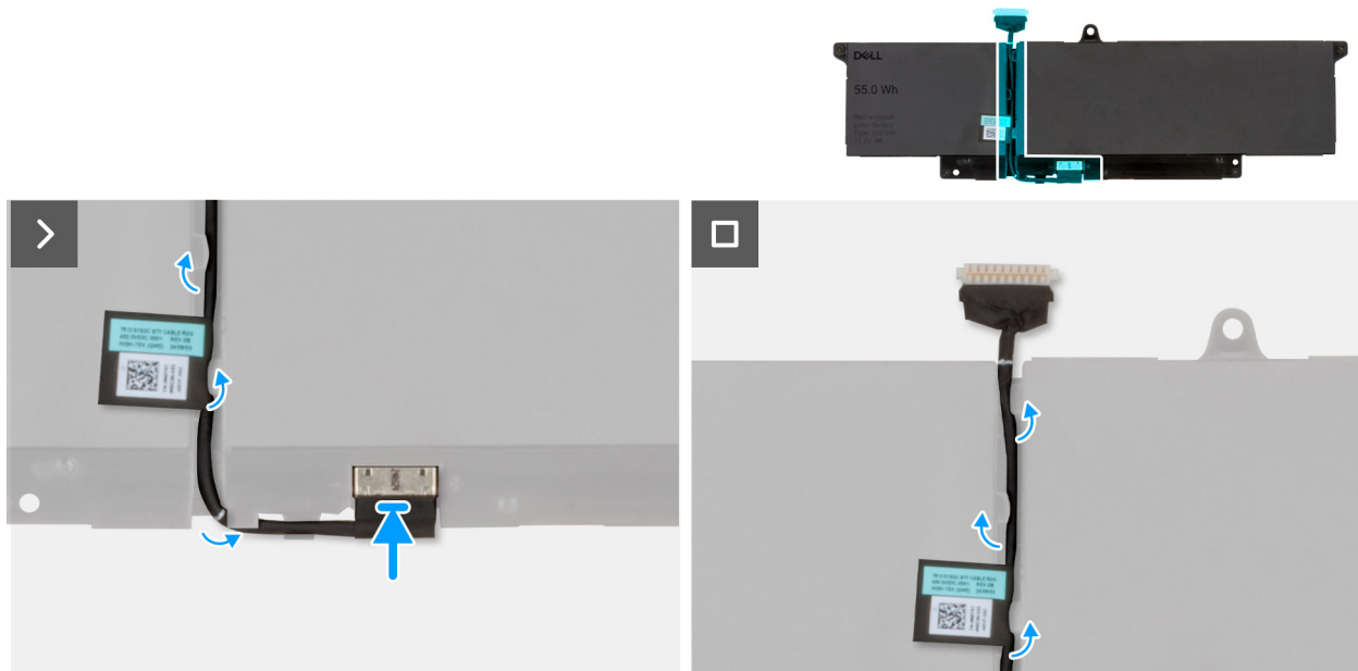
Abbildung 26. Einsetzen des Akkukabels
