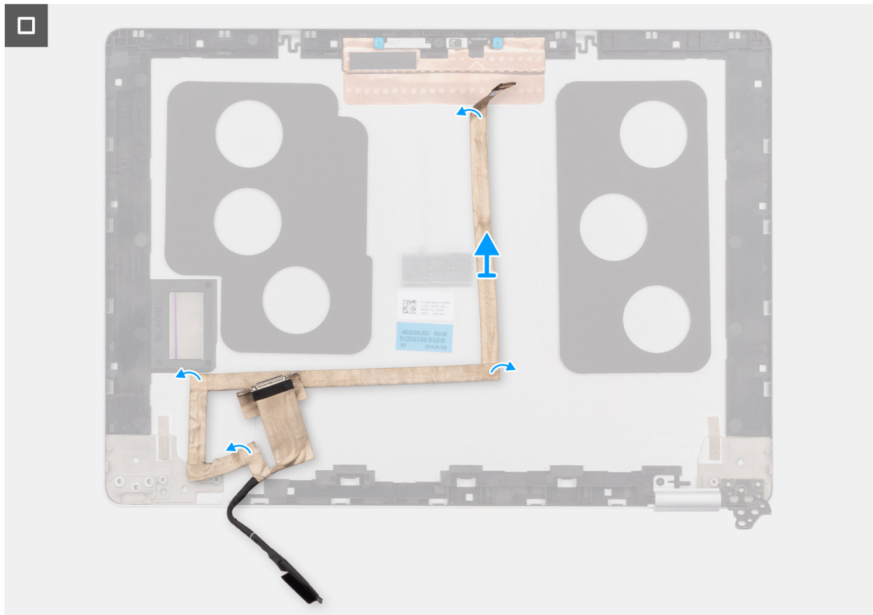
Abbildung 83. Entfernen des Bildschirmkabels
