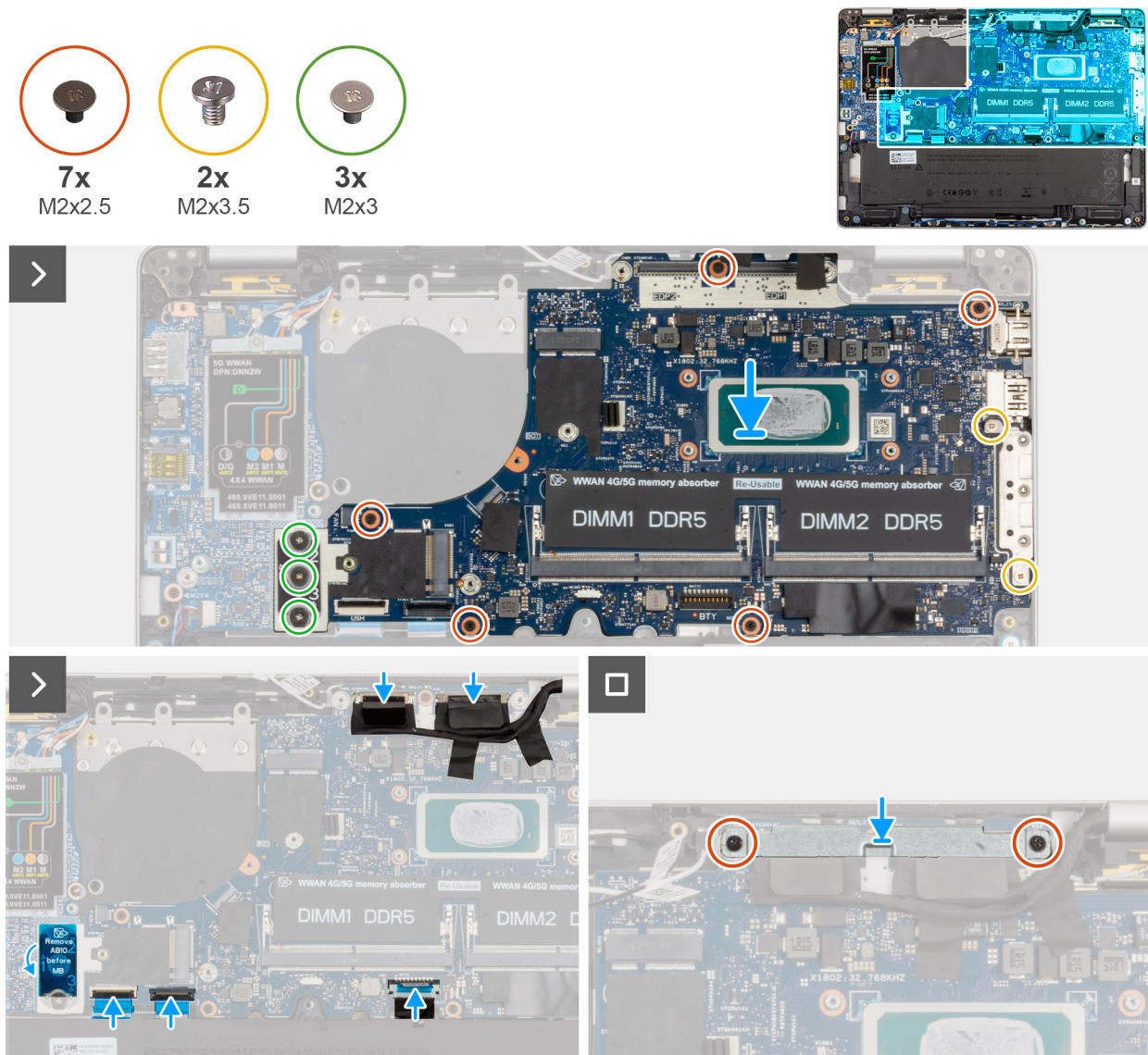
Abbildung 59. Einbau der Systemplatine
