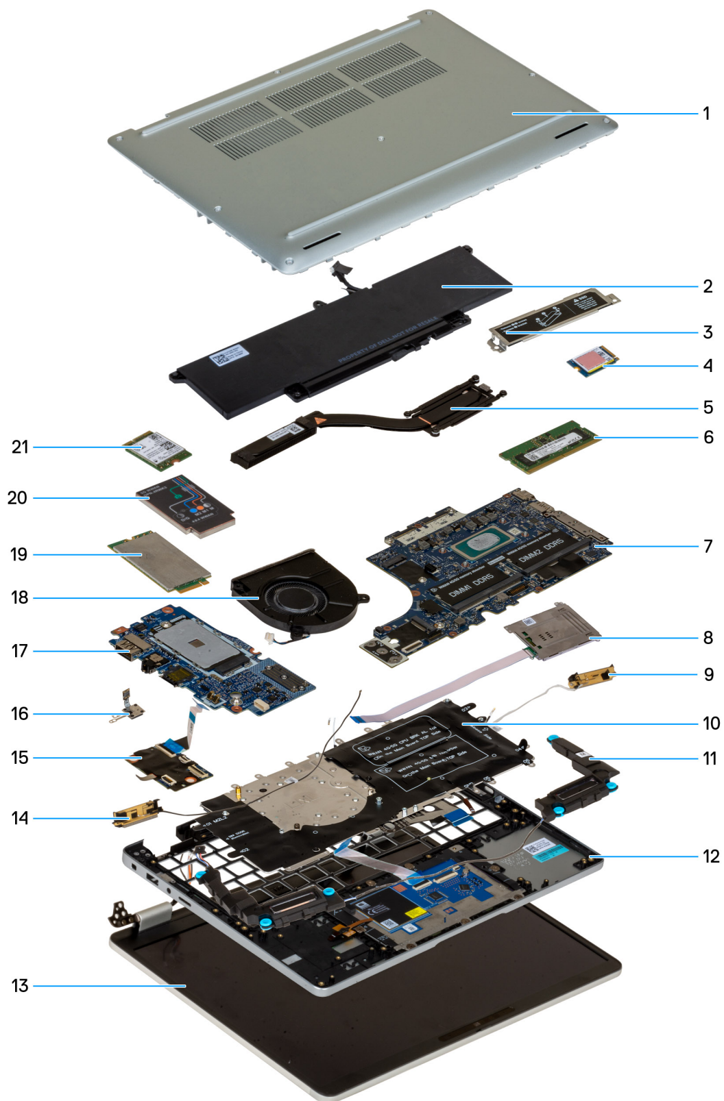
Abbildung 14. Hauptkomponenten Ihres Dell Pro 13 Plus
