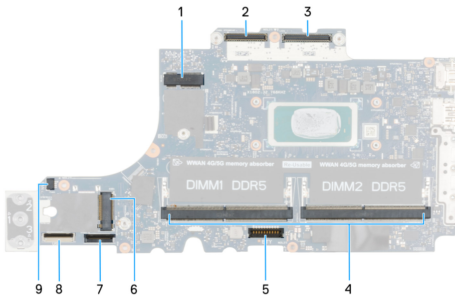
Abbildung 58. Anschlüsse auf der Hauptplatine
