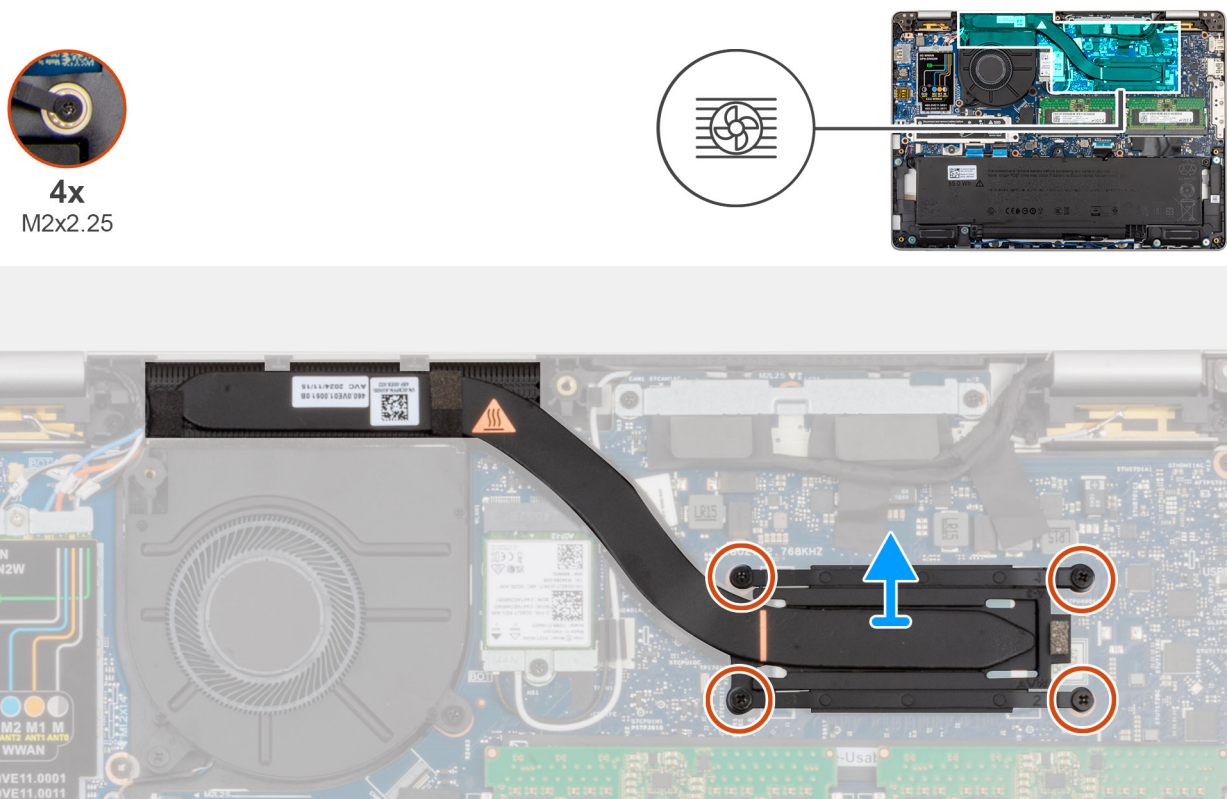
Abbildung 50. Kühlkörper entfernen
