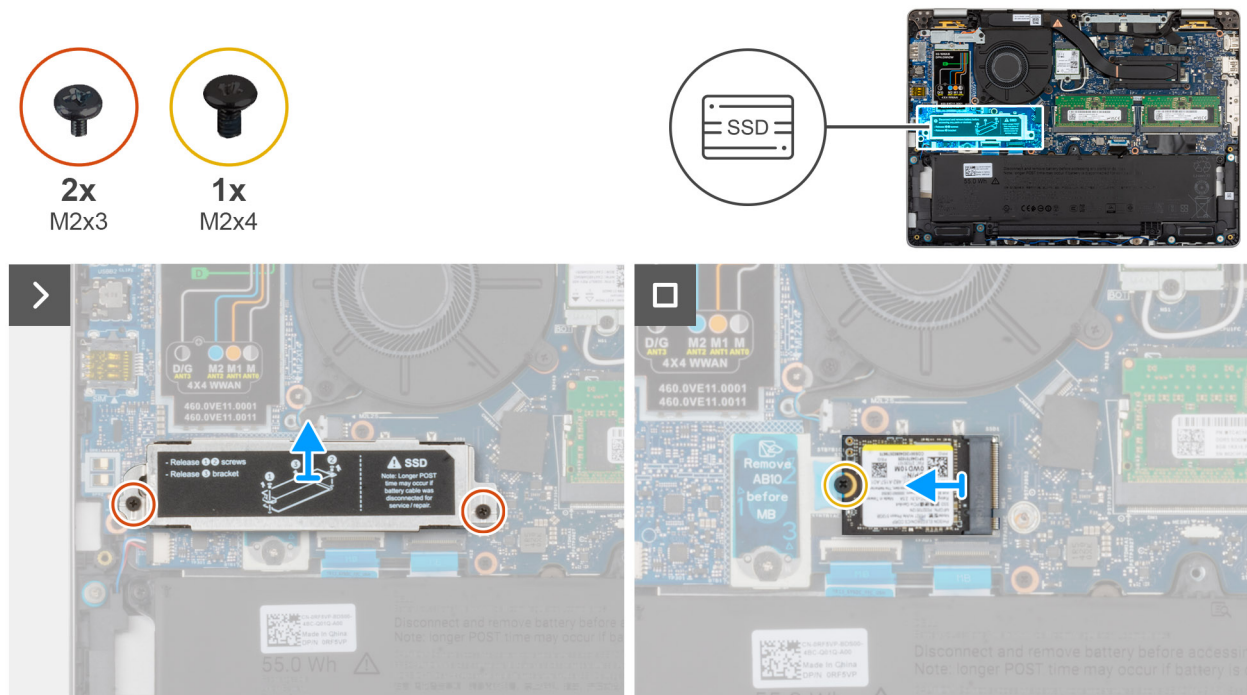
Abbildung 37. Entfernen des M.2-2230-Solid-State-Laufwerks
