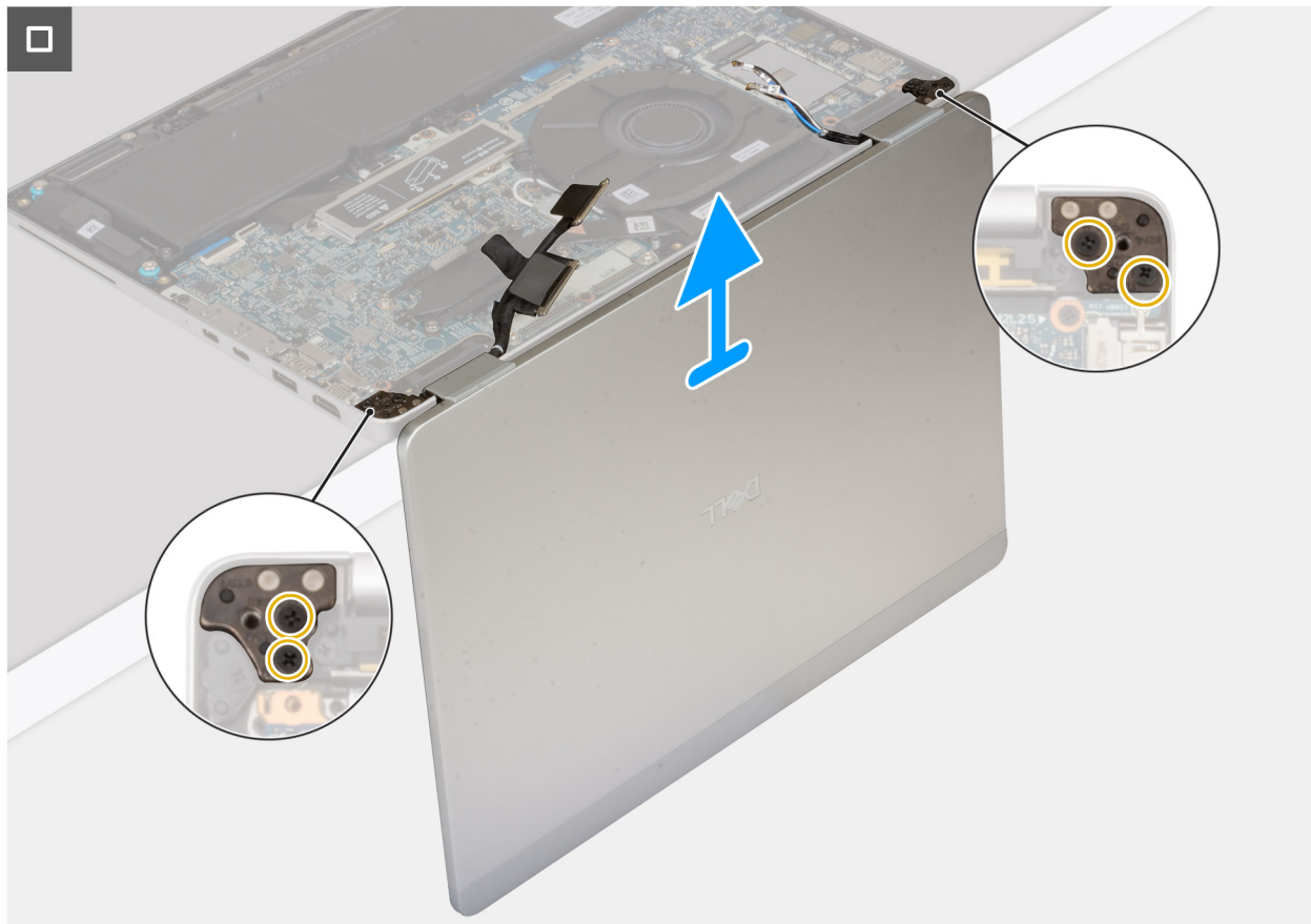
Abbildung 53. Entfernen der Bildschirmbaugruppe
