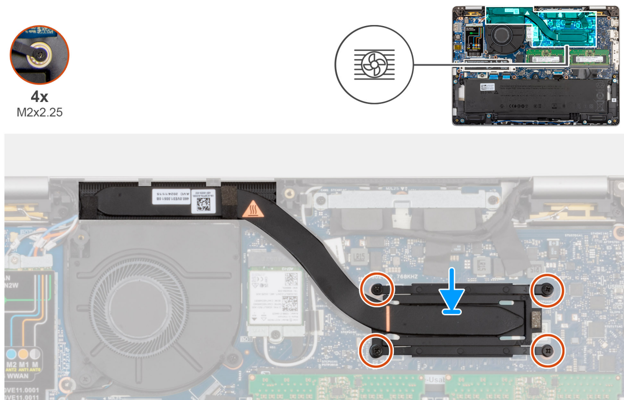
Abbildung 51. Einsetzen des Kühlkörpers
