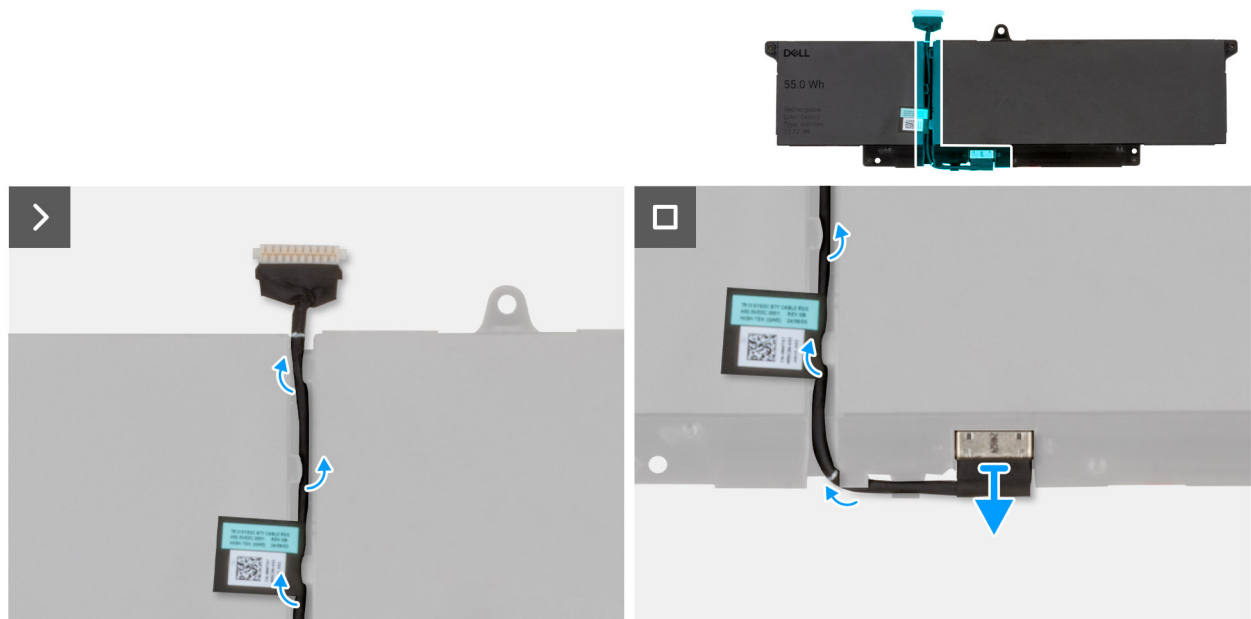
Abbildung 25. Entfernen des Akkukabels
