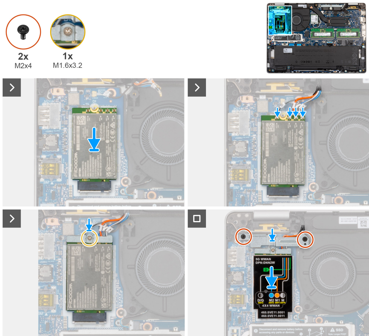
Abbildung 31. Installieren der 5G-WWAN-Karte
