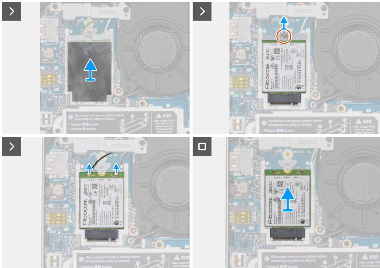
Abbildung 33. Entfernen der 4G-WWAN-Karte
