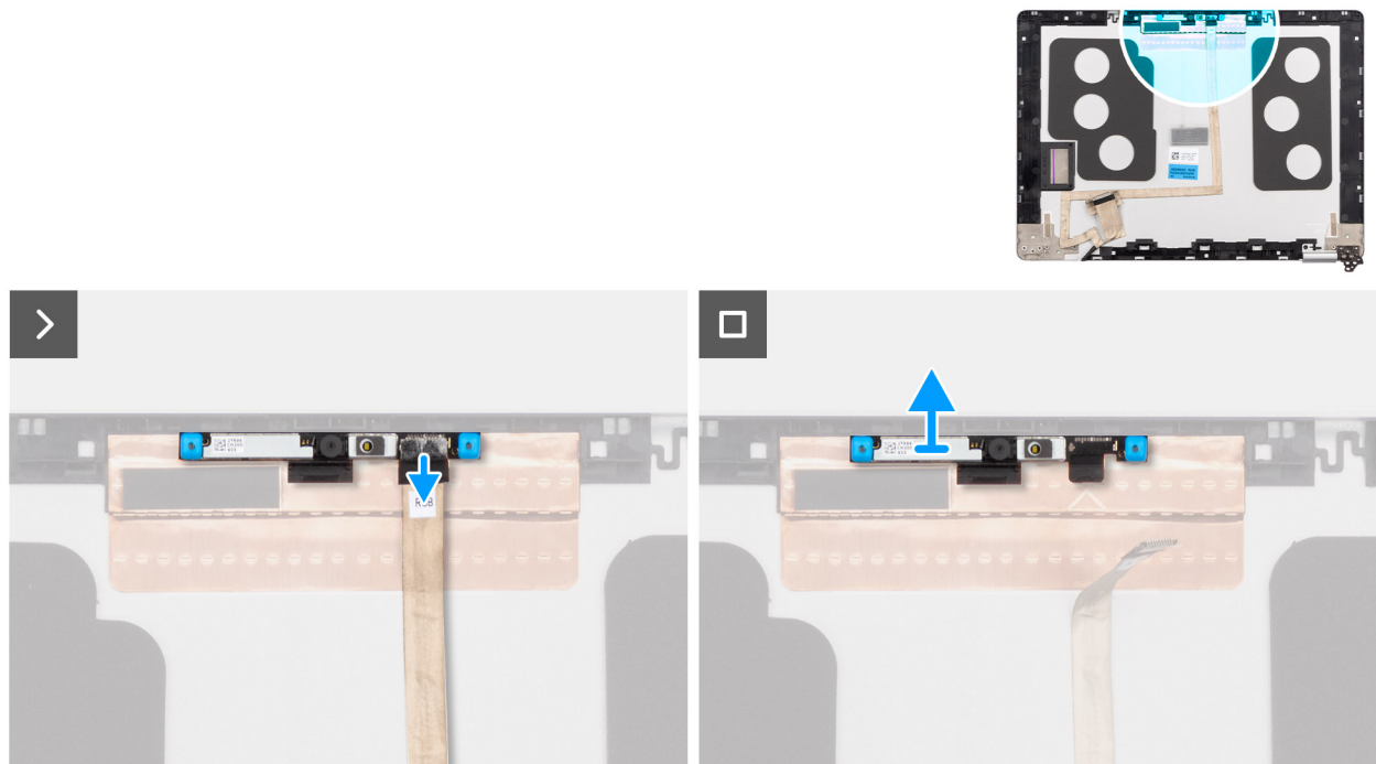
Abbildung 80. Entfernen des Kameramoduls
