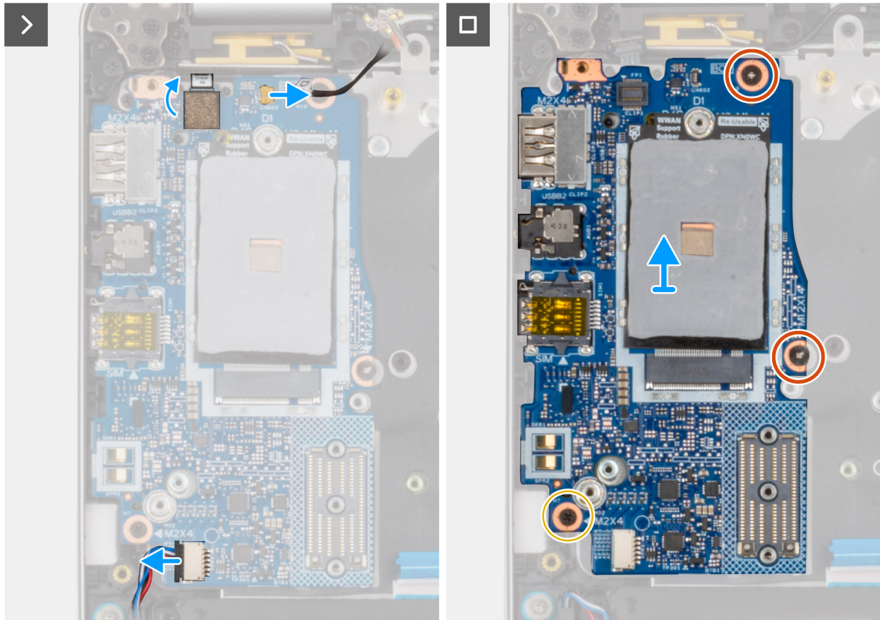
Abbildung 64. Abbildung: Entfernen der I/O-Platine
