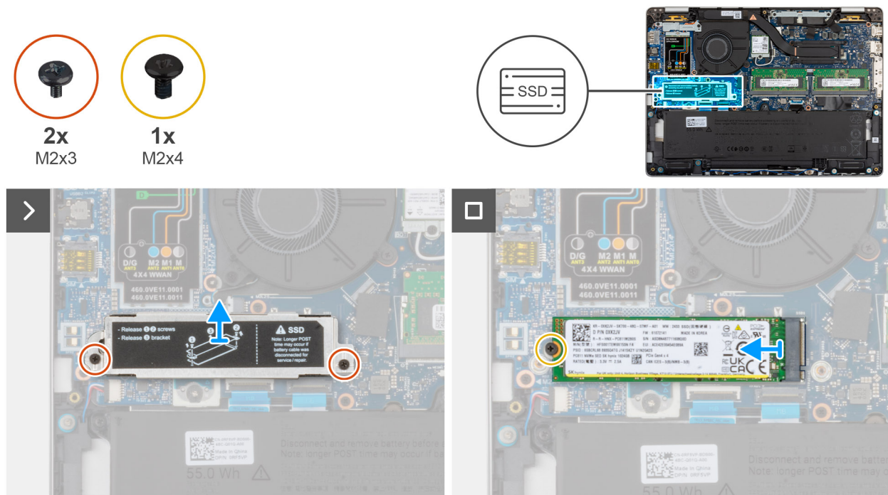
Abbildung 39. Entfernen der M.2-2280-SSD
