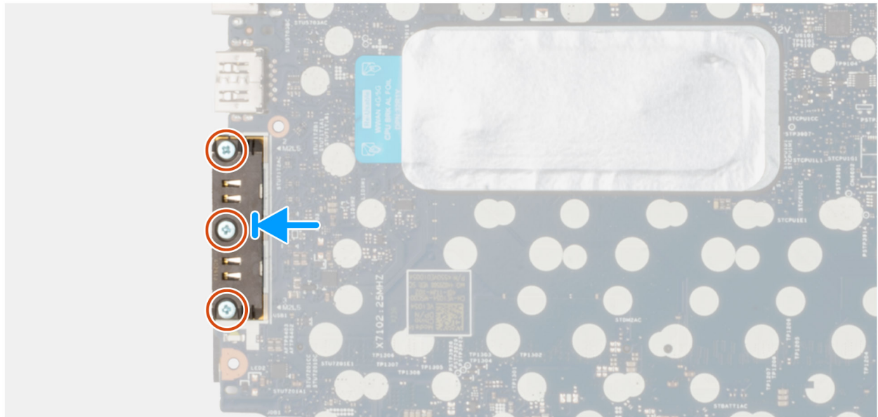
Abbildung 61. Installieren des USB-Type-C-Anschlussmoduls
