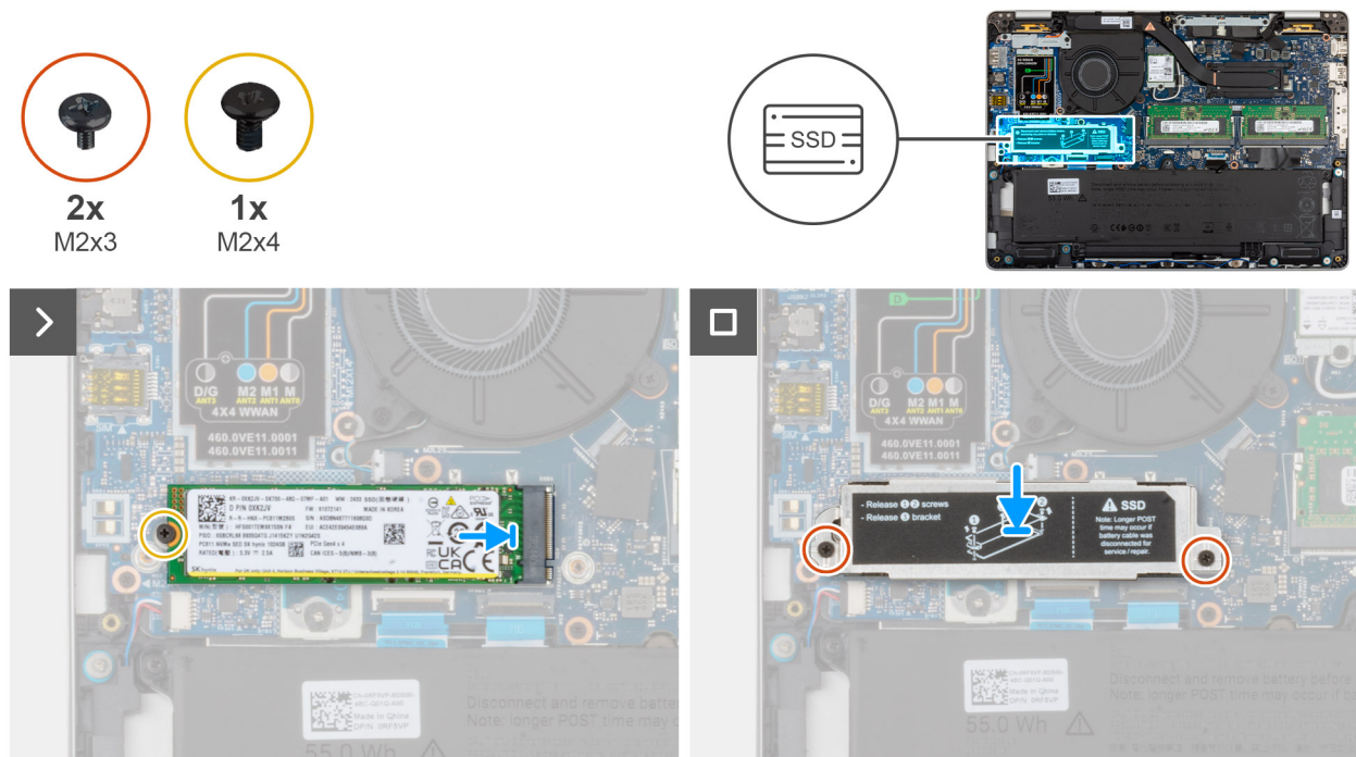
Abbildung 40. Installieren der M.2-2280-SSD
