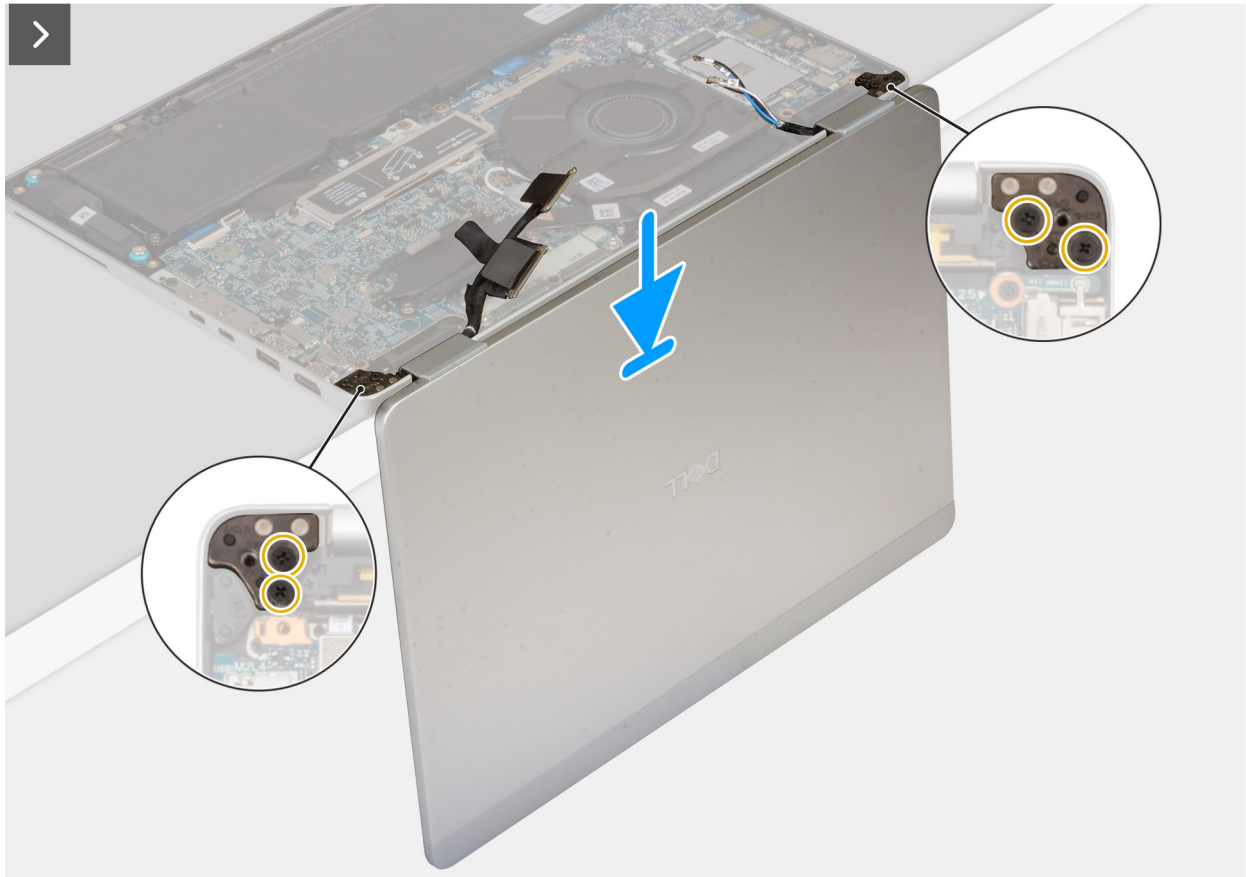
Abbildung 54. Einbauen der Bildschirmbaugruppe
