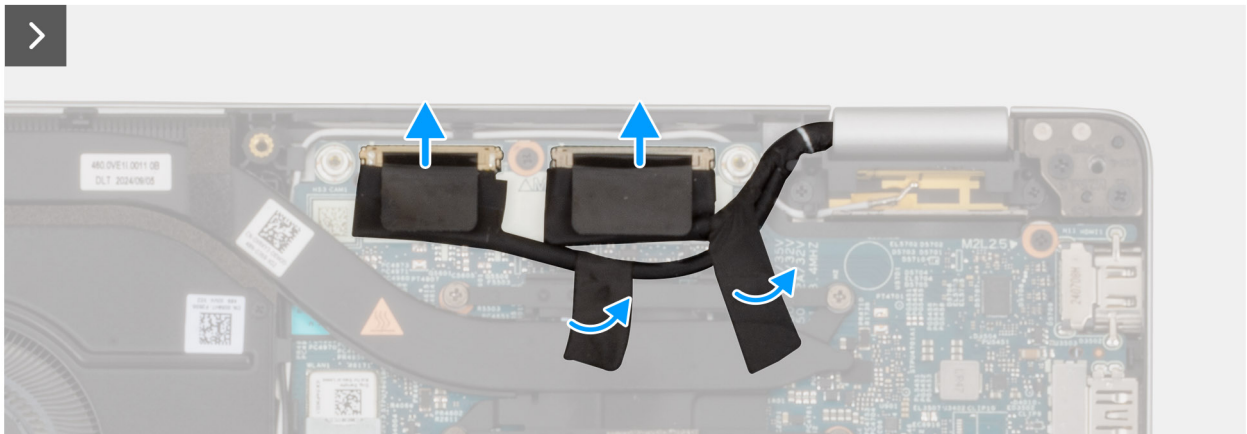
Abbildung 52. Entfernen der Bildschirmbaugruppe
