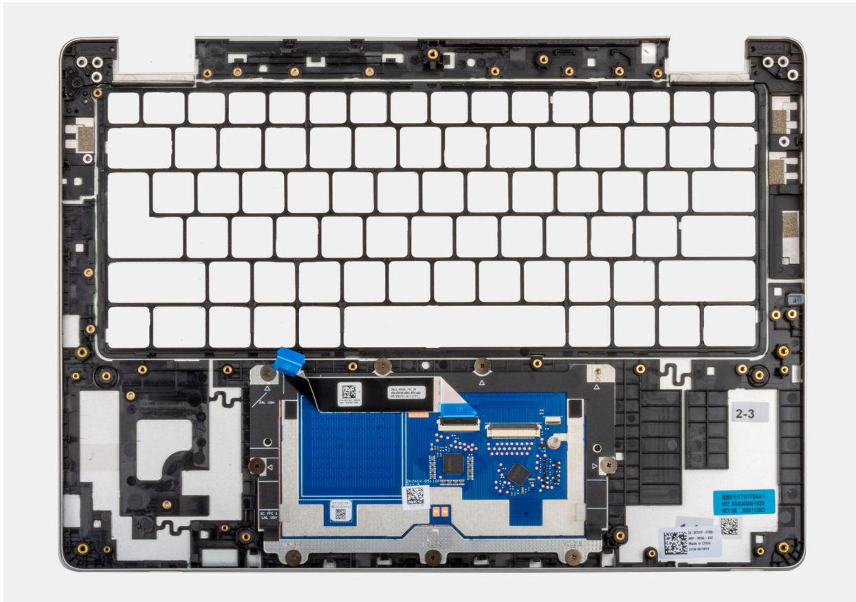
Abbildung 72. Entfernen der Handauflagenbaugruppe
