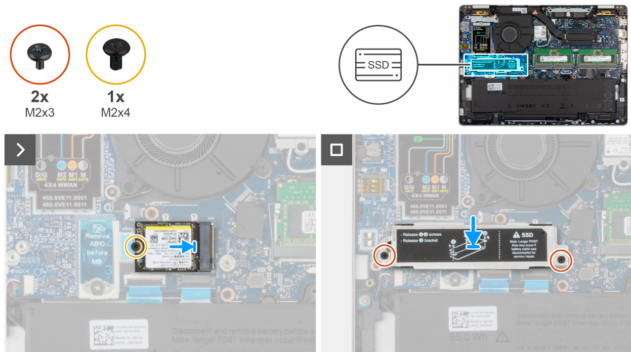
Abbildung 38. Einbauen des M.2-2280-SSD
