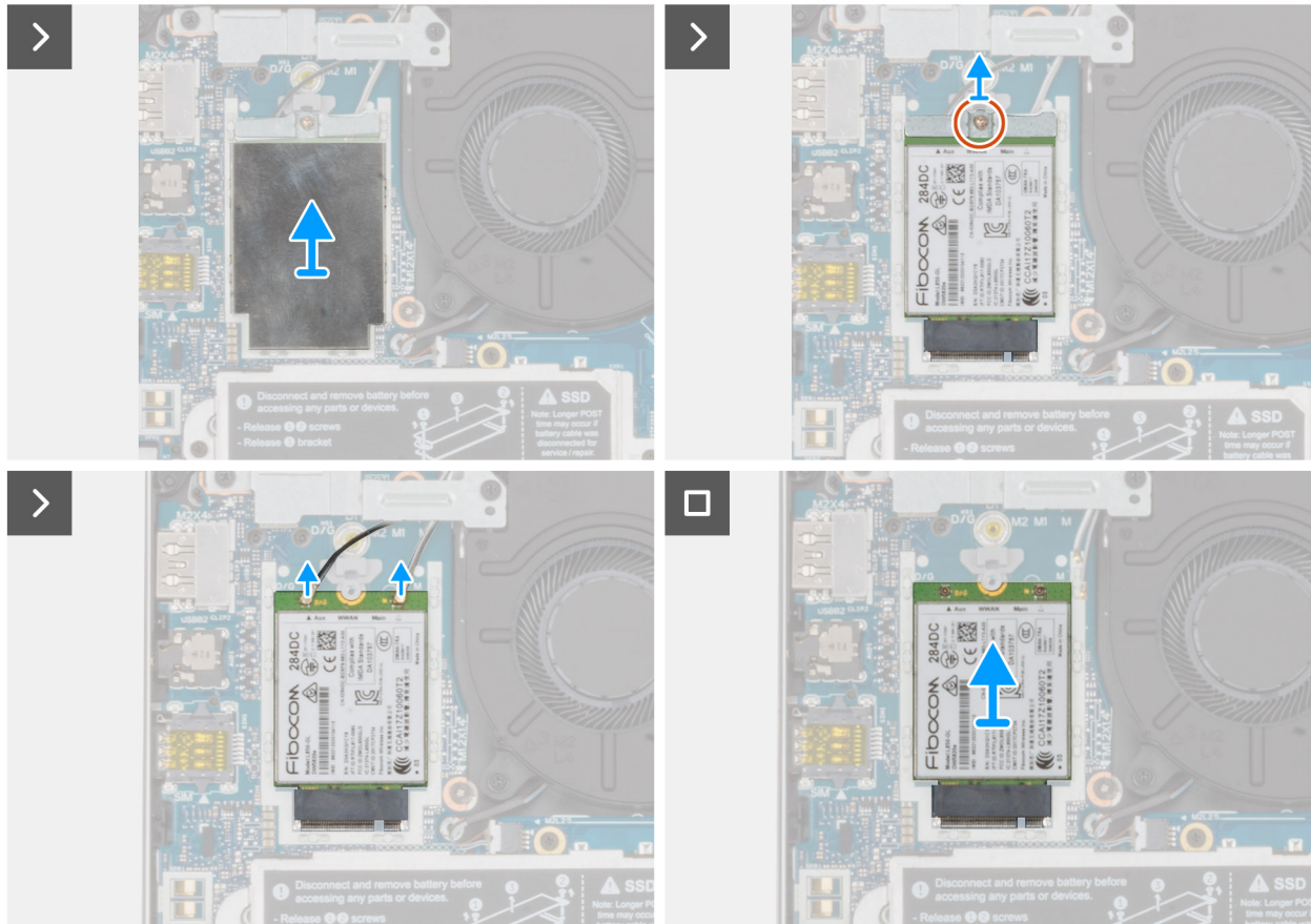
Abbildung 30. Entfernen der 5G-WWAN-Karte
