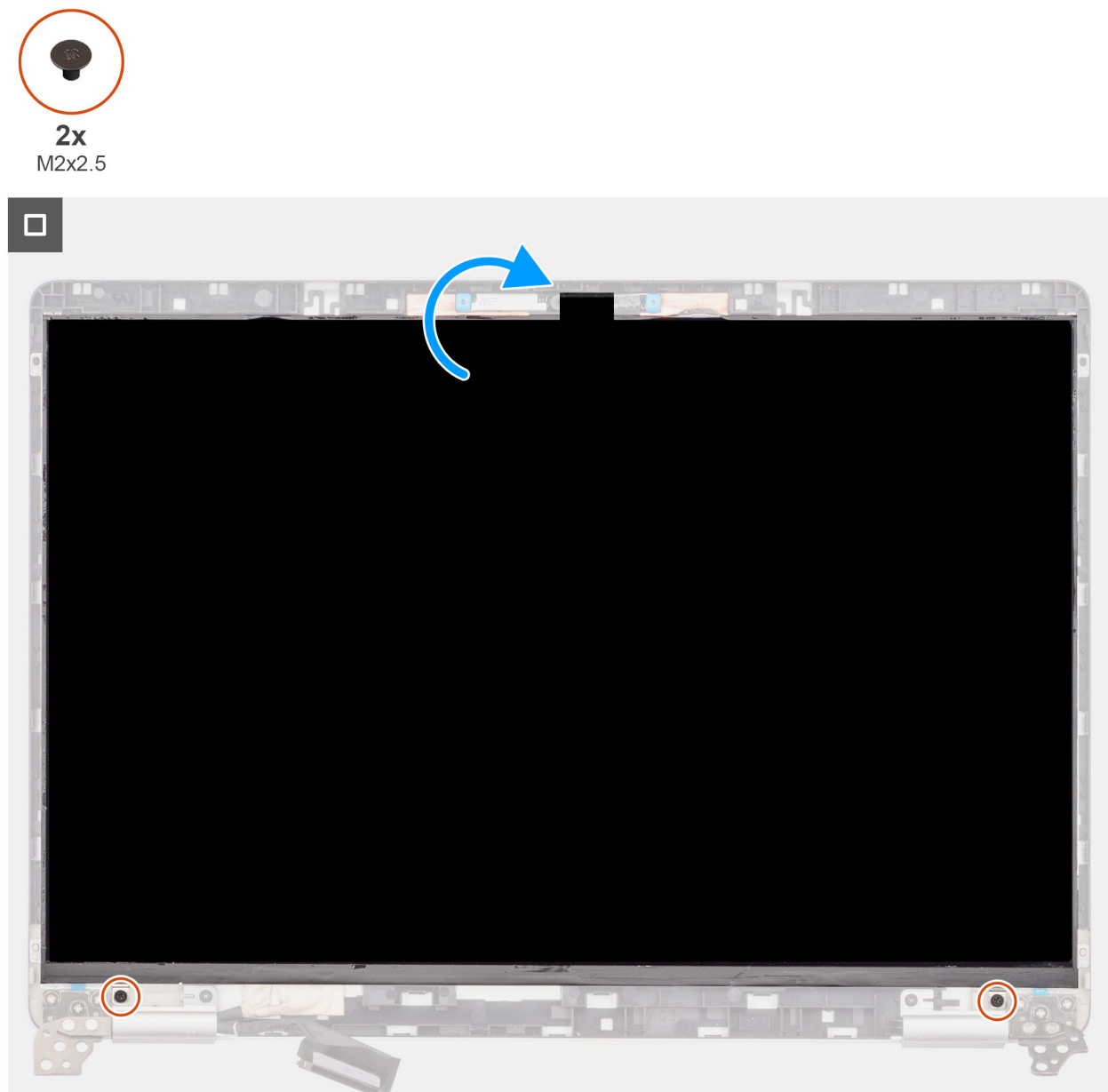
Abbildung 78. Einbauen des Bildschirms
