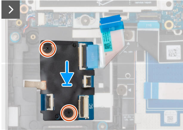
Abbildung 47. Einbauen der USH-Platine
