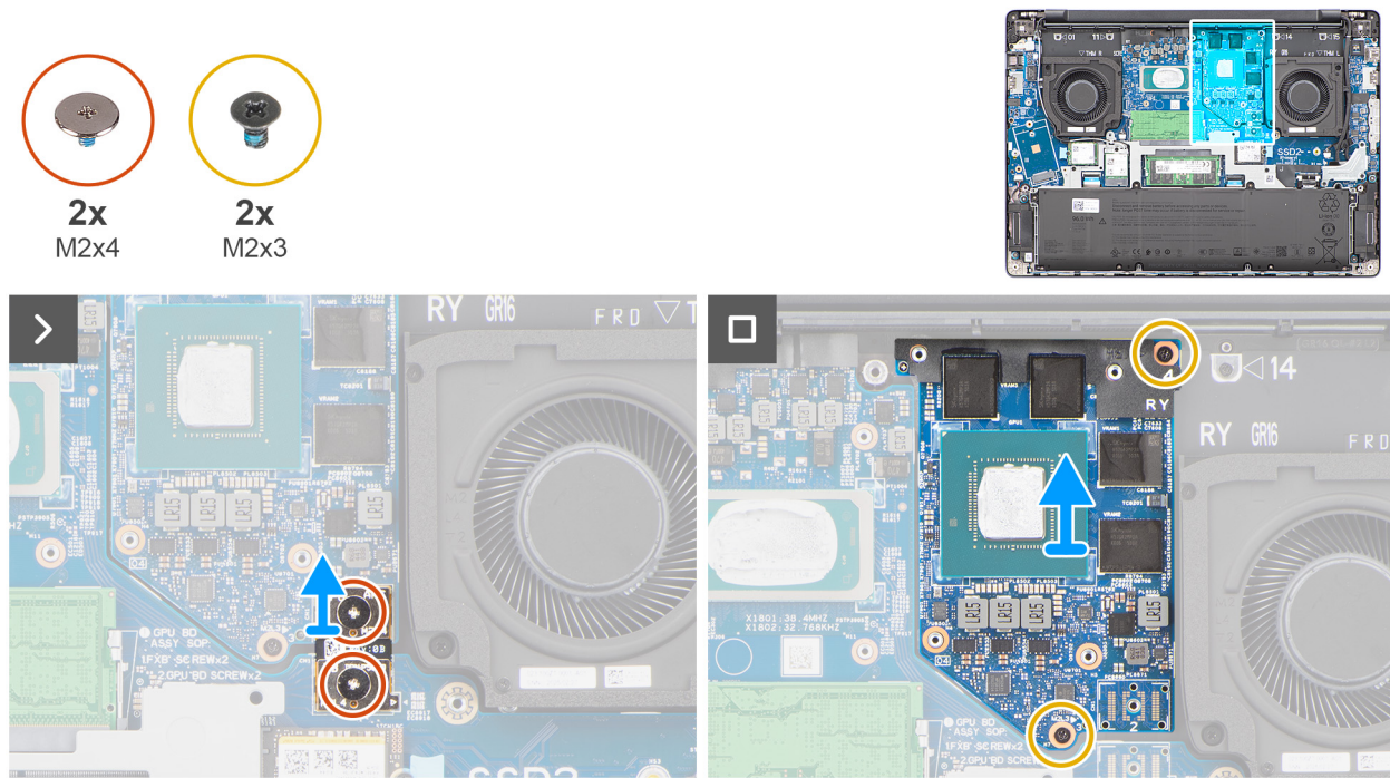
Ilustración 46. Extracción de GPU
