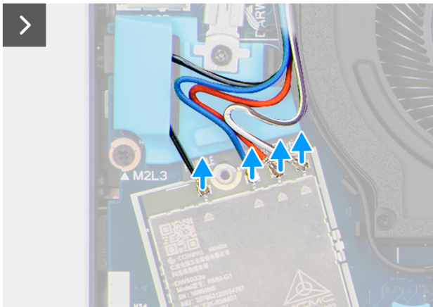
Ilustración 29. Extracción del módulo de WWAN
