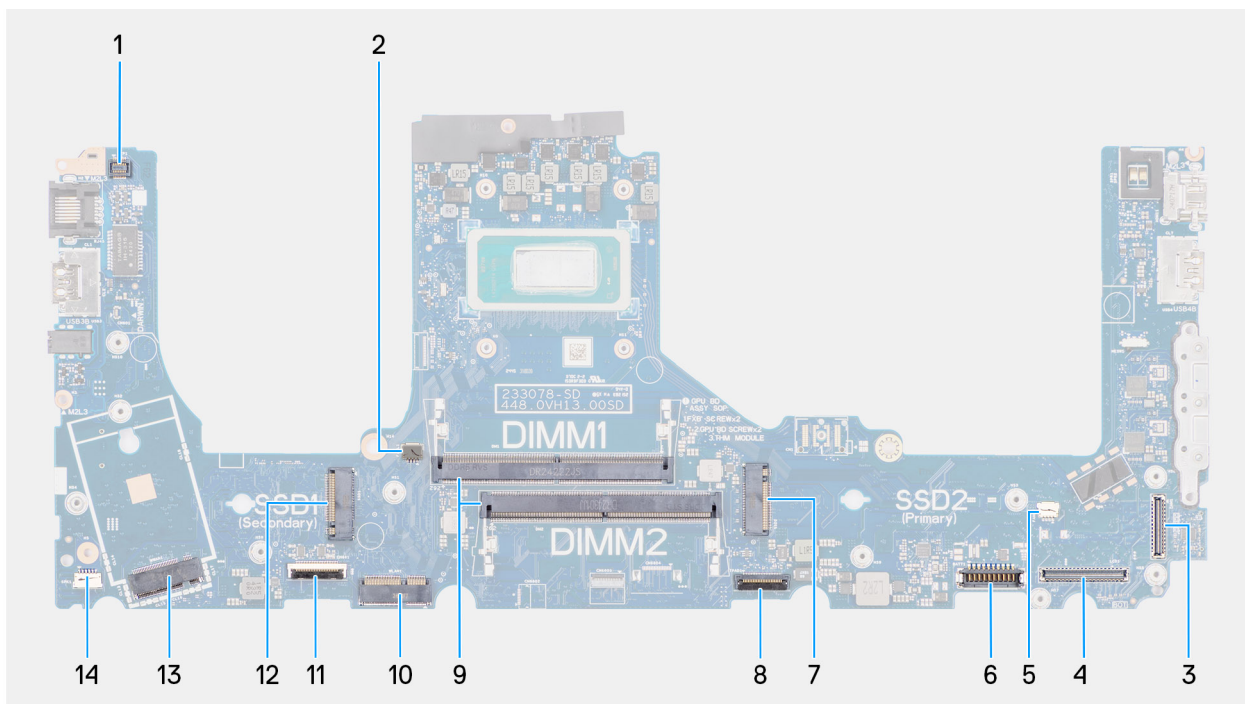
Ilustración 88. Conectores de la tarjeta madre
