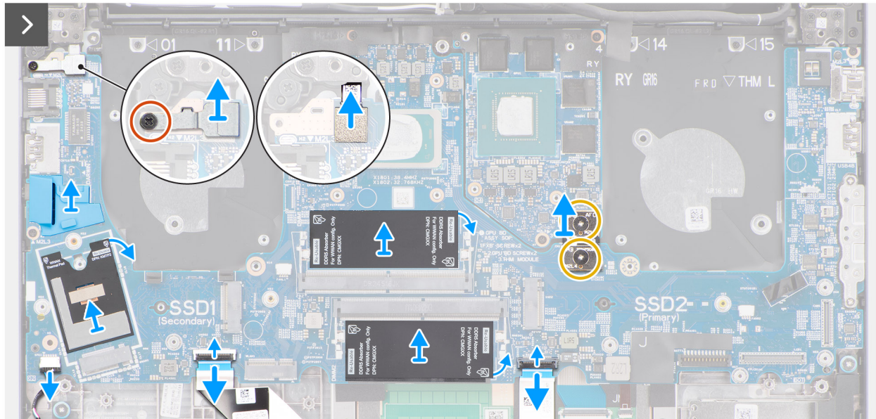
Ilustración 89. Extracción de la tarjeta madre
