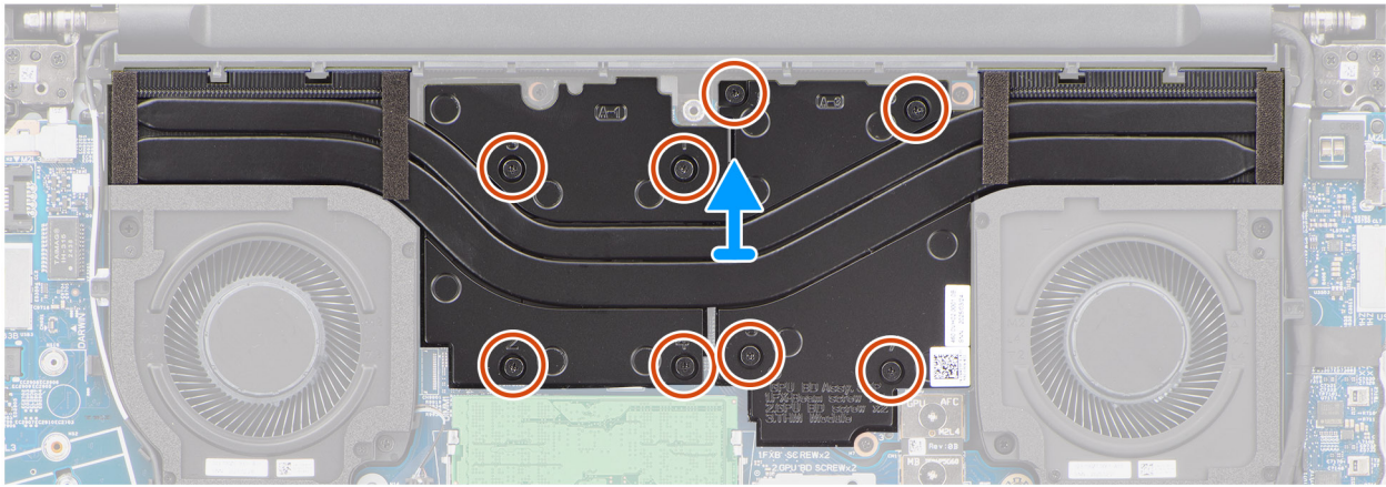
Ilustración 42. Extracción del disipador de calor
