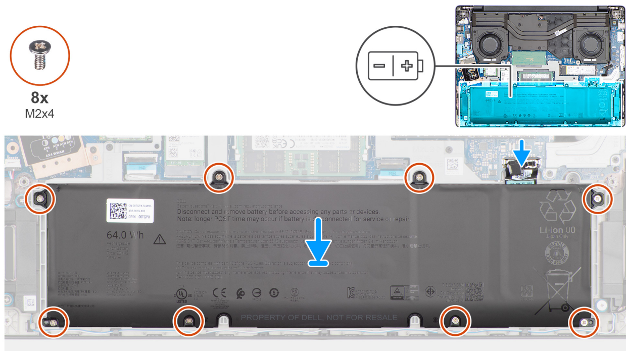
Ilustración 18. Instalación de la batería
