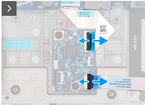
Ilustración 50. Extracción de la placa USH
