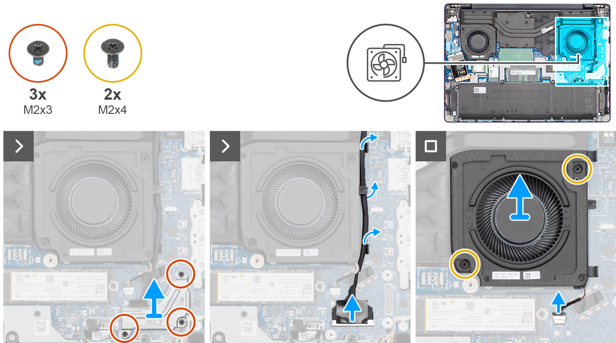
Ilustración 38. Extracción del ventilador izquierdo/de video
