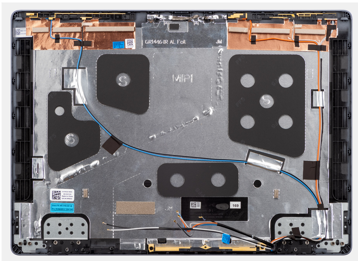
Ilustración 81. Ensamblaje de la antena y la cubierta posterior de la pantalla
