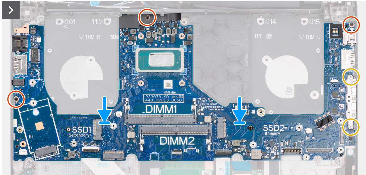
Ilustración 86. Instalación de la tarjeta madre
