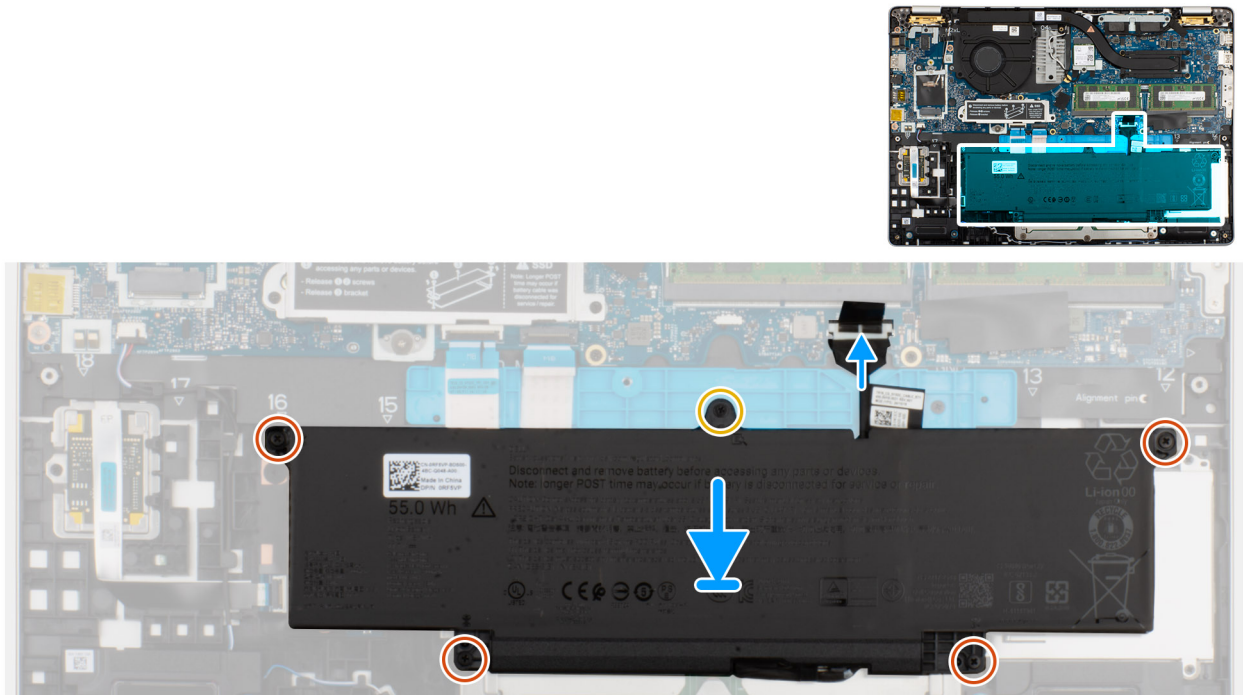
Ilustración 16. Conexión del cable de la batería
