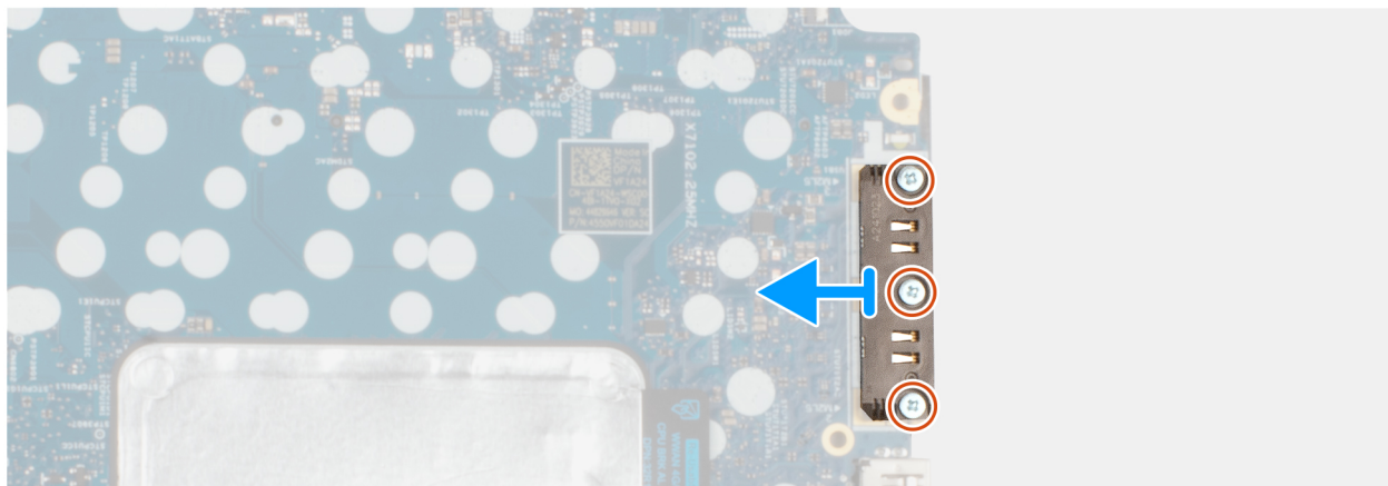
Ilustración 82. Extracción del módulo del conector USB Type-C
