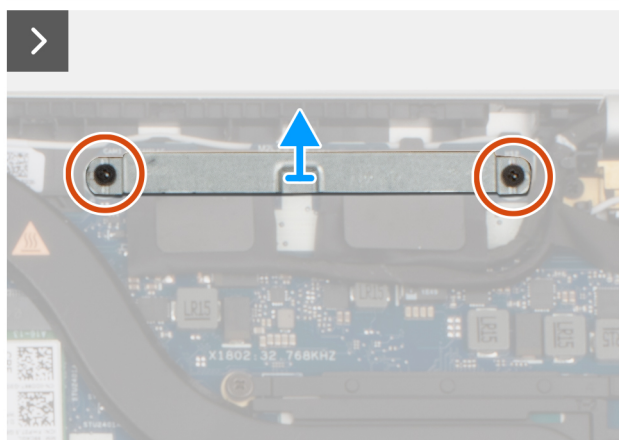
Ilustración 43. Extracción de la antena WLAN
