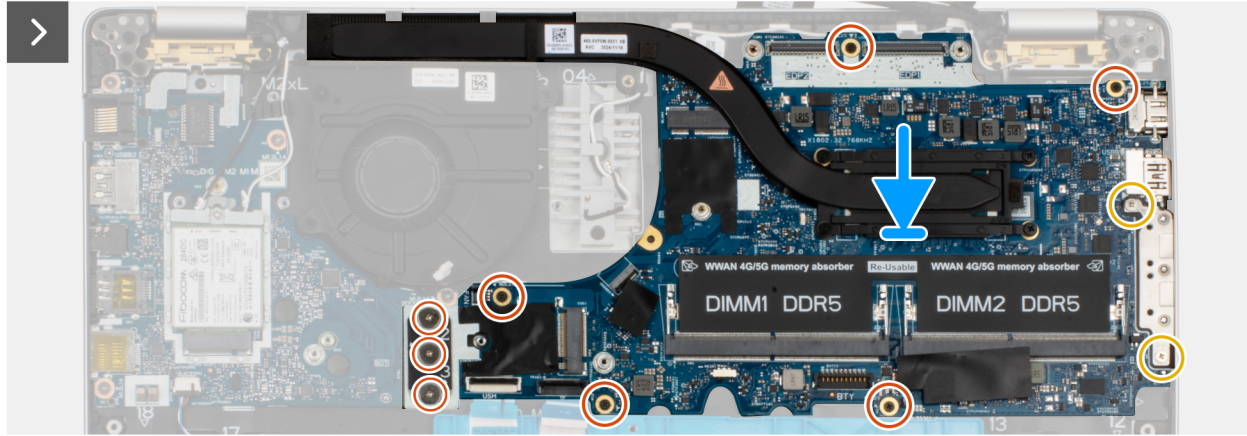
Ilustración 55. Instalación de la tarjeta madre
