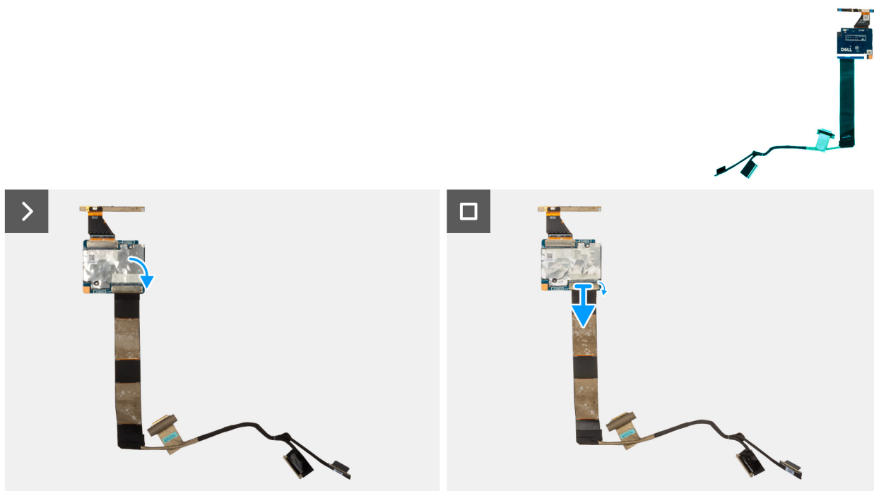
Ilustración 76. Extracción del cable de pantalla
