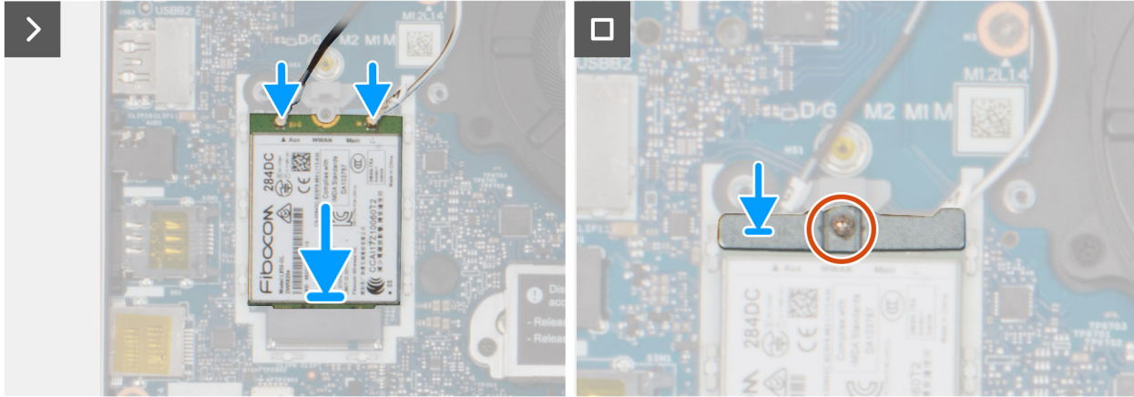
Ilustración 34. Instalación de la tarjeta 4G WWAN
