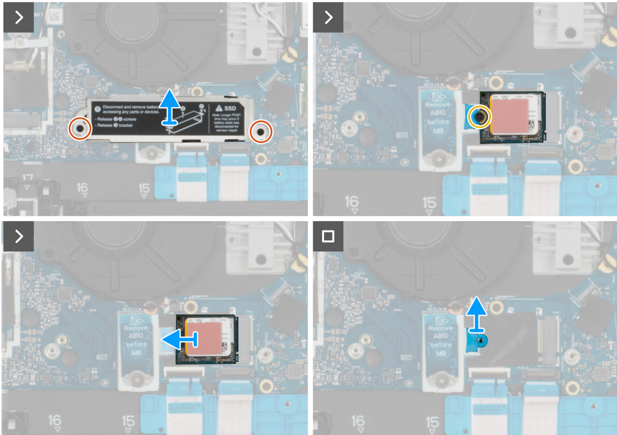
Ilustración 24. Extracción de la SSD M.2 2230
