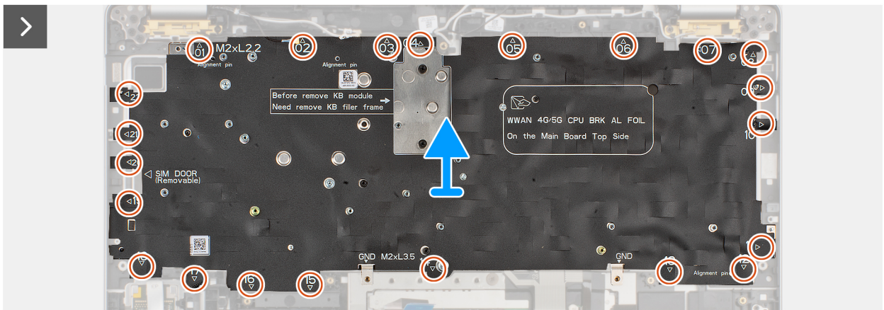
Ilustración 84. Extracción del teclado
