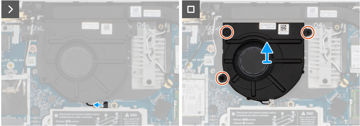
Ilustración 37. Extracción del ventilador
