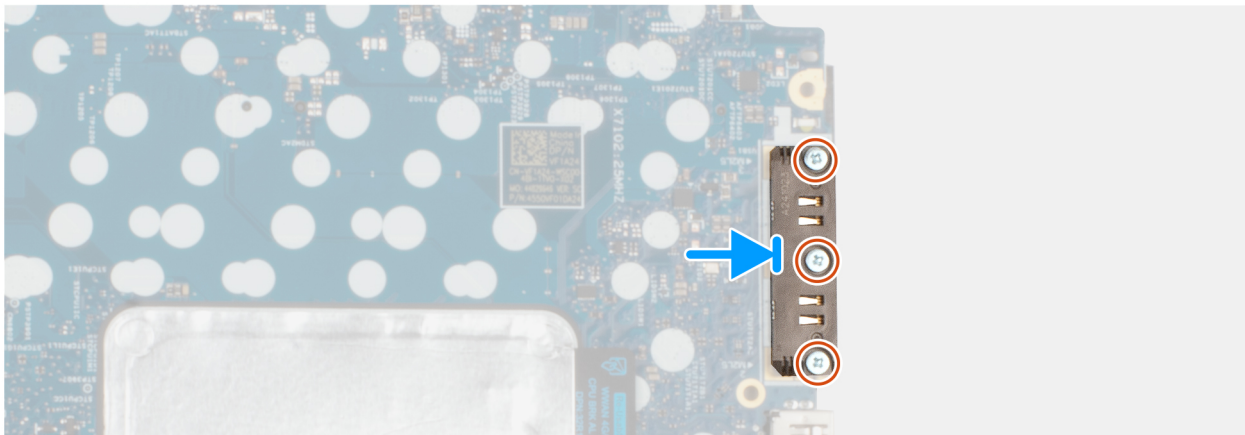
Ilustración 83. Instalación del módulo del conector USB Type-C
