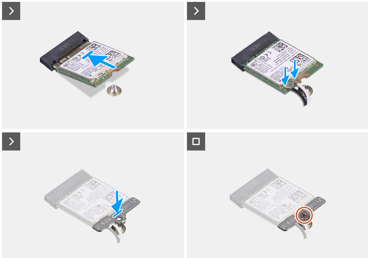
Ilustración 36. Instalación de la tarjeta WLAN
