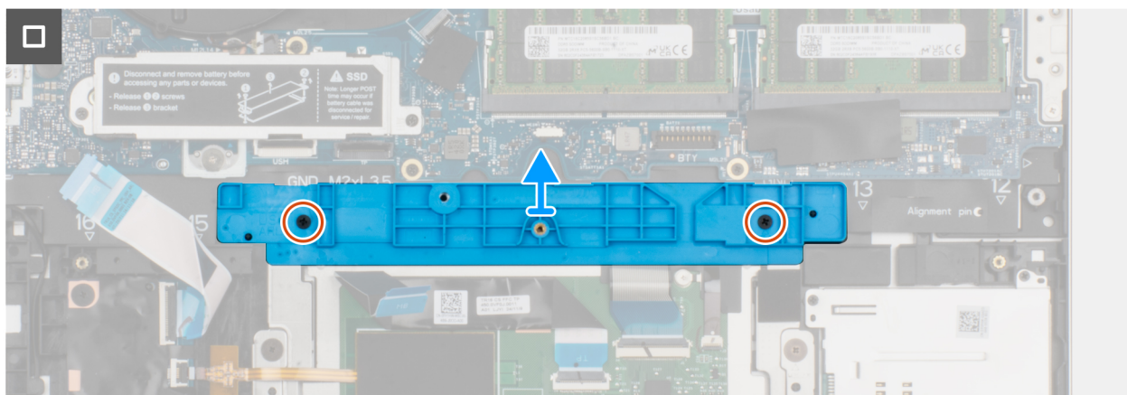
Ilustración 47. Extracción del soporte de la batería
