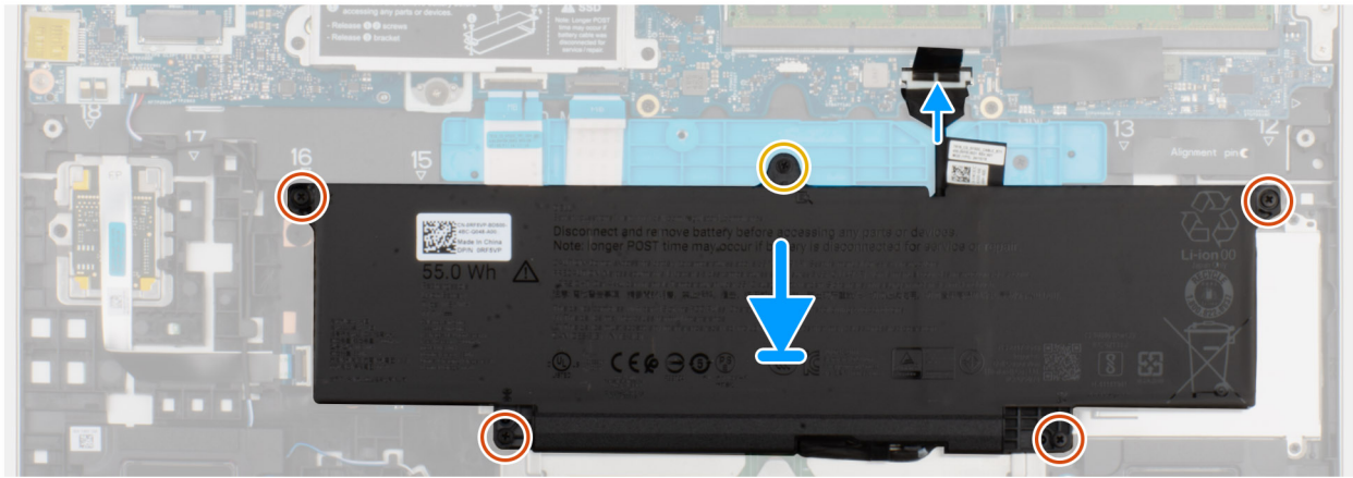
Ilustración 19. Instalación de la batería
