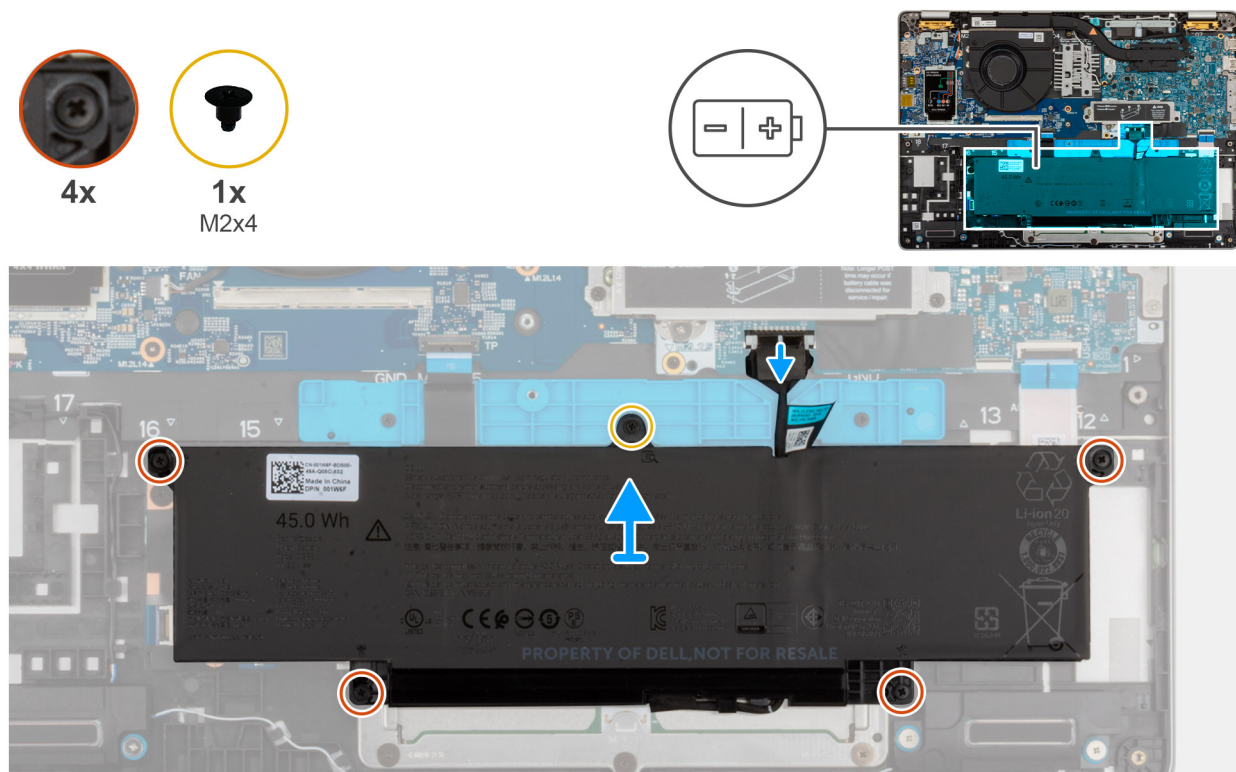
Afbeelding 18. De batterij verwijderen
