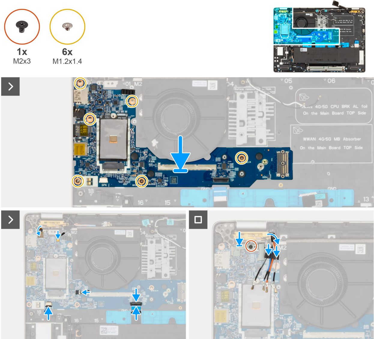
Afbeelding 52. De I/O-kaart installeren
