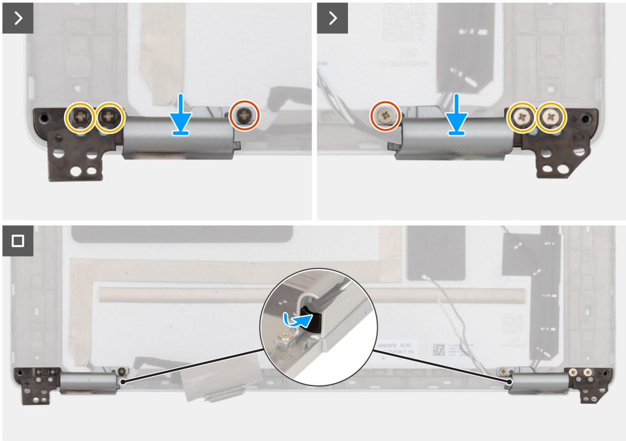
Afbeelding 81. De beeldschermcharnierenkappen plaatsen
