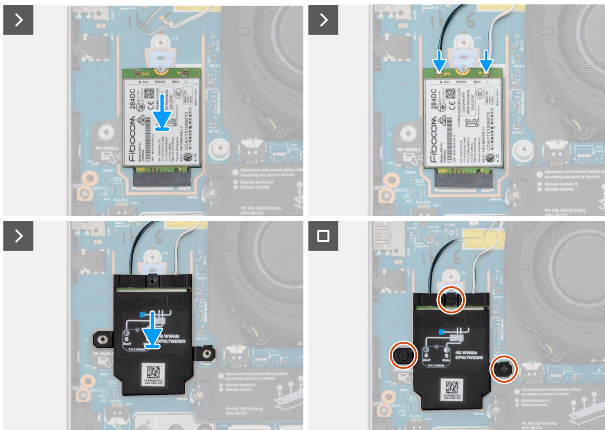
Afbeelding 35. De WWAN-kaart installeren
