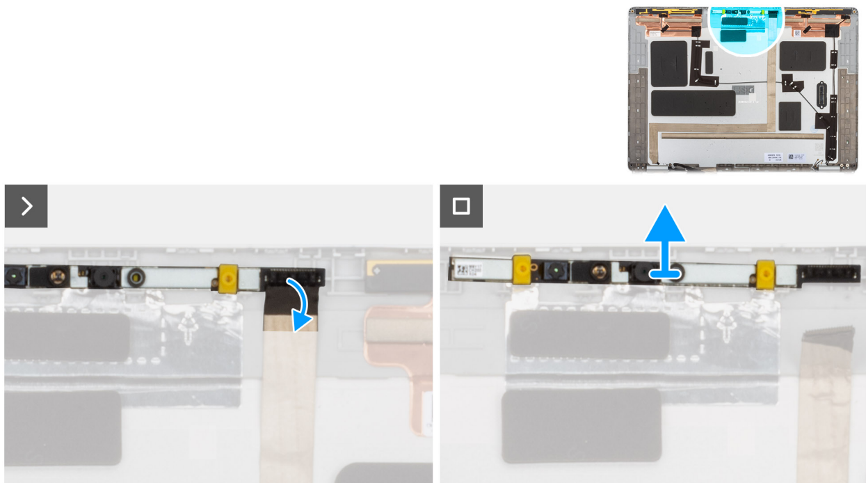
Afbeelding 82. De RGB/IR-camera verwijderen
