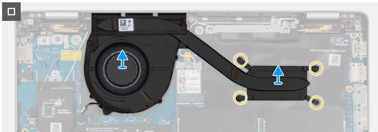
Afbeelding 44. De ventilator- en koelplaateneheid verwijderen
