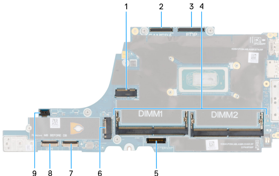
Afbeelding 50. Stroomkaartconnectoren
