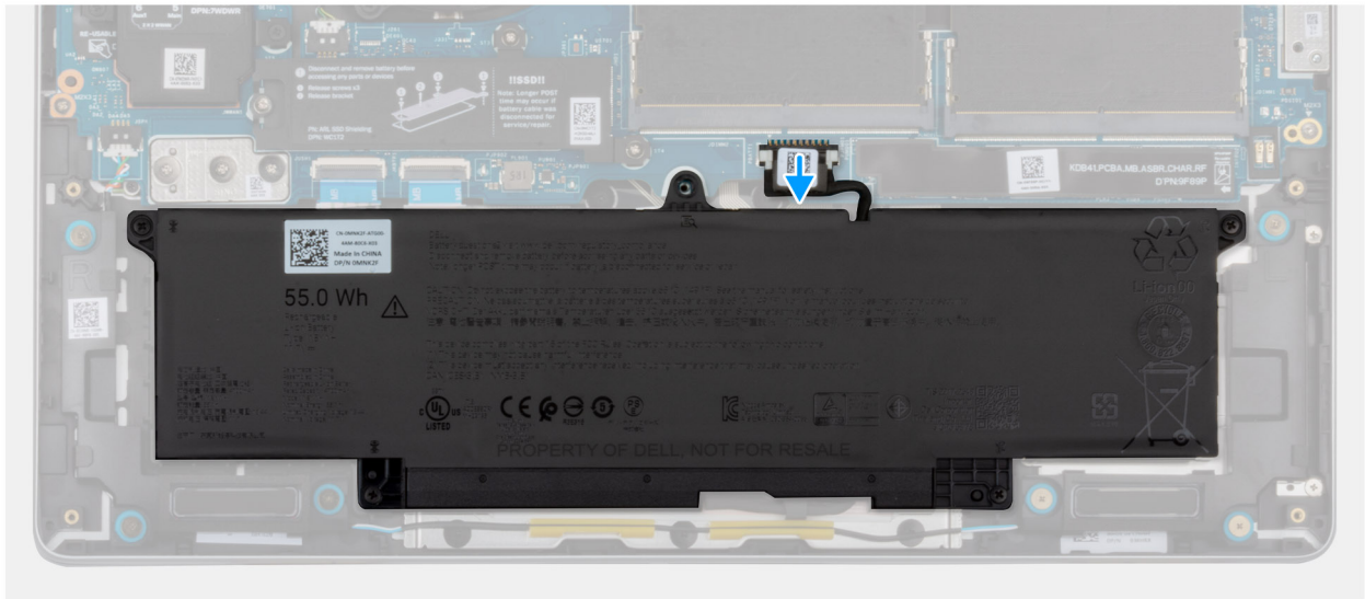
Afbeelding 24. De batterijkabel loskoppelen
