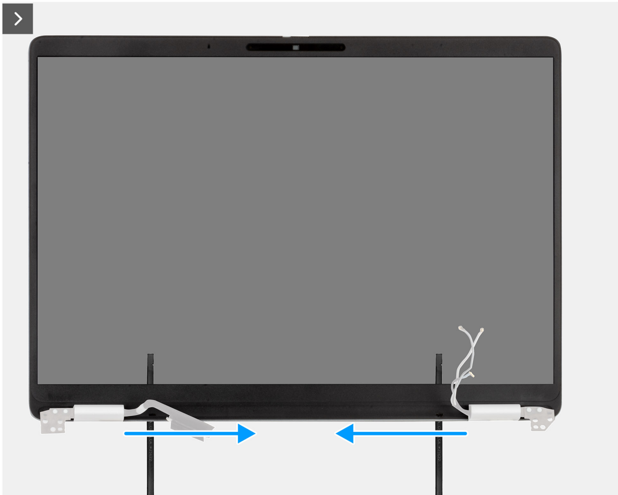
Afbeelding 69. De beeldschermbezel verwijderen
