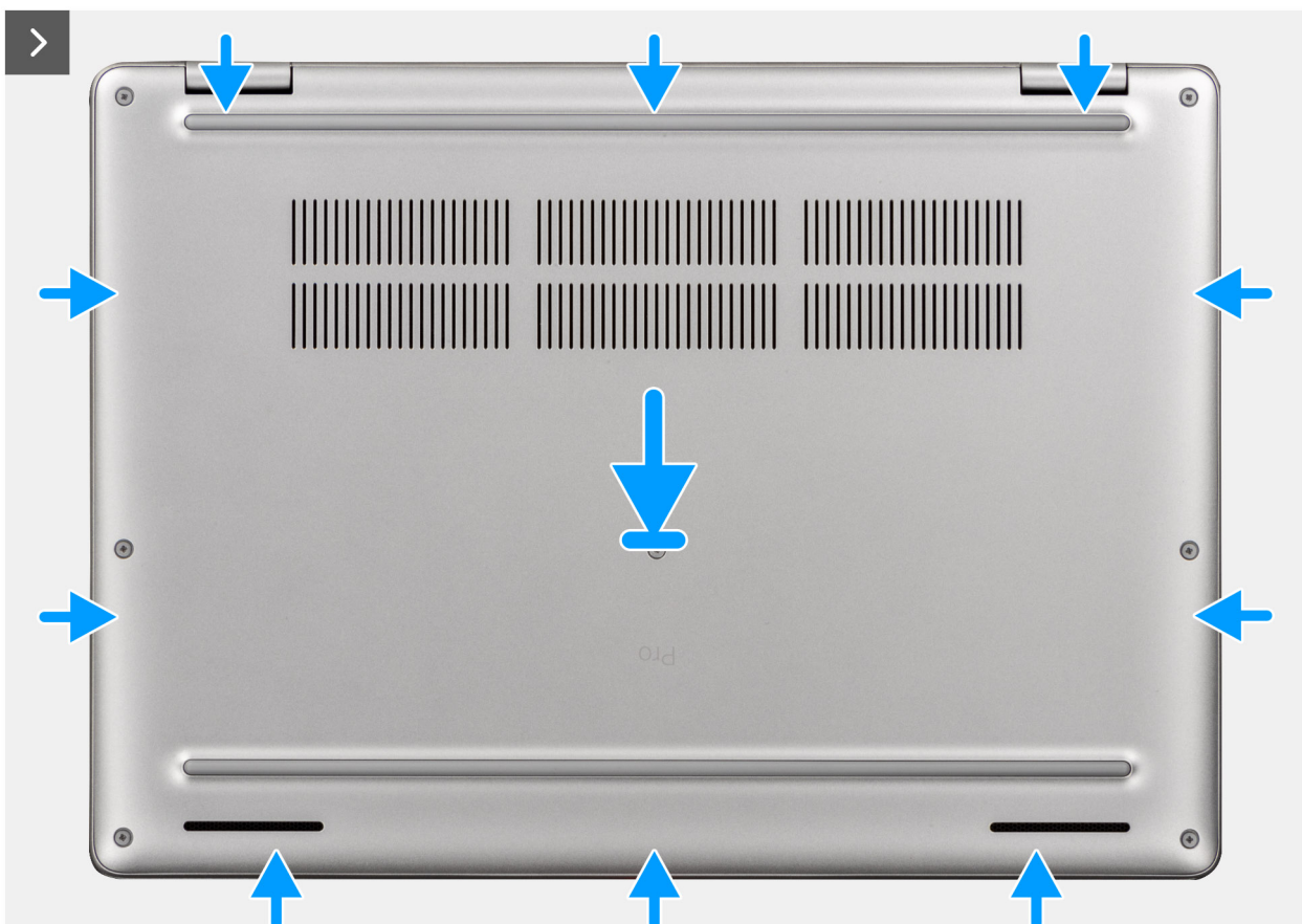
Afbeelding 26. De onderplaat installeren
