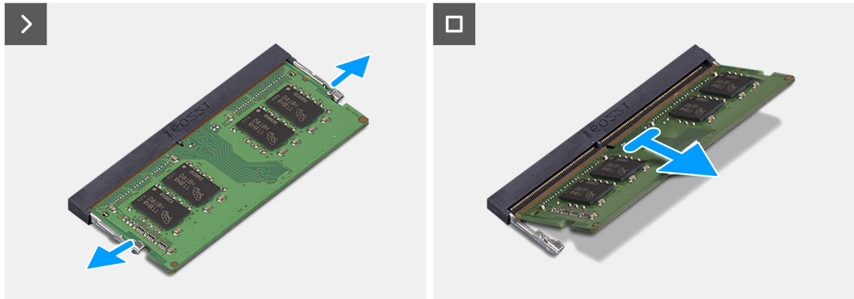
Afbeelding 32. De geheugenmodule verwijderen
