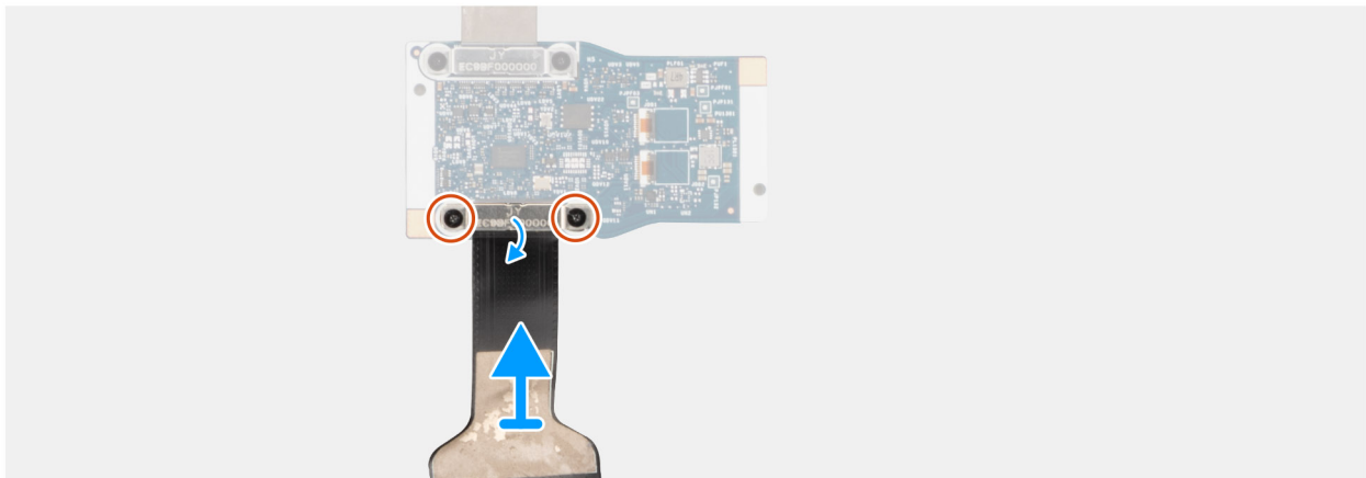
Afbeelding 90. De beeldschermkabel voor de MIPI-camera verwijderen
