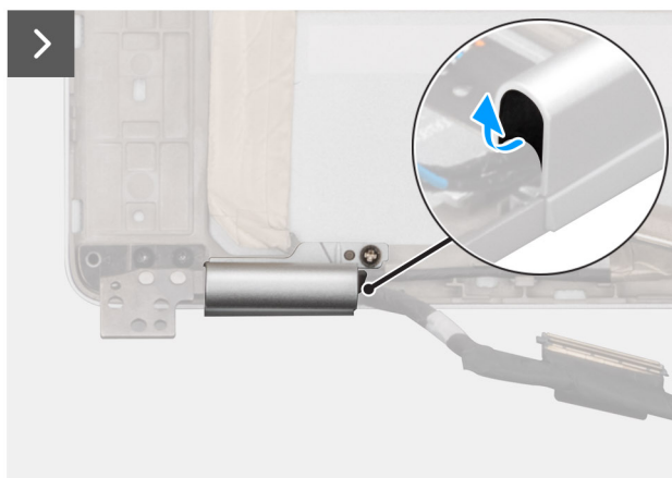
Afbeelding 84. De beeldschermkabel verwijderen
