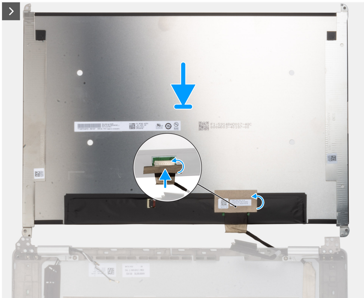
Afbeelding 78. Het beeldschermpaneel installeren
