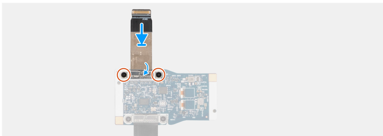
Afbeelding 93. De kabel van het middelste bord plaatsen
