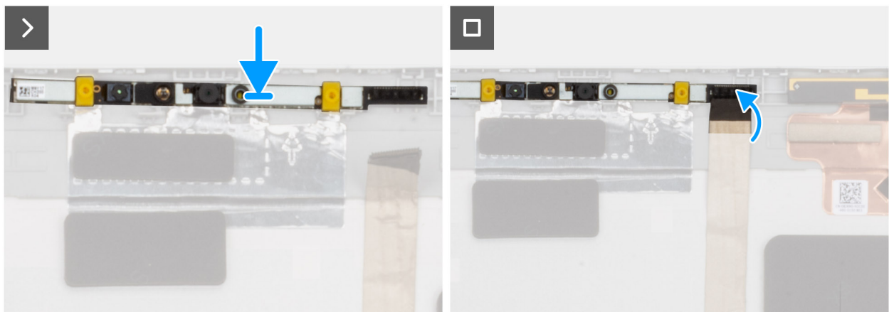
Afbeelding 83. De RGB/IR-camera installeren
