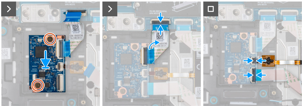
Afbeelding 47. De USH-kaart plaatsen
