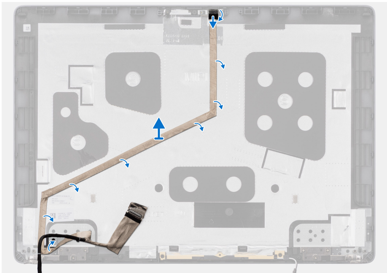
Afbeelding 67. De beeldschermkabel verwijderen
