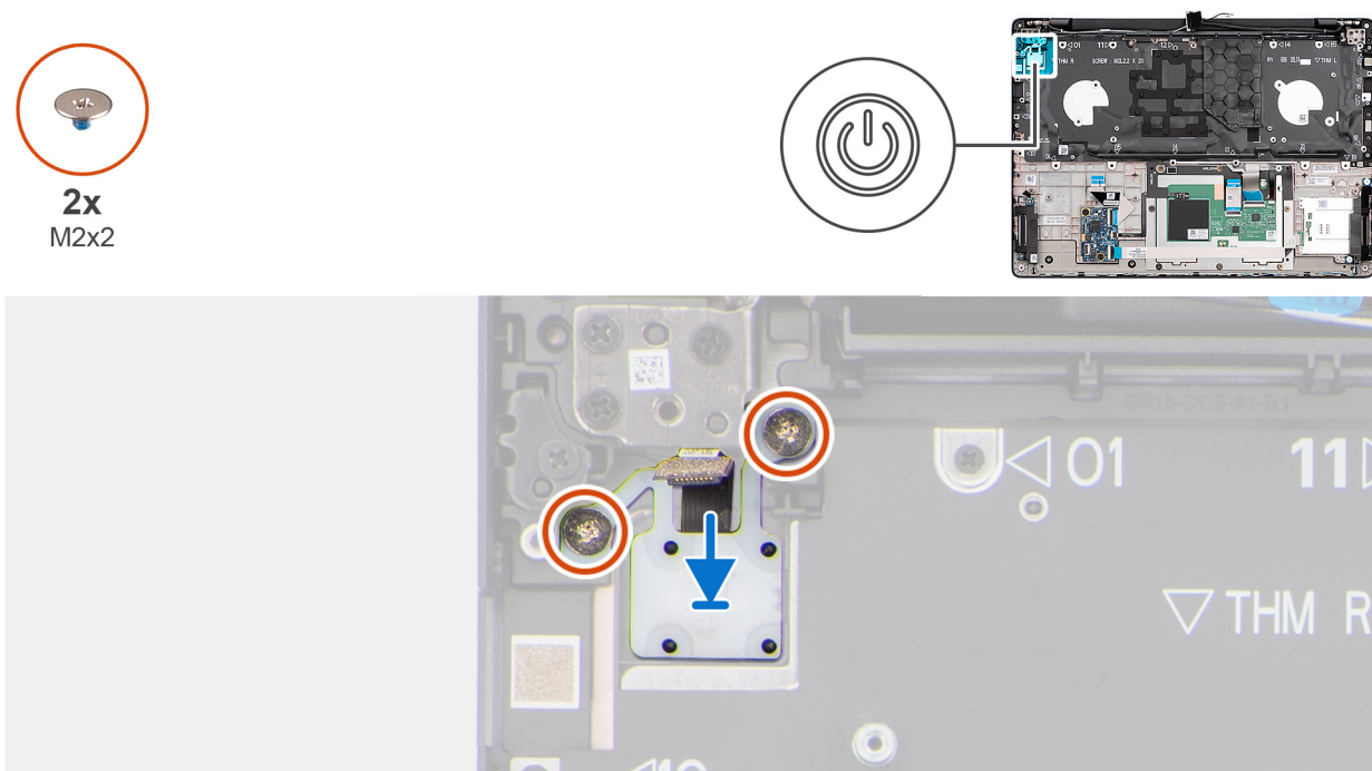
Afbeelding 82. De aan-uitknop plaatsen
