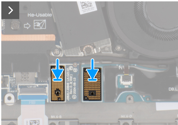
Afbeelding 42. De linker-I/O-kaart installeren
