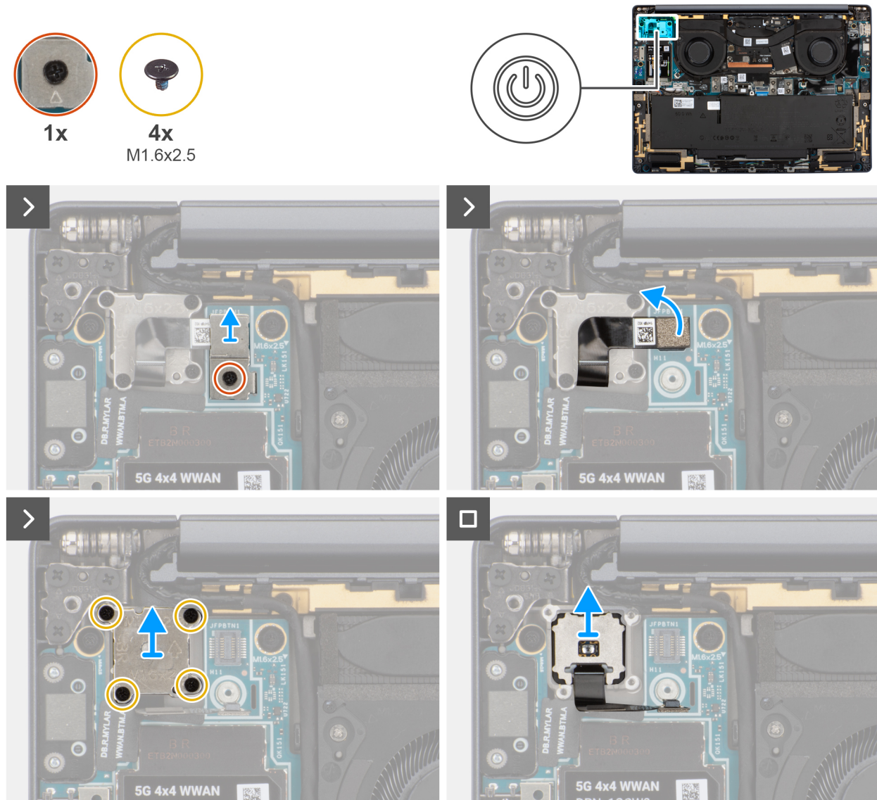
Afbeelding 56. De aan-uitknop verwijderen
