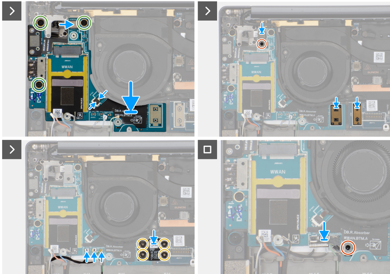
Afbeelding 50. De rechter I/O-kaart installeren (met WWAN)
