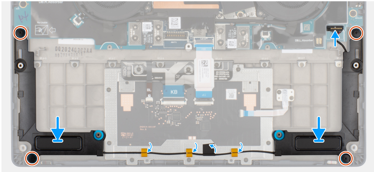
Afbeelding 35. De luidsprekers installeren (zonder WWAN)
