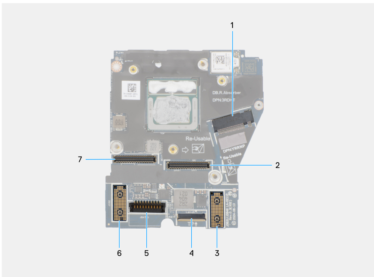
Afbeelding 63. Bijschriften voor de systeemkaart
