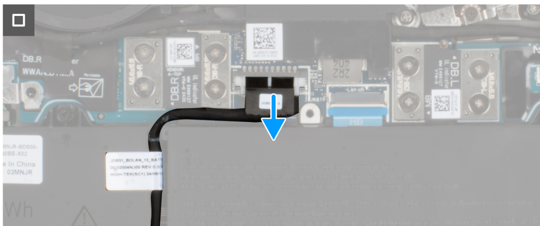
Afbeelding 18. De batterijkabel van de systeemkaart loskoppelen
