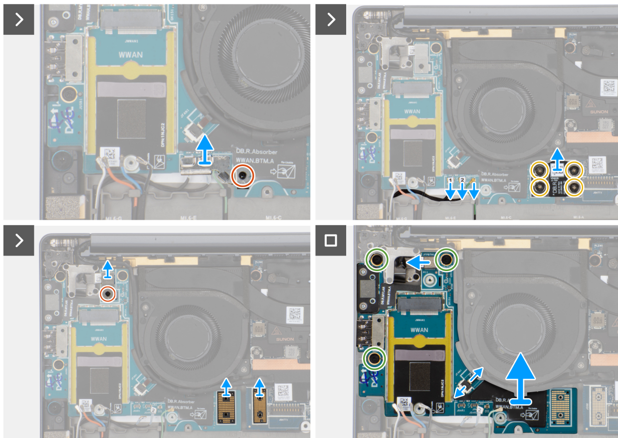
Afbeelding 48. De rechter I/O-kaart verwijderen (met WWAN)
