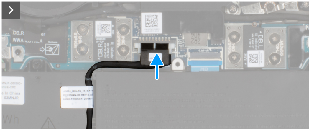
Afbeelding 19. Sluit de batterijkabel aan op de systeemkaart
