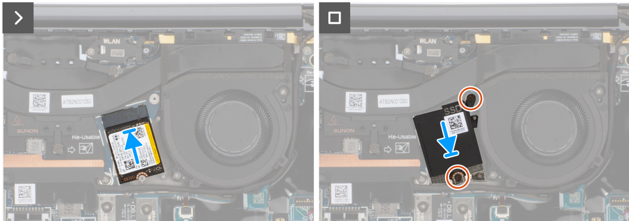
Afbeelding 27. SSD installeren
