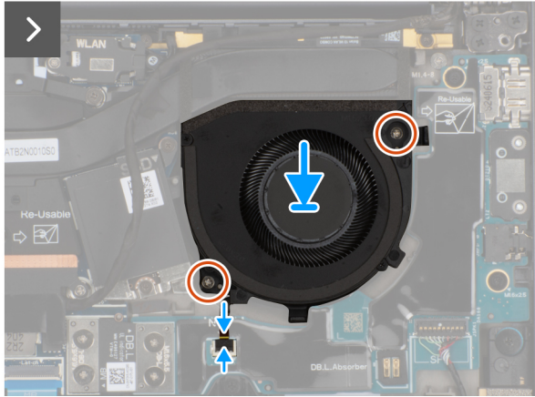
Afbeelding 31. De linkerventilator plaatsen
