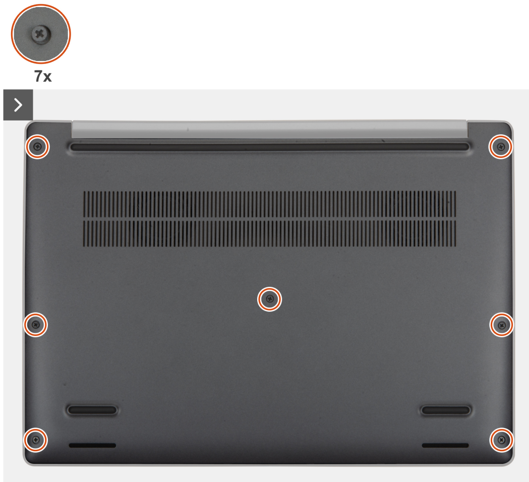
Afbeelding 16. De geborgde schroeven losdraaien
