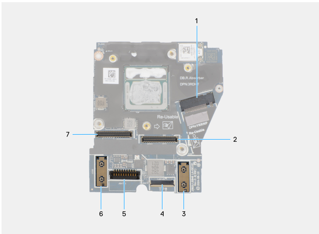
Afbeelding 68. Bijschriften voor de systeemkaart
