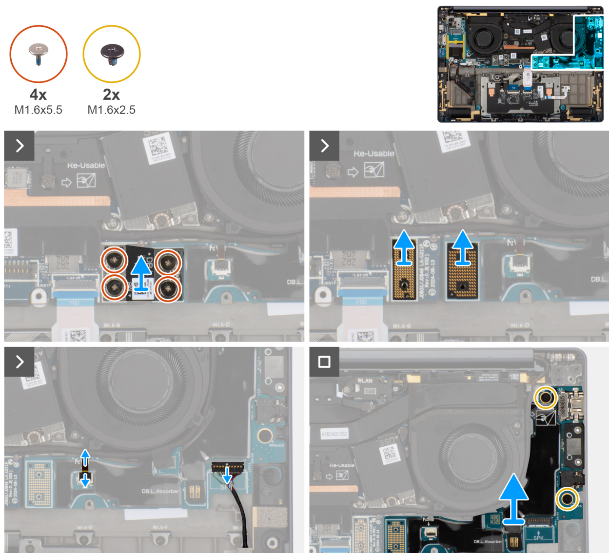
Afbeelding 40. De linker-I/O-kaart verwijderen
