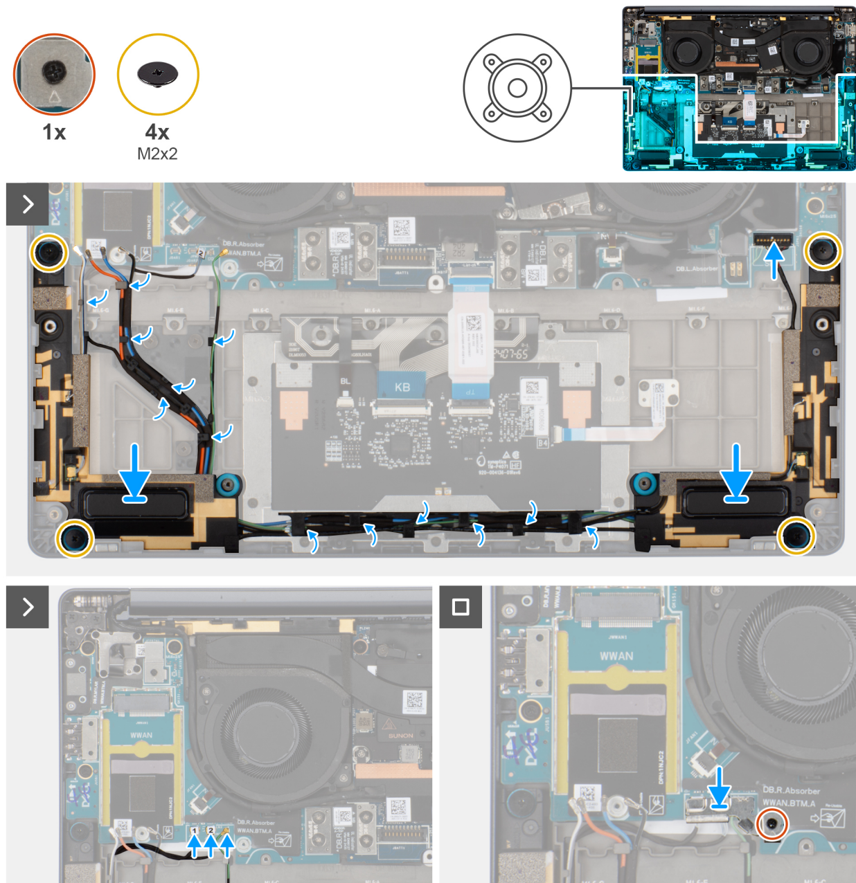
Afbeelding 37. De luidsprekers met antennes installeren (WWAN-configuratie)
