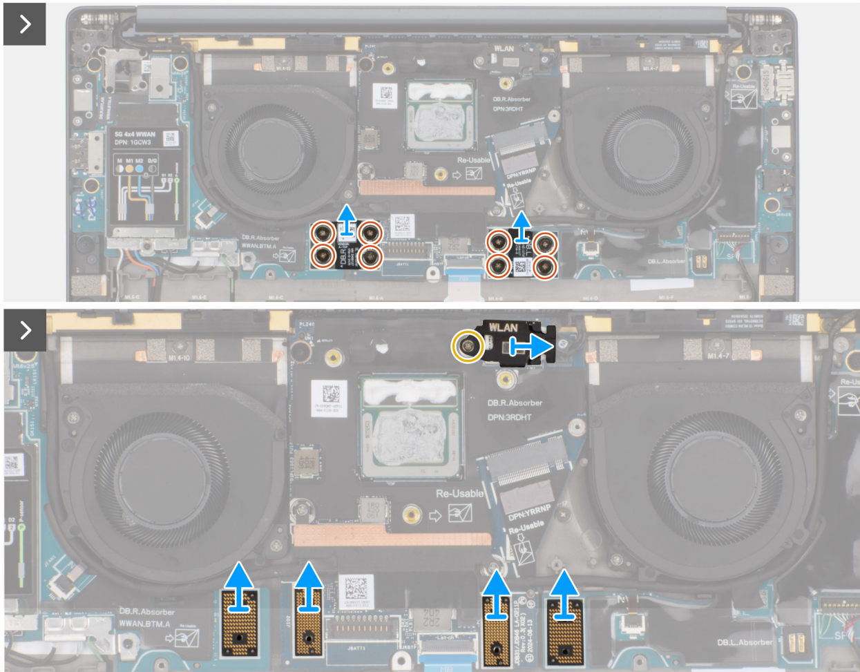
Afbeelding 64. De systeemkaart verwijderen
