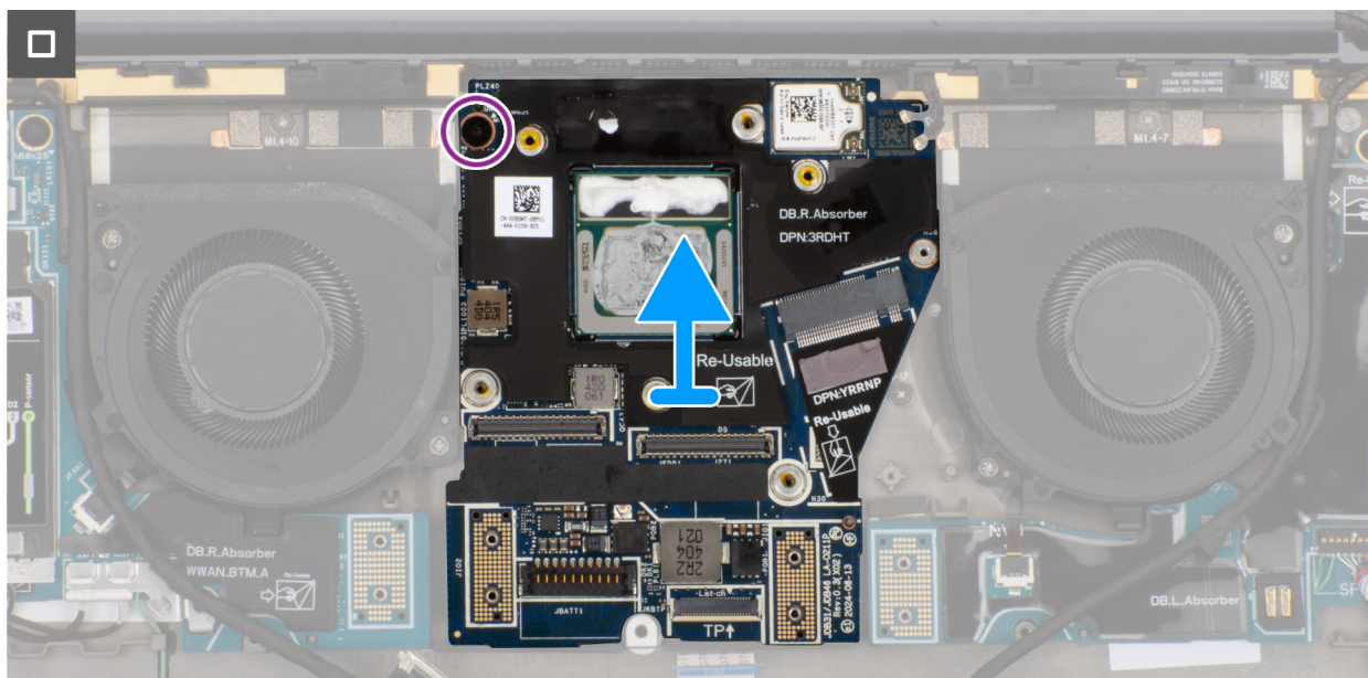
Afbeelding 66. De systeemkaart verwijderen
