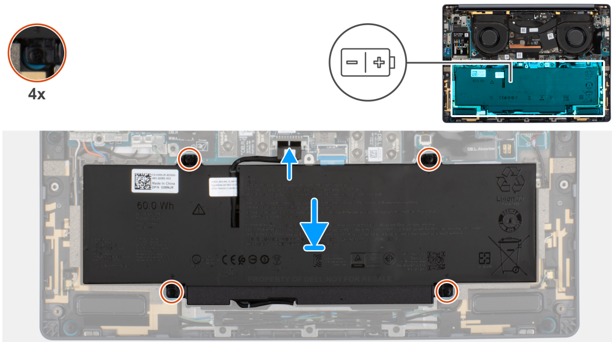
Afbeelding 23. De batterij plaatsen
