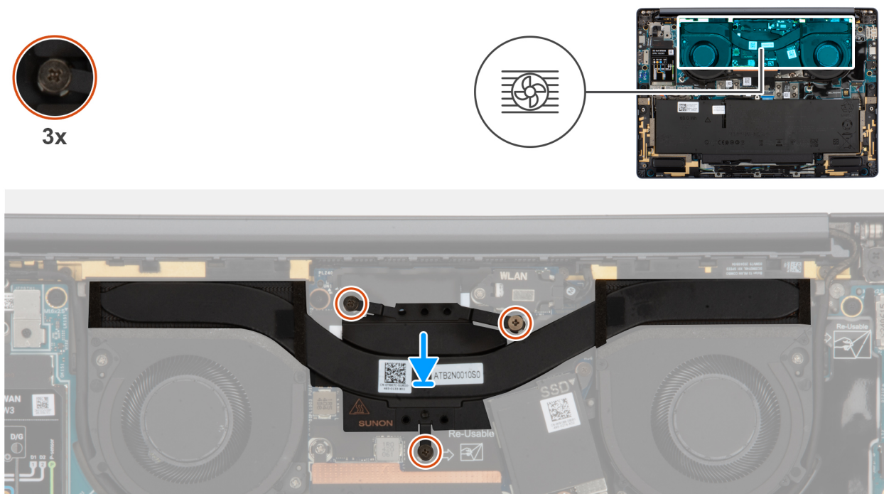
Afbeelding 39. De koelplaat plaatsen
