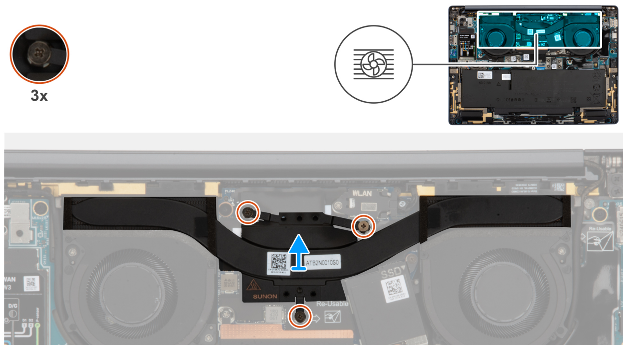
Afbeelding 38. De koelplaat verwijderen
