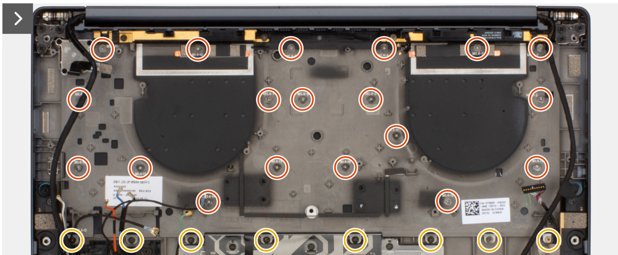
Afbeelding 73. De toetsenbordeenheid verwijderen
