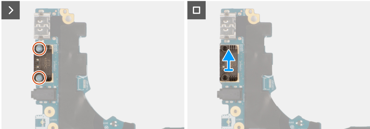
Afbeelding 54. De rechter USB Type-C-module verwijderen
