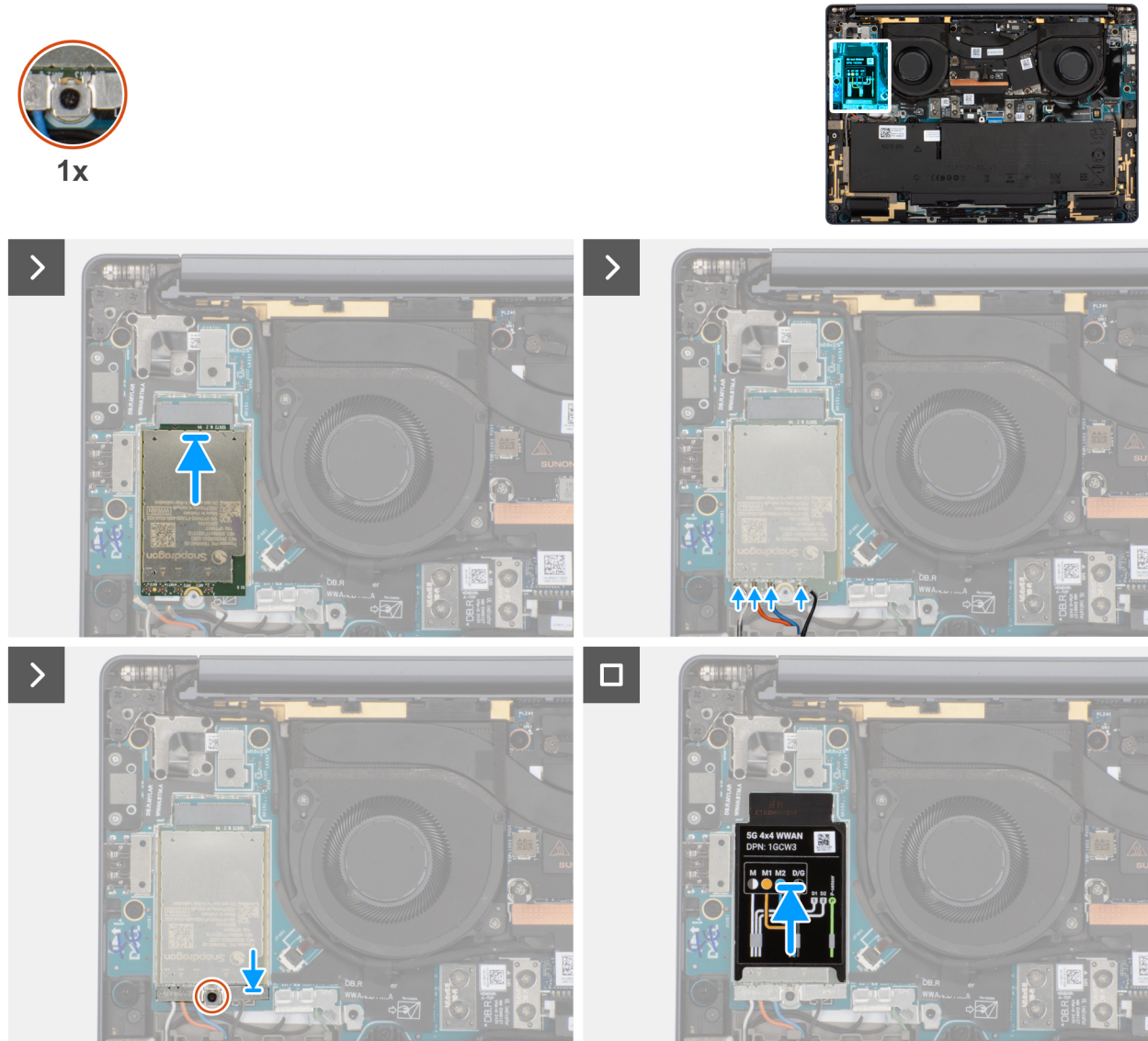
Afbeelding 29. De WWAN-kaart installeren
