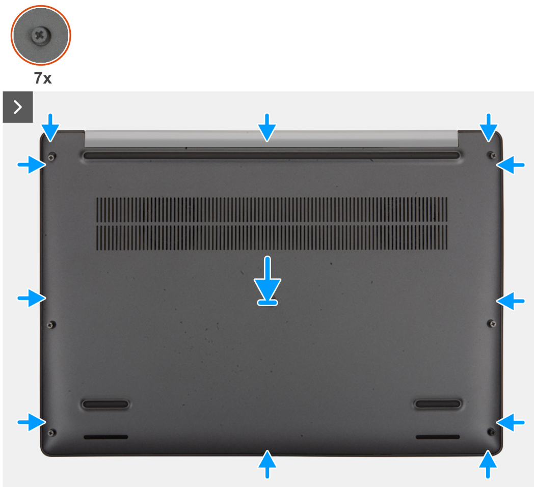
Afbeelding 20. De onderplaat plaatsen
