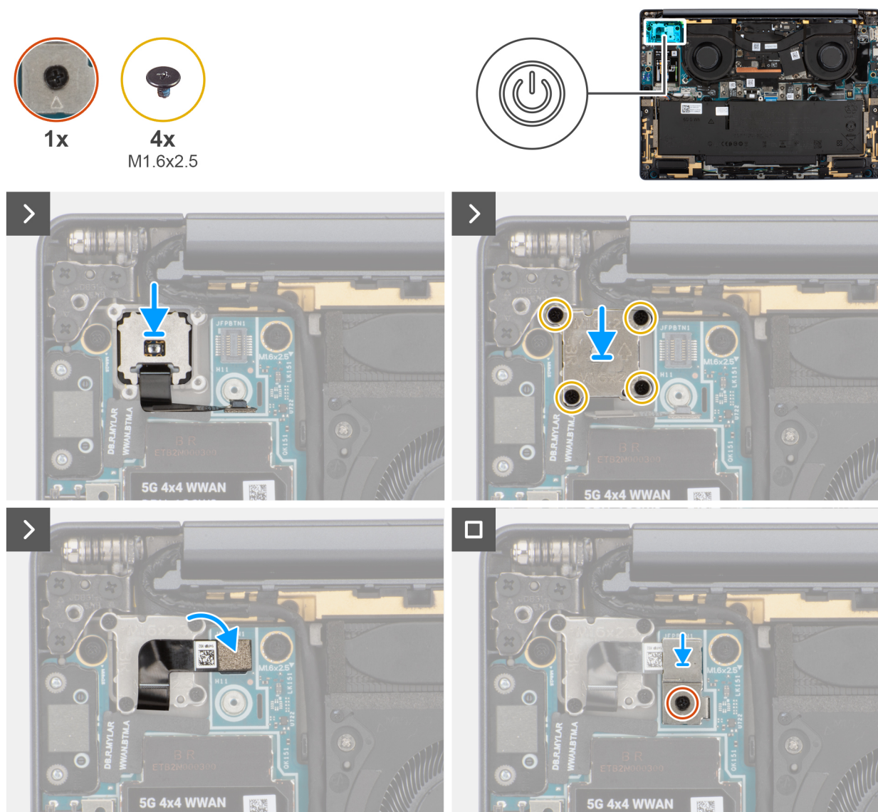
Afbeelding 57. De aan-uitknop plaatsen
