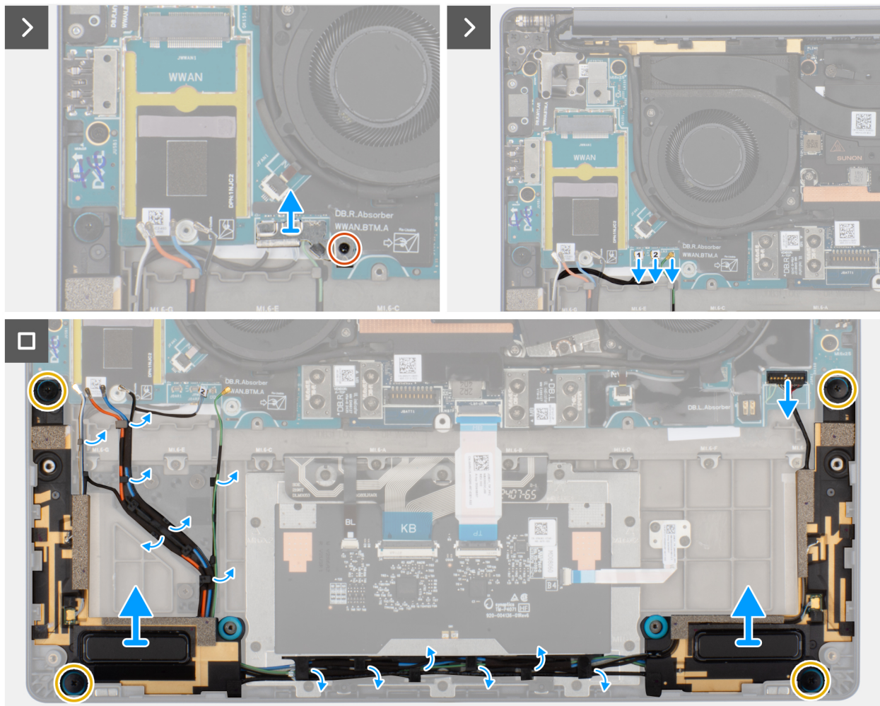
Afbeelding 36. De luidsprekers met antennes verwijderen (WWAN-configuratie)
