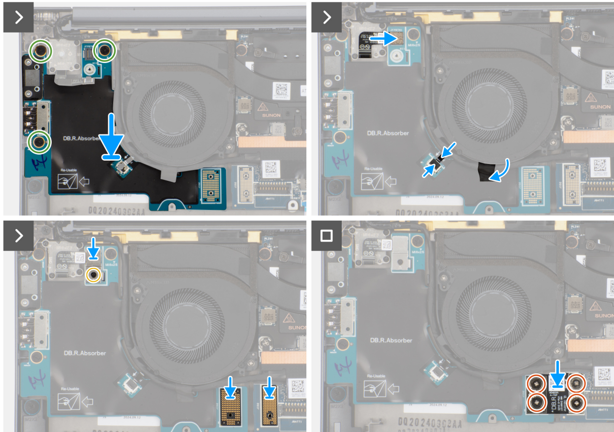
Afbeelding 46. De rechter I/O-kaart installeren (zonder WWAN-antennes)
