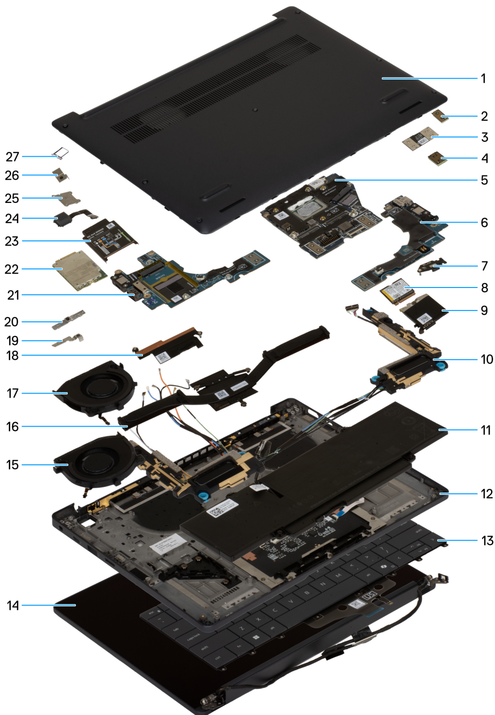
Afbeelding 11. Belangrijkste onderdelen van uw systeem/opengewerkte tekening
