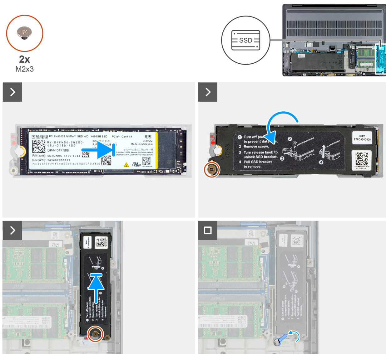
Figure 33. Installation du disque SSD M.2 2280 dans le logement 1 (SSD1)
