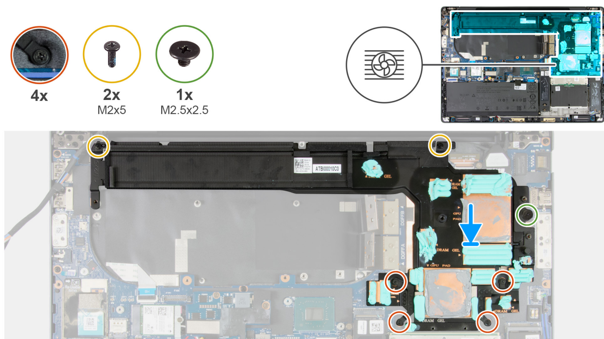
Figure 77. Installation du dissipateur de chaleur pour les ordinateurs équipés d'une carte graphique intégrée
