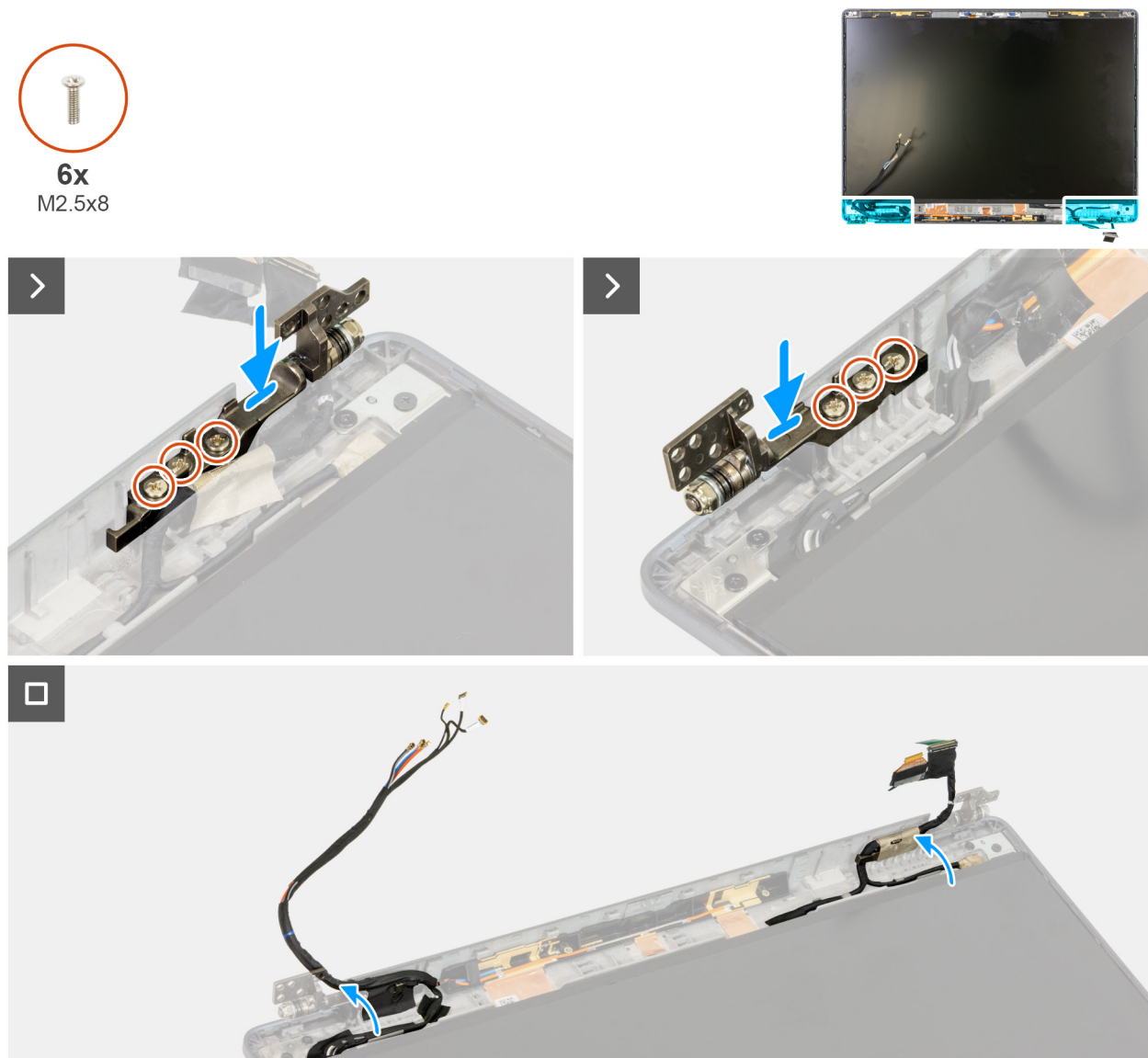
Figure 103. Installation des charnières d'écran
