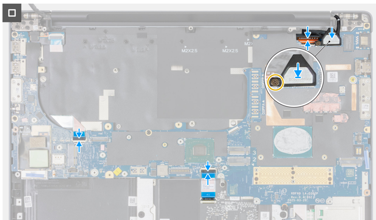
Figure 117. Installation de la carte système
