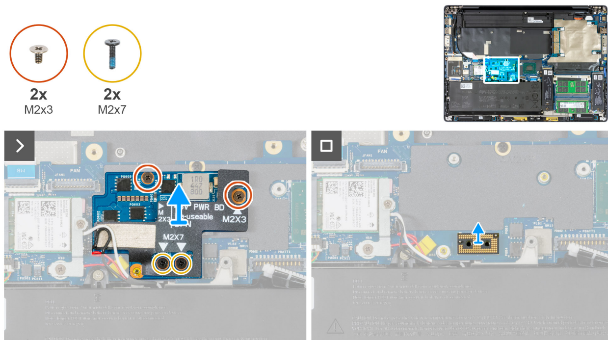
Figure 74. Retrait de la carte d'alimentation
