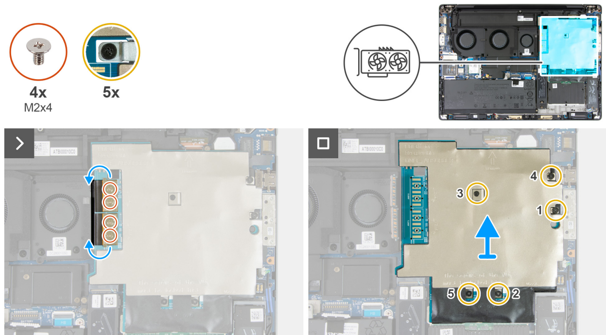
Figure 59. Retrait de la carte NPU
