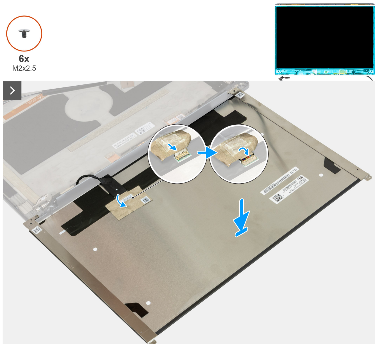
Figure 96. Installation du panneau d'écran pour les écrans tactiles
