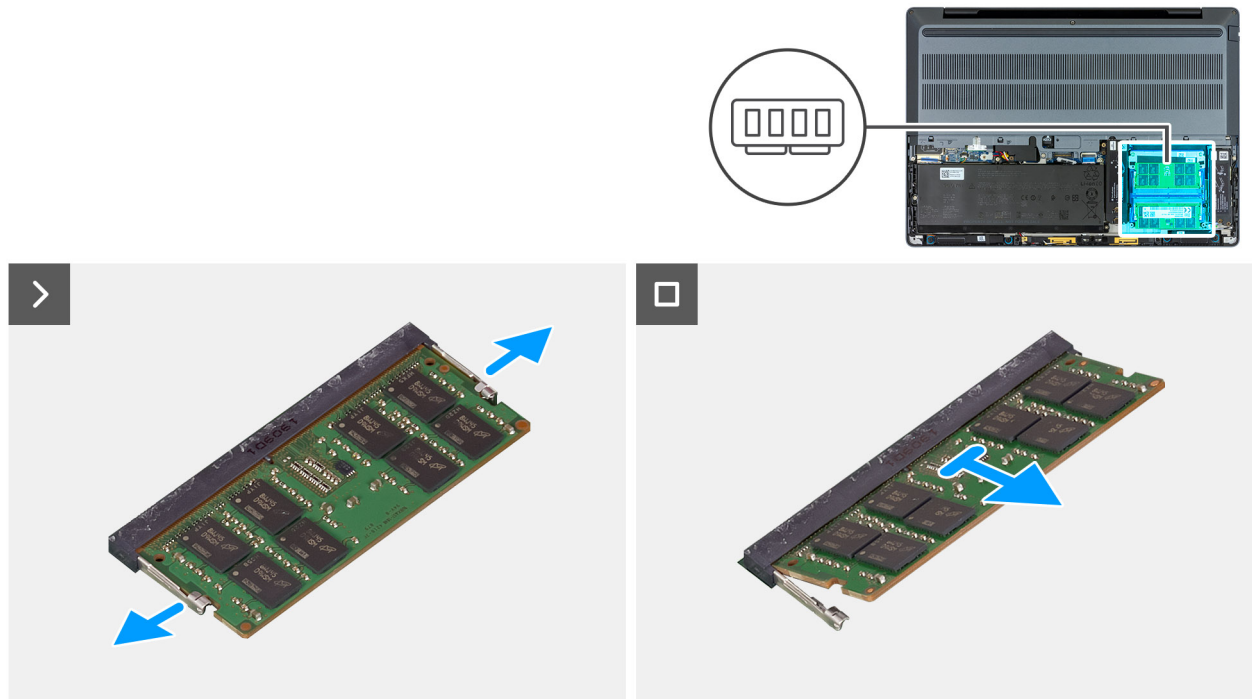
Figure 30. Retrait du module de mémoire
