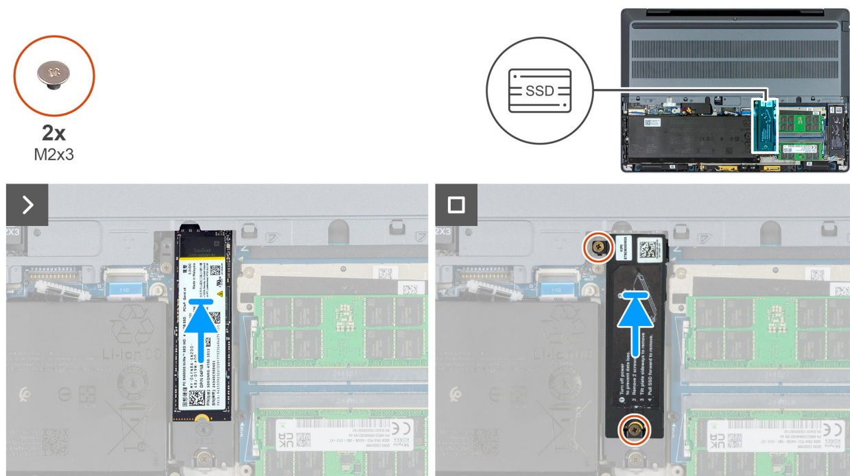
Figure 35. Installation du disque SSD M.2 2280 dans le logement 3 (SSD3)
