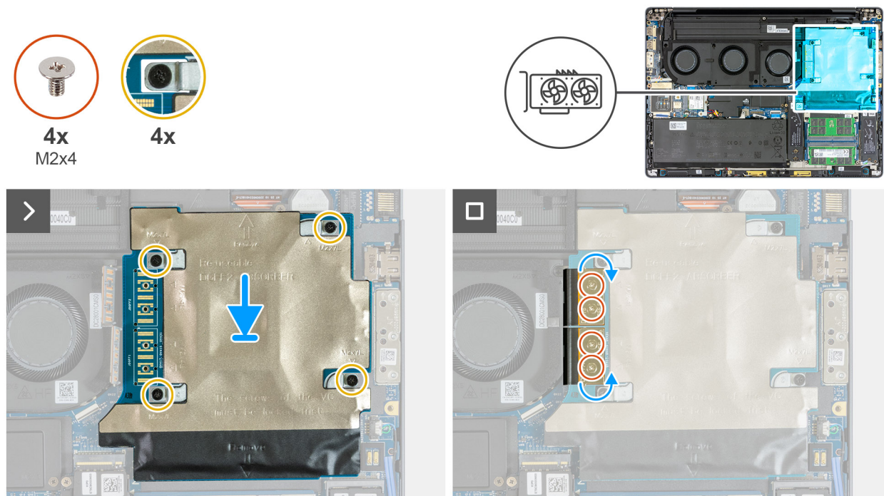
Figure 52. Installation de la carte GPU
