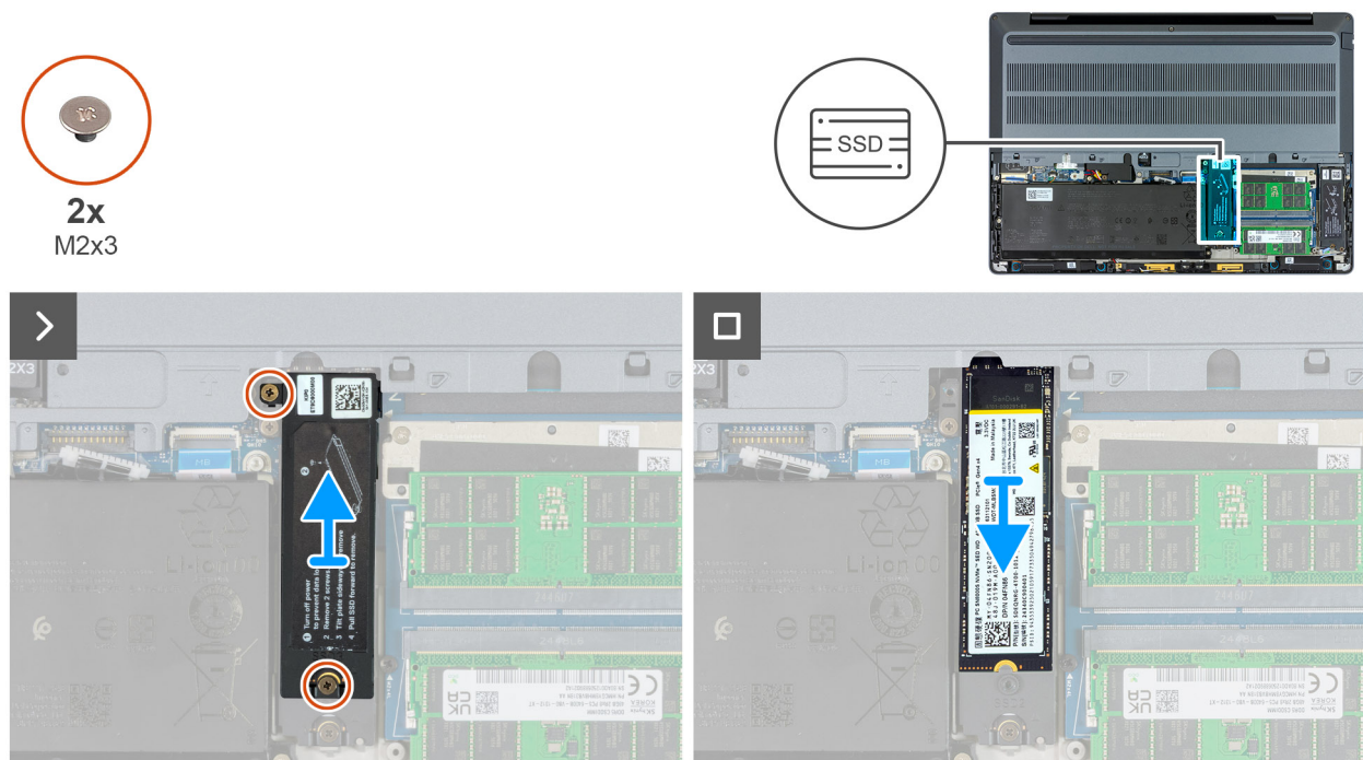
Figure 34. Retrait du disque SSD M.2 2280 du logement 3 (SSD3)
