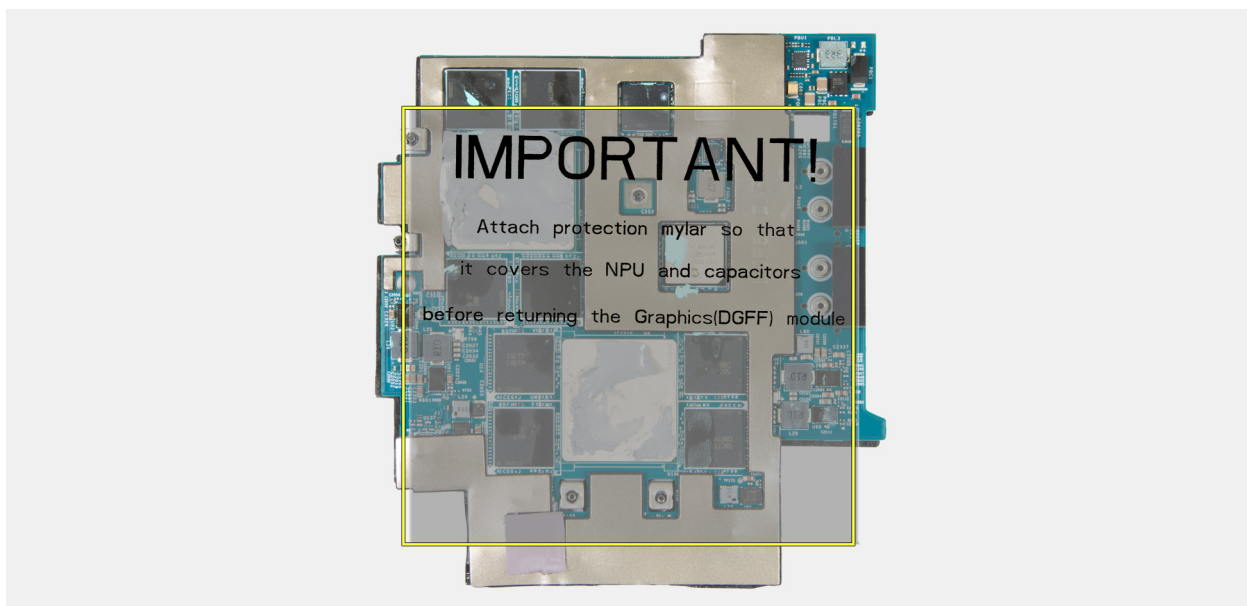
Figure 60. Collage du mylar de protection sur les zones de transfert de chaleur et la mémoire DRAM
