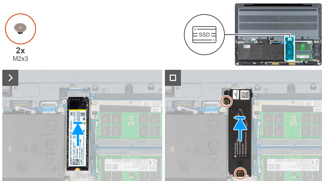
Figure 37. Installation du disque SSD M.2 2280 dans le logement 2 (SSD2)
