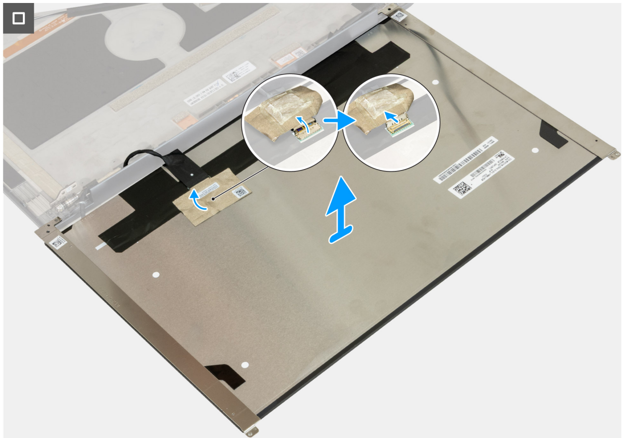
Figure 95. Retrait du panneau d'écran pour les écrans tactiles
