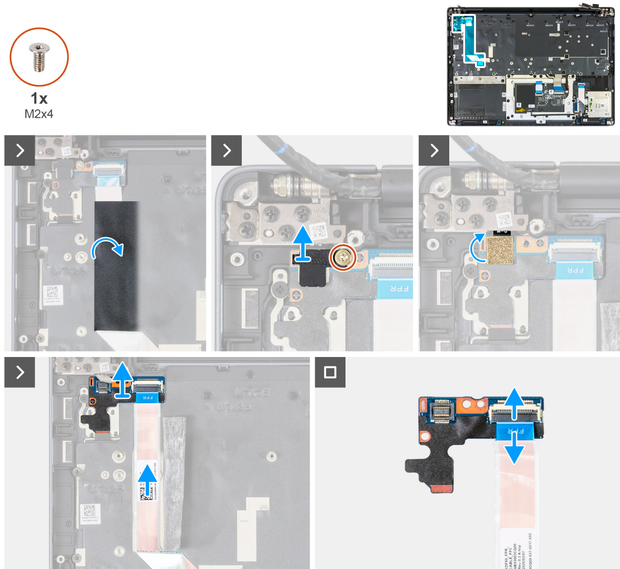
Figure 128. Retrait de la carte du bouton d'alimentation
