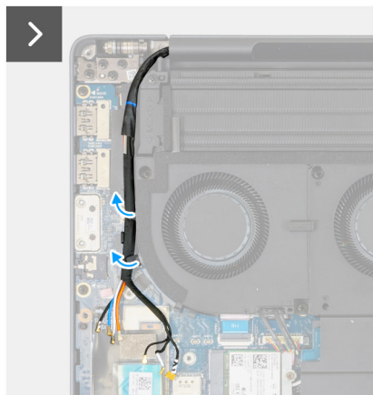
Figure 66. Retrait de l'assemblage d'écran
