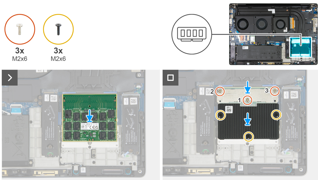
Figure 63. Installation du module CAMM (bicanal)
