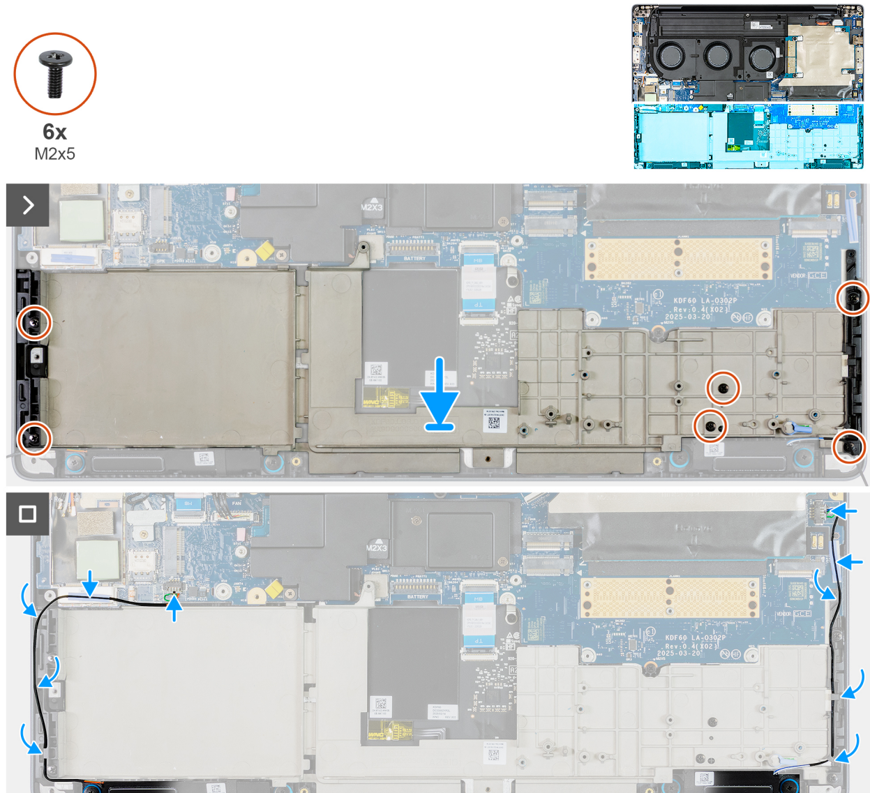
Figure 83. Installation du cadre interne
