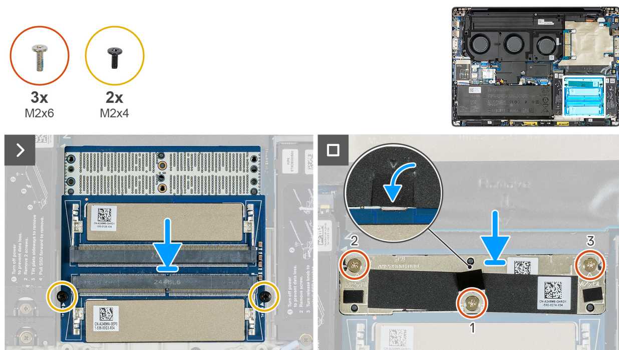
Figure 71. Installation de l'assemblage d'écran
