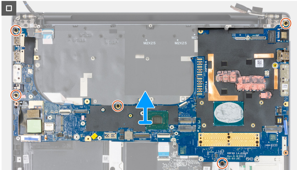
Figure 113. Retrait de la carte système
