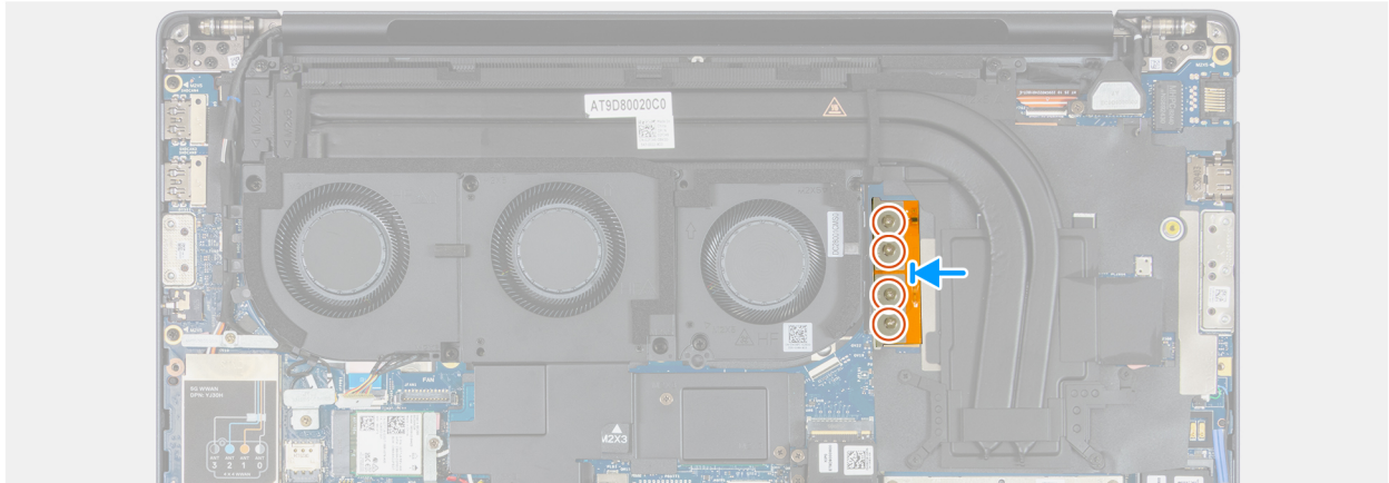
Figure 54. Installation du connecteur de faisceau FPC intégré
