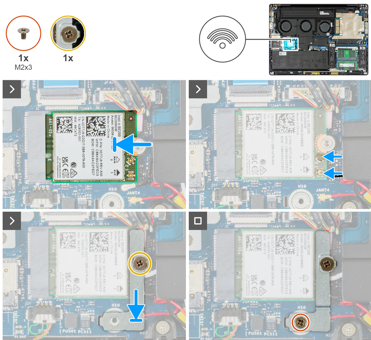
Figure 45. Installation de la carte WLAN
