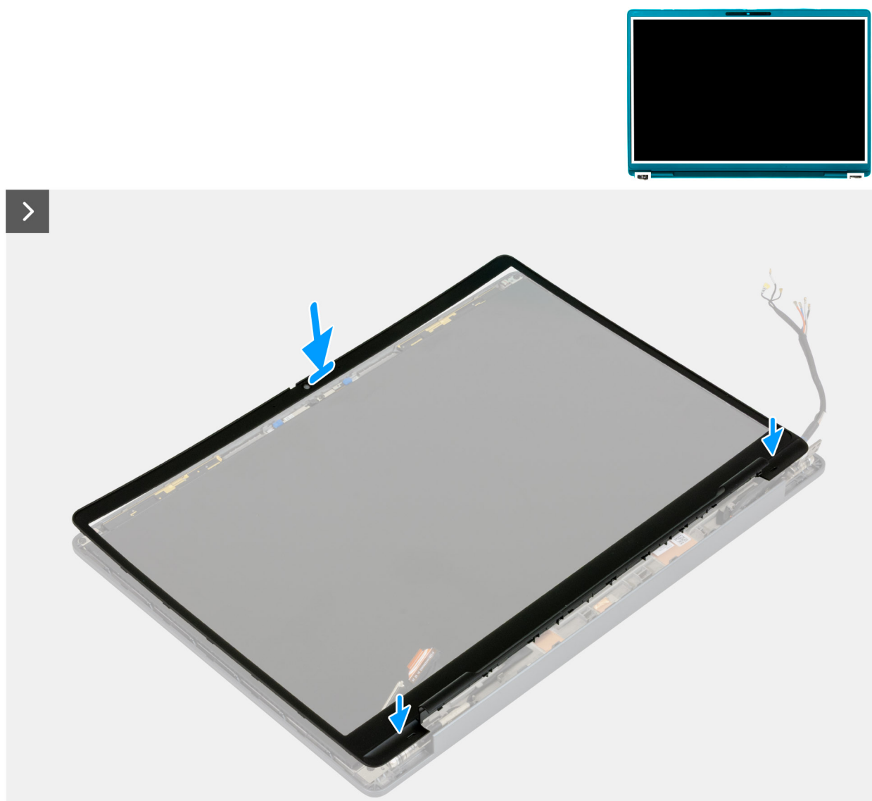
Figure 92. Installation de la bordure d'écran
