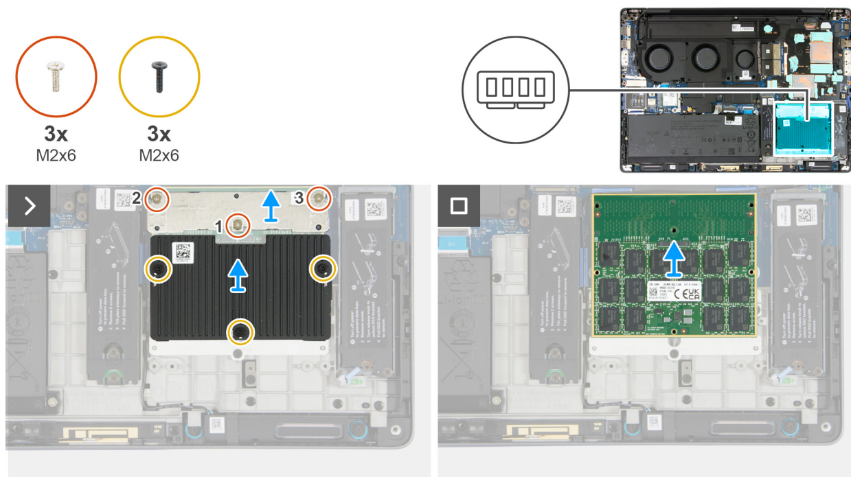
Figure 62. Retrait du module CAMM (bicanal)
