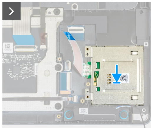
Figure 125. Installation du lecteur de carte à puce
