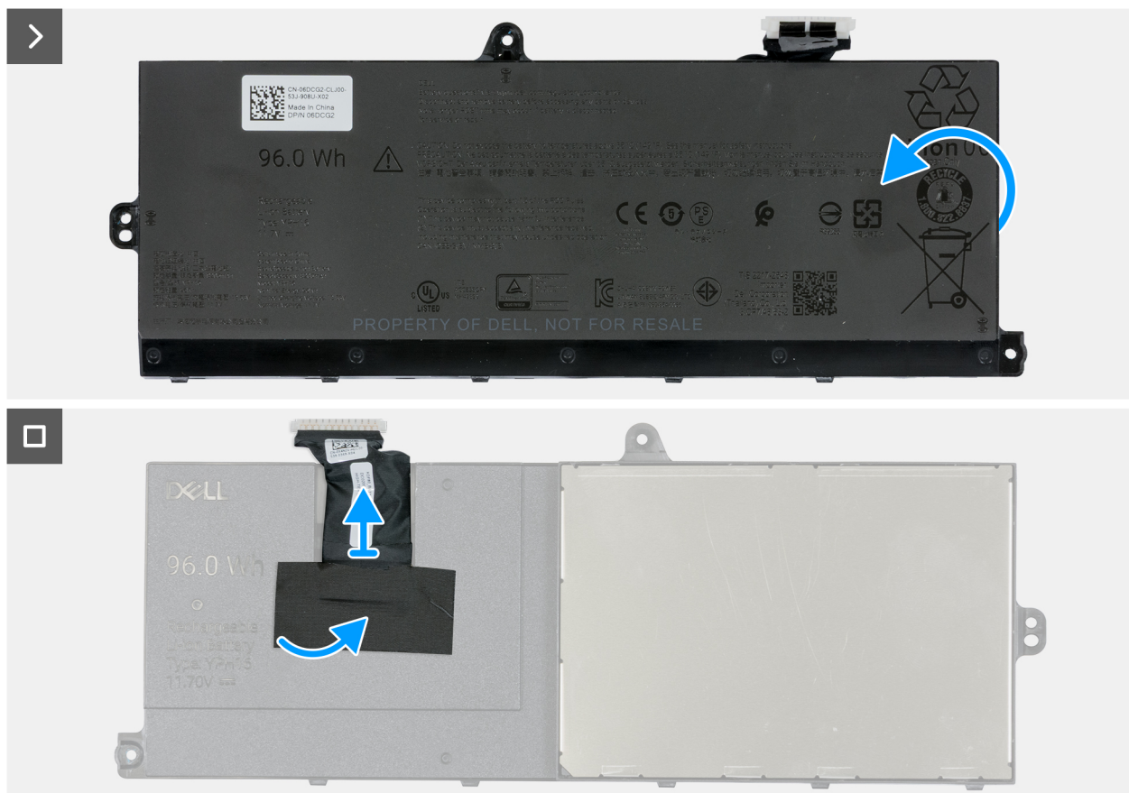
Figure 41. Retrait du câble de la batterie de la batterie
