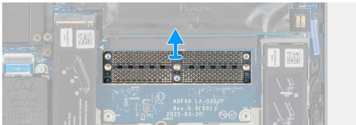
Figure 72. Retrait du connecteur de mémoire
