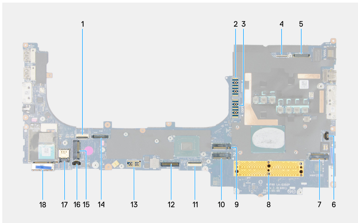
Figure 115. Composants de la carte système
