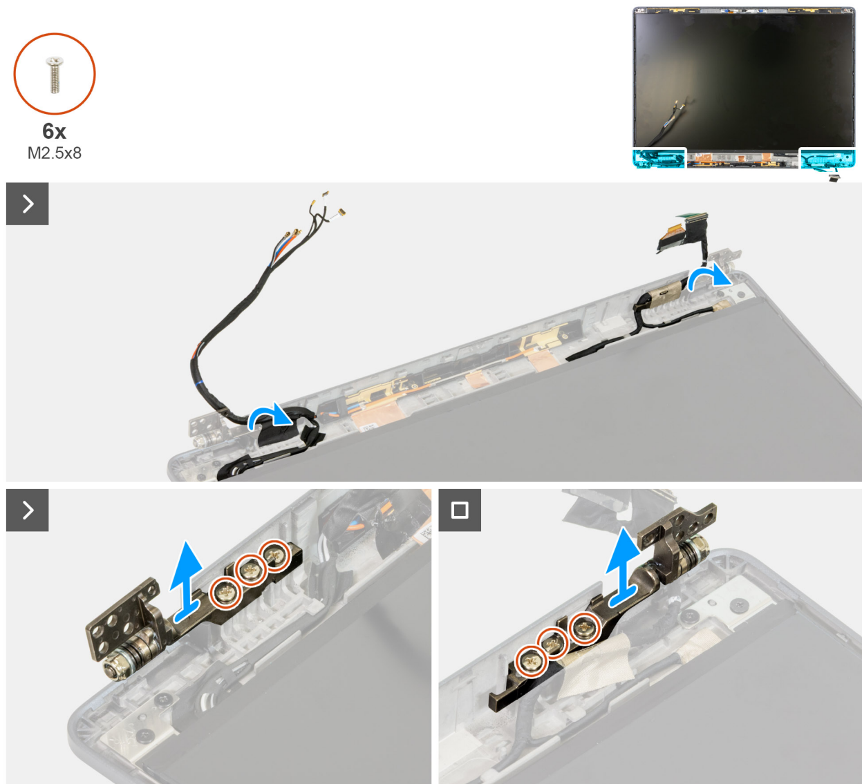
Figure 102. Retrait des charnières d'écran
