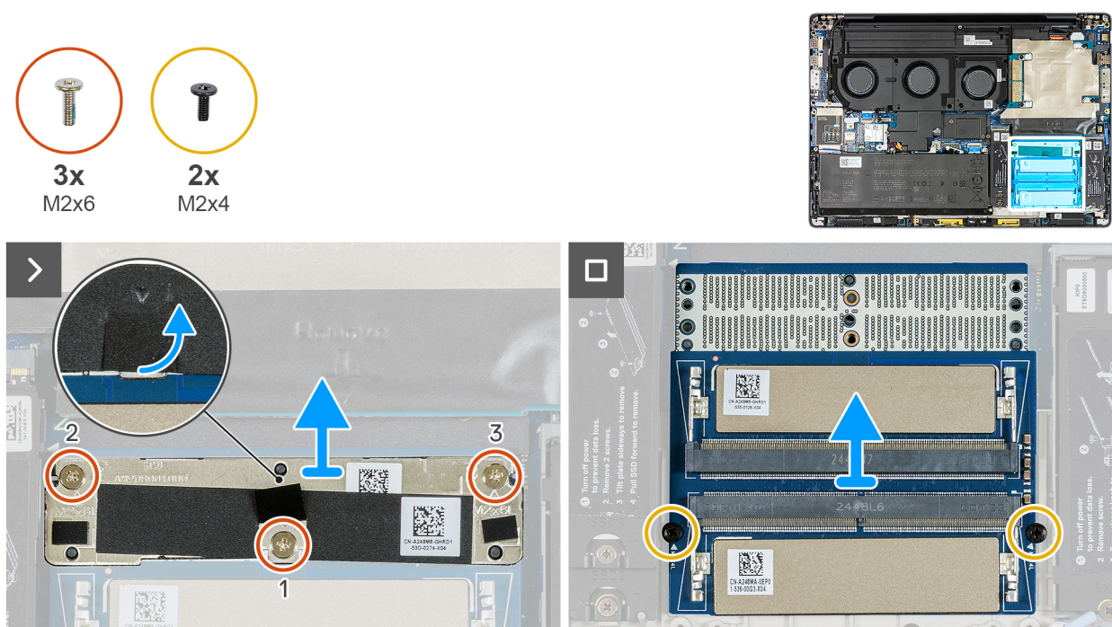
Figure 70. Retrait de la carte intercalaire de mémoire
