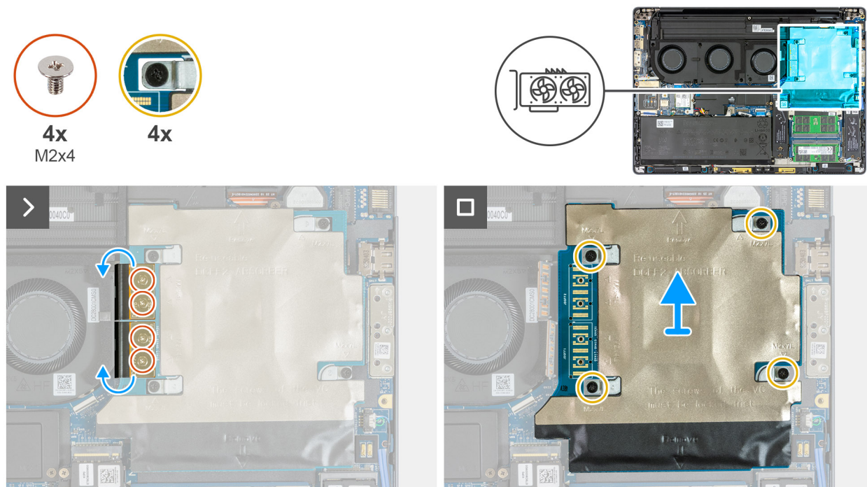
Figure 50. Retrait de la carte GPU
