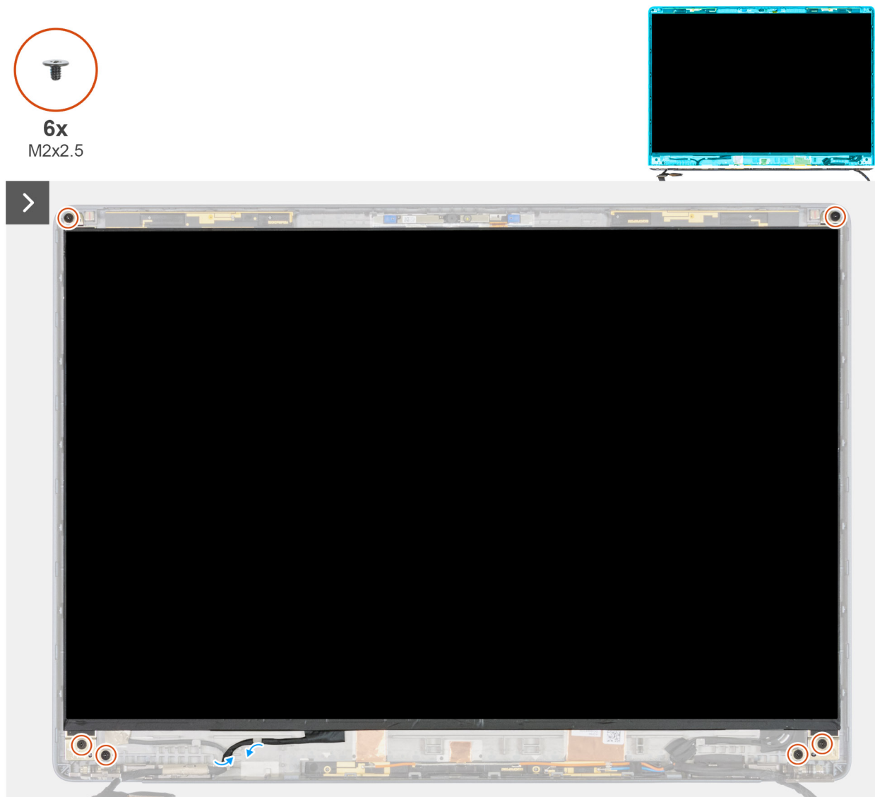
Figure 98. Retrait du panneau d'écran pour les écrans non tactiles
