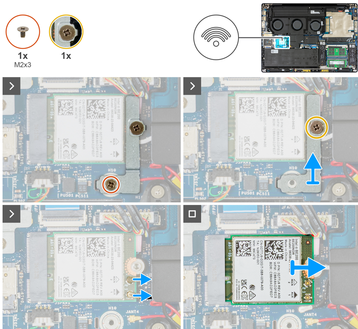
Figure 44. Retrait de la carte WLAN
