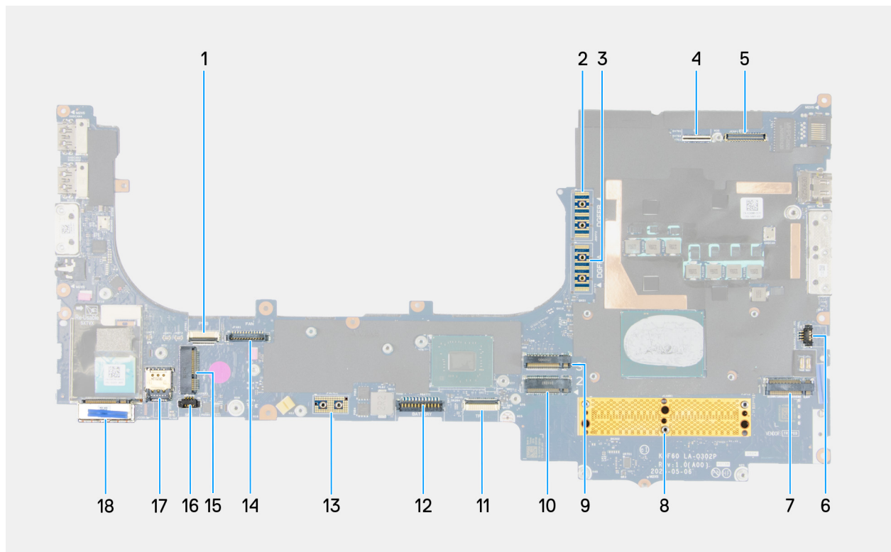
Figure 111. Composants de la carte système
