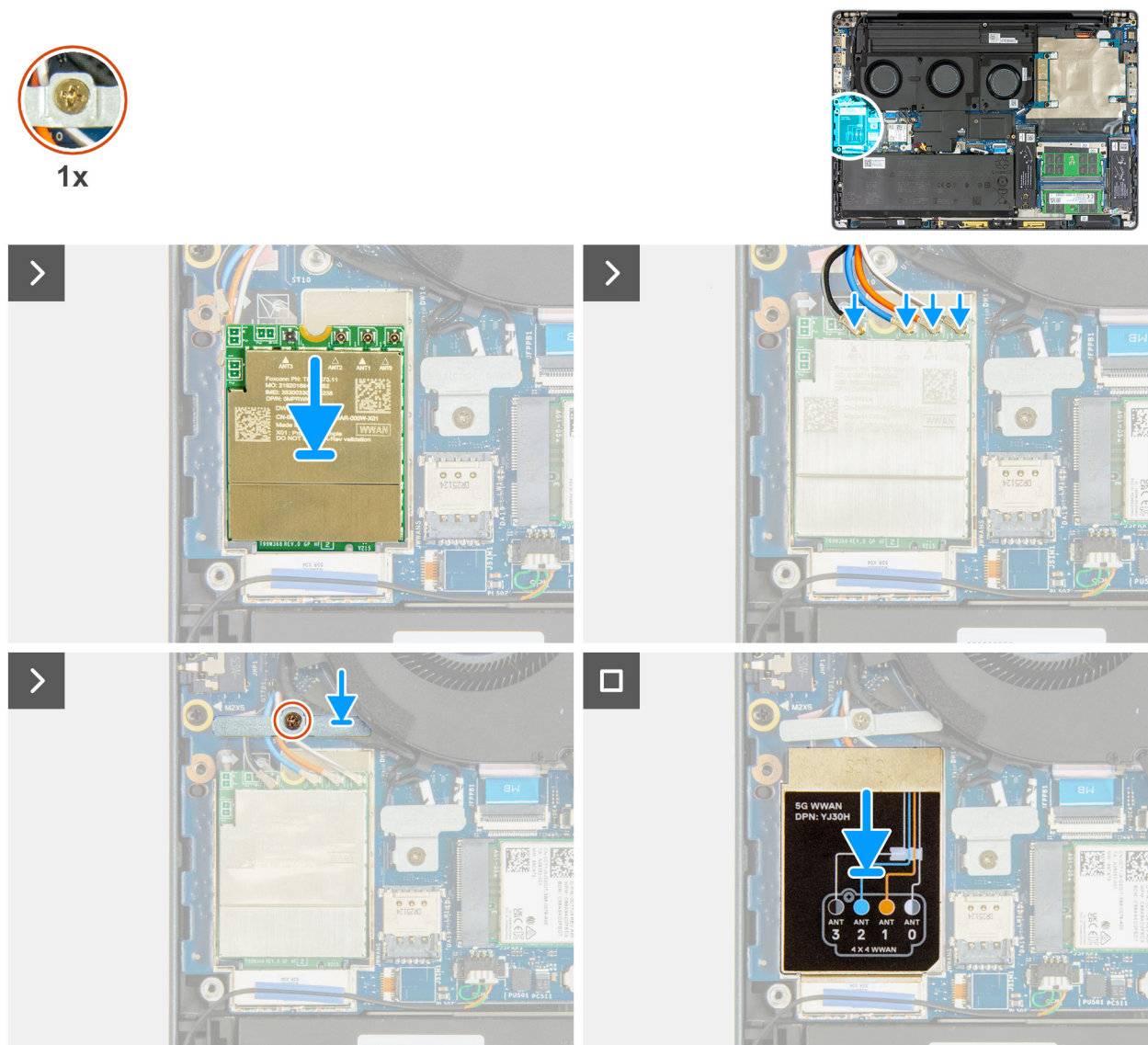
Figure 49. Installation de la carte WWAN
