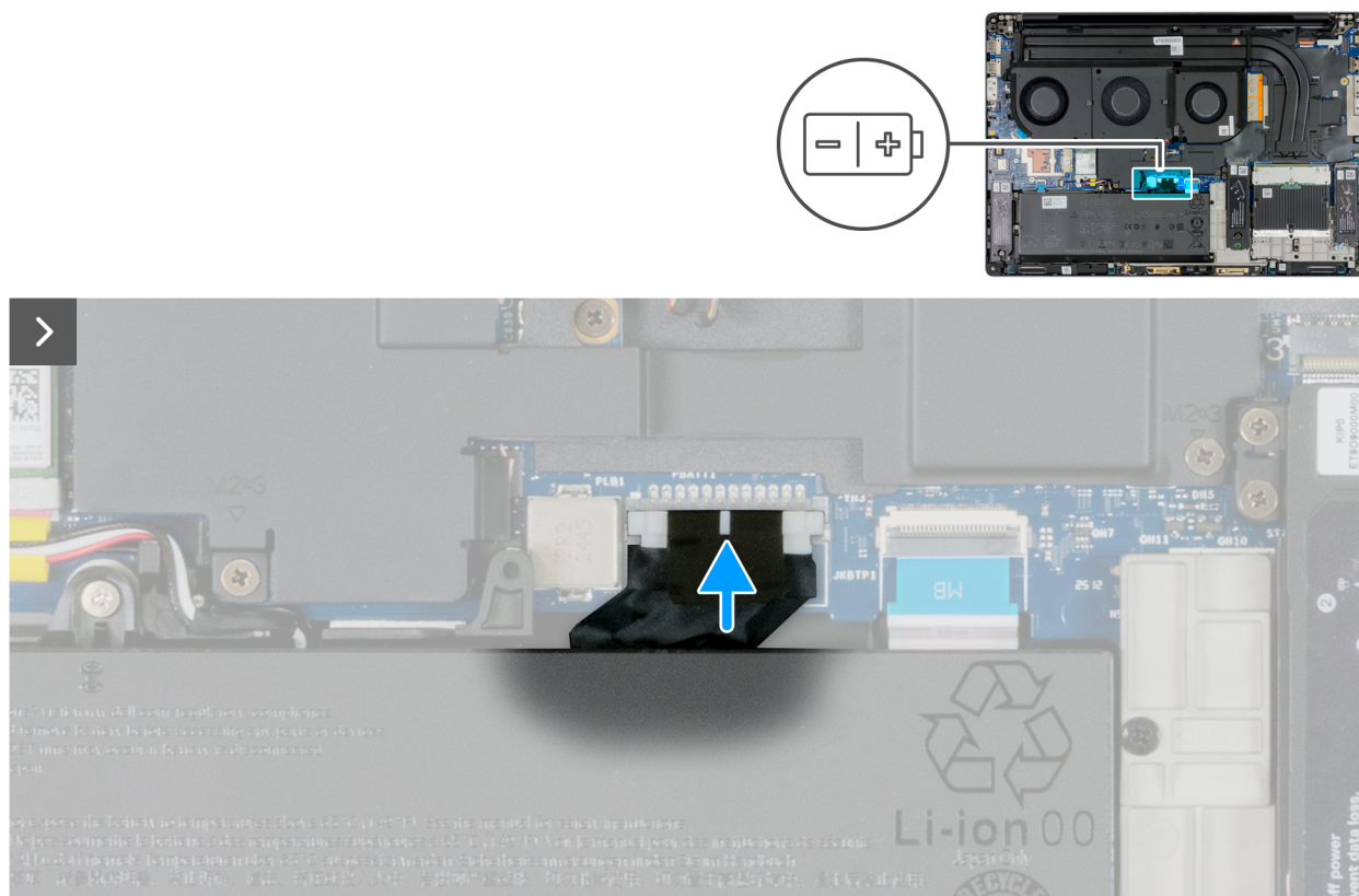
Figure 27. Connexion du câble de la batterie
