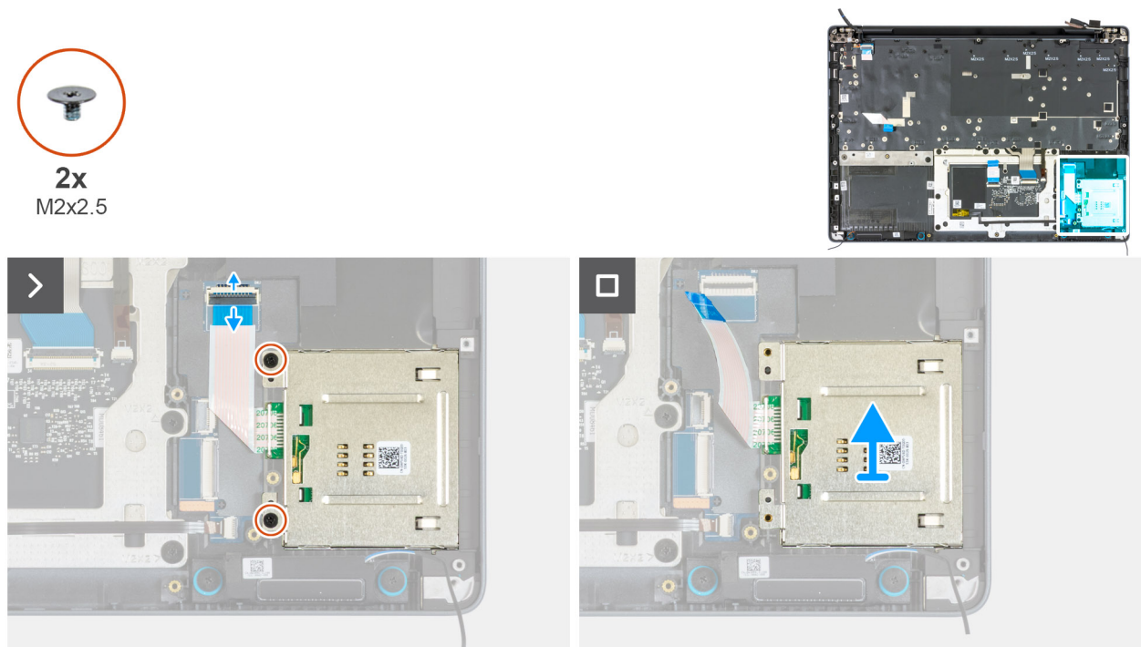
Figure 124. Retrait du lecteur de carte à puce
