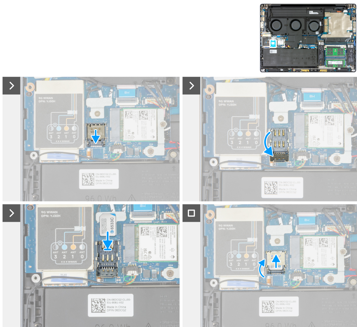
Figure 47. Installation de la carte SIM
