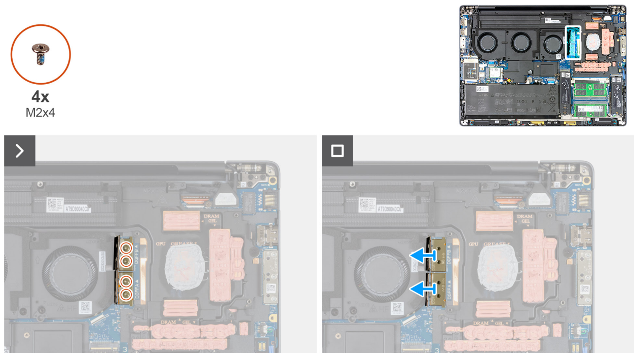
Figure 55. Retrait du connecteur de faisceau de circuit imprimé flexible séparé
