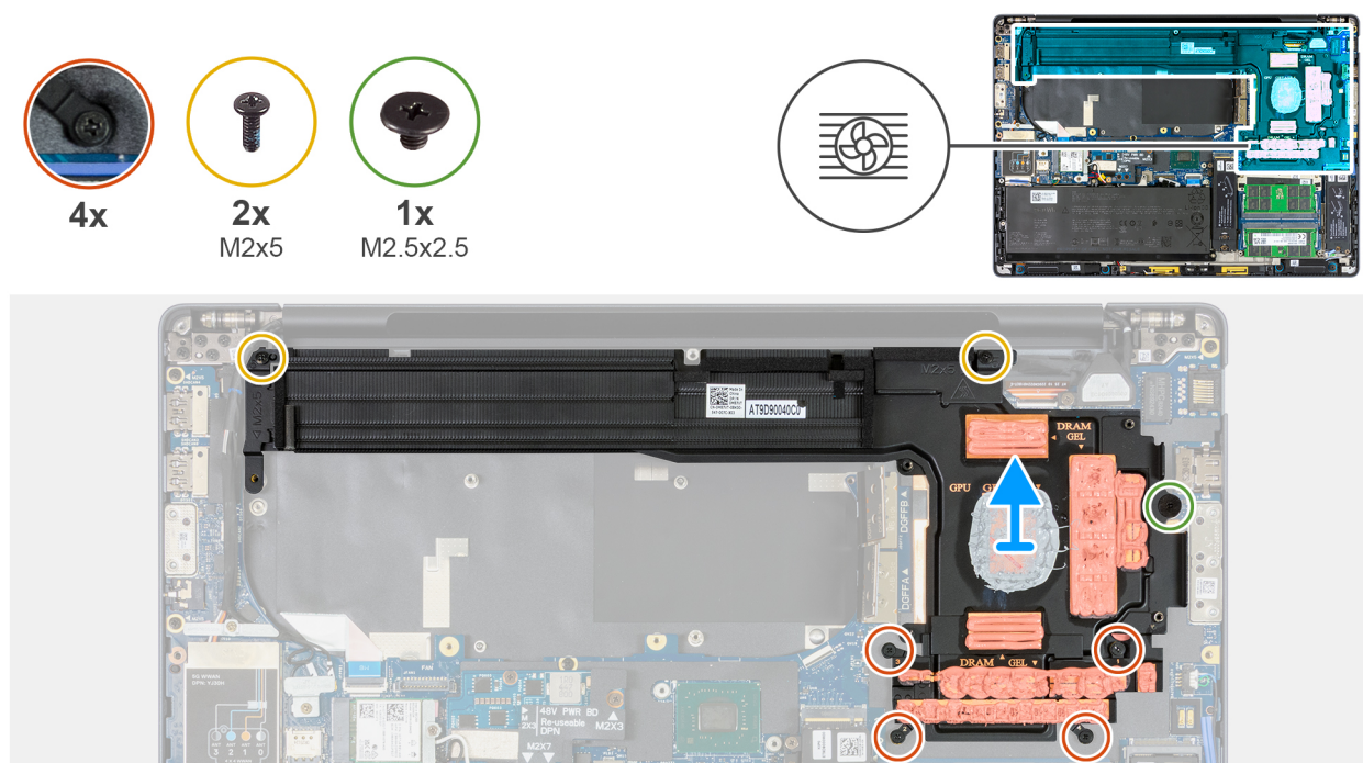
Figure 78. Retrait du dissipateur de chaleur pour les ordinateurs équipés d'une carte graphique séparée
