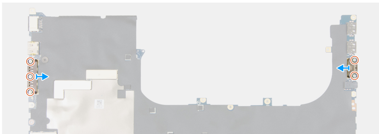
Figure 118. Retrait du module de connecteur USB-C
