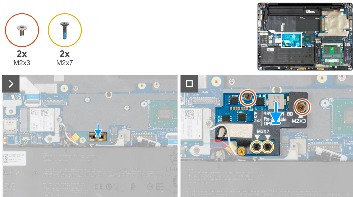
Figure 75. Installation de la carte d'alimentation
