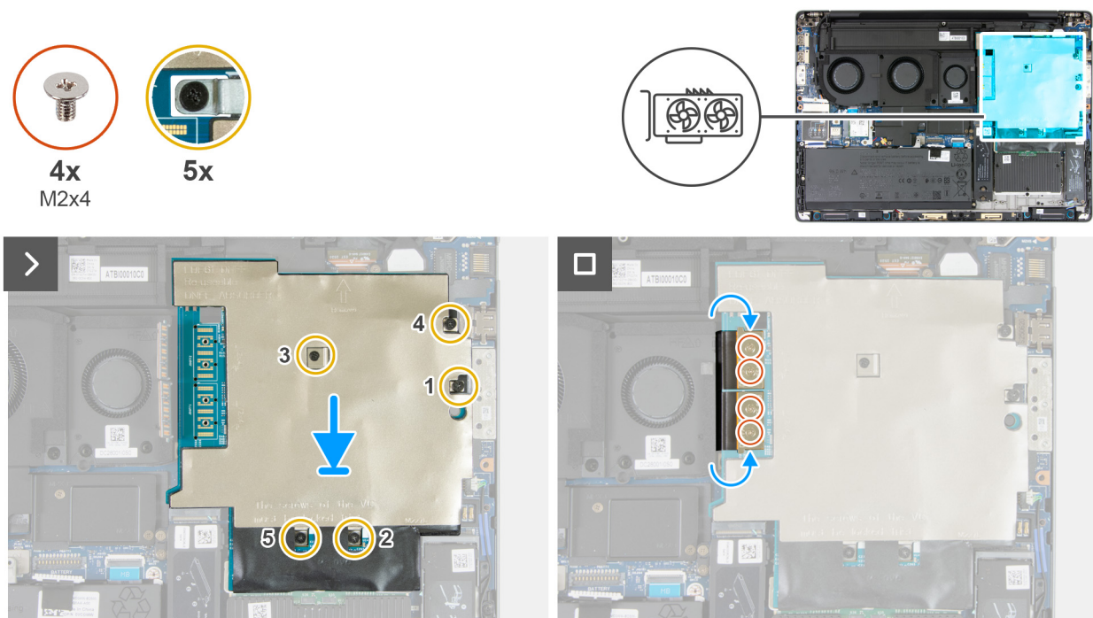
Figure 61. Installation de la carte NPU
