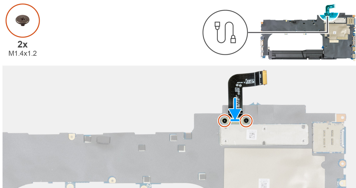
Figure 121. Installation du câble de la carte USH
