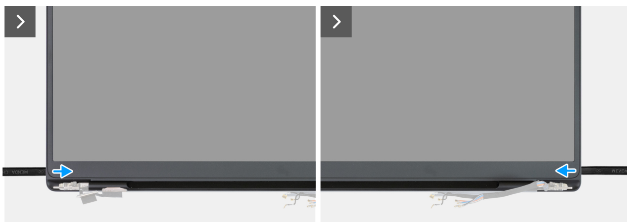
Figure 90. Retrait de la bordure d'écran
