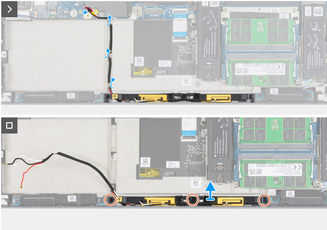
Figure 80. Retrait du module d'antenne WLAN
