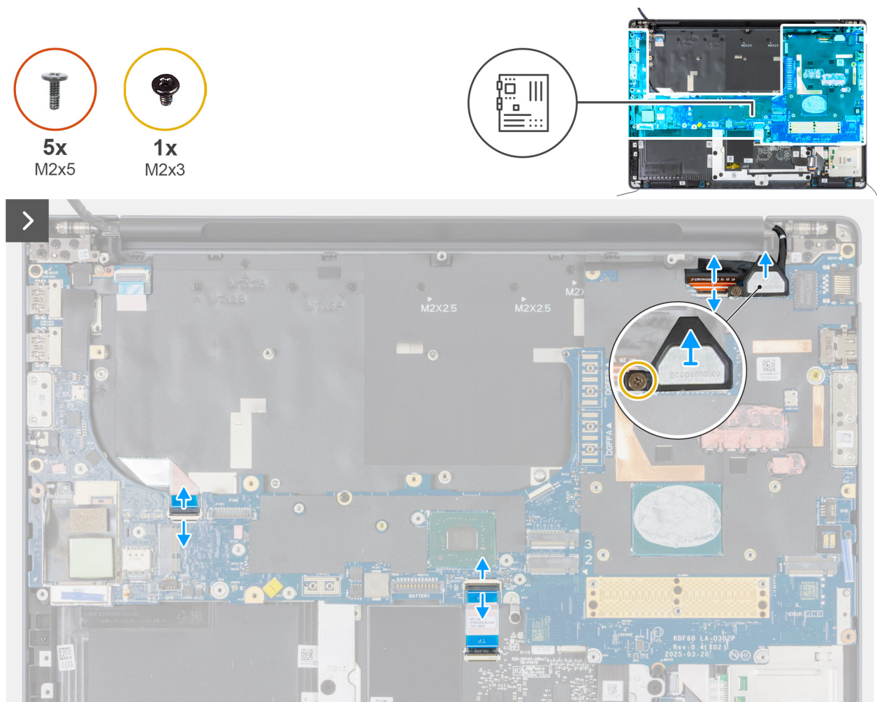
Figure 112. Retrait de la carte système
