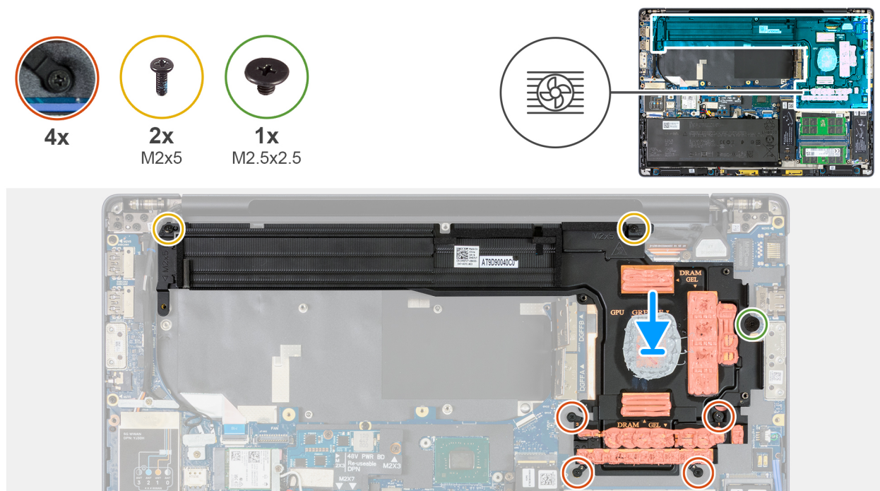
Figure 79. Installation du dissipateur de chaleur pour les ordinateurs expédiés avec une carte graphique séparée
