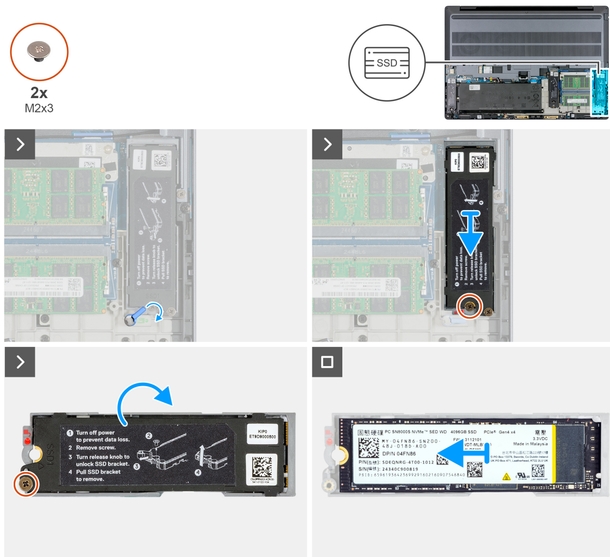
Figure 32. Retrait du disque SSD M.2 2280 du logement 1 (SSD1)
