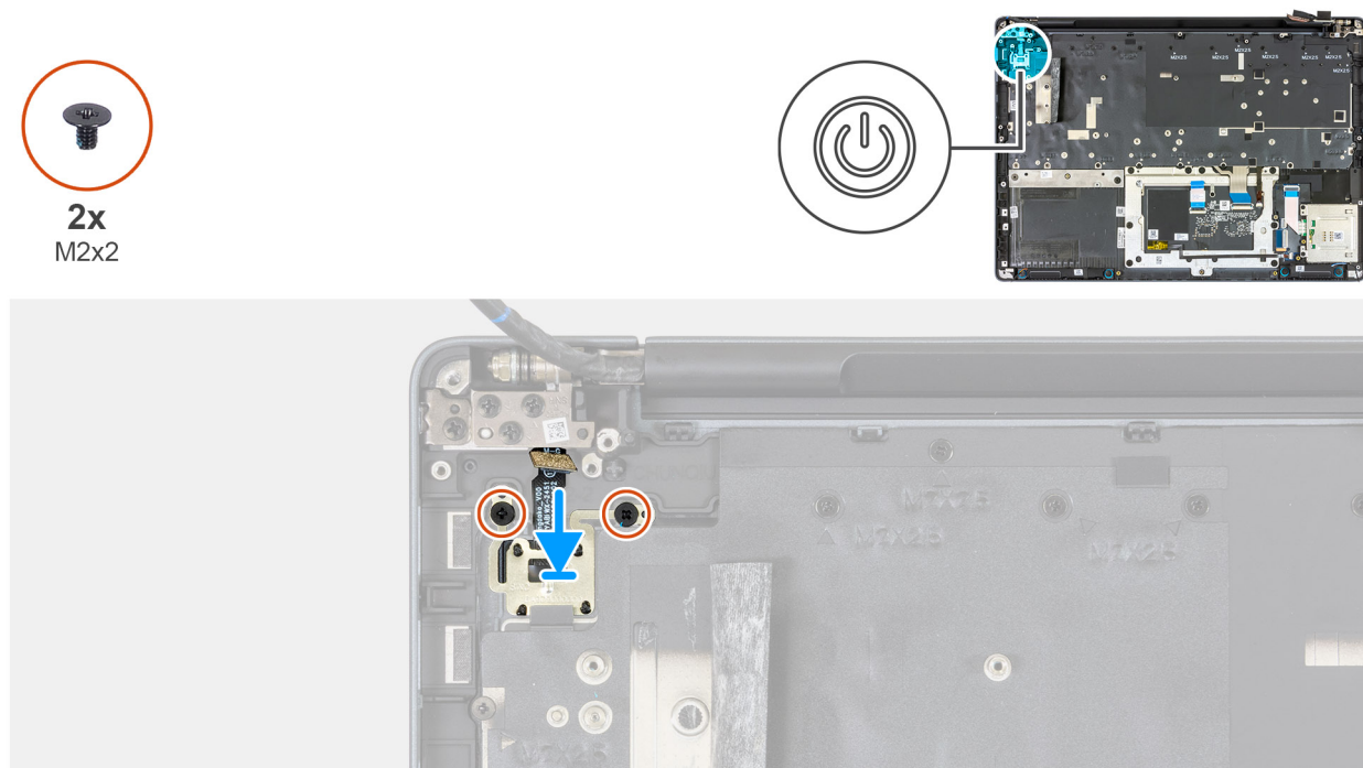
Figure 131. Installation du bouton d'alimentation
