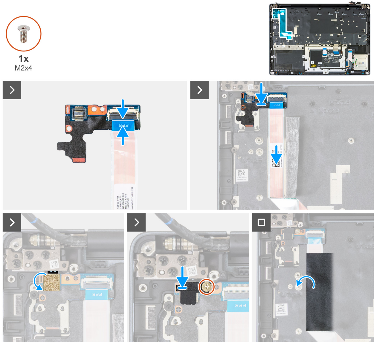
Figure 129. Installation de la carte du bouton d'alimentation
