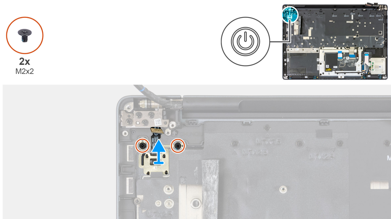
Figure 130. Retrait du bouton d'alimentation
