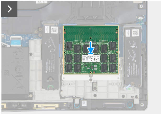
Afbeelding 63. De CAMM-module installeren (dual-channel)
