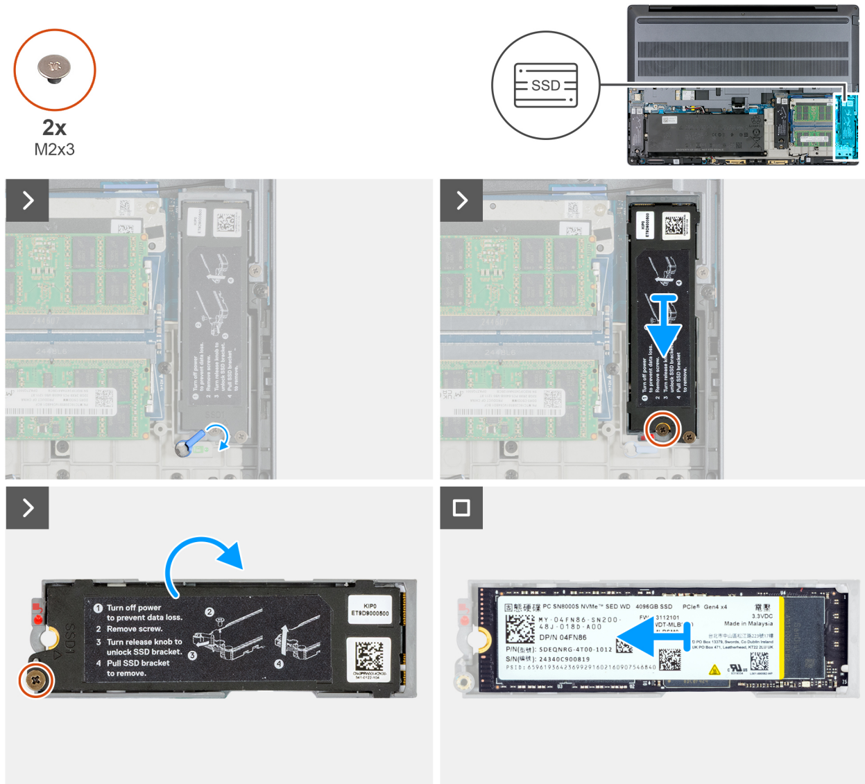
Afbeelding 32. De M.2 2280 SSD verwijderen uit slot 1 (SSD1)
