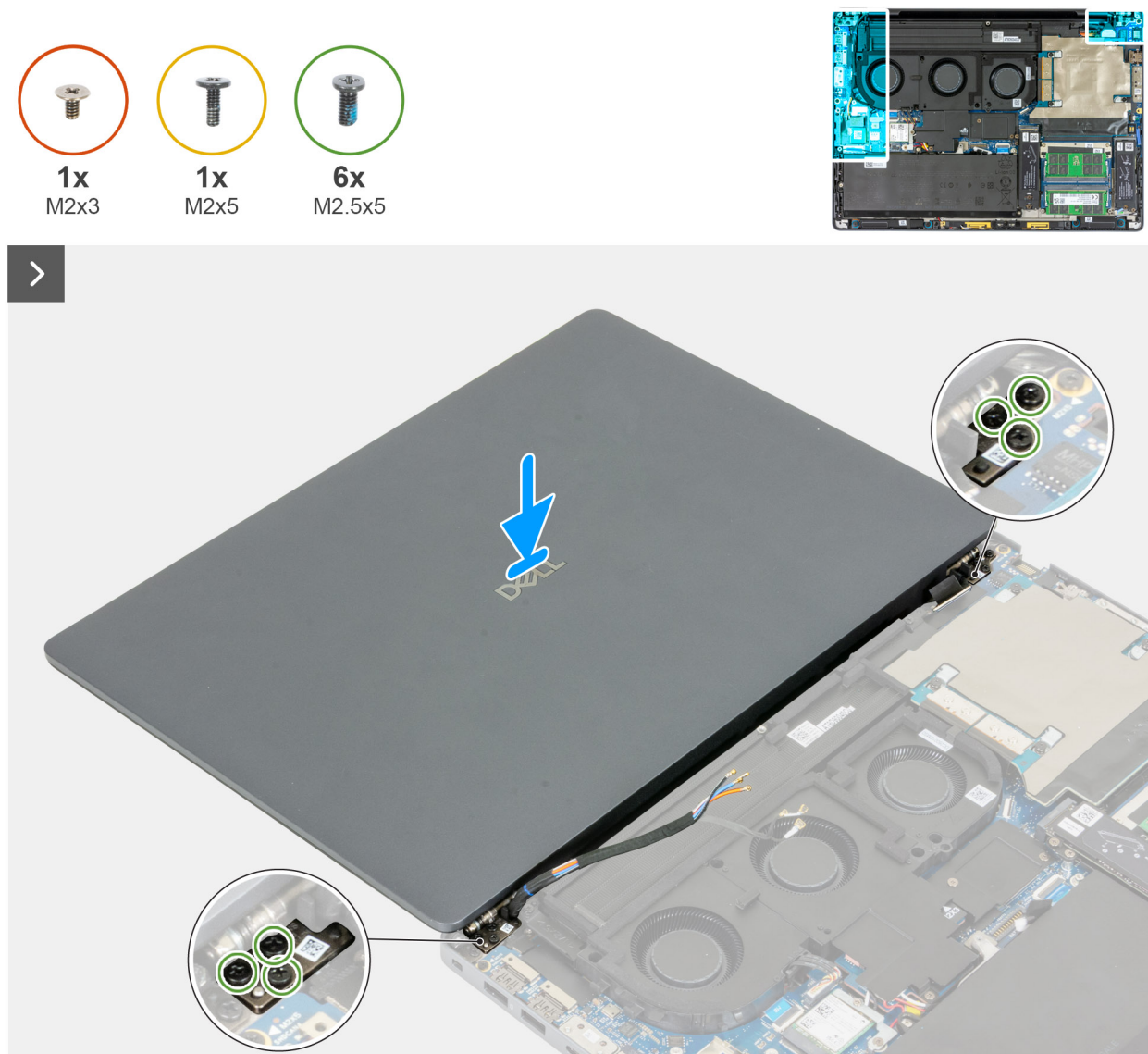
Afbeelding 68. De beeldschermeenheid plaatsen
