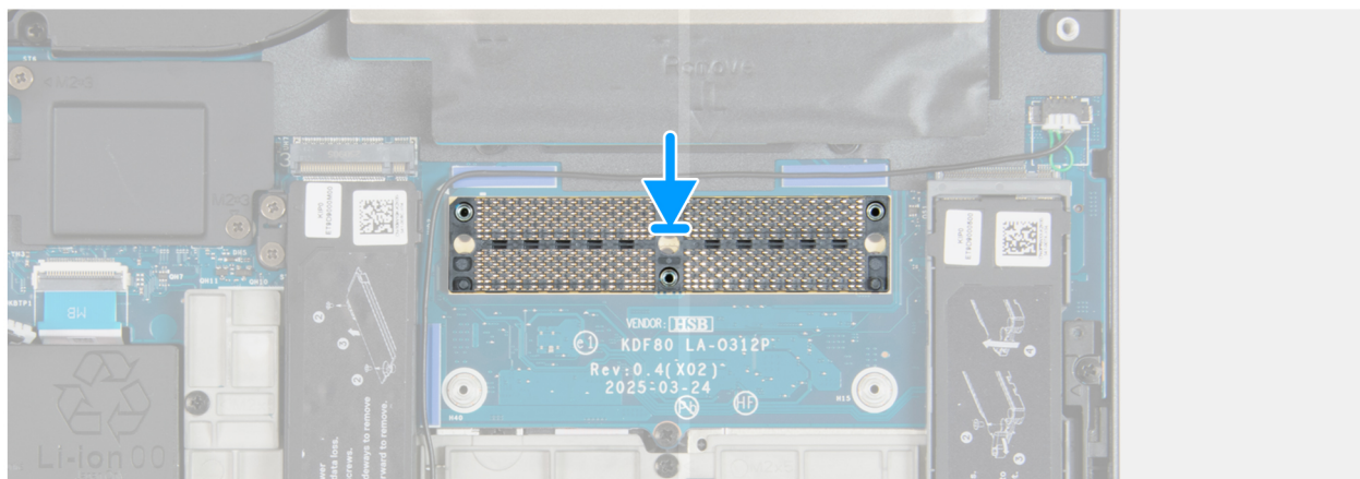
Afbeelding 73. De geheugenconnector plaatsen
