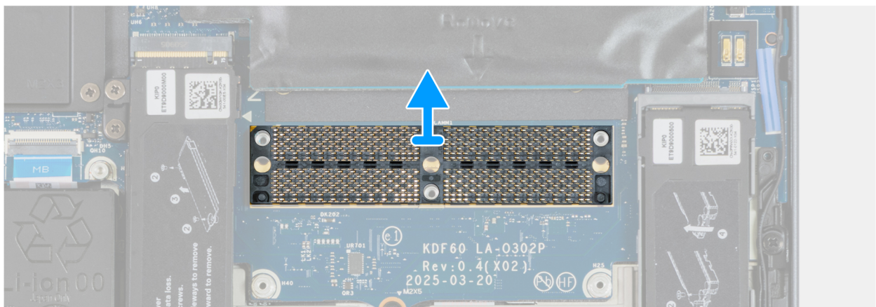
Afbeelding 72. De geheugenconnector verwijderen
