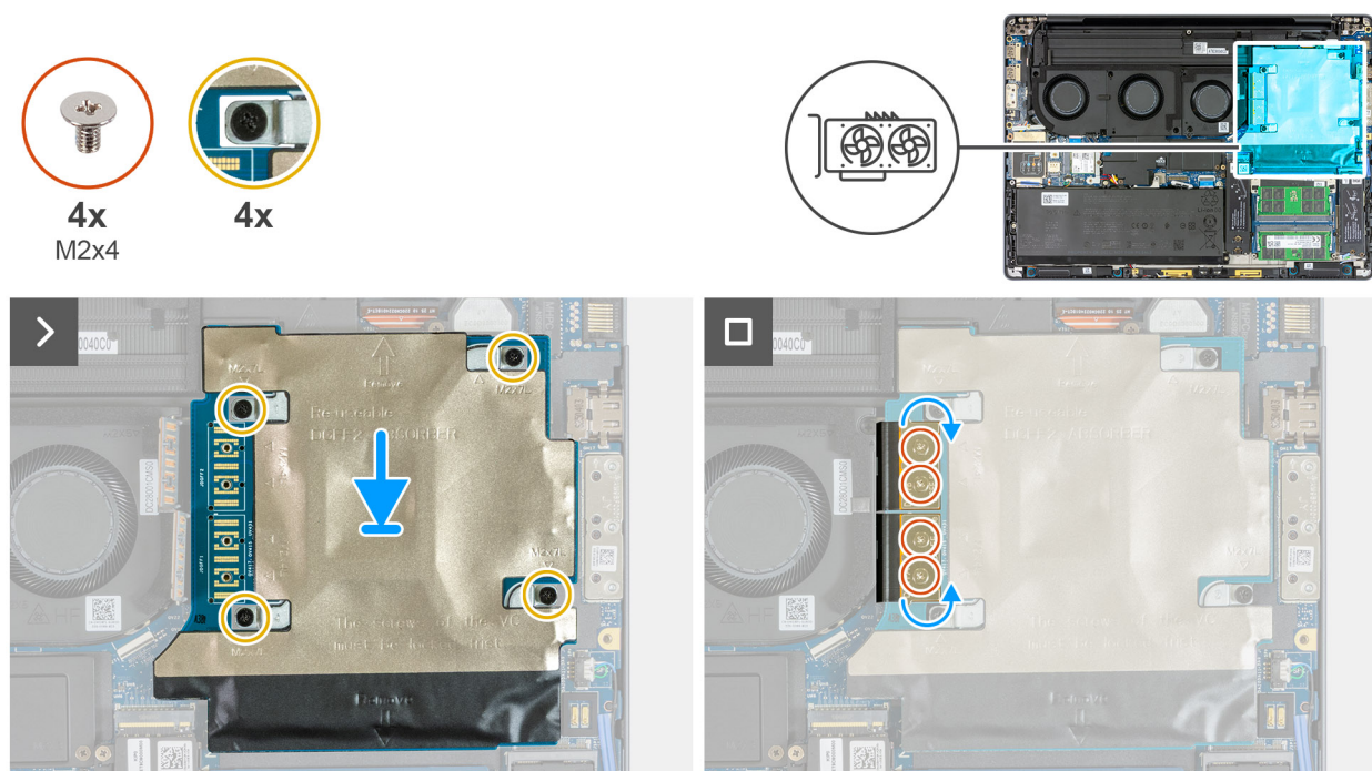
Afbeelding 52. De GPU-kaart installeren
