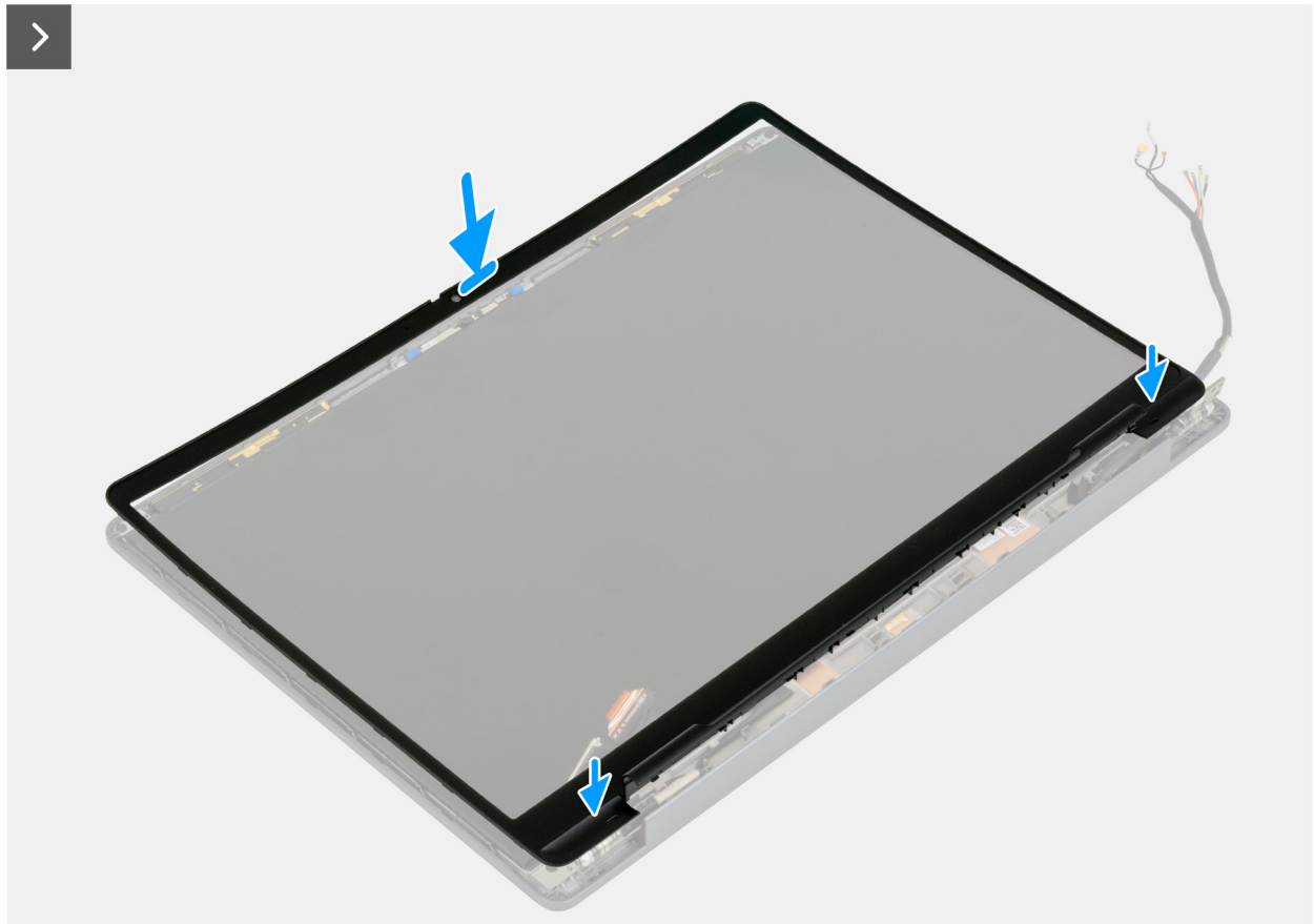
Afbeelding 92. De beeldschermbezel installeren
