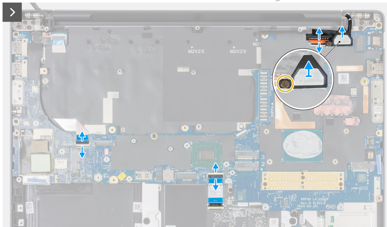
Afbeelding 112. De systeemkaart verwijderen
