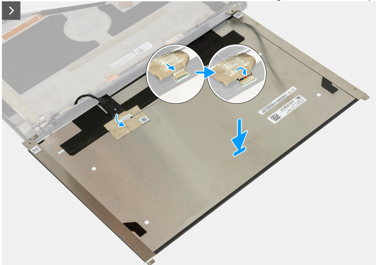
Afbeelding 100. Het beeldschermpaneel installeren voor beeldschermen zonder touchscreen
