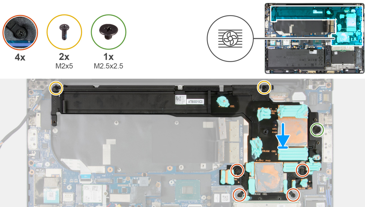
Afbeelding 77. De koelplaat installeren voor computers die met een geïntegreerde grafische kaart worden geleverd
