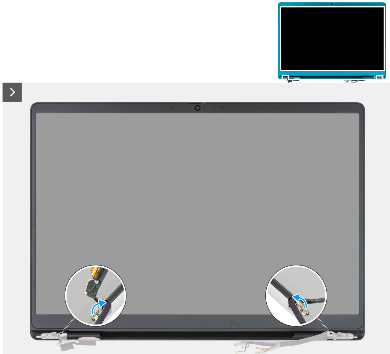
Afbeelding 86. De beeldschermbezel verwijderen
