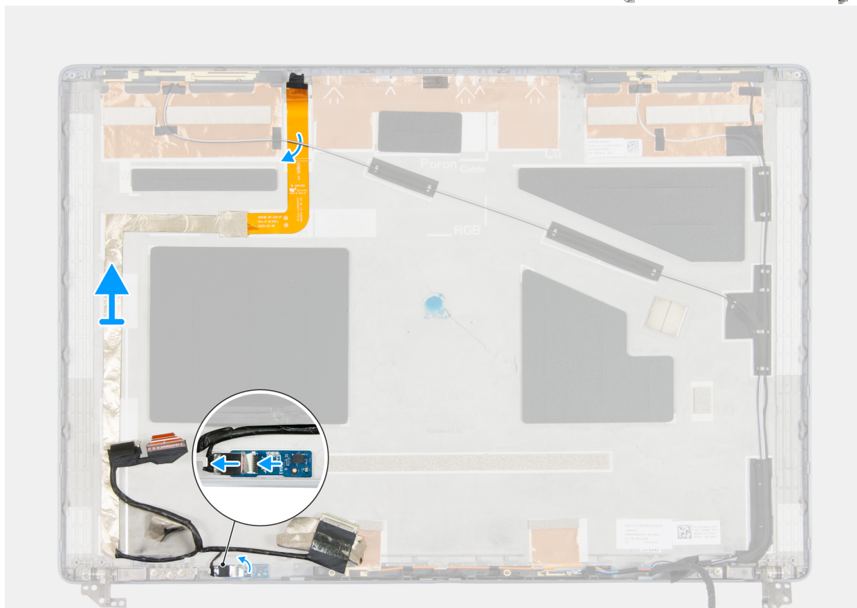
Afbeelding 107. De beeldschermkabel verwijderen
