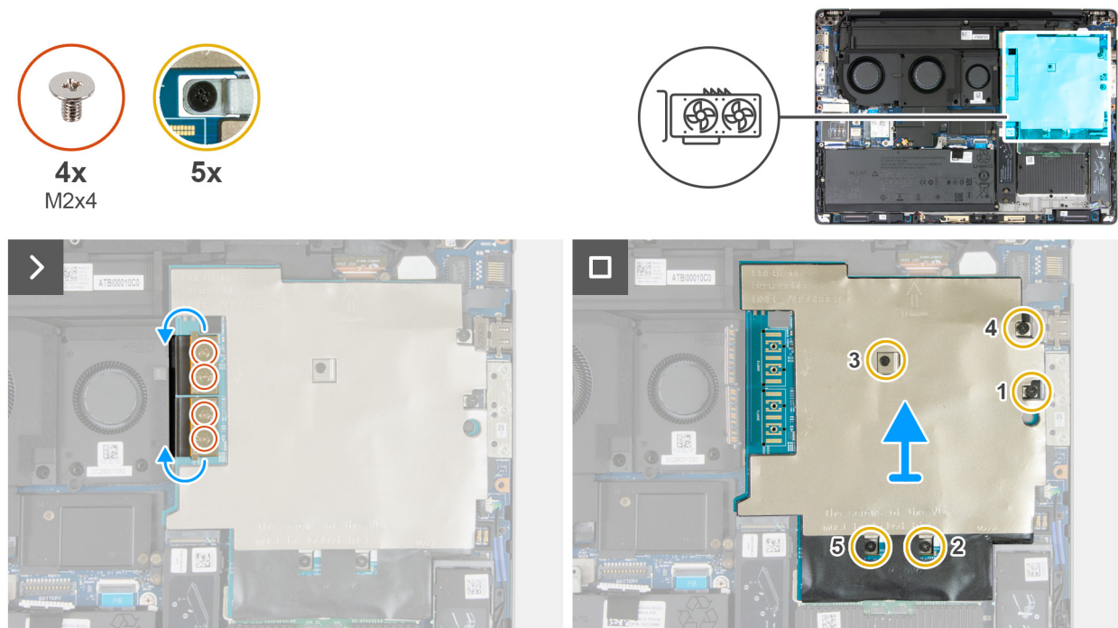
Afbeelding 59. De NPU-kaart verwijderen
