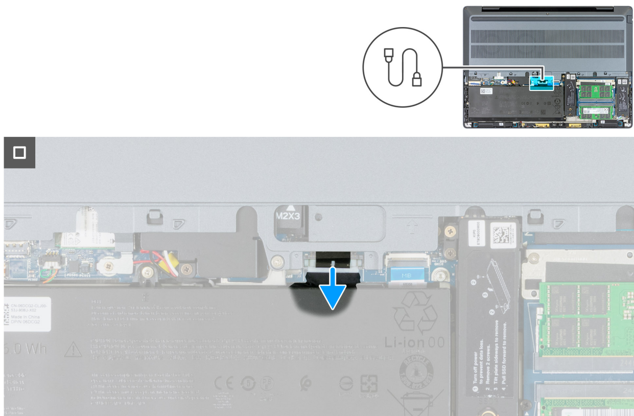
Afbeelding 20. De batterijkabel loskoppelen
