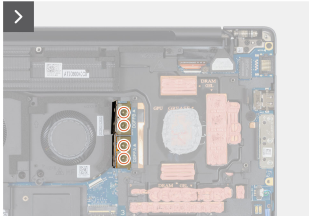
Afbeelding 55. De discrete FPC-balkconnector verwijderen
