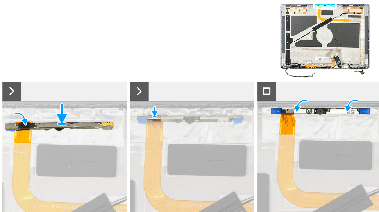
Afbeelding 105. De cameramodule installeren
