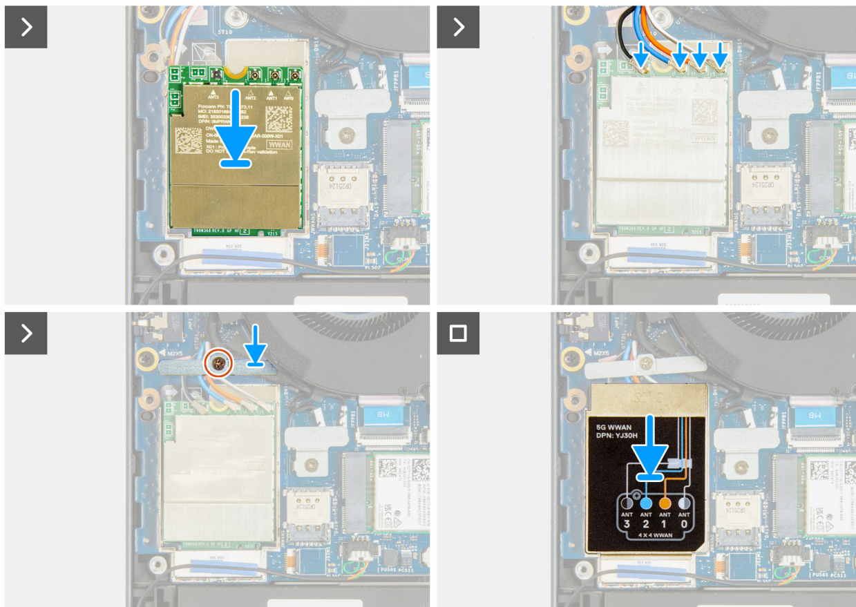
Afbeelding 49. De WWAN-kaart installeren
