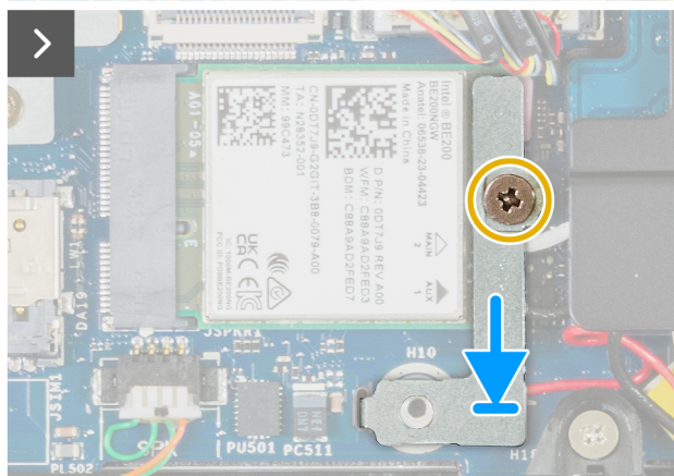
Afbeelding 45. De WLAN-kaart plaatsen
