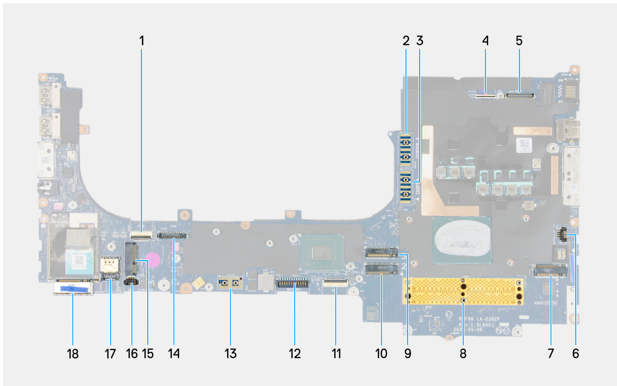
Afbeelding 115. Onderdelen van de systeemkaart
