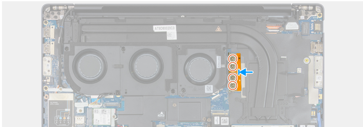
Afbeelding 54. De geïntegreerde FPC-beamconnector installeren
