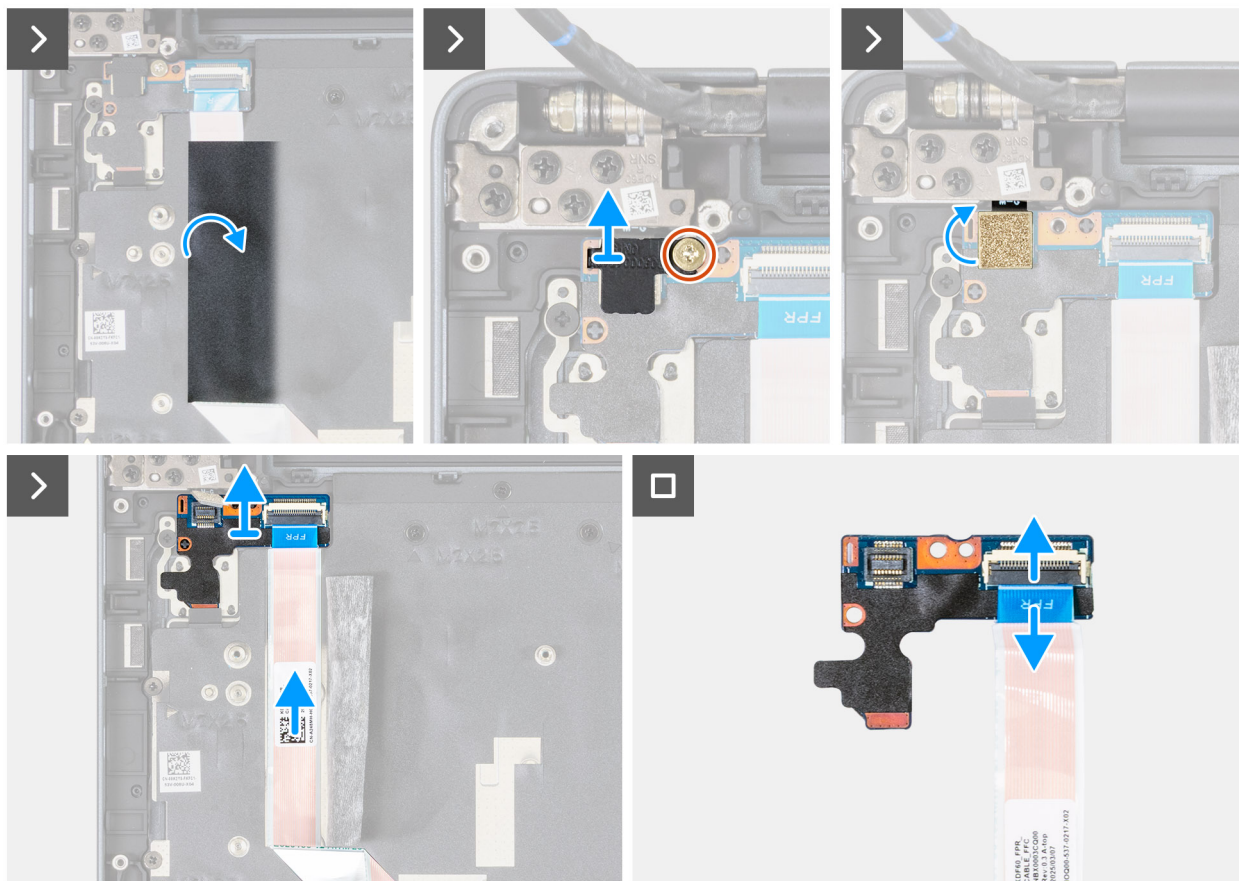
Afbeelding 128. De aan/uit-knopkaart verwijderen
