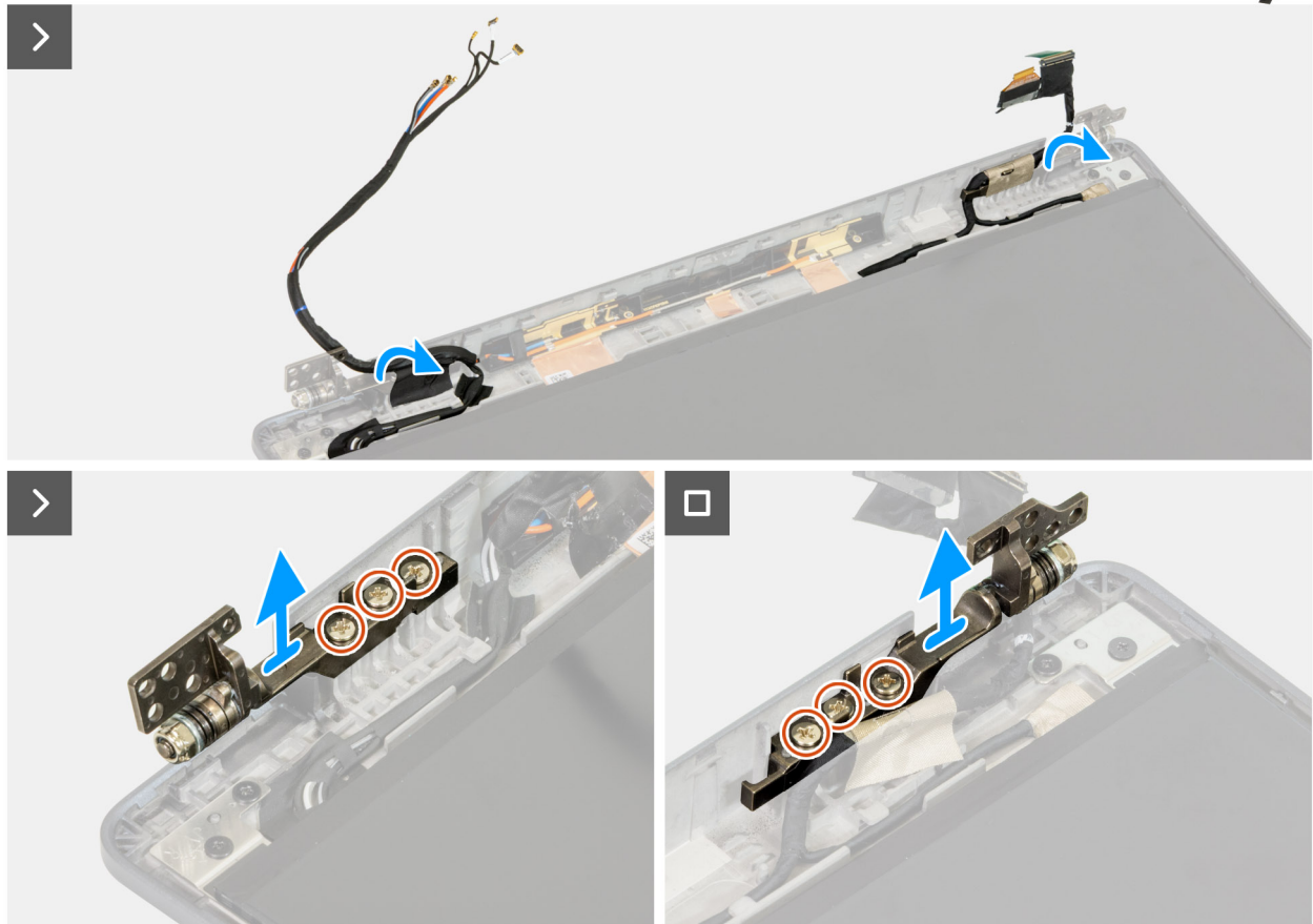
Afbeelding 102. De beeldschermcharnieren verwijderen
