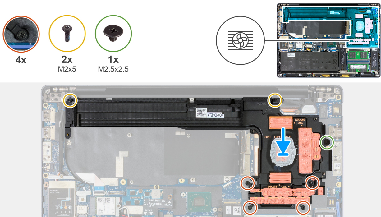
Afbeelding 79. De koelplaat installeren voor computers die met discrete graphics worden geleverd
