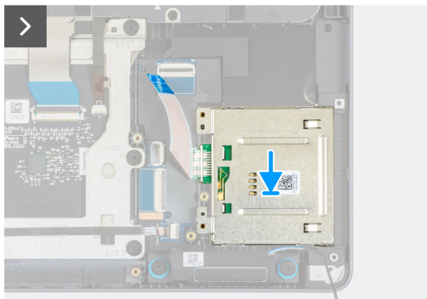
Afbeelding 125. De smartcardlezer installeren
