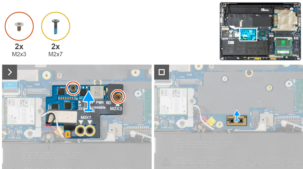
Afbeelding 74. De voedingskaart verwijderen
