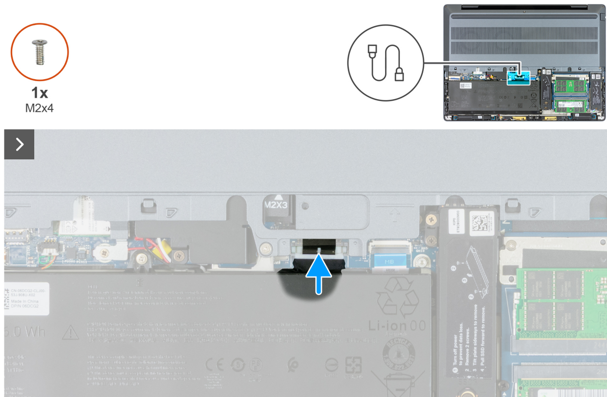
Afbeelding 21. De batterijkabel aansluiten
