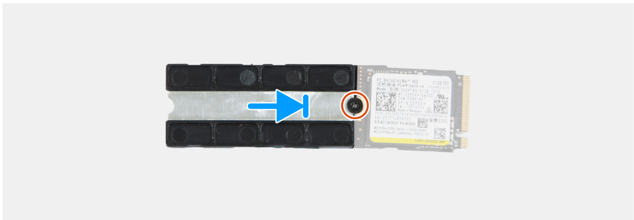
Afbeelding 39. De M.2 2230 SSD installeren
