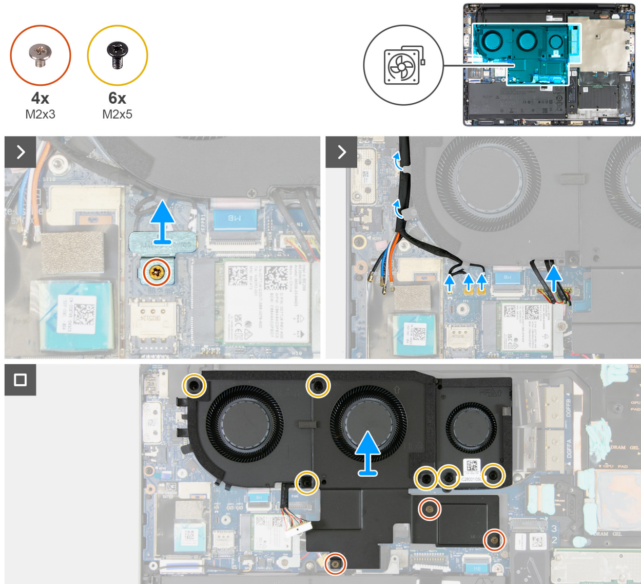
Afbeelding 64. De ventilatoreenheid verwijderen
