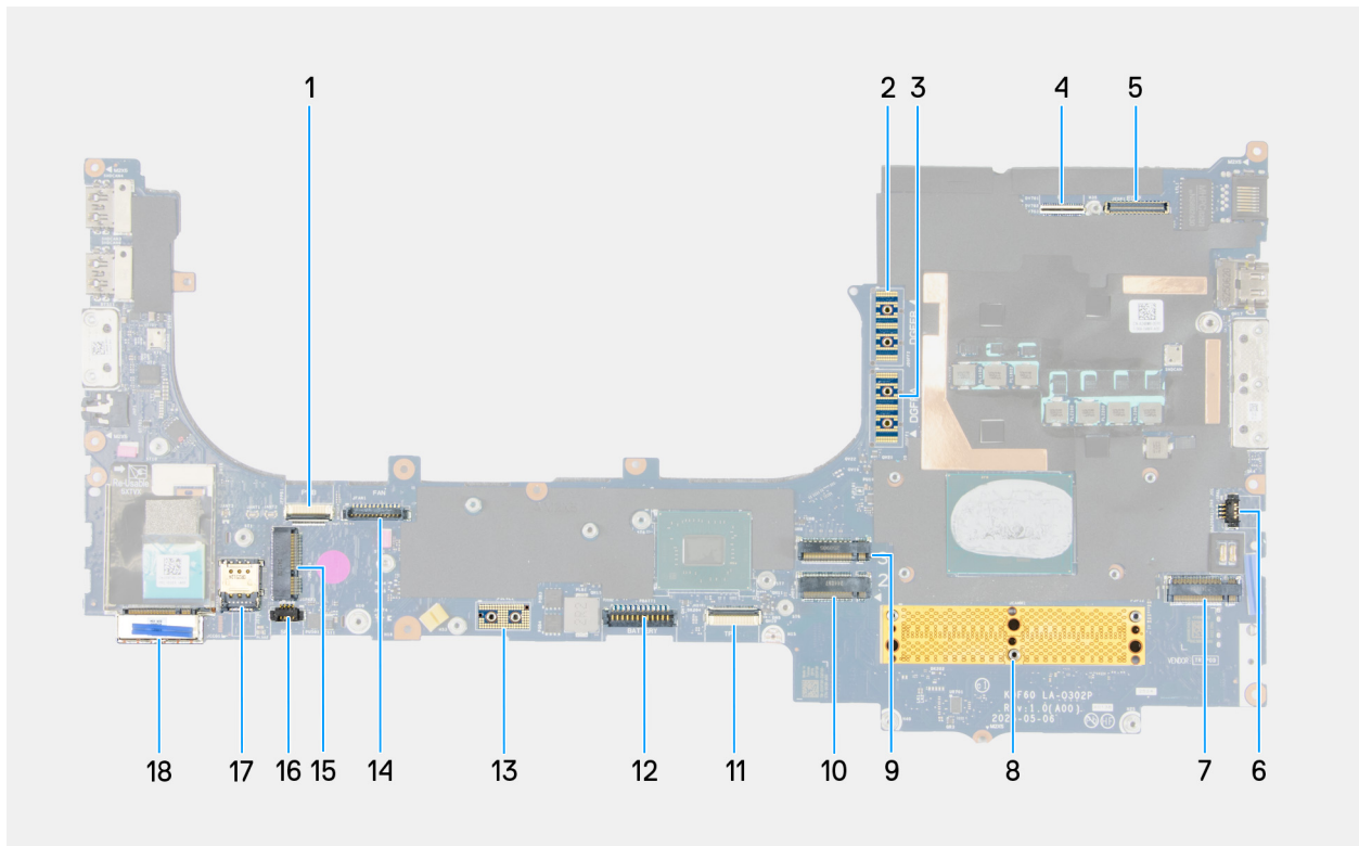
Afbeelding 111. Onderdelen van de systeemkaart
