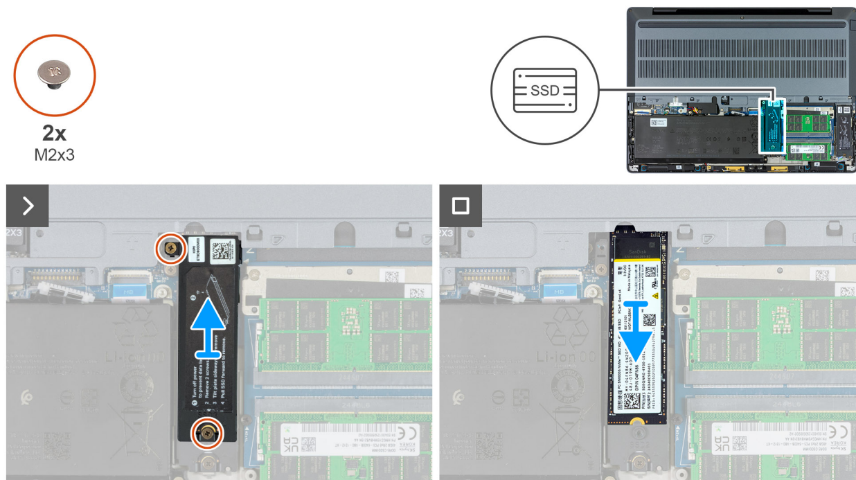
Afbeelding 34. De M.2 2280 SSD verwijderen uit slot 3 (SSD3)
