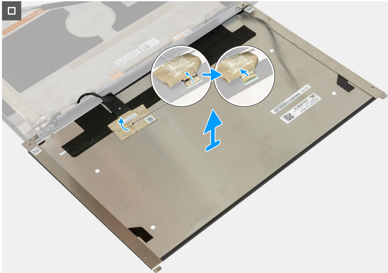
Afbeelding 95. Het beeldschermpaneel voor beeldschermen met touchscreen verwijderen
