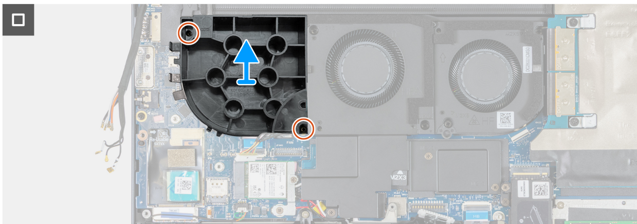
Afbeelding 57. De dummyventilator verwijderen
