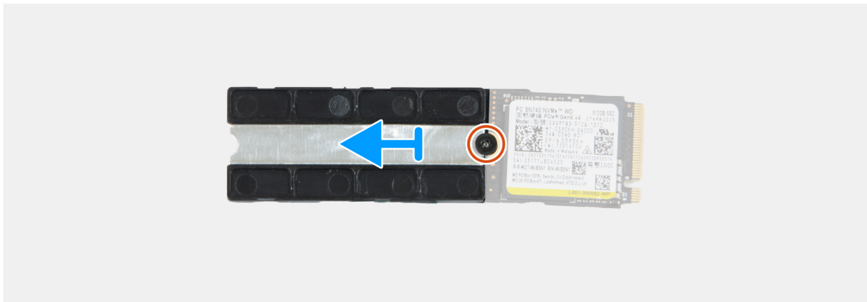
Afbeelding 38. De M.2 2230 SSD verwijderen
