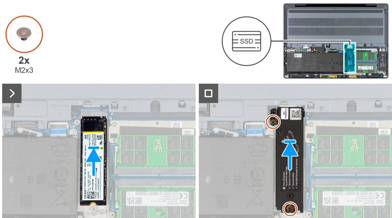
Afbeelding 37. De M.2 2280 SSD in slot 2 (SSD2) installeren
