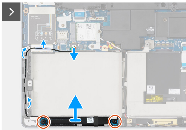
Afbeelding 84. De luidsprekers verwijderen
