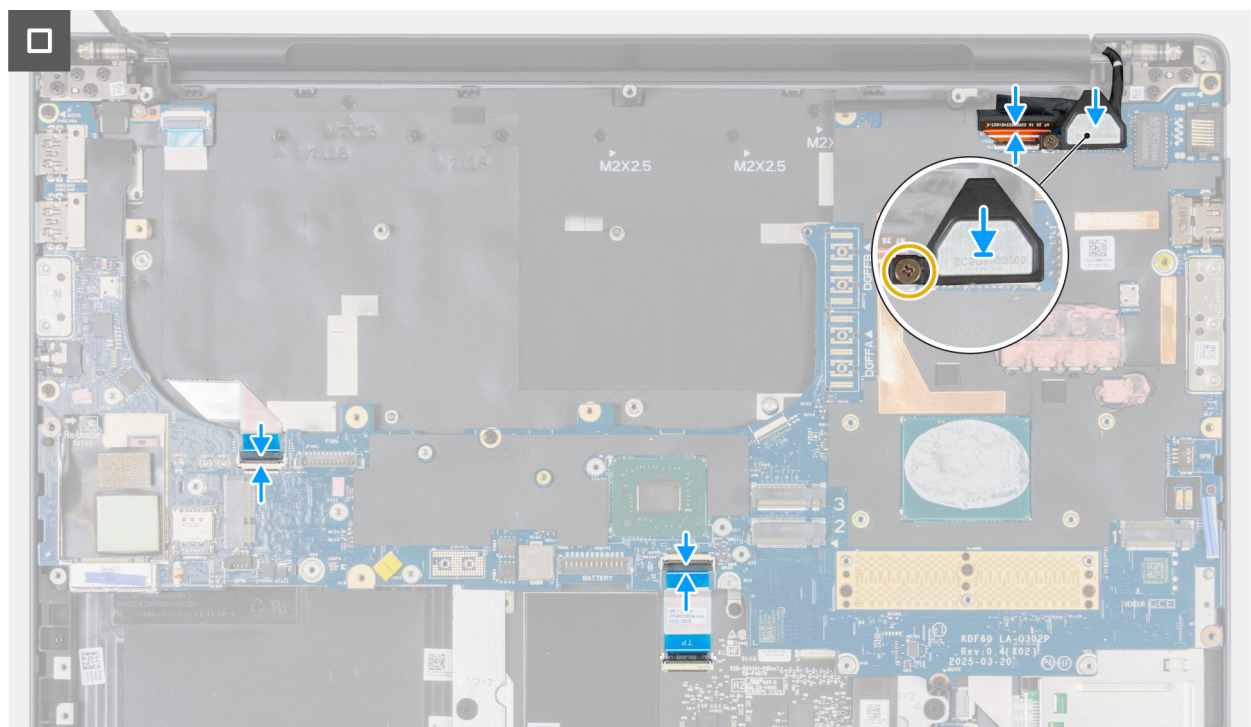
Afbeelding 117. De systeemkaart installeren
