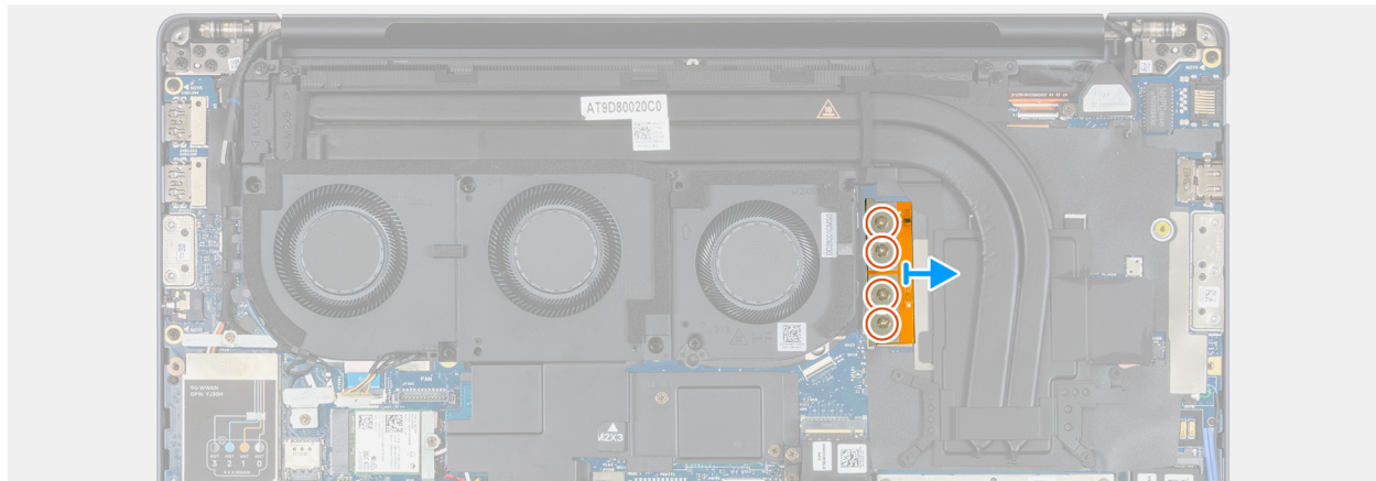
Afbeelding 53. De geïntegreerde FPC-beamconnector verwijderen
