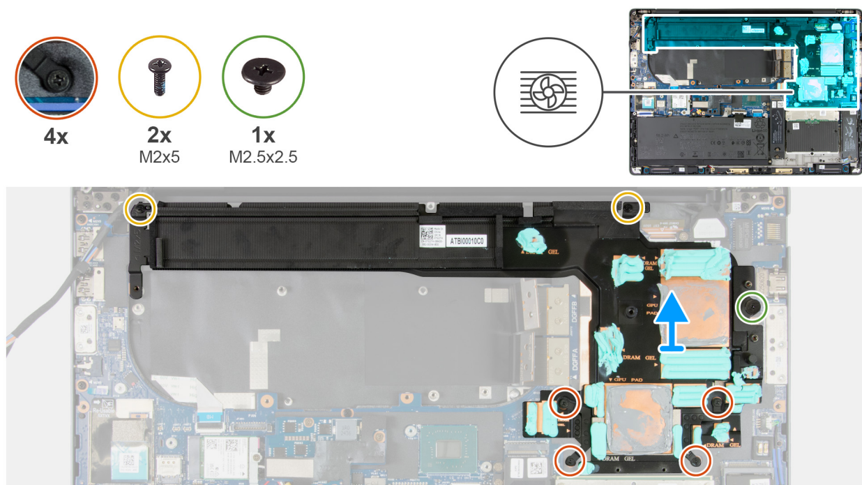
Afbeelding 76. De koelplaat verwijderen voor computers die worden geleverd met een geïntegreerde grafische kaart
