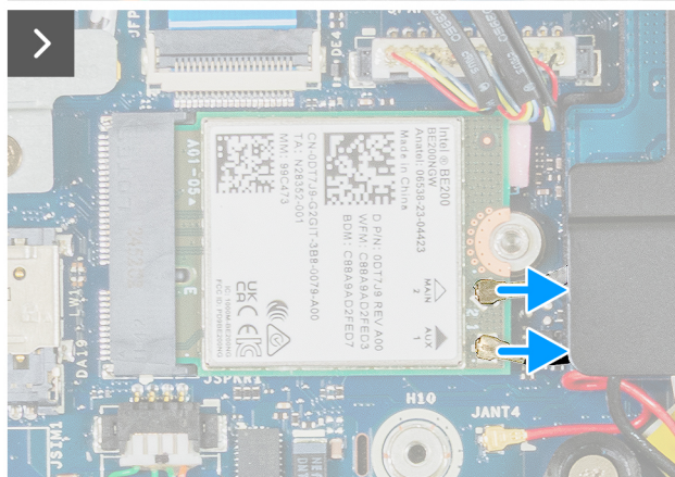
Afbeelding 44. De WLAN-kaart verwijderen
