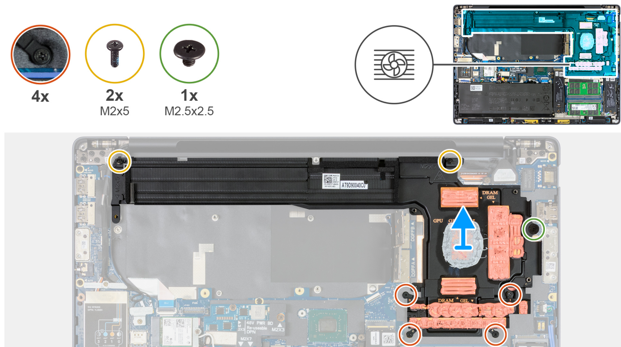
Afbeelding 78. De koelplaat verwijderen voor computers die worden geleverd met discrete graphics
