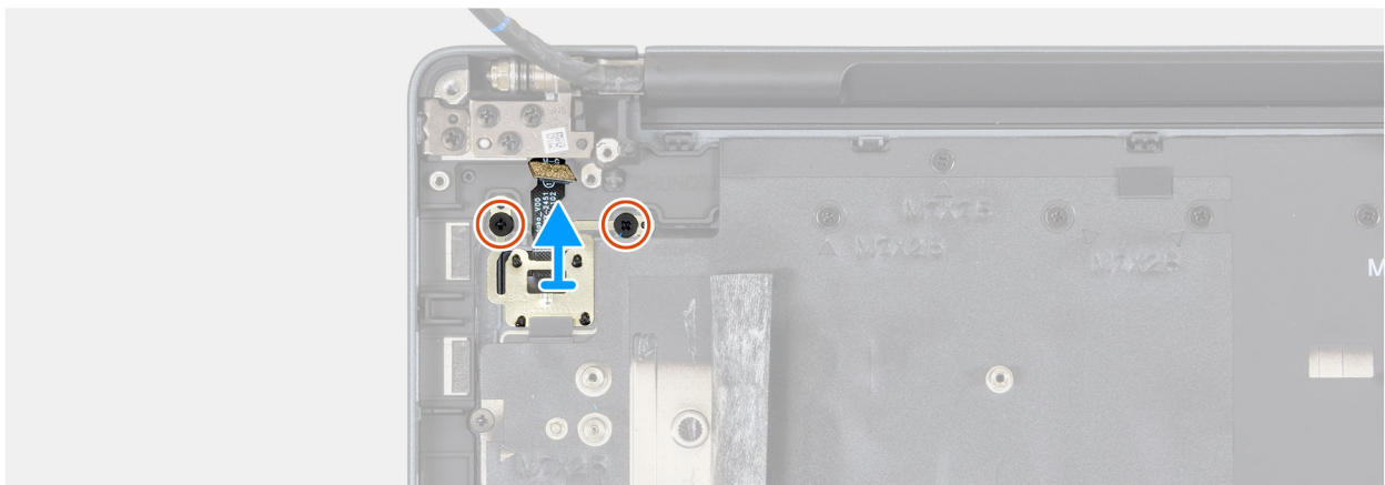
Abbeelding 130. De aan-uitknop verwijderen
