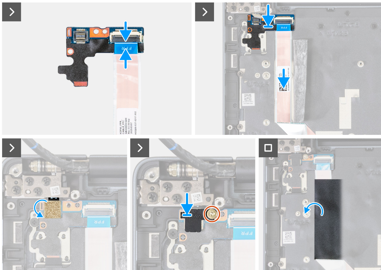
Afbeelding 129. De aan/uit-knopkaart plaatsen
