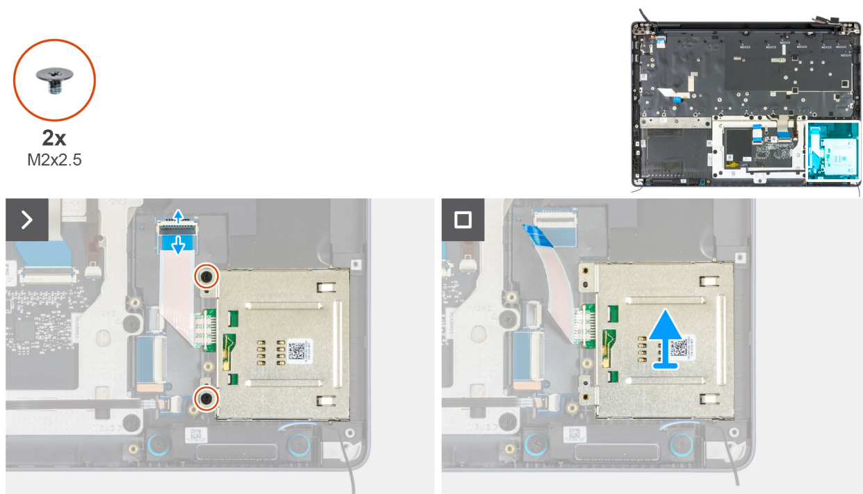
Afbeelding 124. De smartcardlezer verwijderen
