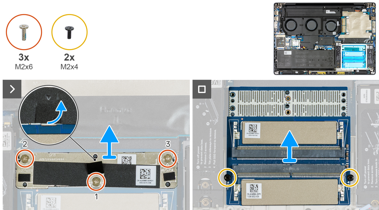
Afbeelding 70. De geheugeninterposerkaart verwijderen
