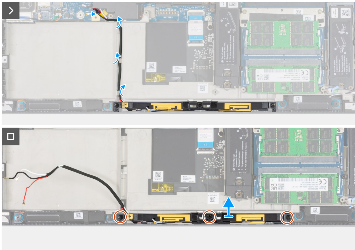
Afbeelding 80. De WLAN-antennemodule verwijderen
