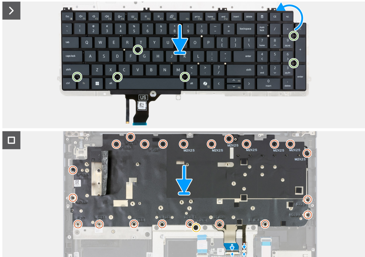
Afbeelding 123. Het toetsenbord plaatsen
