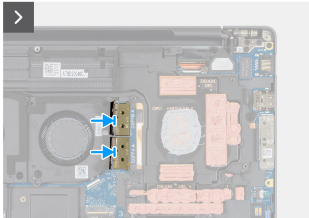
Afbeelding 56. De discrete FPC-balkconnector installeren
