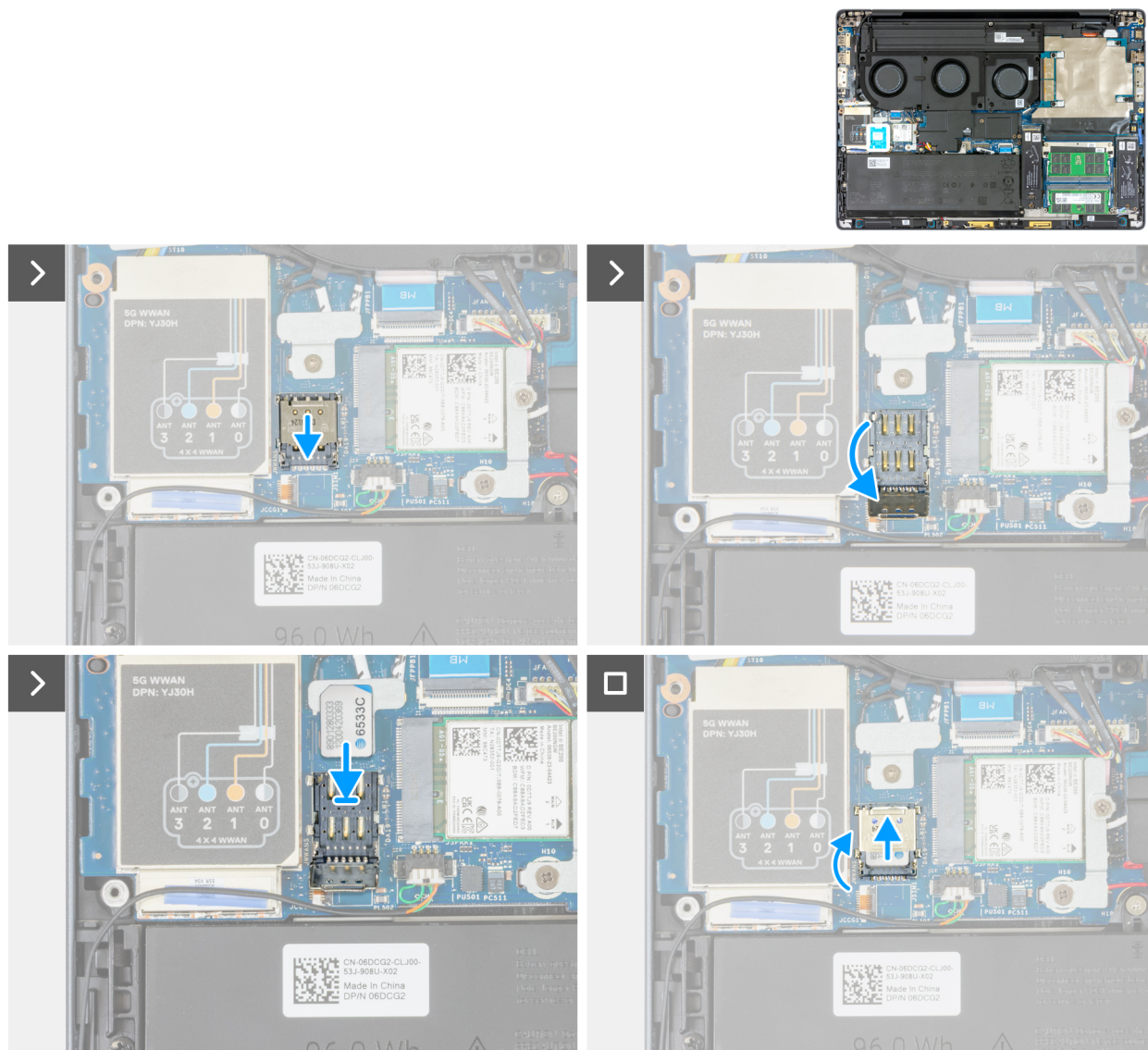
Afbeelding 47. De SIM-kaart installeren
