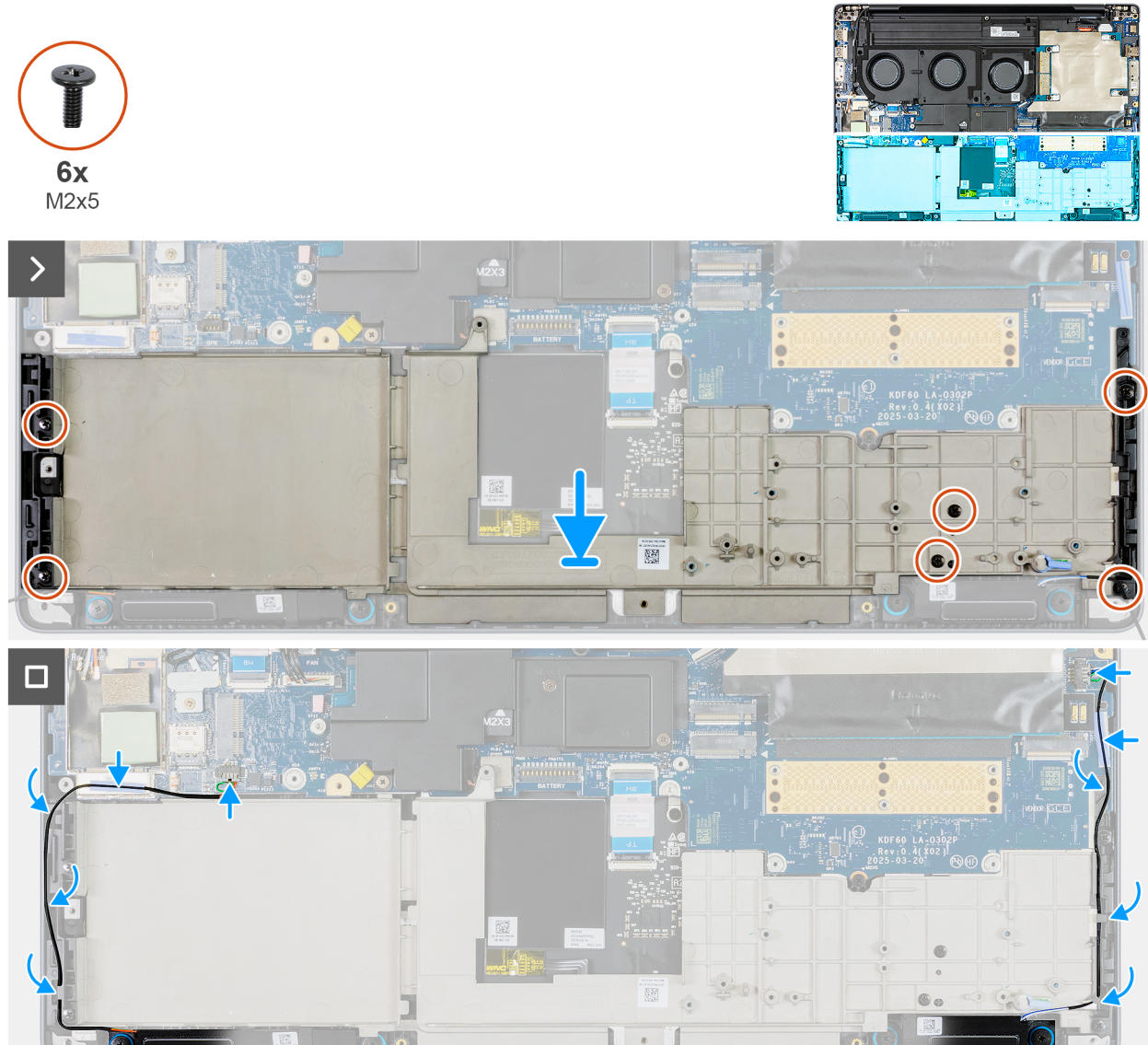
Afbeelding 83. Het binnenframe installeren
