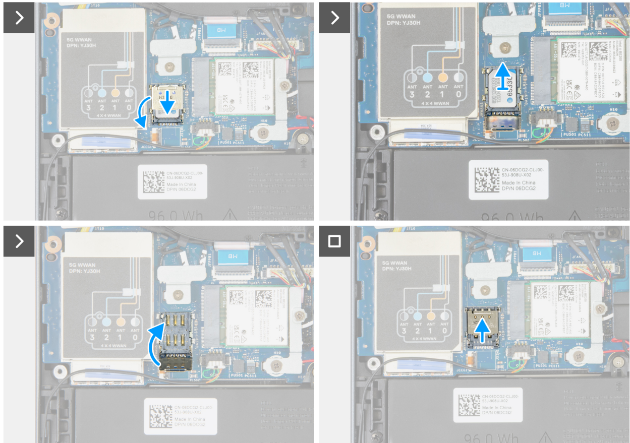
Afbeelding 46. De SIM-kaart verwijderen
