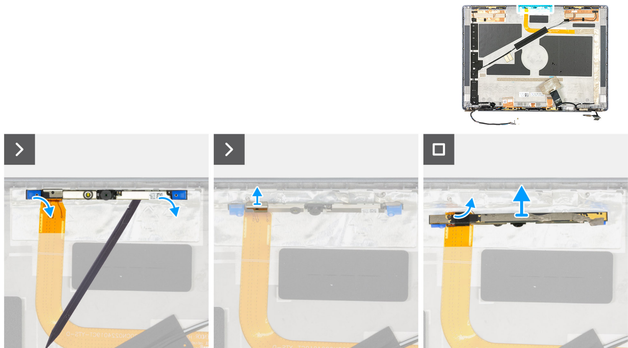
Afbeelding 104. De cameramodule verwijderen
