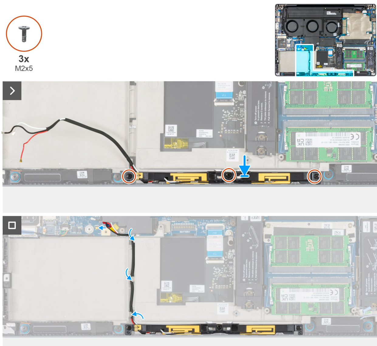
Afbeelding 81. De WLAN-antennemodule plaatsen
