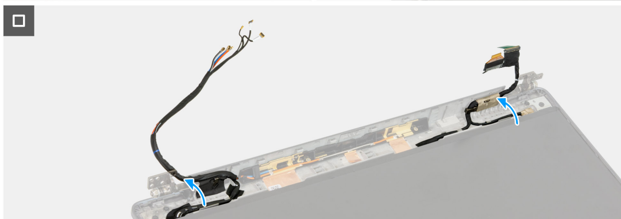
Afbeelding 103. De beeldschermcharnieren installeren
