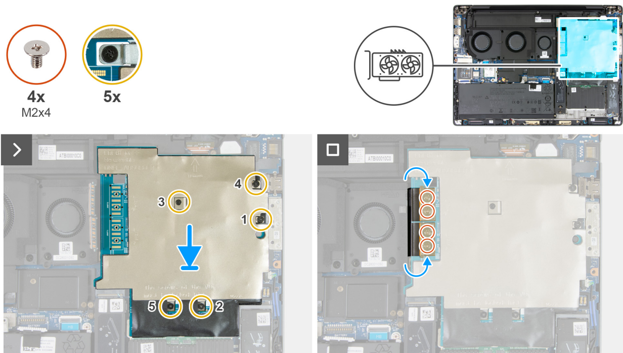
Afbeelding 61. De NPU-kaart installeren
