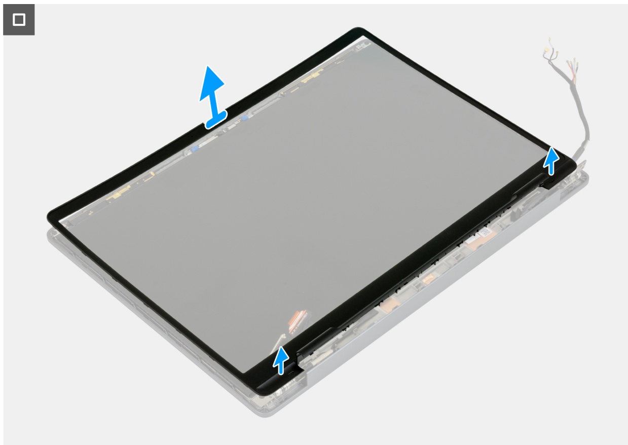
Afbeelding 91. De beeldschermbezel verwijderen
