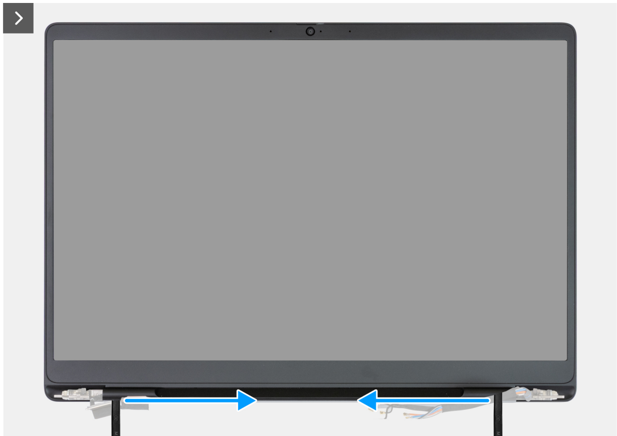
Afbeelding 89. De beeldschermbezel verwijderen
