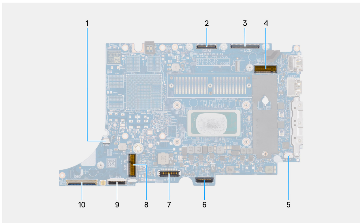
Afbeelding 86. Systeemkaartconnectoren
