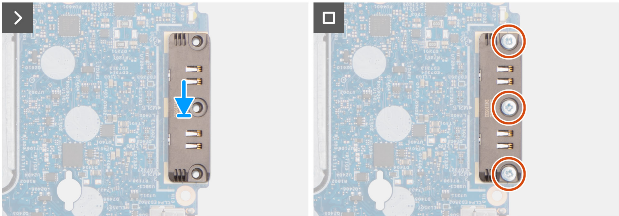
Afbeelding 93. De USB Type-C-module installeren
