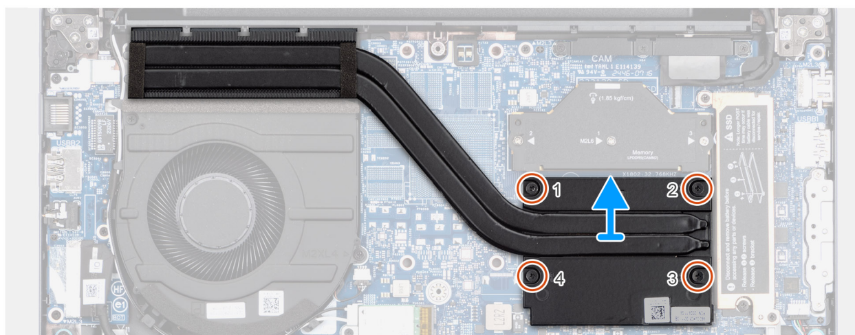
Afbeelding 39. De koelplaat verwijderen
