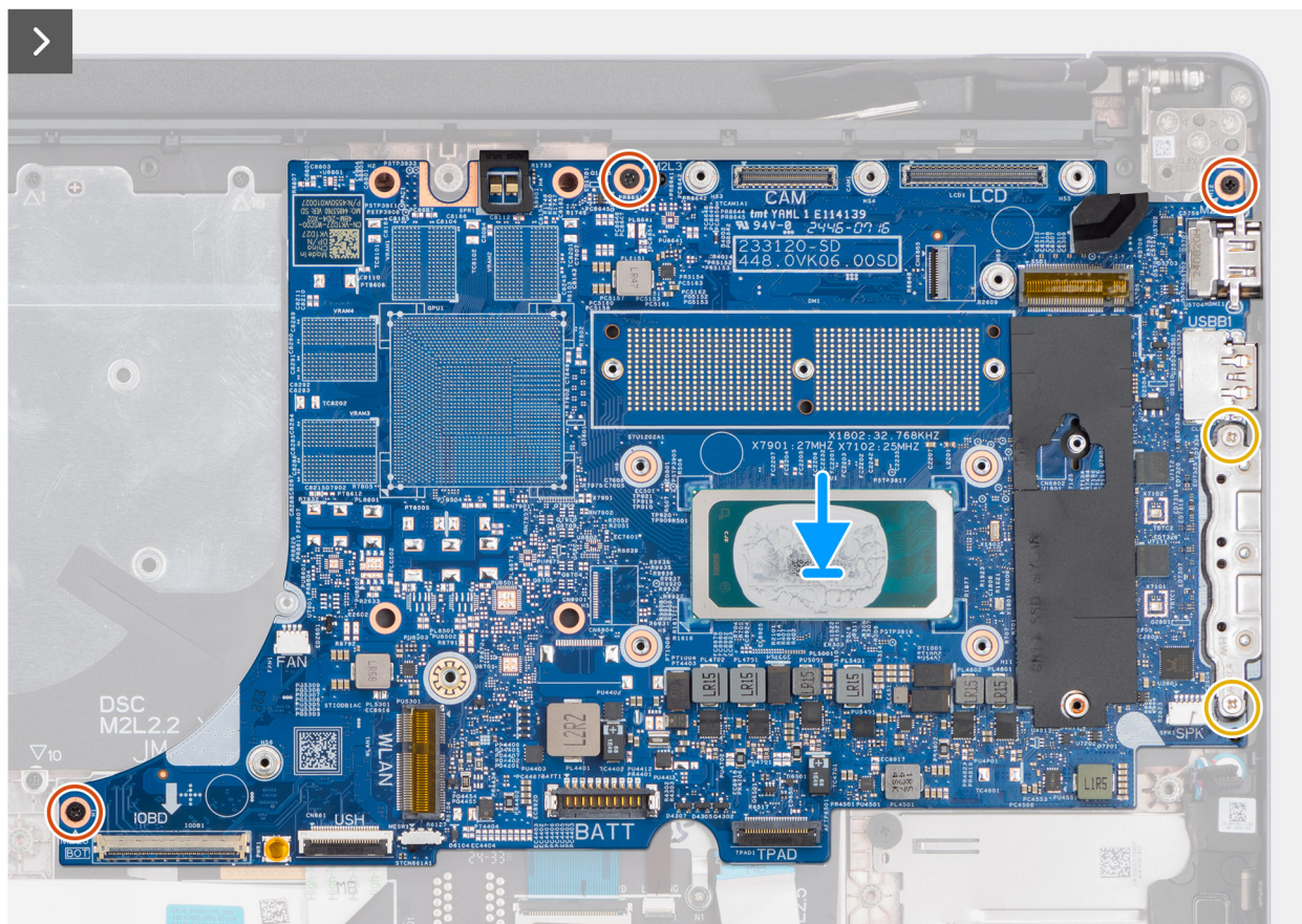
Afbeelding 81. De systeemkaart plaatsen
