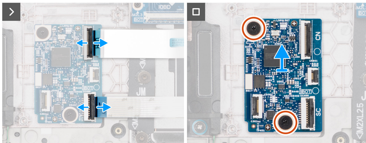
Afbeelding 35. De USH-kaart verwijderen
