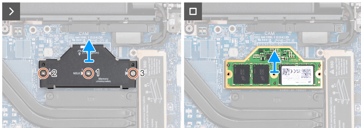
Afbeelding 20. De geheugenmodule verwijderen
