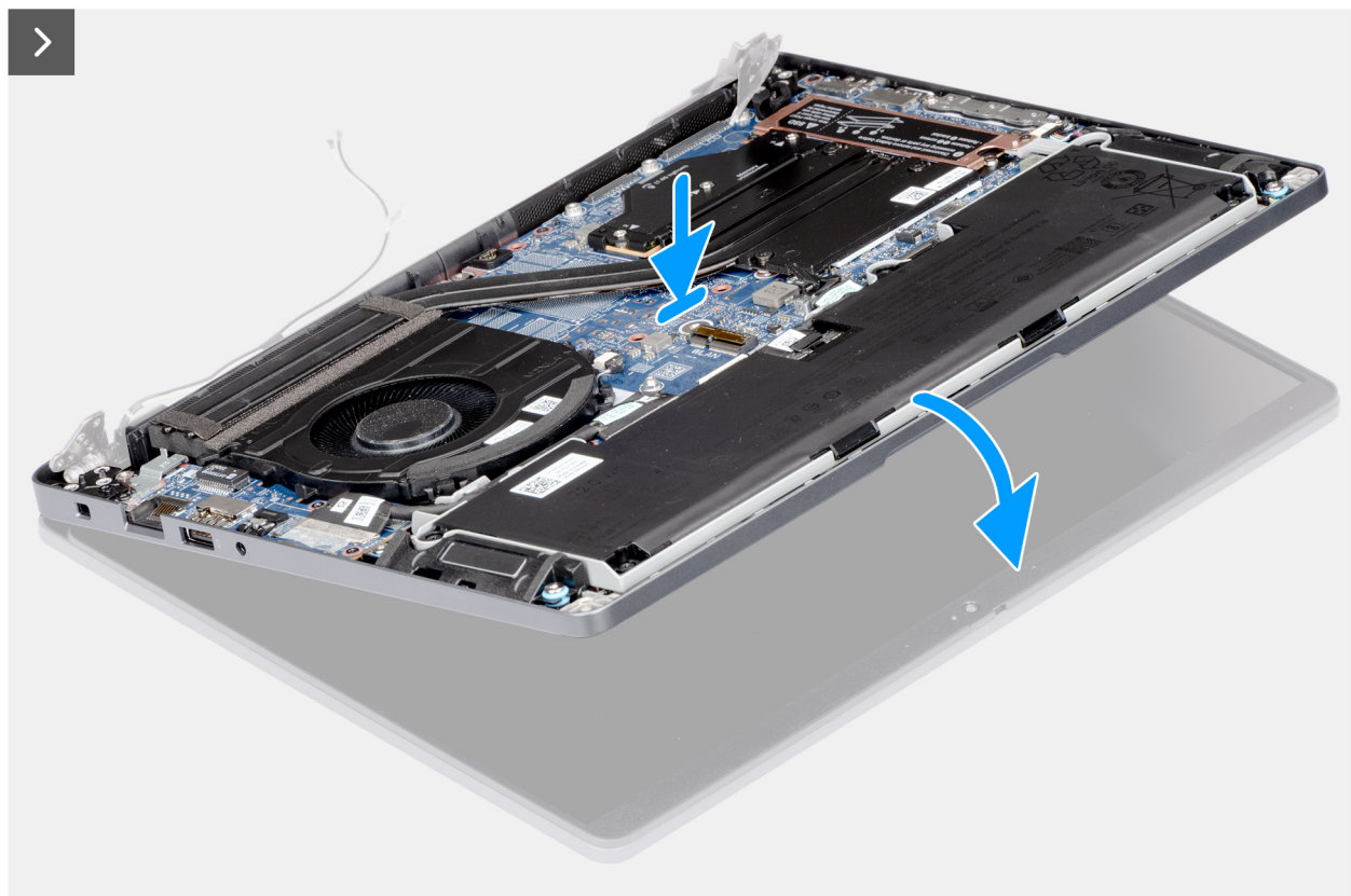
Afbeelding 50. De beeldschermeenheid plaatsen
