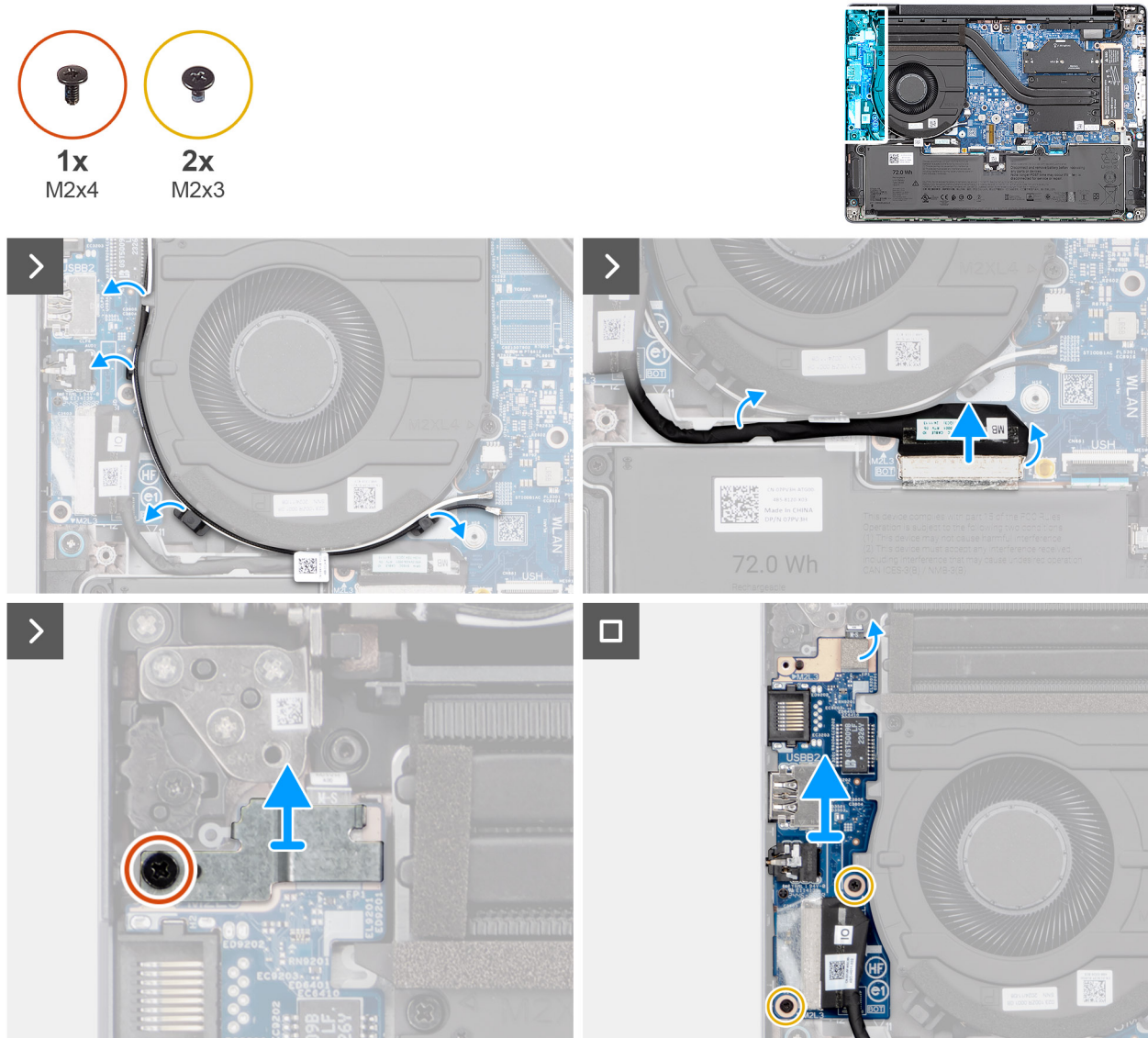
Afbeelding 43. De I/O-kaart verwijderen
