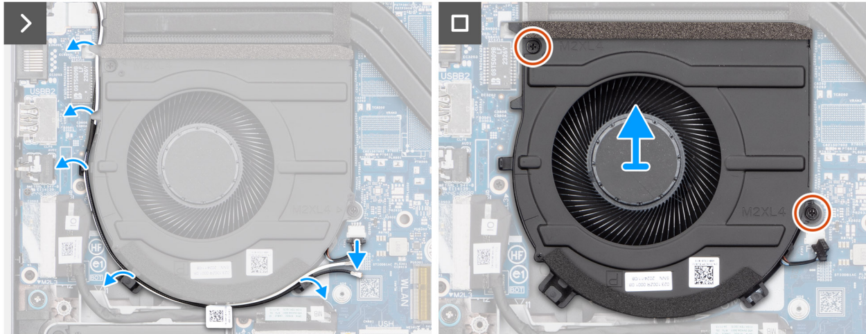
Afbeelding 31. De ventilator verwijderen
