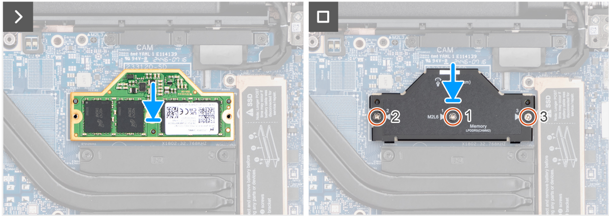
Afbeelding 21. De geheugenmodule plaatsen
