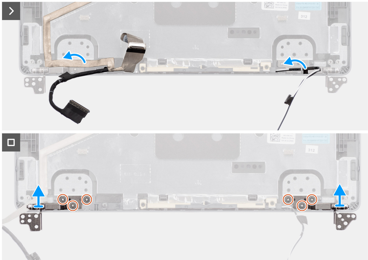
Afbeelding 66. De beeldschermcharnieren verwijderen
