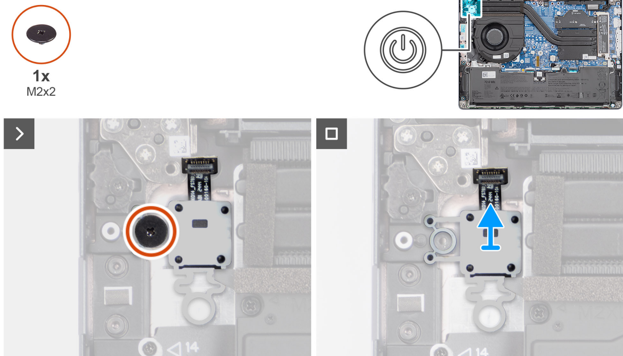
Afbeelding 45. De aan-uitknop verwijderen
