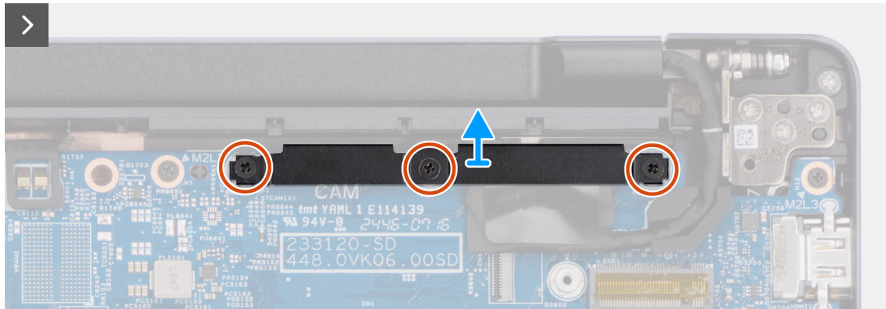
Afbeelding 75. De systeemkaart verwijderen
