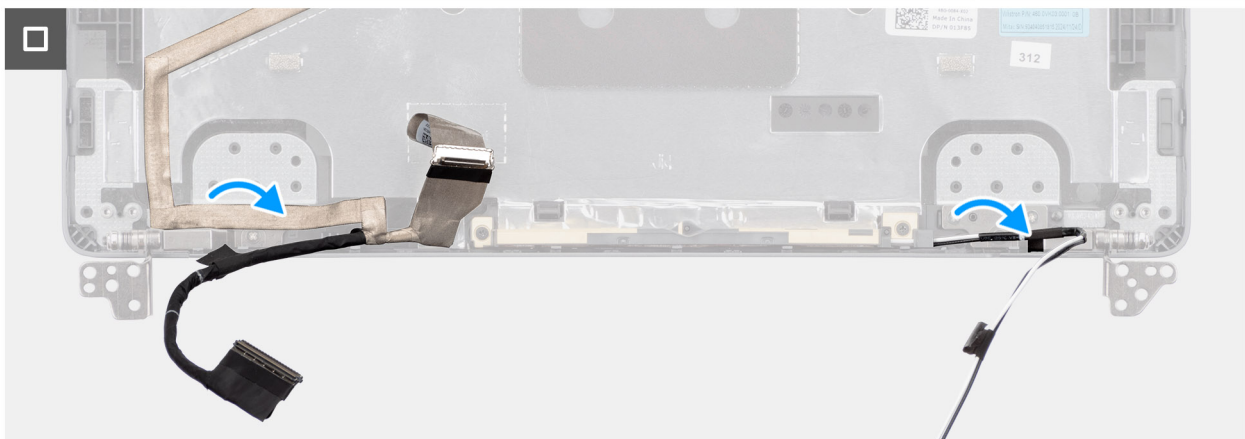
Afbeelding 67. De beeldschermcharnieren installeren
