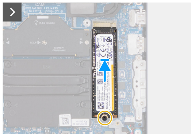
Afbeelding 25. De M.2 2280 SSD installeren
