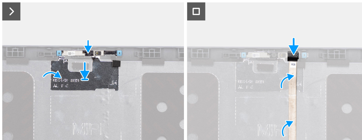
Afbeelding 71. De camera installeren
