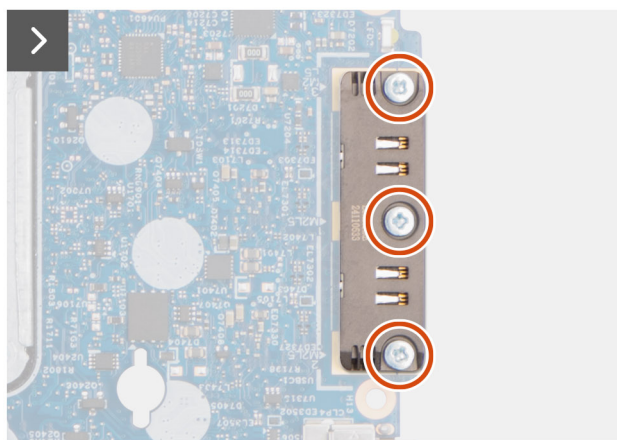
Afbeelding 92. De USB Type-C-module verwijderen
