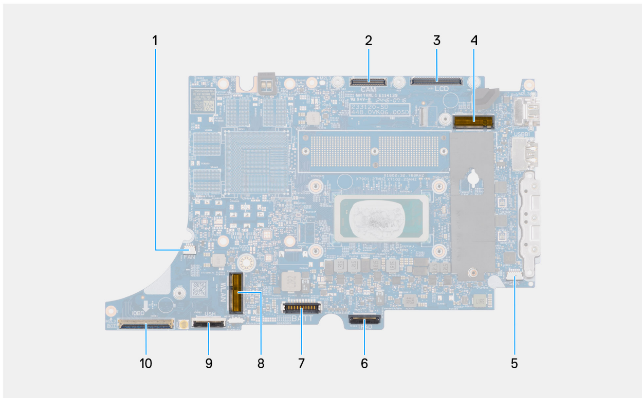
Afbeelding 80. Systemkaartconnectoren
