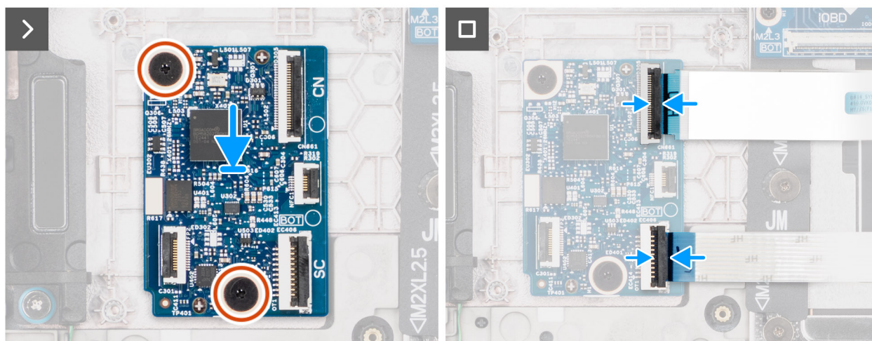
Afbeelding 36. De USH-kaart plaatsen
