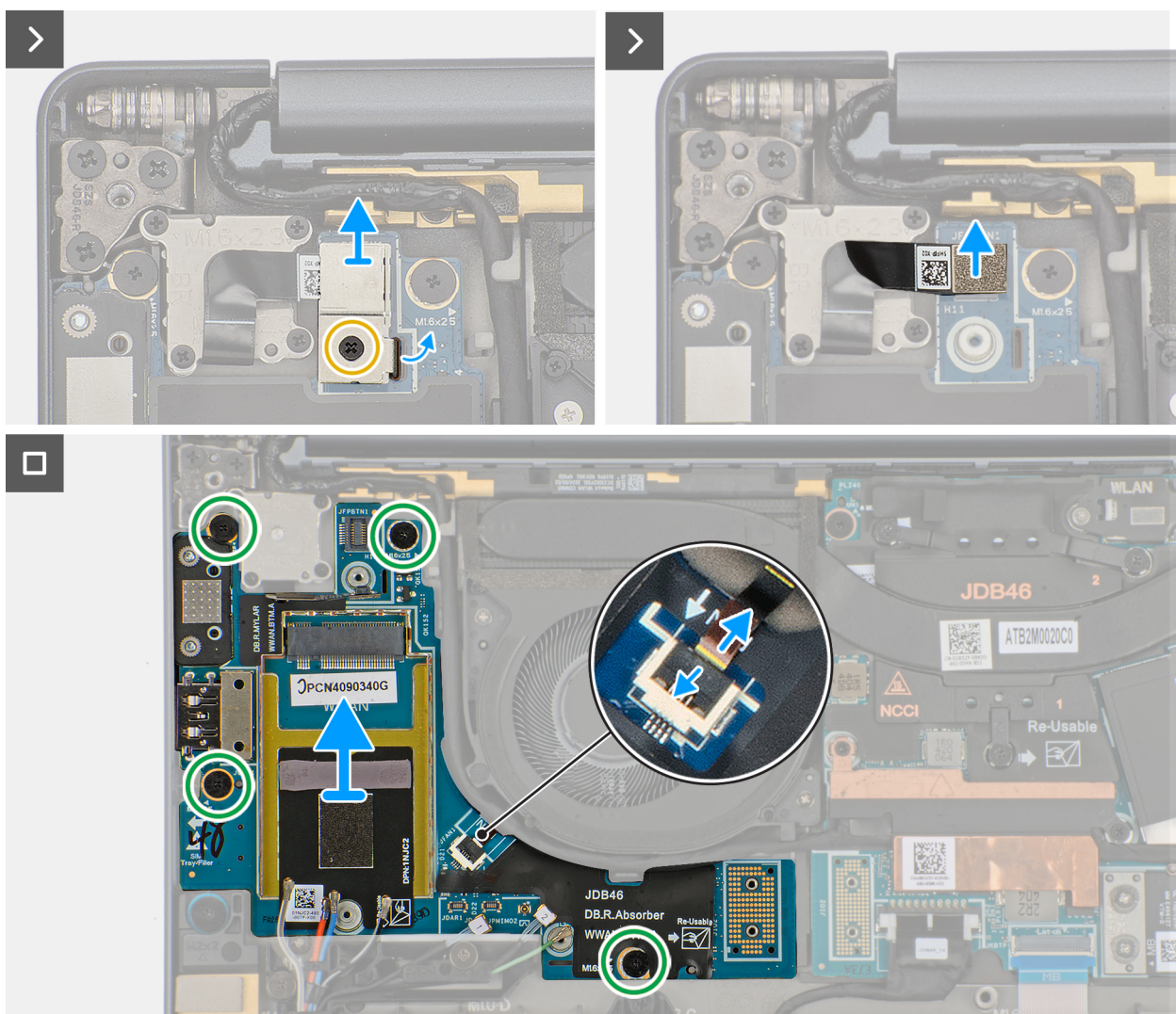
Figure 51. Retrait de la carte d'E/S droite (avec WWAN)
