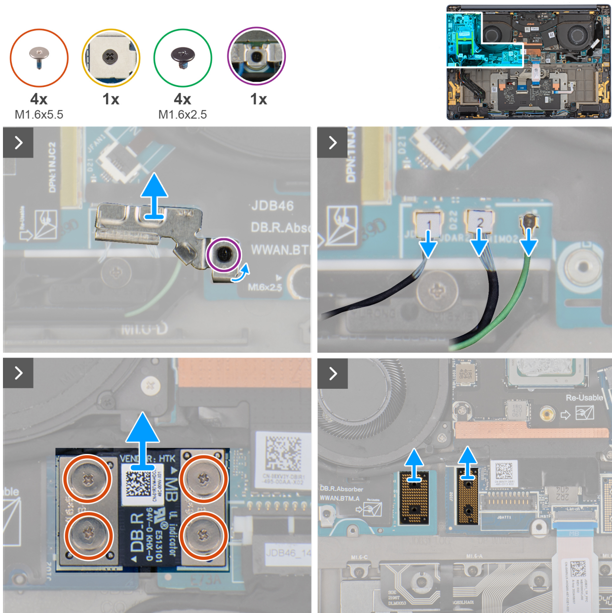
Figure 50. Retrait des vis
