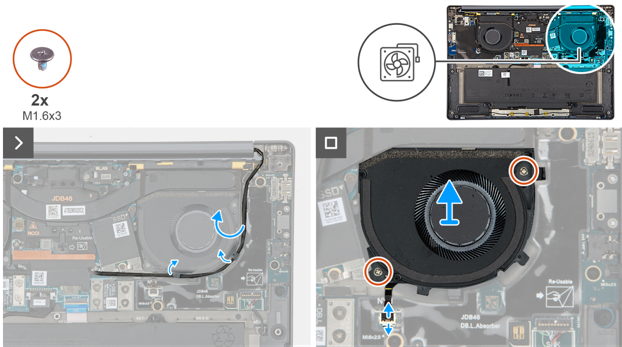
Figure 30. Retrait du ventilateur gauche
