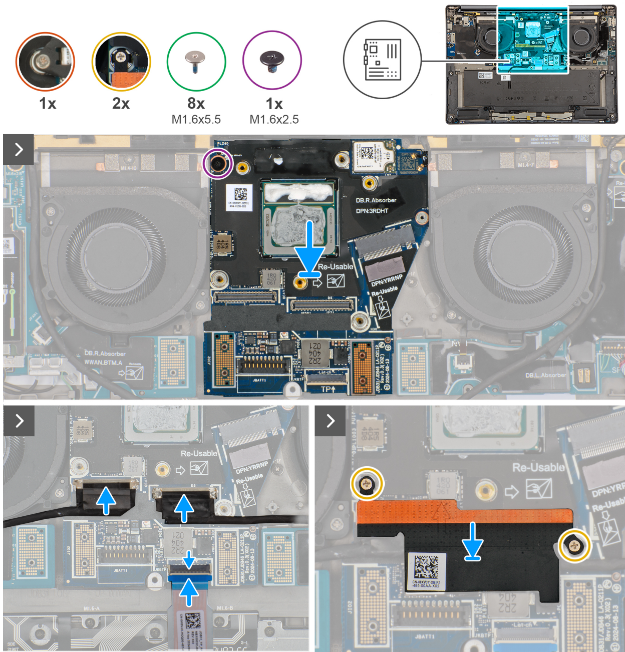
Figure 72. Installation de la carte système
