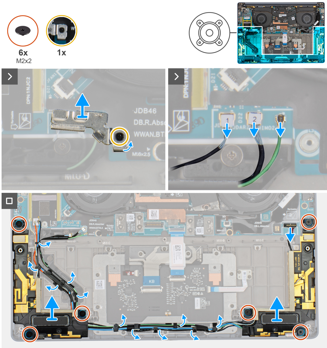
Figure 36. Retrait des haut-parleurs avec antennes (configuration WWAN)
