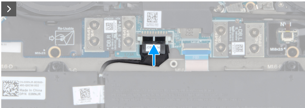
Figure 19. Branchement du câble de la batterie à la carte système
