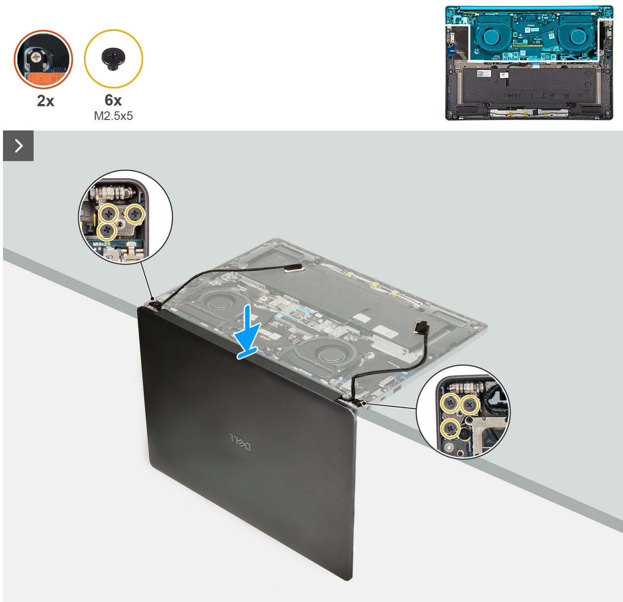
Figure 65. Installation de l'assemblage d'écran
