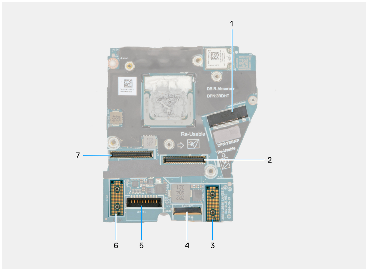
Figure 67. Légendes de la carte système
