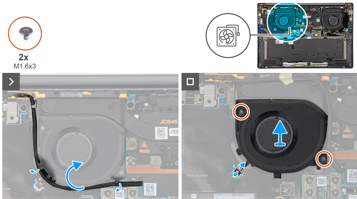
Figure 32. Retrait du ventilateur droit
