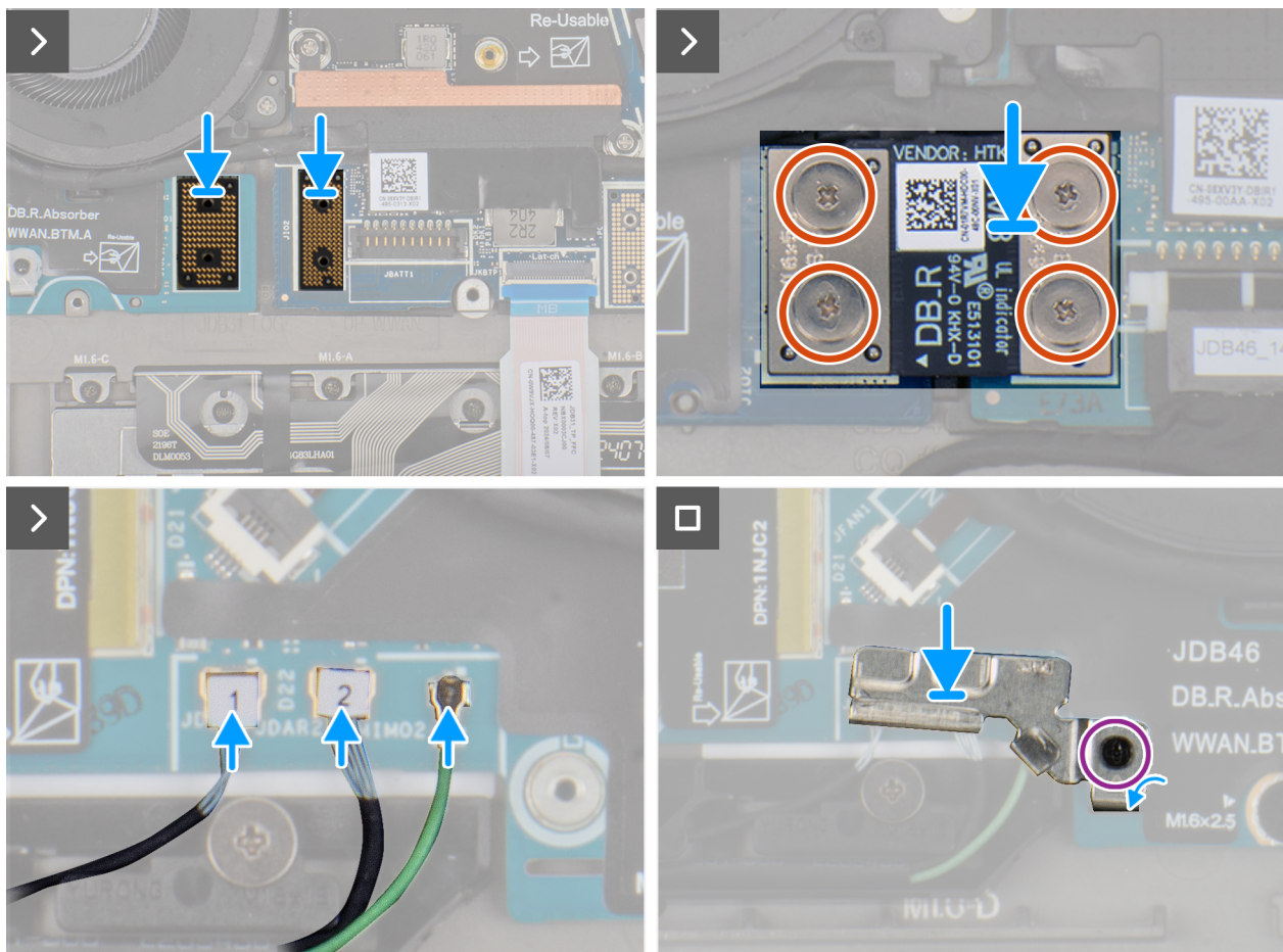
Figure 54. Installation de la carte d'E/S droite (avec WWAN)
