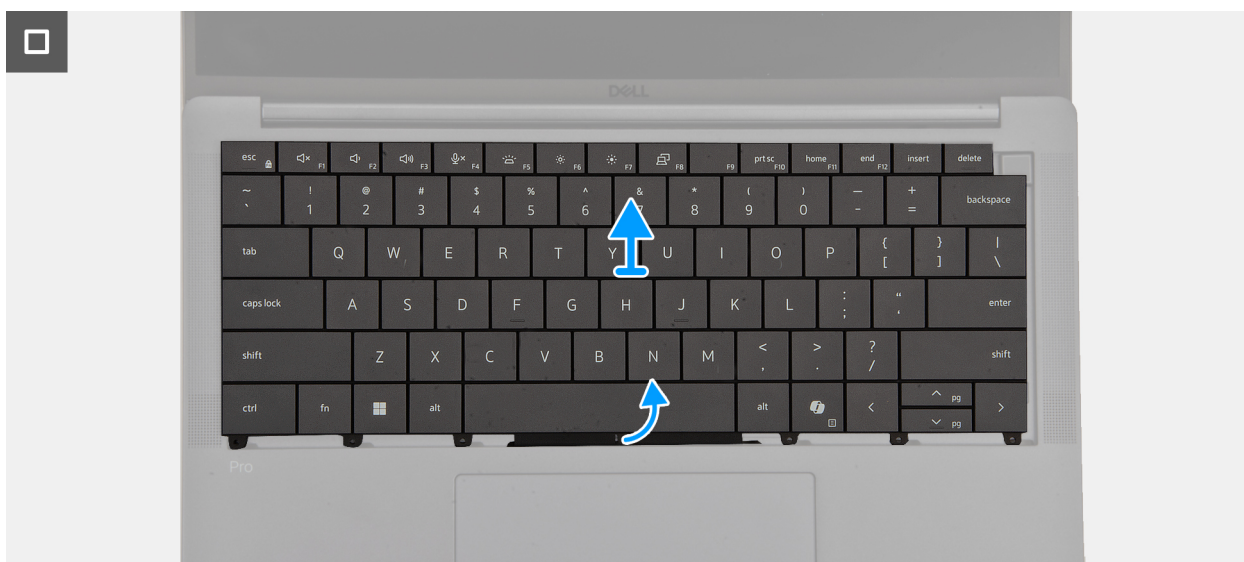
Figure 76. Retrait de l'assemblage du clavier
