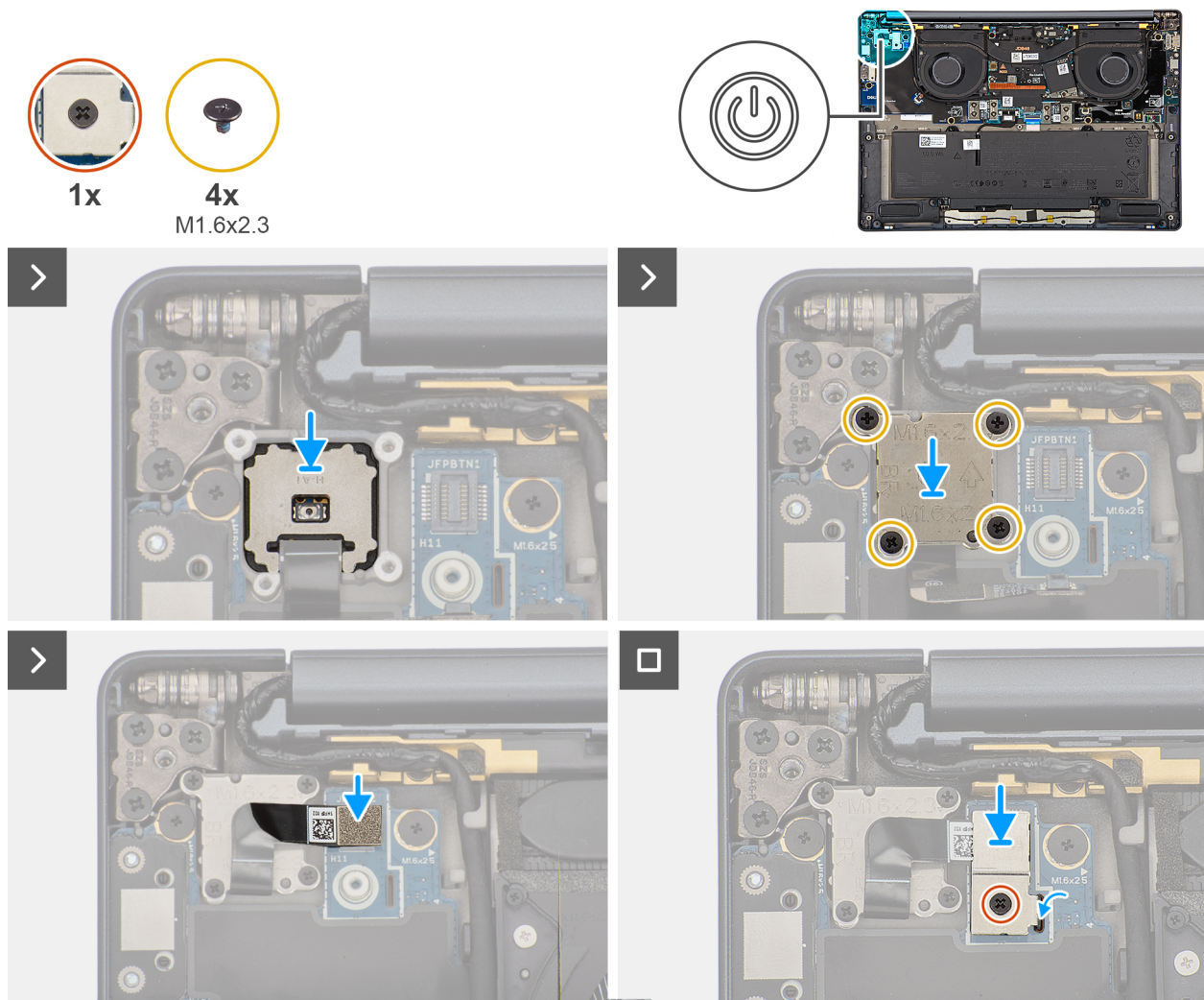
Figure 61. Installation du bouton d'alimentation
