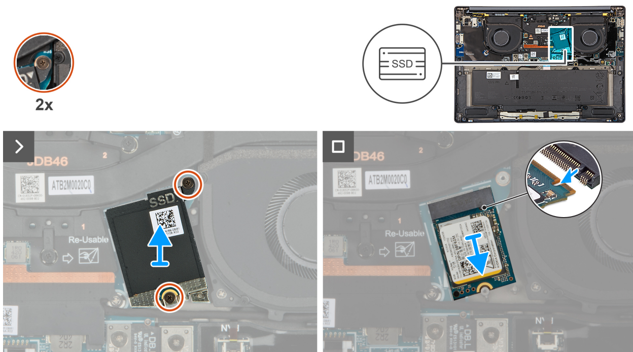
Figure 26. Retrait du module SSD
