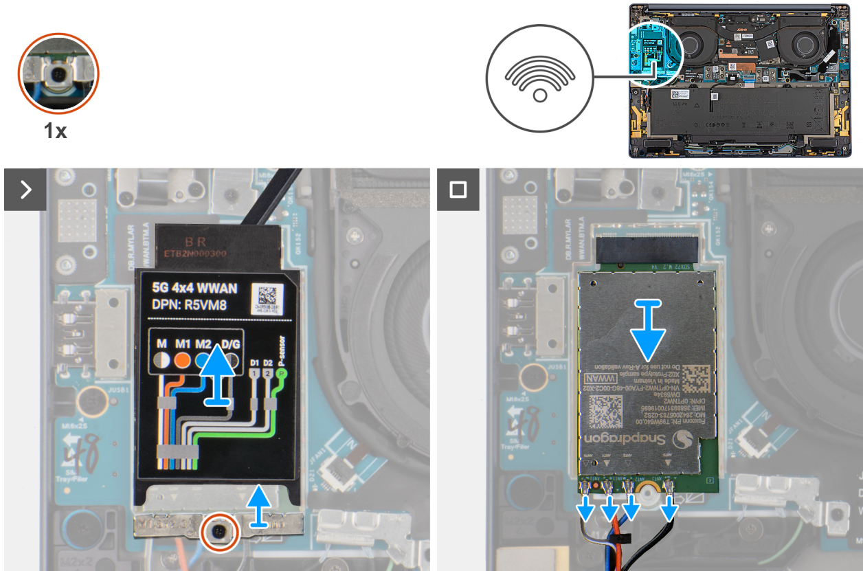
Figure 28. Retrait de la carte WWAN
