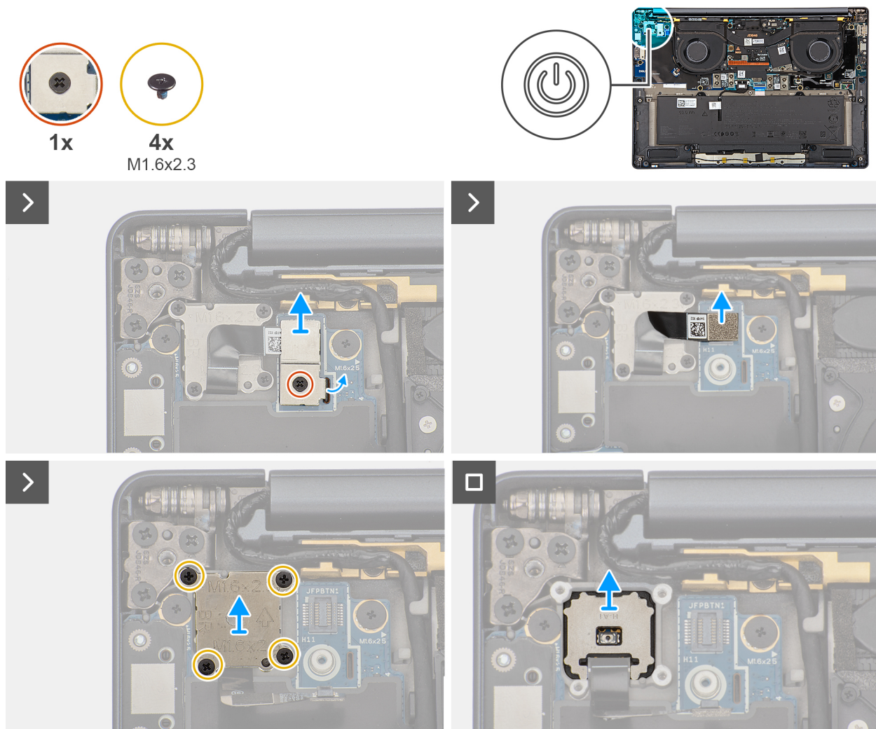
Figure 60. Retrait du bouton d'alimentation
