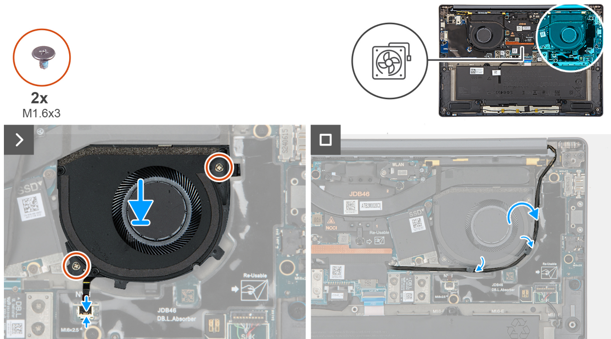
Figure 31. Installation du ventilateur gauche
