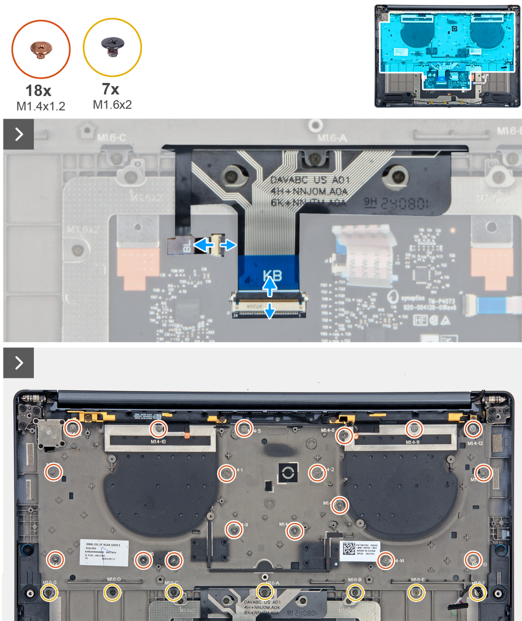
Figure 75. Retrait de l'assemblage du clavier
