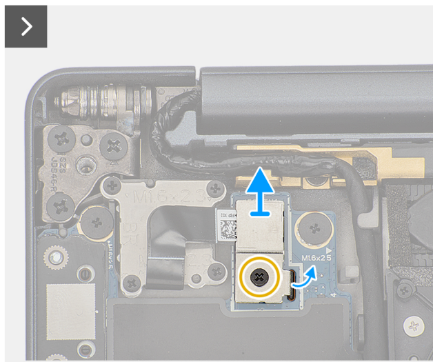
Figure 44. Retrait des vis
