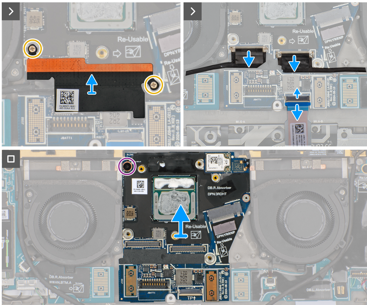
Figure 69. Retrait de la carte système
