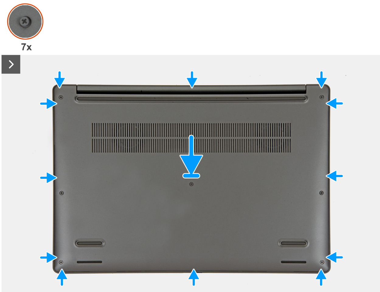
Figure 20. Installation du cache de fond
