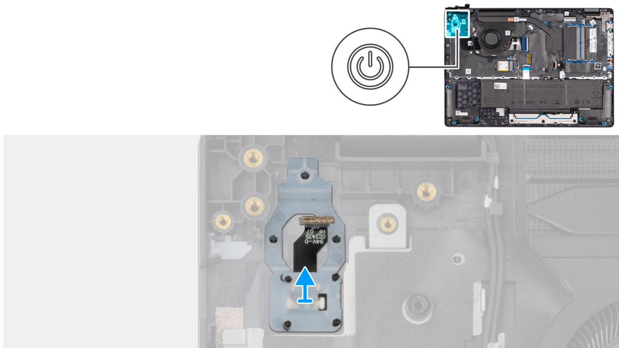
Figure 40. Retrait du bouton d'alimentation avec lecteur d'empreintes digitales
