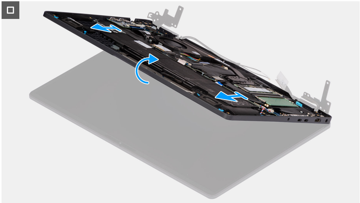
Figure 63. Retrait de l'assemblage d'écran
