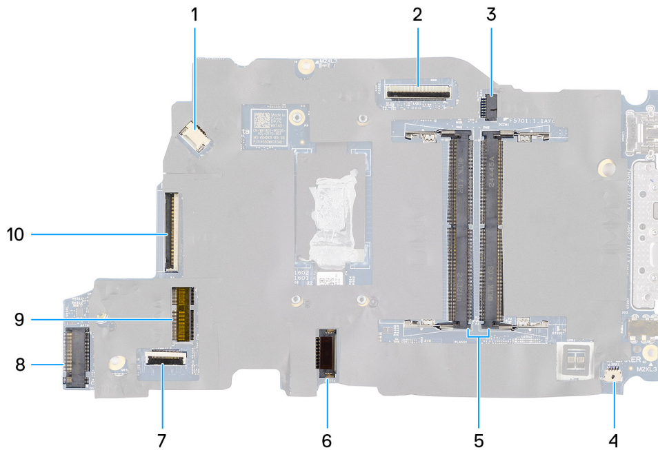
Figure 42. Connecteurs de la carte système
