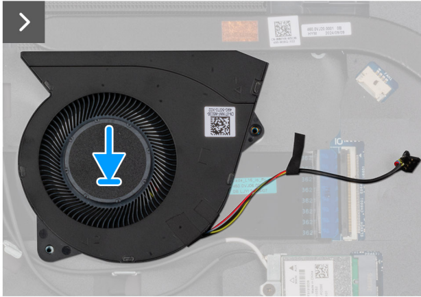
Figure 31. Installation du ventilateur
