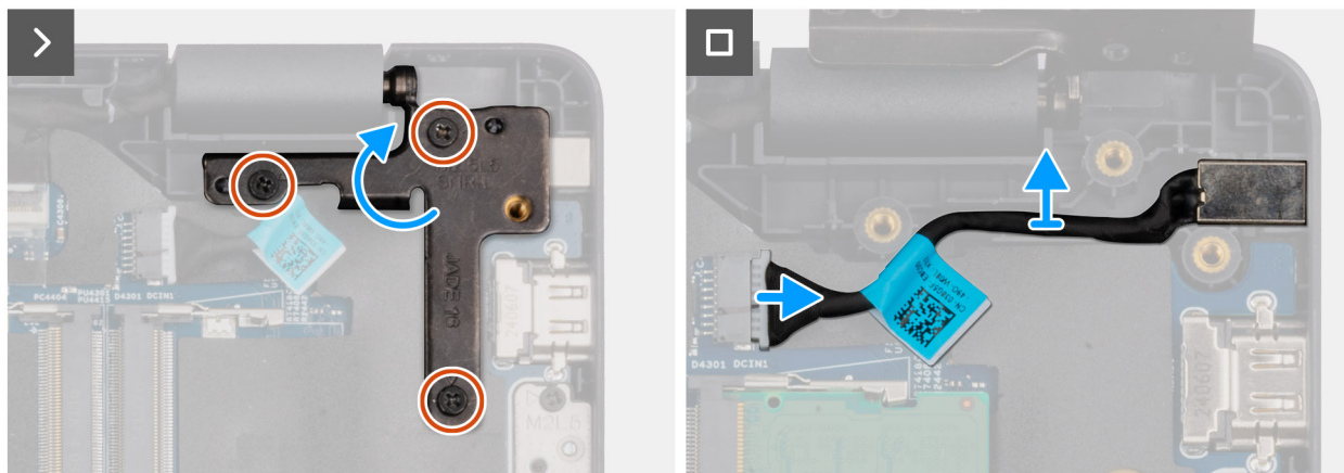
Figure 32. Retrait du port de l'adaptateur secteur
