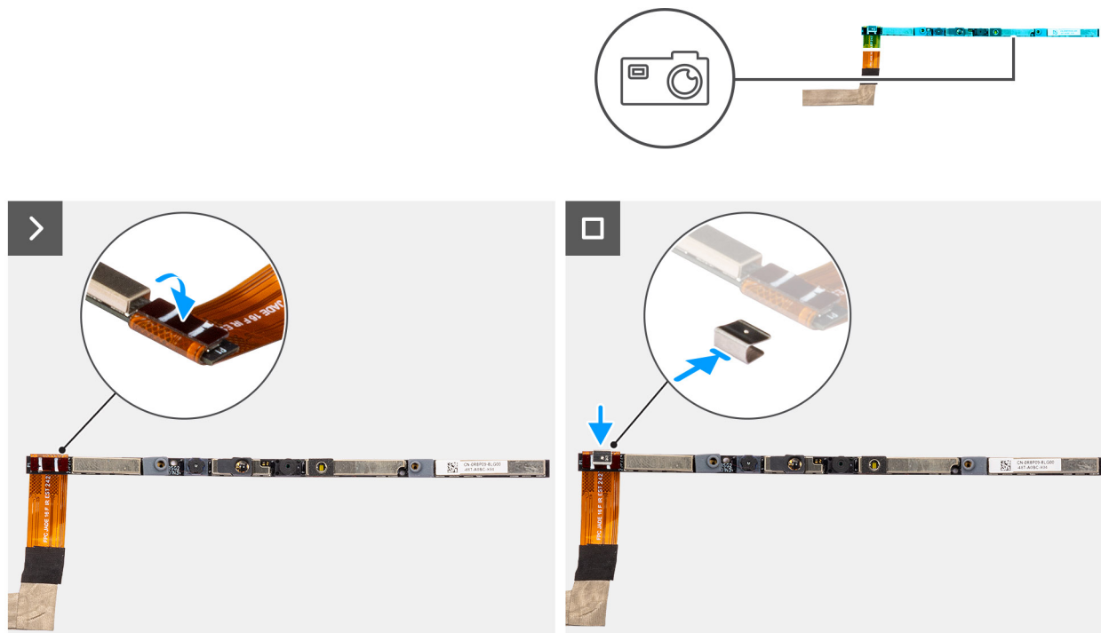
Figure 83. Installation de la caméra
