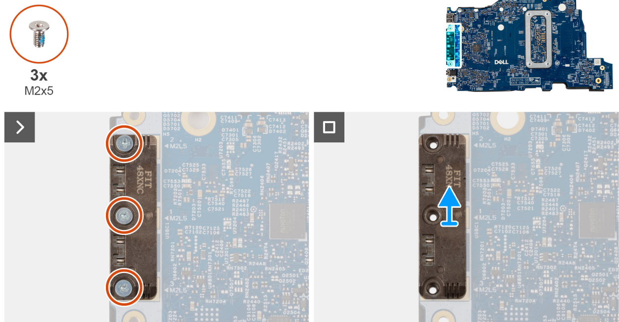
Figure 48. Retrait du module USB-C
