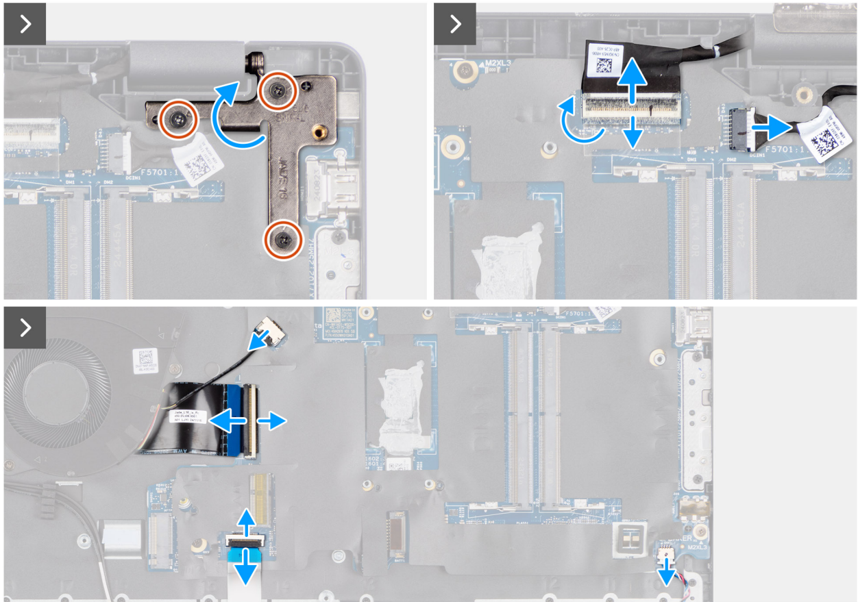
Figure 43. Retrait de la carte système
