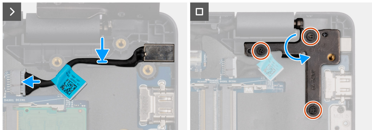
Figure 33. Installation du port de l'adaptateur secteur
