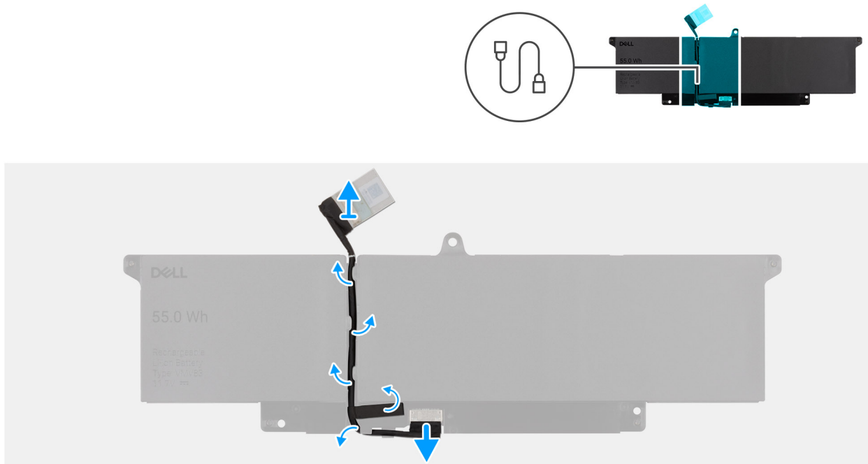
Figure 19. Retrait du câble de la batterie
