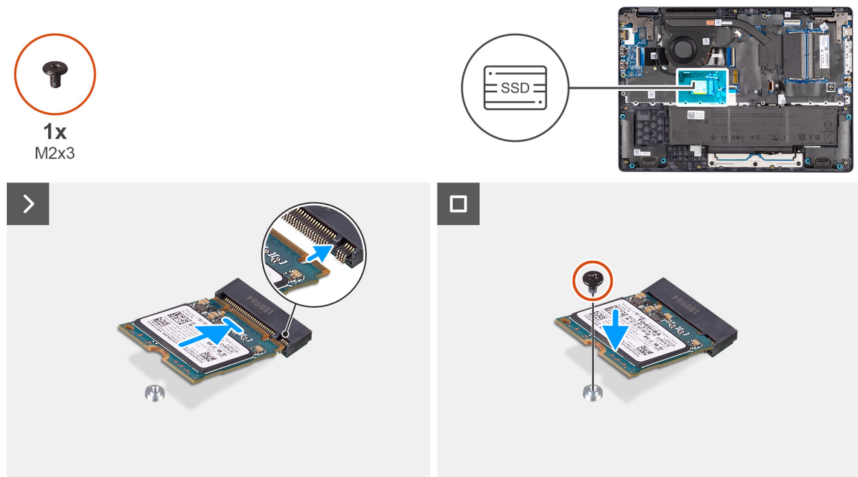
Figure 24. Installation du module SSD
