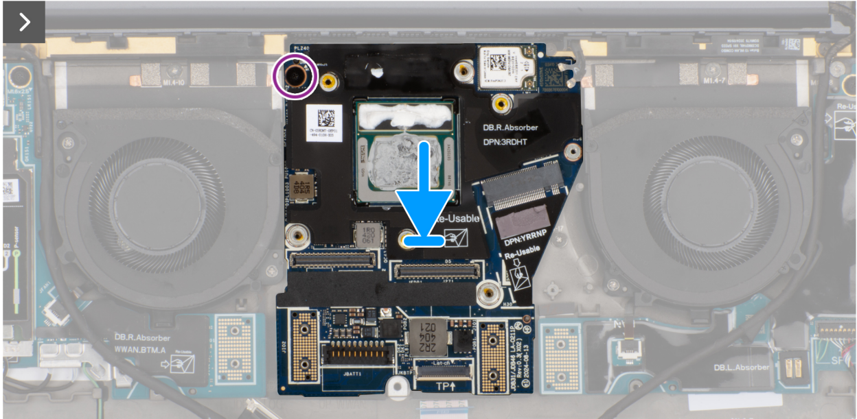
Figure 69. Installation de la carte système
