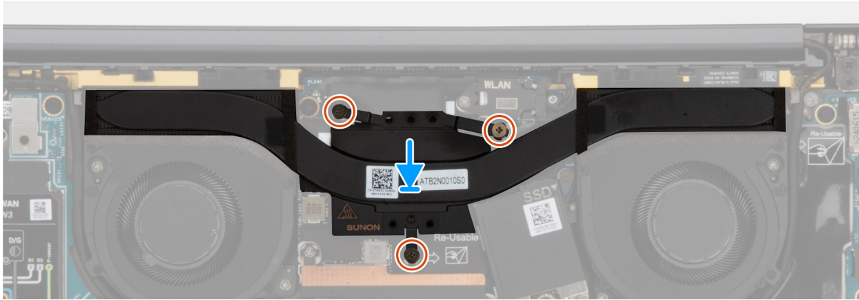
Figure 39. Installation du dissipateur de chaleur
