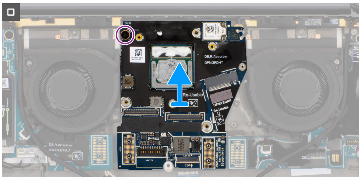
Figure 66. Retrait de la carte système
