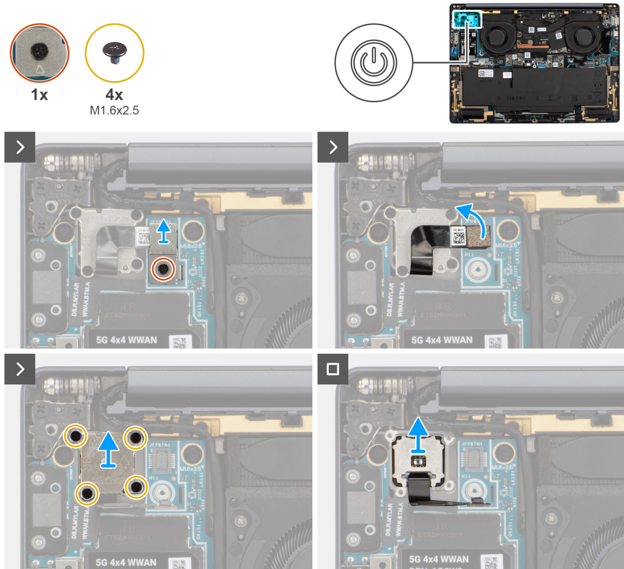
Figure 56. Retrait du bouton d'alimentation
