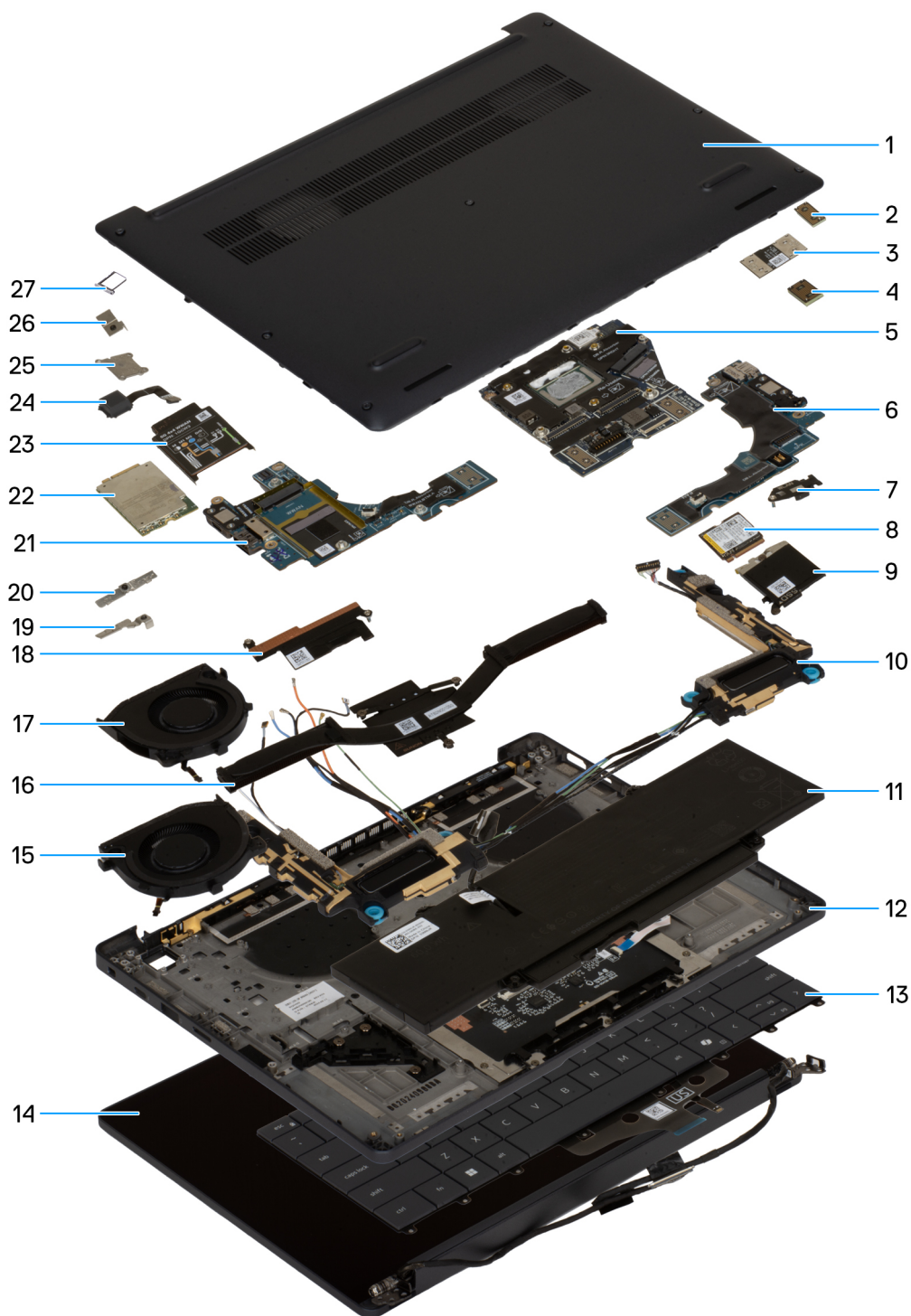
Figure 11. Composants majeurs de votre système/vue éclatée
