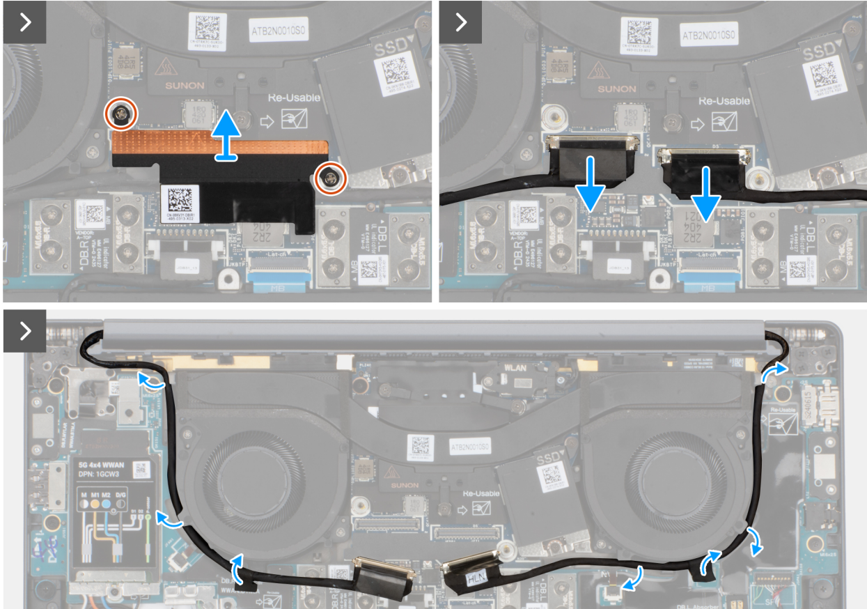
Figure 58. Débranchement des câbles de l'écran et de la caméra
