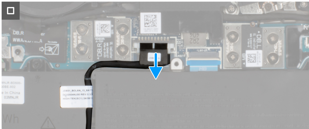
Figure 18. Déconnectez de la carte système le câble de la batterie
