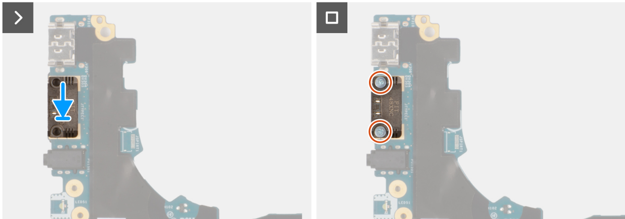
Figure 55. Installation du module USB-C droit
