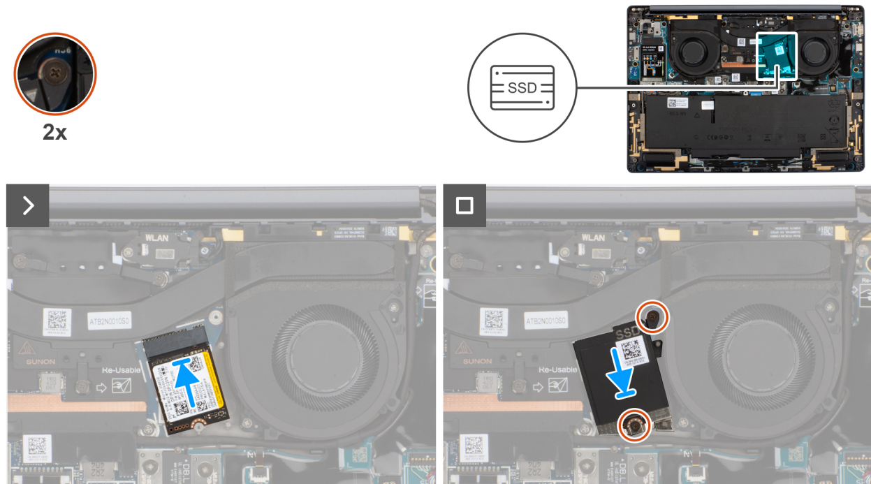
Figure 27. Installation de la carte SSD
