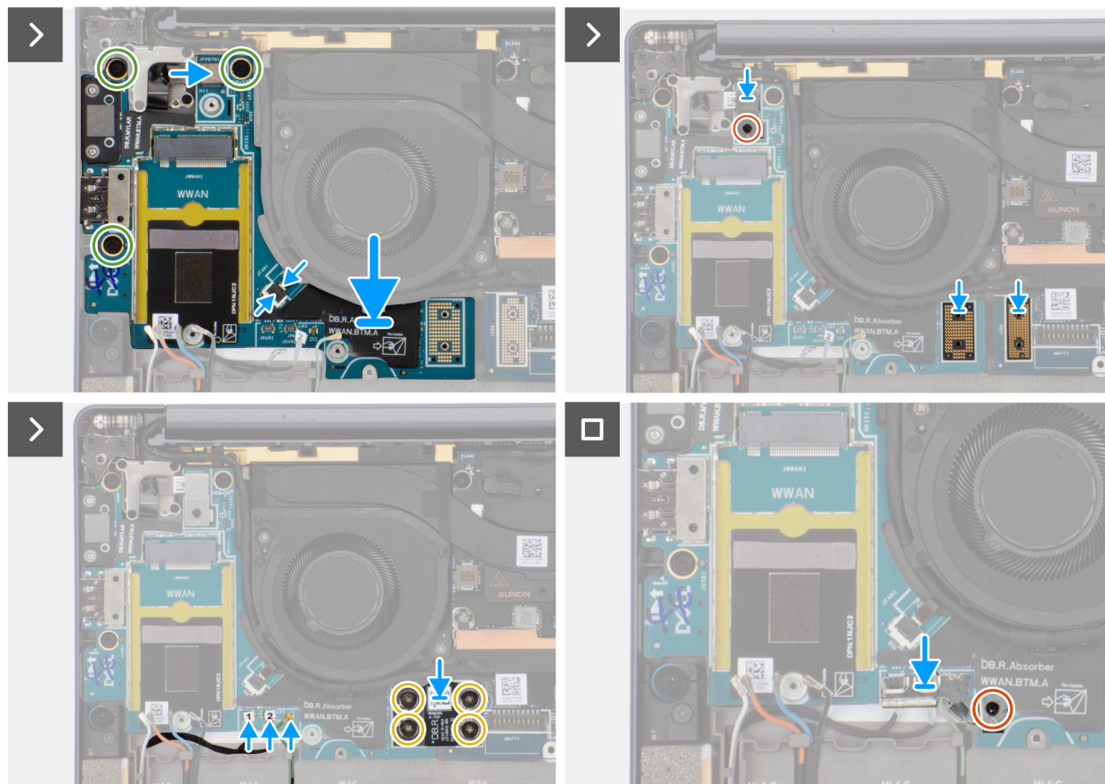
Figure 50. Installation de la carte d'E/S droite (avec WWAN)
