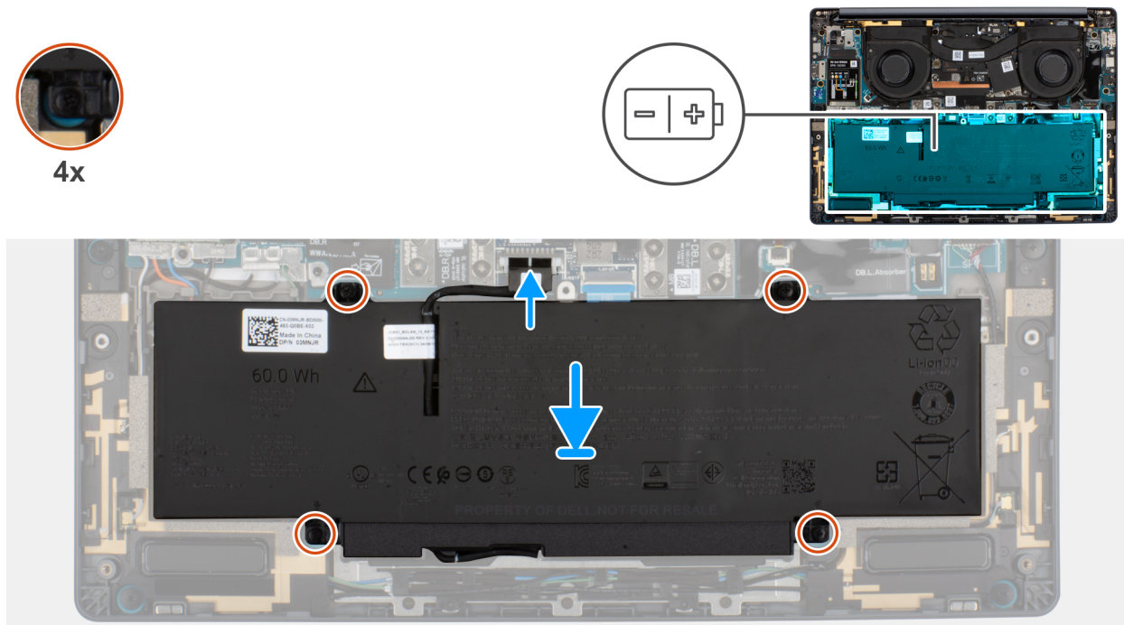
Figure 23. Installation de la batterie
