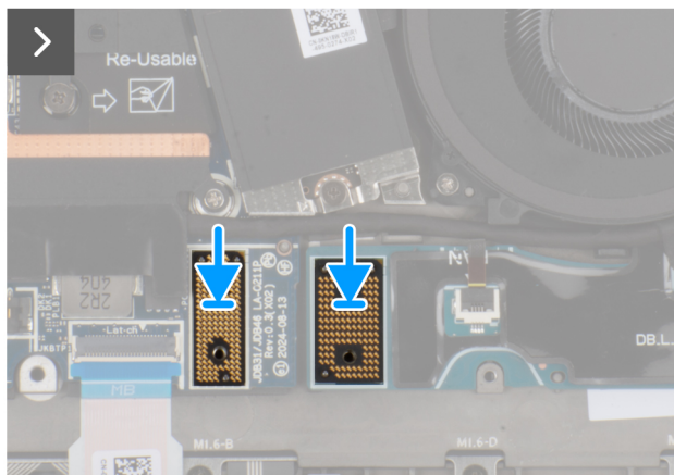
Figure 42. Installation de la carte d'E/S gauche
