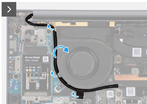
Figure 32. Retrait du ventilateur droit
