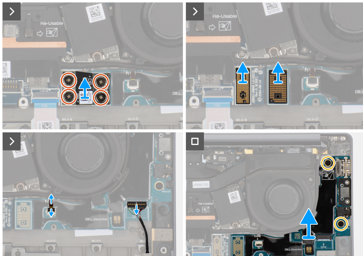
Figure 40. Retrait de la carte d'E/S gauche
