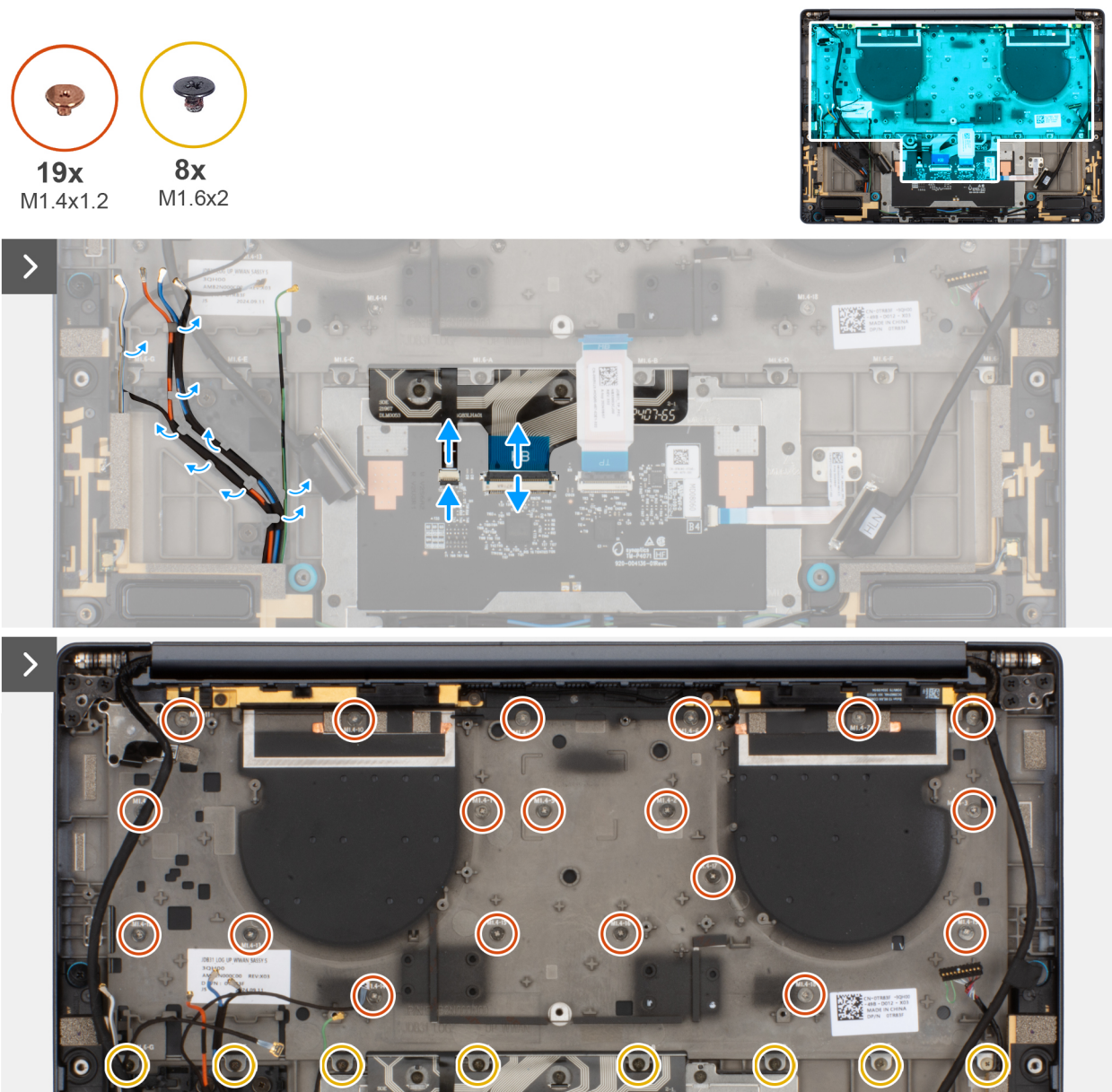
Figure 73. Retrait de l'assemblage du clavier
