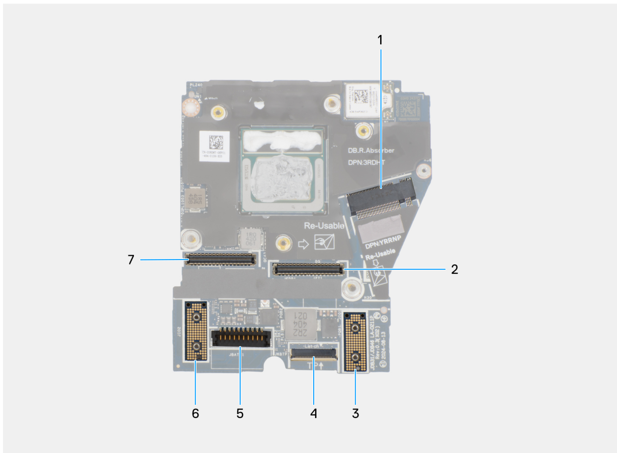
Figure 63. Légendes de la carte système
