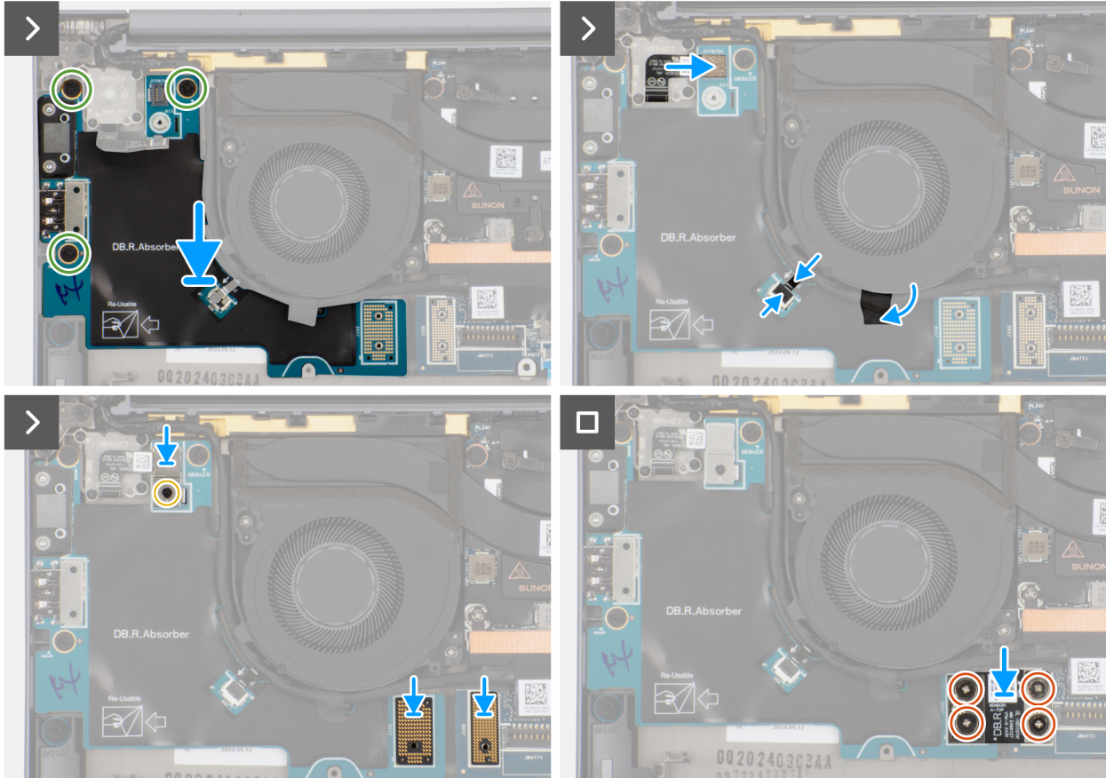
Figure 46. Installation de la carte d'E/S droite (sans antennes WWAN)
