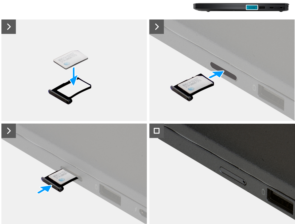
Figure 15. Installation de la carte nano SIM
