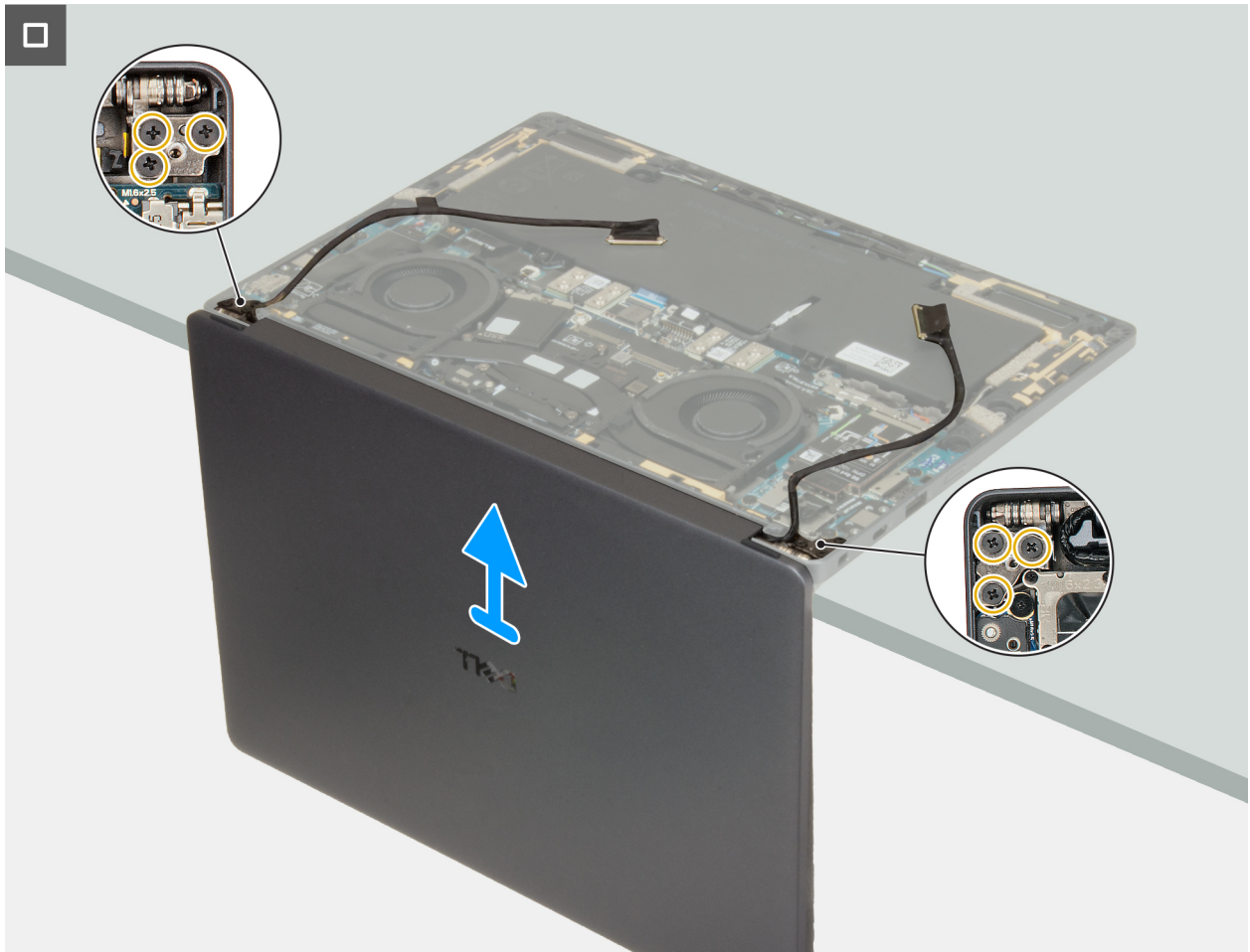
Figure 59. Retrait de l'assemblage d'écran
