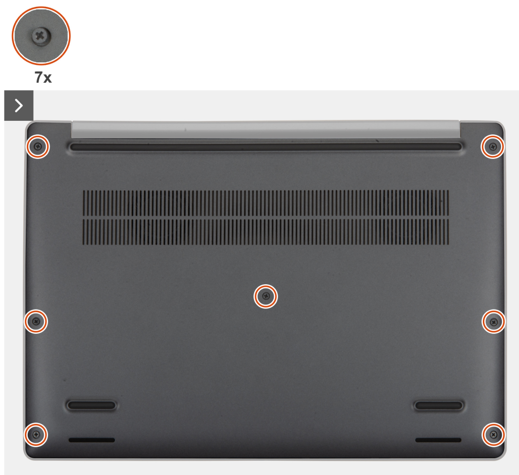
Figure 16. Desserrage des vis imperdables
