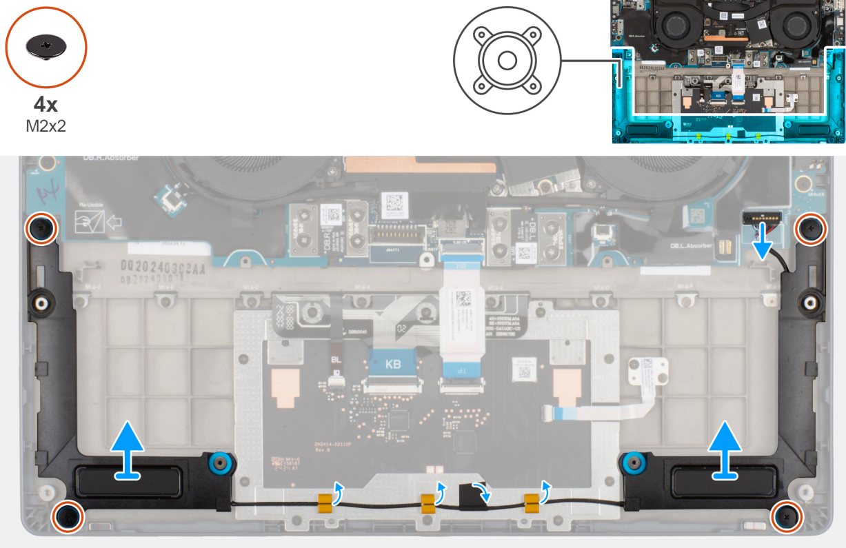
Figure 34. Retrait des haut-parleurs sans antennes (configuration WLAN)
