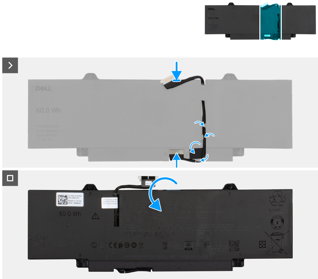
Figure 25. Branchement et installation du câble de la batterie
