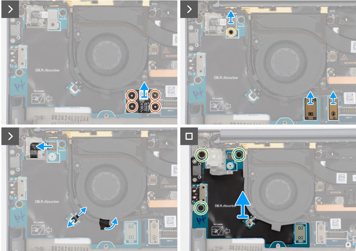
Figure 44. Retrait de la carte d'E/S droite (sans antennes WWAN)
