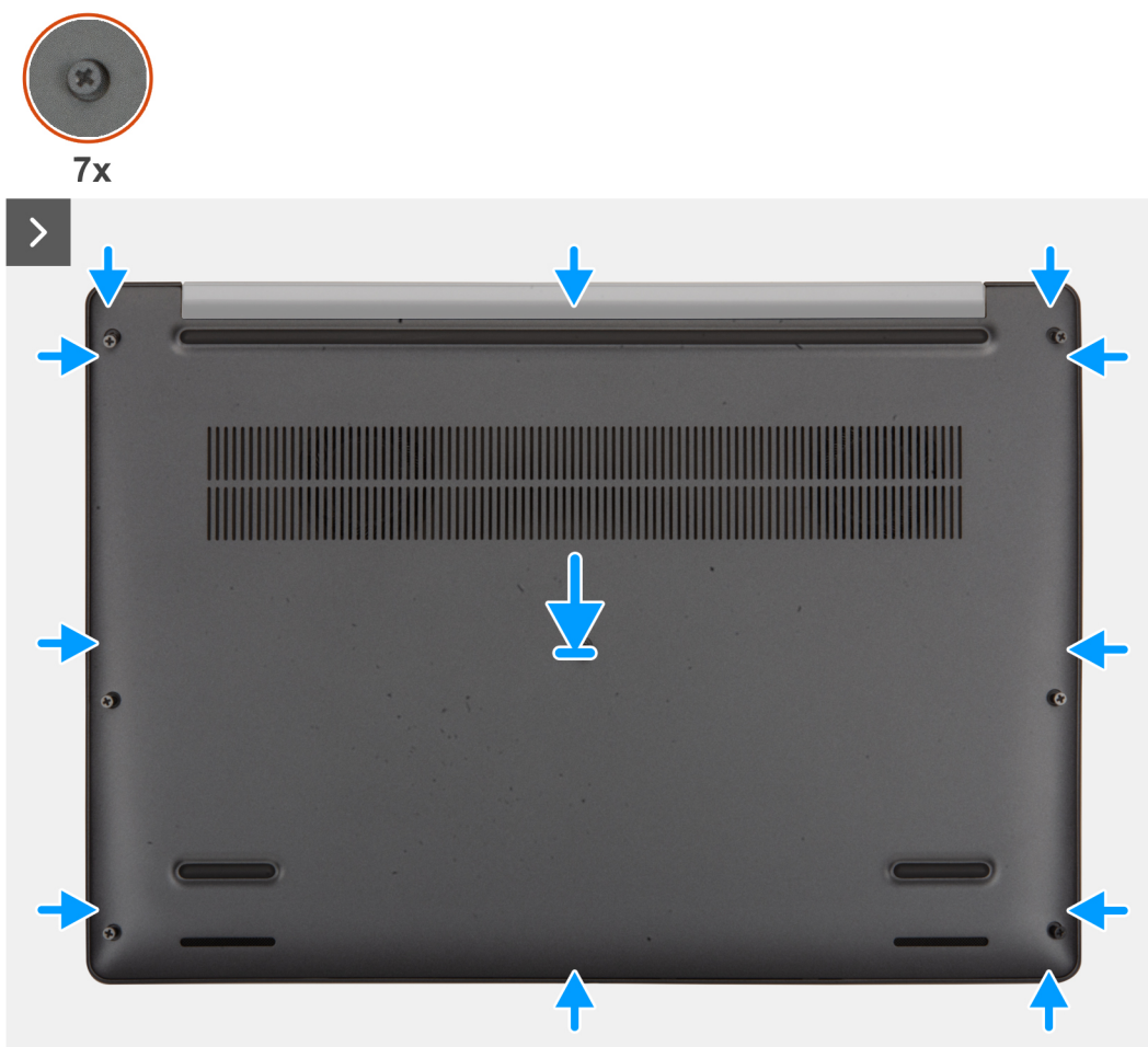
Figure 20. Installation du cache de fond
