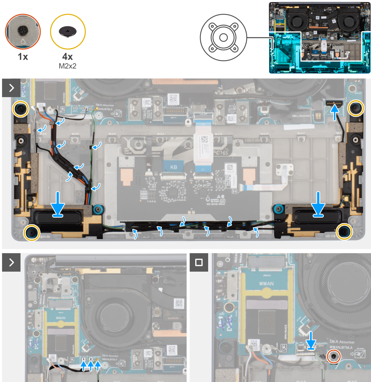
Figure 37. Installation des haut-parleurs avec antennes (configuration WWAN)
