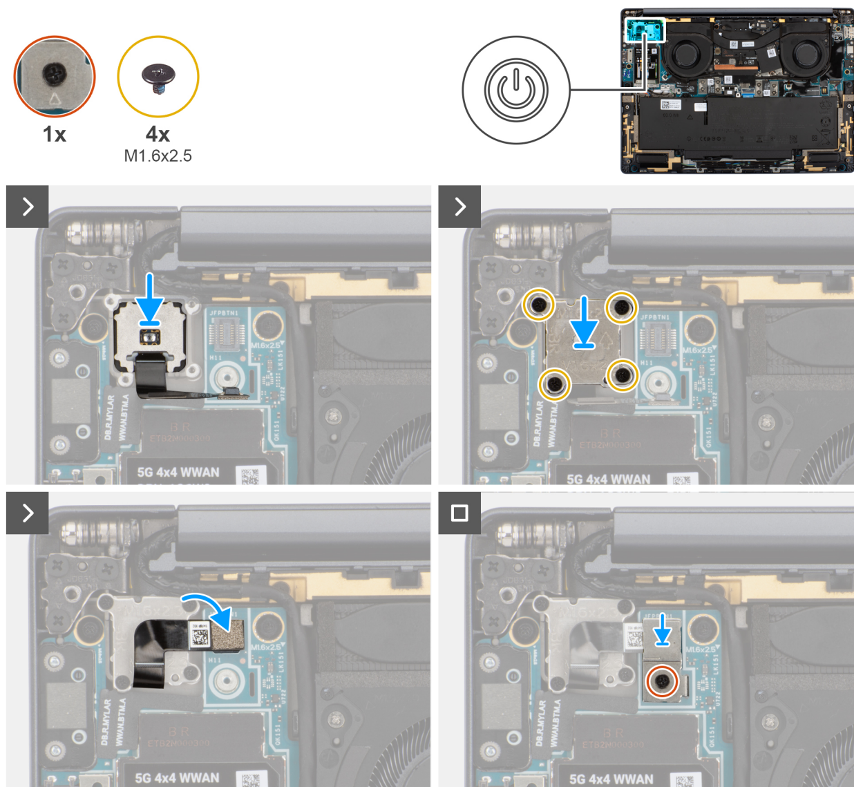
Figure 57. Installation du bouton d'alimentation
