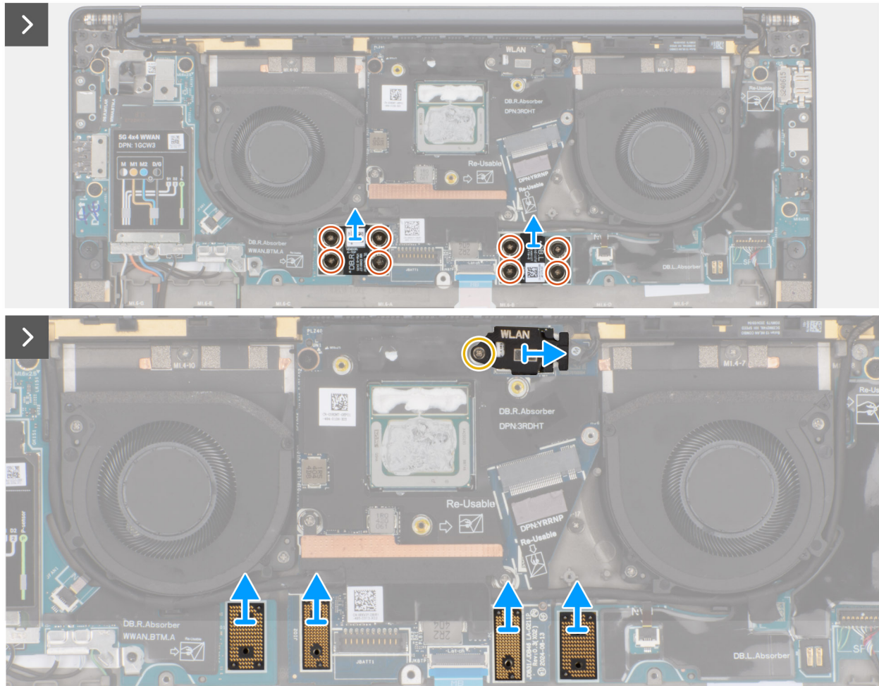
Figure 64. Retrait de la carte système
