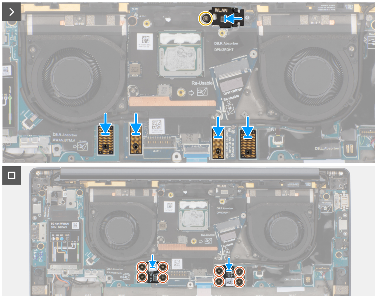
Figure 71. Installation de la carte système
