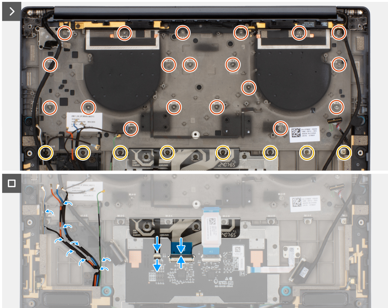
Figure 76. Installation de l'assemblage du clavier
