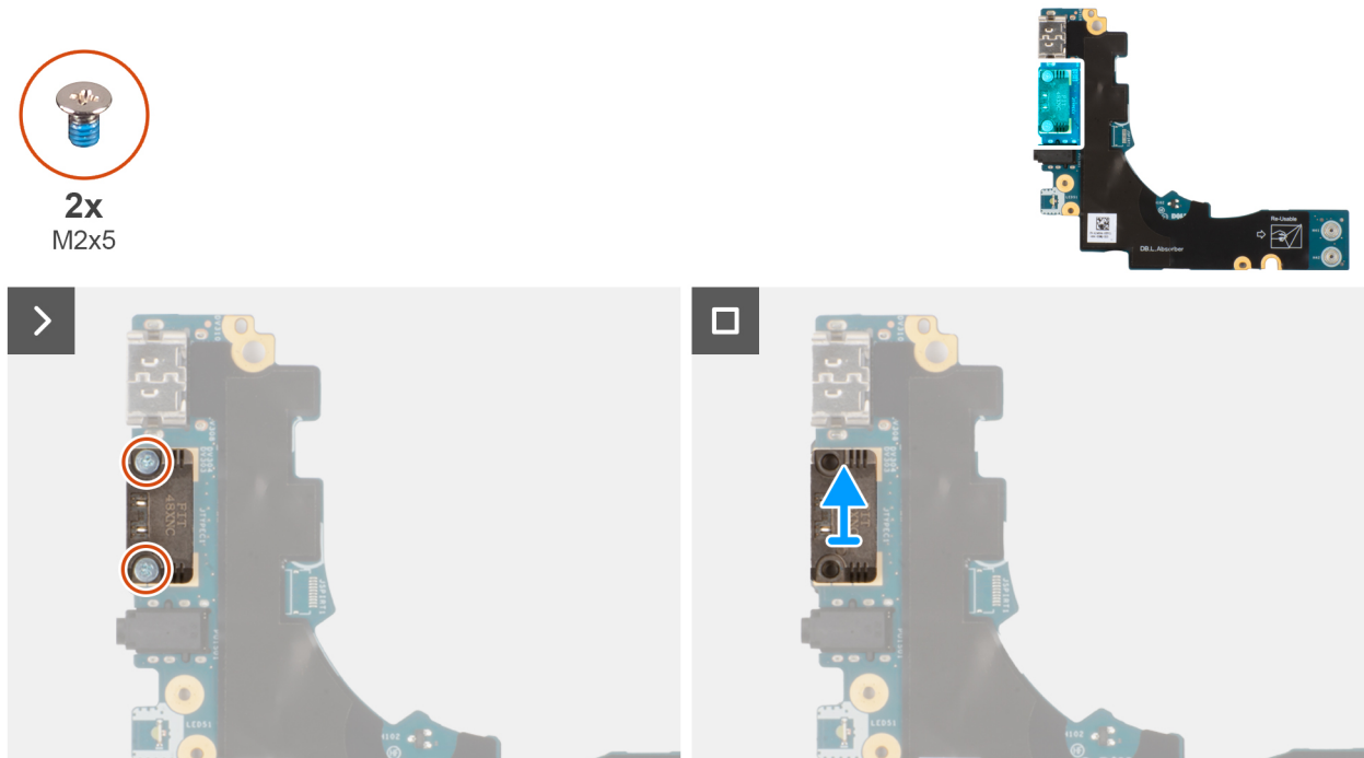
Figure 54. Retrait du module USB-C droit
