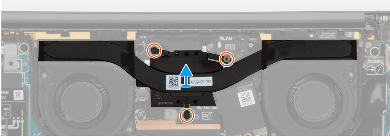
Figure 38. Retrait du dissipateur de chaleur
