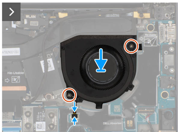
Figure 31. Installation du ventilateur gauche
