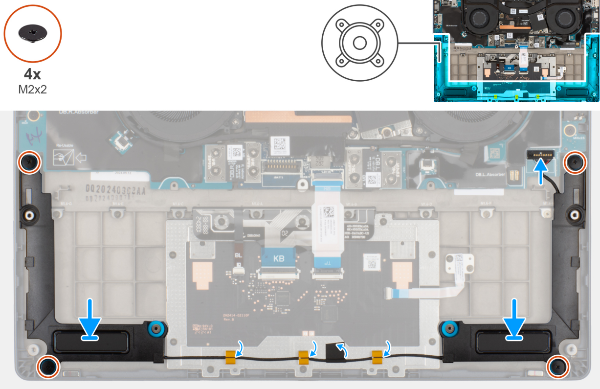
Figure 35. Installation des haut-parleurs (sans WWAN)
