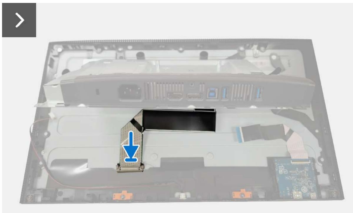
Figure 12. Installer le blindage métallique
