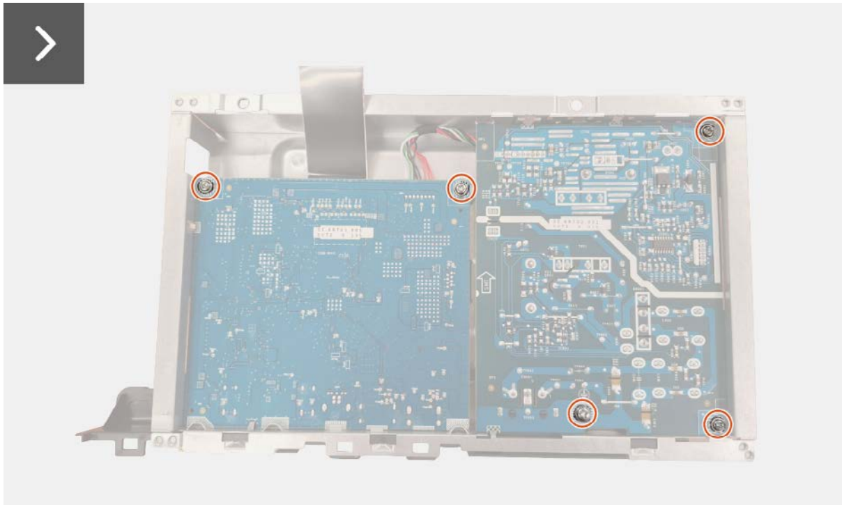
Figure 20. Installer la carte d'alimentation
