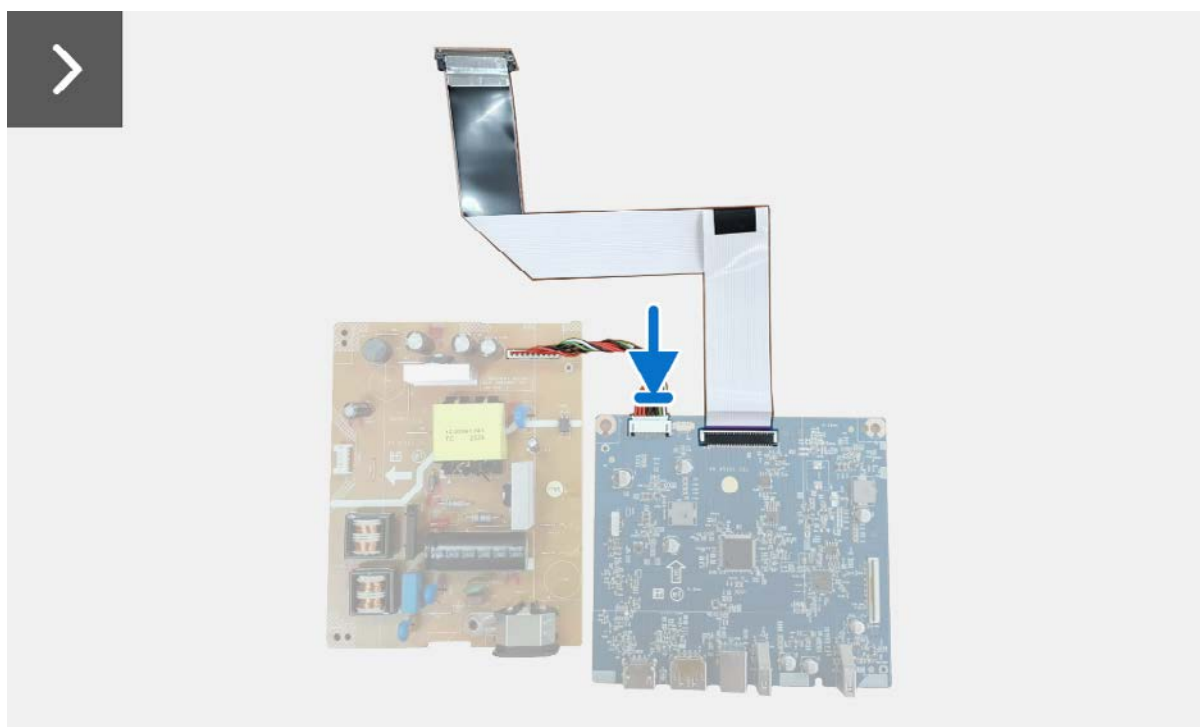
Figure 19. Installer la carte d'alimentation
