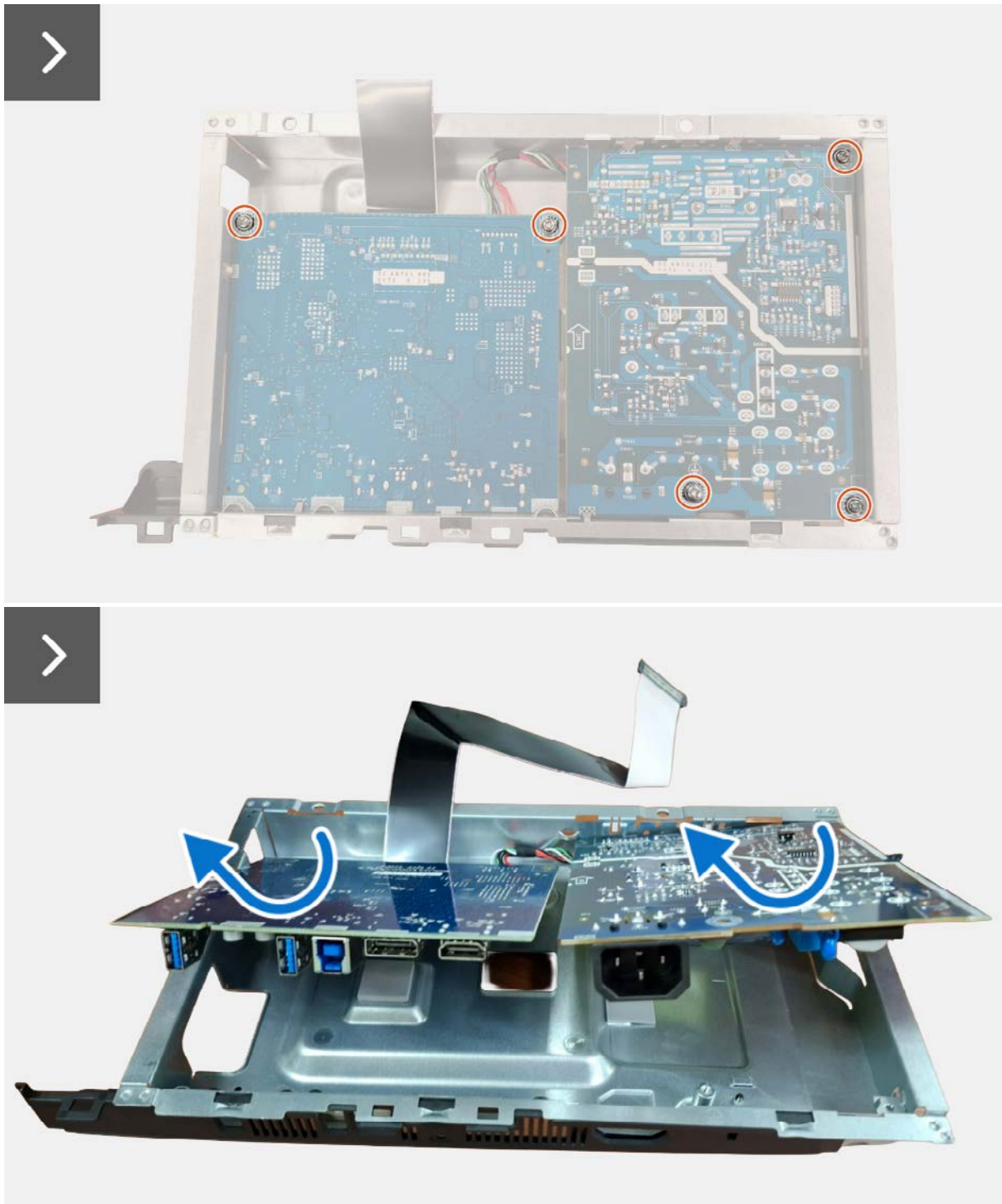
Figure 17. Retirer la carte d'alimentation
