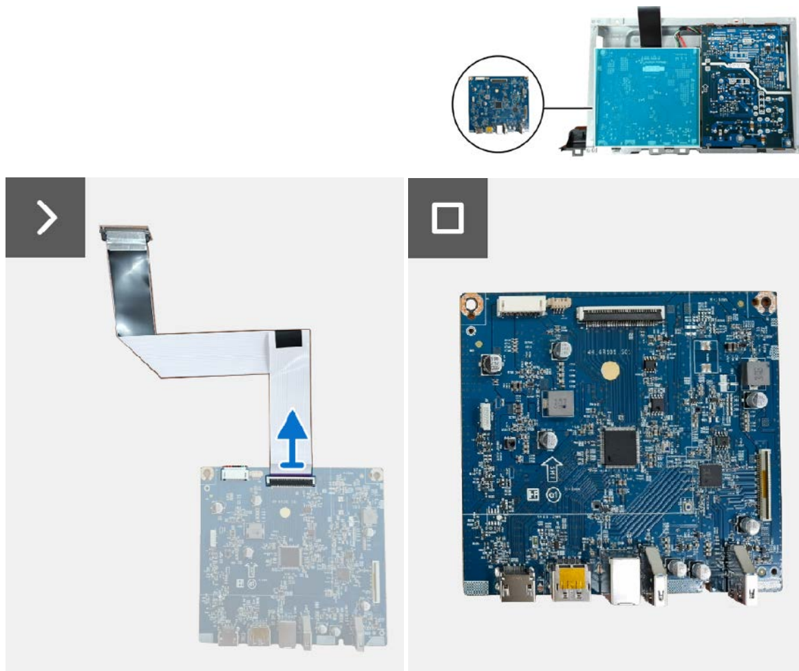
Figure 22. Retirer la carte d'interface
