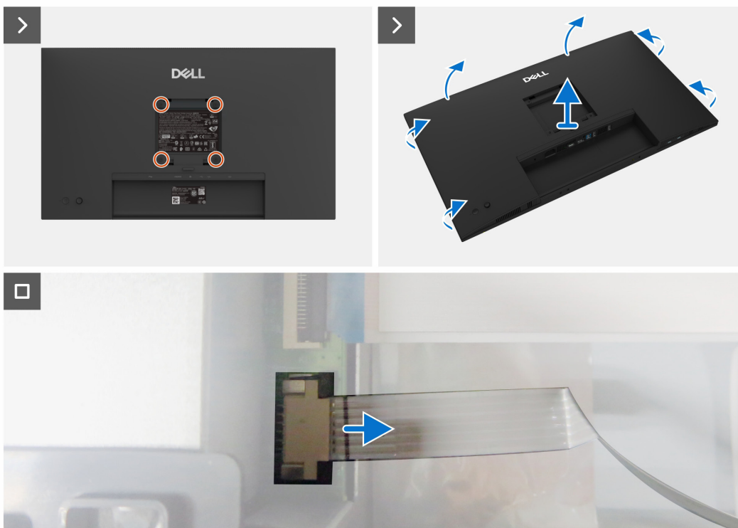
Figure 3. Retrait du couvercle arrière
