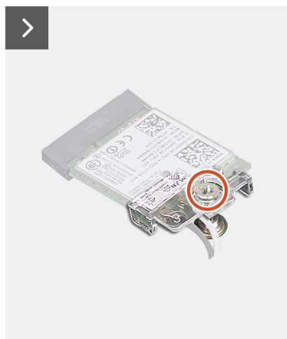
Abbildung 27. Installieren der Wireless-Karte
