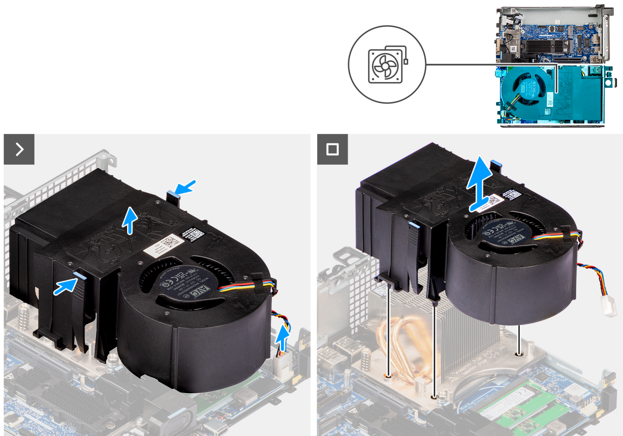
Abbildung 16. Entfernen des Systemlüfters
