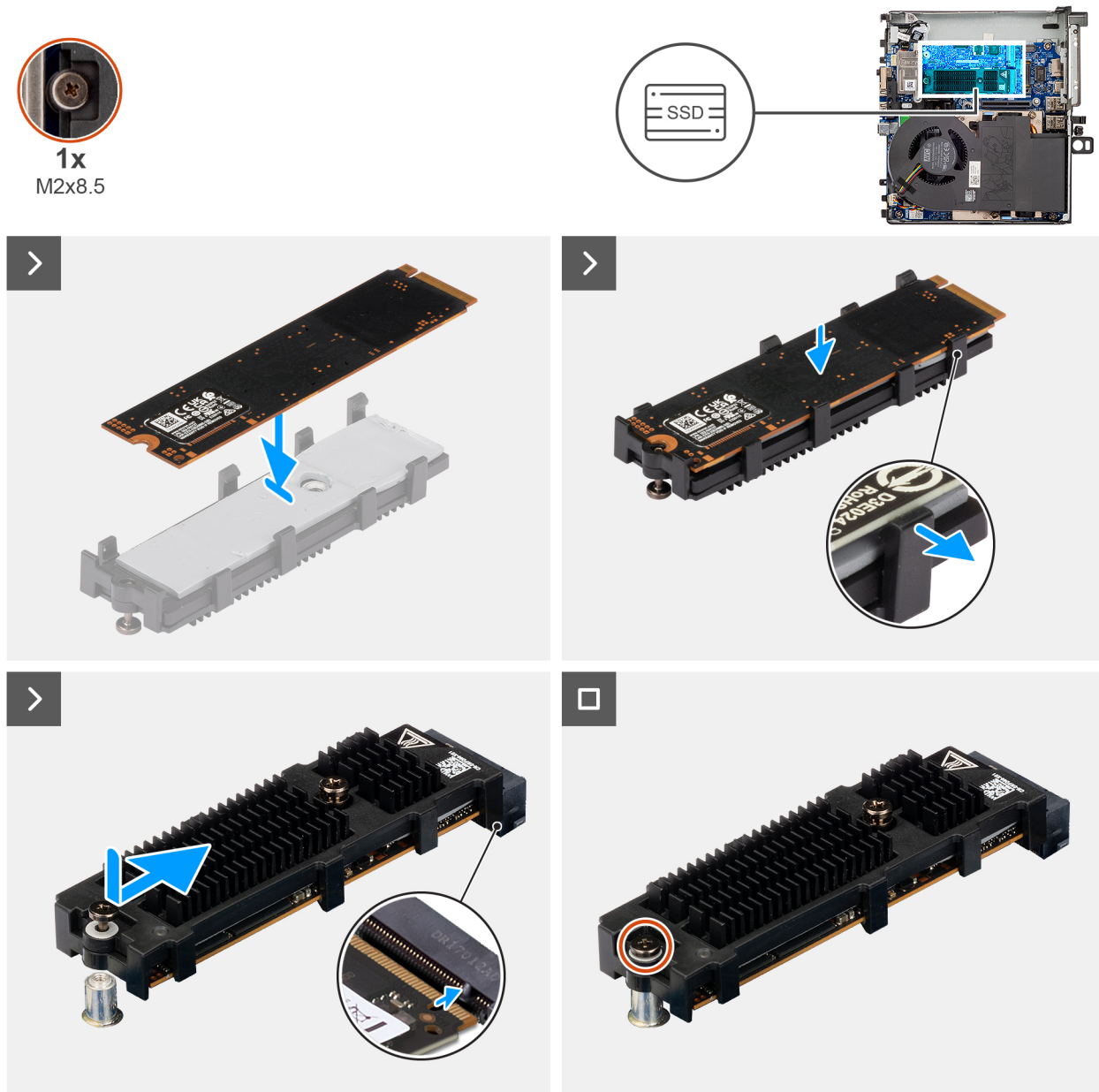
Abbildung 23. Einbauen des M.2-2280-PCIe-SSD-Laufwerks (Steckplatz 1)
