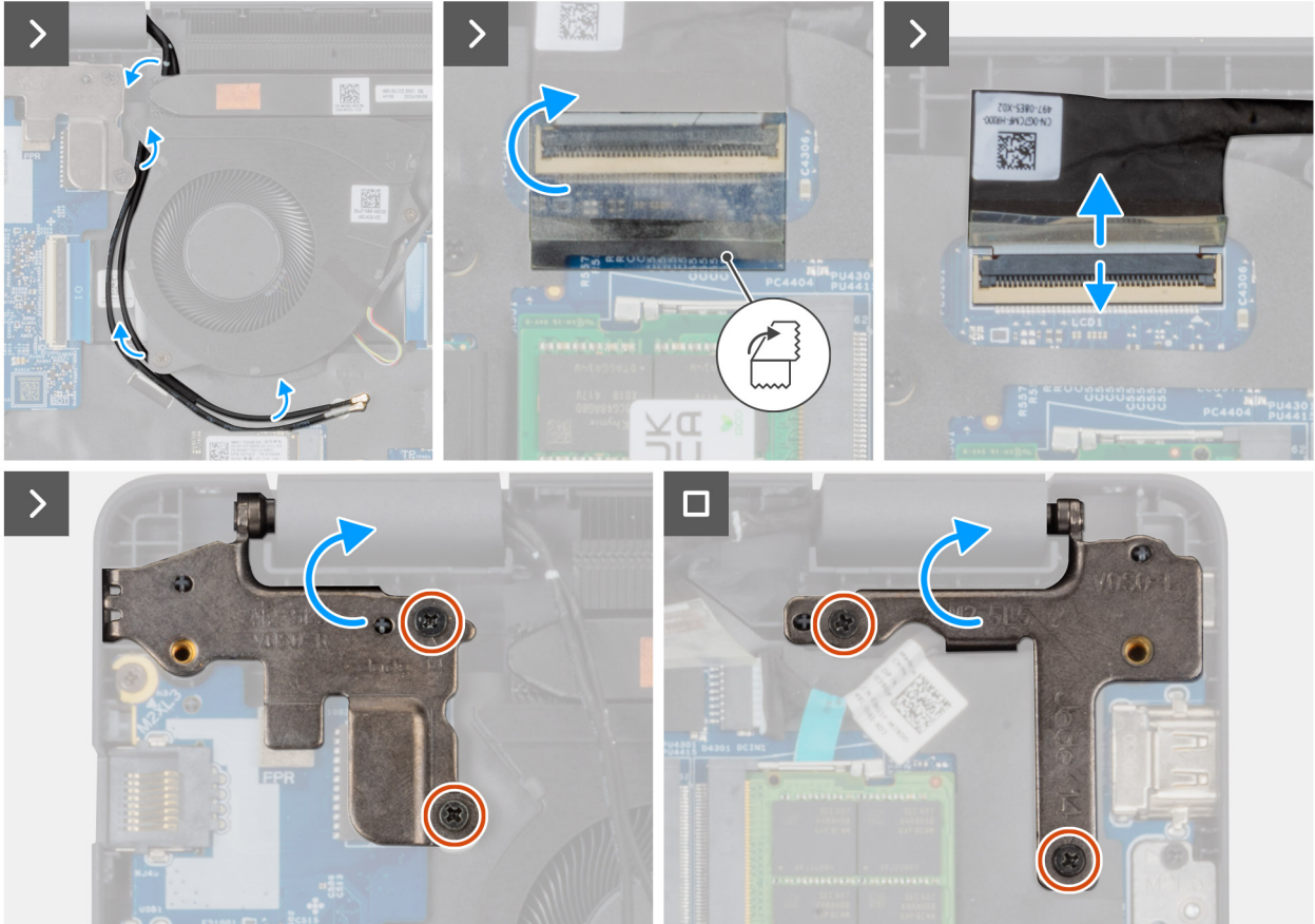
Abbildung 99. Entfernen der Bildschirmbaugruppe
