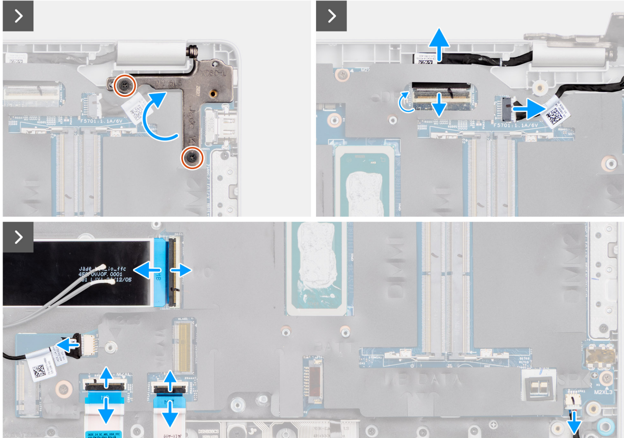
Abbildung 70. Entfernen der Systemplatine
