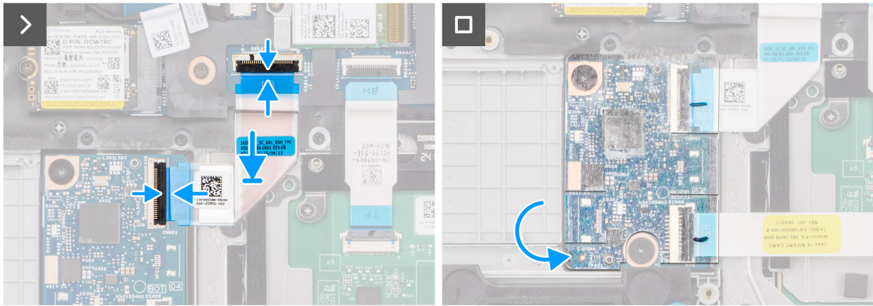
Abbildung 36. Einbauen des USH-Platinen-FPC
