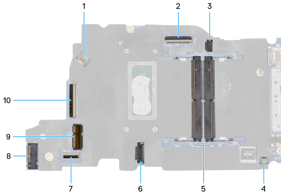
Abbildung 60. Hauptplattenanschlüsse
