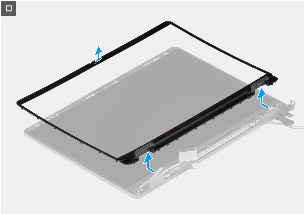
Abbildung 108. Entfernen der Bildschirmblende
