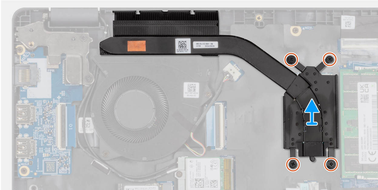
Abbildung 43. Kühlkörper entfernen
