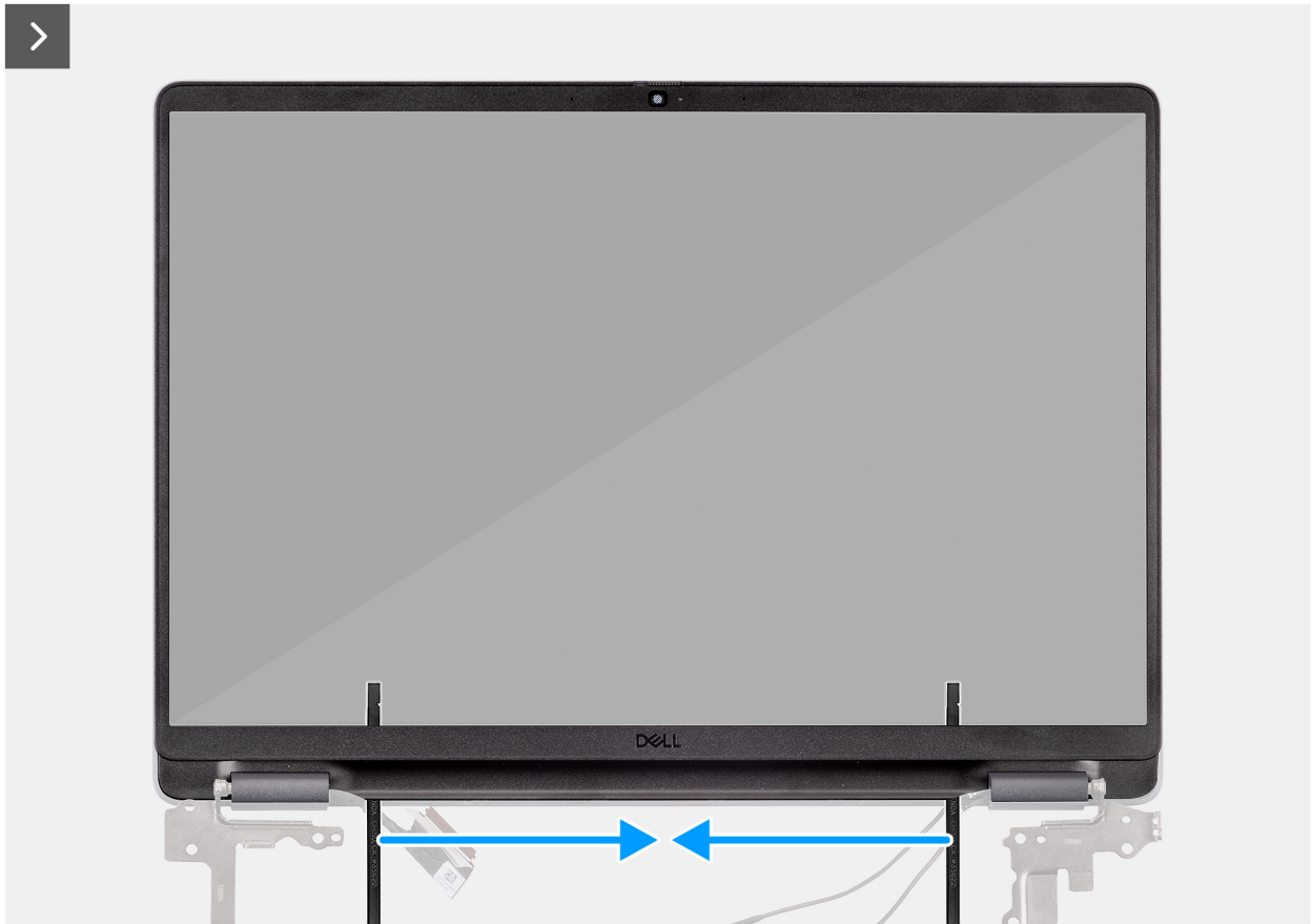
Abbildung 105. Entfernen der Bildschirmblende
