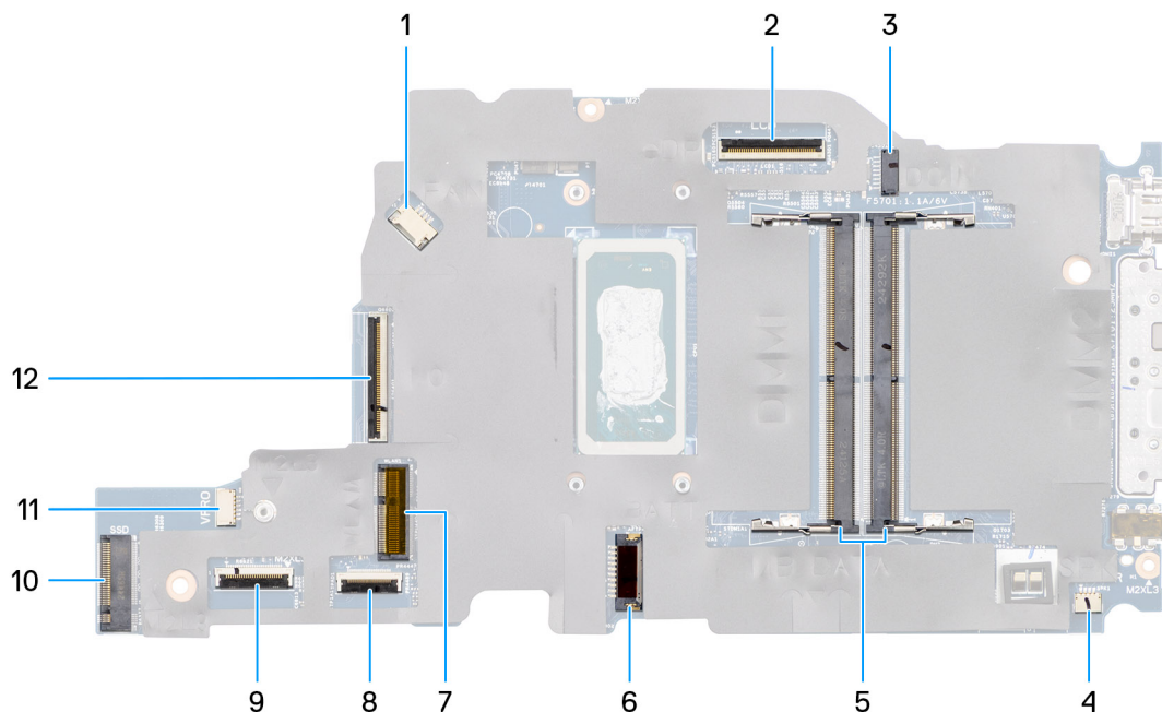
Abbildung 69. Hauptplattenanschlüsse
