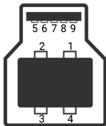
Figura 9. Conector USB Type-B
