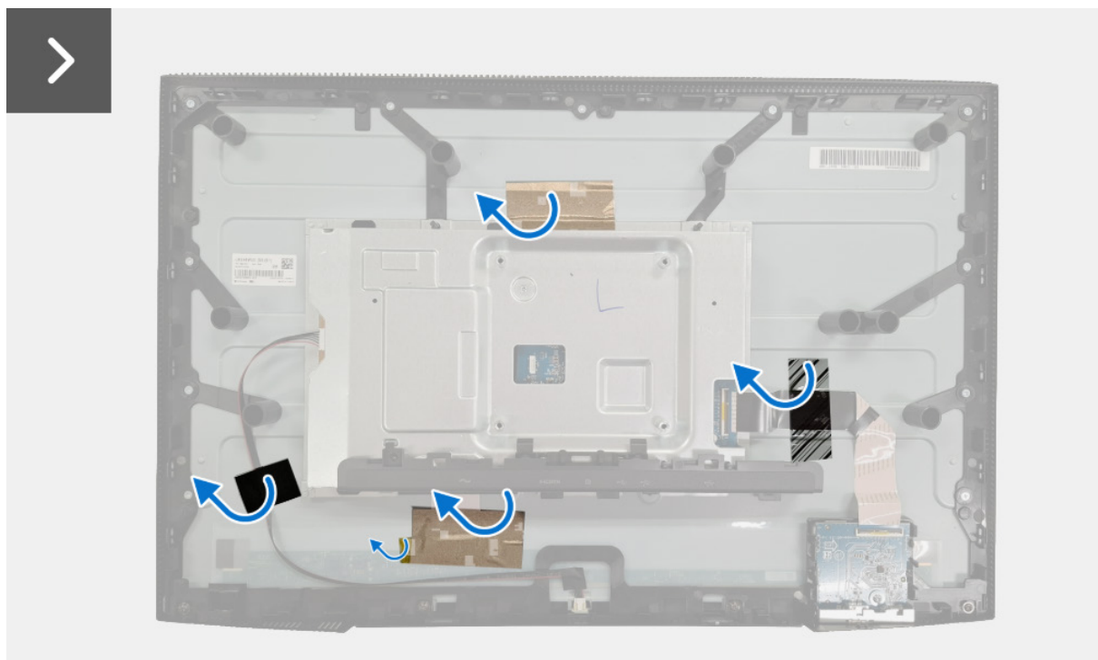
Figura 18. Retirar el protector metálico
