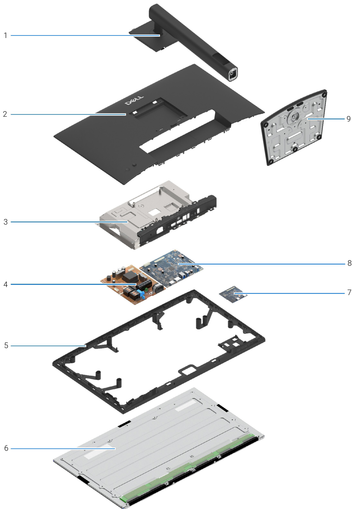
Figura 6. Componentes principales
