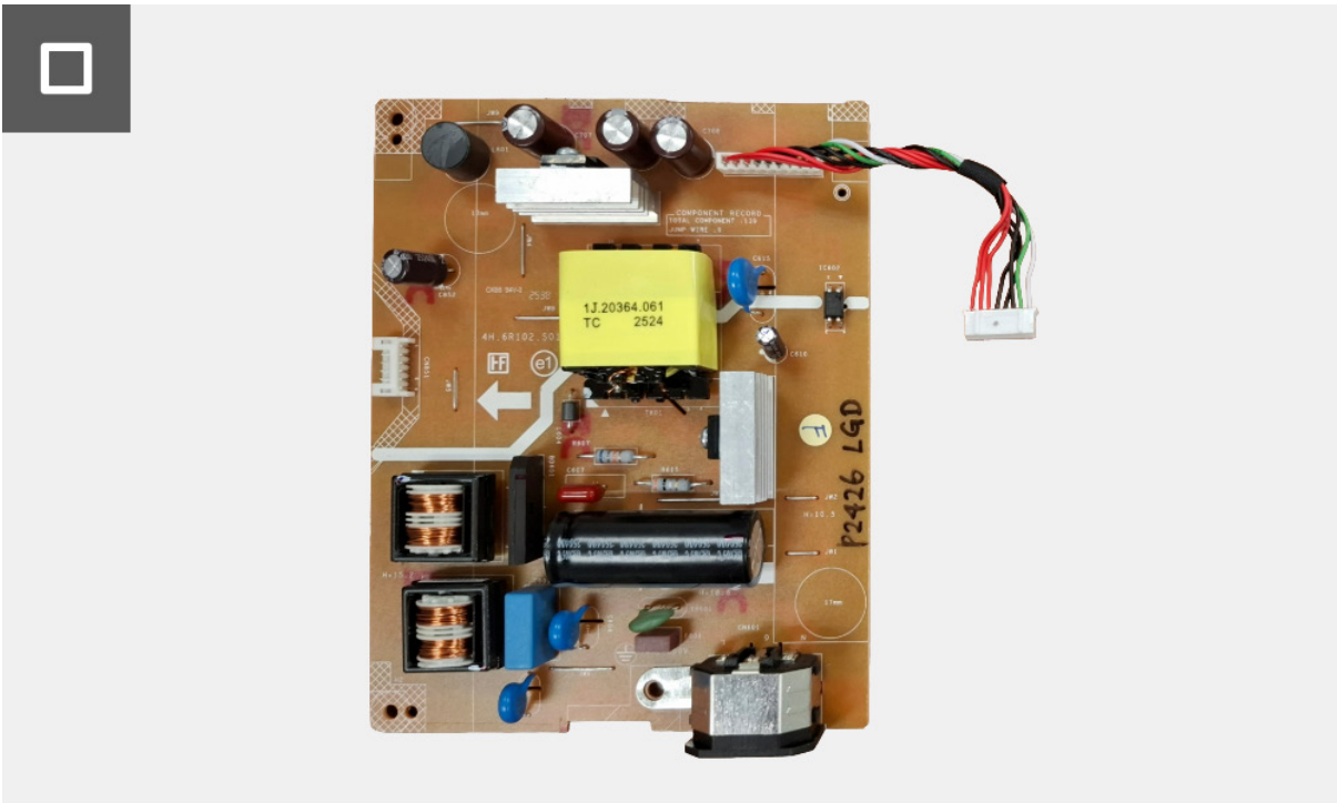
Figura 26. Retirar la placa de alimentación
