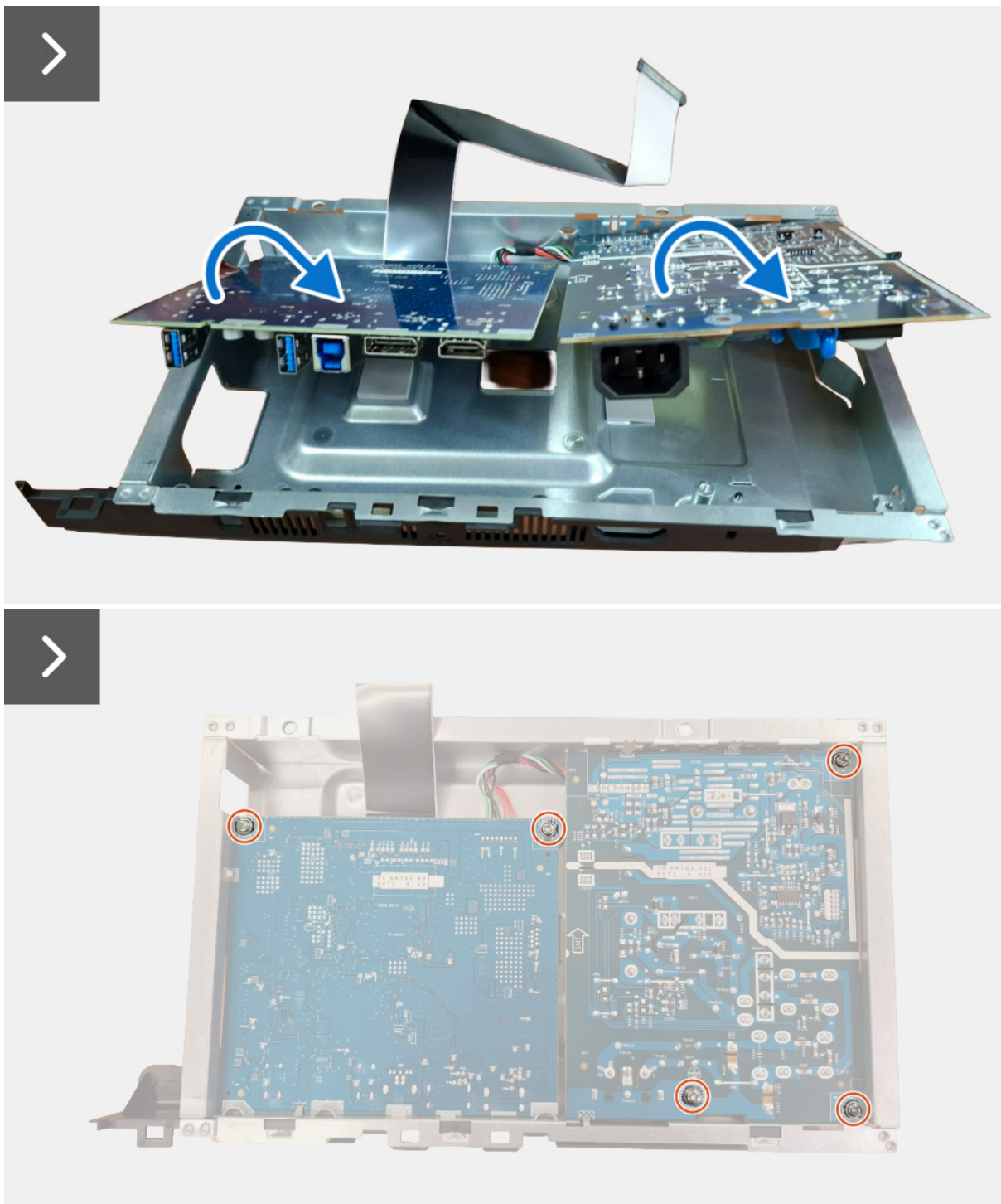
Figure 28. Installer la carte d'alimentation
