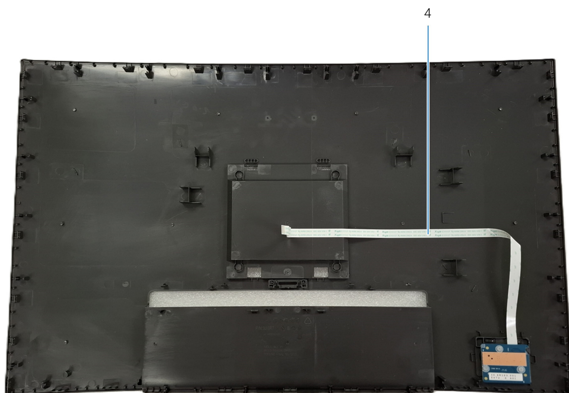
Figure 8. Connectivité du câblage sur le couvercle arrière de l'écran
