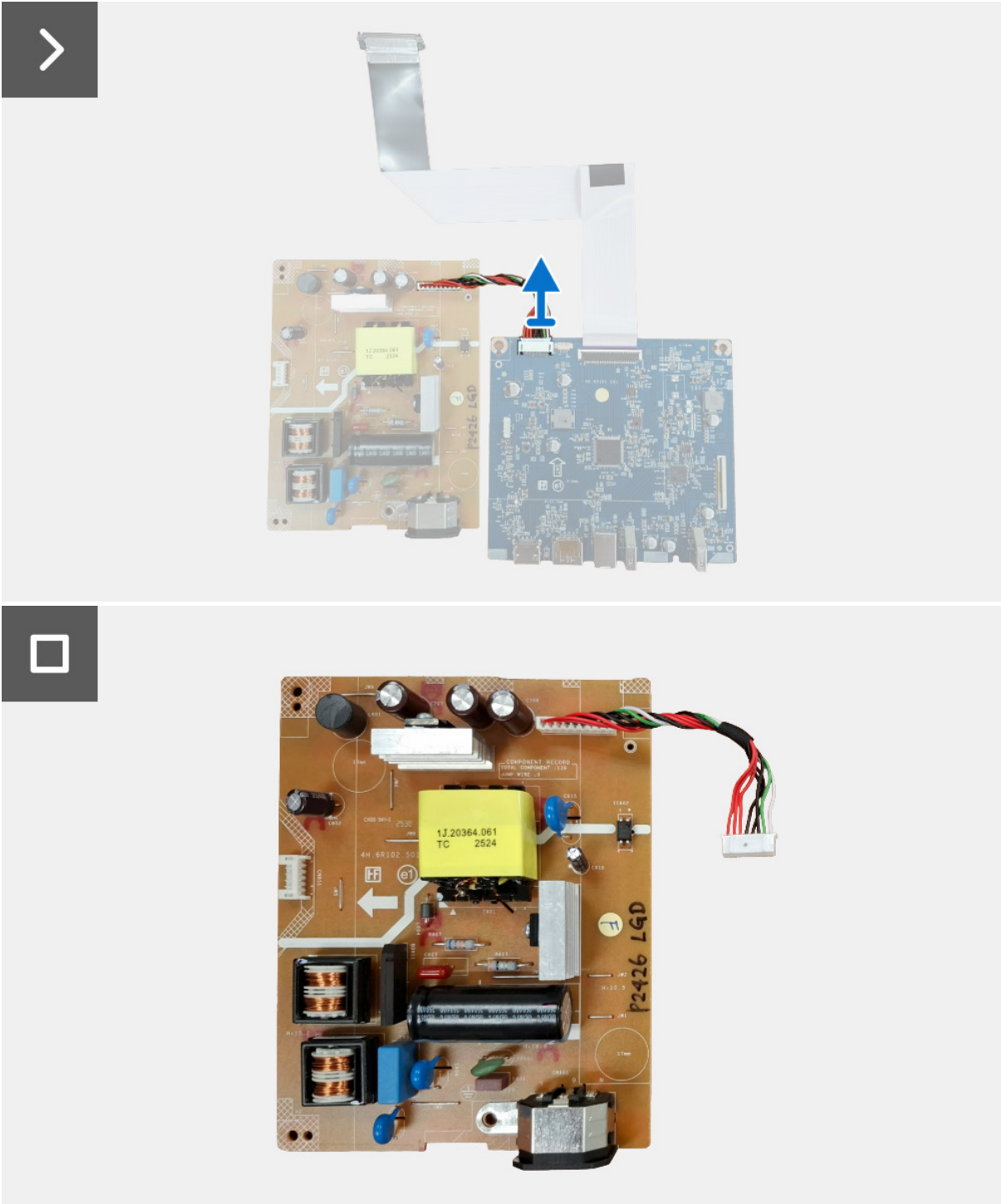
Figure 26. Retirer la carte d'alimentation
