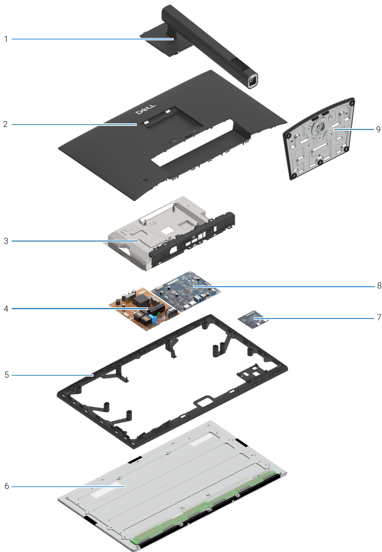
Figure 6. Principaux composants
