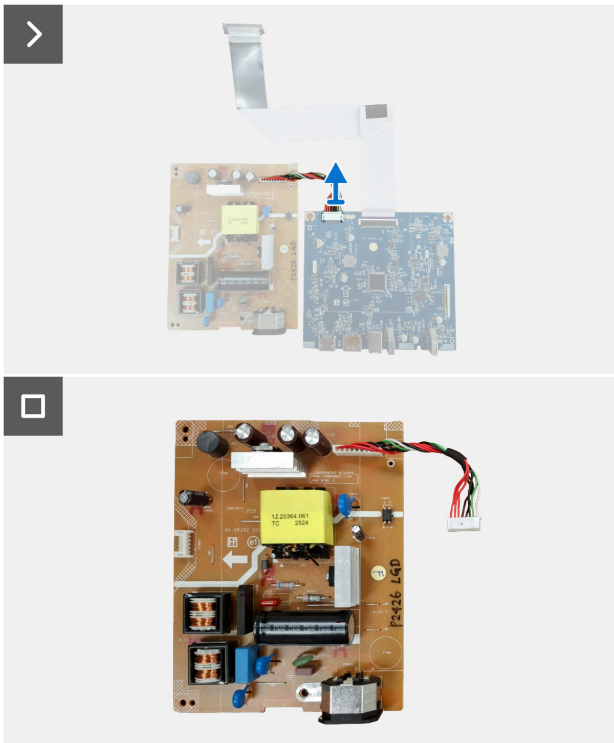
Figura 16. Retirar la placa de alimentación
