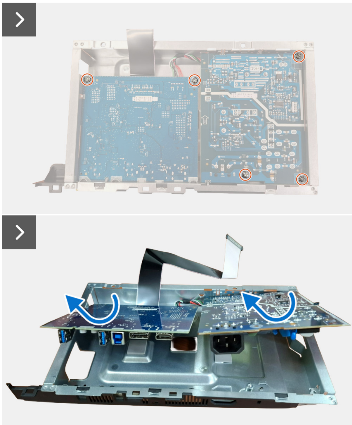
Figura 15. Retirar la placa de alimentación
