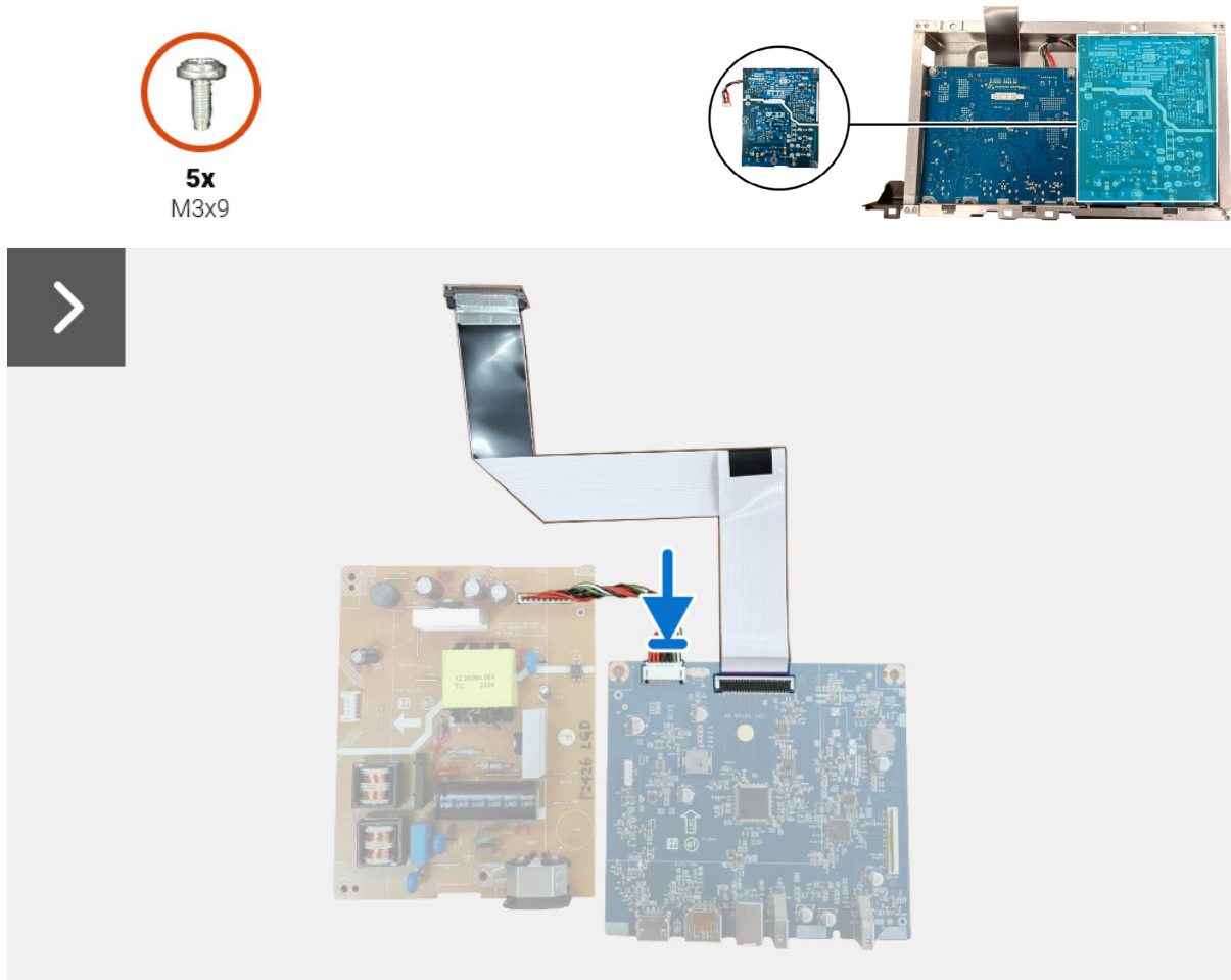
Figura 17. Instalar la placa de alimentación
