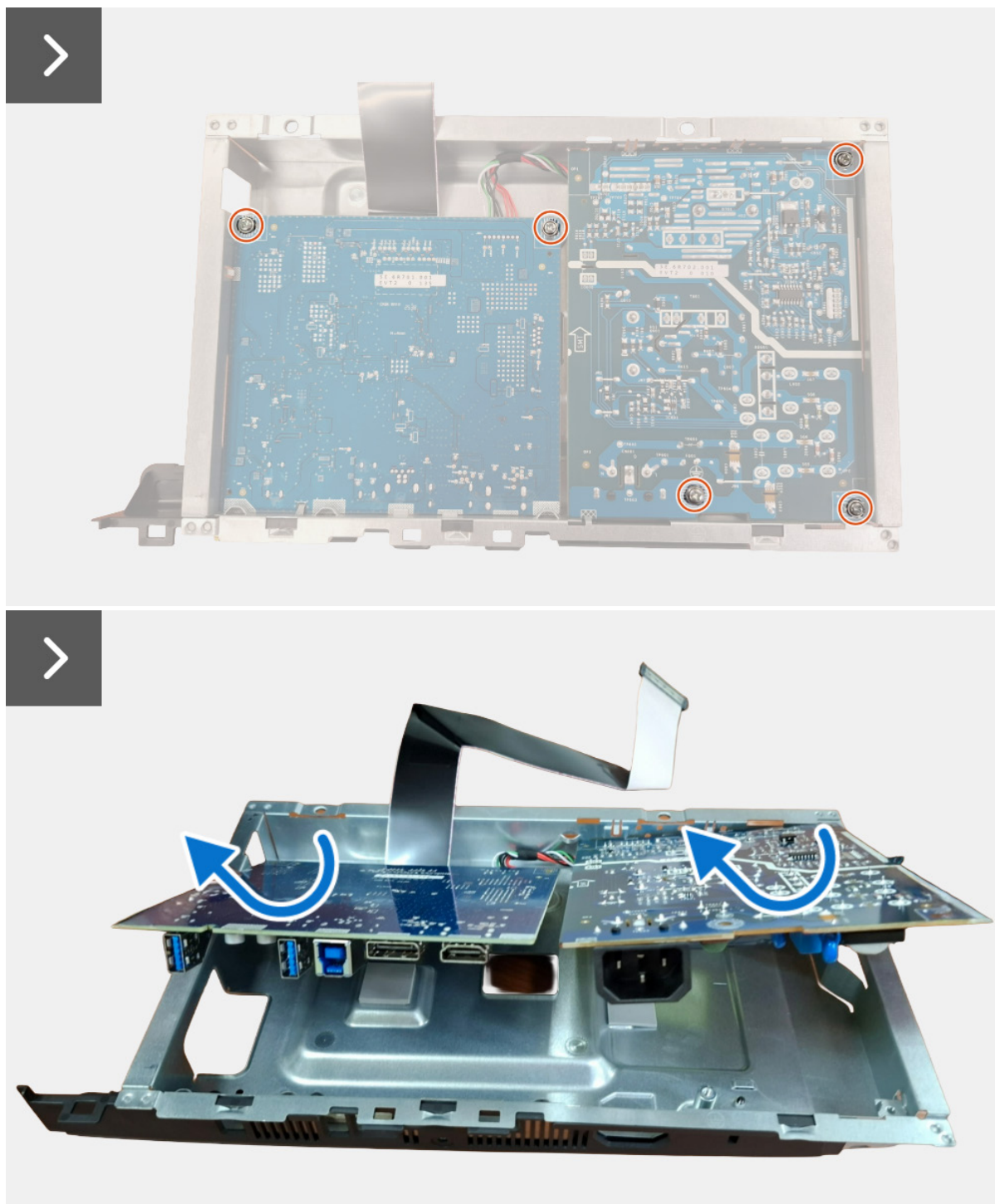
Figura 25. Retirar la placa de alimentación
