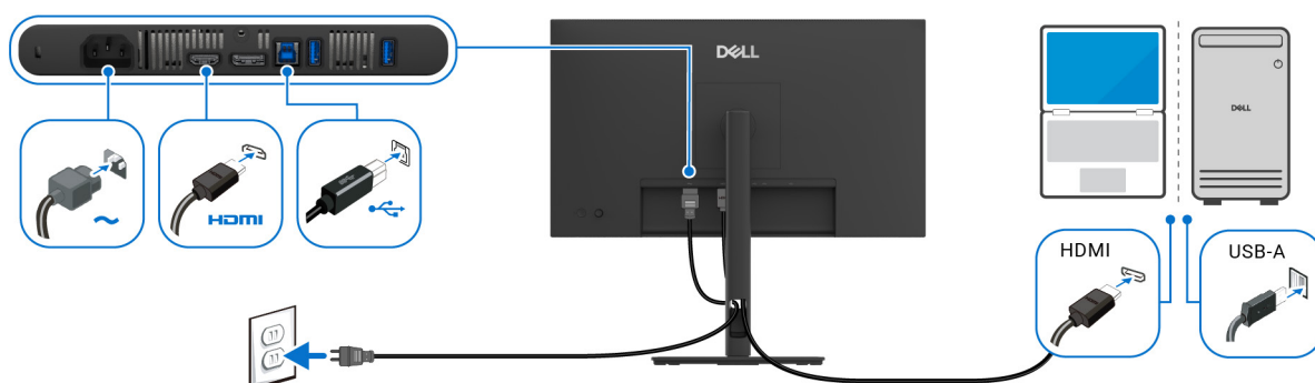
Figura 10. Conexión HDMI
