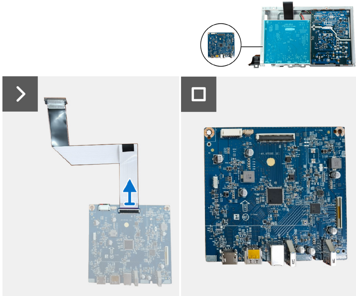
Figura 30. Retirar la placa de la interfaz
