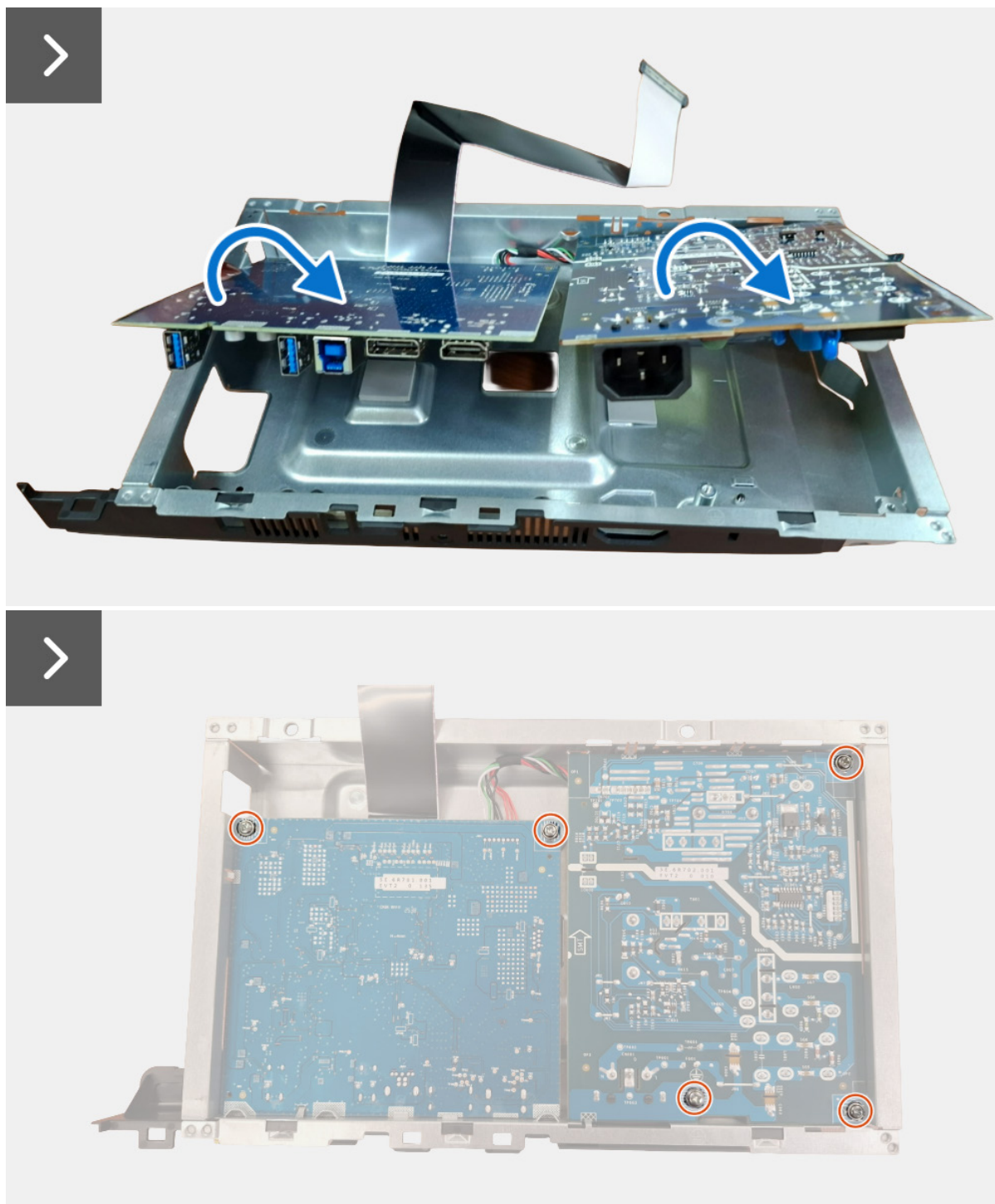
Figura 28. Instalar la placa de alimentación
