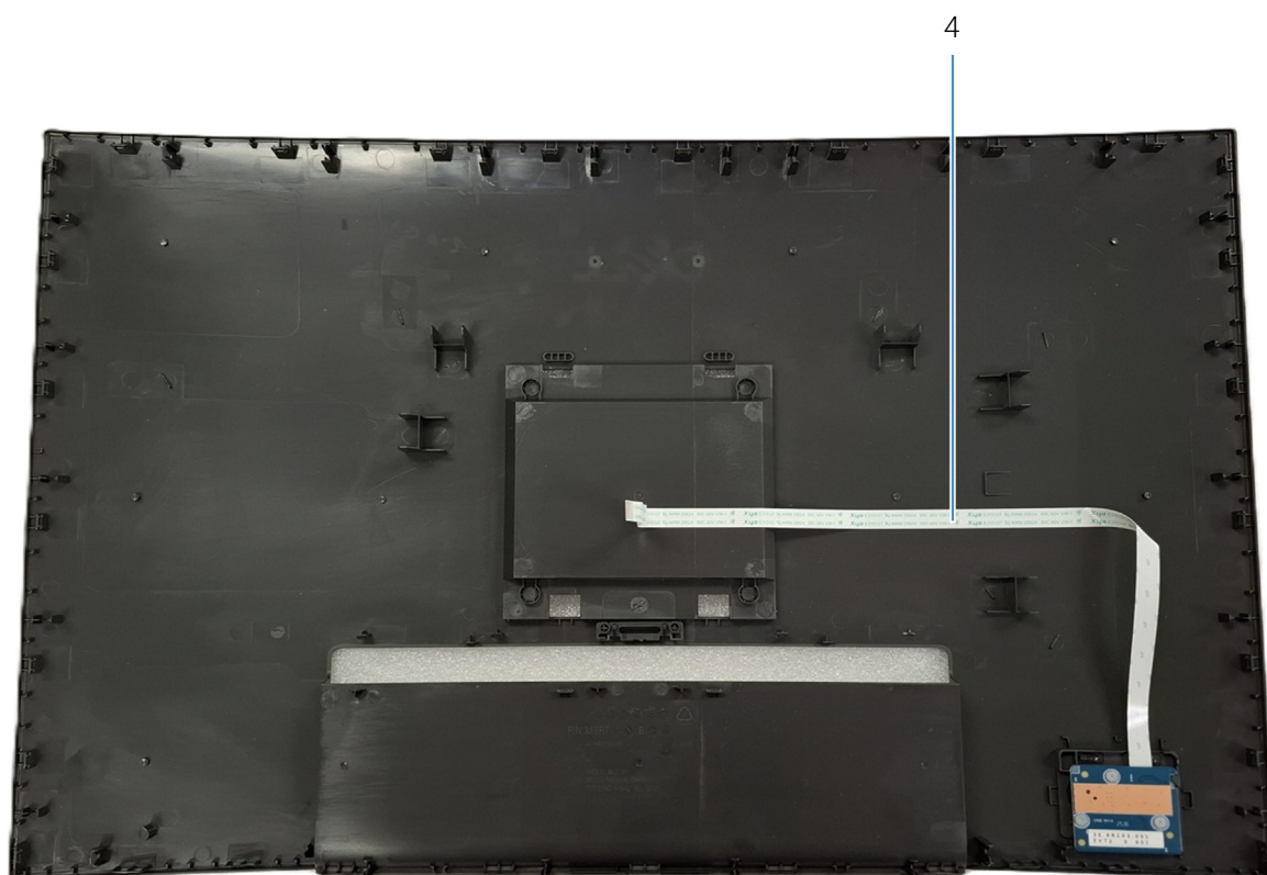
Figura 8. Conectividad de cables en la cubierta posterior de la pantalla
