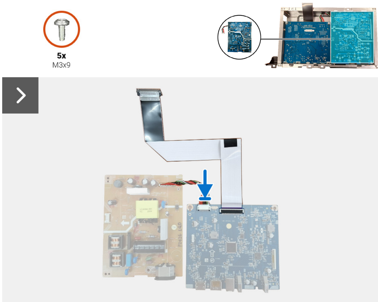
Figura 27. Instalar la placa de alimentación
