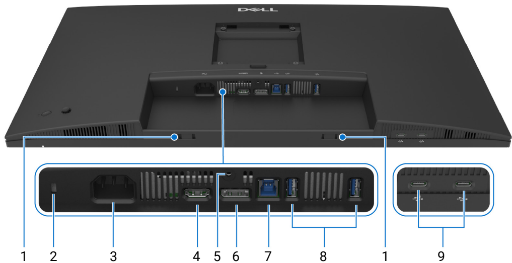
Figura 6. Vista inferior sin soporte de monitor
