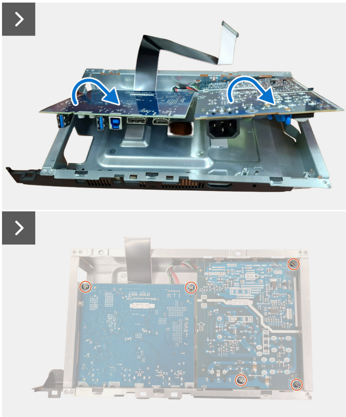
Figure 18. Installer la carte d'alimentation
