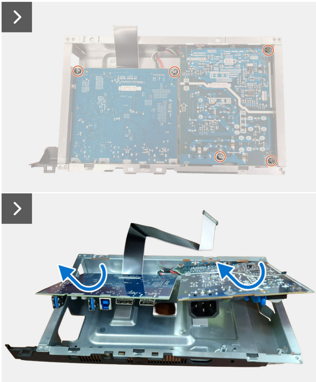
Figure 15. Retirer la carte d'alimentation
