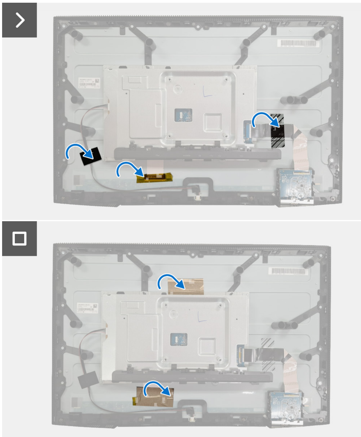
Figure 13. Installer le blindage métallique
