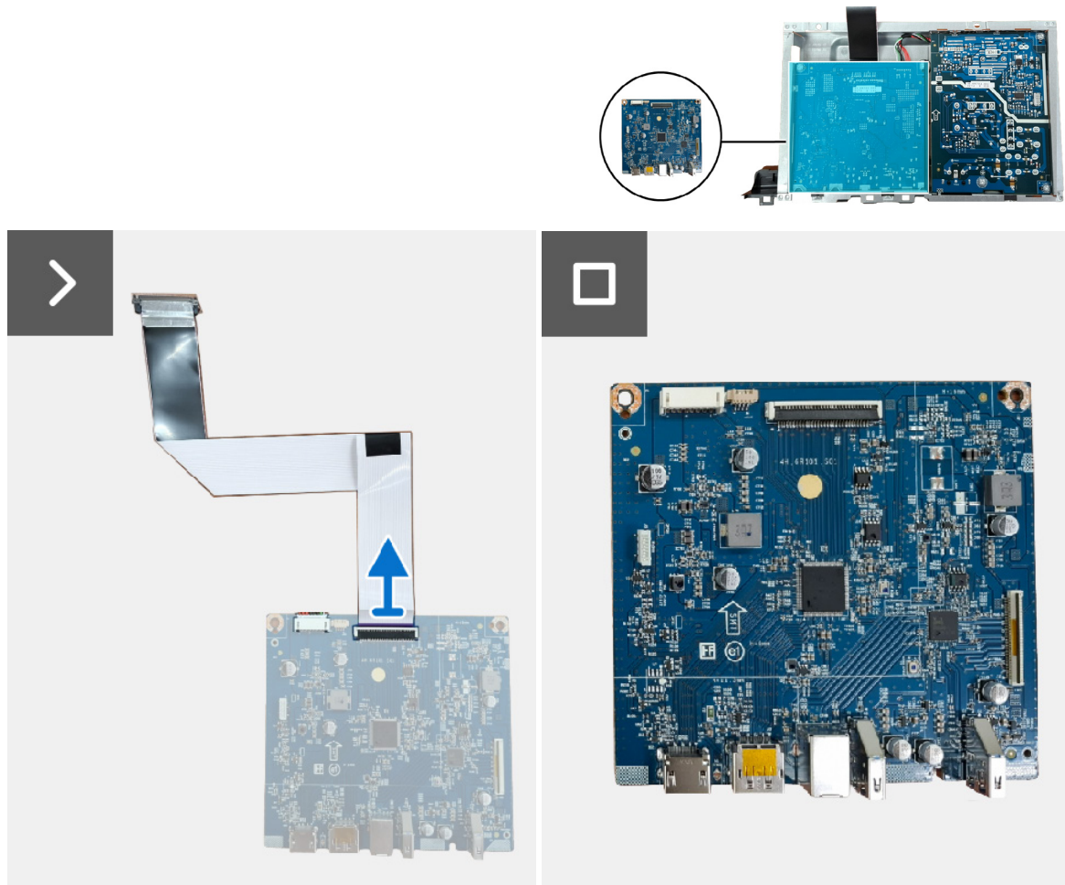
Figure 20. Retirer la carte d'interface
