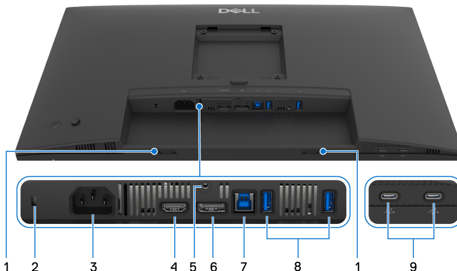
Figure 4. Vue de dessous sans le pied du moniteur
