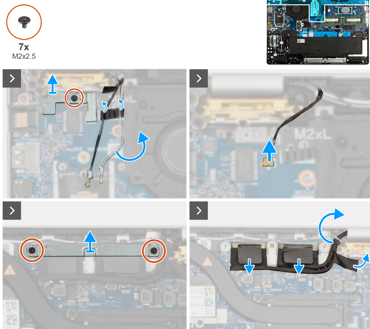
Figure 43. Retrait de l'antenne WLAN
