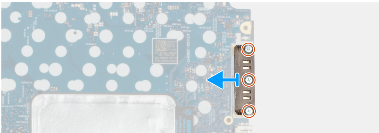
Figure 82. Retrait du module de connecteur USB-C
