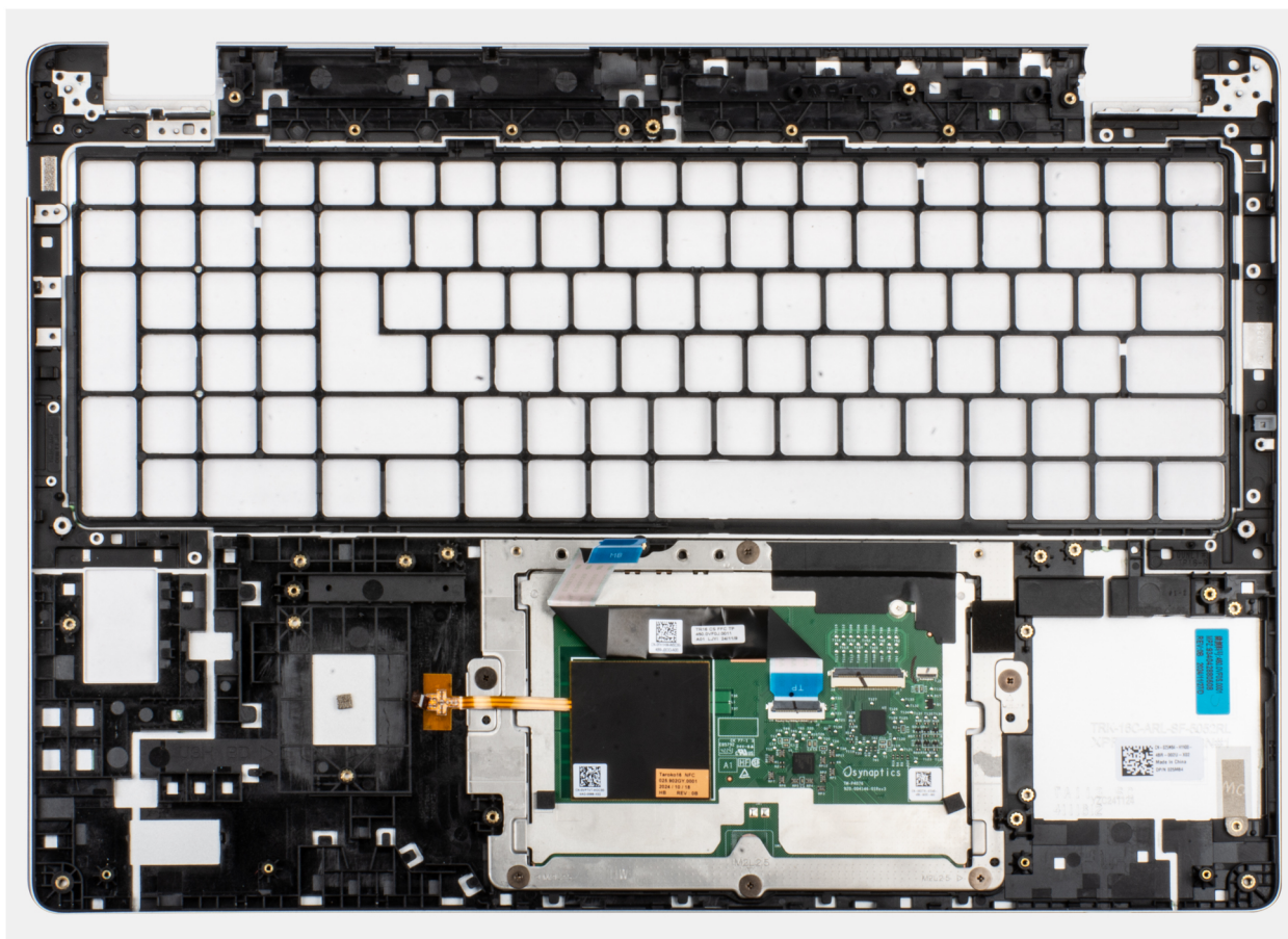
Figure 90. Retrait de l'assemblage du repose-poignets
