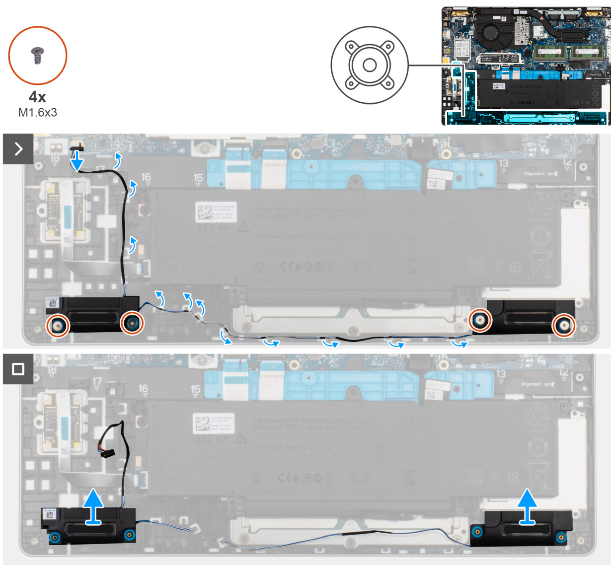
Figure 38. Retrait des haut-parleurs
