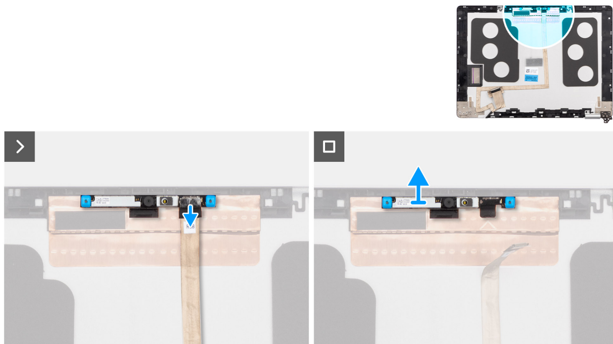
Figure 78. Retrait du module de caméra
