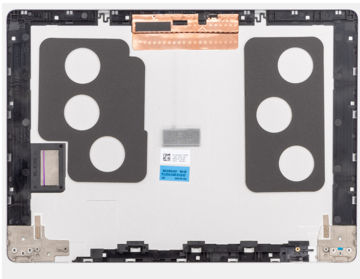
Figure 81. Installation du capot arrière de l'écran
