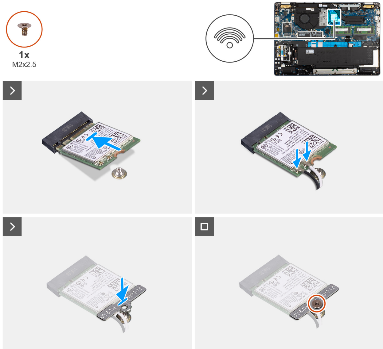
Figure 36. Installation de la carte WLAN
