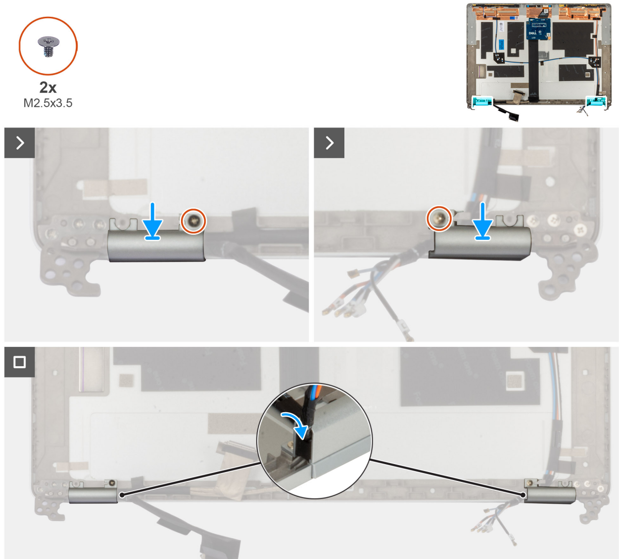
Figure 75. Installation du cache de la charnière d'écran
