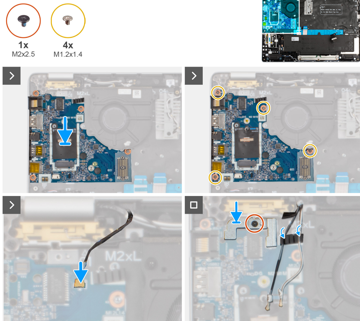
Figure 58. Retrait de la carte d'E/S
