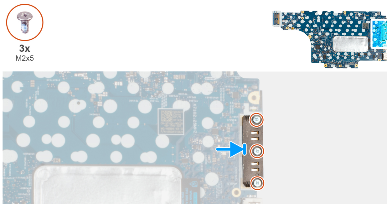
Figure 83. Installation du module de connecteur USB-C
