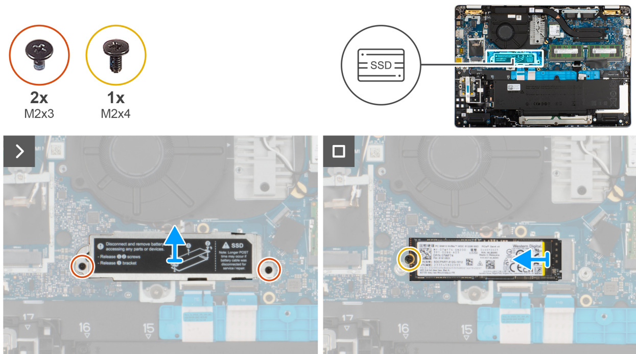
Figure 26. Retrait du disque SSD M.2 2280
