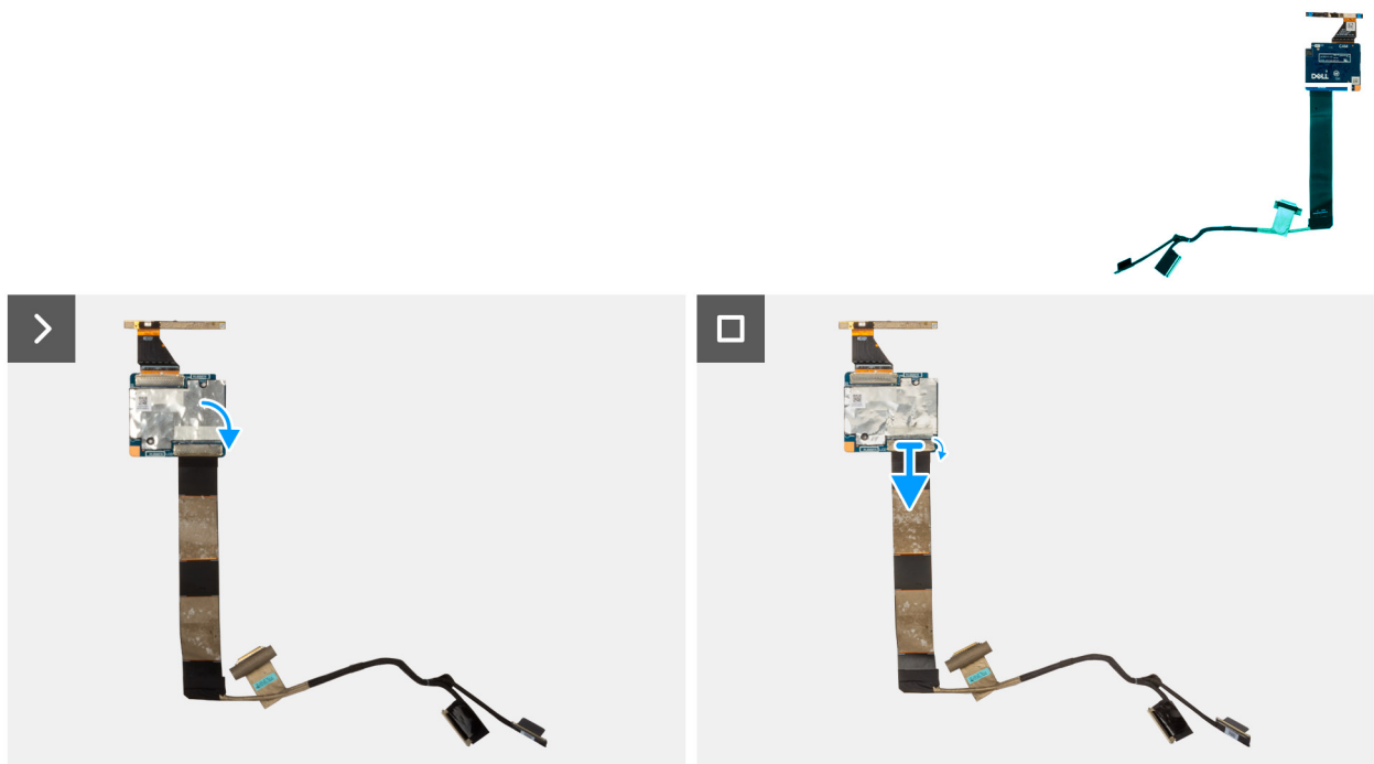
Figure 76. Retrait du câble de l'écran
