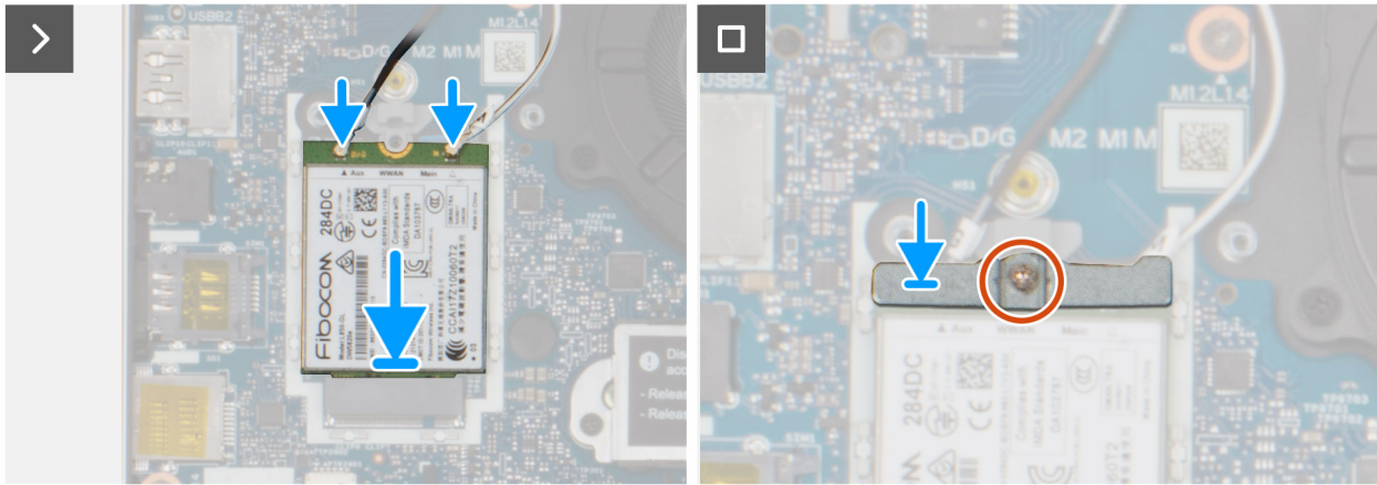
Figure 34. Installation de la carte WWAN 4G
