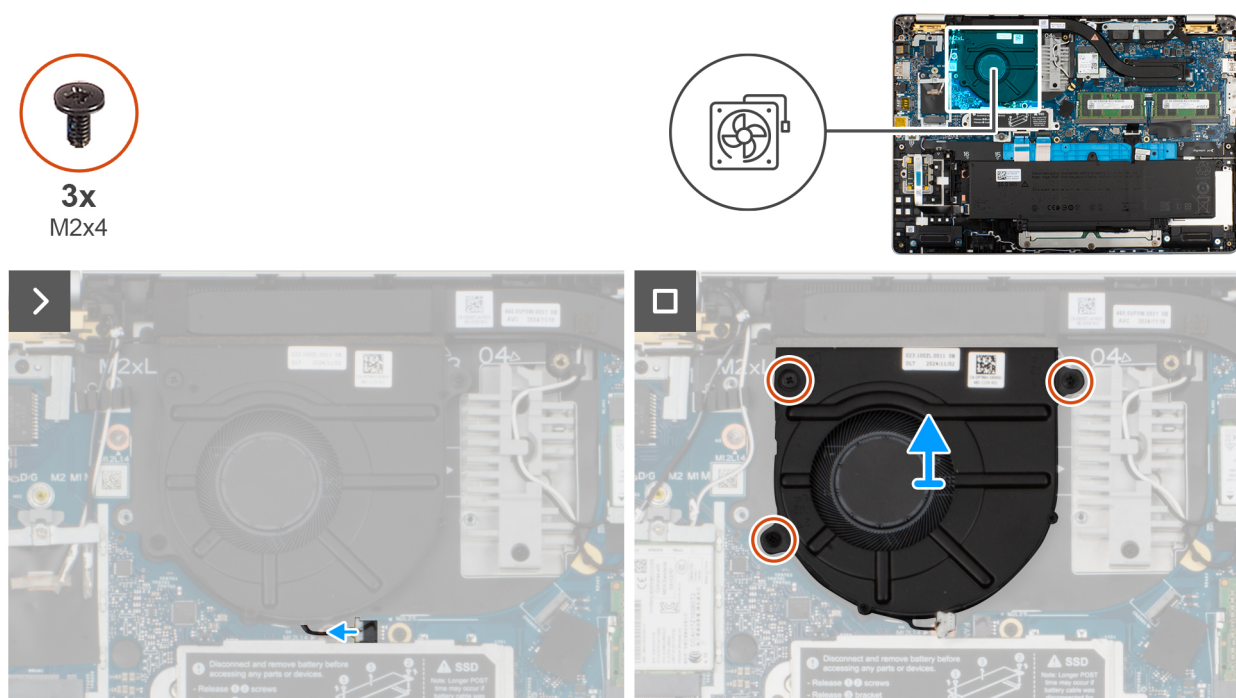
Figure 37. Retrait du ventilateur
