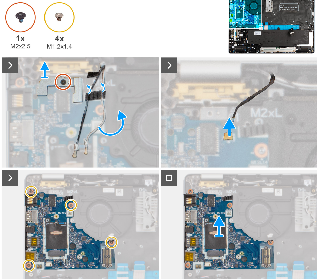
Figure 57. Retrait de la carte d'E/S
