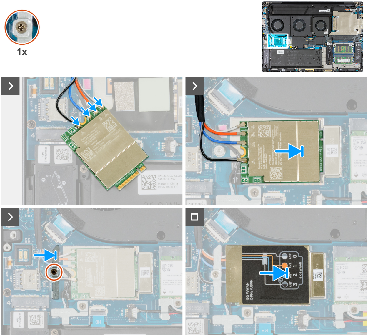
Ilustración 53. Instalación de la tarjeta WWAN
