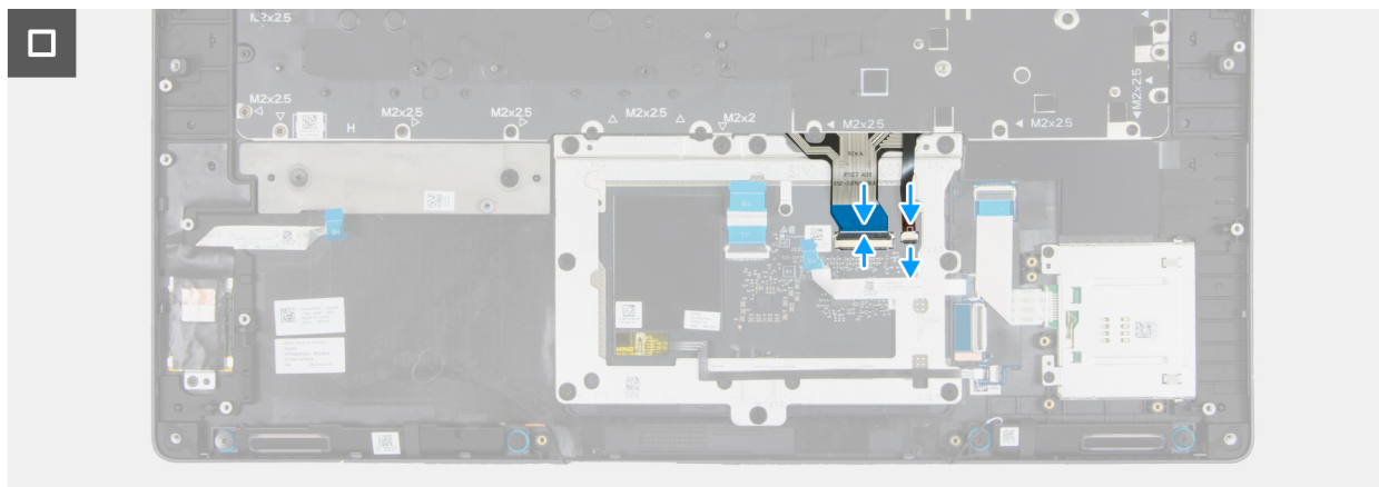
Ilustración 120. Instalación del teclado
