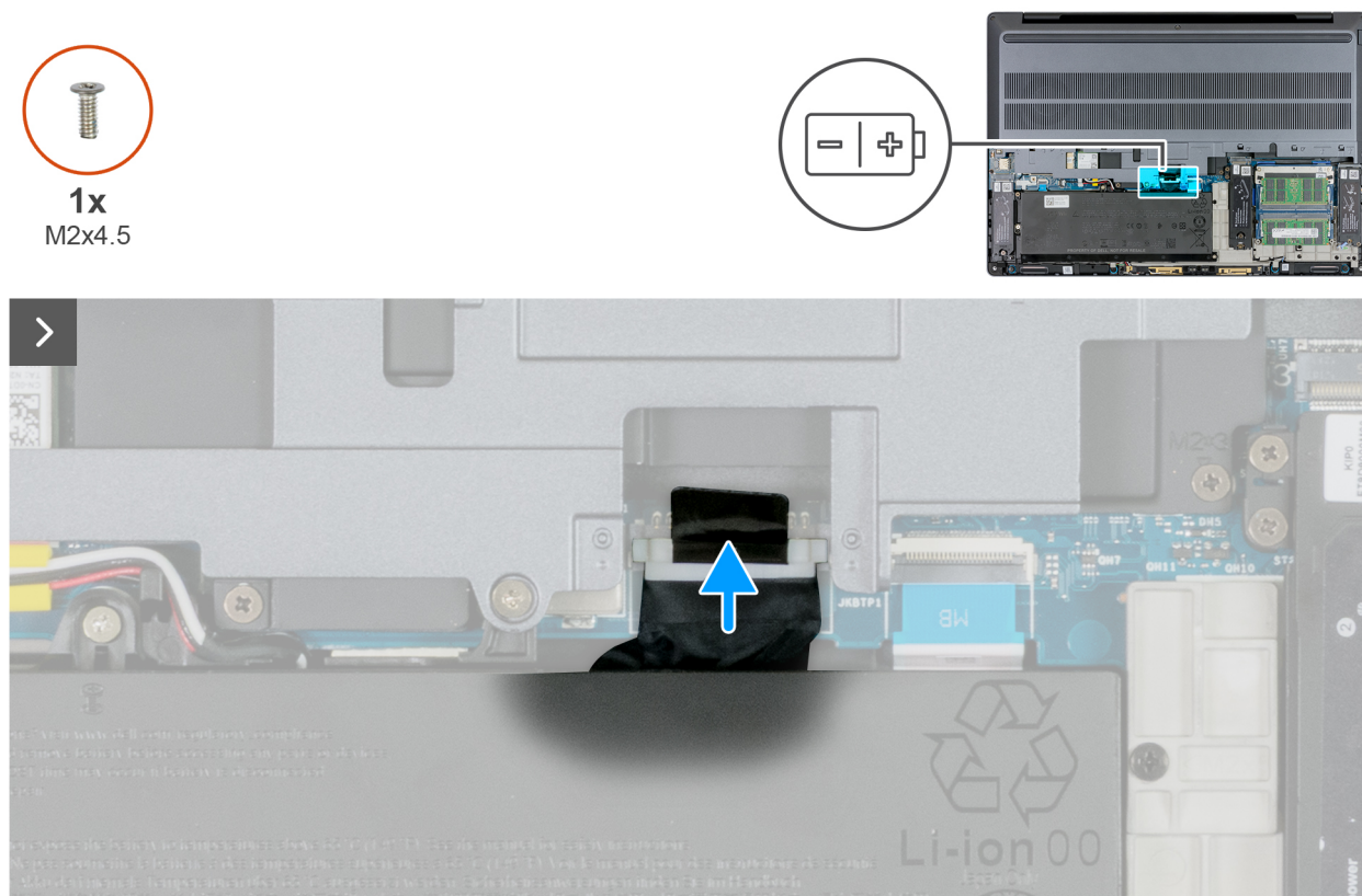
Ilustración 15. Conexión del cable de la batería
