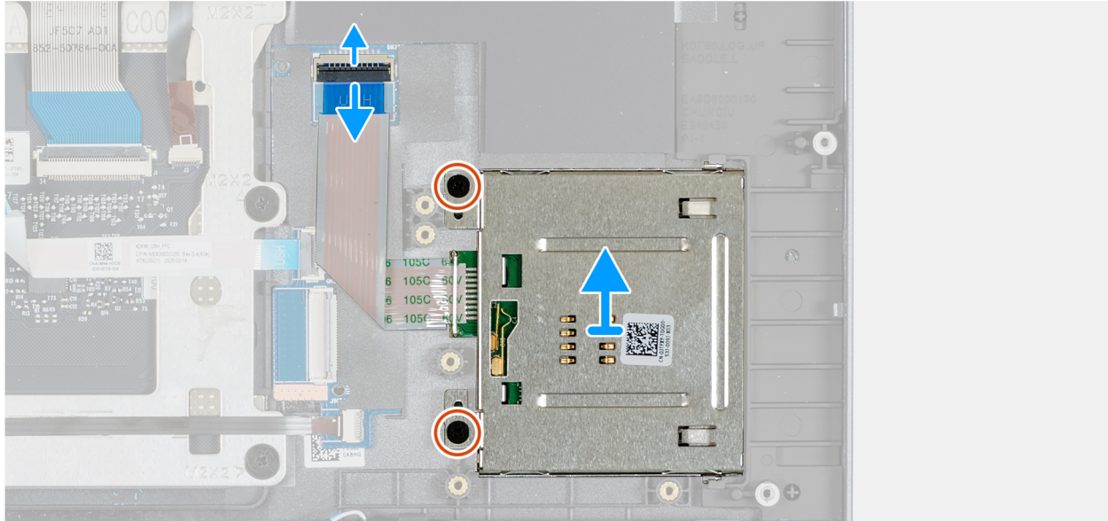
Ilustración 121. Extracción del lector de tarjetas inteligentes
