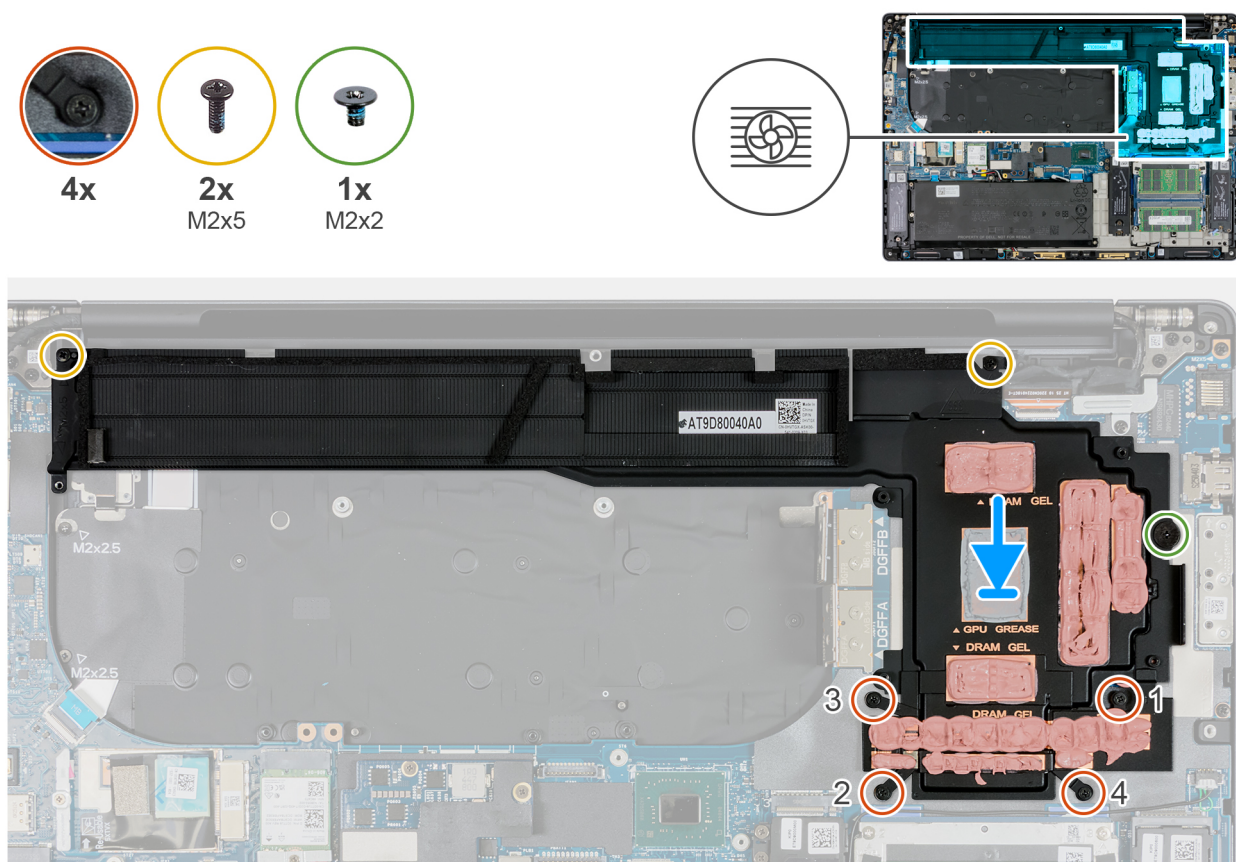
Ilustración 76. Instalación del disipador de calor en computadoras enviadas con gráficos discretos
