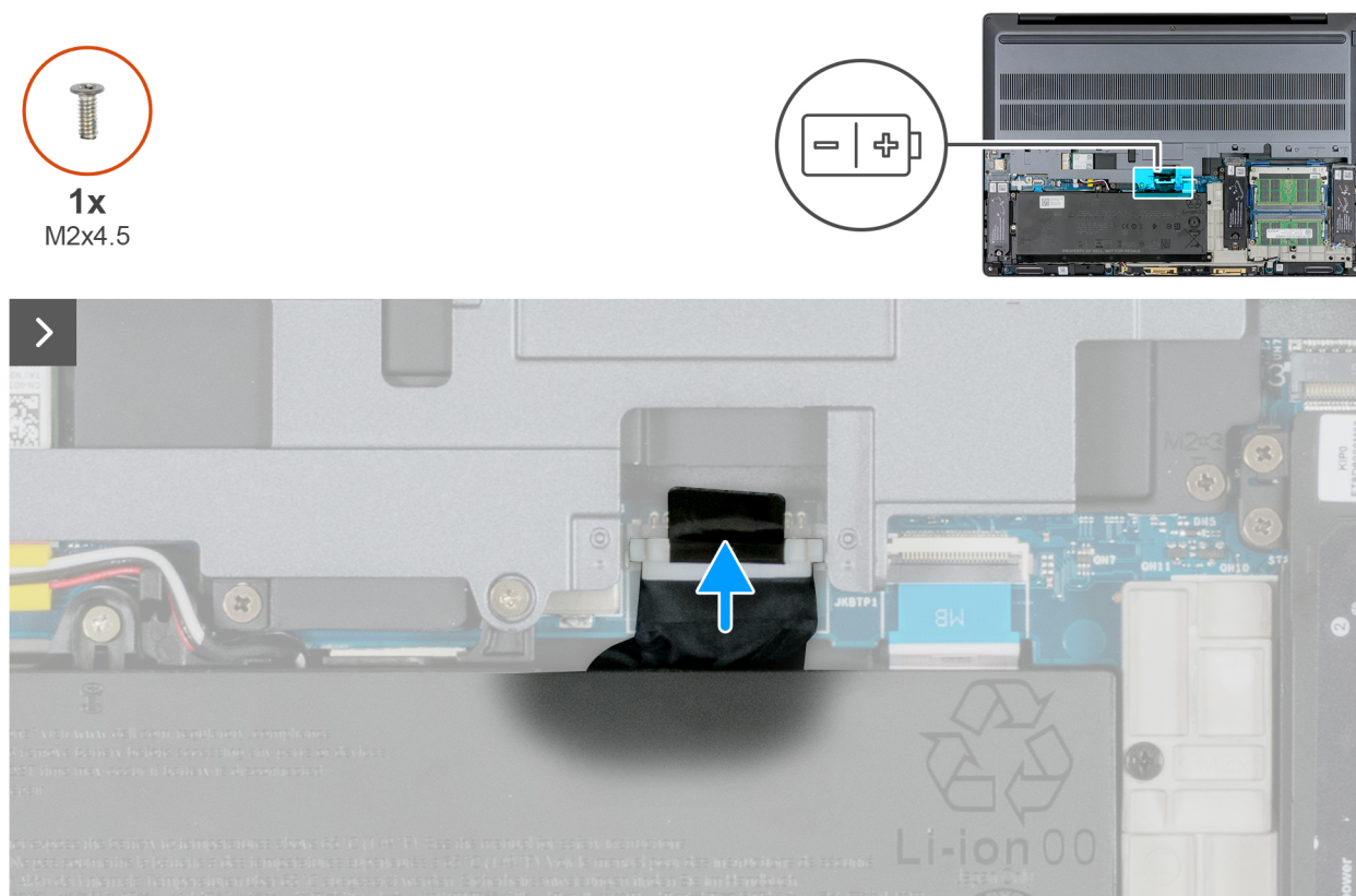
Ilustración 21. Conexión del cable de la batería
