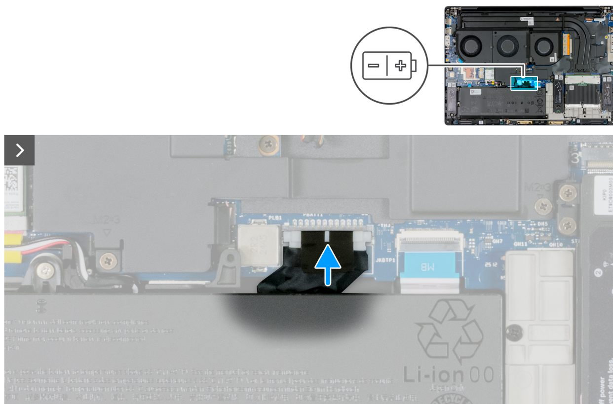
Ilustración 27. Conexión del cable de la batería
