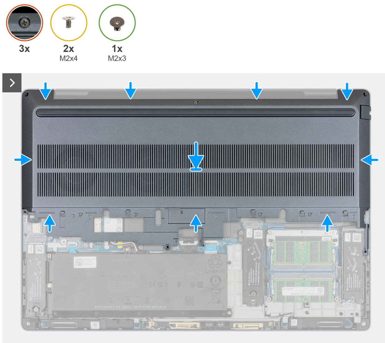
Ilustración 22. Alineación de los orificios para tornillos de la cubierta de la base con los orificios para tornillos del ensamblaje del teclado y el reposamanos
