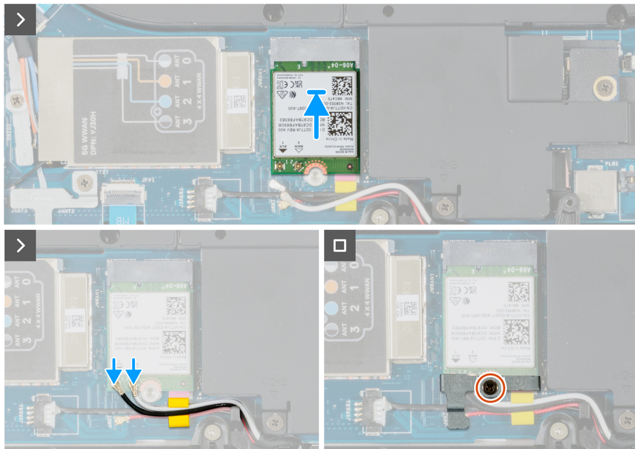
Ilustración 49. Instalación de la tarjeta WLAN
