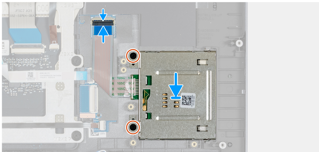
Ilustración 122. Instalación del lector de tarjetas inteligentes
