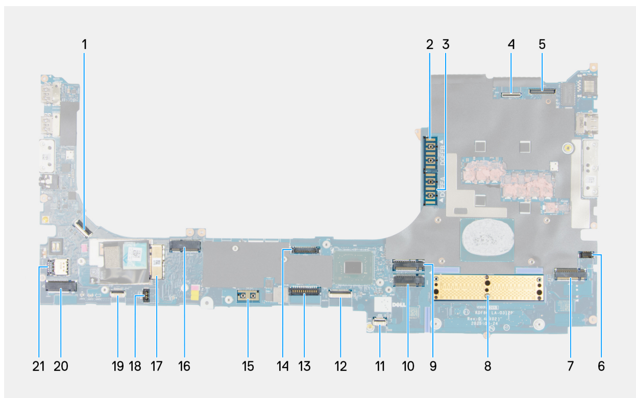
Ilustración 110. Conectores de la tarjeta madre
