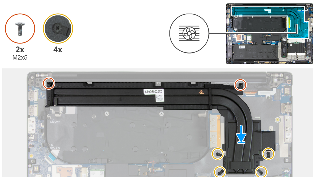
Ilustración 74. Instalación del disipador de calor en computadoras enviadas con gráficos integrados
