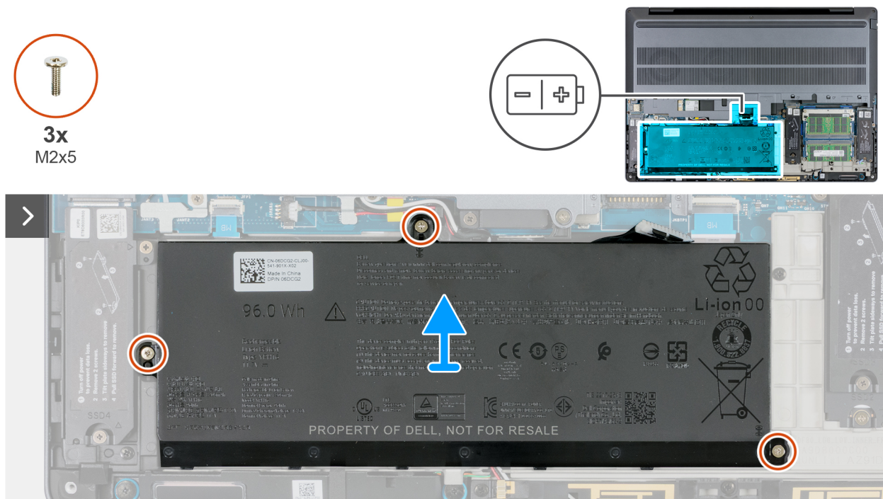
Ilustración 44. Extracción de la batería
