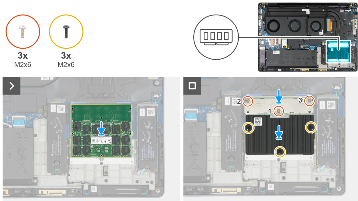
Ilustración 33. Instalación del módulo CAMM (doble canal)
