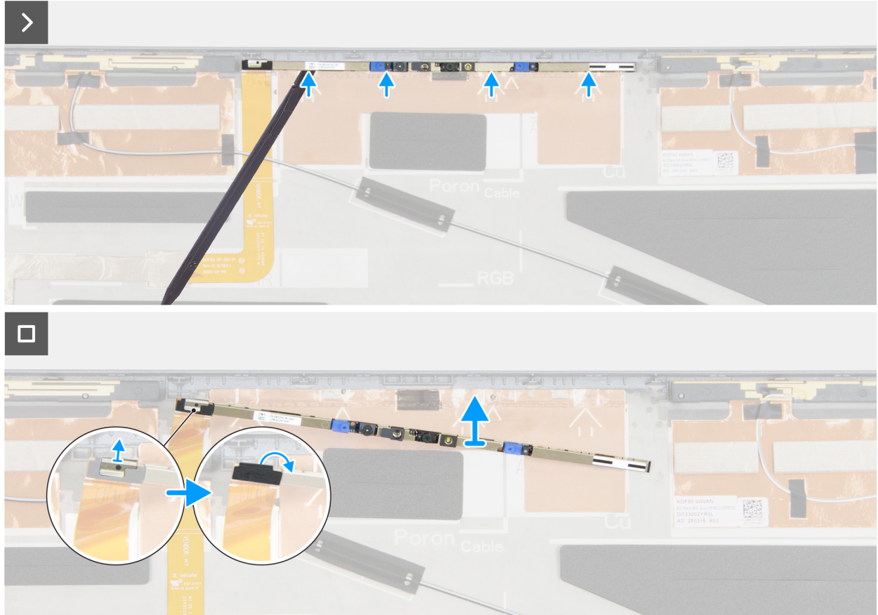
Ilustración 101. Extracción del módulo de la cámara
