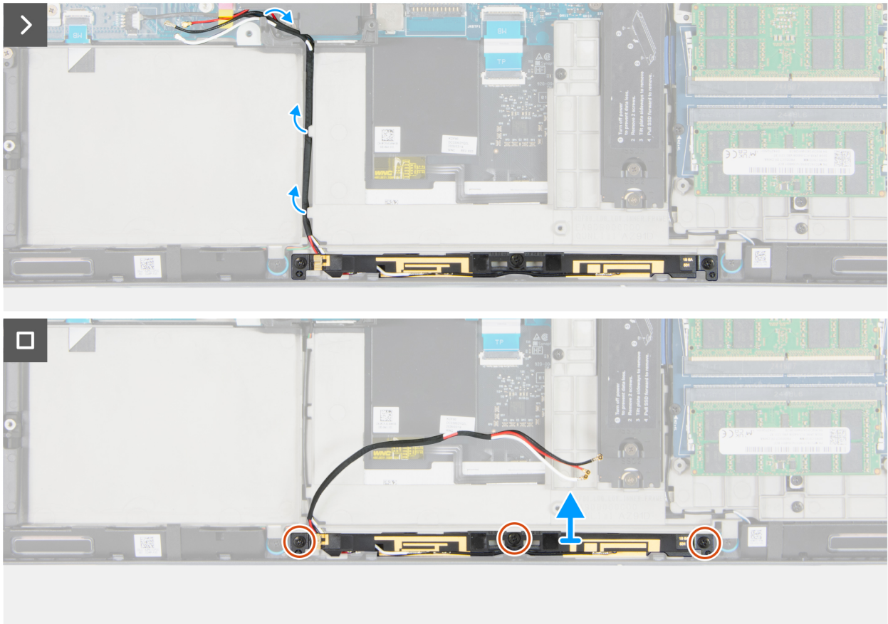
Ilustración 77. Extracción del módulo de la antena WLAN.
