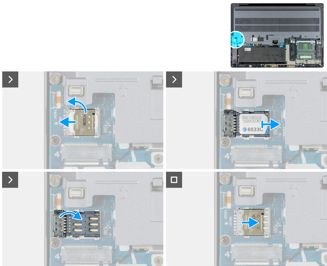
Ilustración 50. Extracción de la tarjeta SIM
