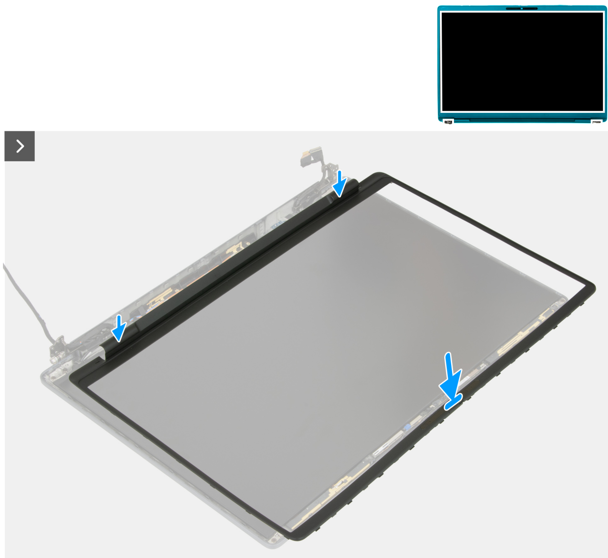
Ilustración 89. Instalación del bisel de la pantalla
