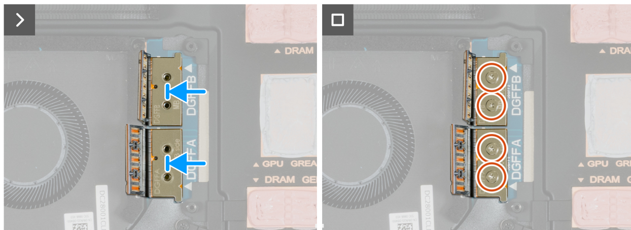
Ilustración 60. Instalación del conector de haz discreto del FPC
