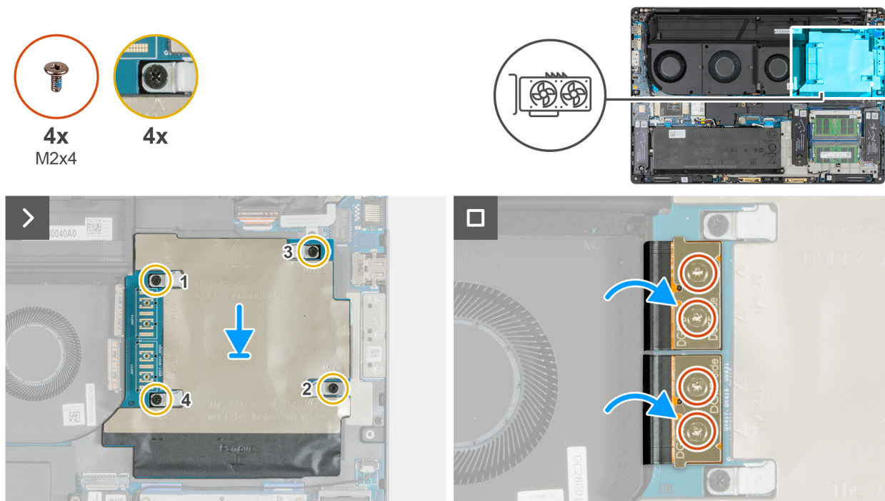
Ilustración 56. Instalación de la tarjeta GPU
