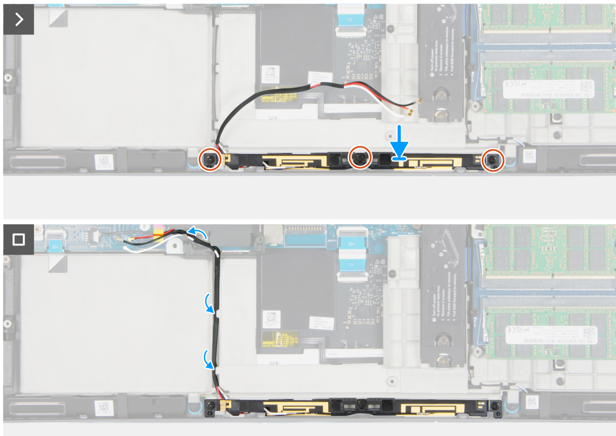
Ilustración 78. Instalación del módulo de la antena WLAN
