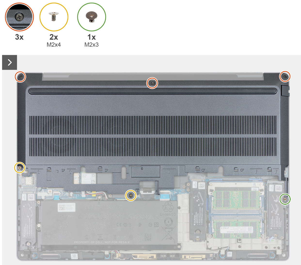
Ilustración 18. Aflojar los tres tornillos cautivos y quitar los tres tornillos
