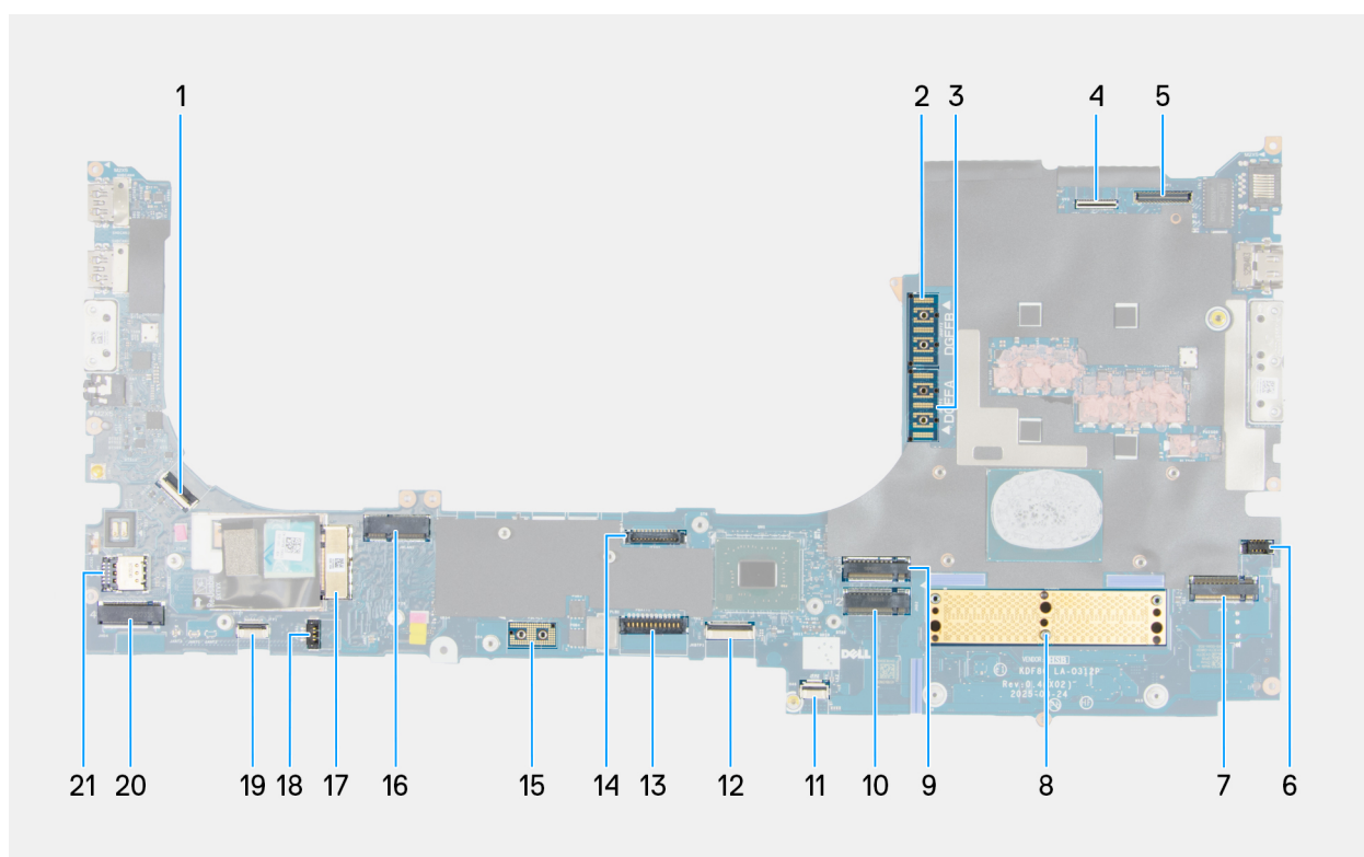
Ilustración 106. Conectores de la tarjeta madre
