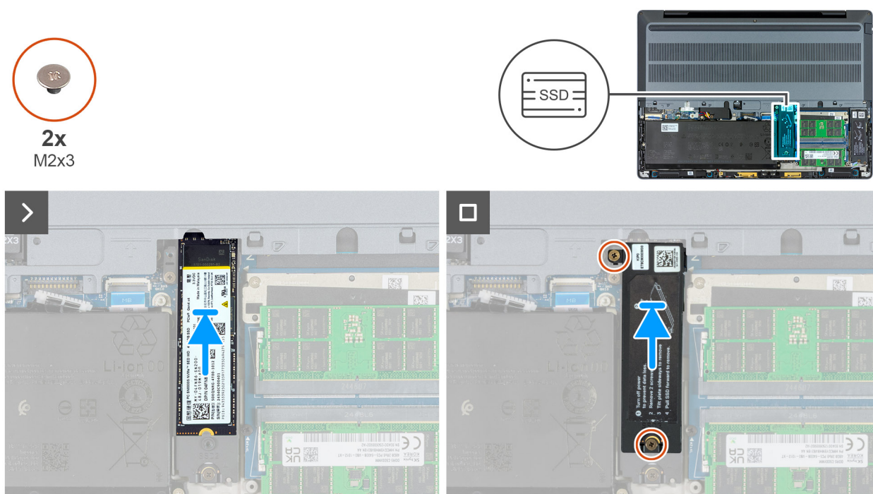
Ilustración 37. Instalación de la SSD M.2 2280 en la ranura 3 (SSD3)
