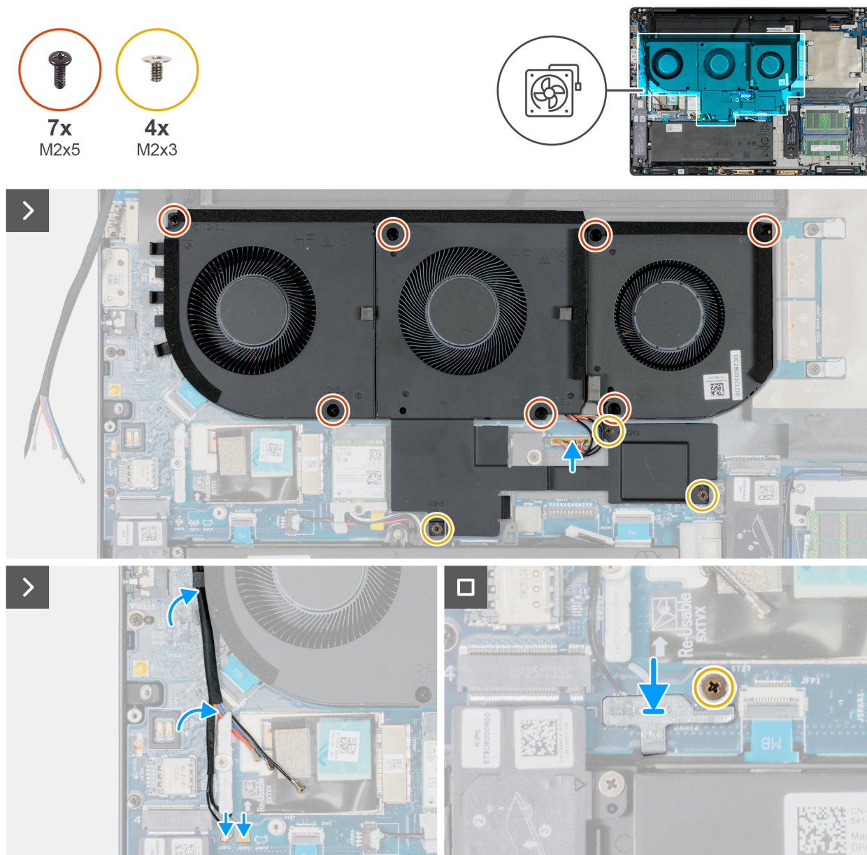
Ilustración 62. Instalación del ensamblaje del ventilador
