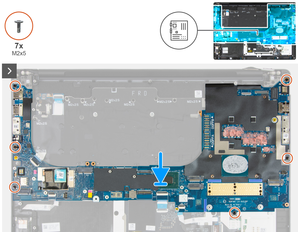
Ilustración 111. Instalación de la tarjeta madre
