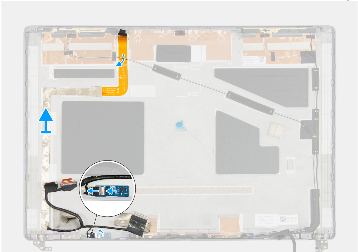
Ilustración 102. Extracción del cable de pantalla
