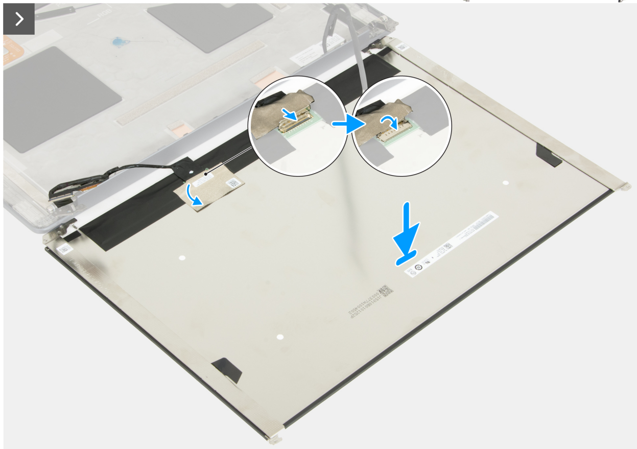
Ilustración 97. Instalación del panel de pantalla
