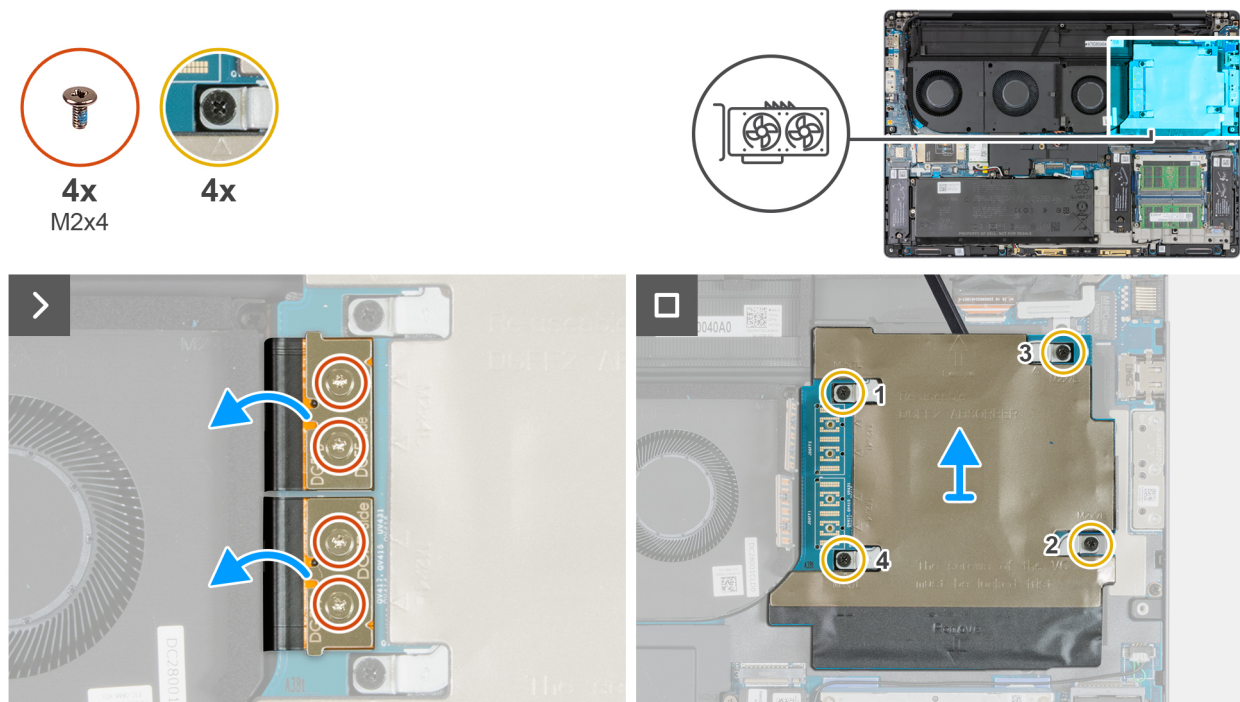
Ilustración 54. Extracción de la tarjeta GPU
