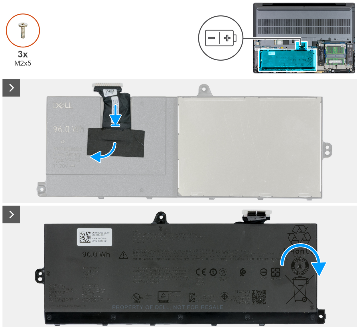
Ilustración 46. Reemplazo del cable de la batería
