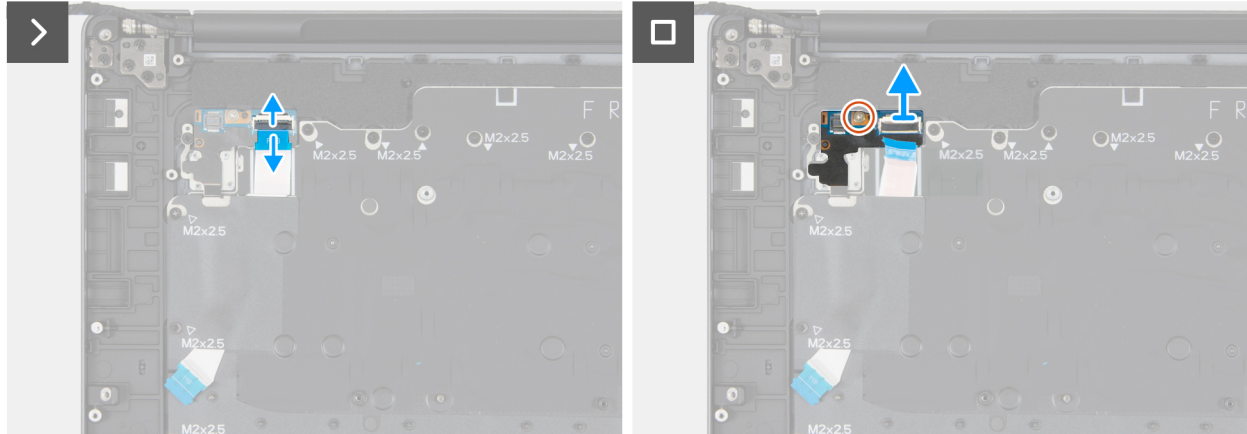
Ilustración 125. Extracción de la placa del botón de encendido
