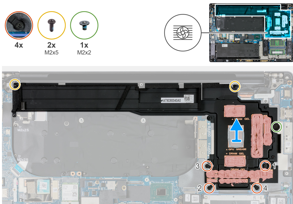
Ilustración 75. Extracción del disipador de calor en computadoras enviadas con gráficos discretos
