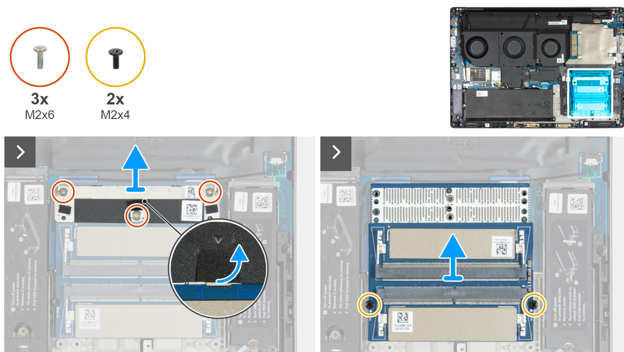
Ilustración 67. Extracción de la placa intercaladora de memoria
