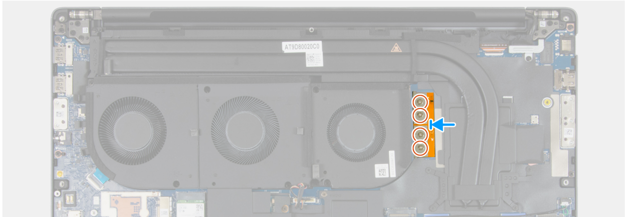
Ilustración 58. Instalación del conector de haz FPC integrado
