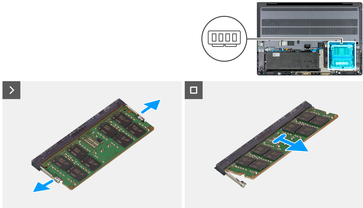
Ilustración 30. Extracción del módulo de memoria
