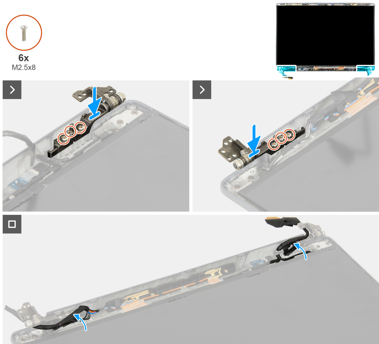
Ilustración 100. Instalación de las bisagras de la pantalla
