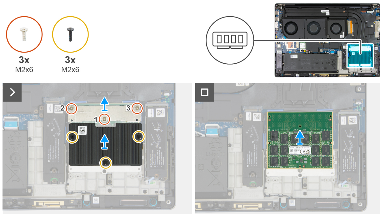
Ilustración 32. Extracción del módulo de CAMM
