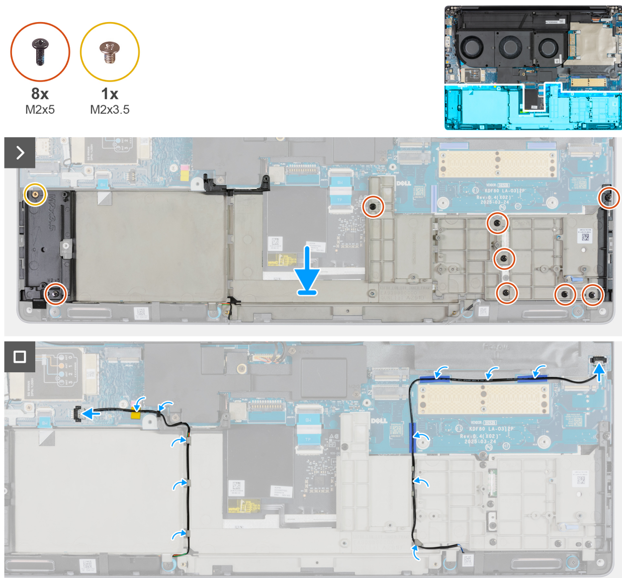
Ilustración 80. Instalación de la trama interna
