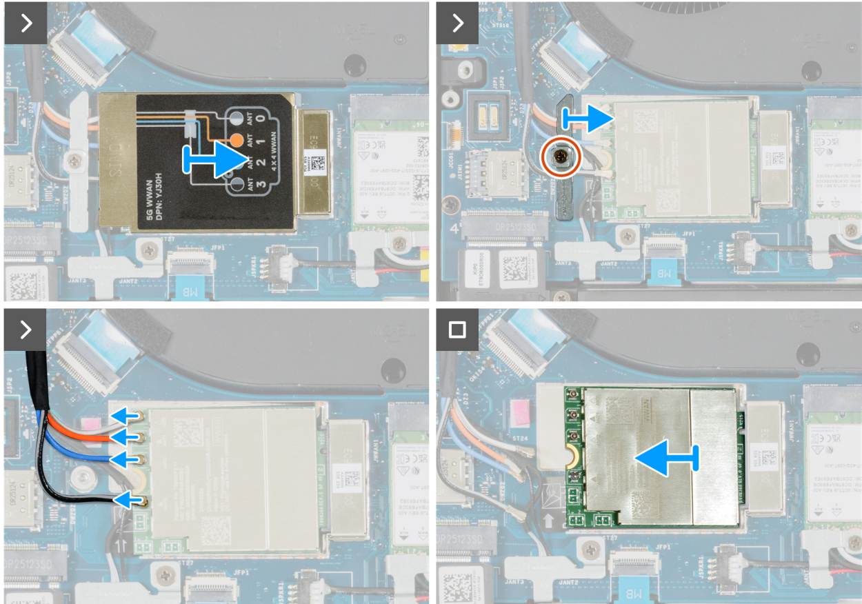
Ilustración 52. Extracción de la tarjeta WWAN
