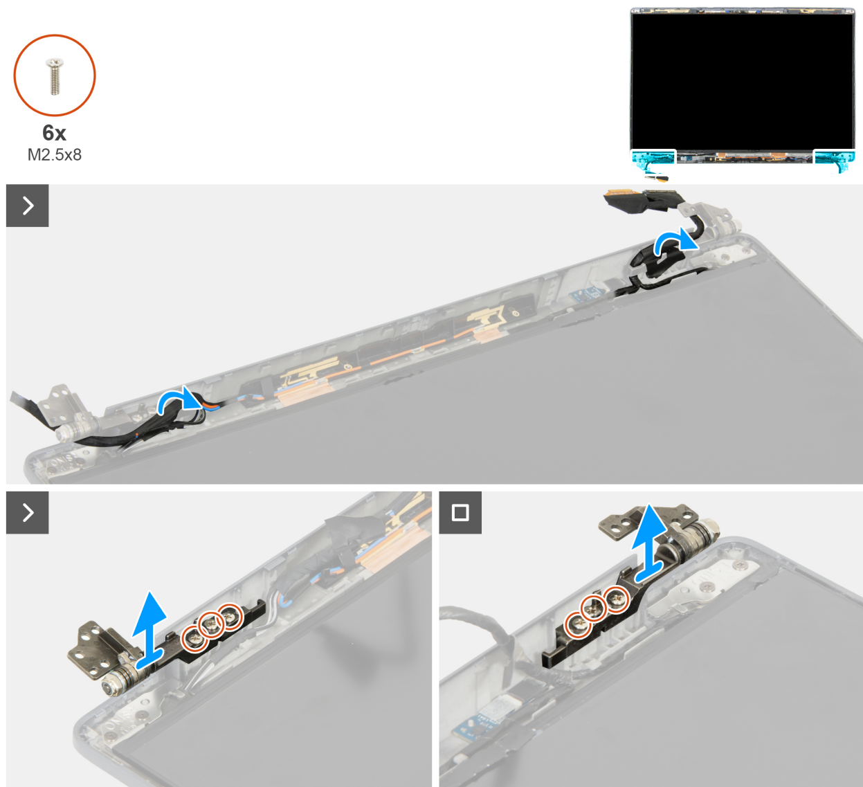
Ilustración 99. Extracción de las bisagras de la pantalla
