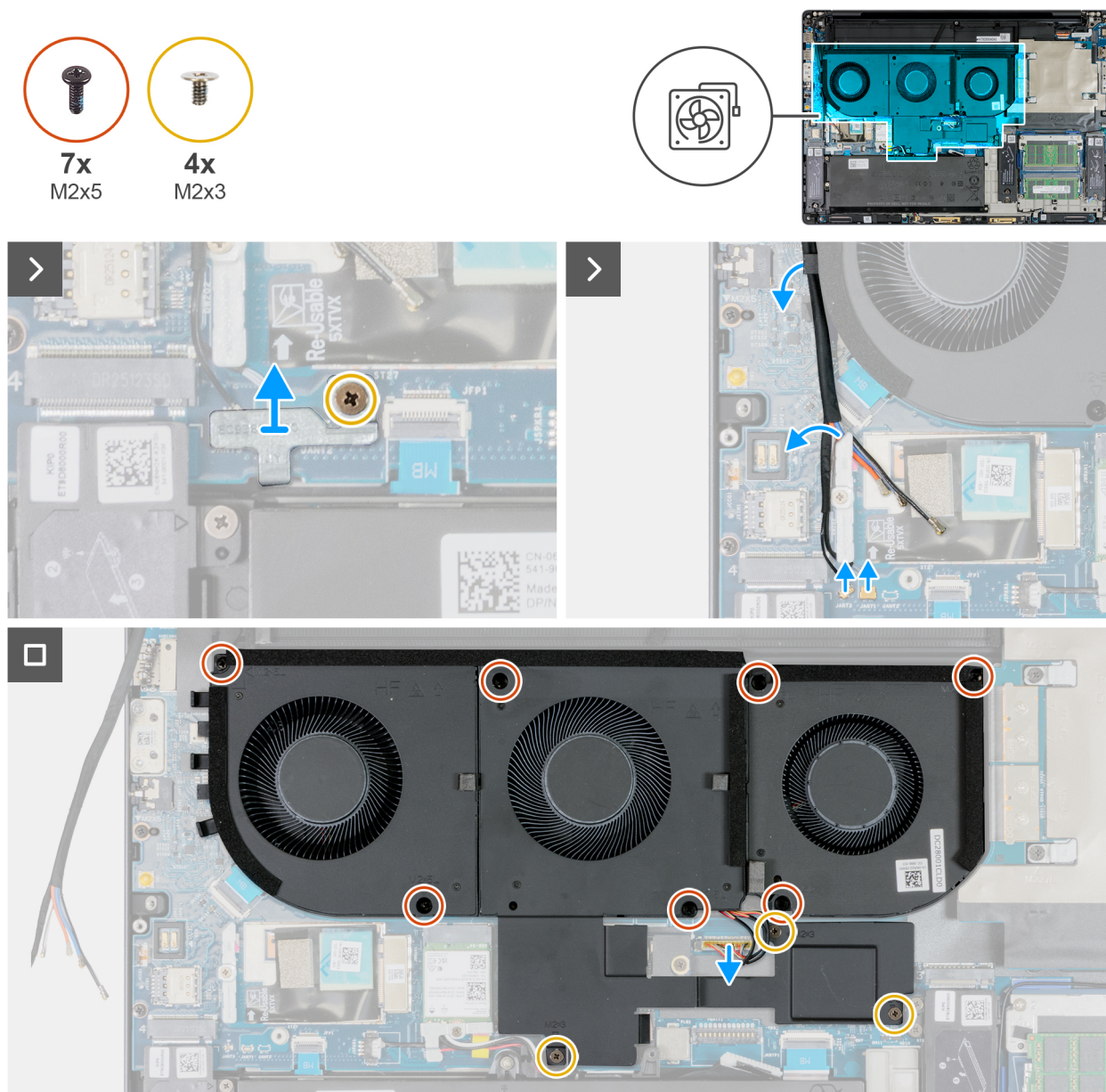
Ilustración 61. Extracción del ensamblaje del ventilador
