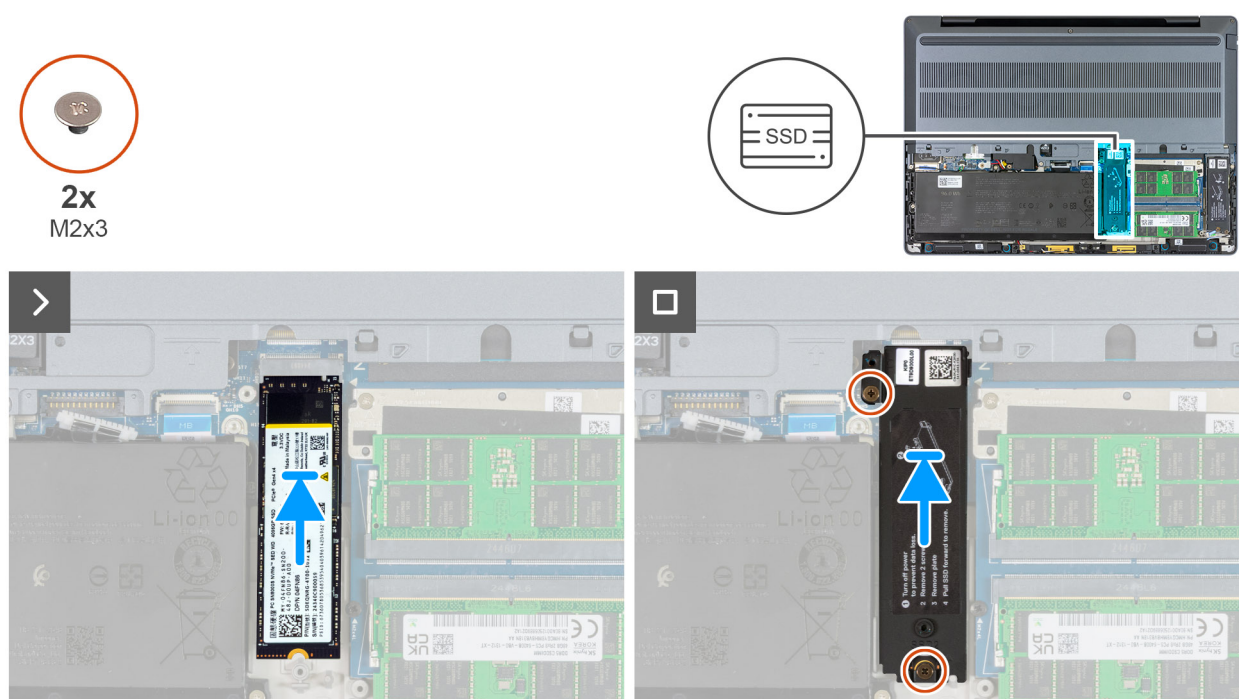
Ilustración 39. Instalación de la SSD M.2 2280 en la ranura 2 (SSD2)
