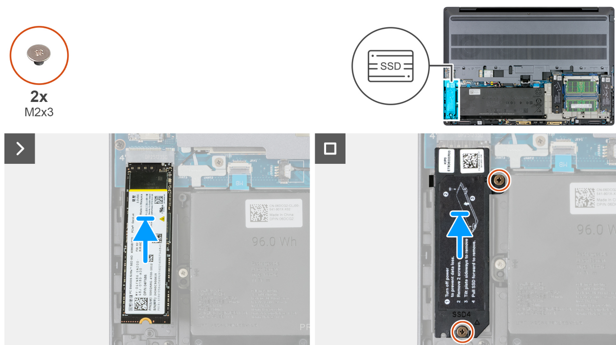
Ilustración 41. Instalación de la SSD M.2 2280 en la ranura 4 (SSD4)
