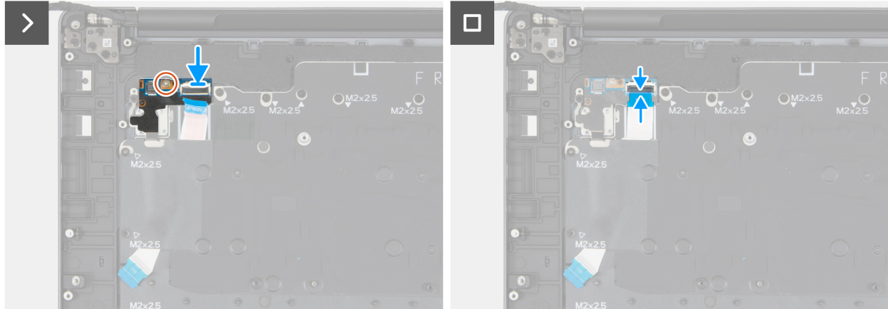
Ilustración 126. Instalación de la placa del botón de encendido
