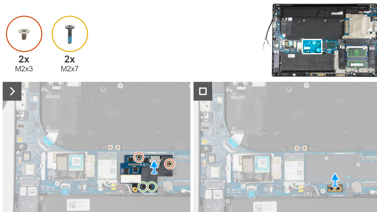
Ilustración 71. Extracción de la placa de alimentación
