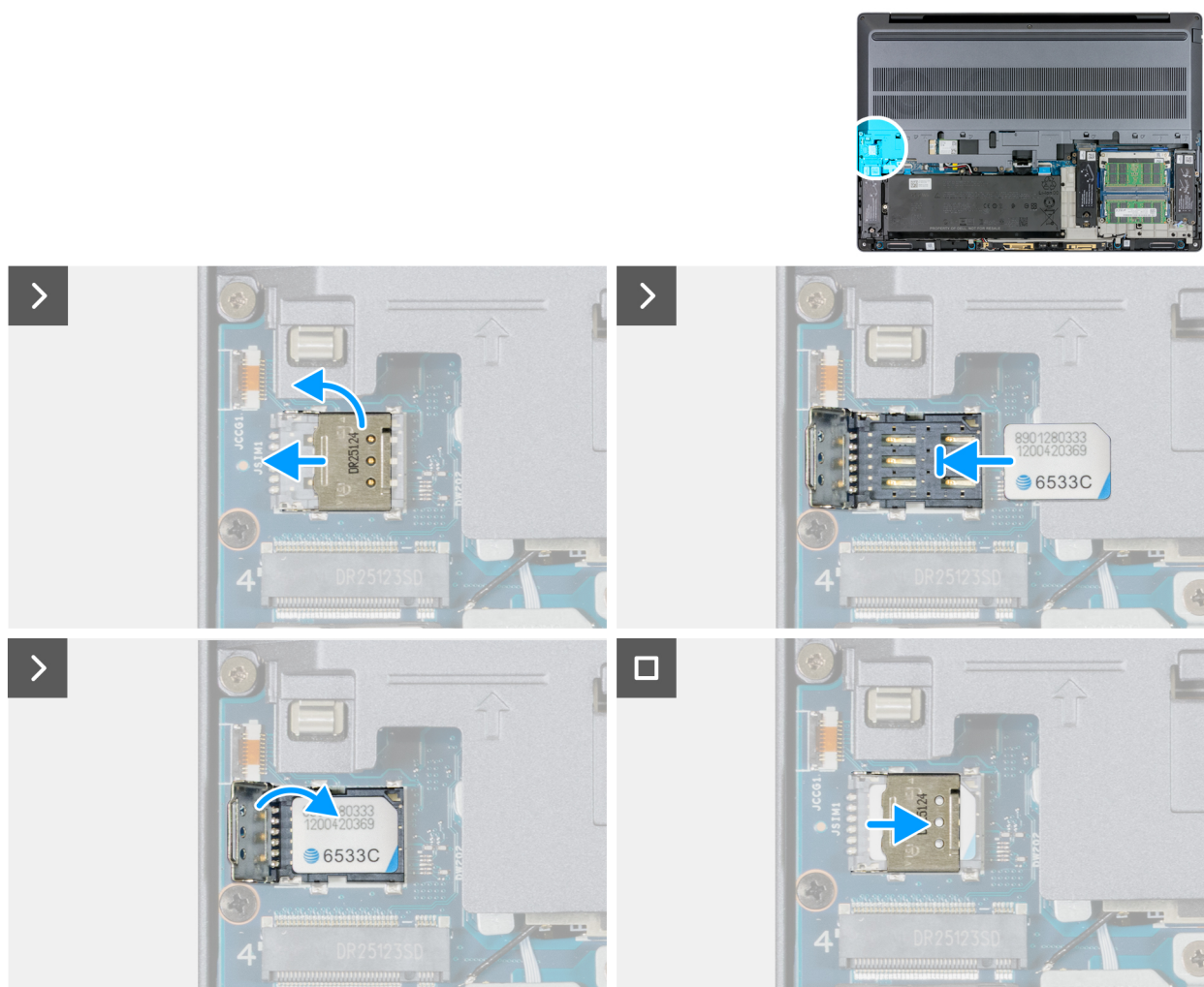
Ilustración 51. Instalación de la tarjeta SIM
