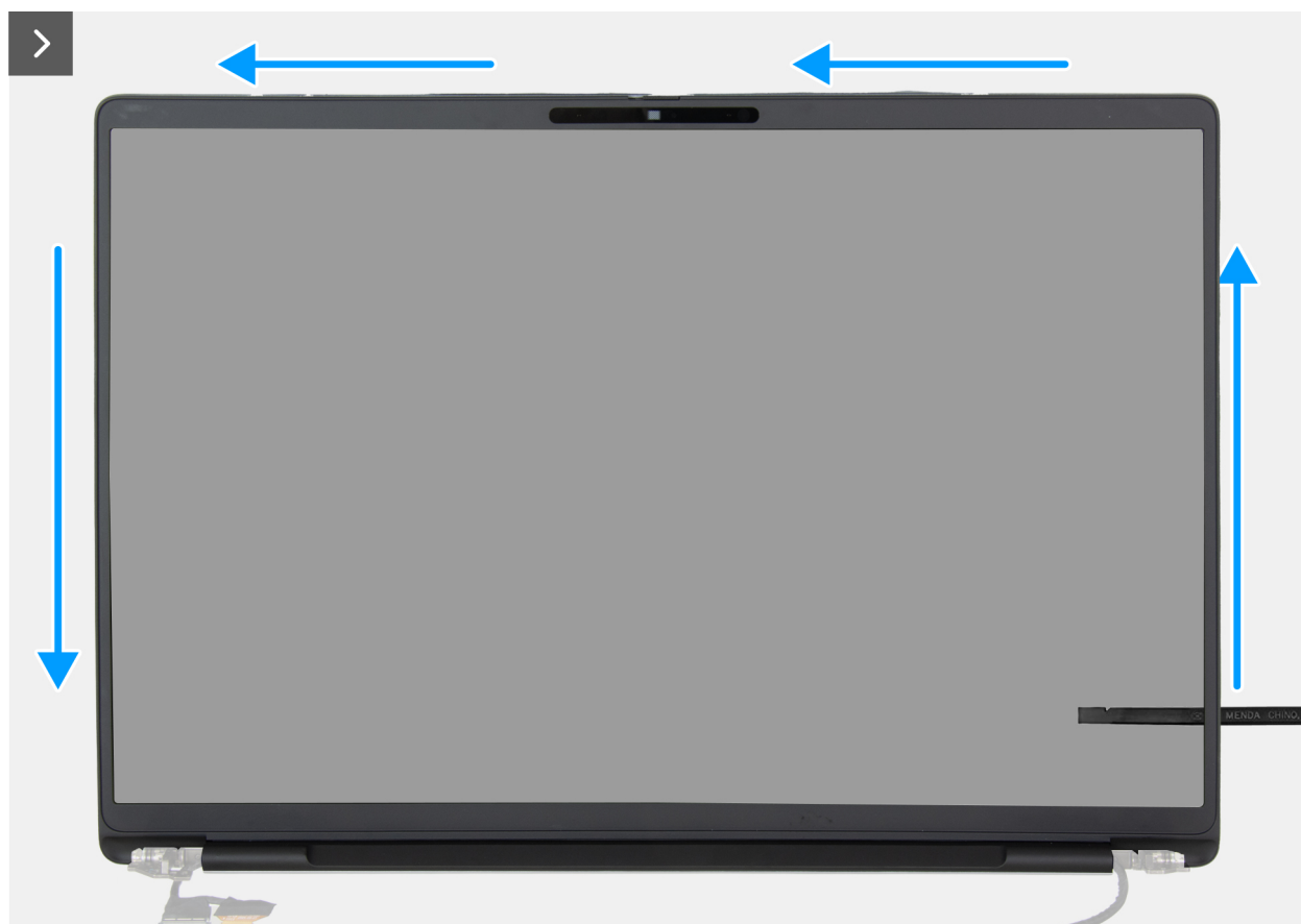
Ilustración 85. Extracción del embellecedor de la pantalla
