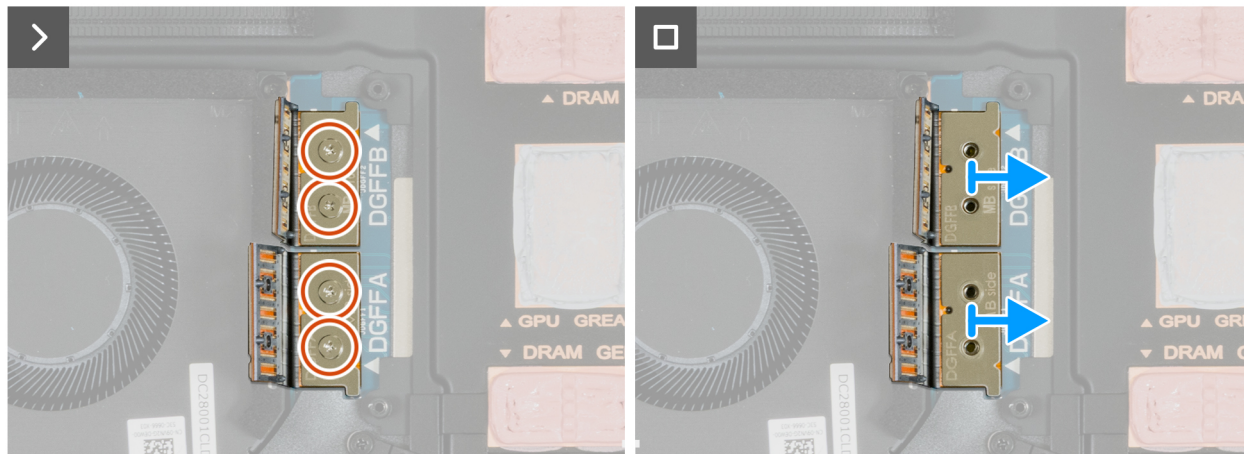
Ilustración 59. Extracción del conector de haz discreto FPC
