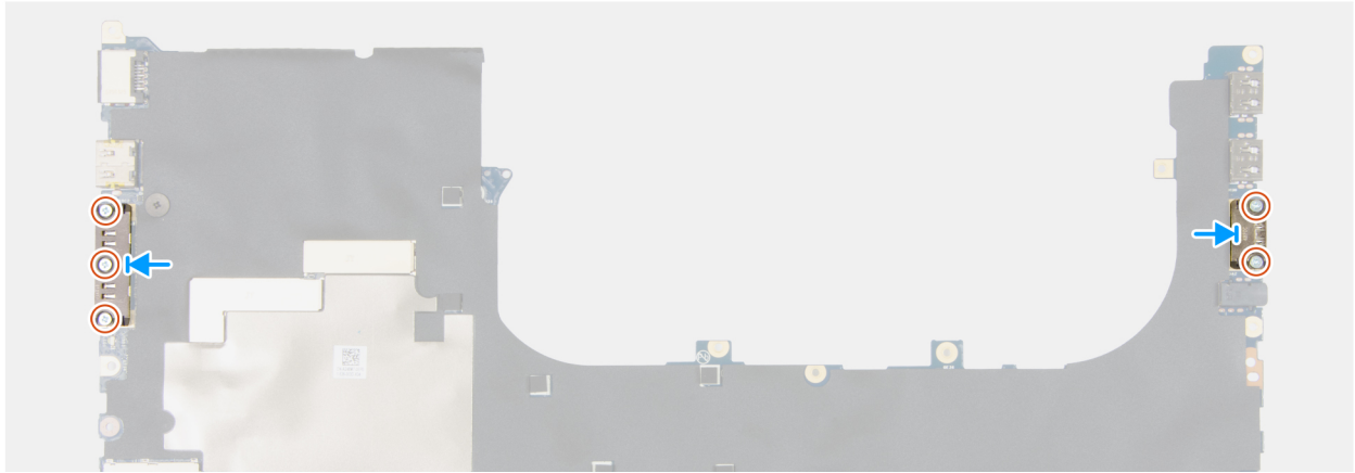
Ilustración 119. Instalación del módulo del conector USB Type-C
