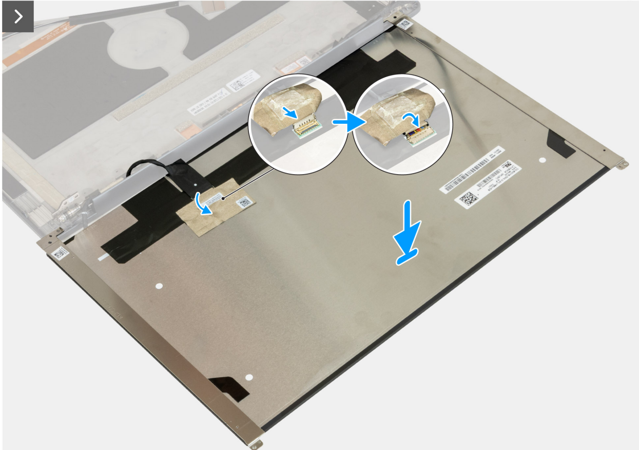
Ilustración 96. Instalación del panel de pantalla para pantallas táctiles
