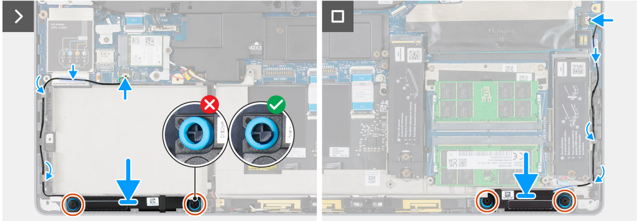
Ilustración 85. Instalación de los altavoces
