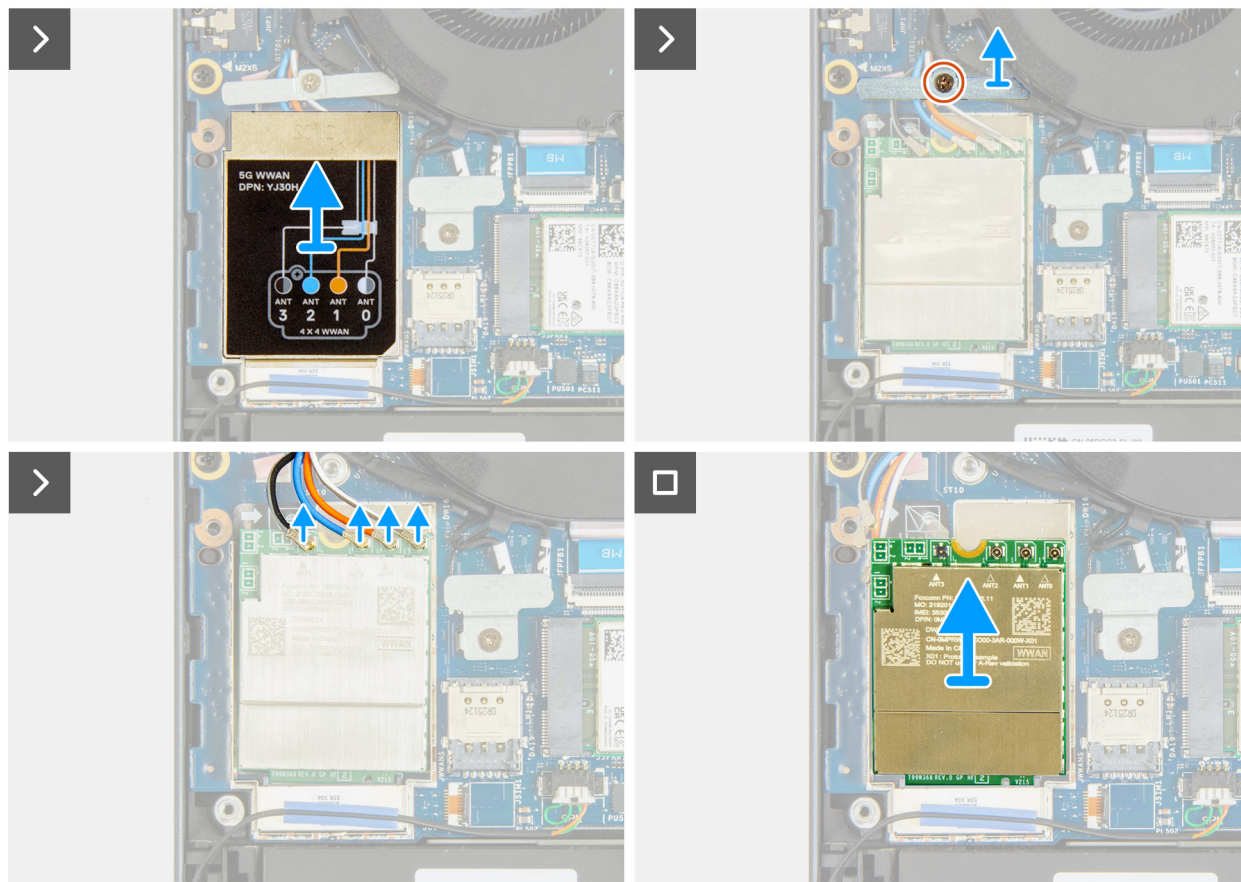
Ilustración 48. Extracción de la tarjeta WWAN
