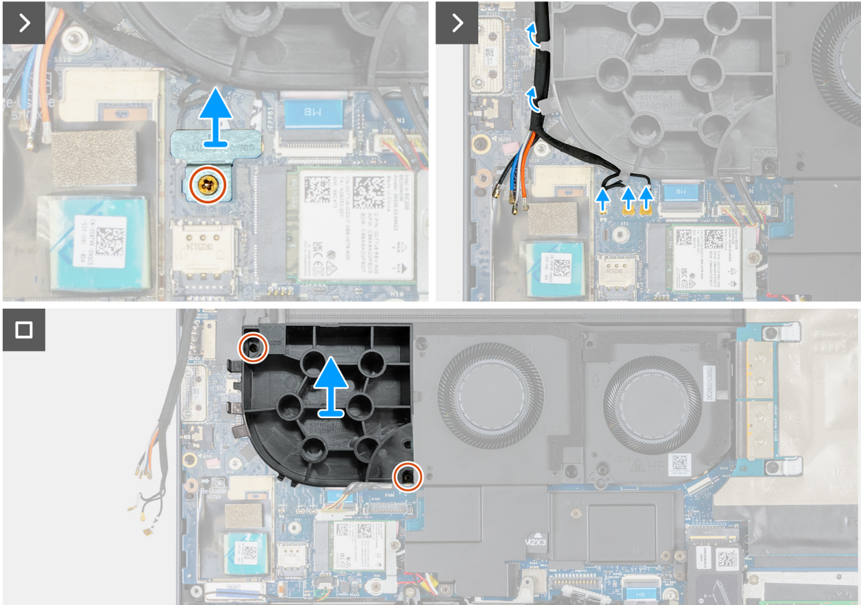
Ilustración 57. Extracción del ventilador ficticio
