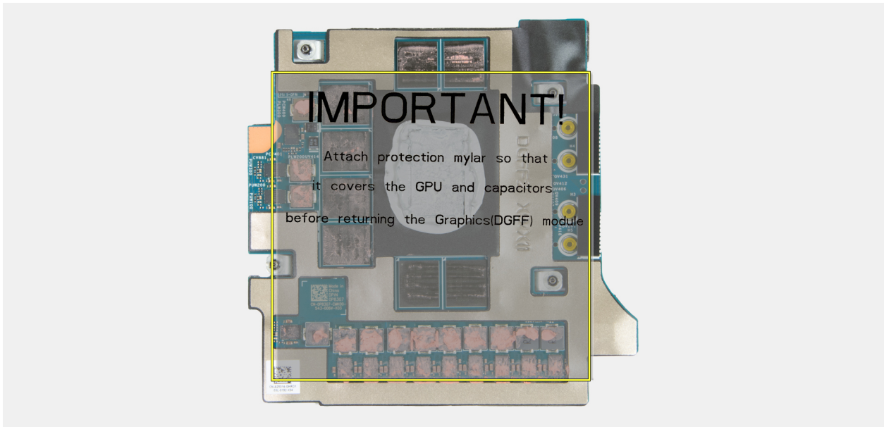
Ilustración 51. Preparación de la tarjeta GPU defectuosa para la devolución
