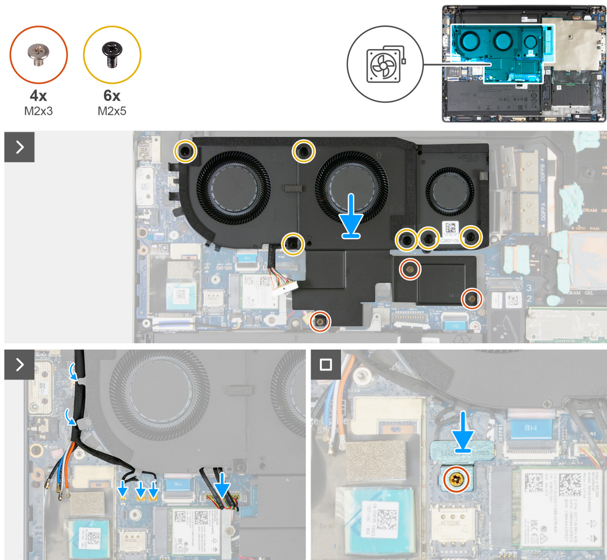
Ilustración 65. Instalación del ensamblaje del ventilador
