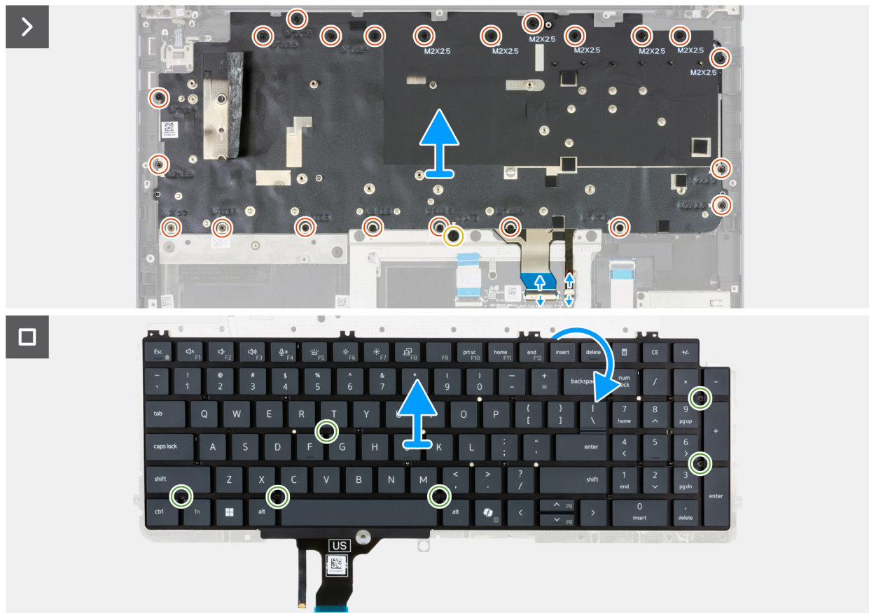
Ilustración 122. Extracción del teclado
