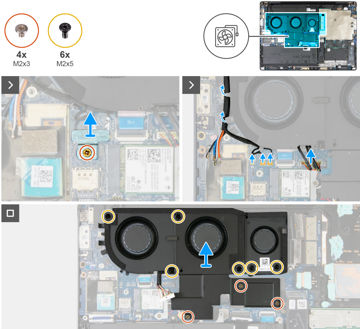
Ilustración 64. Extracción del ensamblaje del ventilador
