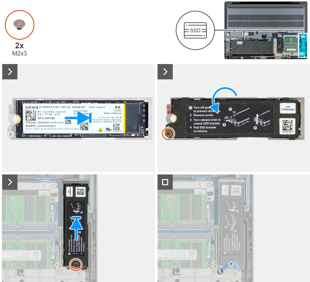
Ilustración 33. Instalación de la SSD M.2 2280 en la ranura 1 (SSD1)
