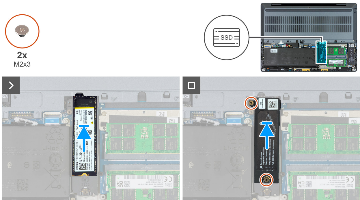
Ilustración 35. Instalación de la SSD M.2 2280 en la ranura 3 (SSD3)
