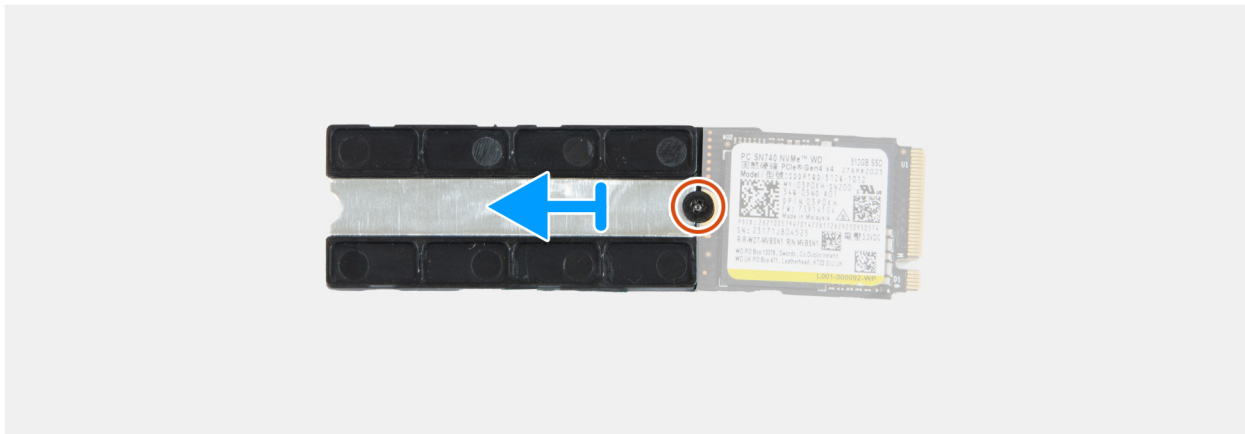
Ilustración 38. Extracción de la SSD M.2 2230
