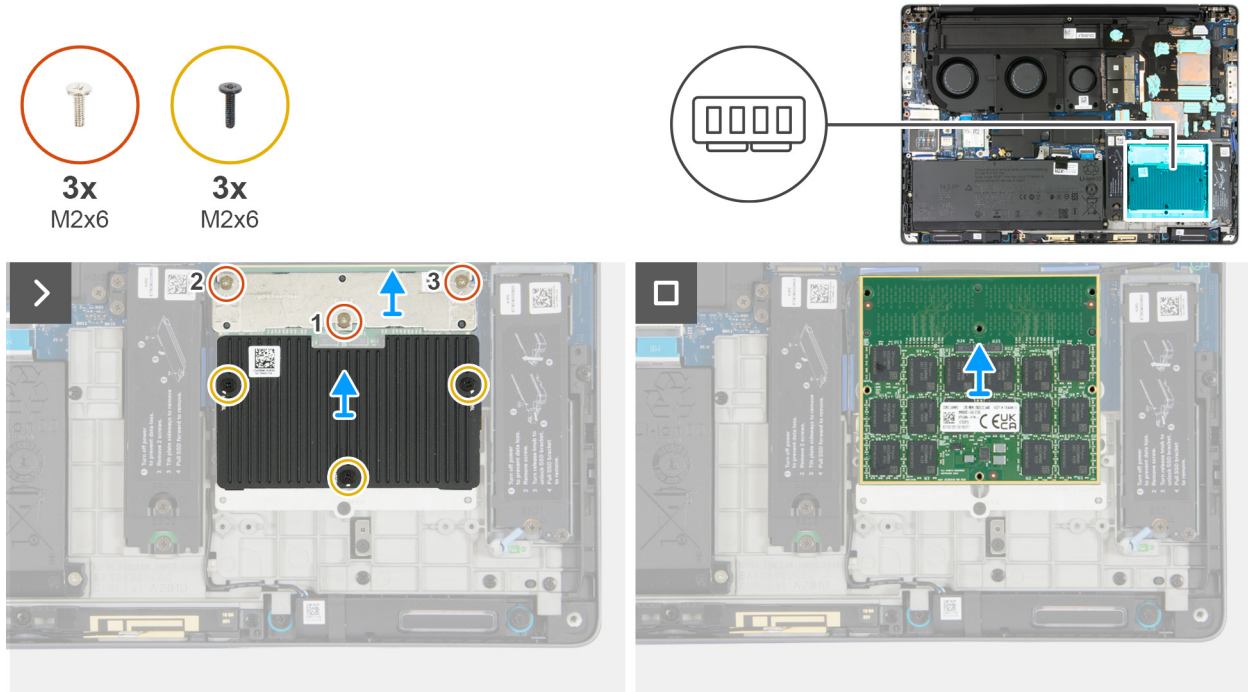
Ilustración 62. Extracción del módulo CAMM (doble canal)
