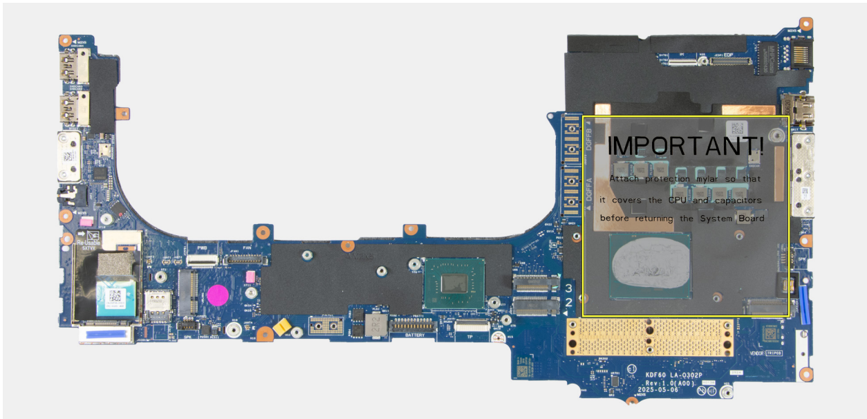
Ilustración 114. Preparación de la tarjeta madre defectuosa para su devolución
