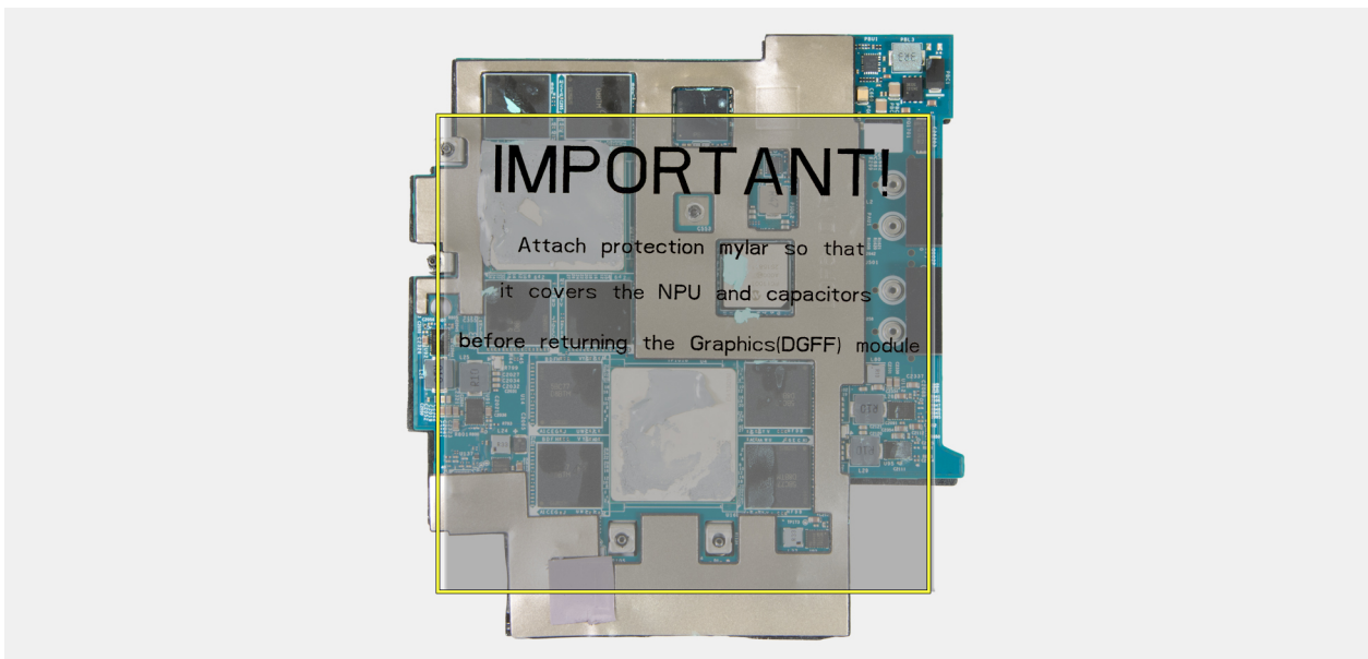
Ilustración 60. Pegue el mylar protector sobre las áreas de transferencia de calor y la DRAM
