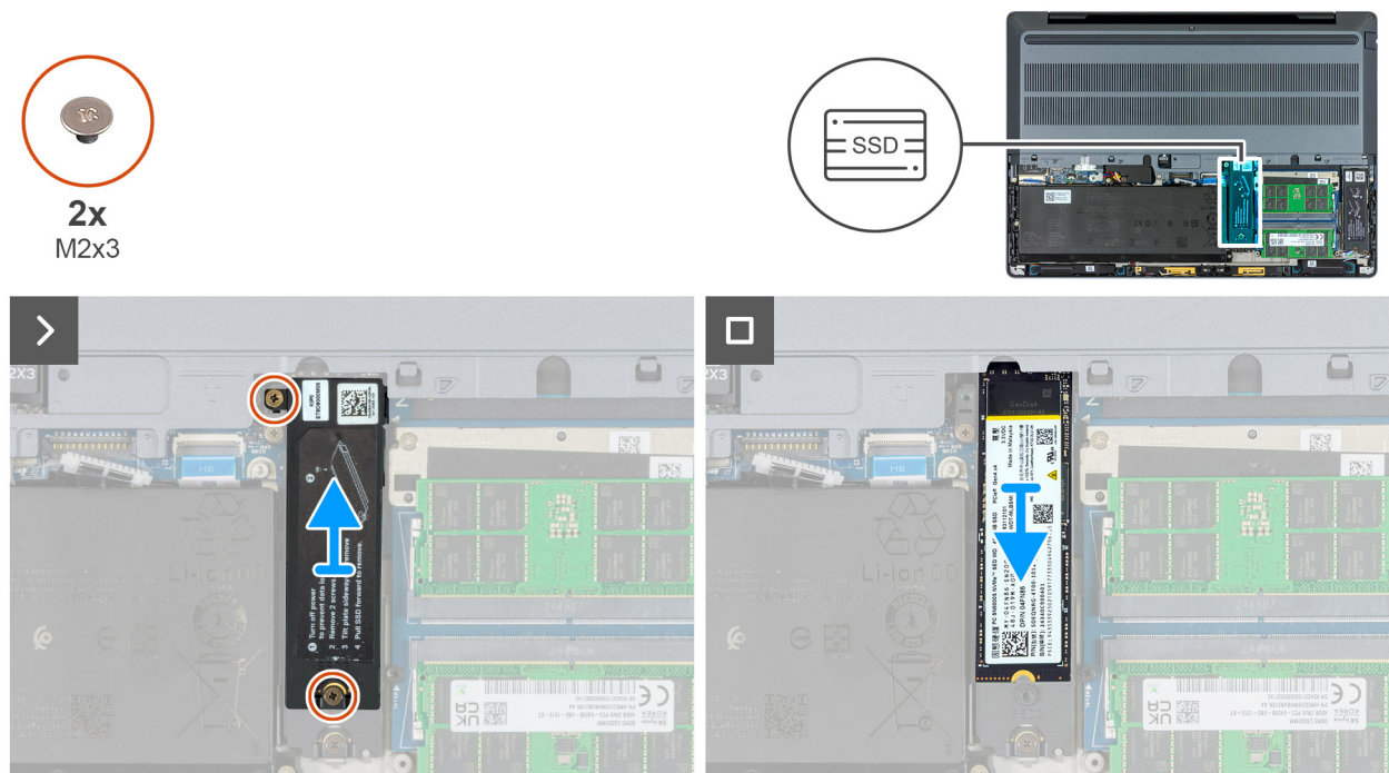
Ilustración 34. Extracción de la SSD M.2 2280 de la ranura 3 (SSD3)
