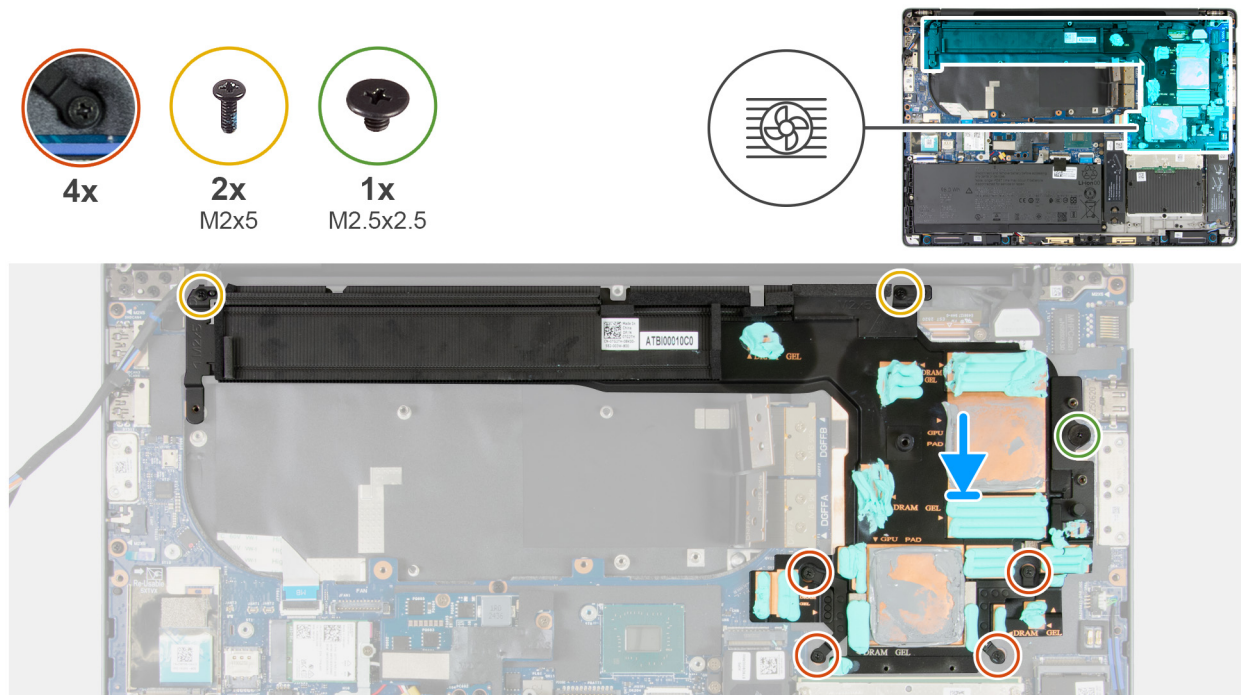
Ilustración 77. Instalación del disipador de calor en computadoras enviadas con gráficos integrados
