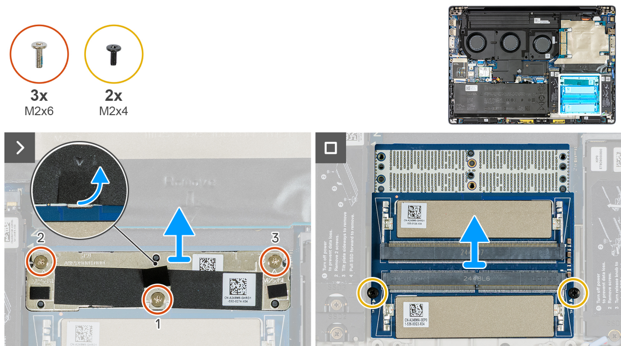
Ilustración 70. Extracción de la placa intercaladora de memoria
