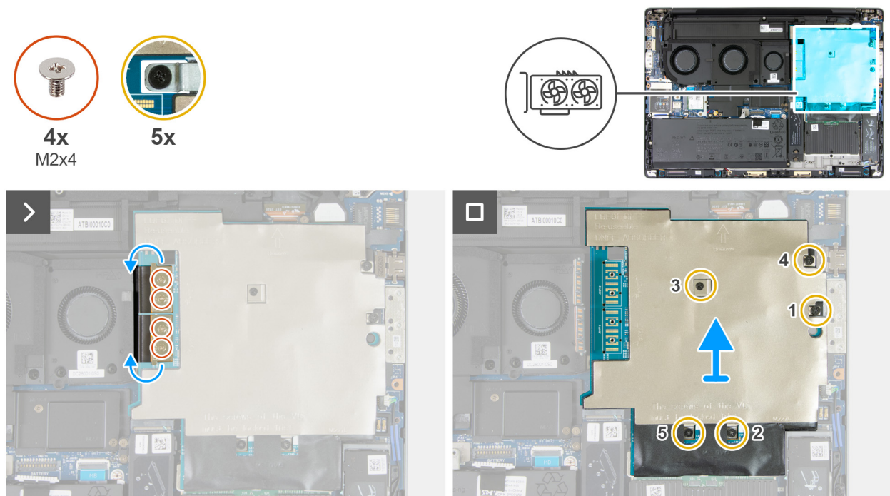
Ilustración 59. Extracción de la tarjeta NPU
