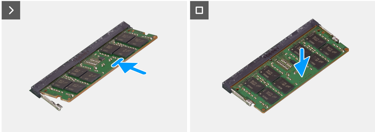
Ilustración 31. Instalación del módulo de memoria
