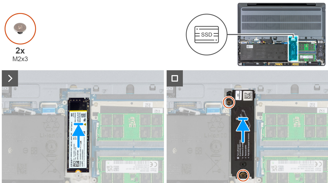
Ilustración 37. Instalación de la SSD M.2 2280 en la ranura 2 (SSD2)
