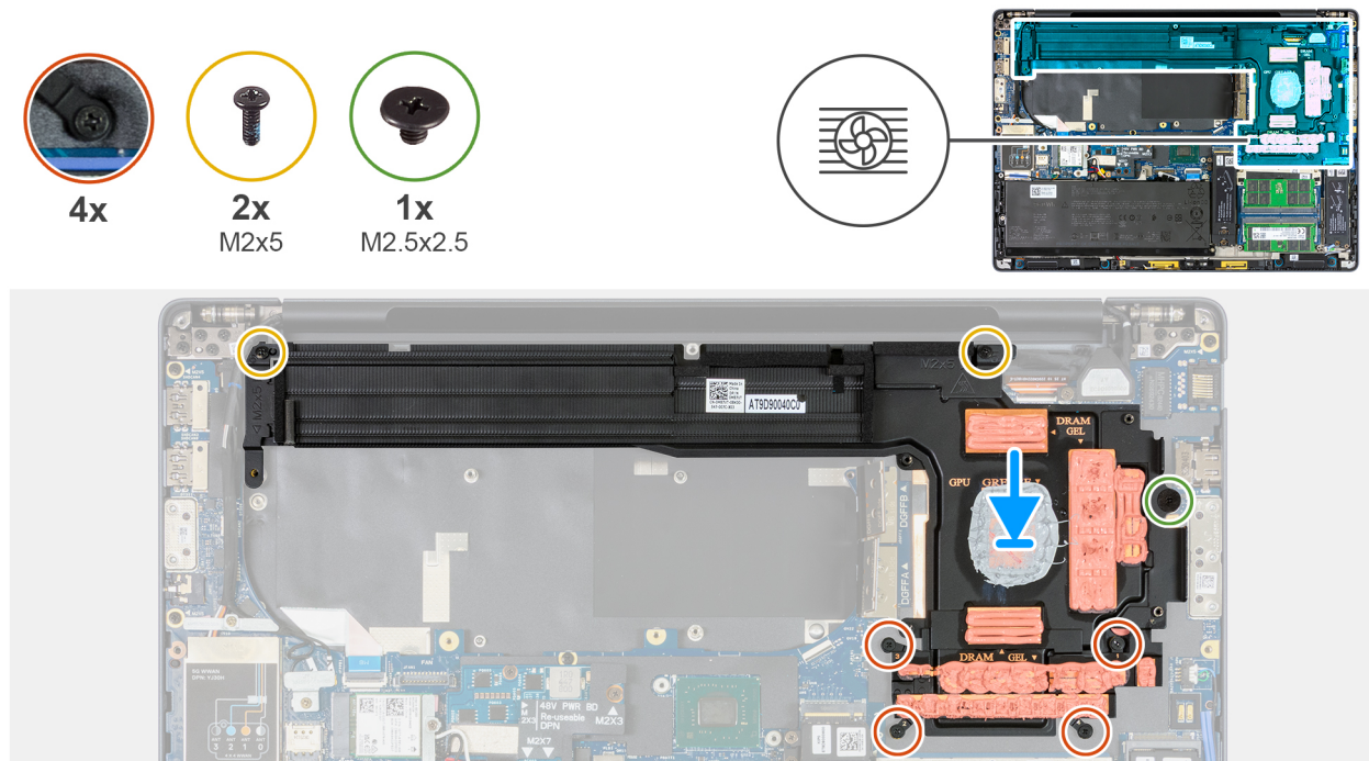
Ilustración 79. Instalación del disipador de calor en computadoras enviadas con gráficos discretos
