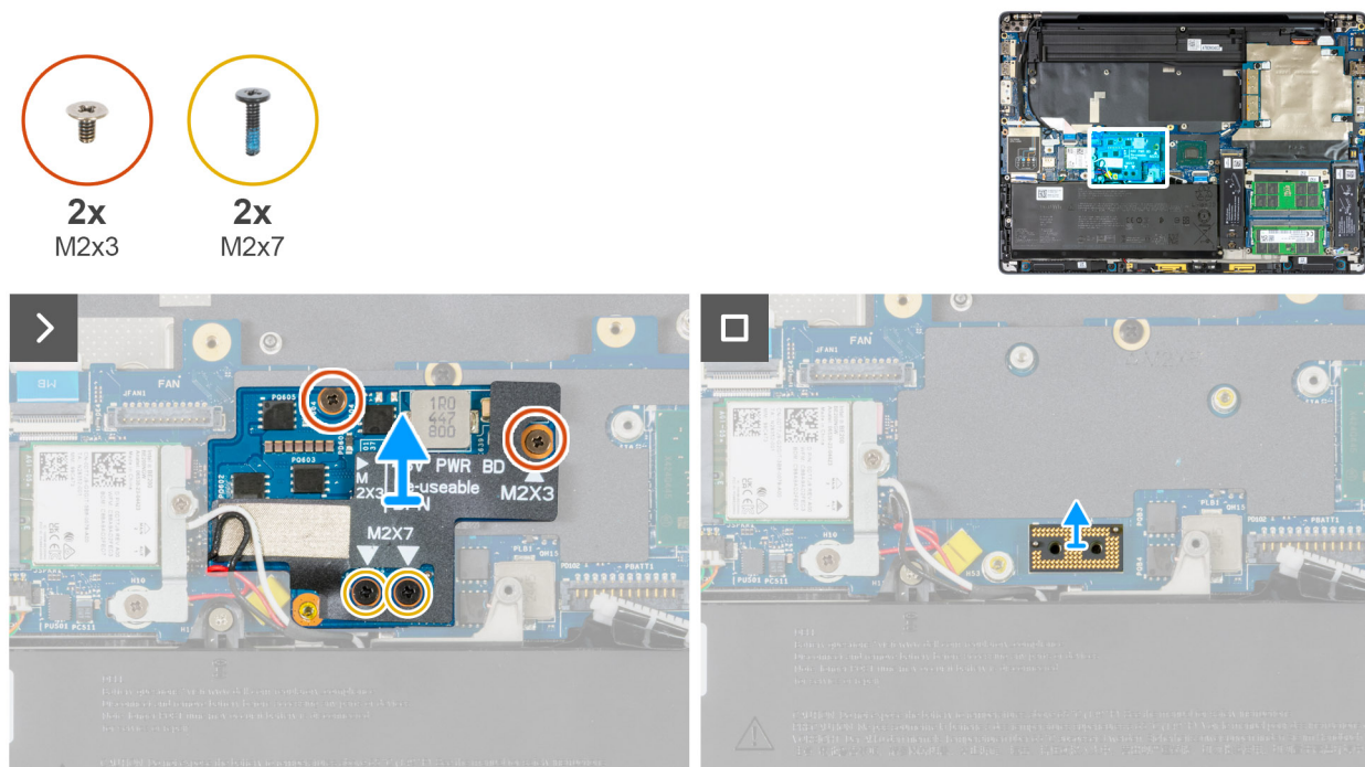
Ilustración 74. Extracción de la placa de alimentación
