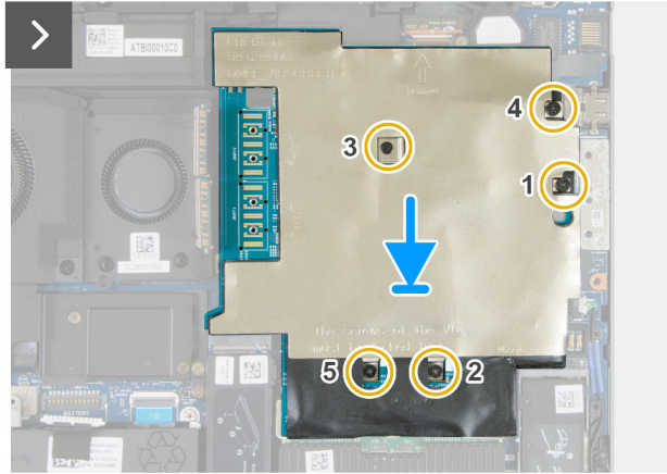
Ilustración 61. Instalación de la tarjeta NPU
