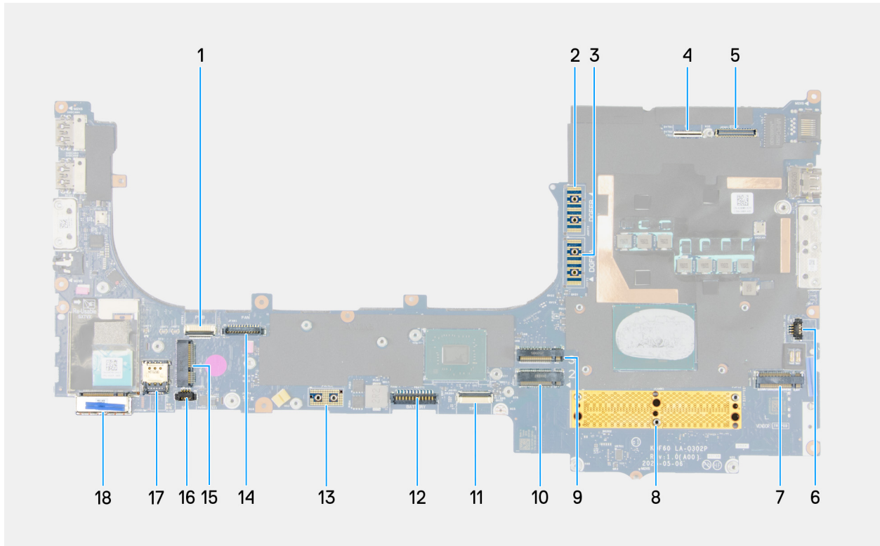
Ilustración 115. Componentes de la tarjeta madre del sistema
