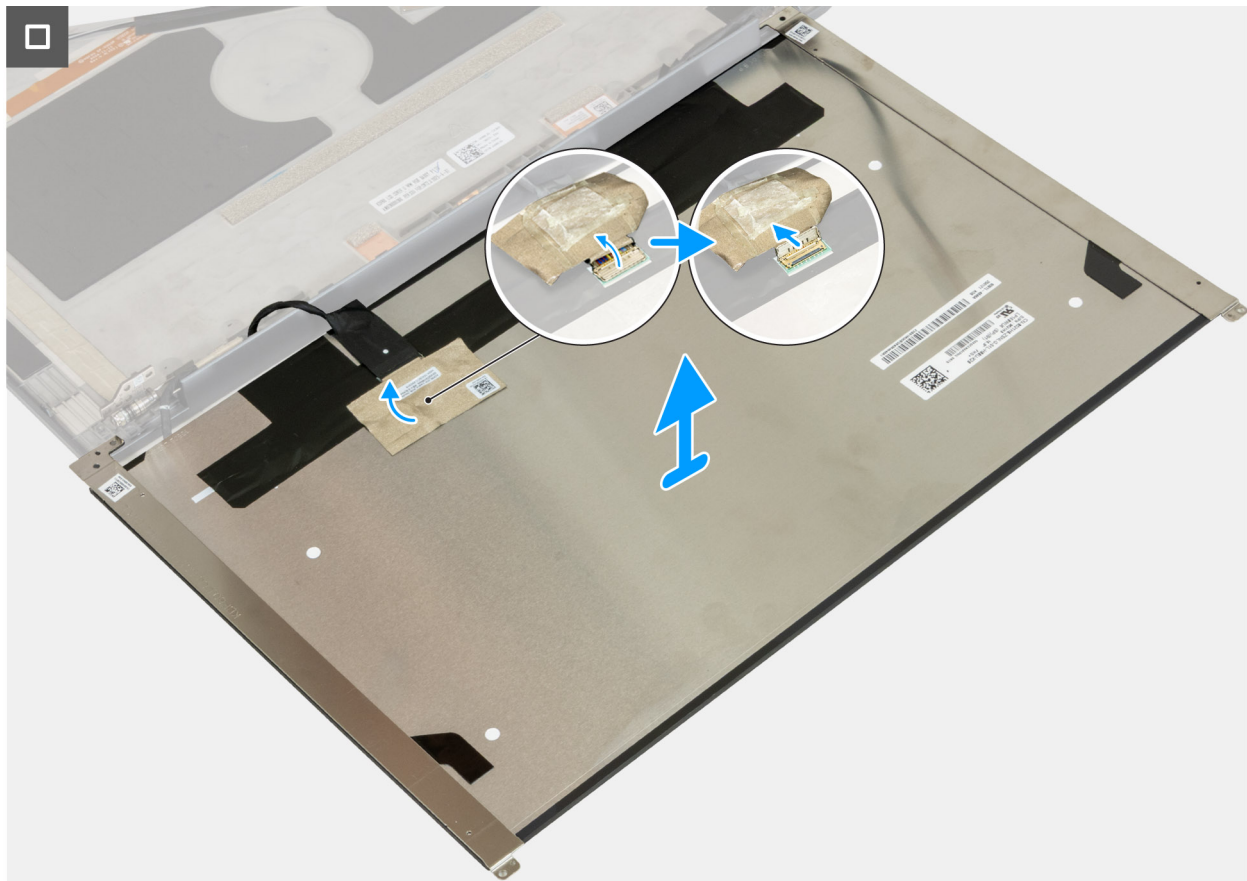
Ilustración 95. Extracción del panel de pantalla para pantallas táctiles
