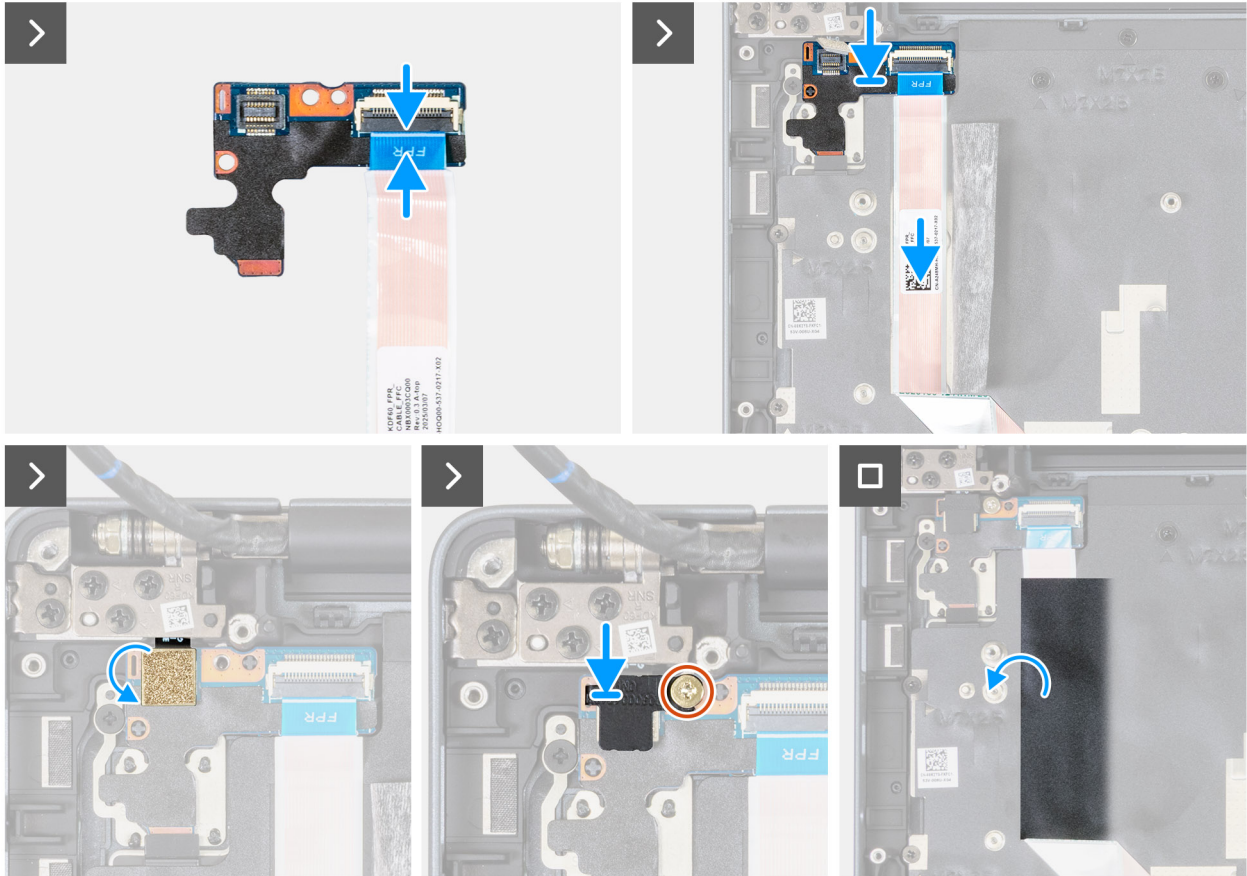
Ilustración 129. Instalación de la placa del botón de encendido
