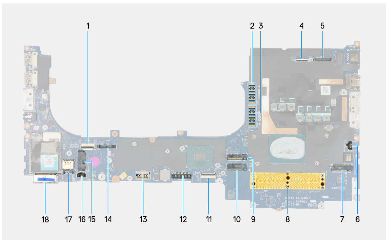
Ilustración 111. Componentes de la tarjeta madre del sistema
