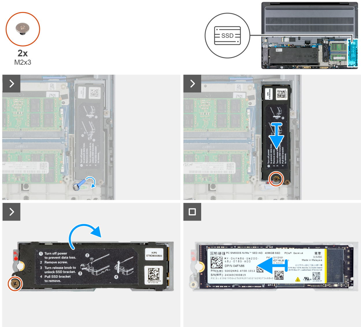
Ilustración 32. Extracción de la SSD M.2 2280 de la ranura 1 (SSD1)
