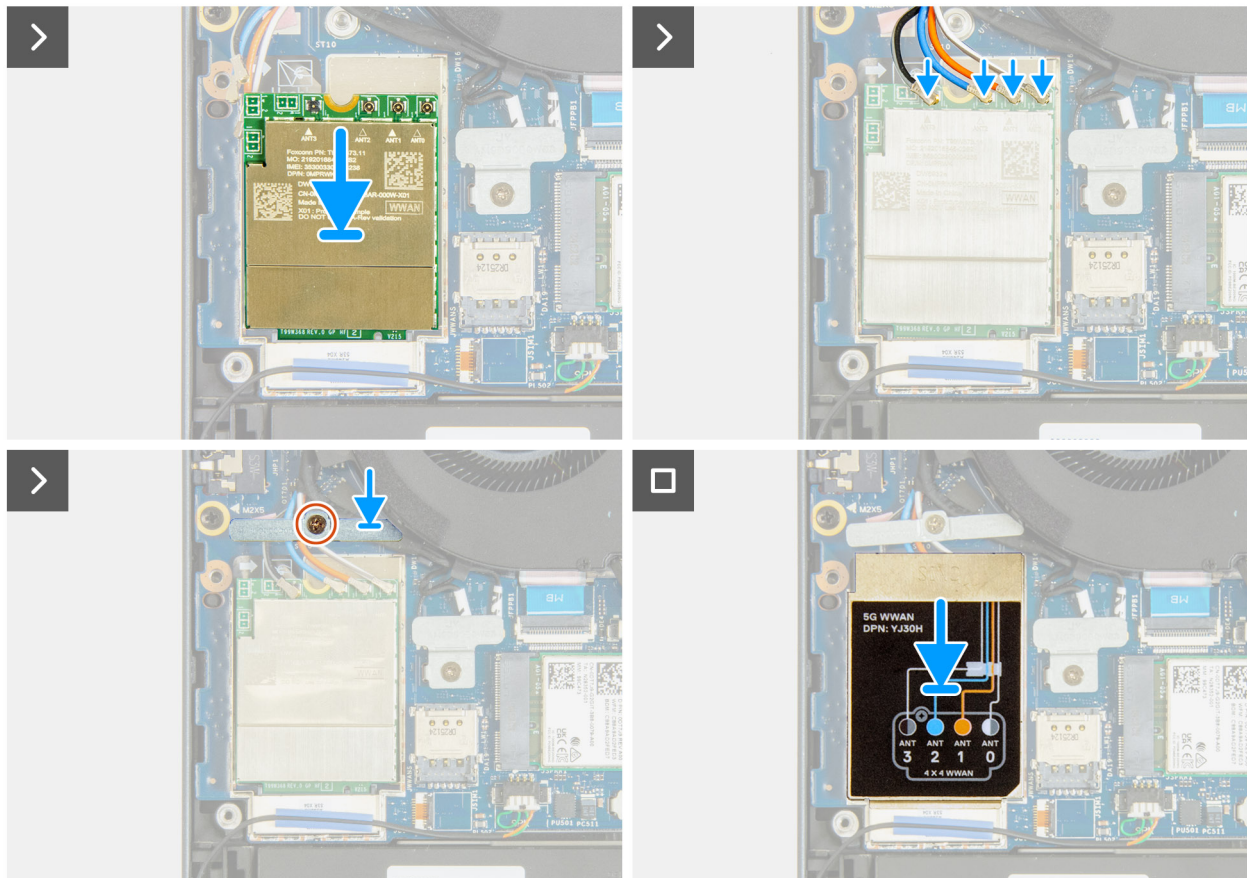
Ilustración 49. Instalación de la tarjeta WWAN
