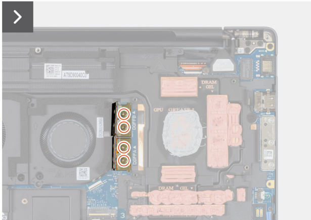
Ilustración 55. Extracción del conector de haz discreto FPC
