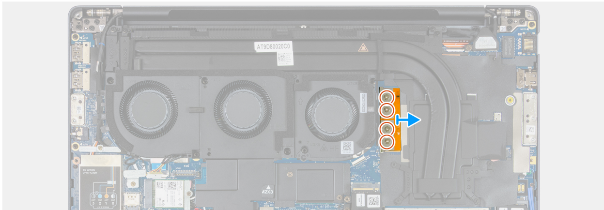
Ilustración 53. Extracción del conector de haz FPC integrado
