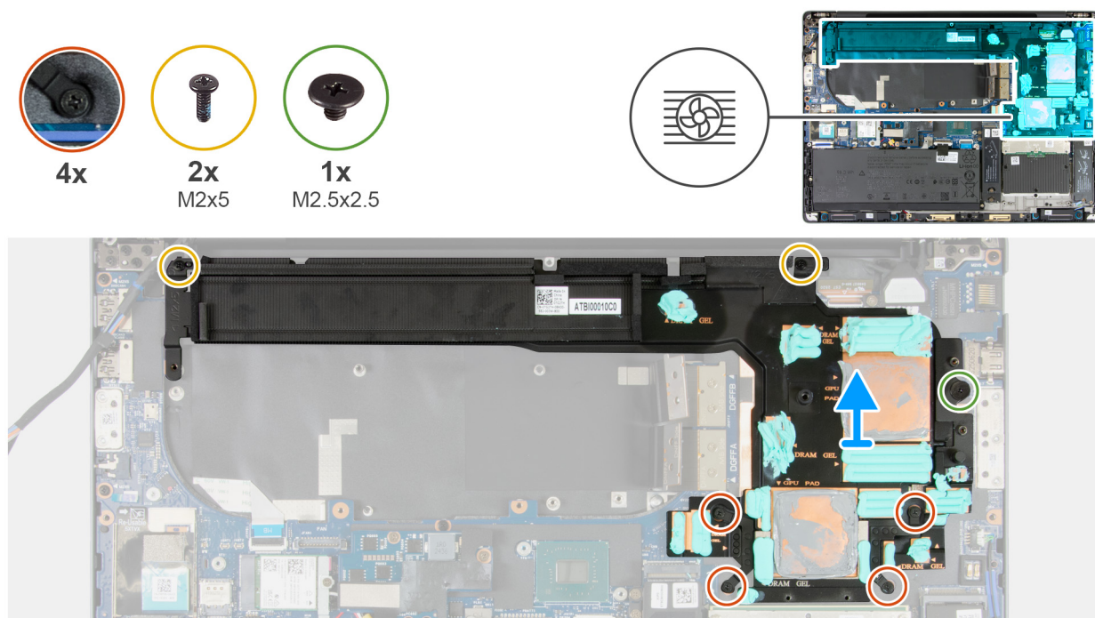
Ilustración 76. Extracción del disipador de calor en computadoras enviadas con gráficos integrados
