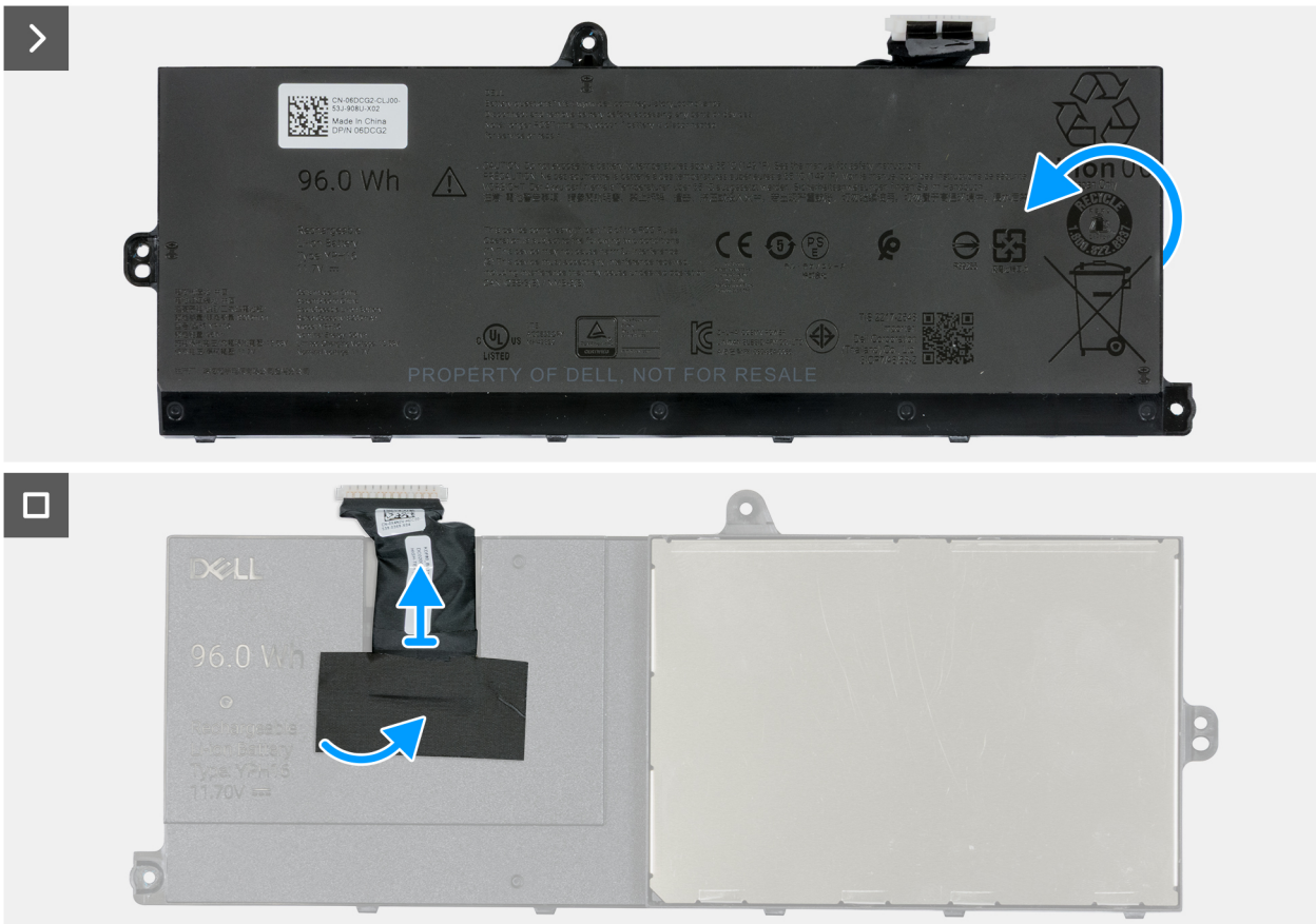
Ilustración 41. Extracción del cable de la batería de la batería
