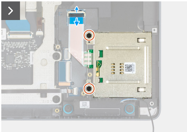
Ilustración 124. Extracción del lector de tarjetas inteligentes
