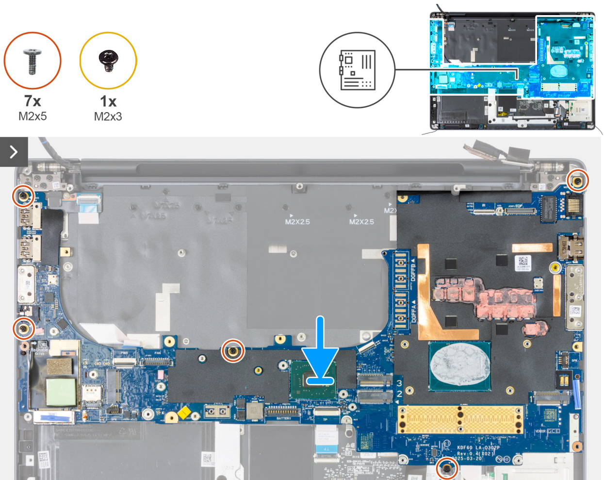
Ilustración 116. Instalación de la tarjeta madre
