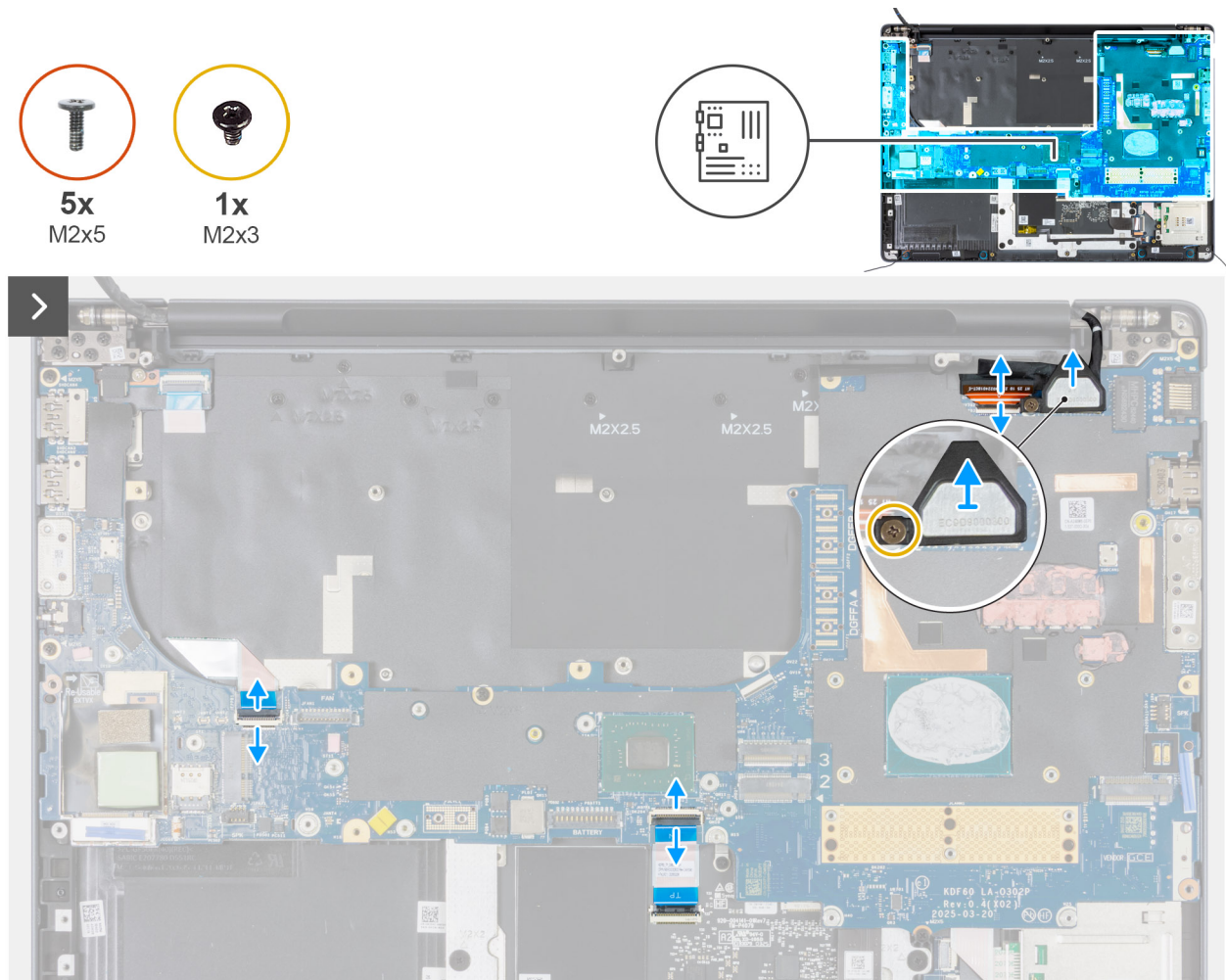
Ilustración 112. Extracción de la tarjeta madre
