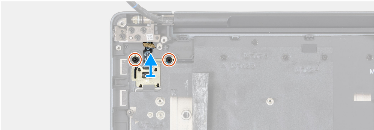
Ilustración 130. Extracción del botón de encendido
