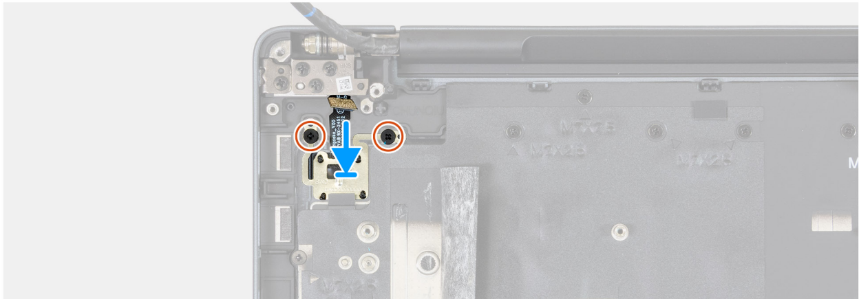
Ilustración 131. Instalación del botón de encendido
