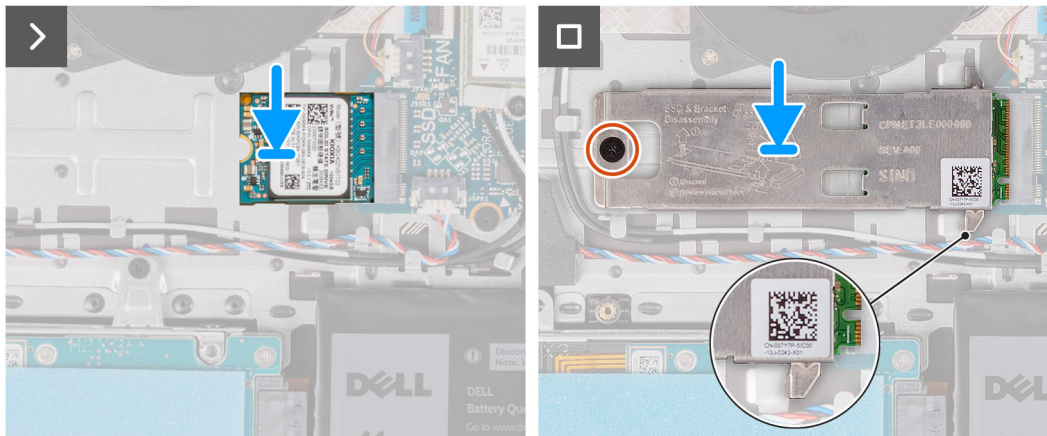
Ilustración 6. Instalación de la unidad de estado sólido
