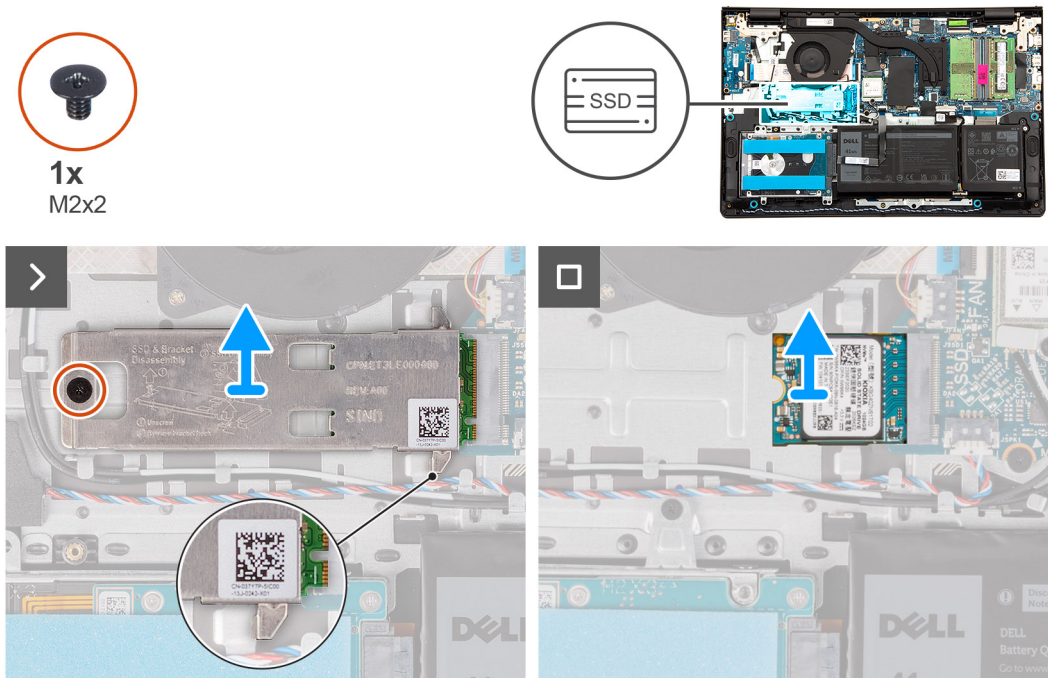
Ilustración 5. Extracción de la unidad de estado sólido
