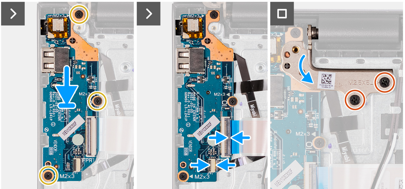
Ilustración 7. Instalación de la placa secundaria de I/O
