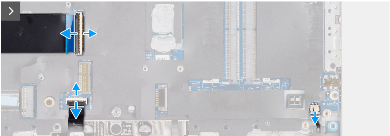
Figure 43. Retrait de la carte système
