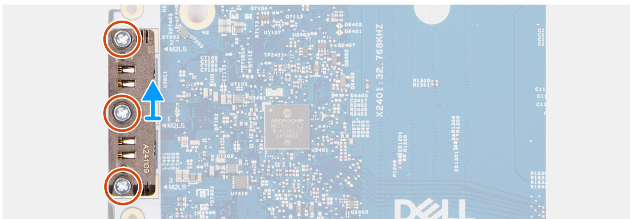
Figure 48. Retrait du module USB-C
