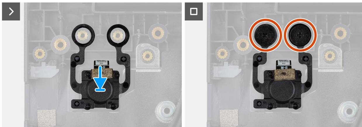
Figure 41. Installation du bouton d'alimentation avec lecteur d'empreintes digitales
