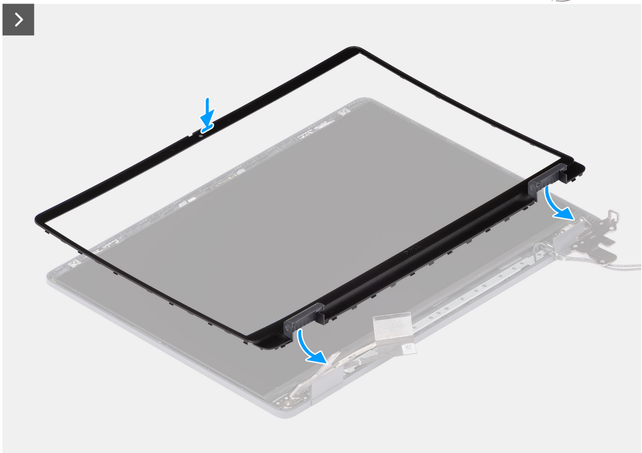
Figure 72. Installation de la bordure d'écran
