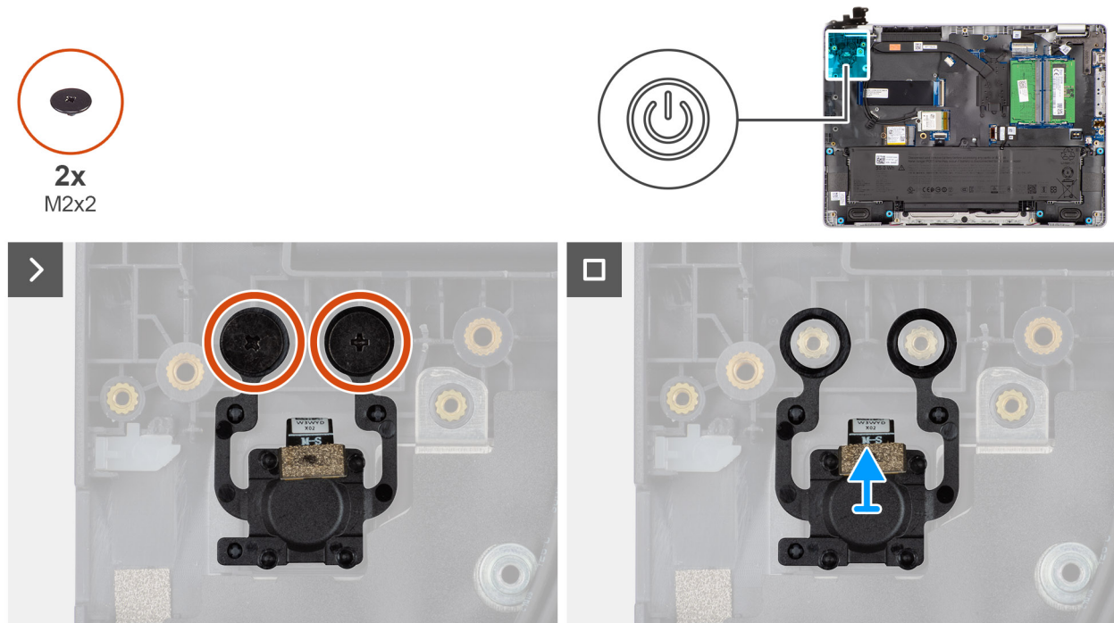
Figure 40. Retrait du bouton d'alimentation avec lecteur d'empreintes digitales
