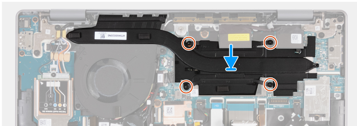
Figure 46. Installation du dissipateur de chaleur
