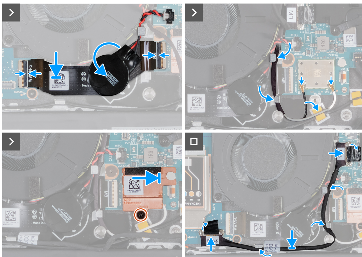
Figure 58. Installation du câble FPC de la carte des E/S
