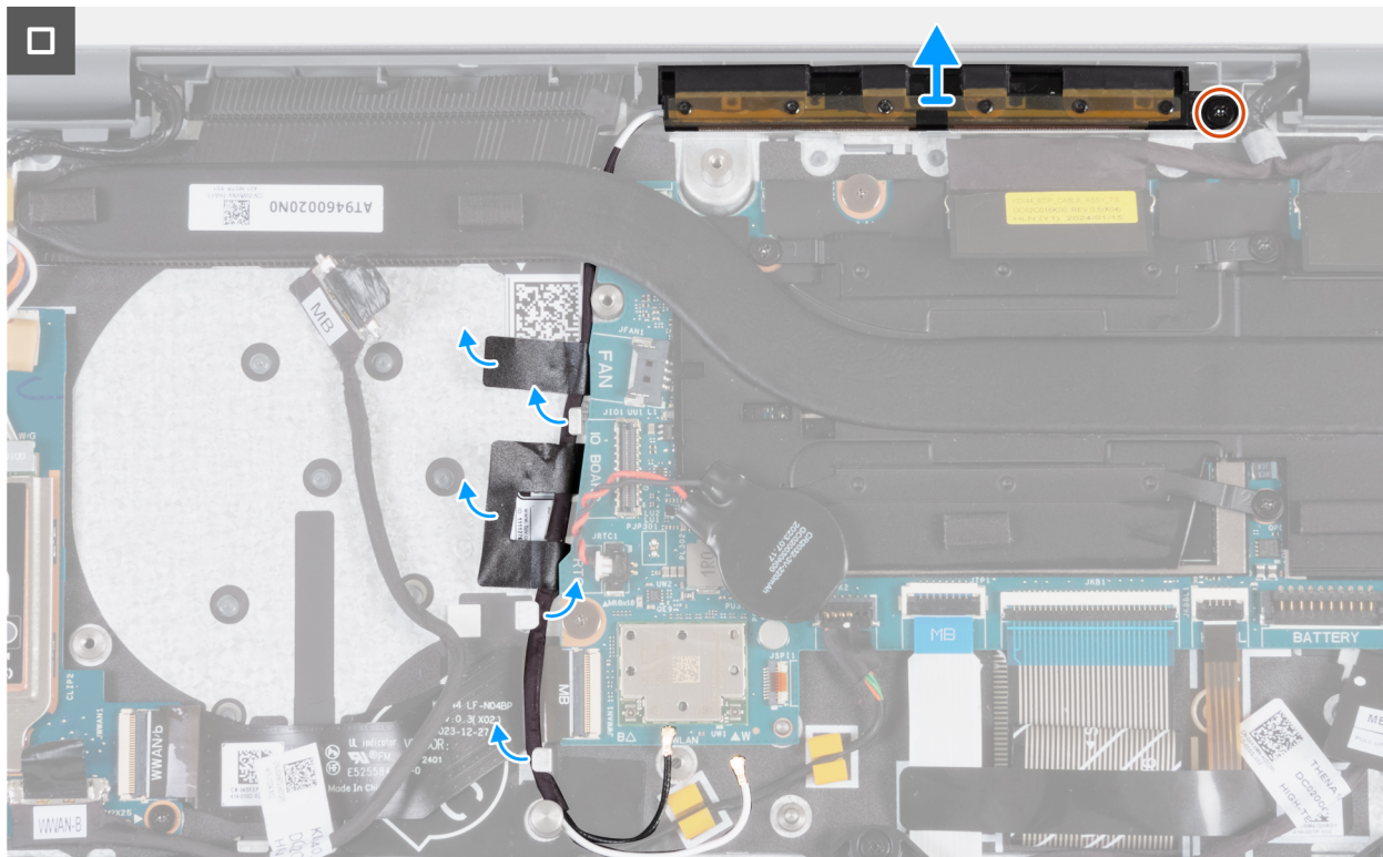
Figure 67. Retrait du module d'antenne WLAN
