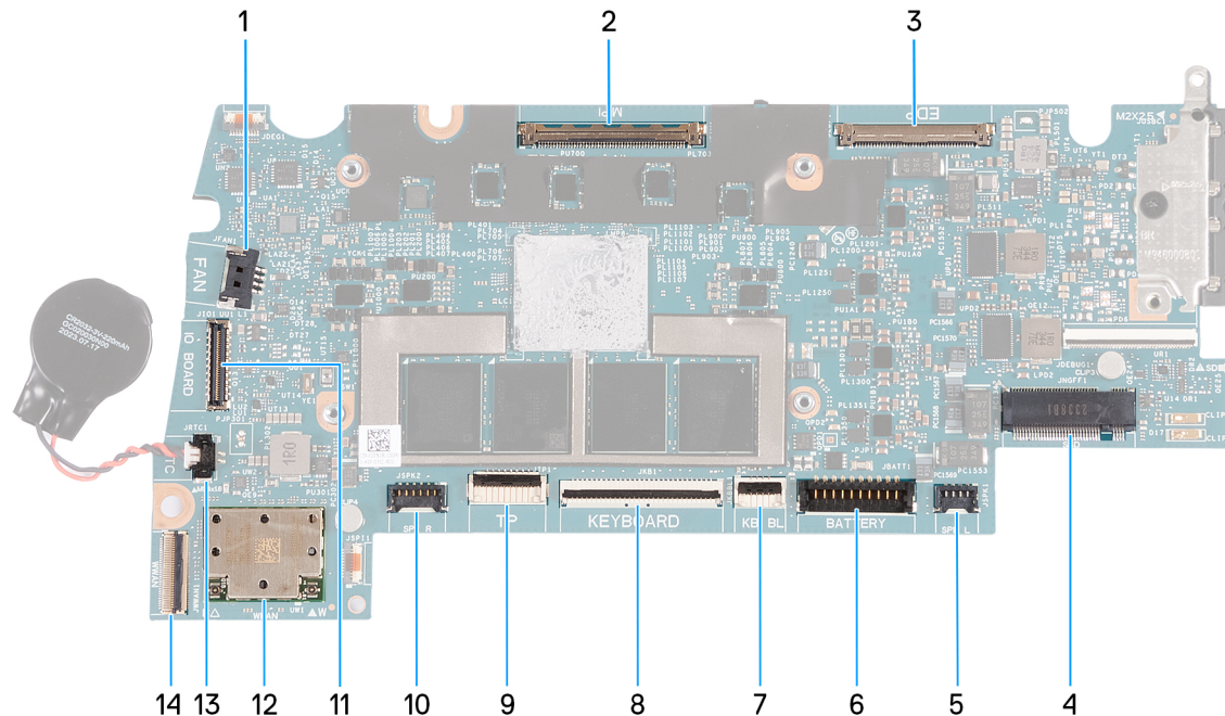
Figure 98. Connecteurs de la carte système
