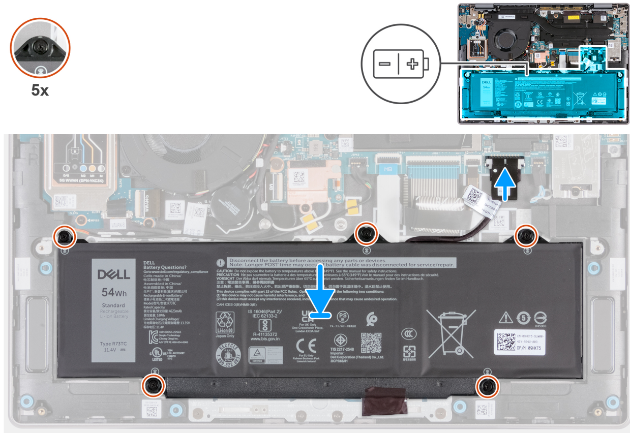
Figure 41. Installation de la batterie
