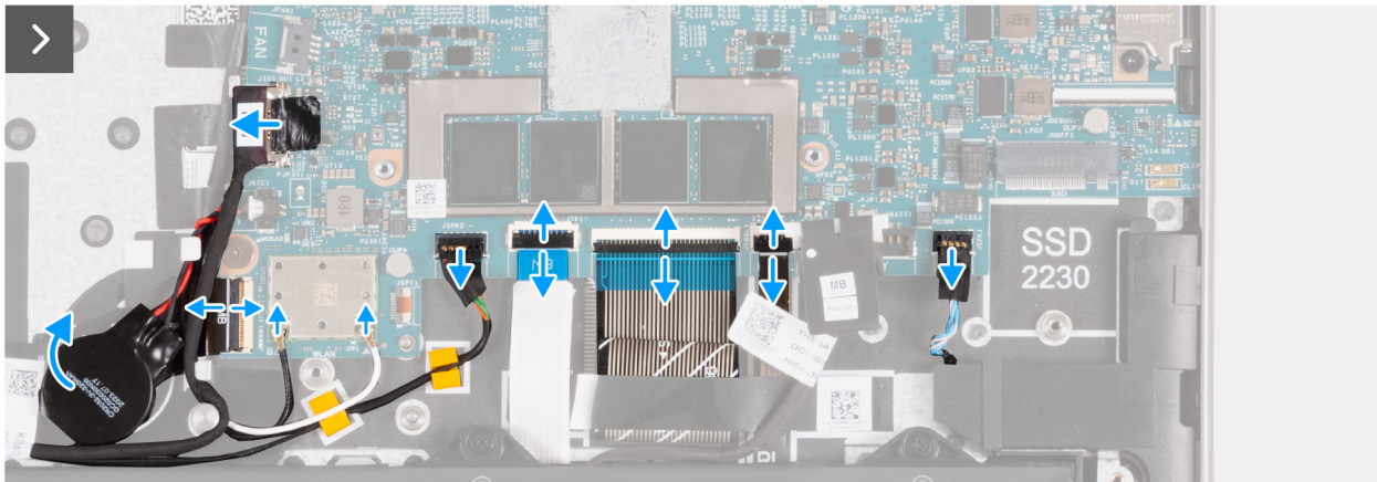
Figure 95. Retrait de la carte système
