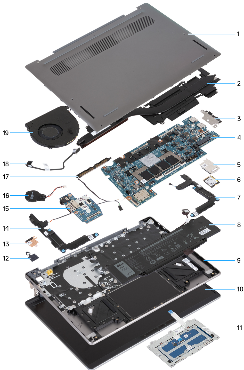
Figure 10. Principaux composants de l'ordinateur Latitude 7455 (ordinateurs expédiés avec une prise en charge WLAN uniquement)
