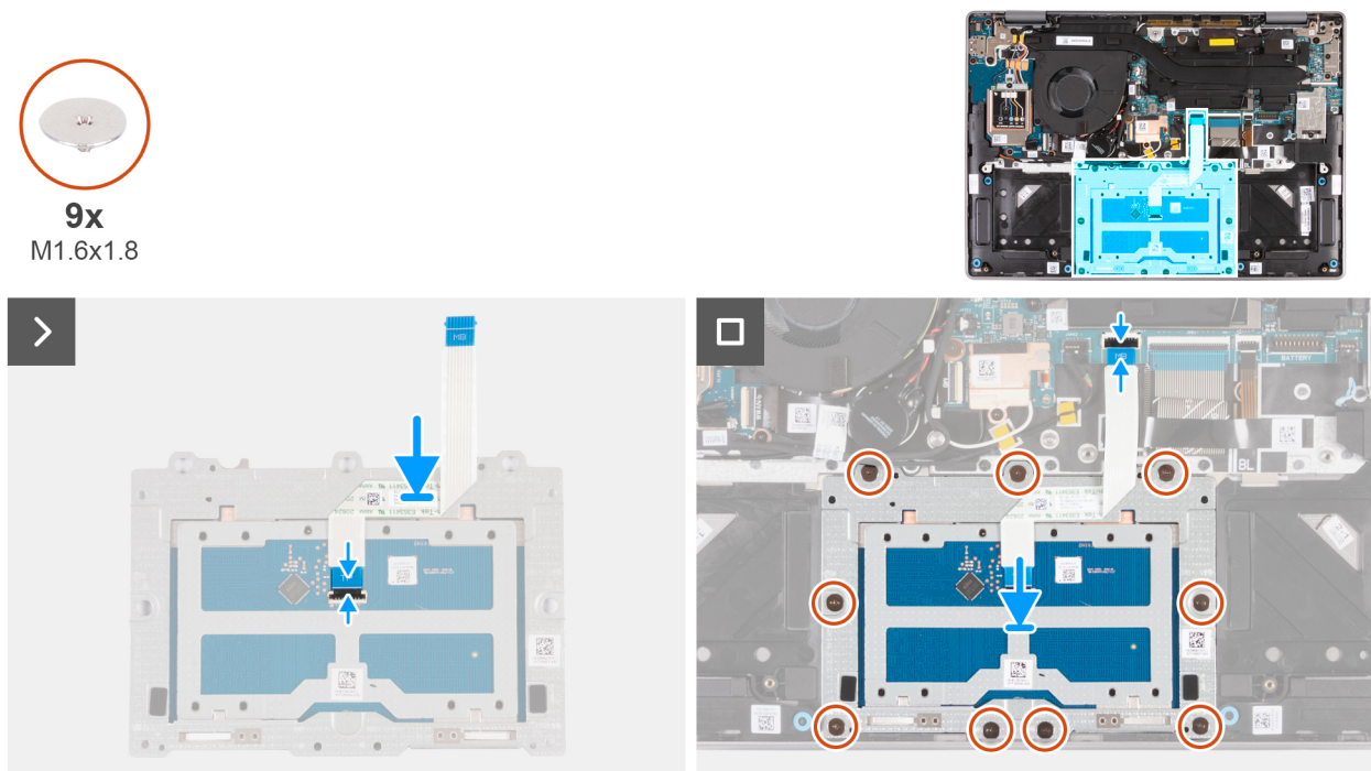
Figure 88. Installation de l'assemblage du pavé tactile
