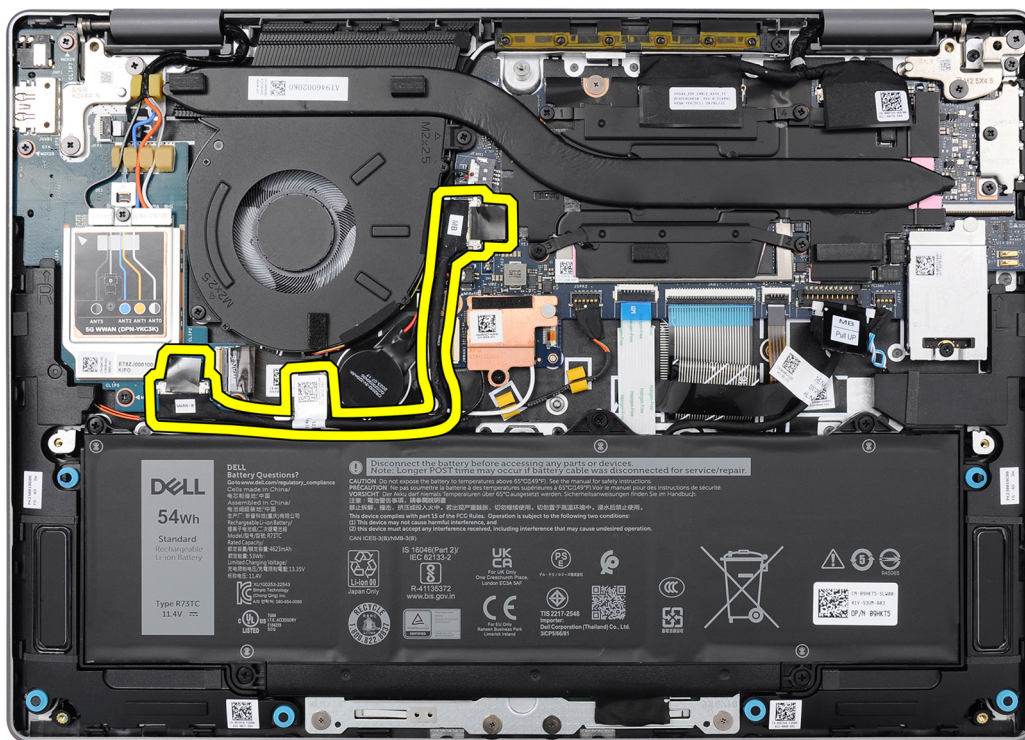
Figure 55. Emplacement du câble de la carte d'E/S
