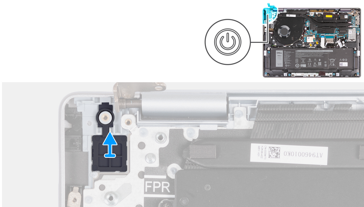
Figure 89. Retrait du bouton d'alimentation
