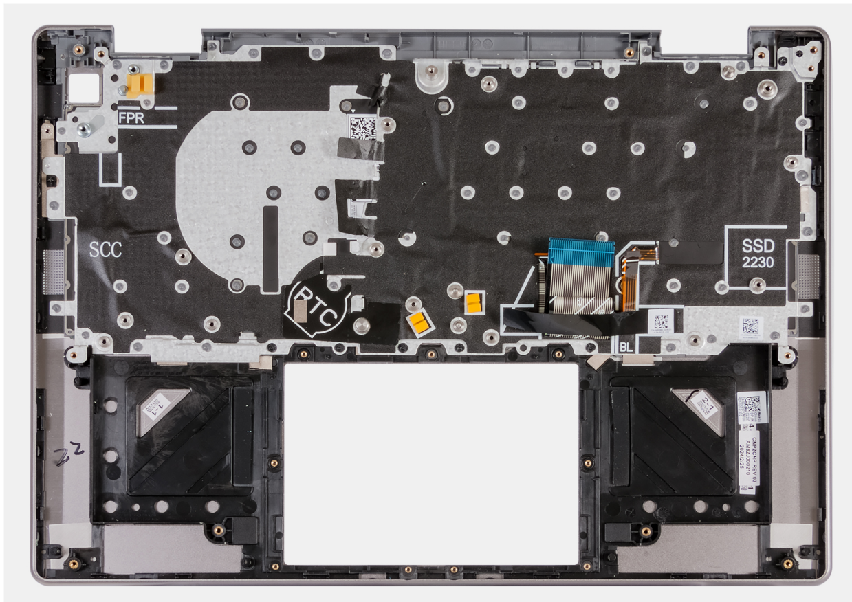
Figure 102. Assemblage du repose-poignets et du clavier
