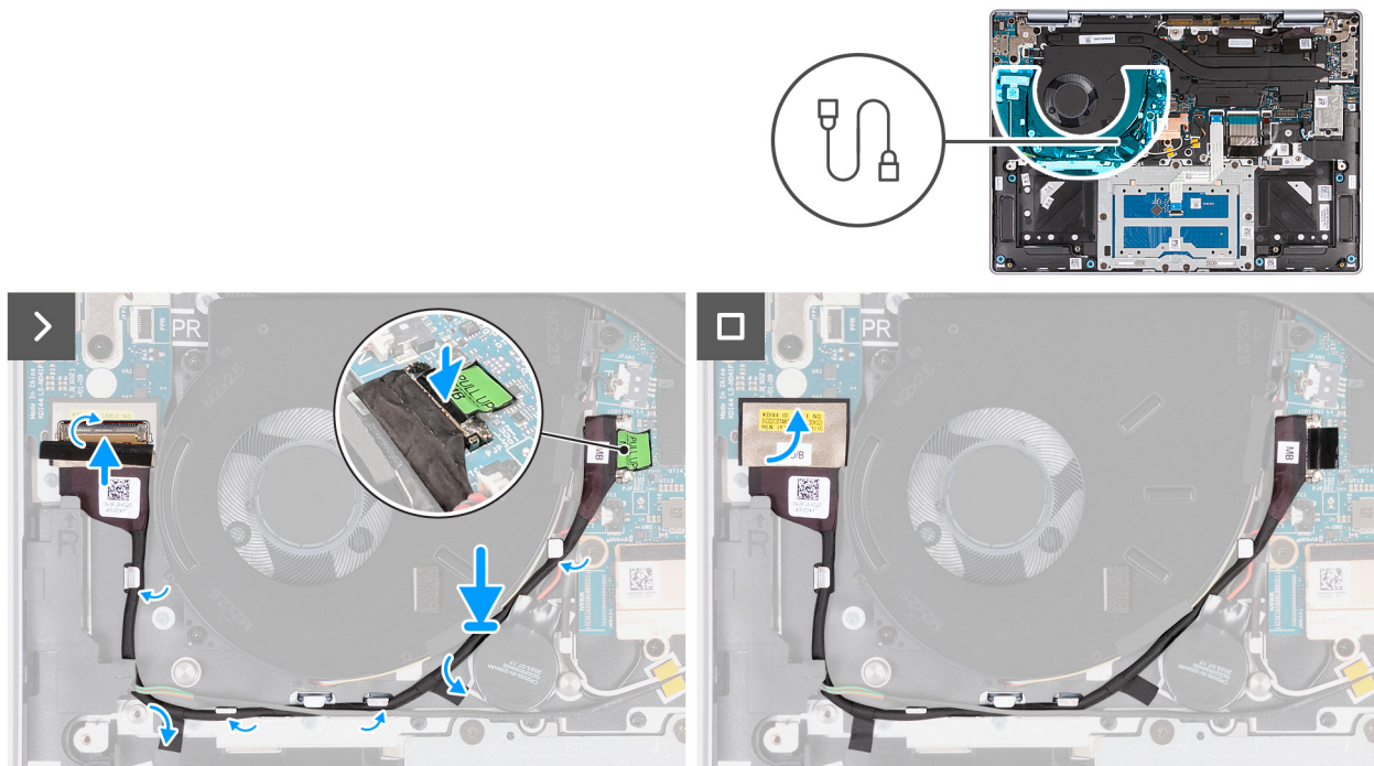
Figure 52. Installation du câble de la carte d'E/S (pour les ordinateurs expédiés avec une prise en charge WLAN uniquement)
