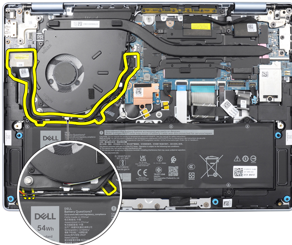
Figure 51. Emplacement du câble de la carte d'E/S
