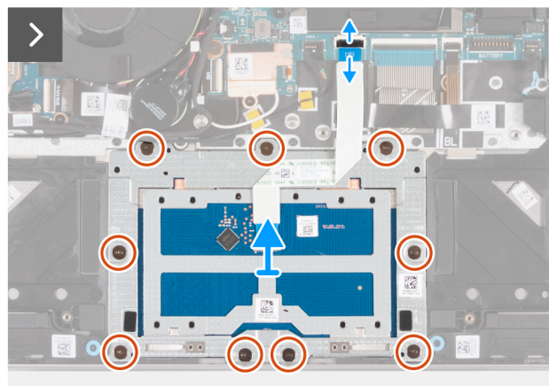
Figure 87. Retrait de l'assemblage du pavé tactile
