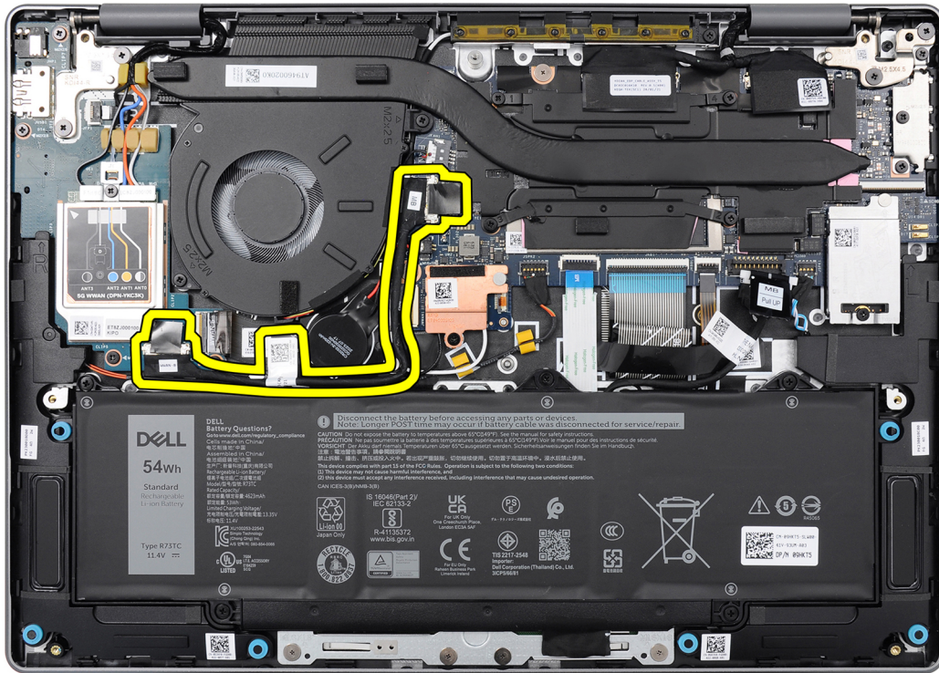
Figure 53. Emplacement du câble de la carte d'E/S
