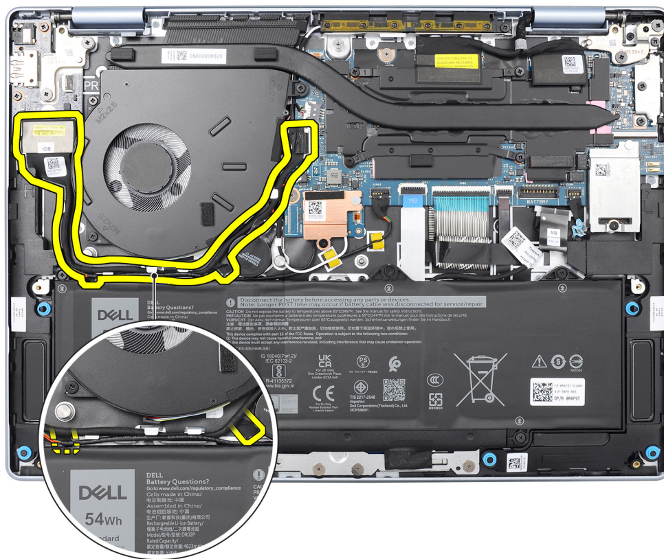
Figure 49. Emplacement du câble de la carte d'E/S
