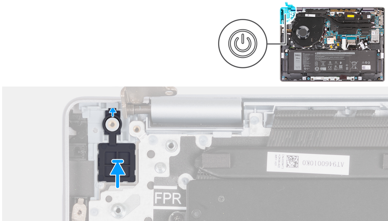
Figure 91. Installation du bouton d'alimentation
