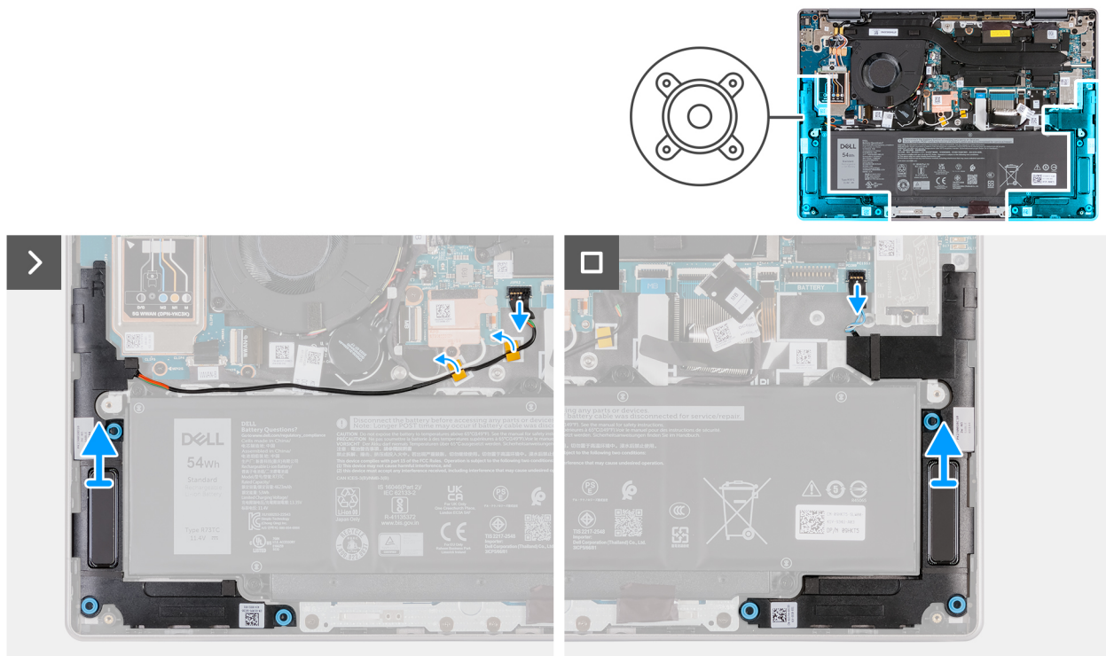
Figure 32. Retrait des haut-parleurs
