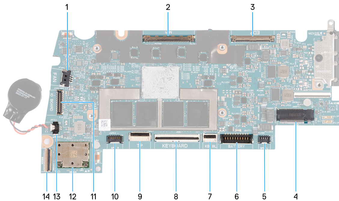
Figure 94. Connecteurs de la carte système
