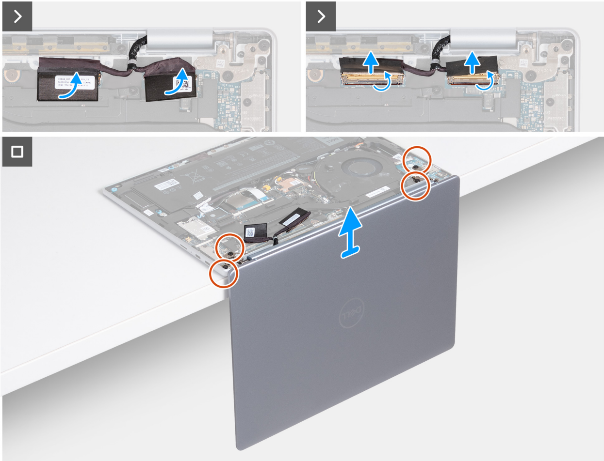
Figure 75. Retrait de l'assemblage d'écran (pour les ordinateurs expédiés avec une prise en charge WLAN uniquement)
