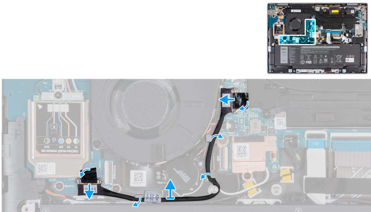
Figure 54. Retrait du câble de la carte d'E/S (pour les ordinateurs expédiés avec une prise en charge WWAN)
