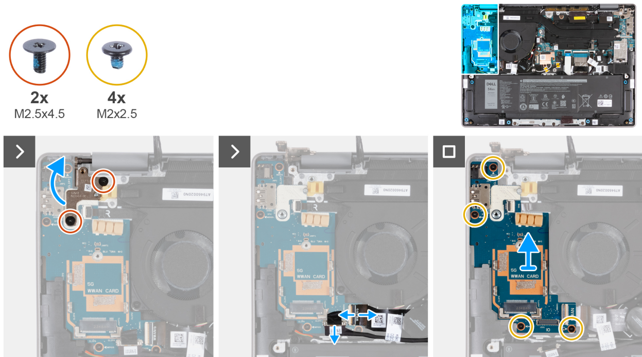
Figure 85. Retrait de la carte d'E/S (pour les ordinateurs expédiés avec une prise en charge WWAN)
