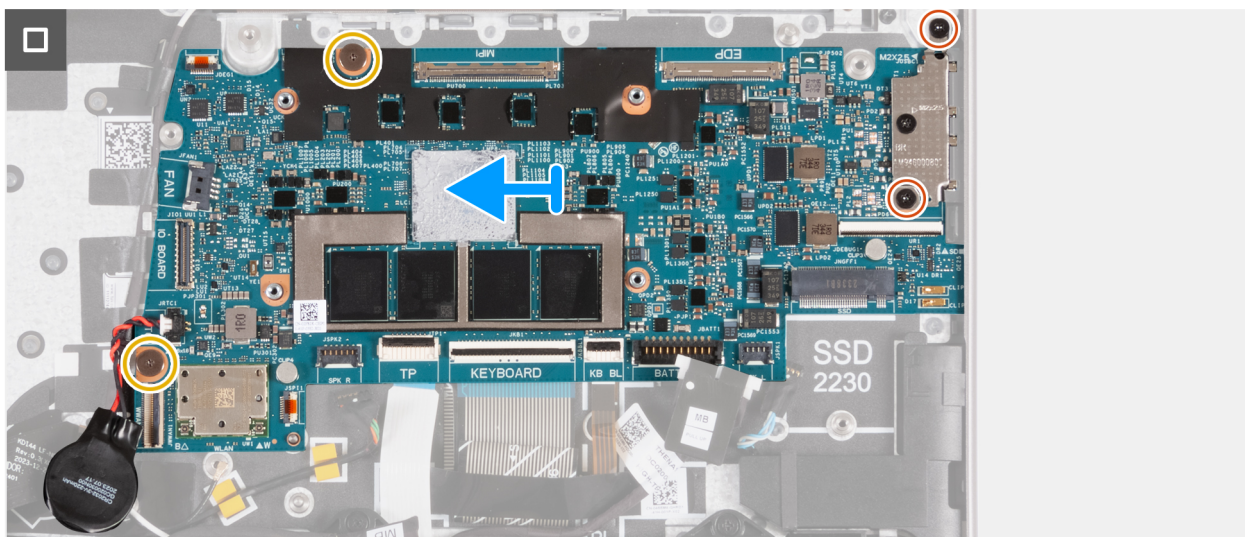
Figure 96. Retrait de la carte système
