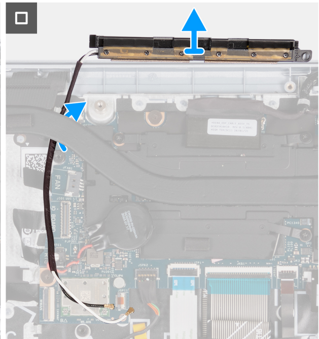
Figure 59. Retrait du module d'antenne WLAN (pour les ordinateurs expédiés avec une prise en charge WLAN uniquement)
