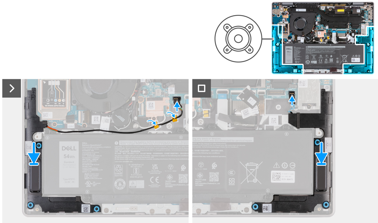
Figure 34. Installation des haut-parleurs
