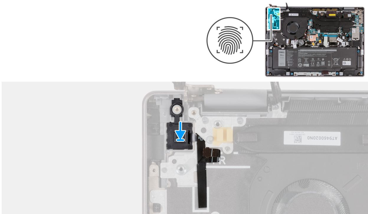
Figure 92. Installation du bouton d'alimentation avec lecteur d'empreintes digitales
