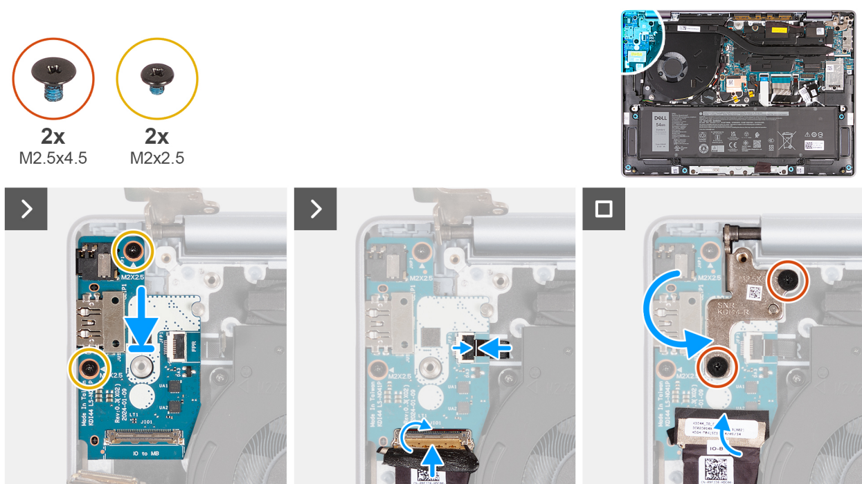
Figure 84. Installation de la carte d'E/S (pour les ordinateurs expédiés avec une prise en charge WLAN uniquement)
