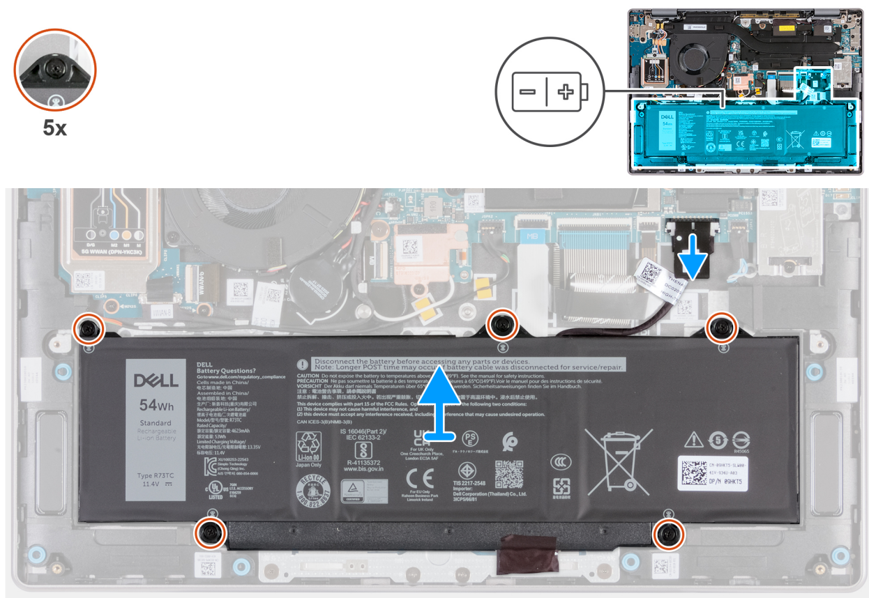
Figure 40. Retrait de la batterie
