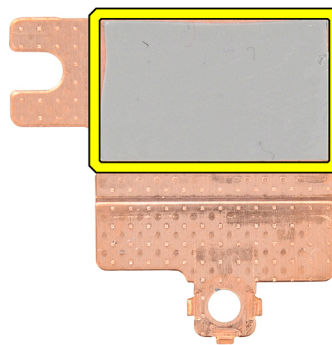
Figure 68. Tampon thermique sous la protection thermique WLAN
