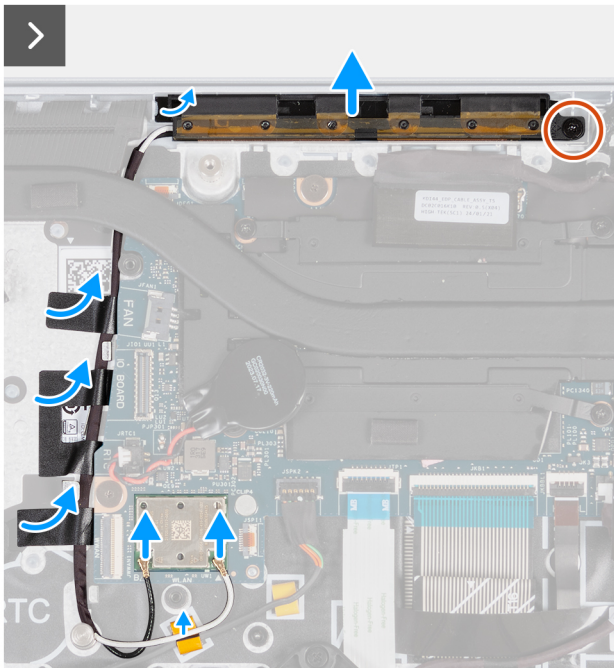
Figure 59. Retrait du module d'antenne WLAN (pour les ordinateurs expédiés avec une prise en charge WLAN uniquement)
