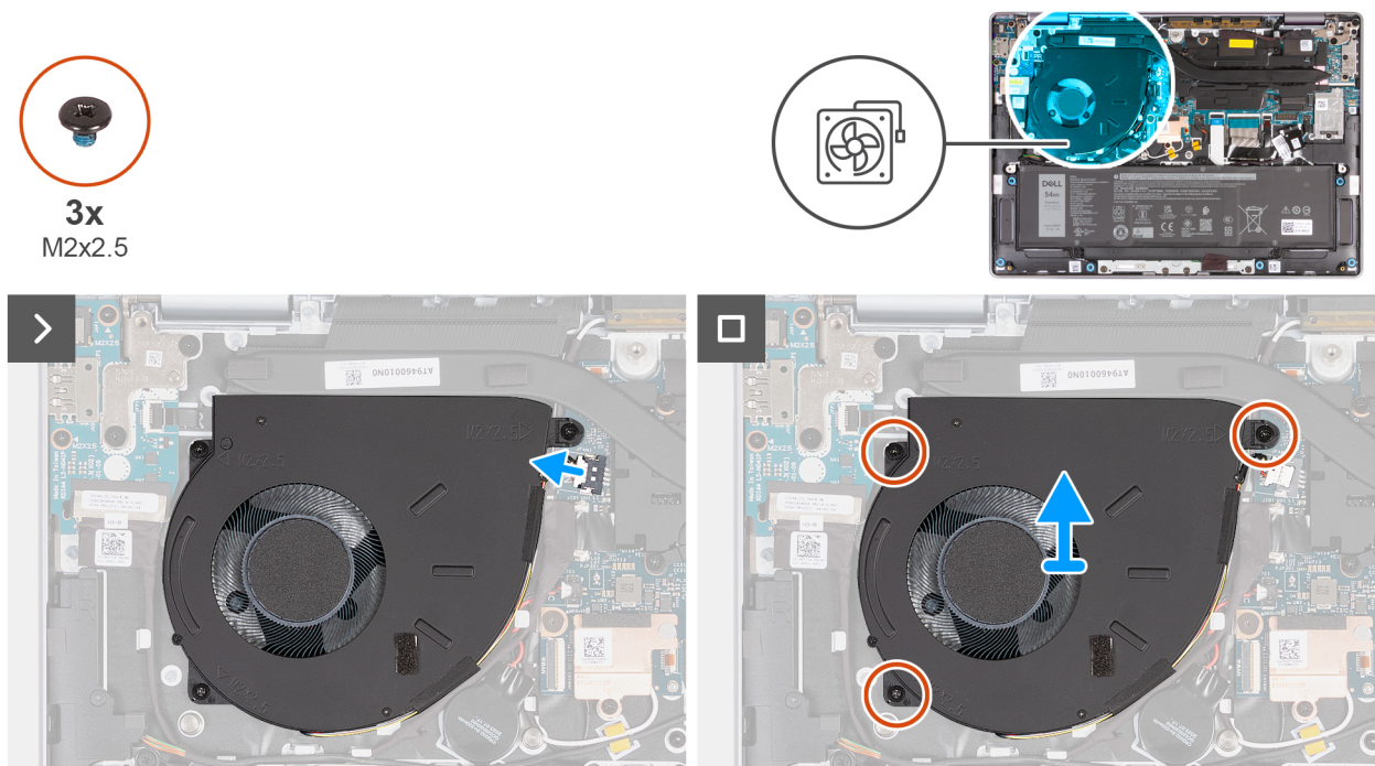
Figure 36. Retrait du ventilateur (pour les ordinateurs expédiés avec une prise en charge WLAN uniquement)
