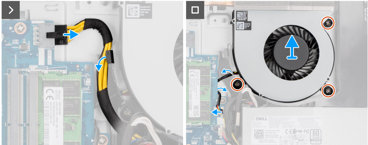
Ilustración 39. Extracción del ventilador
