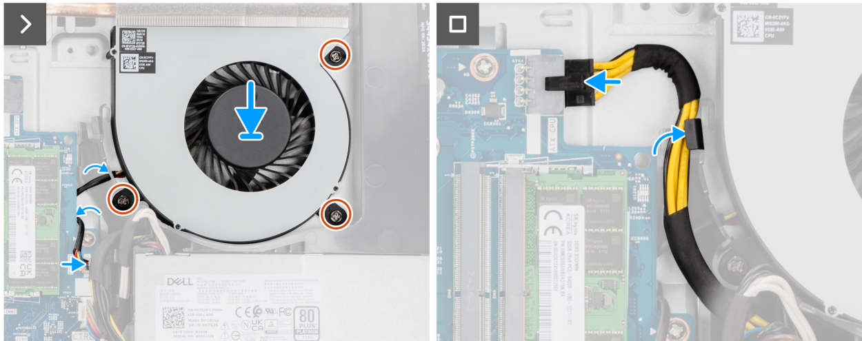
Ilustración 40. Instalación del ventilador
