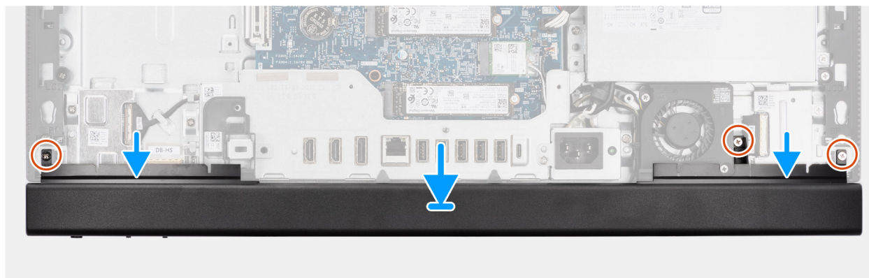
Ilustración 36. Instalación de la cubierta inferior
