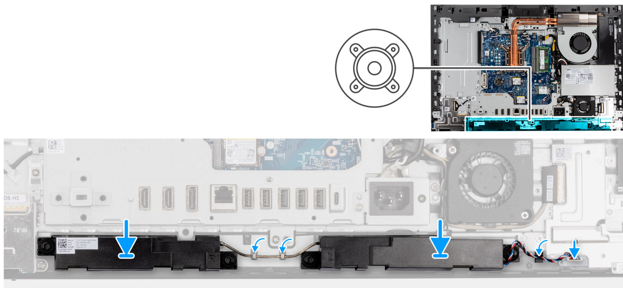
Ilustración 48. Instalación de los parlantes
