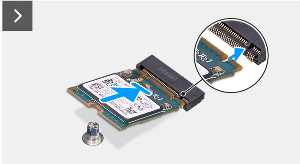
Ilustración 29. Instalación de la unidad de estado sólido M.2 2230 en la ranura M.2 1
