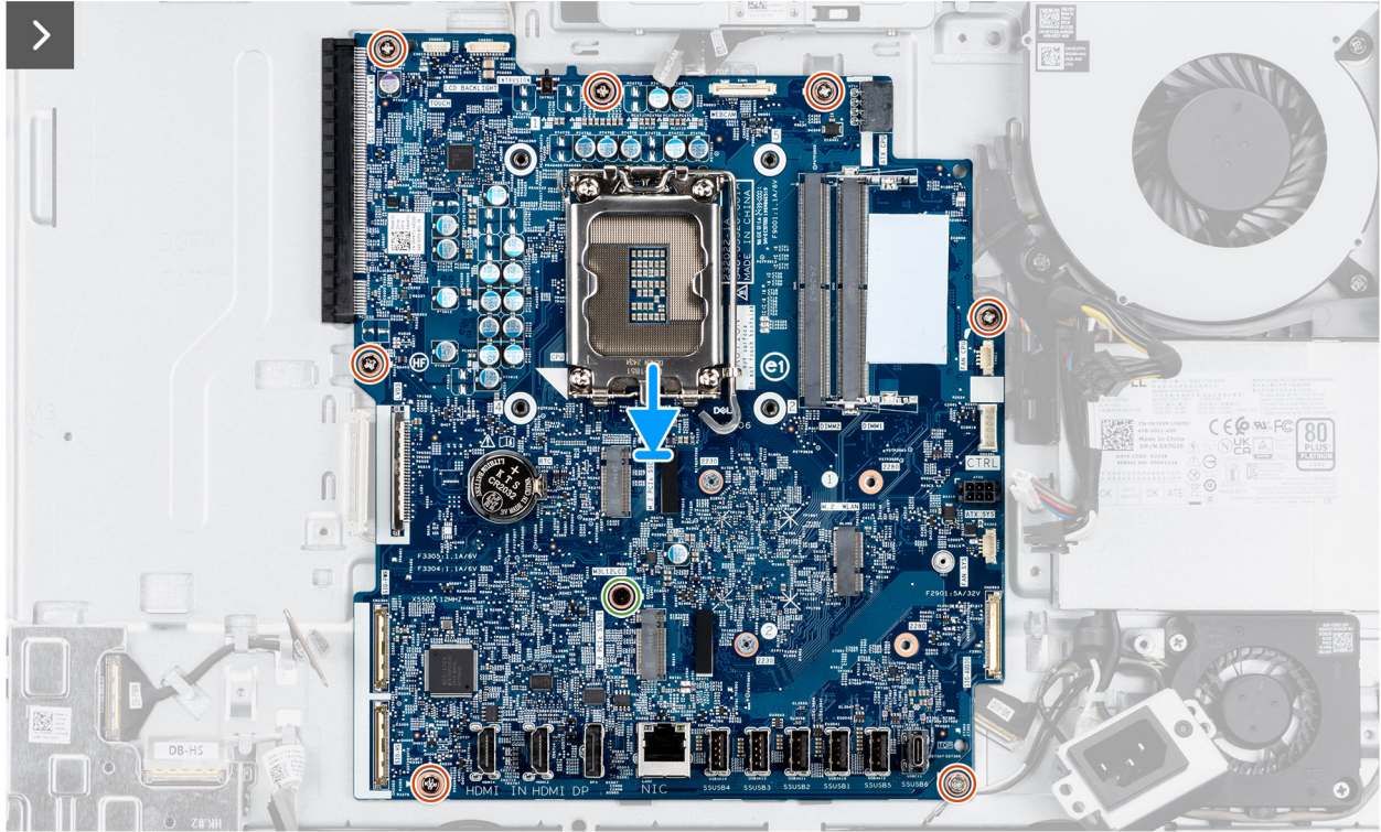
Ilustración 57. Instalación de la tarjeta madre
