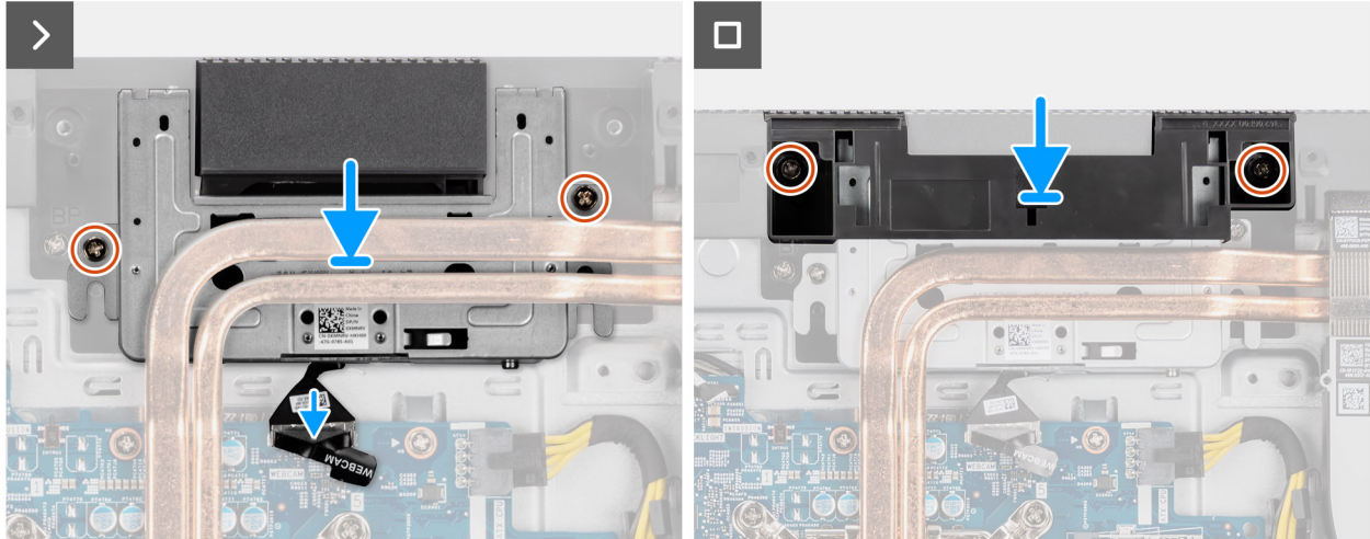
Ilustración 38. Instalación del ensamblaje de la cámara retráctil
