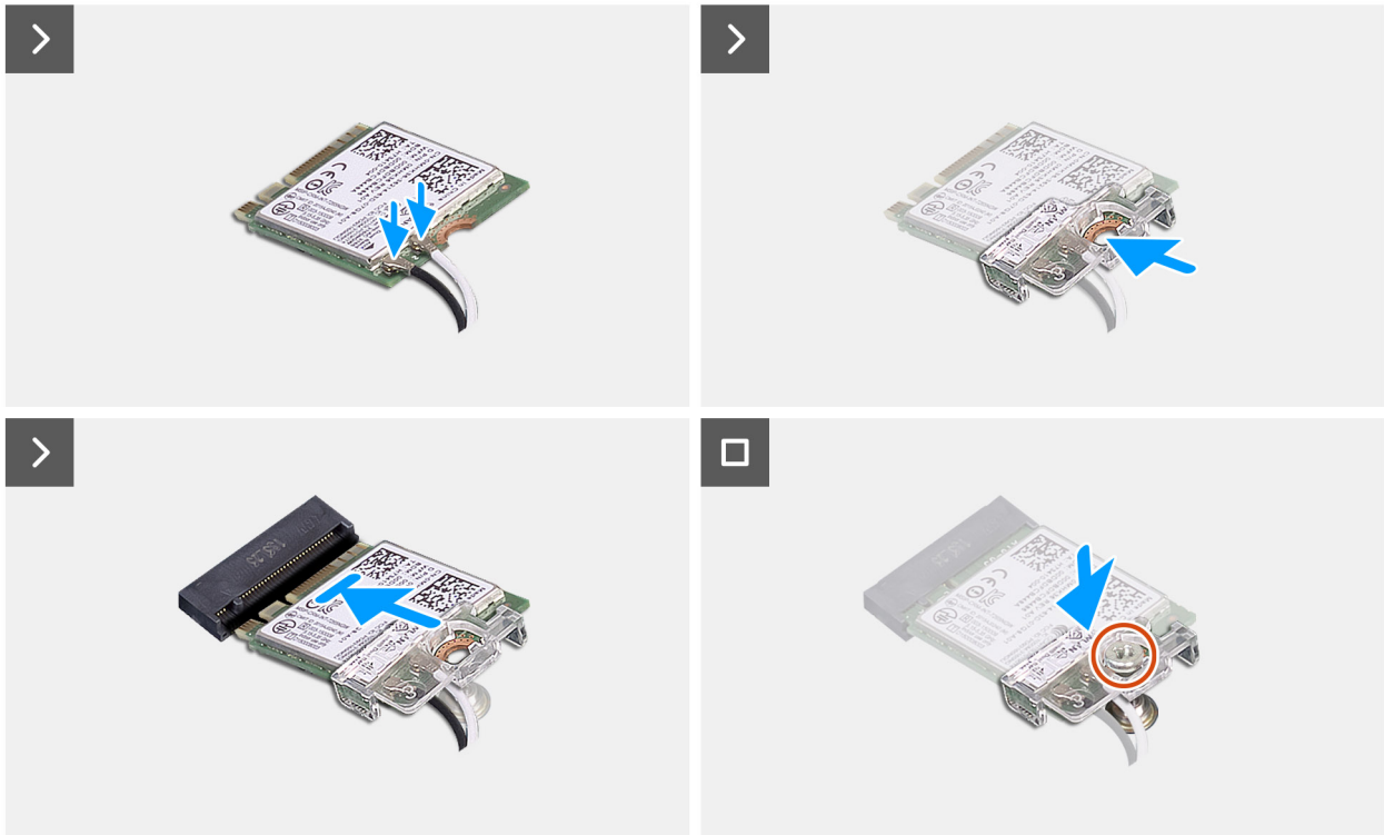
Ilustración 24. Instalación de la tarjeta inalámbrica
