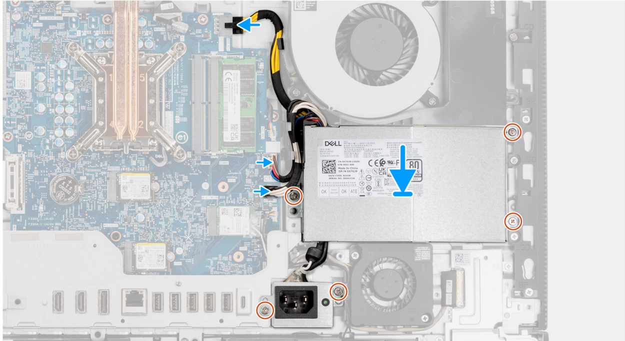
Ilustración 42. Instalación de la fuente de alimentación
