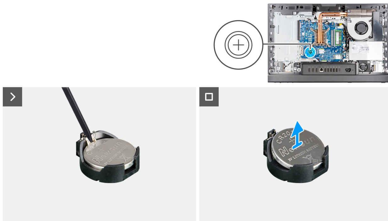
Ilustración 31. Extracción de la batería de tipo botón
