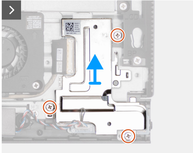
Ilustración 61. Extracción de la placa de audio
