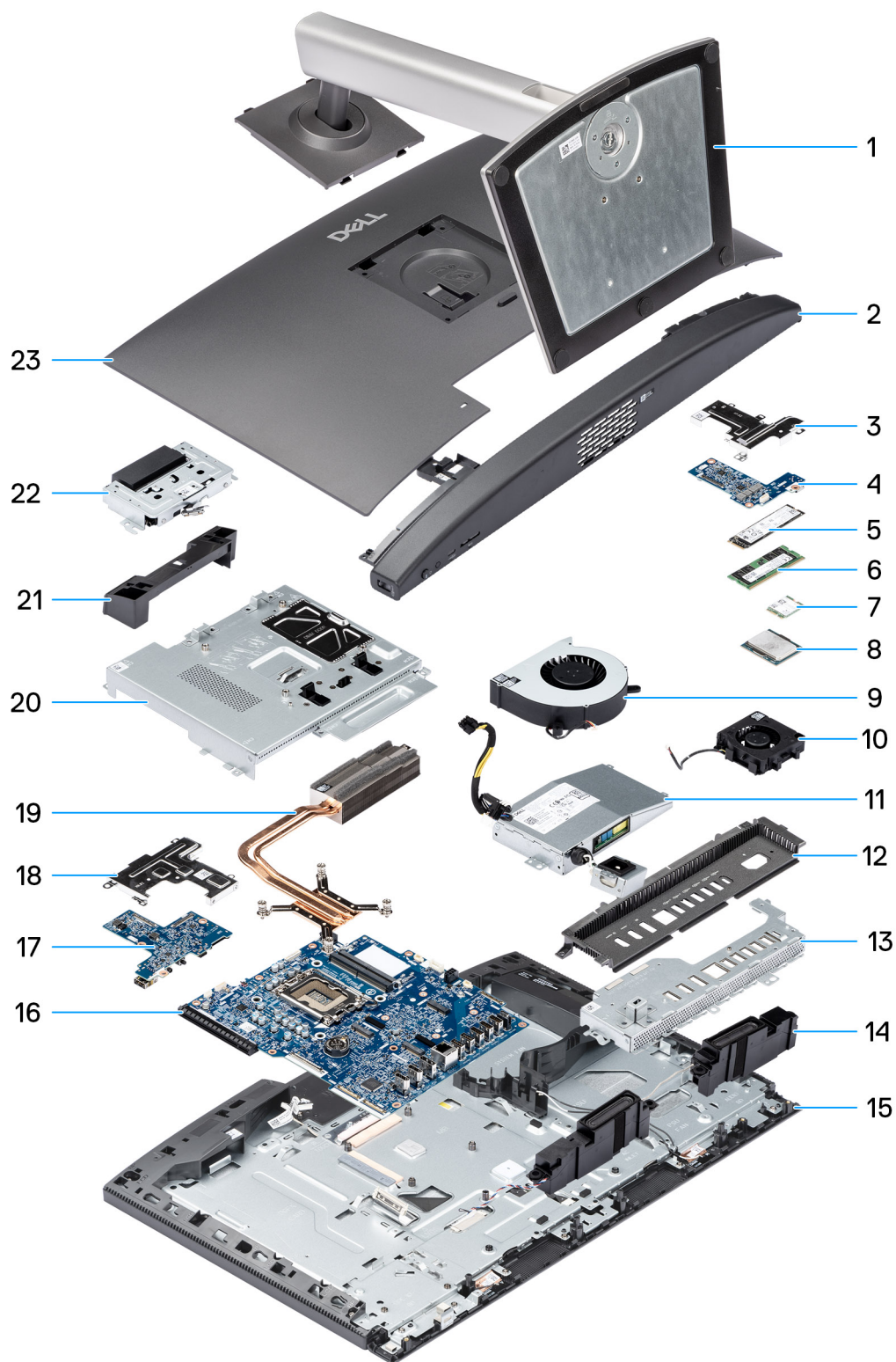
Ilustración 12. Componentes principales de la Dell Pro 24 todo en uno QC24250
