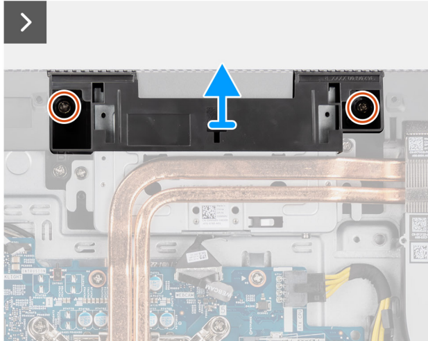
Ilustración 37. Extracción del ensamblaje de la cámara retráctil
