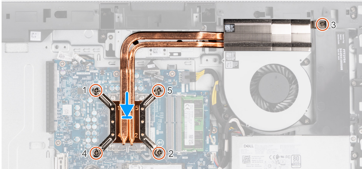
Ilustración 50. Instalación del disipador de calor
