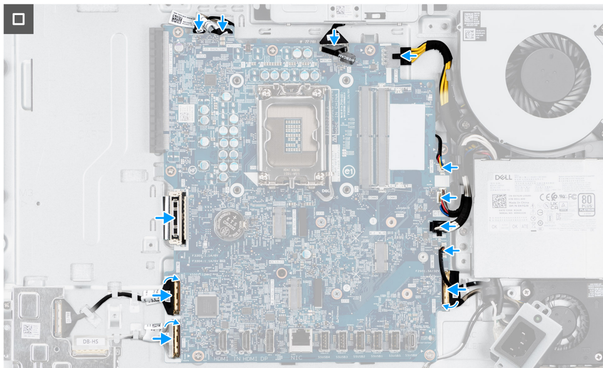
Ilustración 58. Instalación de la tarjeta madre
