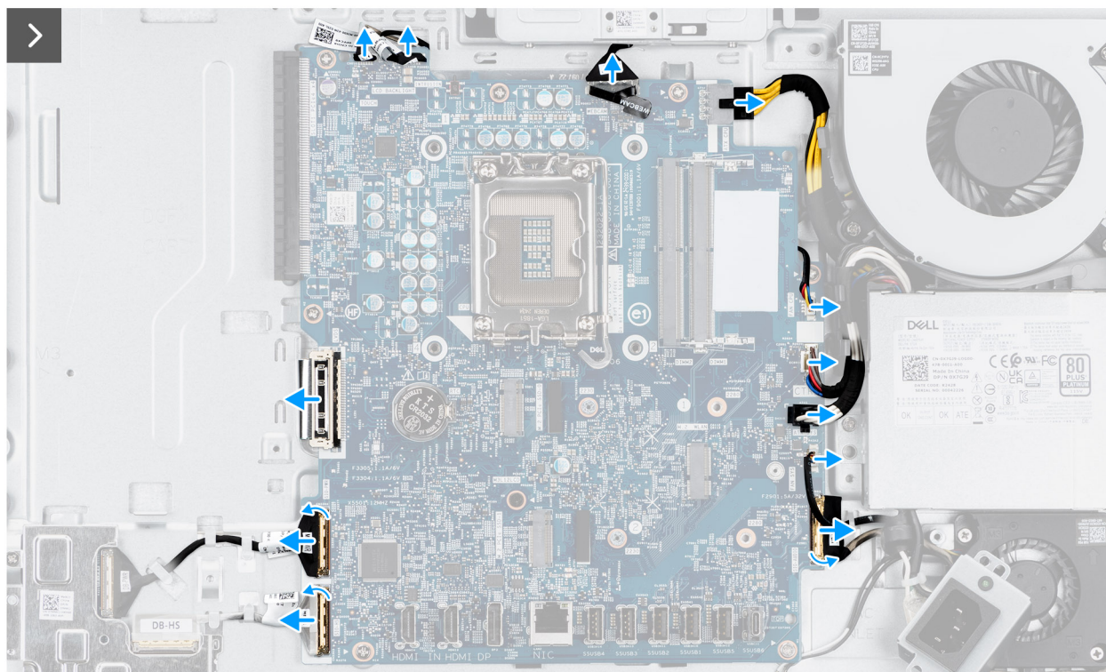
Ilustración 54. Extracción de la tarjeta madre
