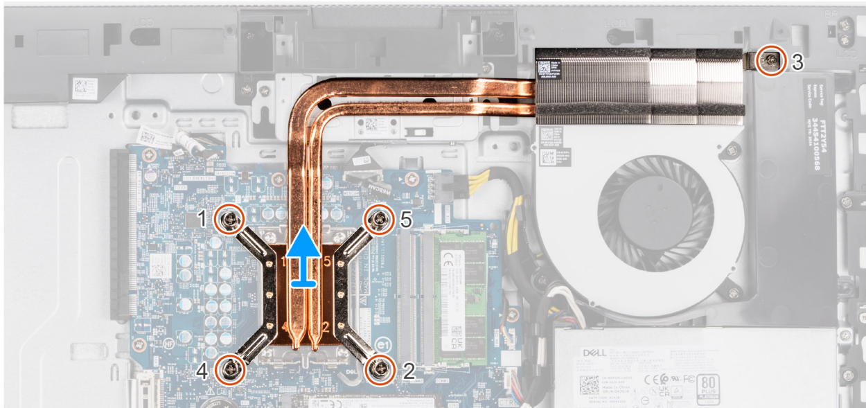
Ilustración 49. Extracción del disipador de calor
