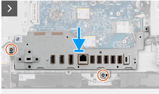
Ilustración 46. Instalación del soporte de I/O
