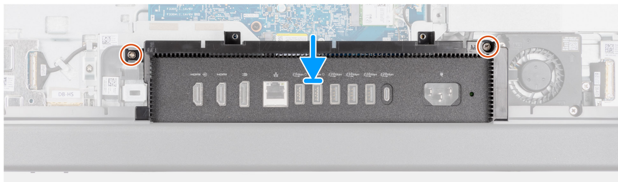
Ilustración 34. Instalación de la cubierta de I/O
