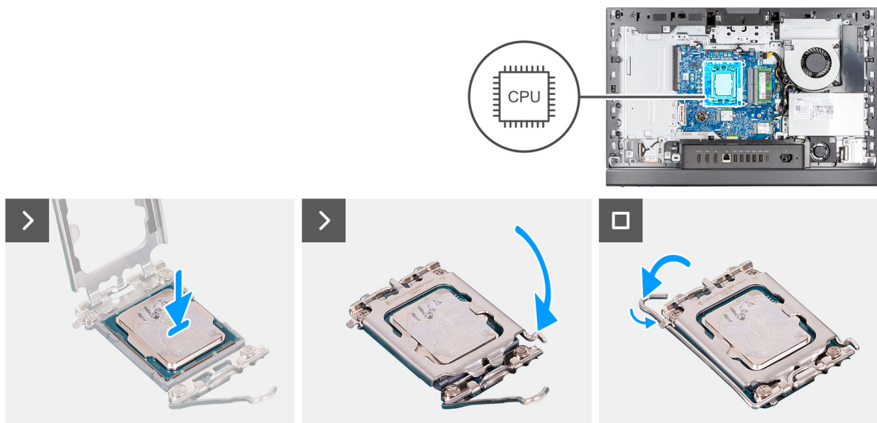
Ilustración 52. Instalación del procesador
