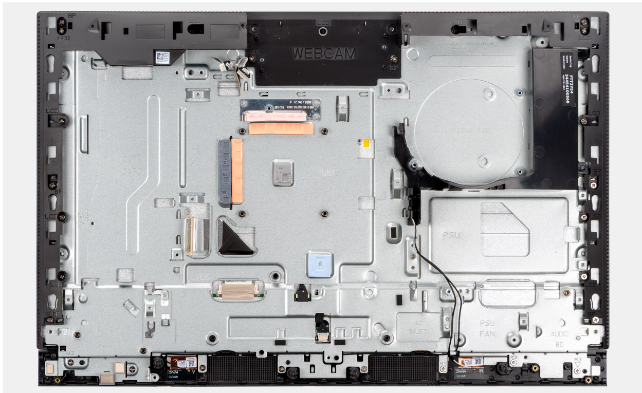
Ilustración 64. Extracción de la base del ensamblaje de la pantalla
