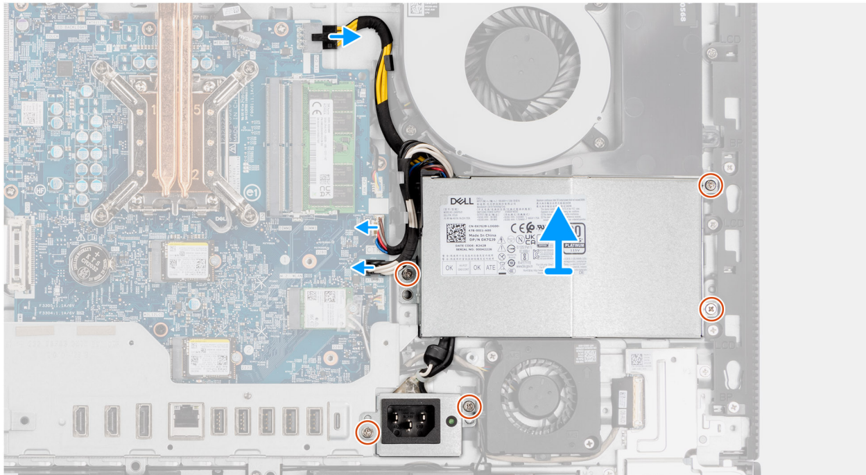
Ilustración 41. Extracción de la fuente de alimentación
