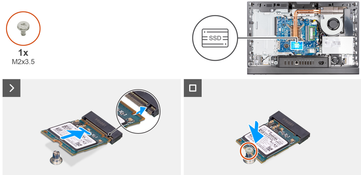
Ilustración 26. Instalación de la unidad de estado sólido M.2 2230 en la ranura M.2 0
