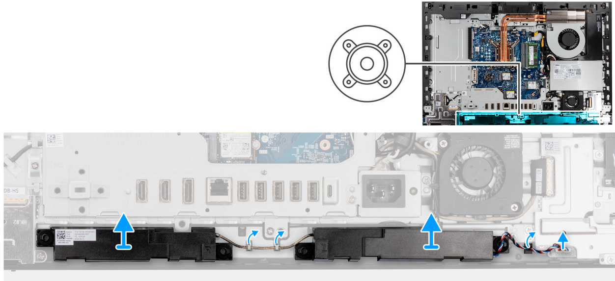
Ilustración 47. Extracción de los parlantes
