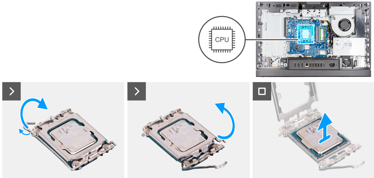
Ilustración 51. Extracción del procesador
