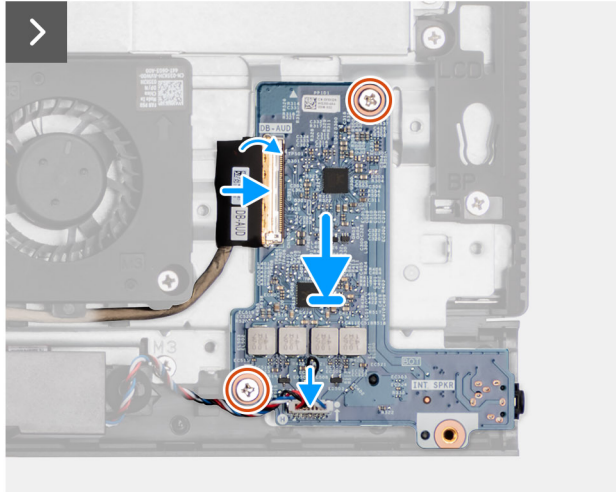
Ilustración 62. Instalación de la placa de audio
