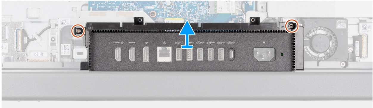
Ilustración 33. Extracción de la cubierta de I/O
