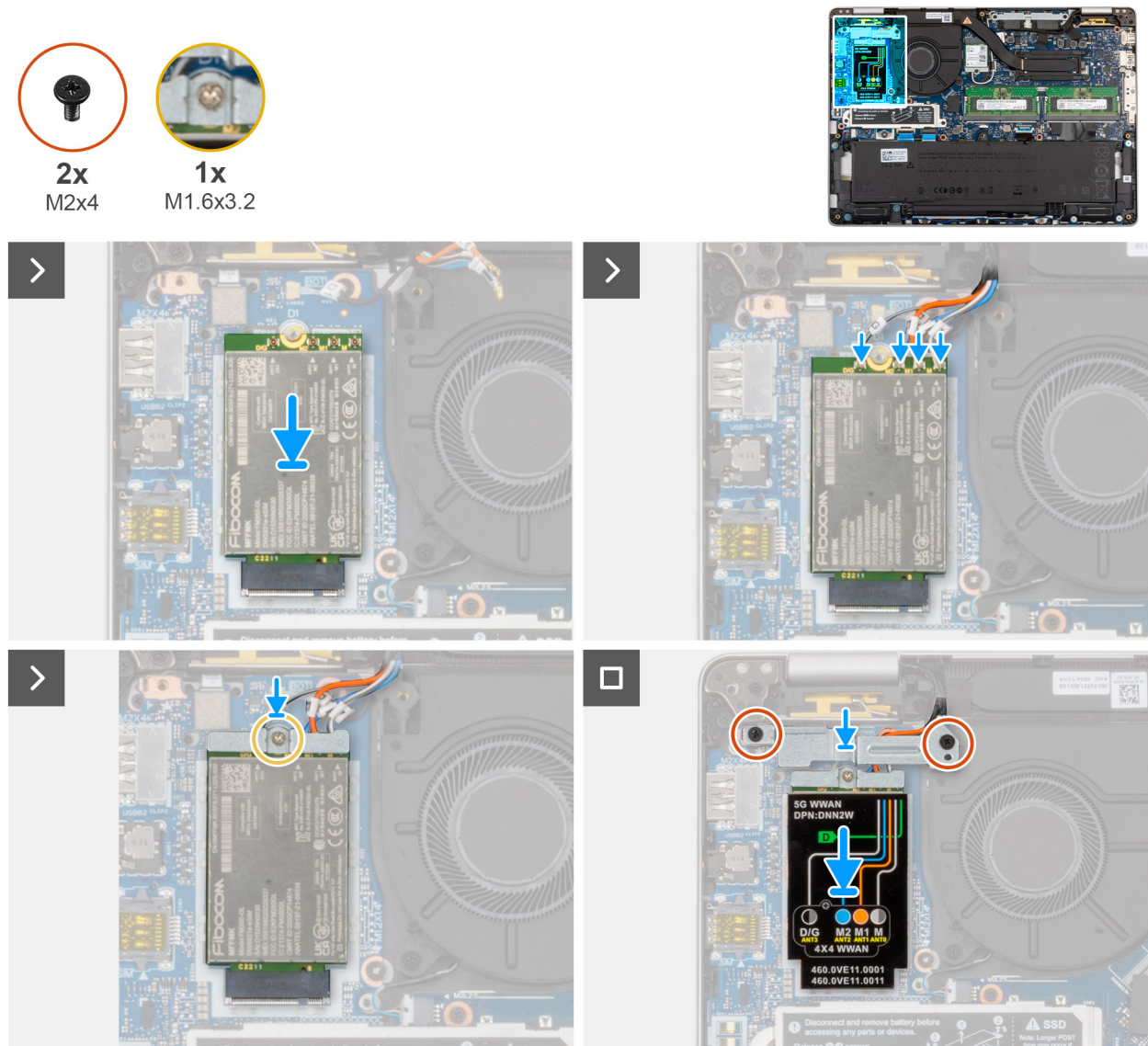
Figure 31. Installation de la carte WWAN 5G
