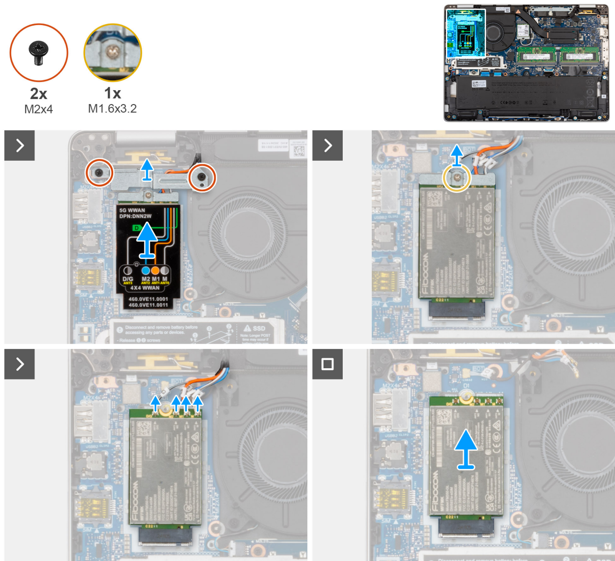
Figure 29. Retrait de la carte WWAN 5G
