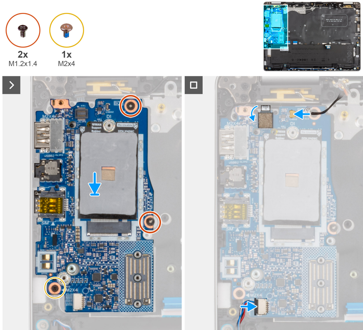
Figure 65. Installation de la carte d'E/S
