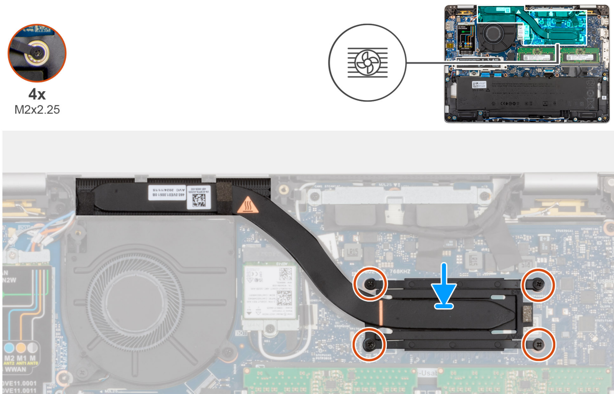
Figure 51. Installation du dissipateur de chaleur
