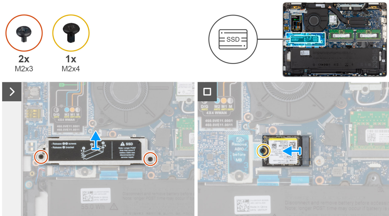
Figure 37. Retrait du disque SSD M.2 2230
