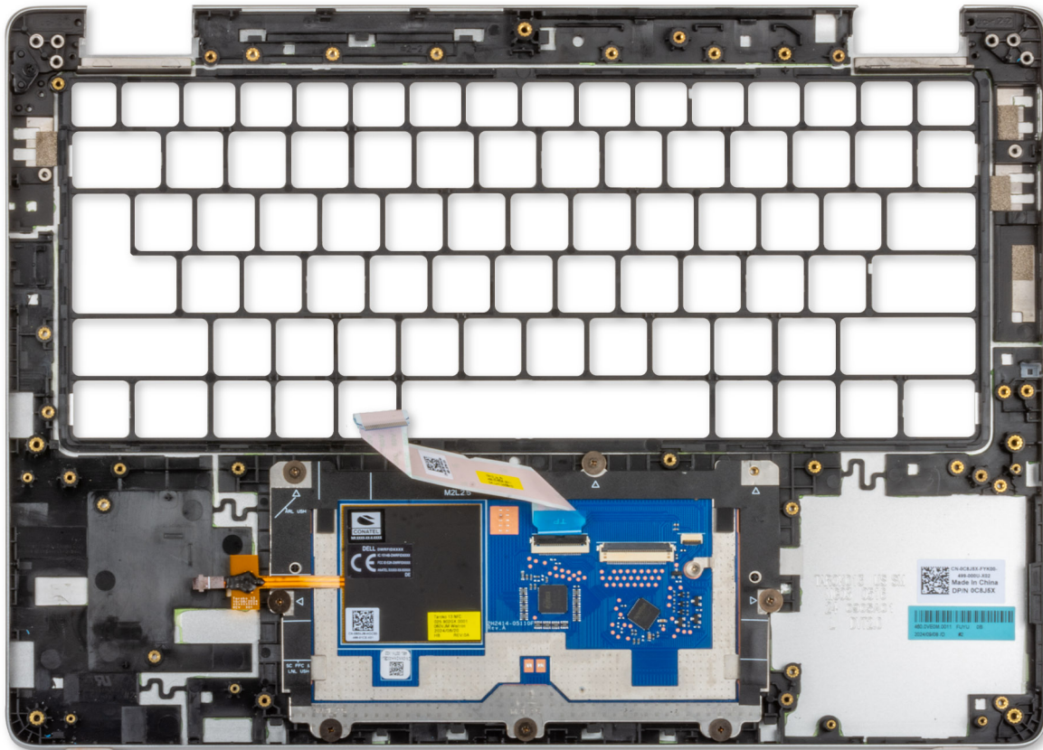
Figure 73. Installation de l'assemblage du repose-poignets
