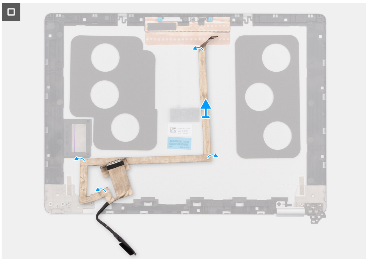
Figure 83. Retrait du câble de l'écran
