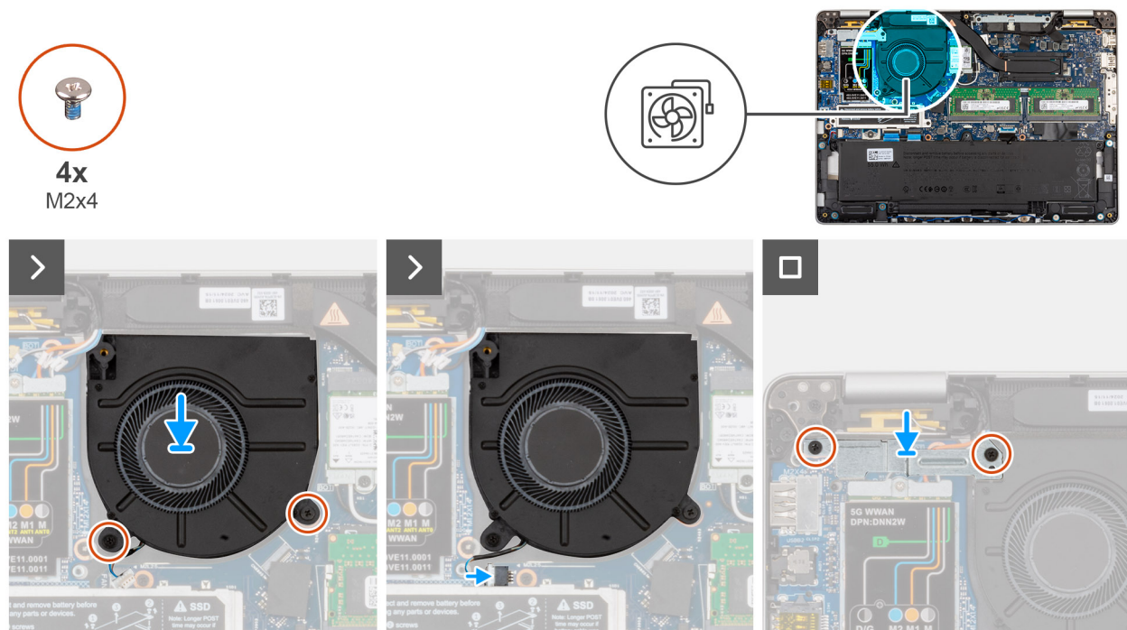
Figure 44. Installation du ventilateur
