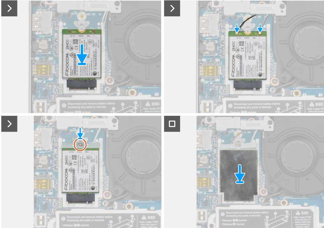
Figure 34. Installation de la carte WWAN 4G
