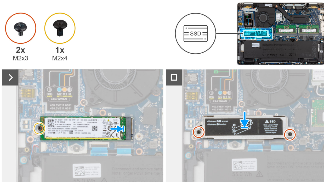
Figure 40. Installation du disque SSD M.2 2280
