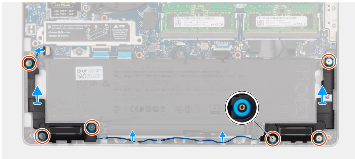
Figure 41. Retrait des haut-parleurs
