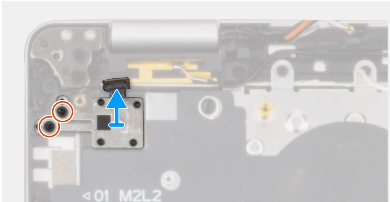
Figure 66. Retrait du bouton d'alimentation avec lecteur d'empreintes digitales (en option)
