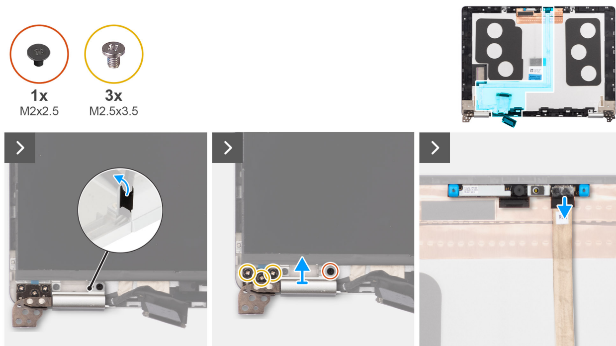
Figure 82. Retrait du câble de l'écran
