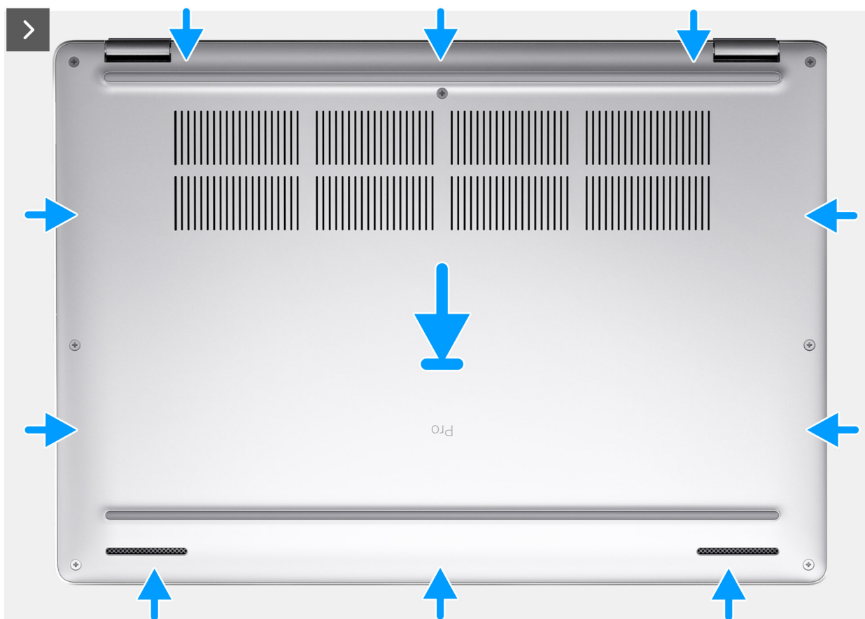
Figure 21. Installation du cache de fond
