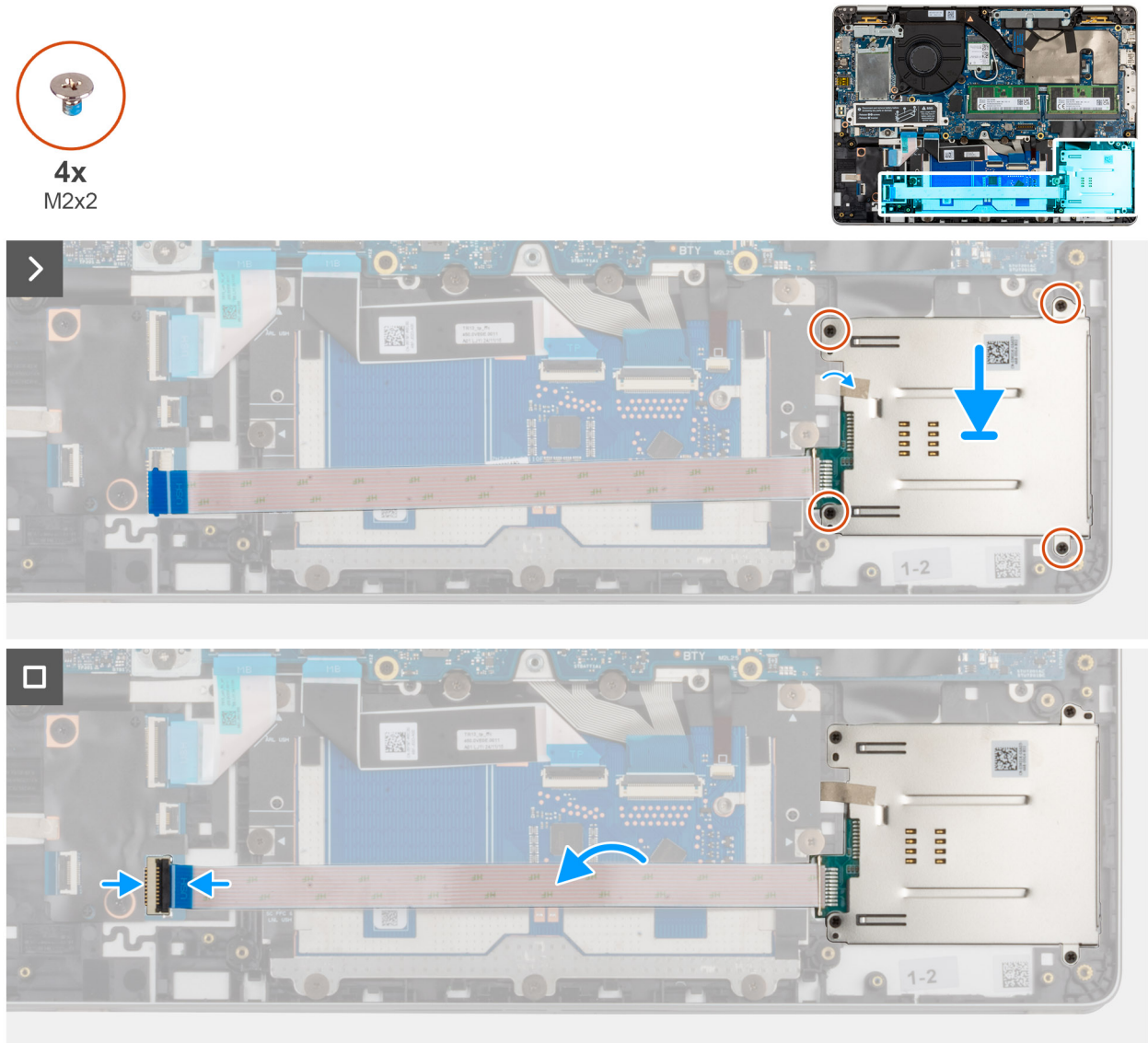
Figure 49. Installation du lecteur de carte à puce
