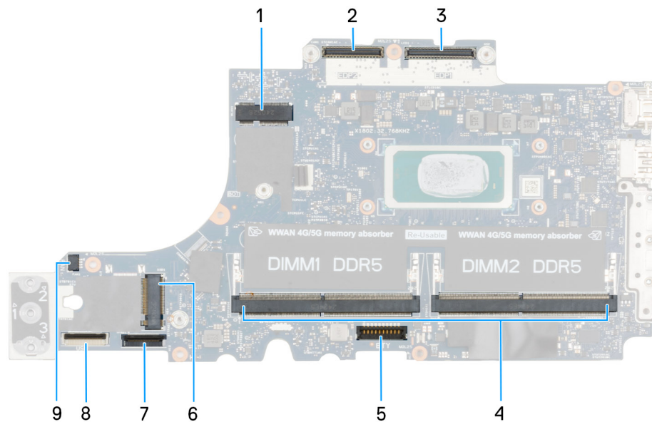
Figure 56. Connecteurs de la carte système
