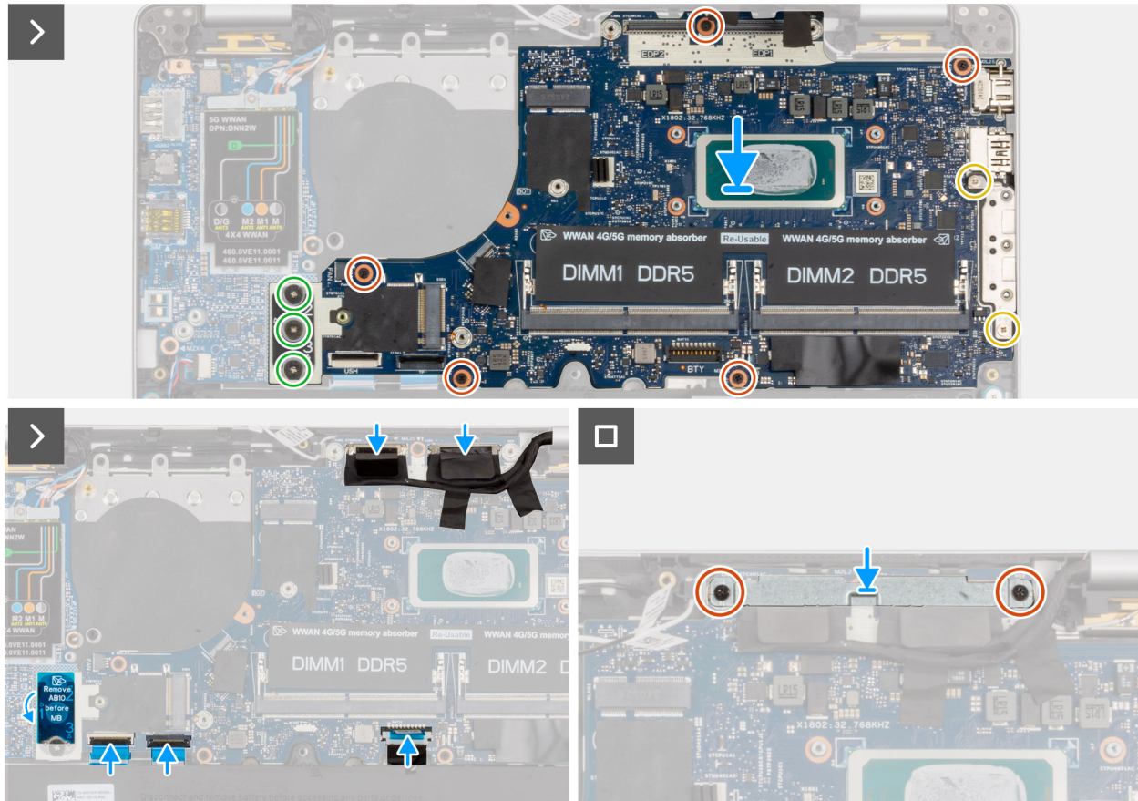
Figure 59. Installation de la carte système
