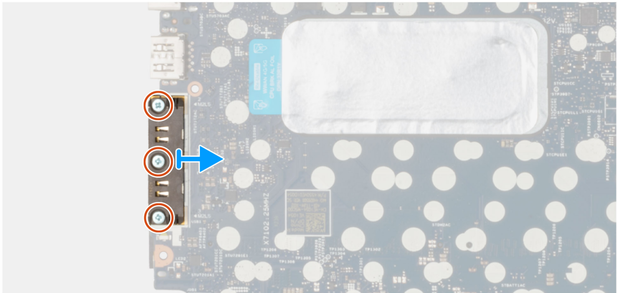
Figure 60. Retrait du module de connecteur USB-C
