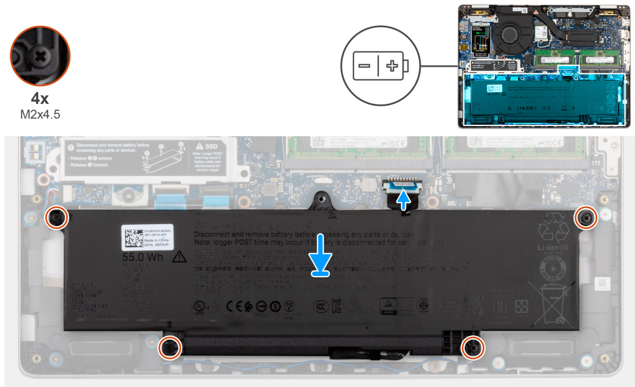
Figure 24. Installation de la batterie
