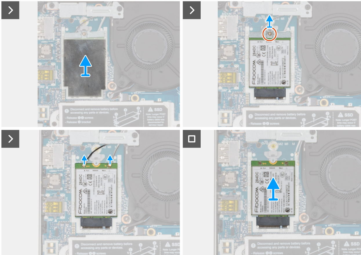
Figure 33. Retrait de la carte WWAN 4G
