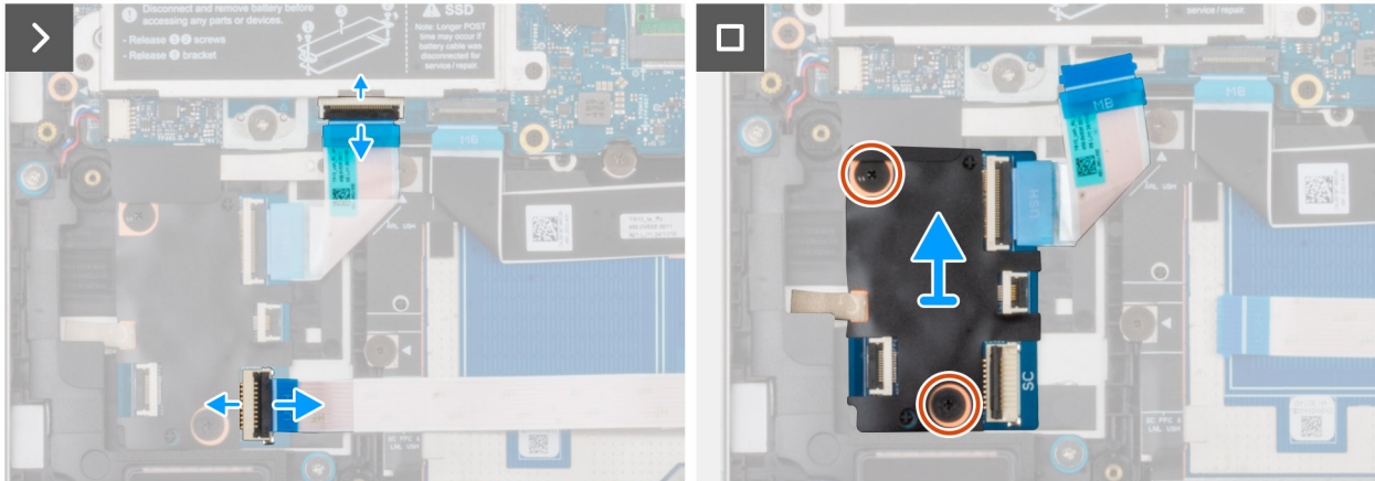
Figure 45. Retrait de la carte USH
