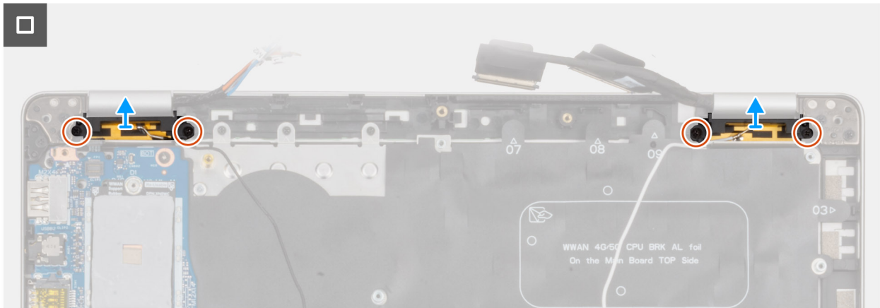
Figure 62. Retrait du module d'antenne sans fil
