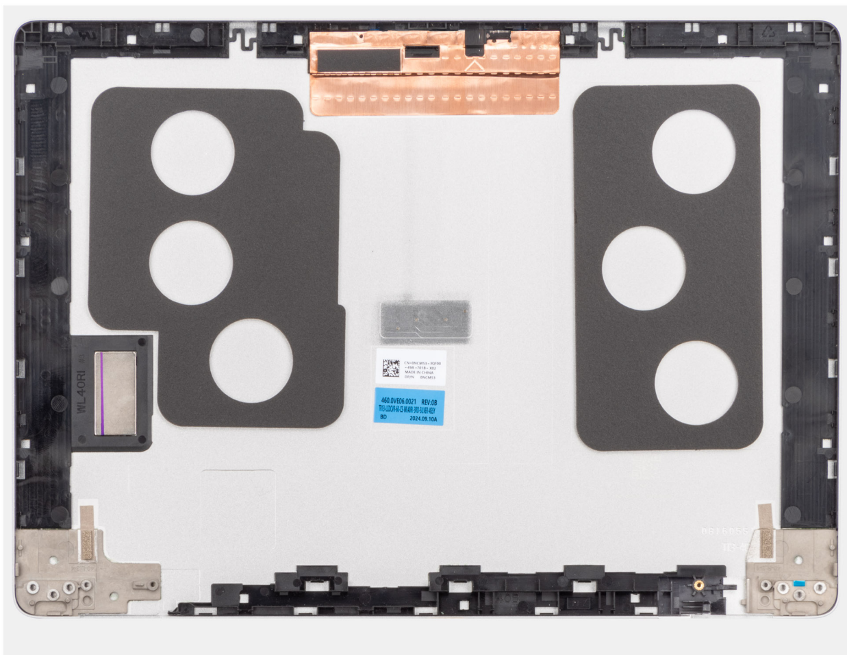
Figure 86. Retrait du capot arrière d'écran
