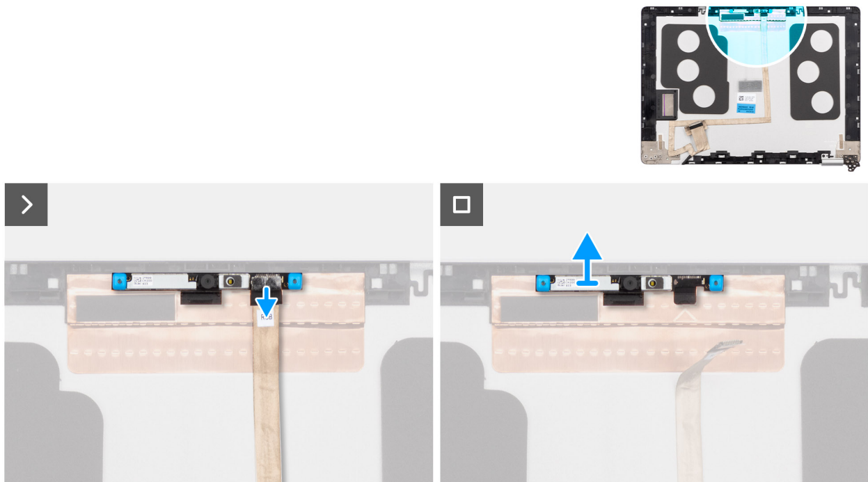
Figure 80. Retrait du module de caméra
