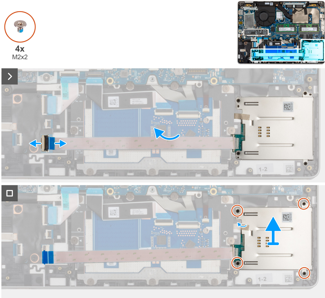
Figure 48. Retrait du lecteur de carte à puce
