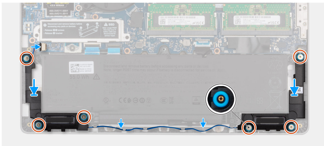
Figure 42. Installation des haut-parleurs
