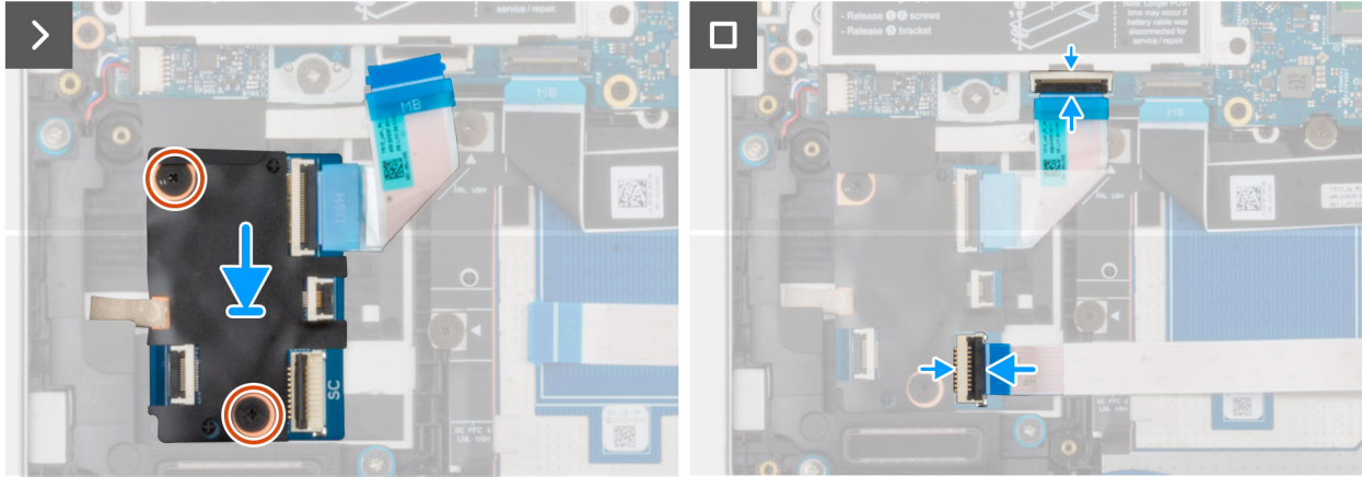
Figure 47. Installation de la carte USH
