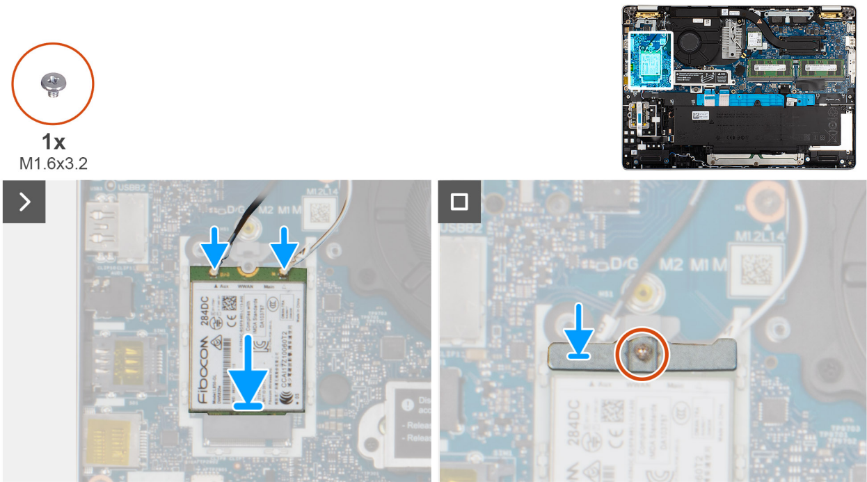
Abbildung 34. Installieren der 4G-WWAN-Karte
