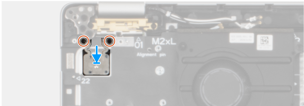
Abbildung 60. Installieren des Netzschalters mit optionalem Fingerabdruck-Lesegerät
