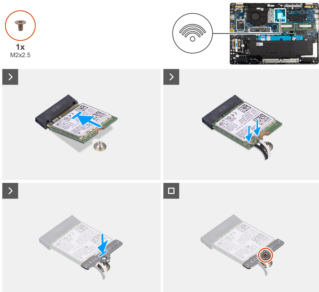
Abbildung 36. Einbauen der WLAN-Karte
