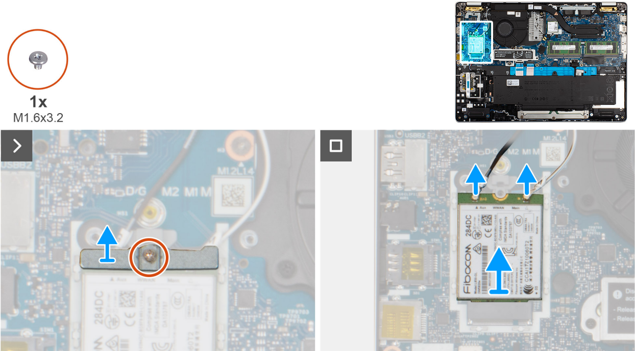
Abbildung 33. Entfernen der 4G-WWAN-Karte
