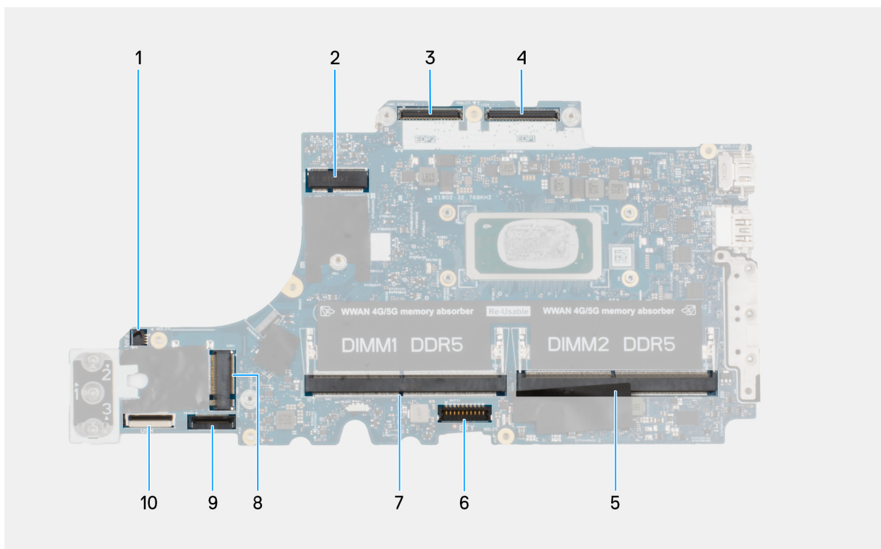
Abbildung 54. Hauptplattenanschluss
