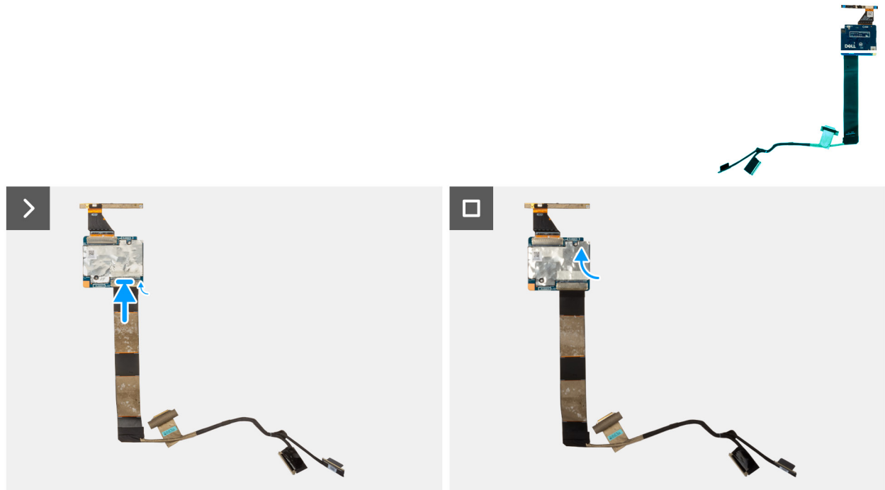
Abbildung 77. Einbauen des Bildschirmkabels
