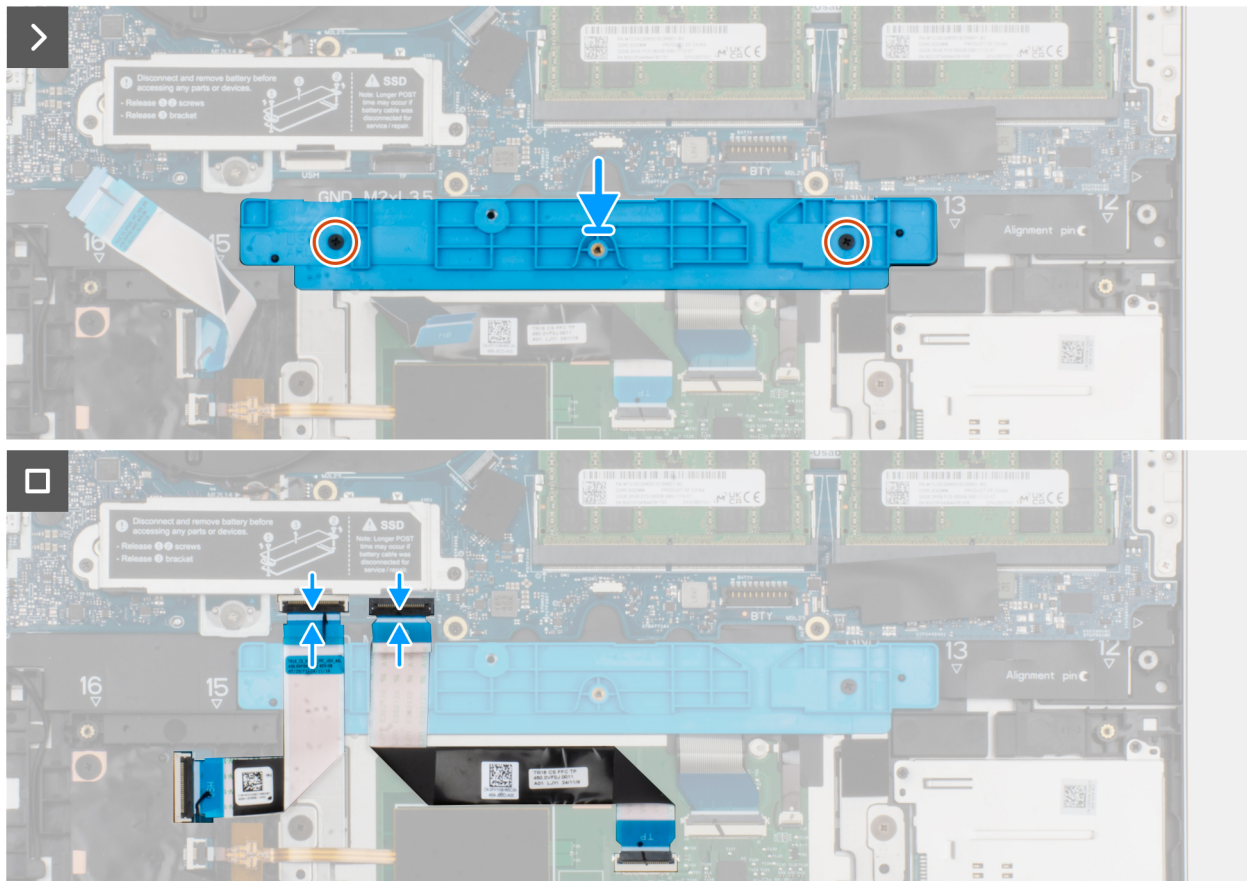
Abbildung 48. Installieren der Akkuhalterung
