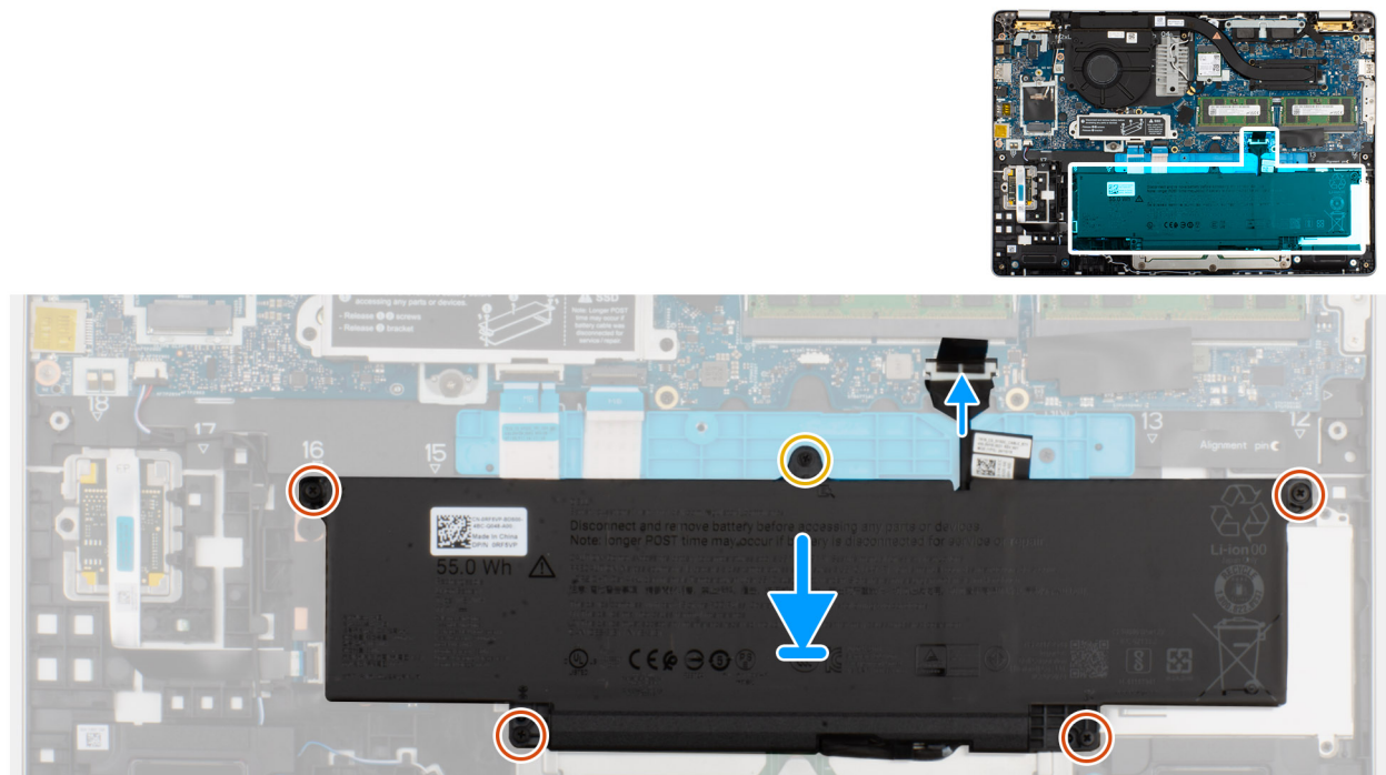
Abbildung 16. Verbinden des Akkukabels
