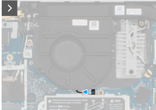
Abbildung 37. Entfernen des Lüfters
