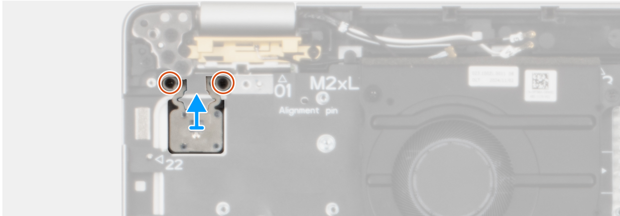
Abbildung 59. Installieren des Netzschalters mit optionalem Fingerabdruck-Lesegerät
