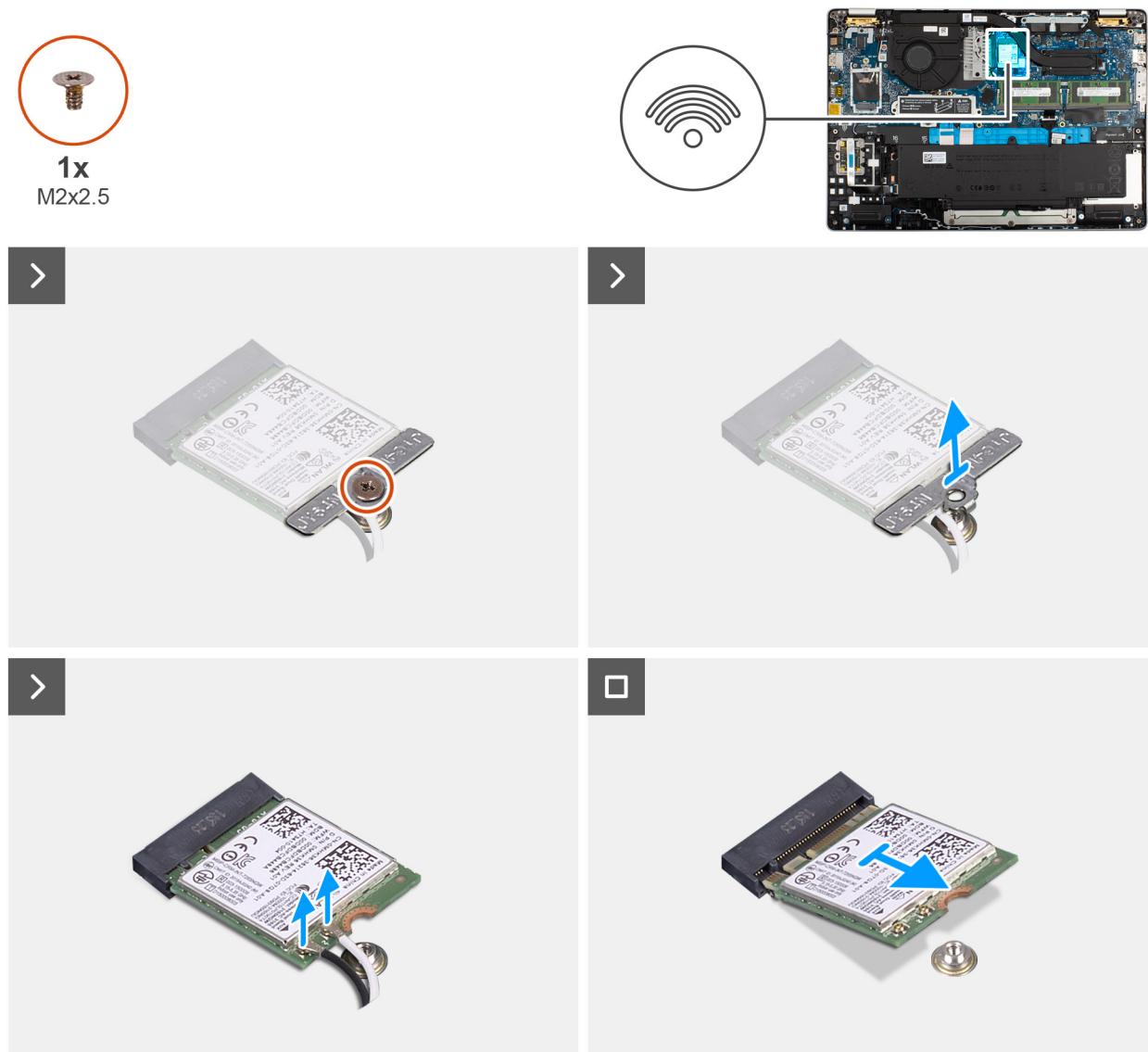
Abbildung 35. Entfernen der WLAN-Karte
