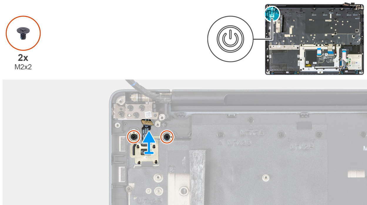
Abbeelding 130. De aan-uitknop verwijderen
