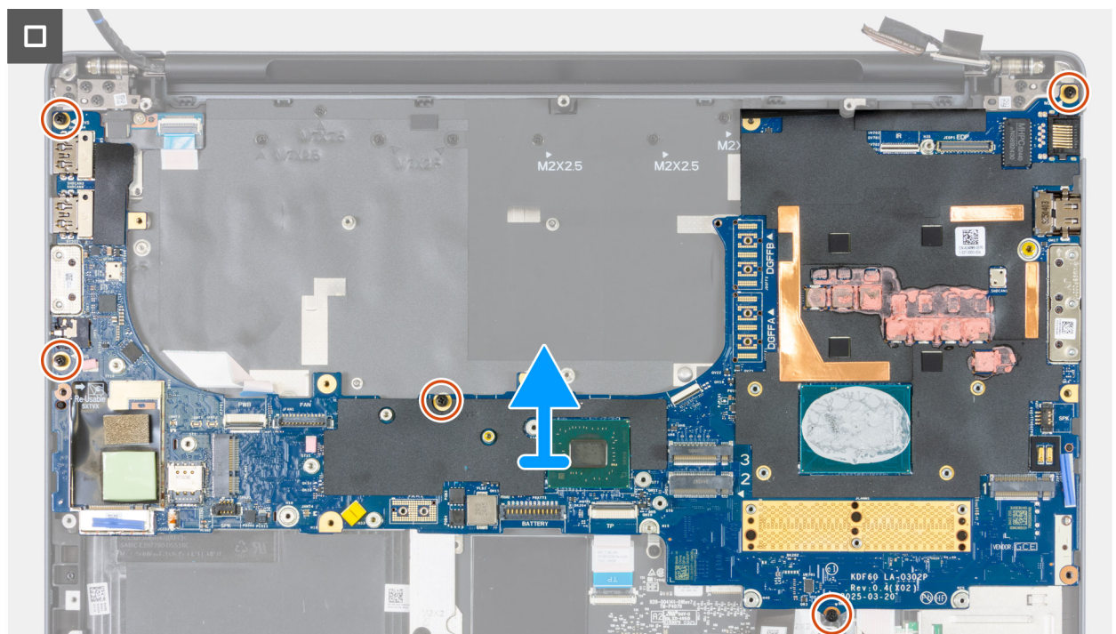
Afbeelding 113. De systeemkaart verwijderen
