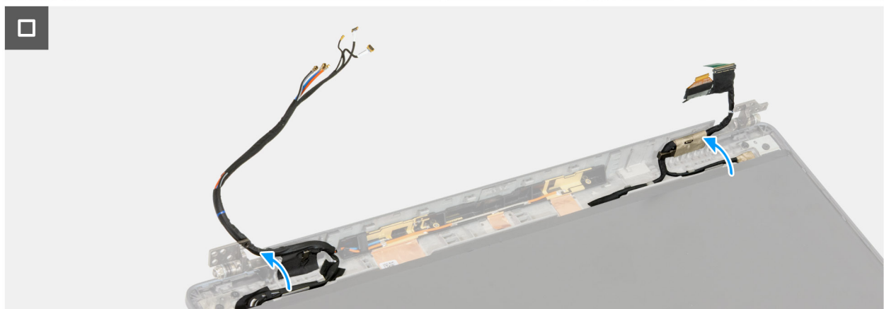
Afbeelding 103. De beeldschermsscharnieren installeren
