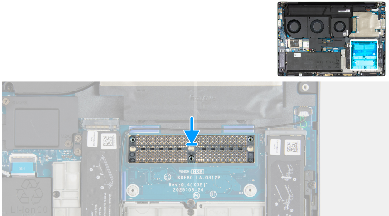
Afbeelding 73. De geheugenconnector plaatsen
