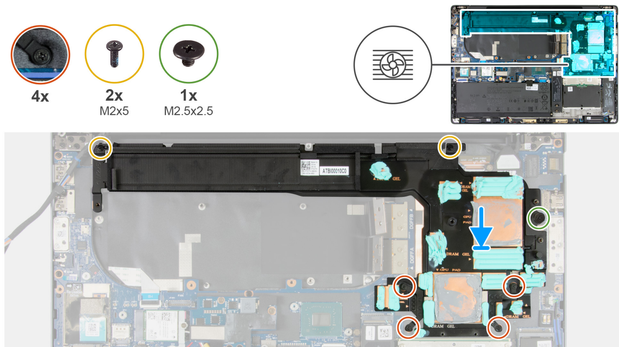
Afbeelding 77. De koelplaat installeren voor computers die met een geïntegreerde grafische kaart worden geleverd
