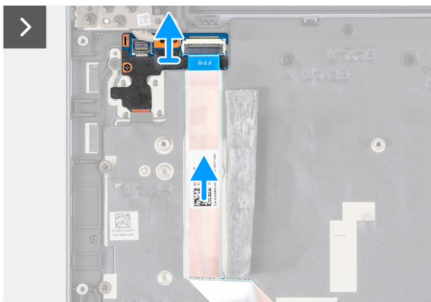
Afbeelding 128. De aan/uit-knopkaart verwijderen
