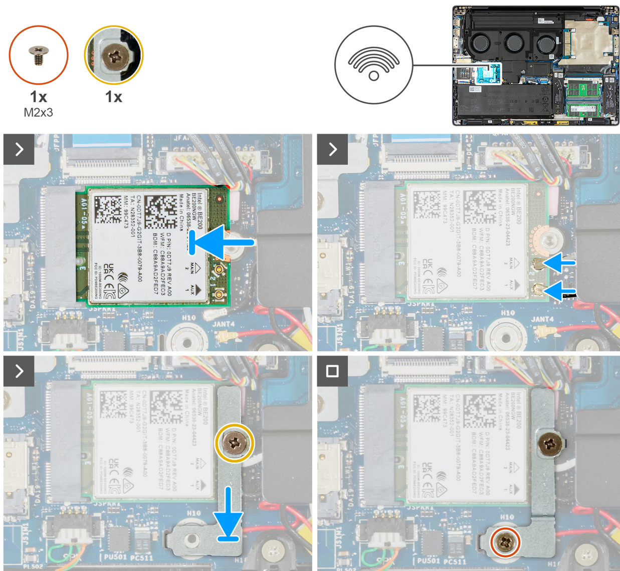
Afbeelding 45. De WLAN-kaart plaatsen
