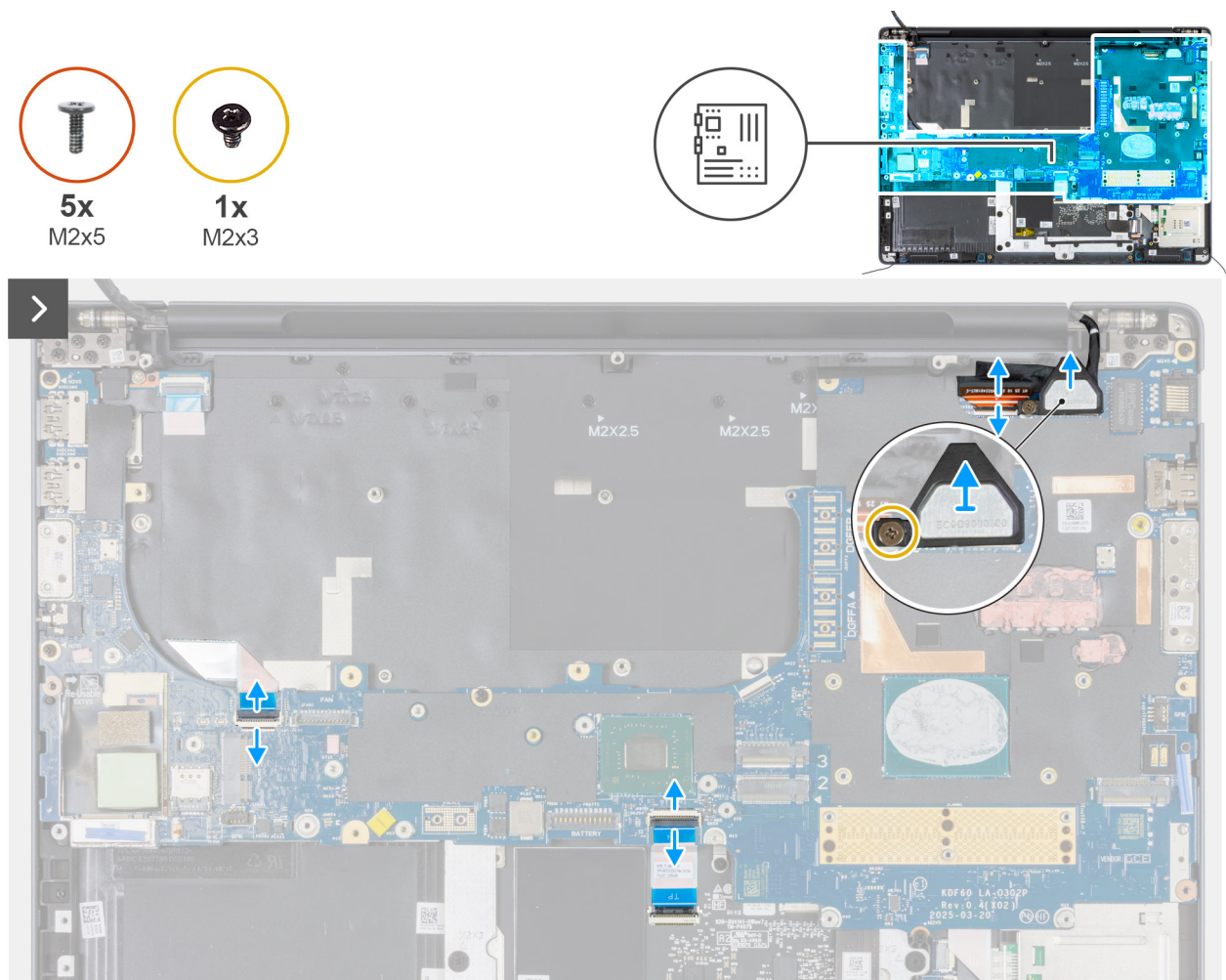
Afbeelding 112. De systeemkaart verwijderen
