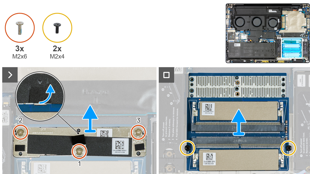
Afbeelding 70. De geheugeninterposerkaart verwijderen
