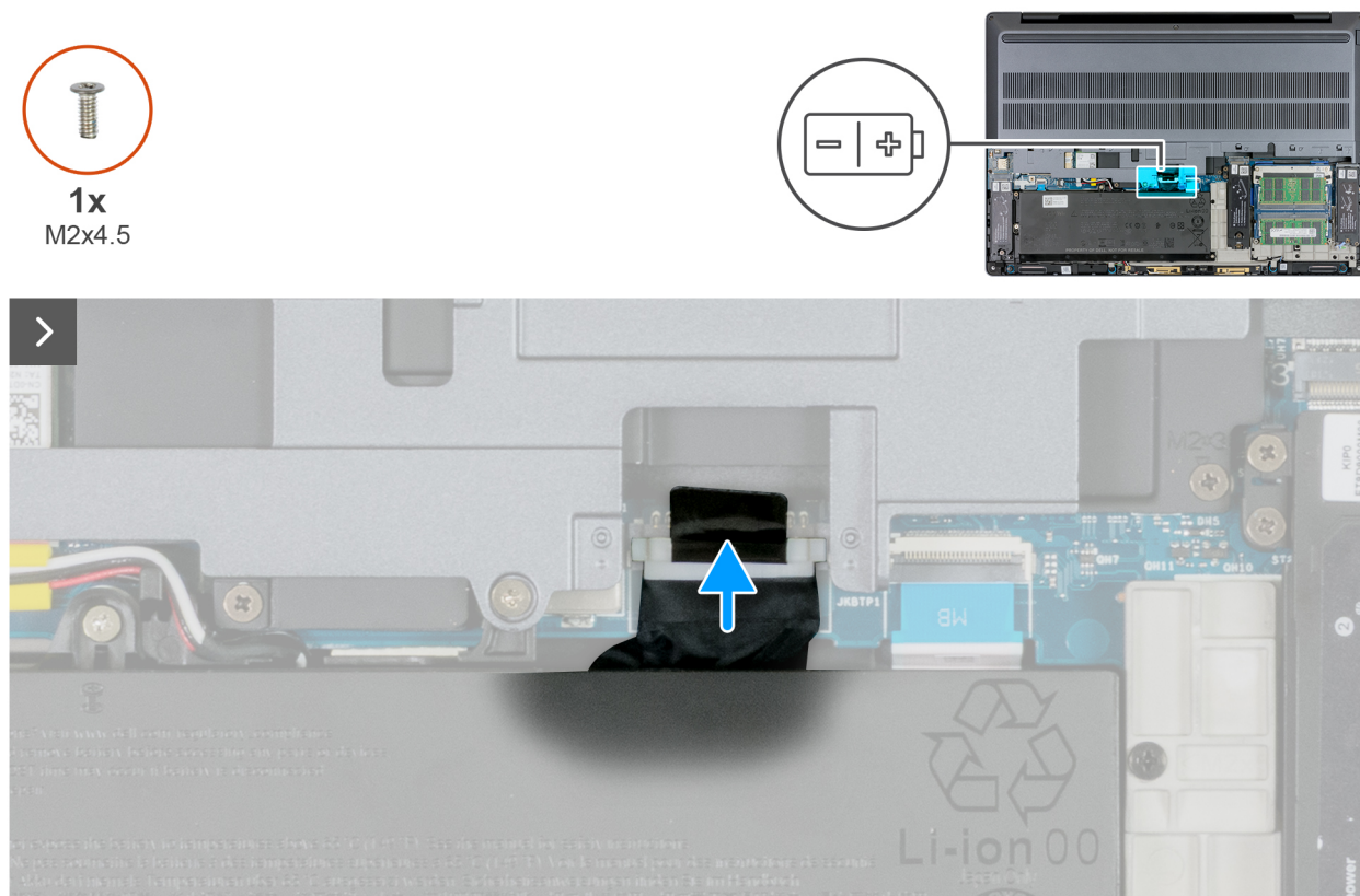
Afbeelding 15. De batterijkabel aansluiten
