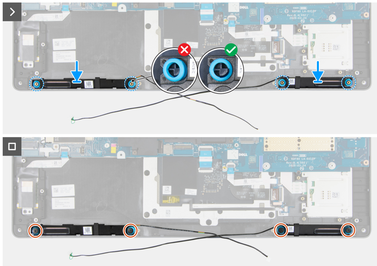
Afbeelding 82. De luidsprekers plaatsen
