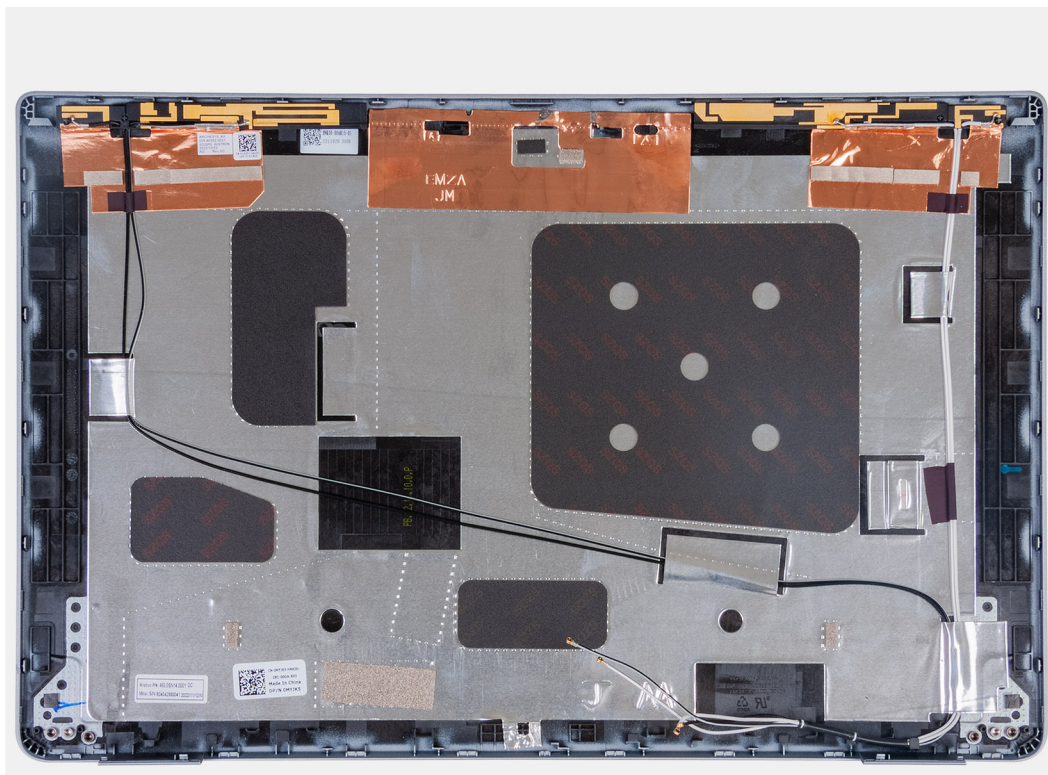
Afbeelding 105. Achterpaneel beeldscherm
