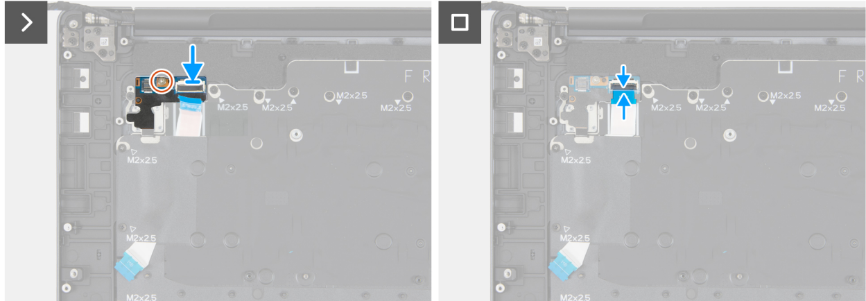
Afbeelding 126. De aan/uit-knopkaart plaatsen
