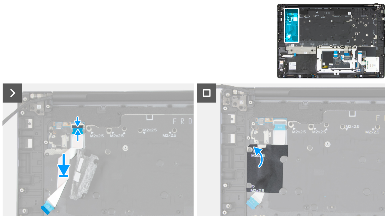
Afbeelding 124. De kabel van de aan/uit-knopkaart plaatsen
