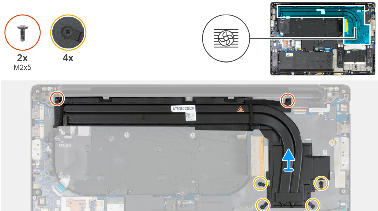
Abbeelding 73. De koelplaat verwijderen voor computers die worden geleverd met een geïntegreerde grafische kaart
