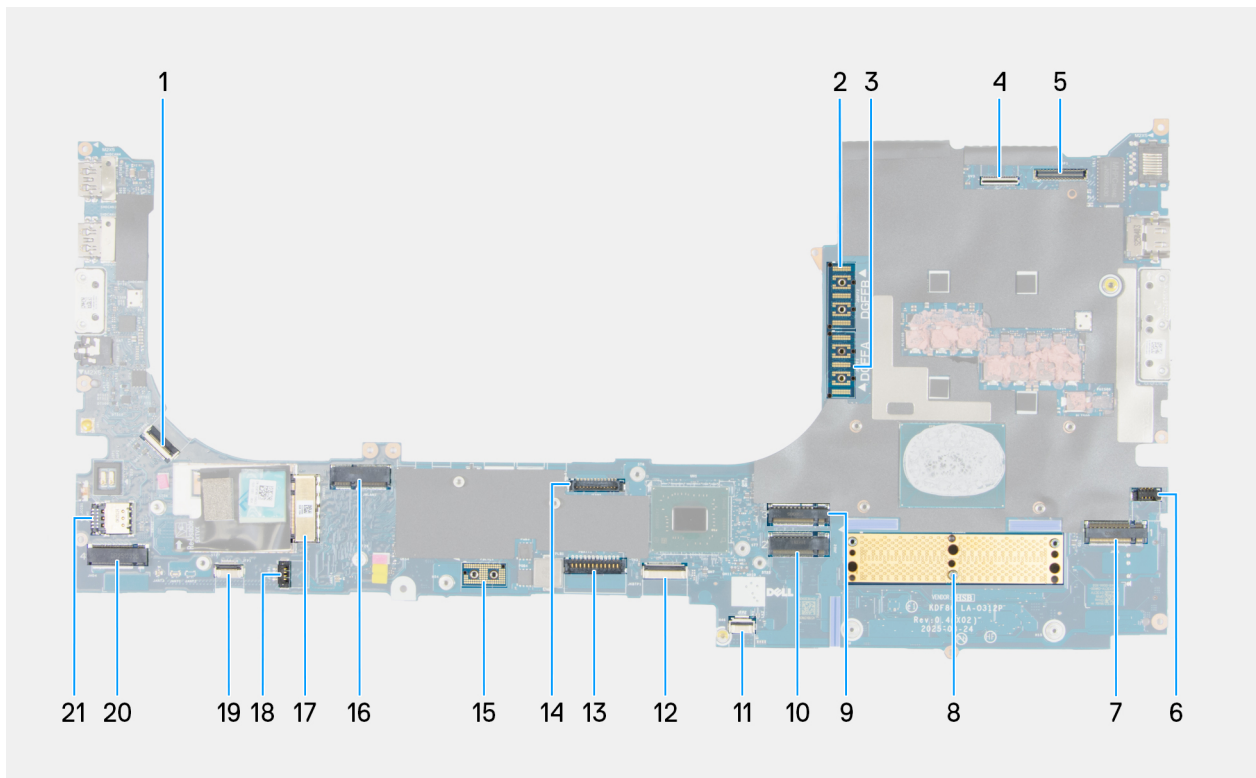
Afbeelding 110. Systeemkaartconnectoren
