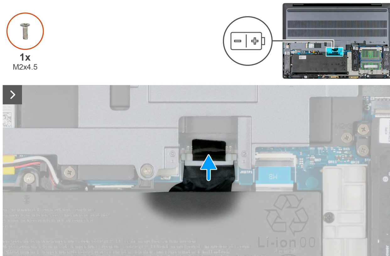
Figure 21. Connexion du câble de la batterie
