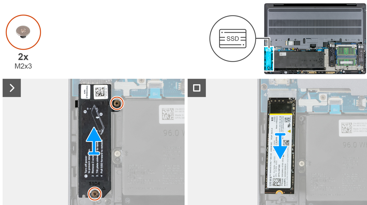
Figure 40. Retrait du disque SSD M.2 2280 du logement 4 (SSD4)
