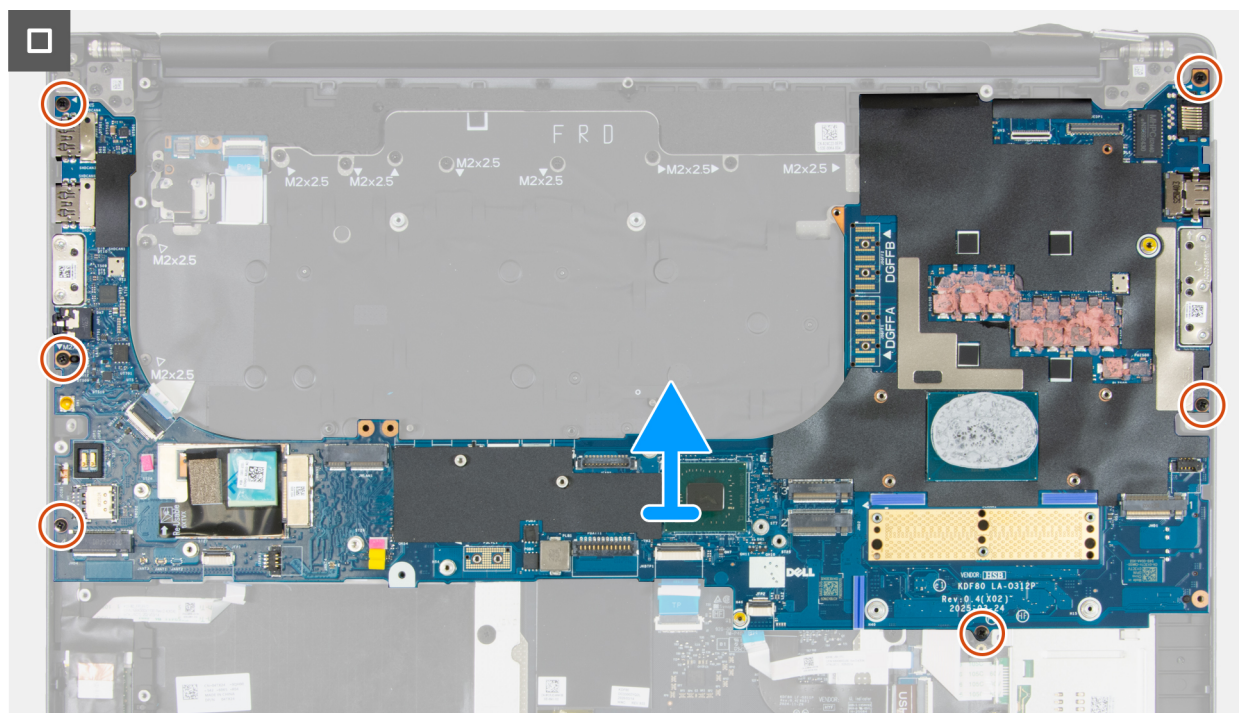
Figure 108. Retrait de la carte système
