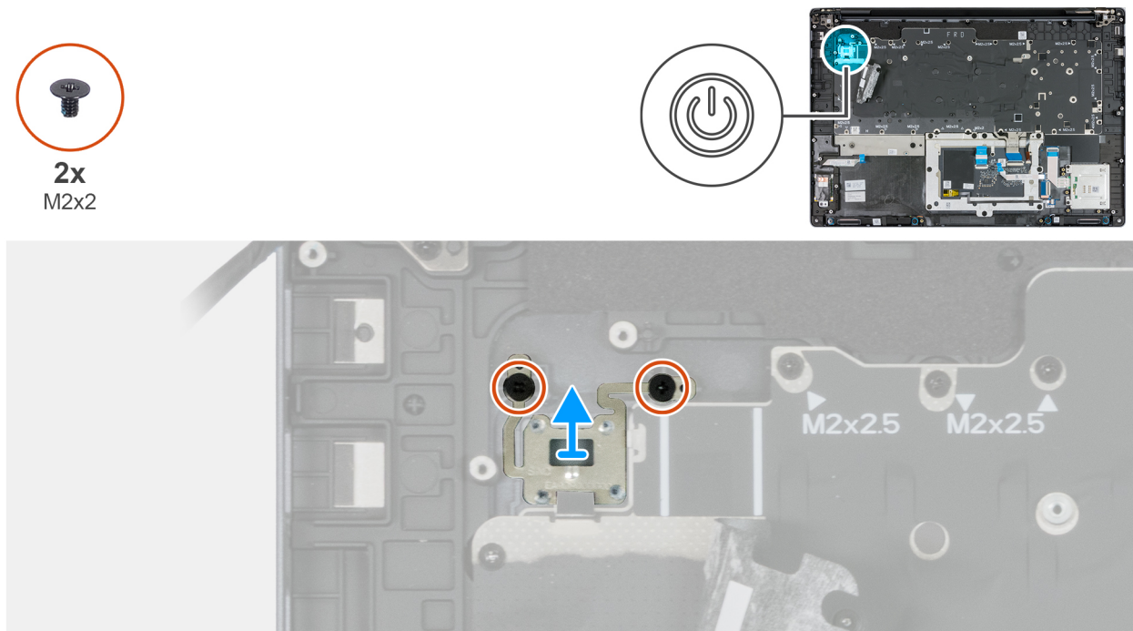
Figure 127. Retrait du bouton d'alimentation
