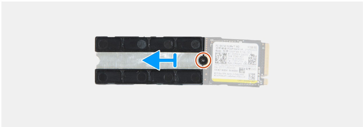
Figure 42. Retrait du disque SSD M.2 2230
