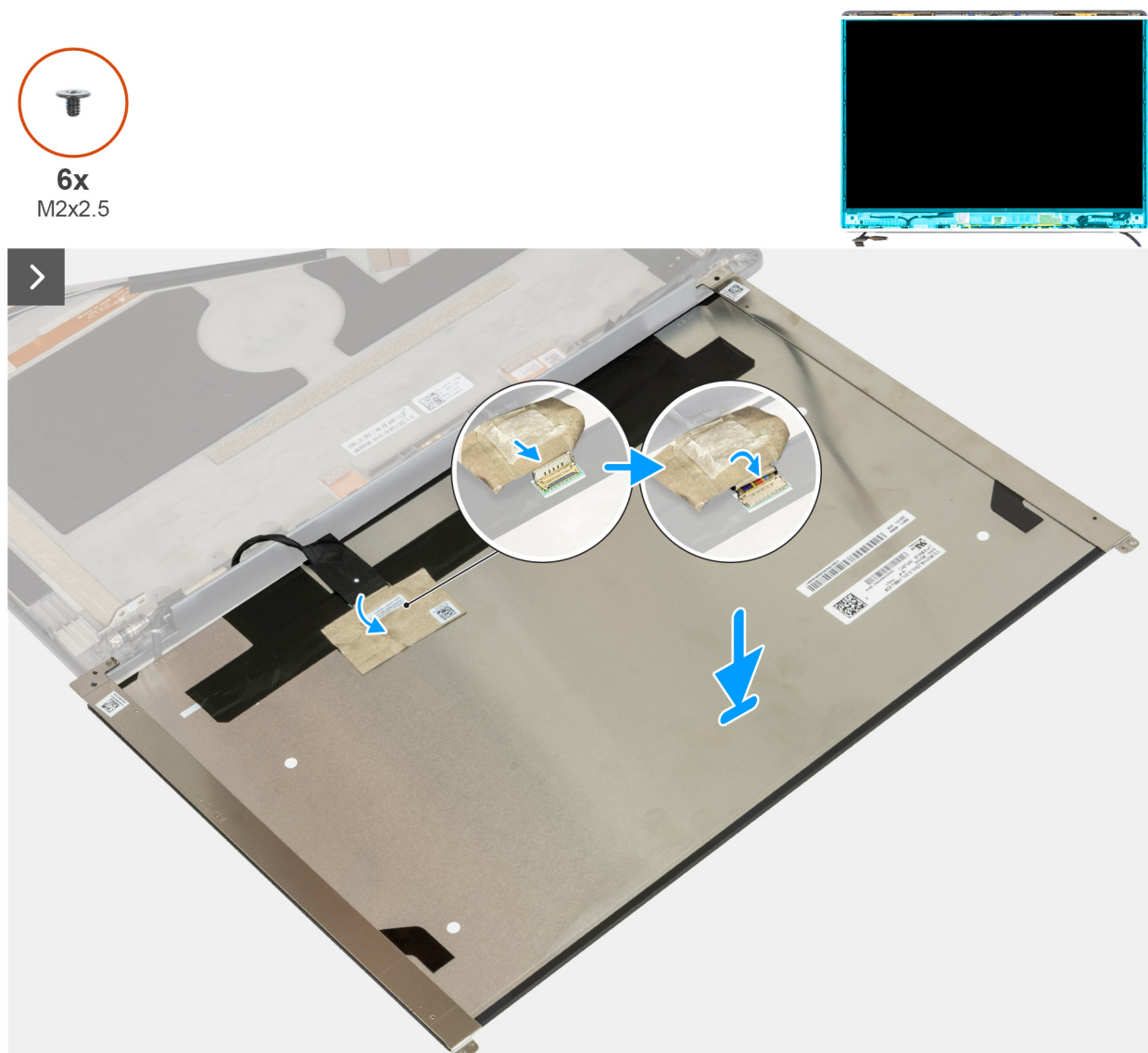
Figure 93. Installation du panneau d'écran pour les écrans tactiles
