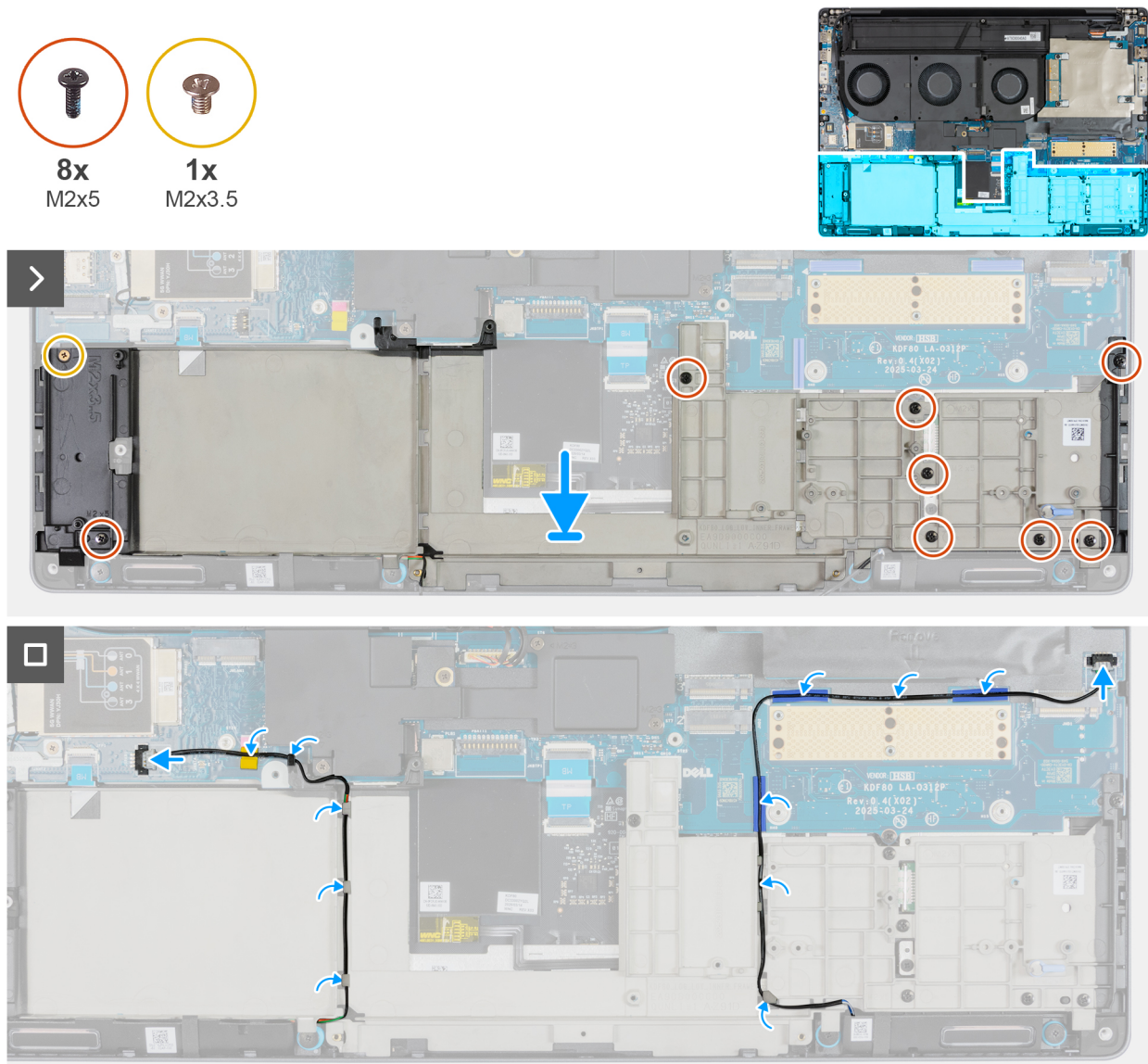
Figure 80. Installation du cadre interne
