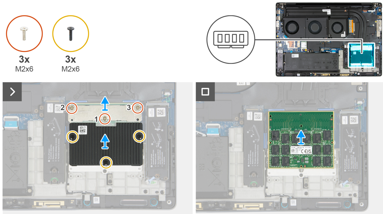
Figure 32. Retrait du module de la carte CAMM
