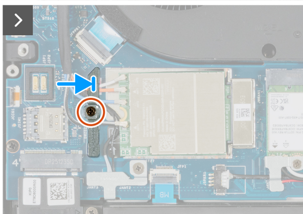
Figure 53. Installation de la carte WWAN
