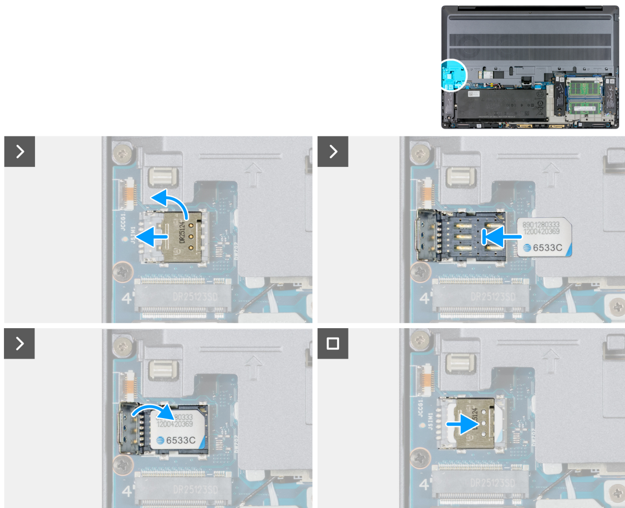
Figure 51. Installation de la carte SIM
