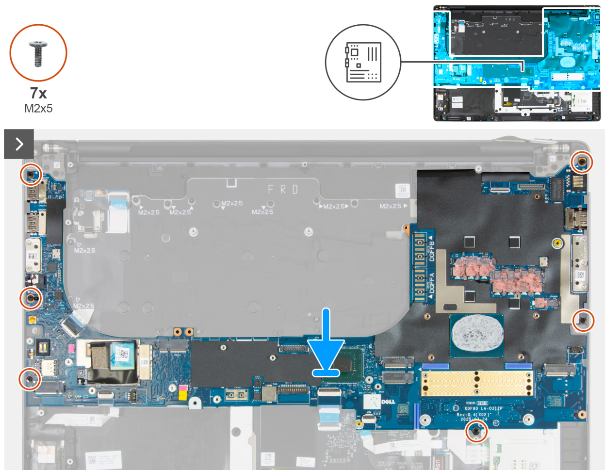
Figure 111. Installation de la carte système
