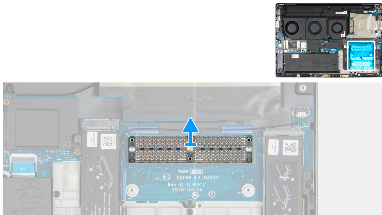
Figure 69. Retrait du connecteur de mémoire
