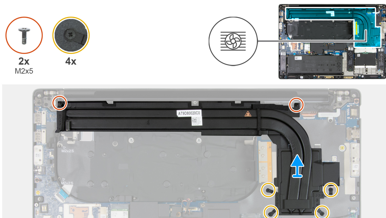
Figure 73. Retrait du dissipateur de chaleur pour les ordinateurs équipés d'une carte graphique intégrée
