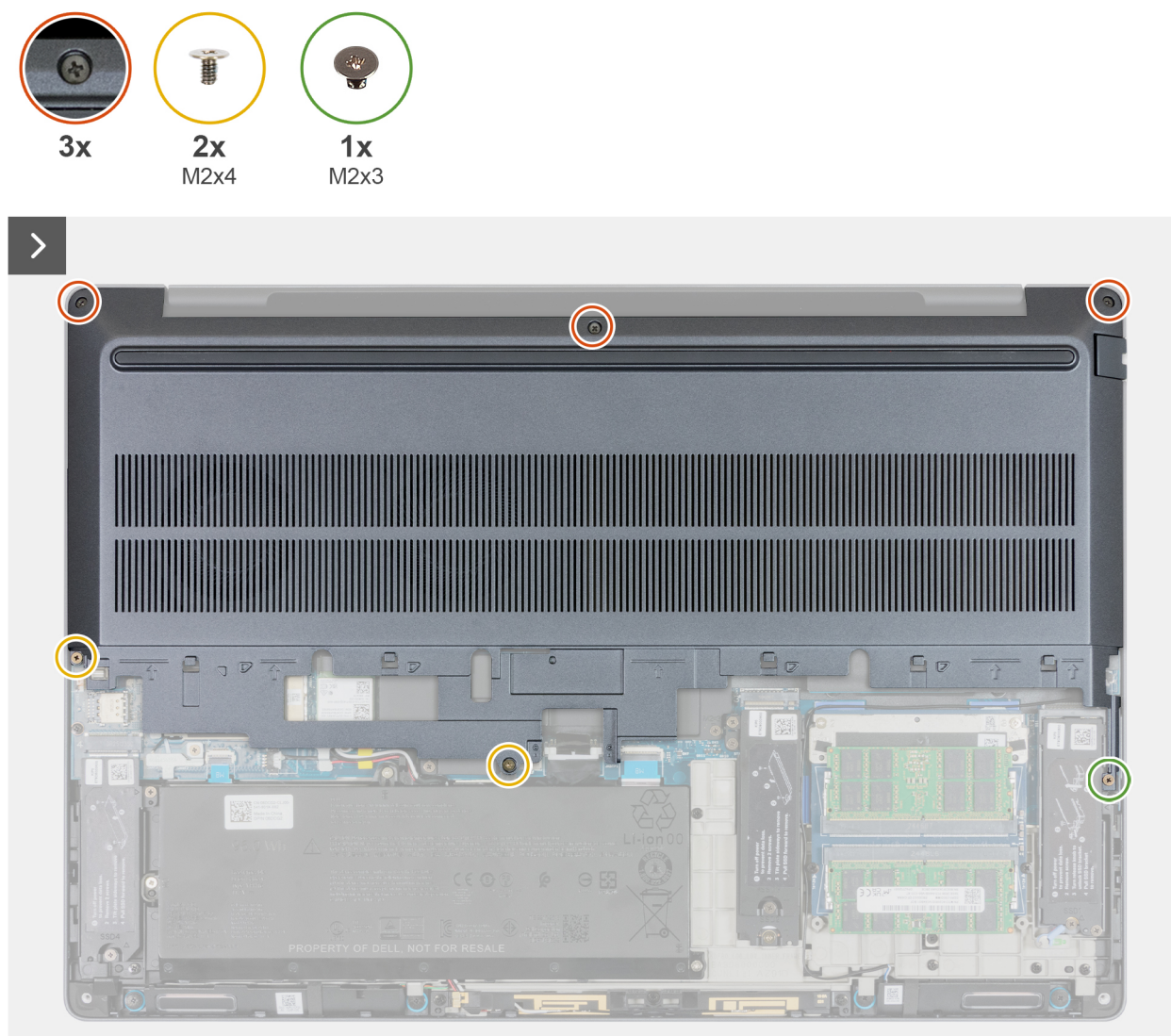
Figure 18. Desserrage des trois vis imperdables et retrait des trois vis
