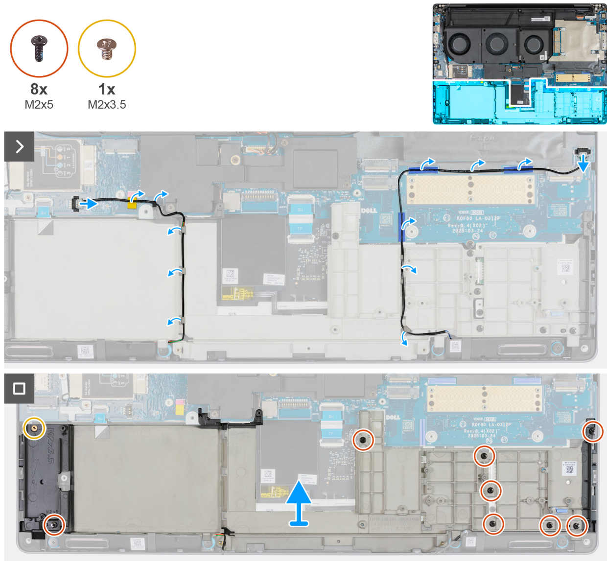
Figure 79. Retrait du cadre interne
