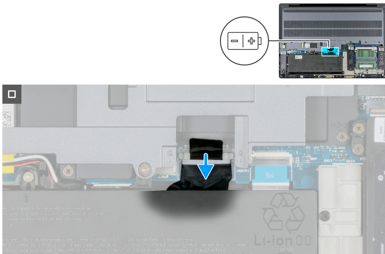
Figure 20. Déconnexion du câble de la batterie
