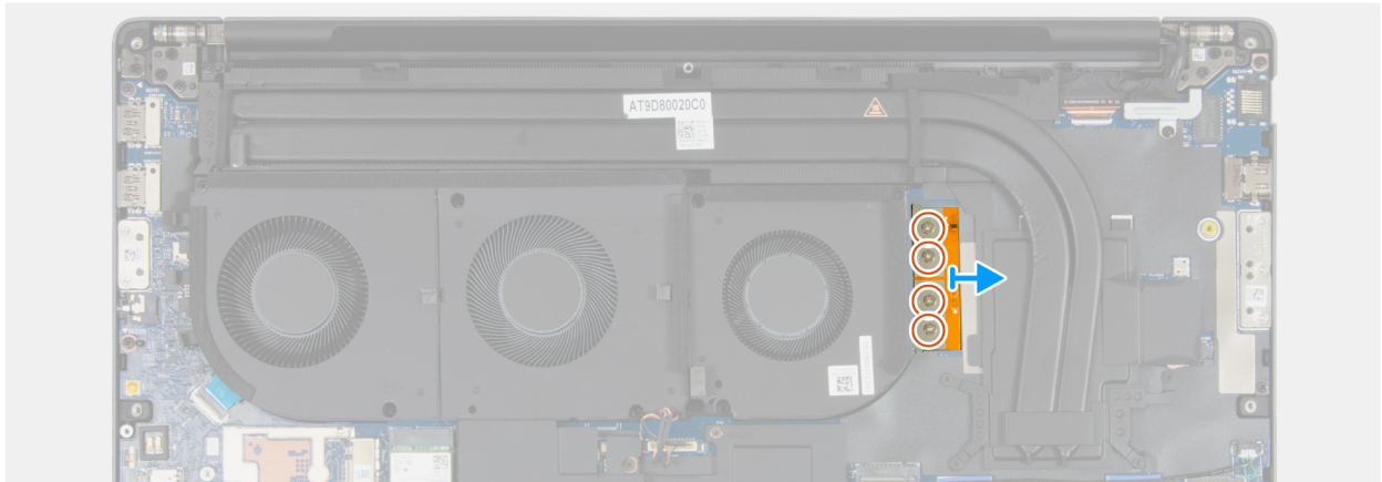
Figure 57. Retrait du connecteur de faisceau FPC intégré
