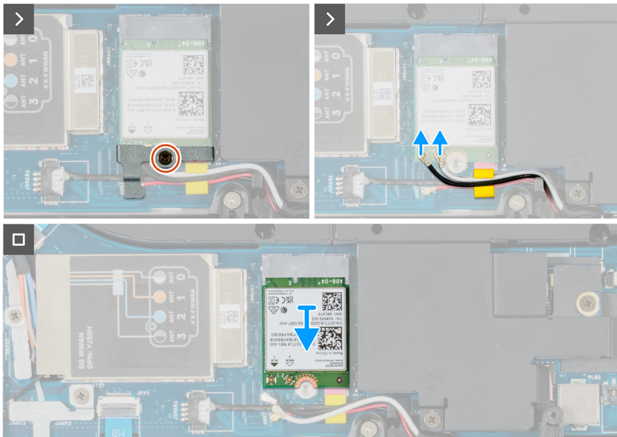
Figure 48. Retrait de la carte WLAN
