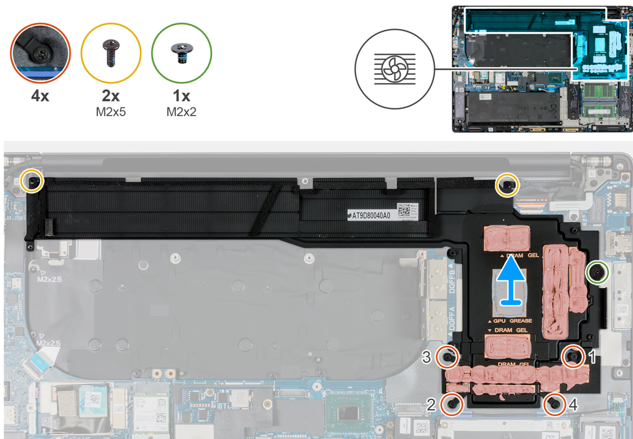
Figure 75. Retrait du dissipateur de chaleur pour les ordinateurs équipés d'une carte graphique séparée
