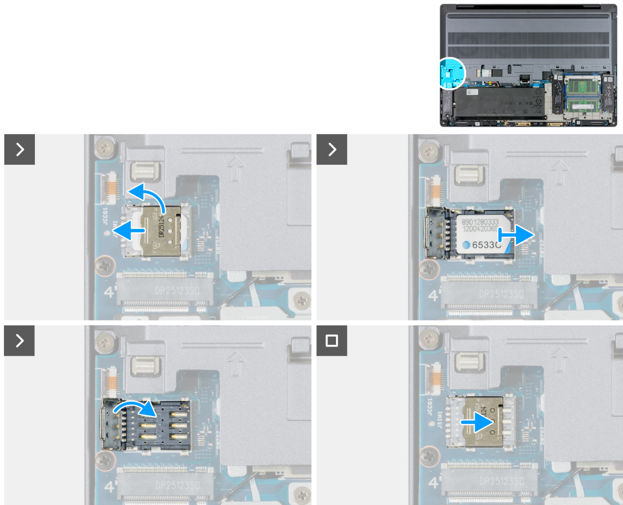
Figure 50. Retrait de la carte SIM
