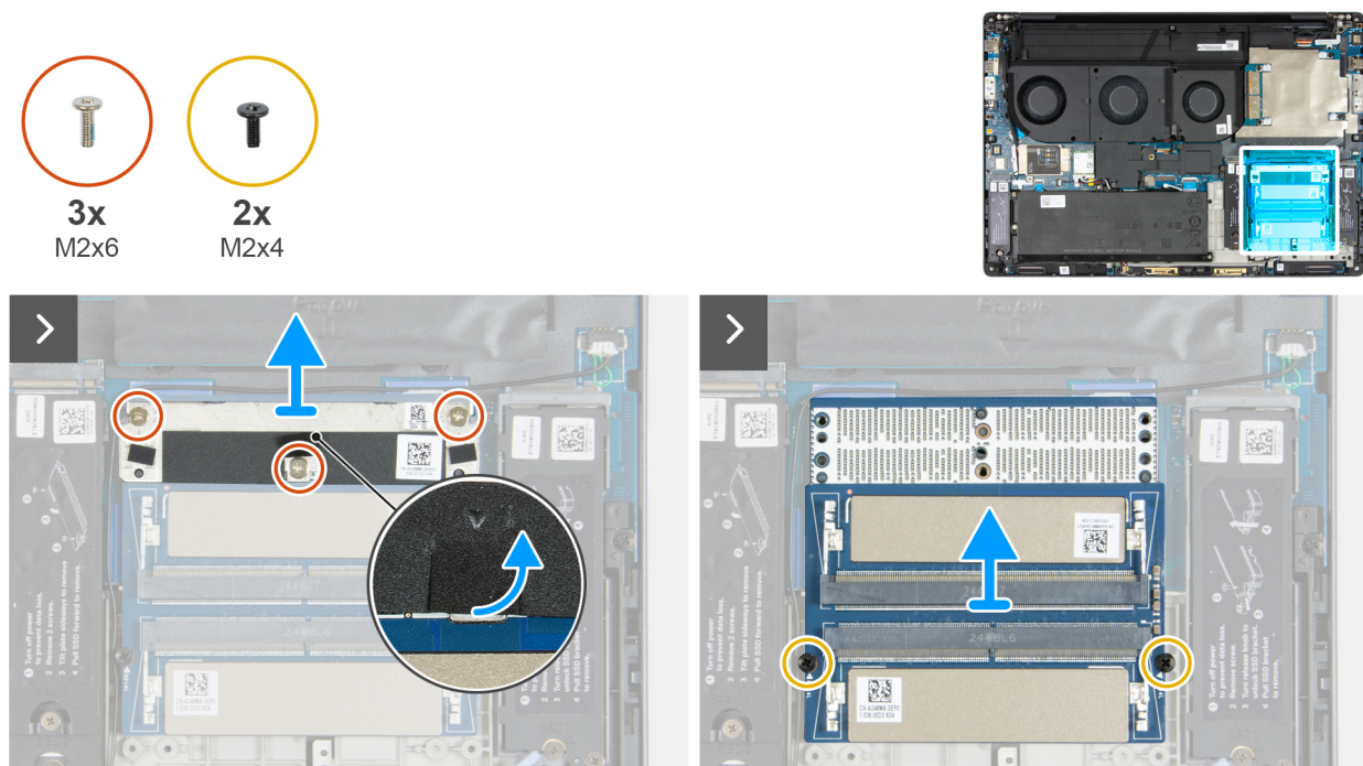
Figure 67. Retrait de la carte intercalaire de mémoire
