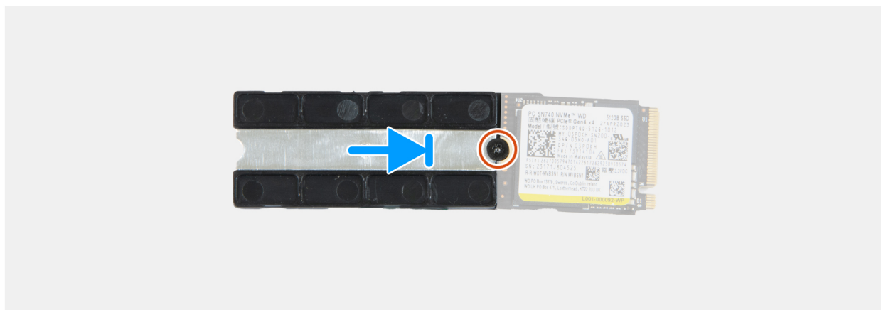
Figure 43. Installation du disque SSD M.2 2230
