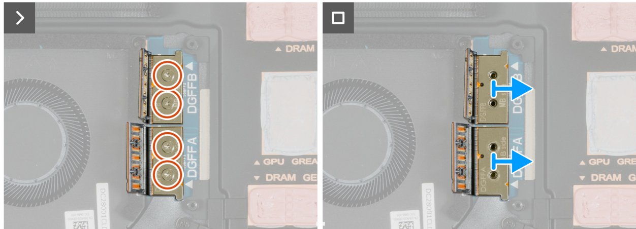
Figure 59. Retrait du connecteur de faisceau de circuit imprimé flexible séparé
