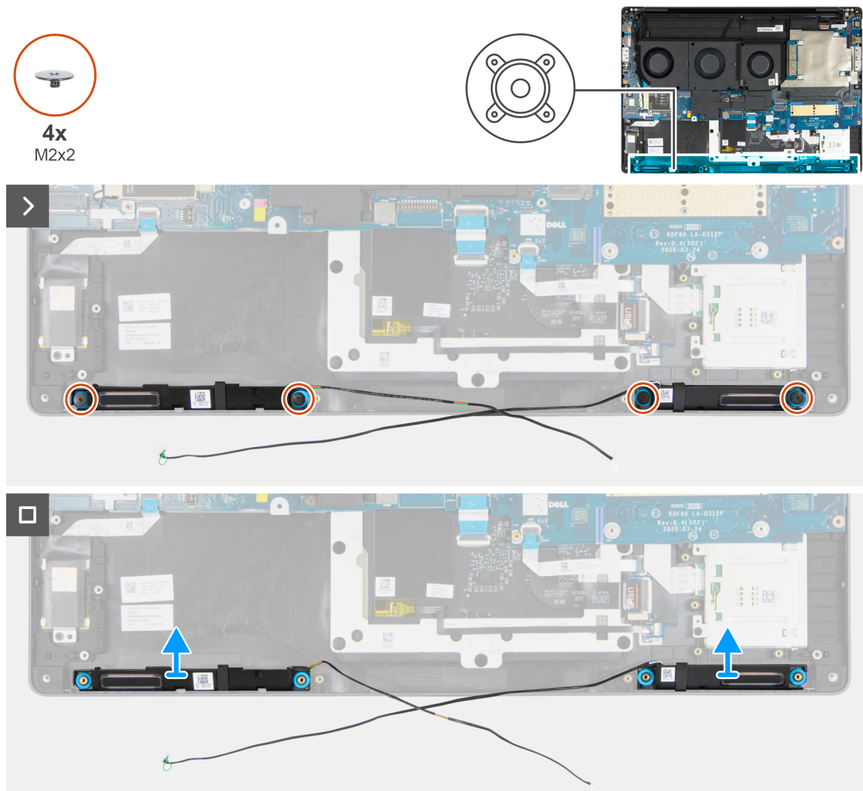
Figure 81. Retrait des haut-parleurs
