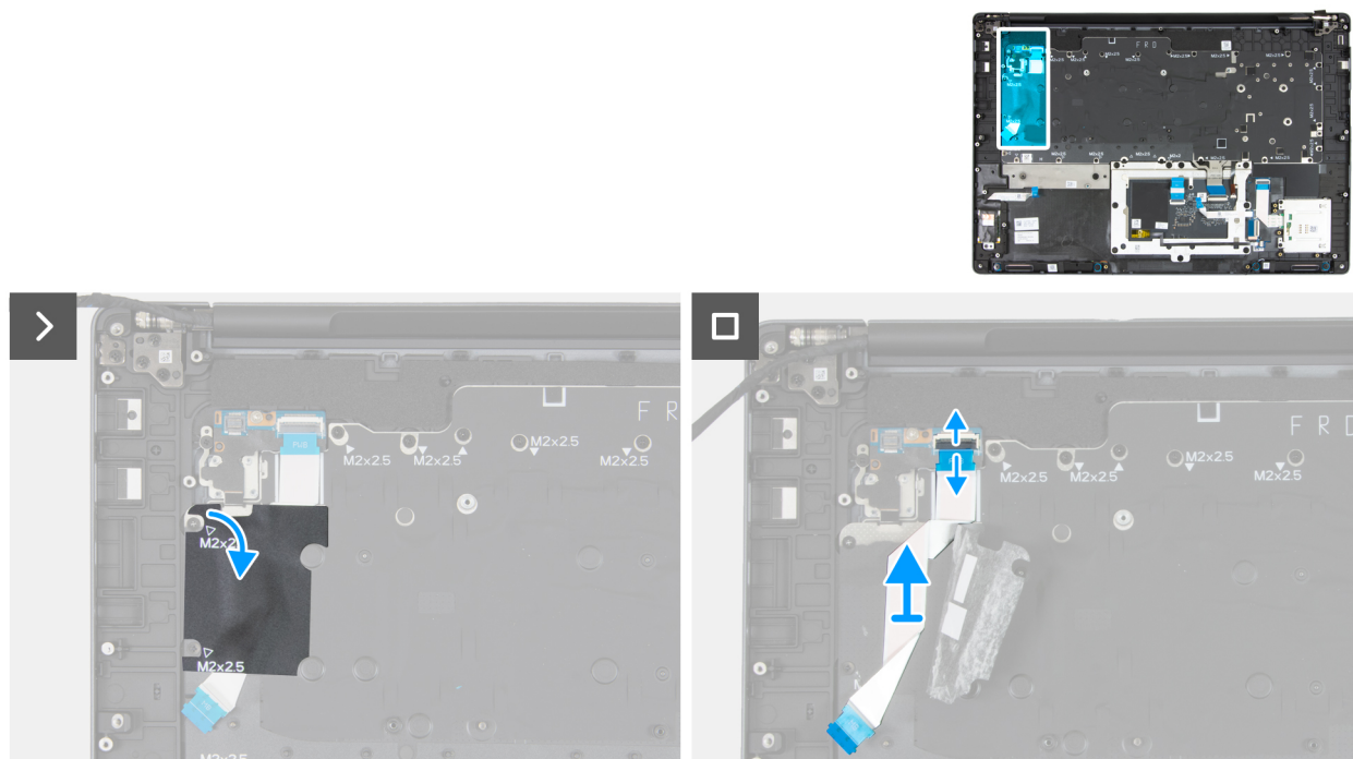
Figure 123. Retrait du câble de la carte du bouton d'alimentation
