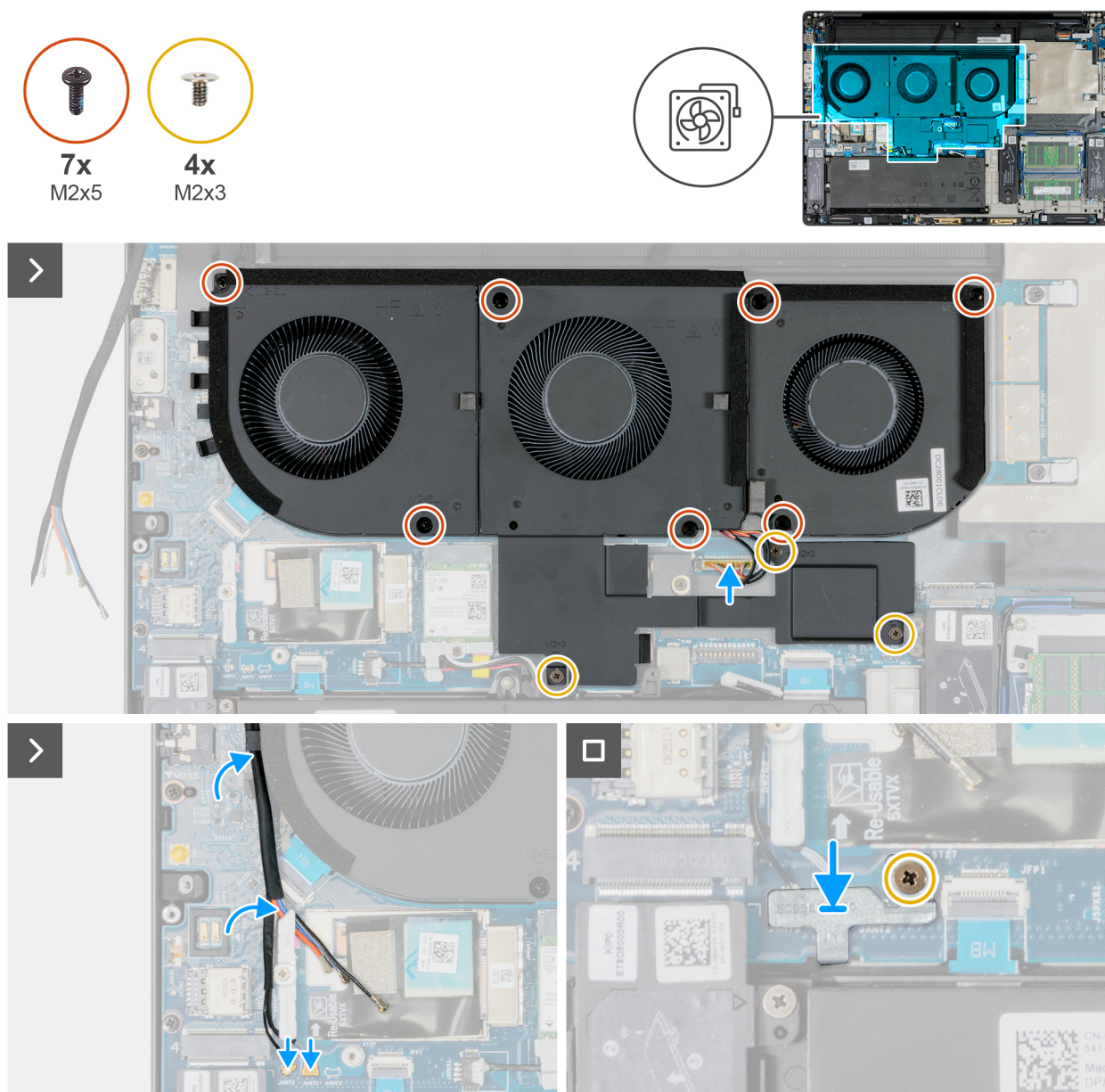
Figure 62. Installation de l'assemblage du ventilateur
