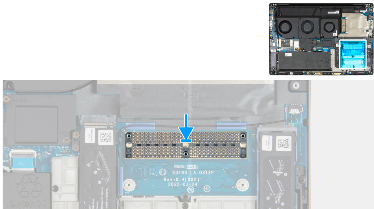
Figure 70. Installation du connecteur de mémoire
