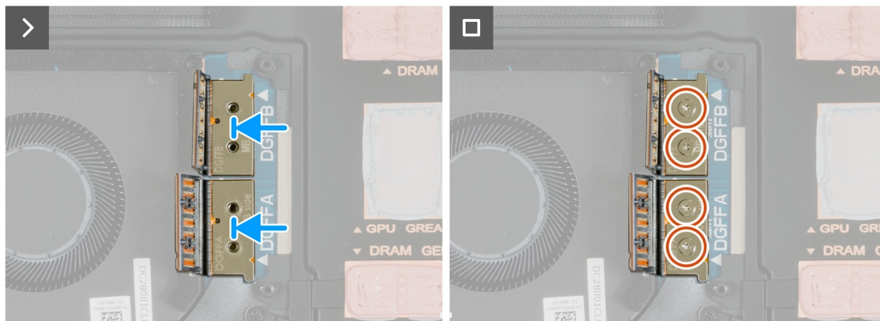
Figure 60. Installation du connecteur de faisceau FPC séparé
