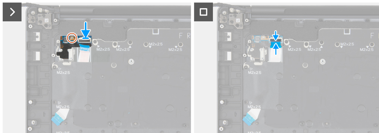
Figure 126. Installation de la carte du bouton d'alimentation
