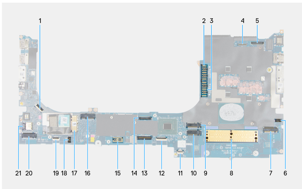
Figure 106. Connecteurs sur la carte système
