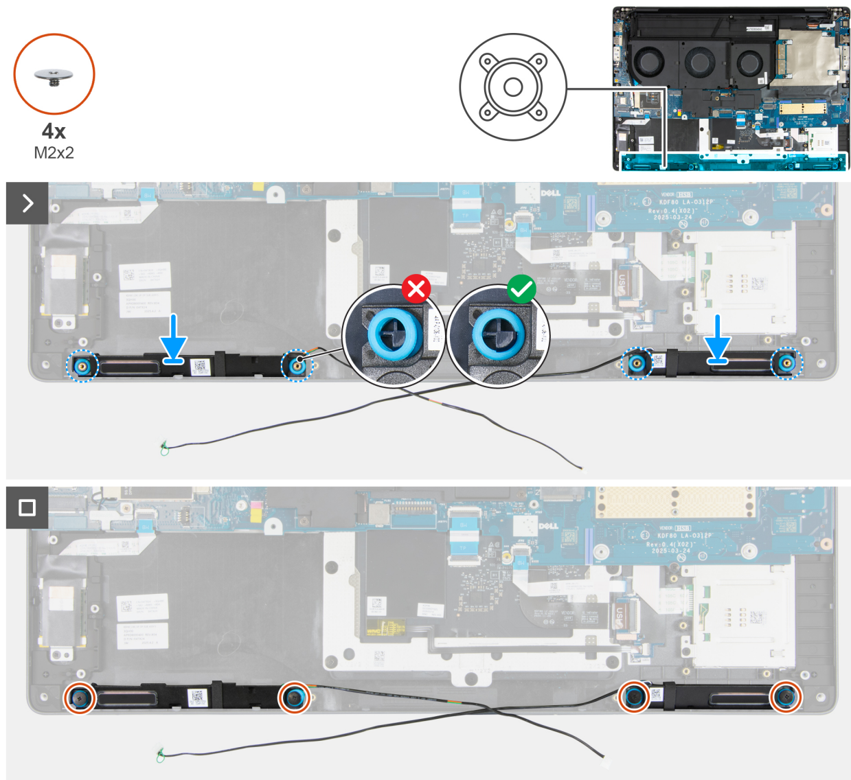
Figure 82. Installation des haut-parleurs
