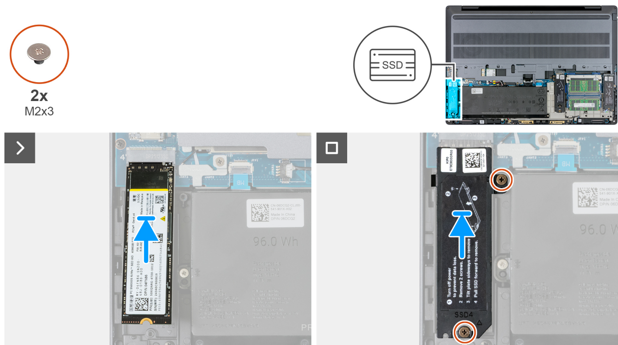
Figure 41. Installation du disque SSD M.2 2280 dans le logement 4 (SSD4)
