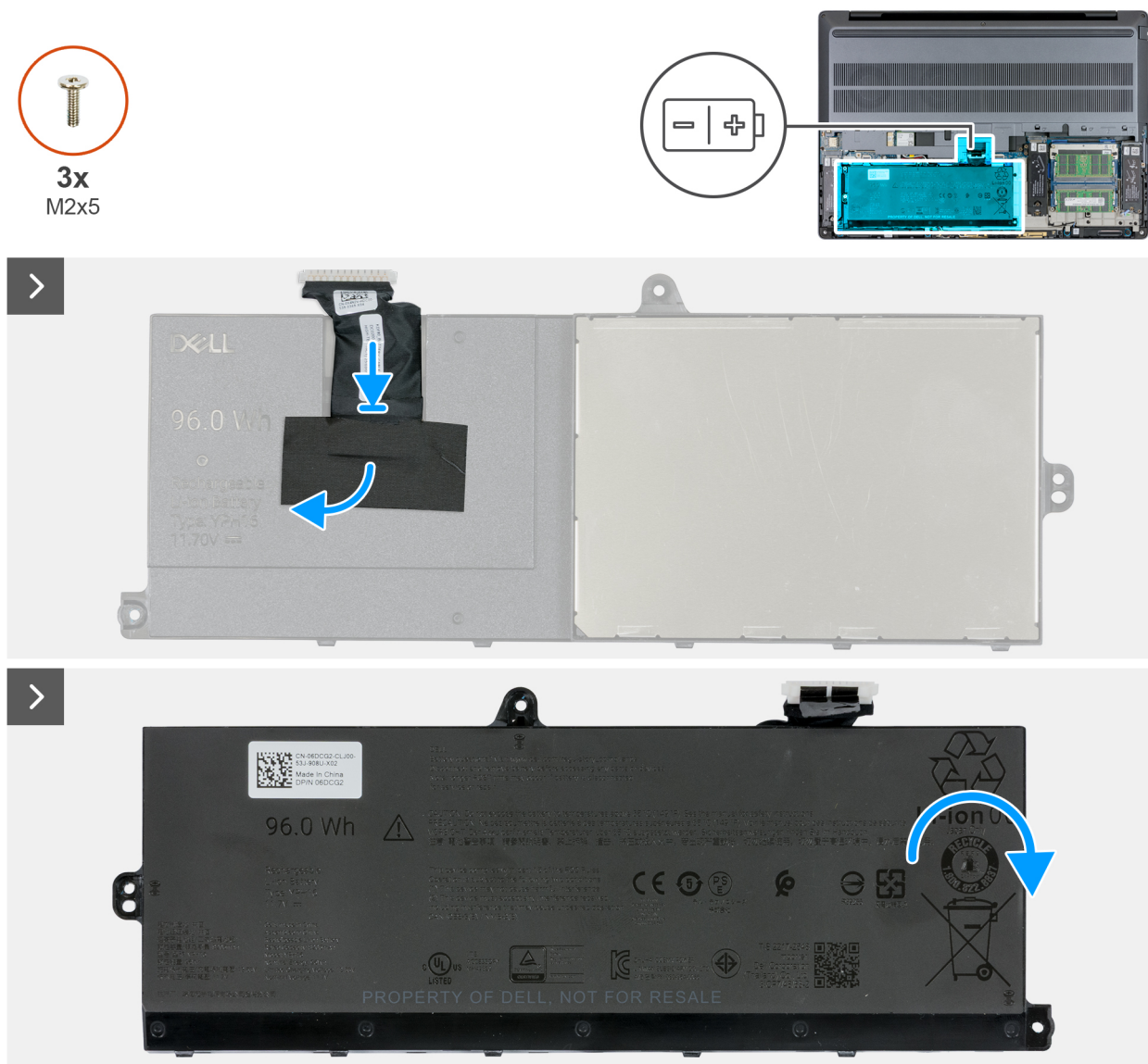
Figure 46. Remplacement du câble de la batterie
