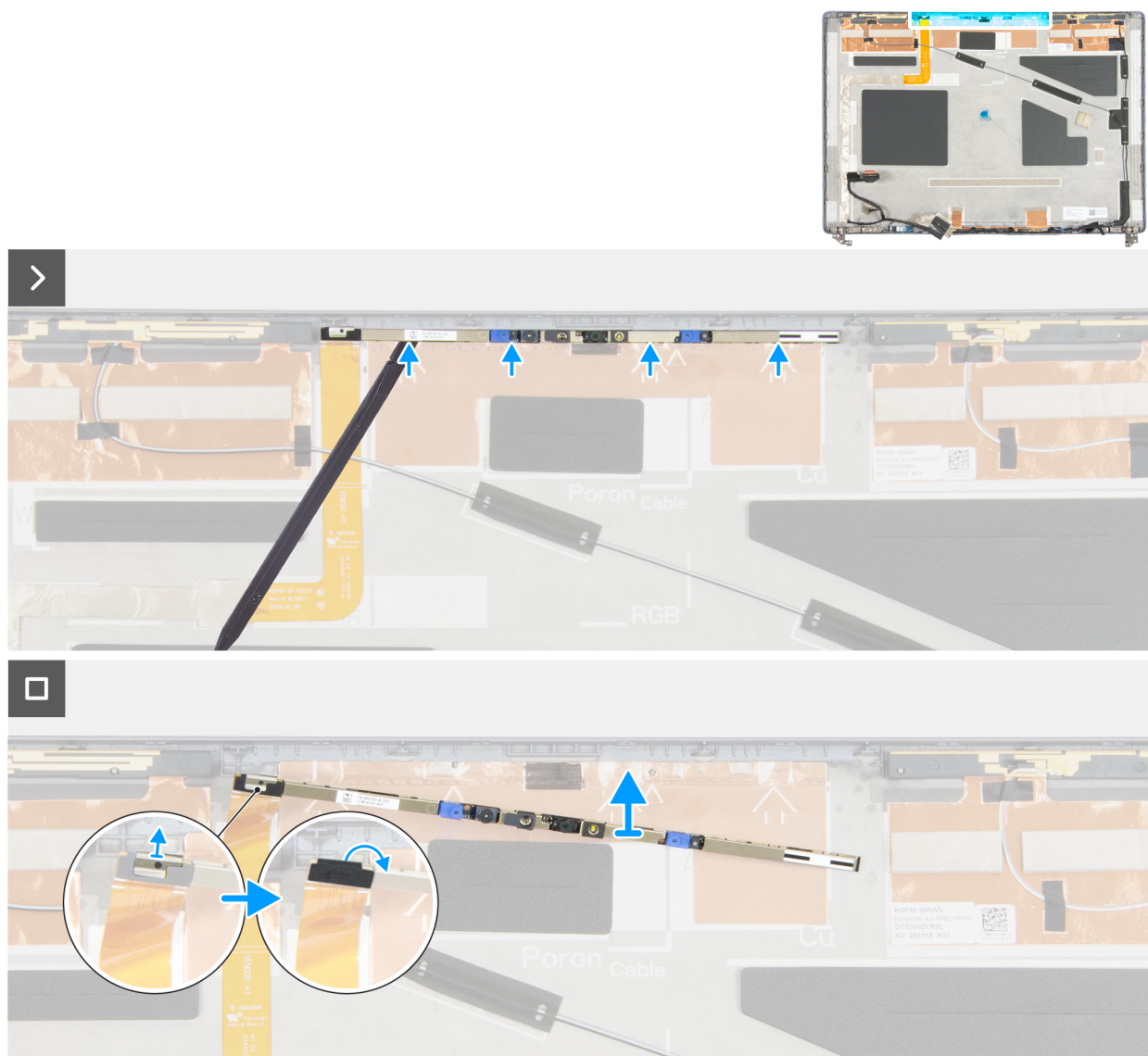
Figure 101. Retrait du module de caméra
