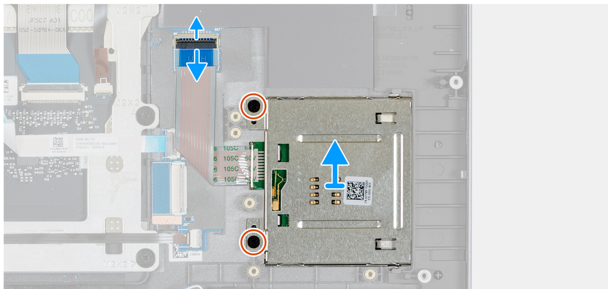
Figure 121. Retrait du lecteur de carte à puce
