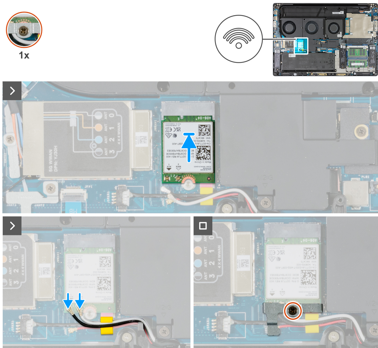
Figure 49. Installation de la carte WLAN
