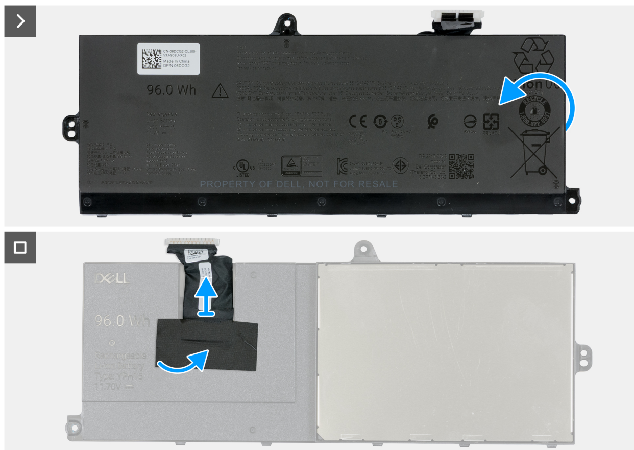
Figure 45. Retrait du câble de la batterie de la batterie
