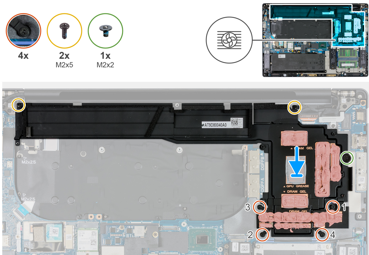
Figure 76. Installation du dissipateur de chaleur pour les ordinateurs expédiés avec une carte graphique séparée
