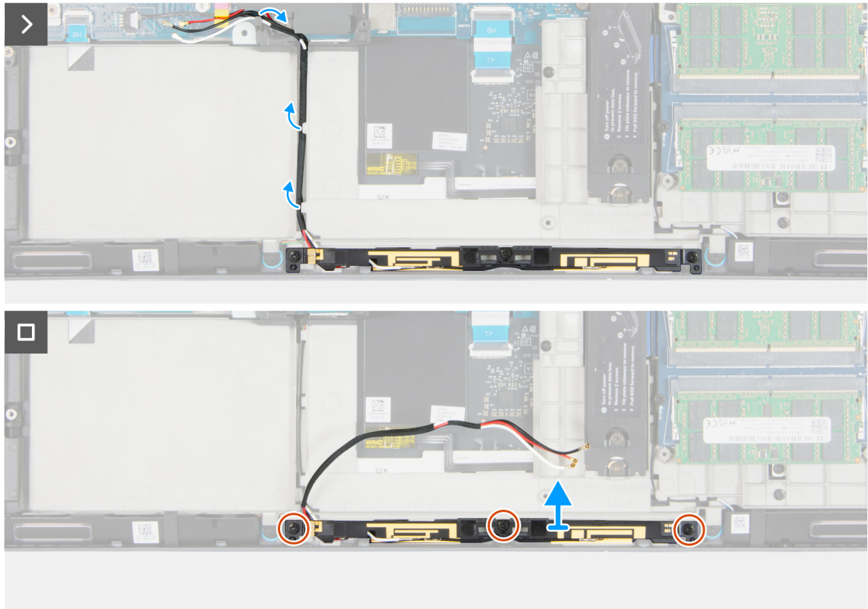
Figure 77. Retrait du module d'antenne WLAN
