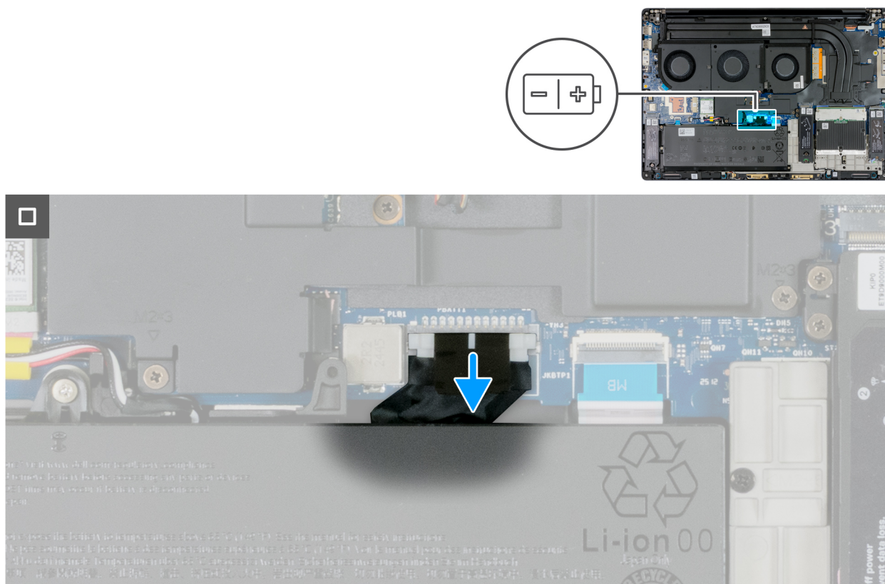
Figure 26. Déconnexion du câble de la batterie
