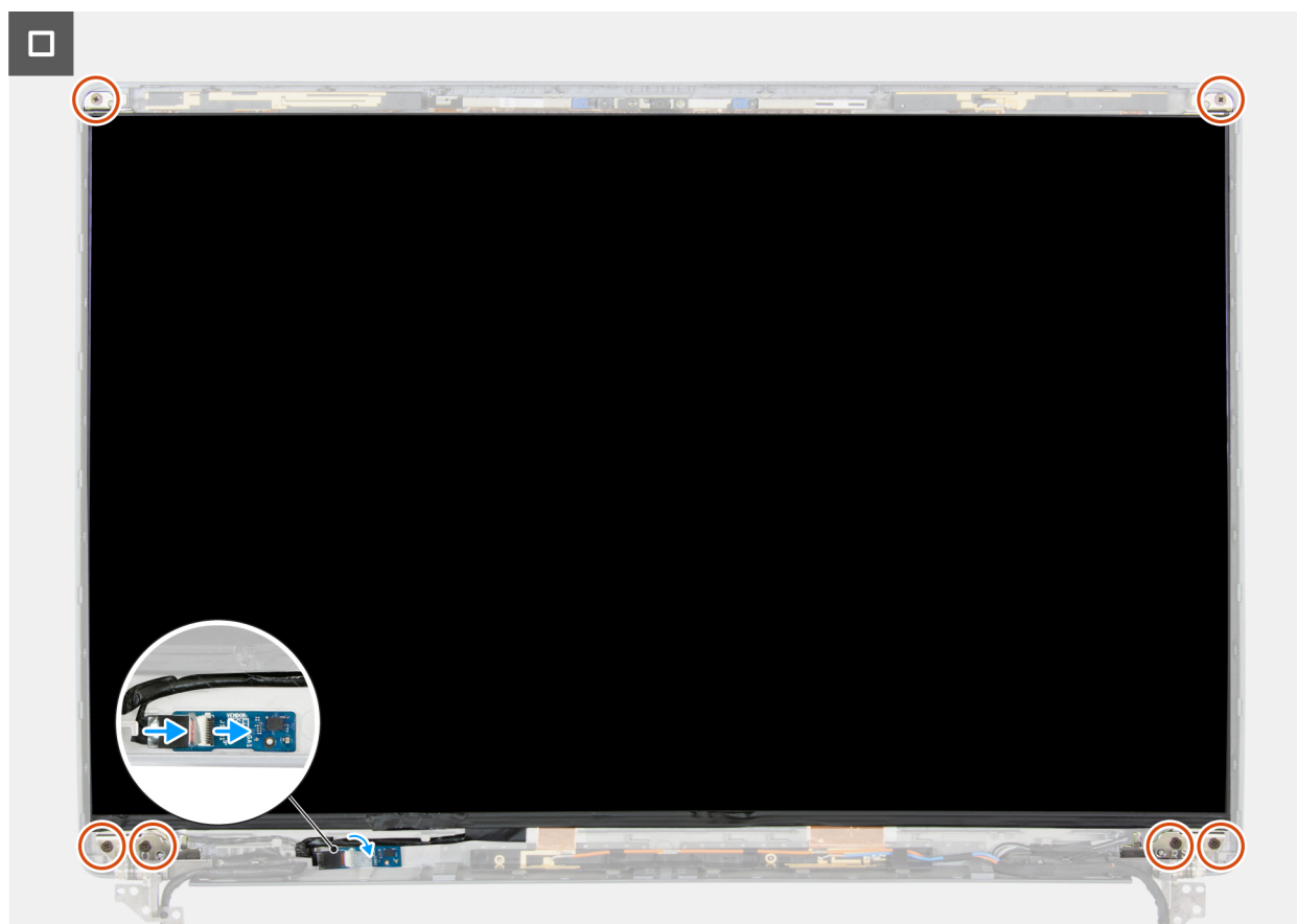
Figure 98. Installation du panneau d'écran
