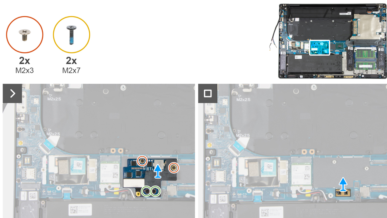
Figure 71. Retrait de la carte d'alimentation
