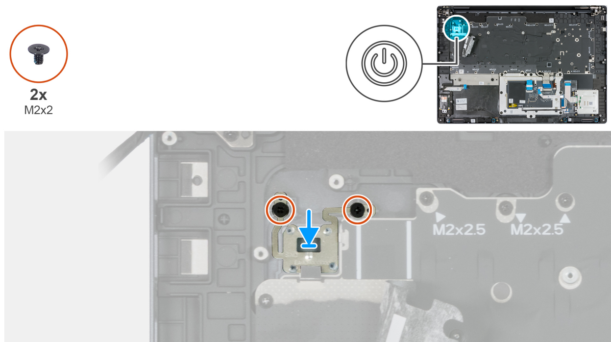
Figure 128. Installation du bouton d'alimentation
