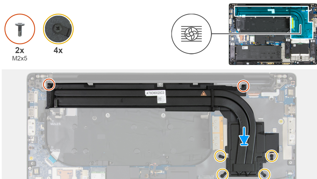
Figure 74. Installation du dissipateur de chaleur pour les ordinateurs équipés d'une carte graphique intégrée
