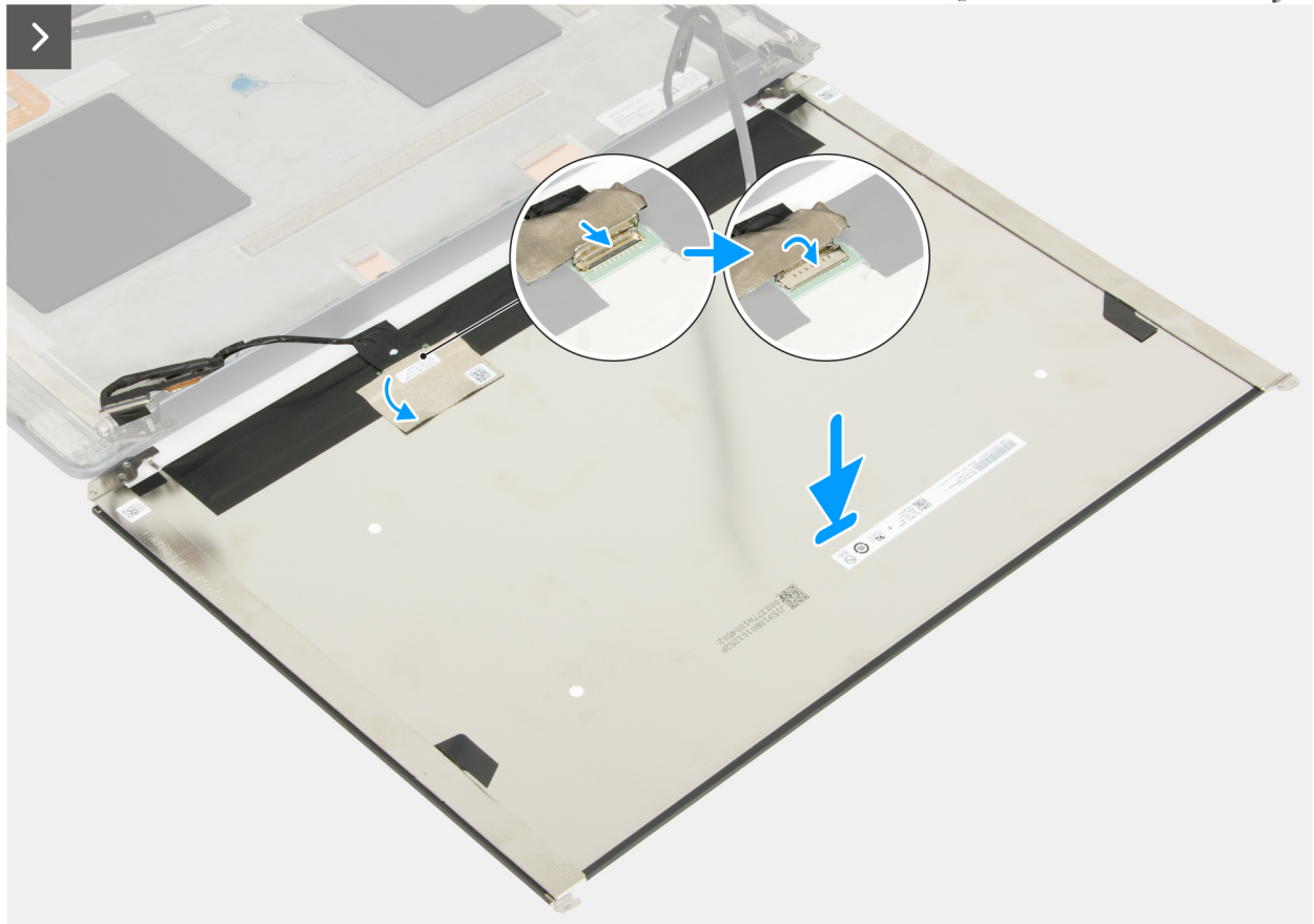
Figure 97. Installation du panneau d'écran
