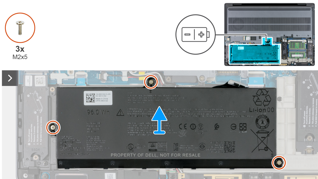
Figure 44. Retrait de la batterie
