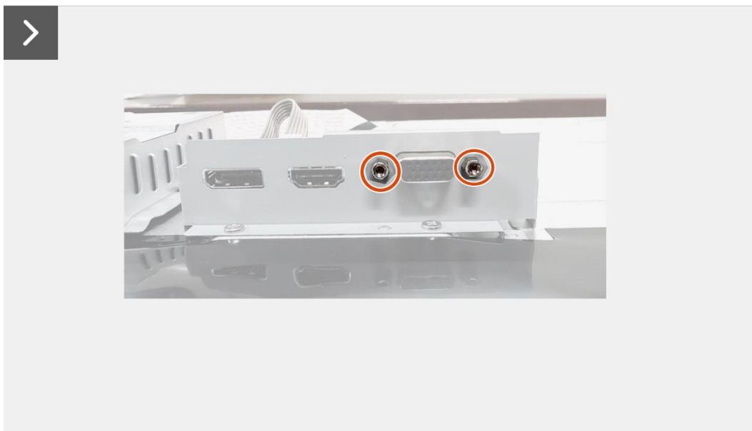
Rysunek 28. Wyjmowanie płytki interfejsu
