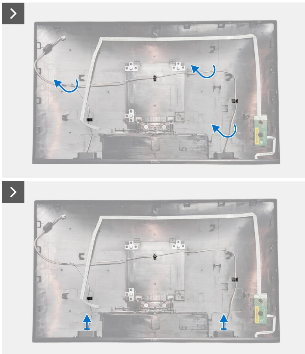
Rysunek 16. Zdejmowanie głośnika
