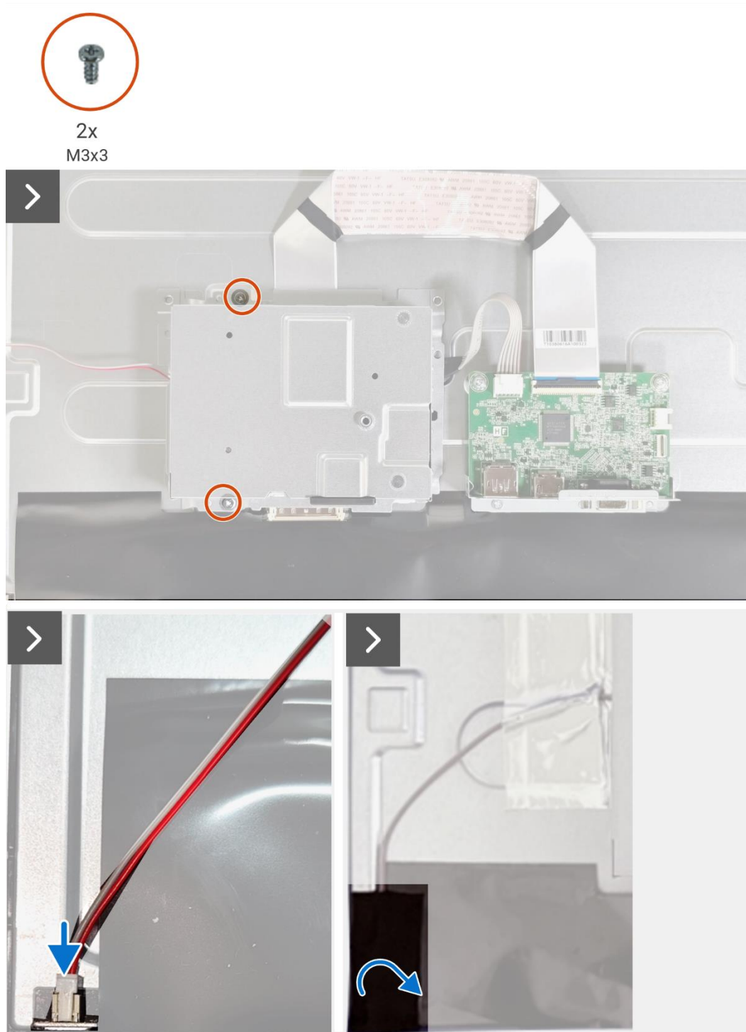
Rysunek 25. Instalacja zespołu obudowy
