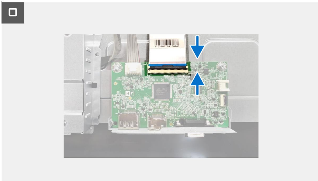
Rysunek 32. Instalacja płytki interfejsu
