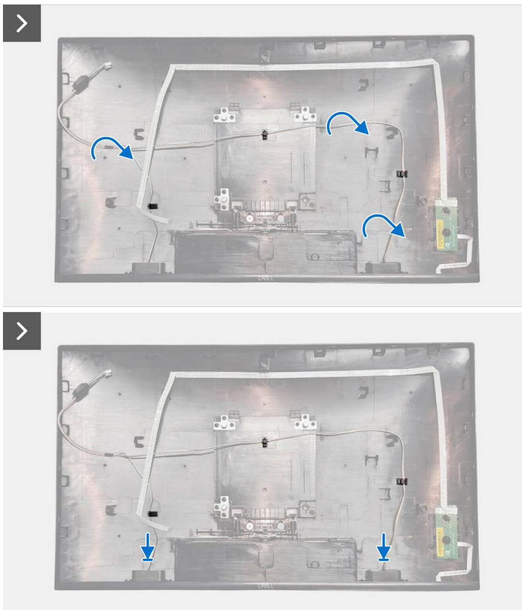
Rysunek 18. Instalacja głośnika
