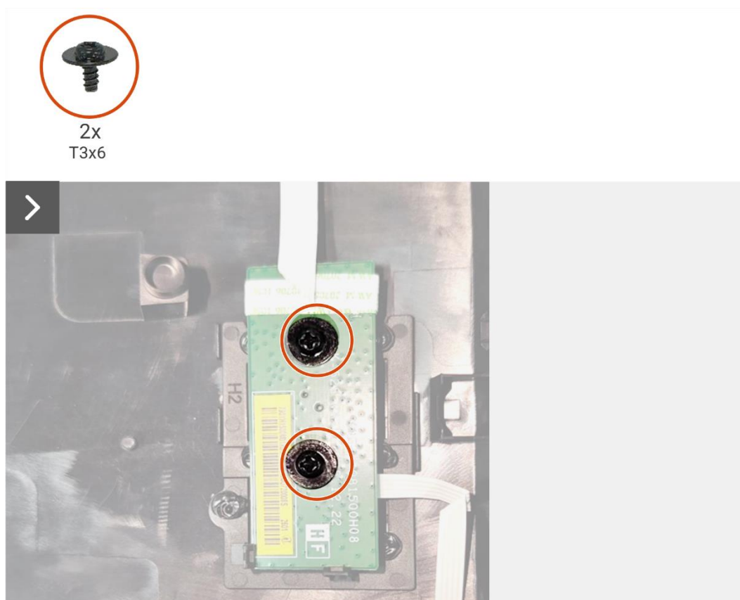
Rysunek 9. Wyjmowanie płytki bloku przycisków
