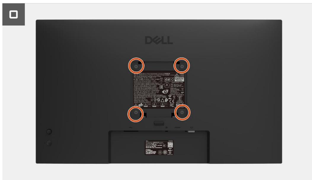
Rysunek 8. Instalacja tylnej pokrywy
