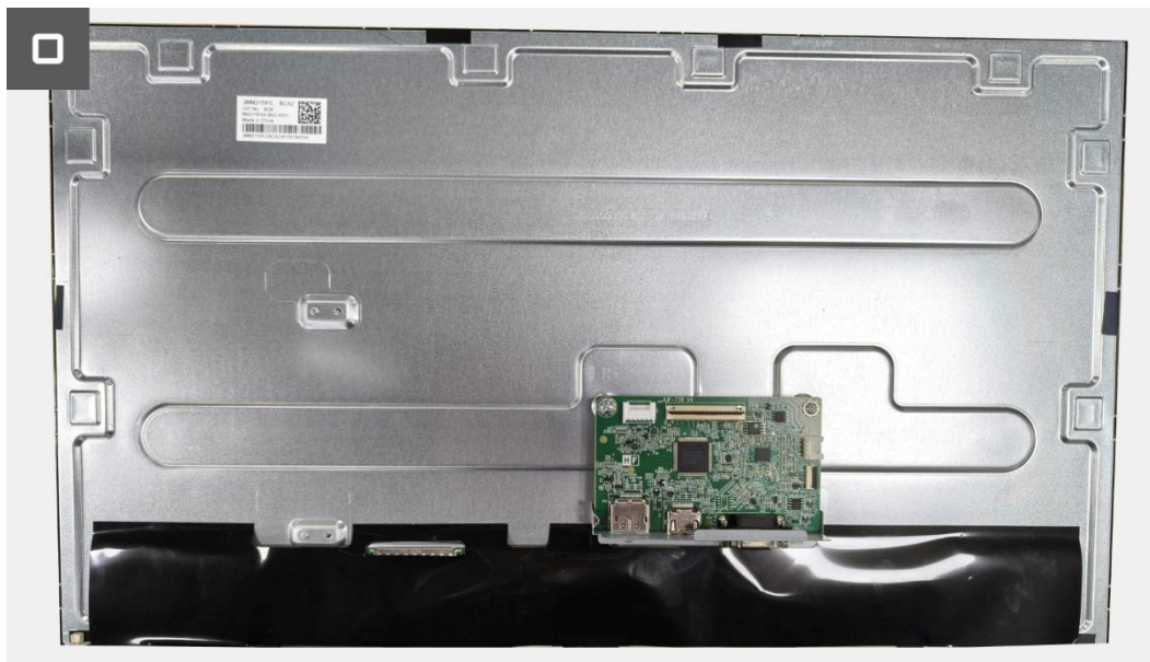
Rysunek 23. Zdejmowanie zespołu obudowy
