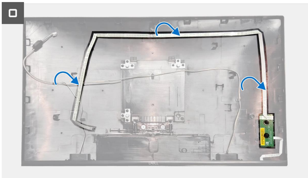
Rysunek 12. Instalacja płytki bloku przycisków
