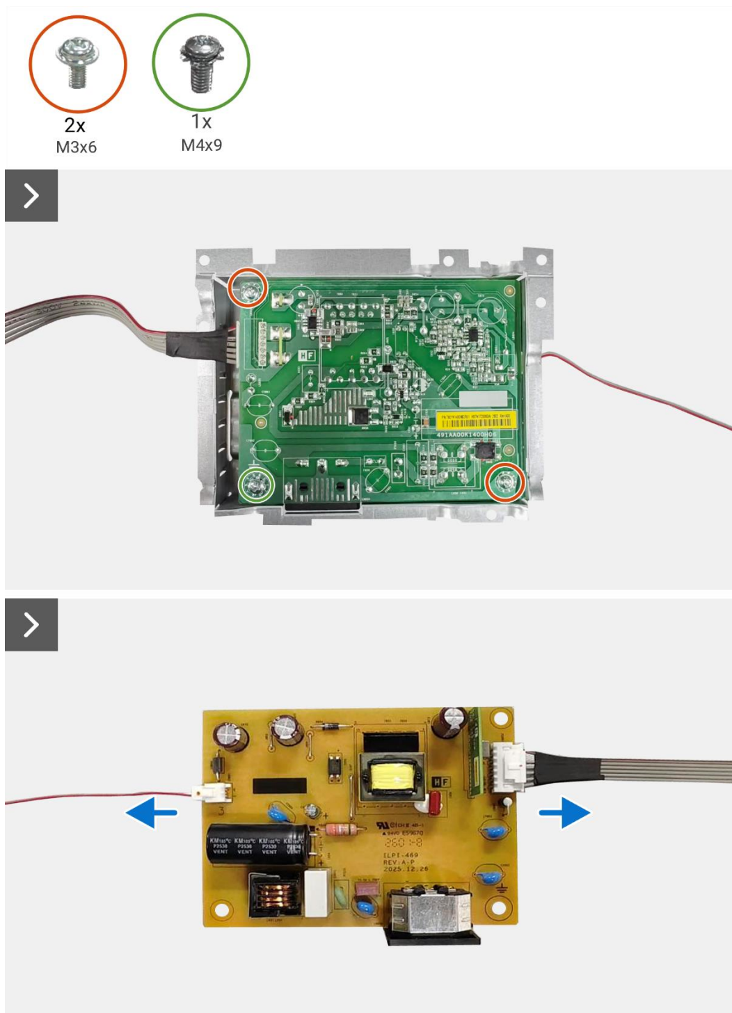
Rysunek 34. Wyjmowanie płytki zasilającej
