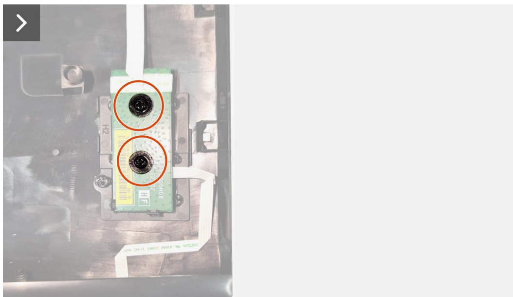
Rysunek 11. Instalacja płytki bloku przycisków
