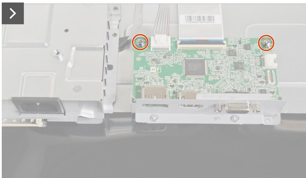
Rysunek 31. Instalacja płytki interfejsu
