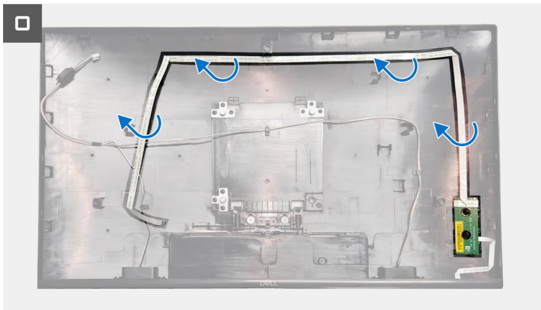
Rysunek 10. Wyjmowanie płytki bloku przycisków
