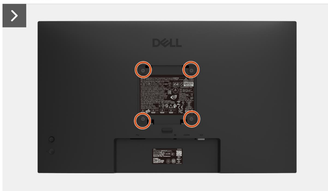
Rysunek 5. Zdejmowanie tylnej pokrywy
