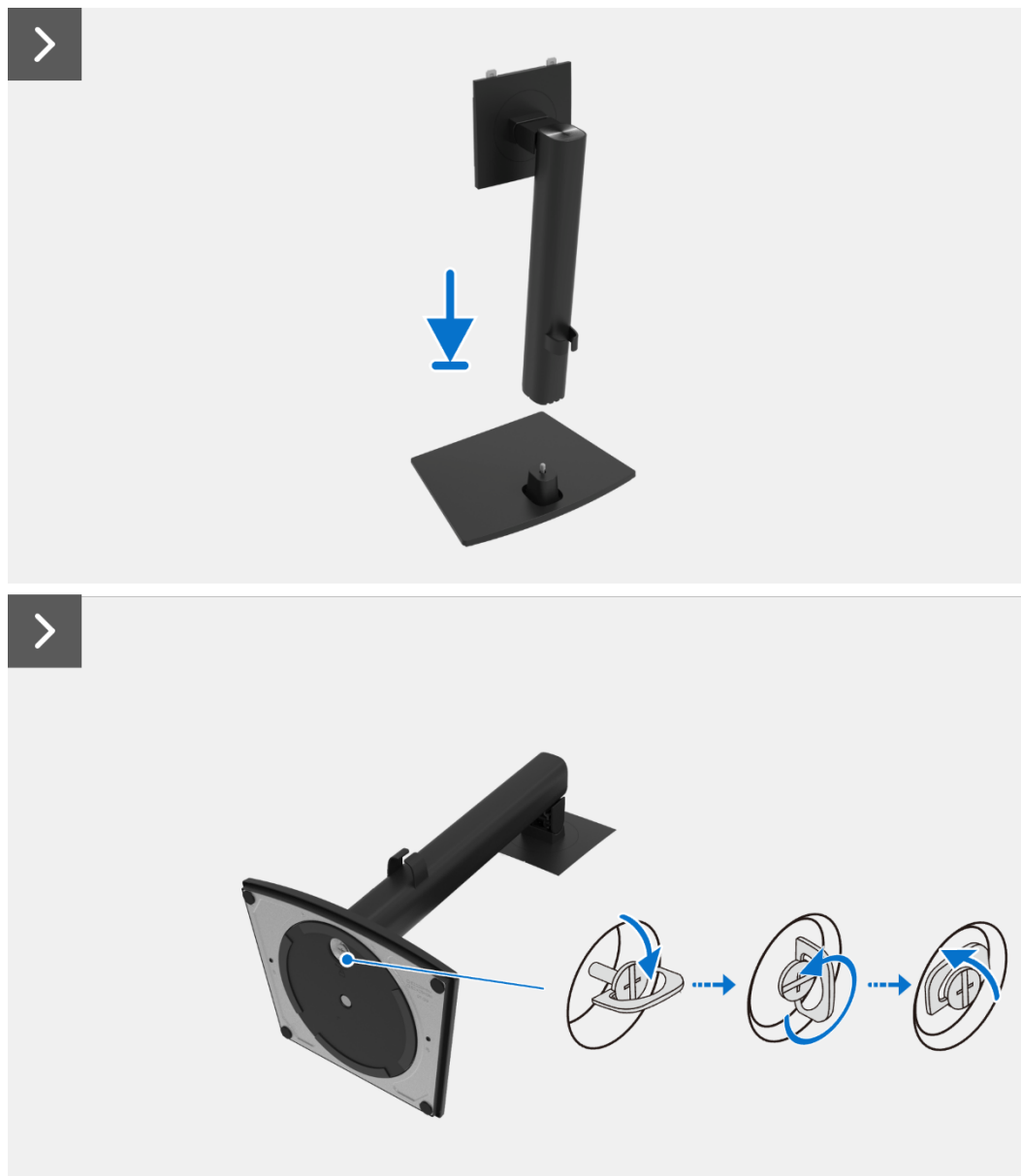
Rysunek 3. Instalacja podstawy
