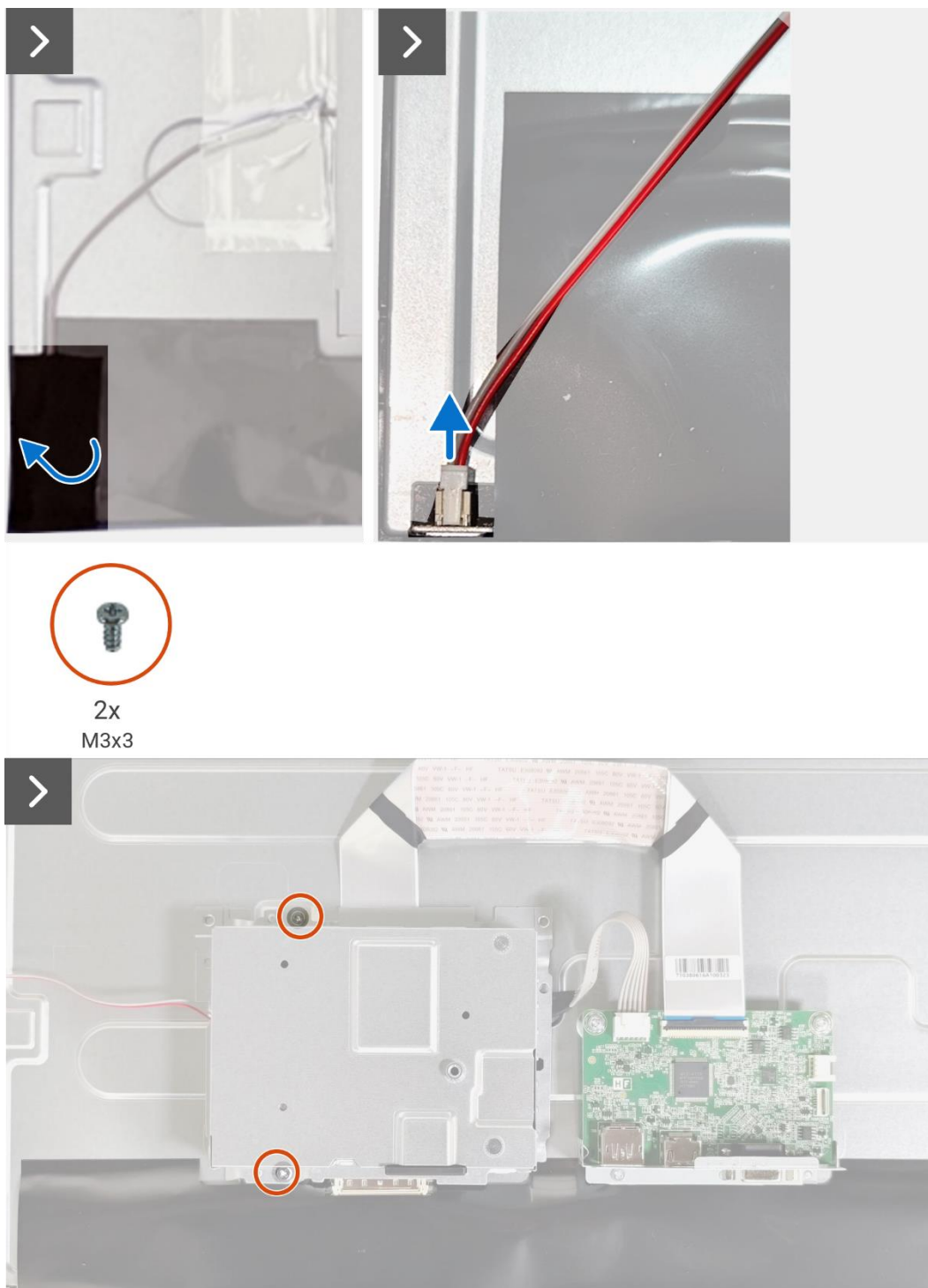
Rysunek 21. Zdejmowanie zespołu obudowy
