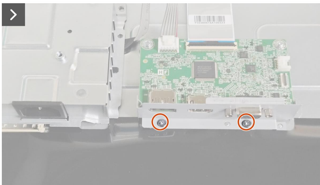
Rysunek 30. Instalacja płytki interfejsu
