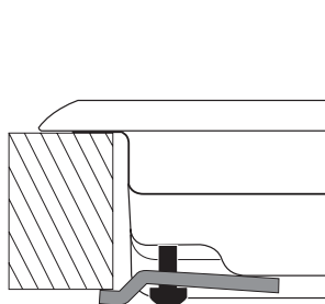
Stand haak voor keukenblad H=40mm
