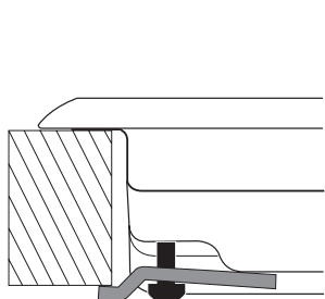
Монтаж крюка для опорных брусков H=40\text{mm}
