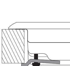
Posición del gancho para superficies H=40mm
