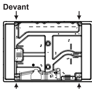
Position du crochet pour top H=30mm
