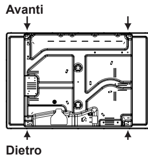
Posizione gancio per top H=30mm
