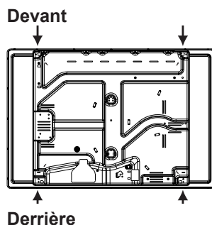
Position du crochet pour top H=30mm
