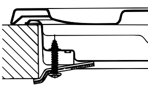
Stand haak voor keukenblad H=40mm
