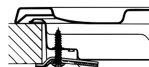
Posizione gancio per top H=30\text{mm}
