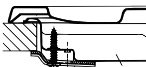
Posizione gancio per top H=20\text{mm}
