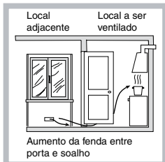
Exemplos de abertura de ventilação para ar comburente
