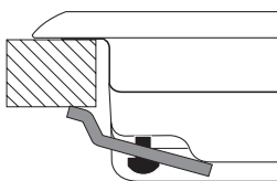
Posição do gancho para H=20mm
