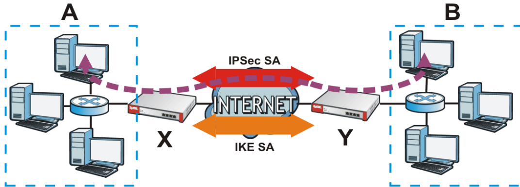
Figure 260 VPN: IKE SA and IPsec SA
