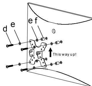
Per TV con retro curvo For curved back TV
