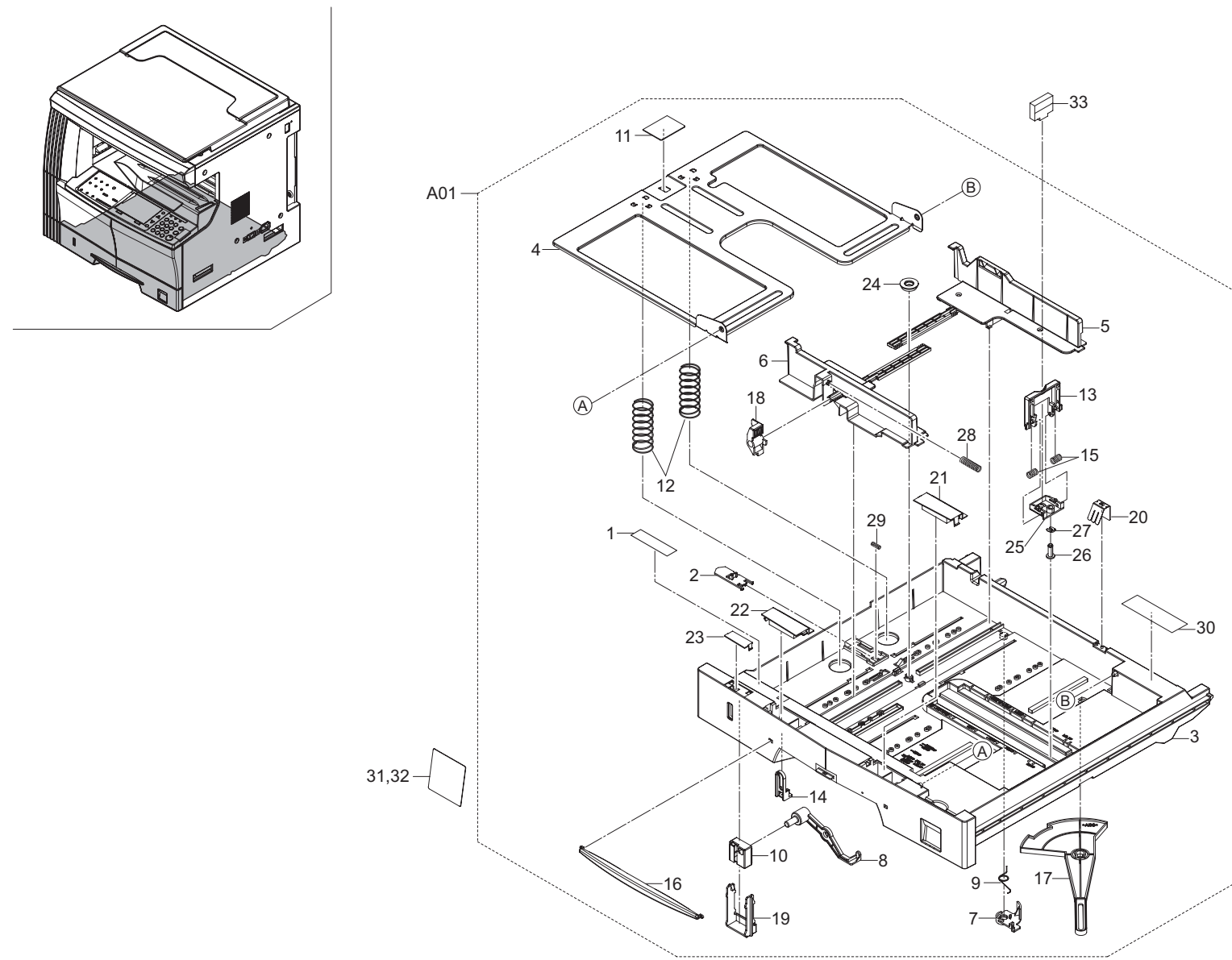
FIG. 3 Cassette
